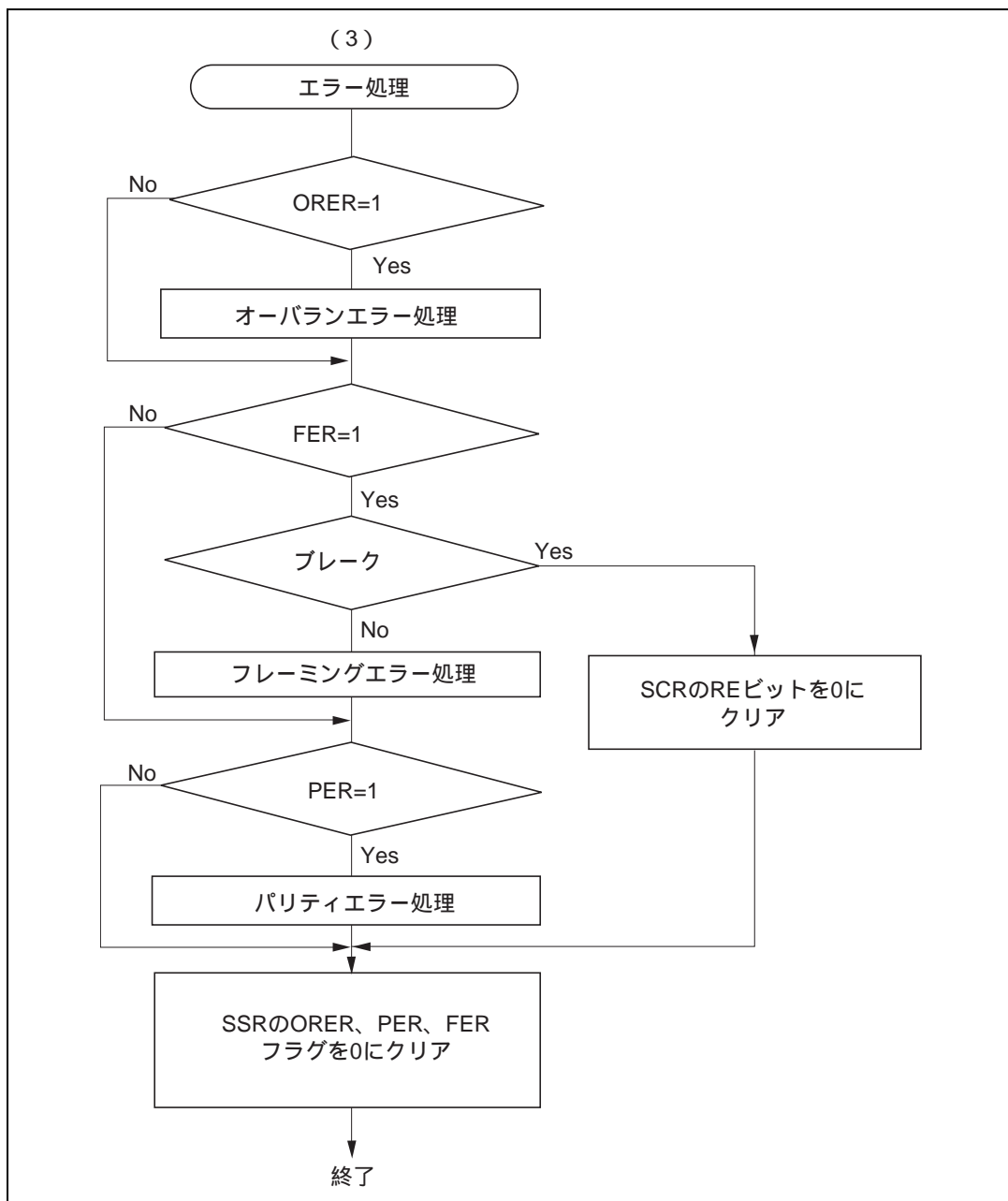
図 13.7 シリアル受信データフローチャートの例(2)
