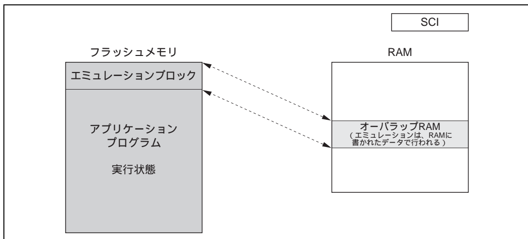
図 18.3 ユーザモード、ユーザプログラムモードのオーバーラップ RAM データの読み出し
