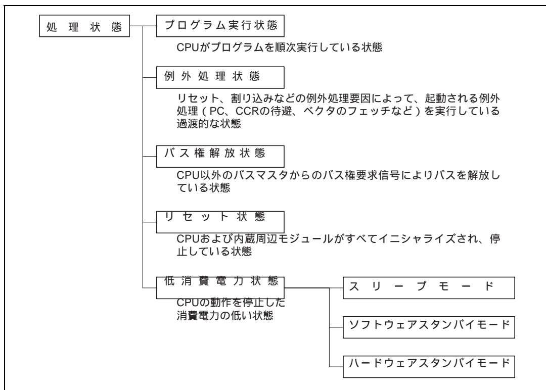
図 2.11 処理状態の分類
