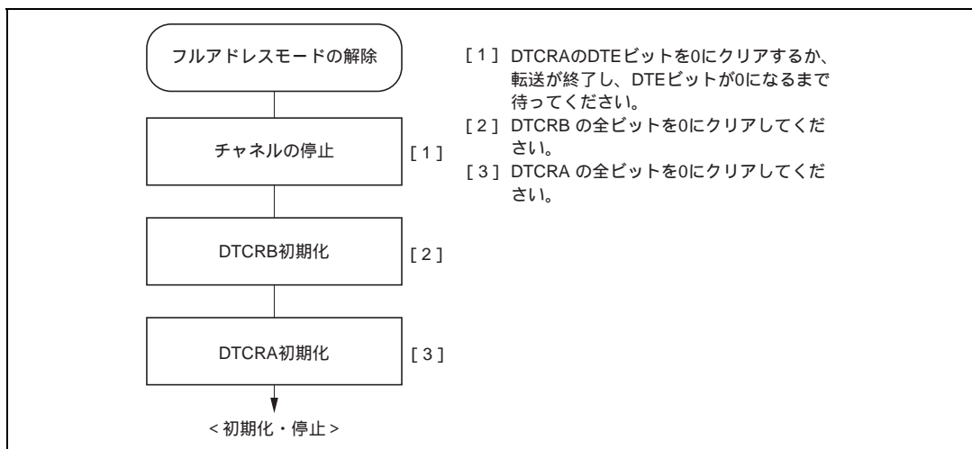
図 7.23 フルアドレスモードの解除手順例
