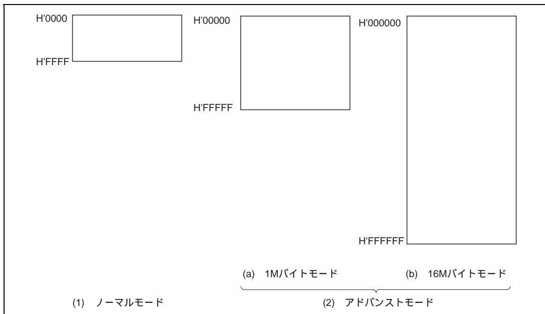
図 2.2 メモリマップ
