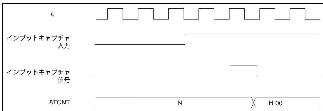
図 10.12 インพุットキャプチャによるクリアタイミング
