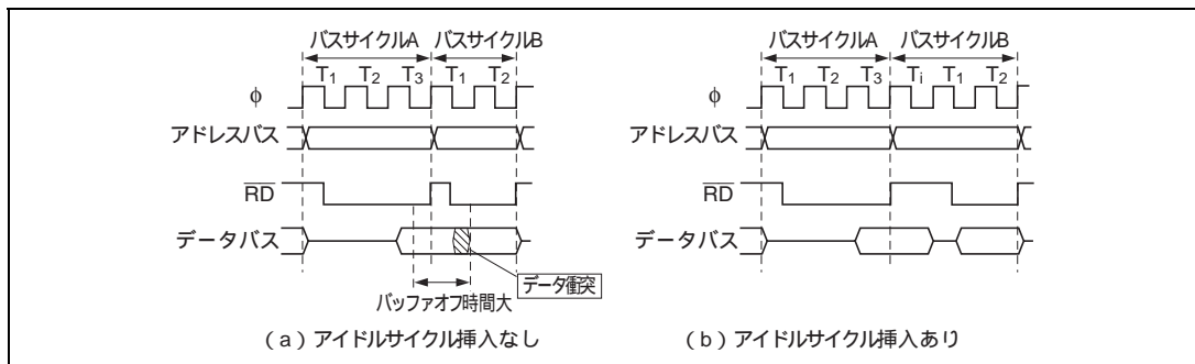
図 6.43 アイドルサイクル動作例 (1) (ICIS1=1 のとき)
