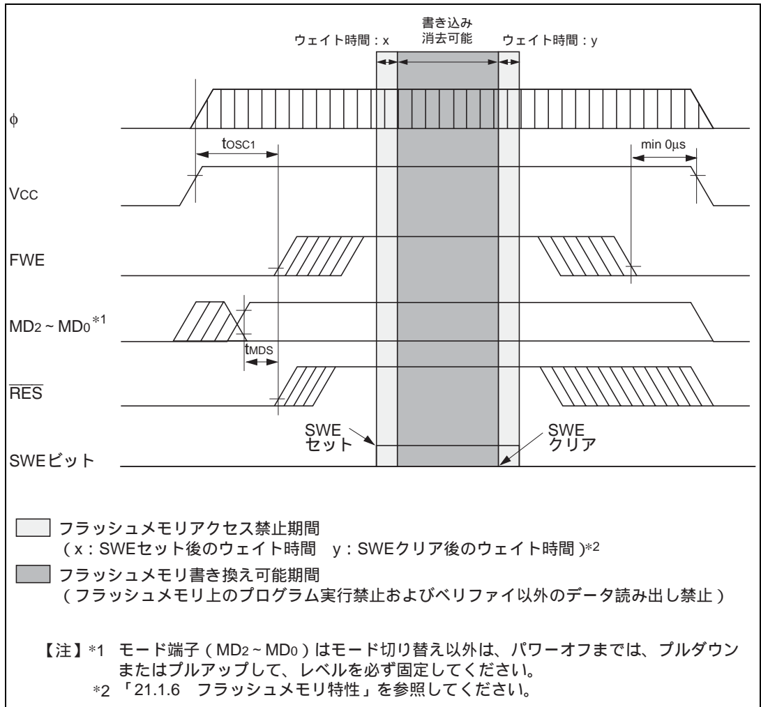
図 18.17 電源投入/切断タイミング (ユーザプログラムモード)
