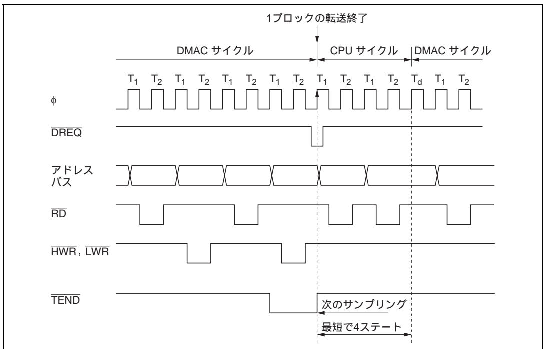
図 7.18 ブロック転送モード時の \overline{\text{DREQ}} 端子の立ち下がりエッジによる DMAC 起動タイミング
