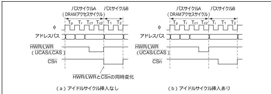
図 6.45 アイドルサイクル動作例 (3) (UCAS/LCAS として HWR/LWR を使用した場合)
