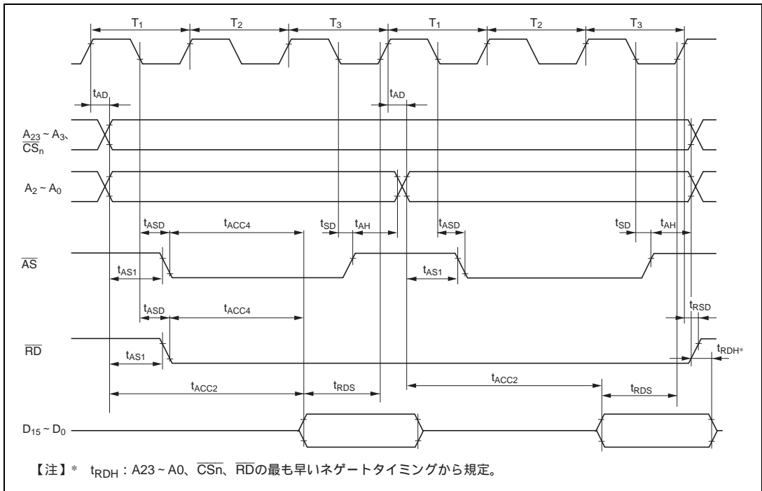
図 21.12 パースト ROM アクセスタイミング (パーストサイクル3ステート)
