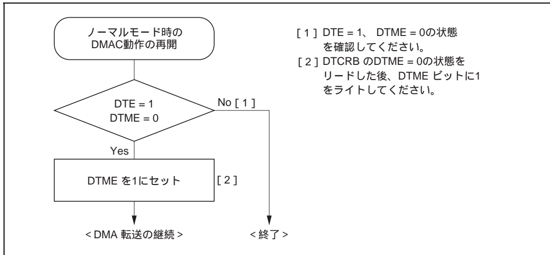
図 7.21 NMI 割り込みにより停止した DMAC 動作再開手順例
