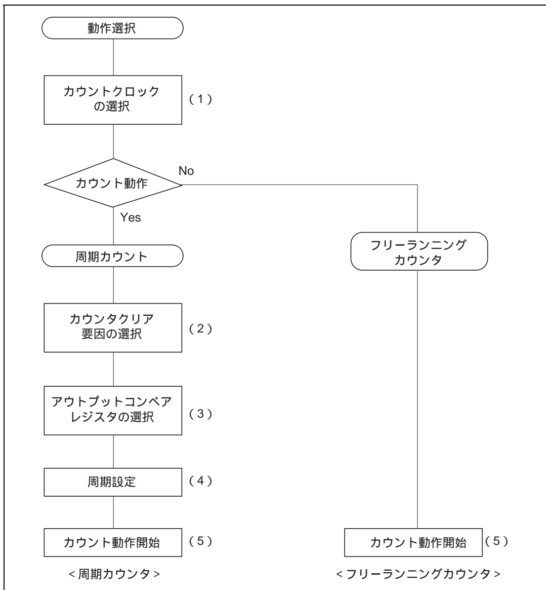
図 9.12 カウント動作設定手順例
