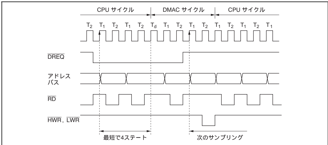
図 7.17 ノーマルモード時の \overline{\text{DREQ}} 端子の Low レベルによる DMAC 起動タイミング
