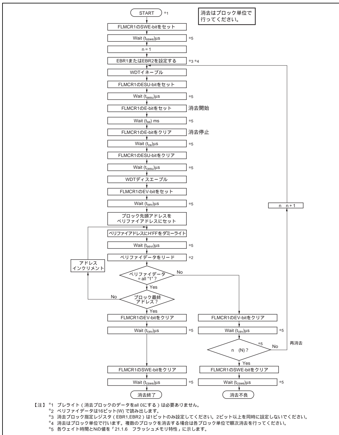
図 18.11 イレース/イレースペリファイフロー（単一ブロック消去）
