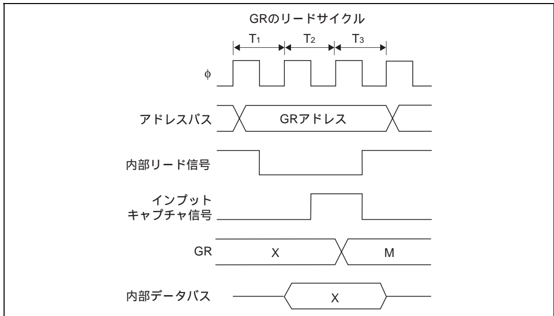
図9.42 GRのリードとインプットキャプチャの競合
