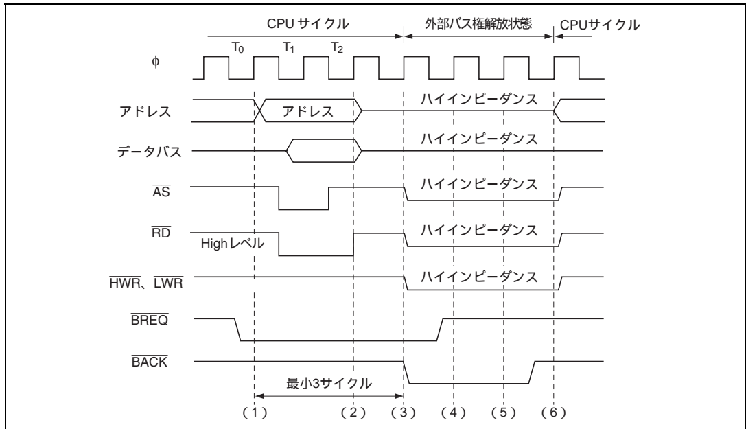
図 6.48 外部バスマスタ動作例
