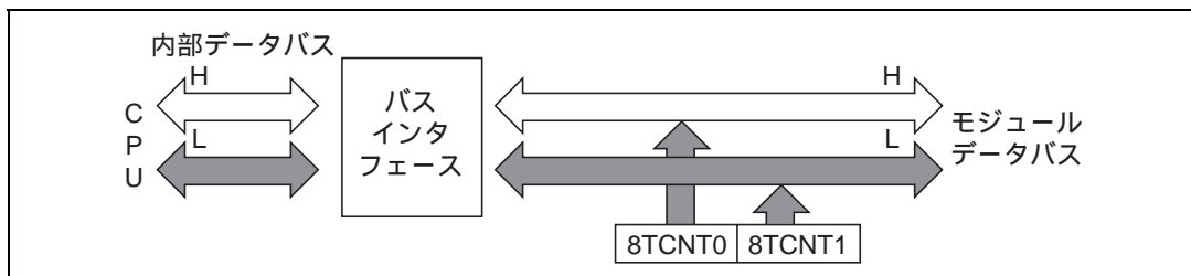
図 10.7 8TCNT1 のアクセス動作 [ 8TCNT1 CPU (下位バイト) ]
