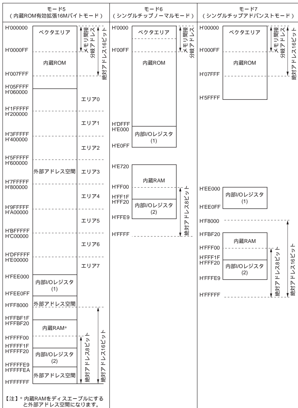
図 3.1 H8/3068F の各動作モードにおけるメモリマップ (EMC ビット=1 のとき) (2)
