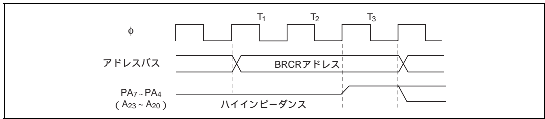
図 6.51 BRCR ライトタイミング
