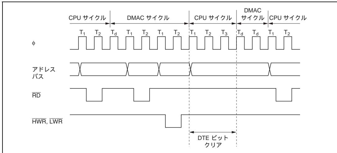
図 7.27 サイクルスチールモード DMA 転送の強制終了バスタイミング
