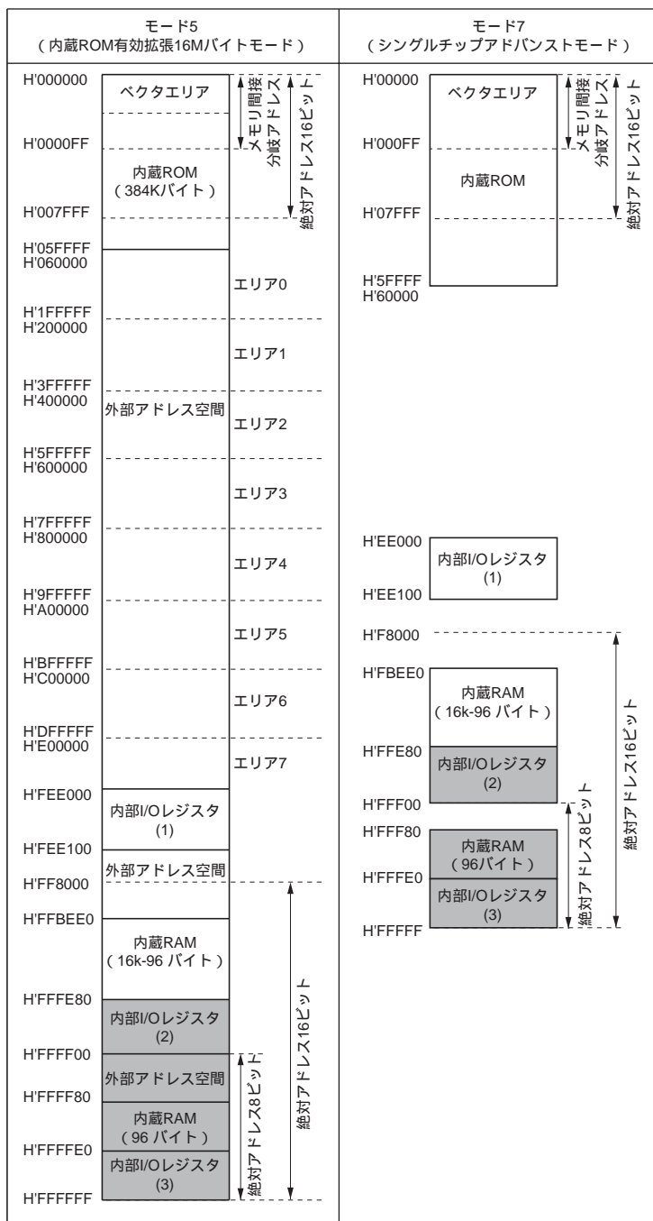
図 3.2 H8/3068F の各動作モードにおけるメモリマップ (EMC ビット=0 のとき) (2)
