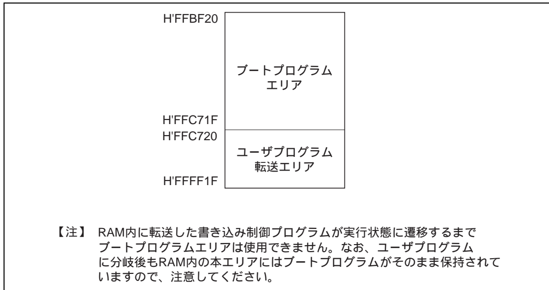
図 18.7 ブートモード時のRAMエリア
