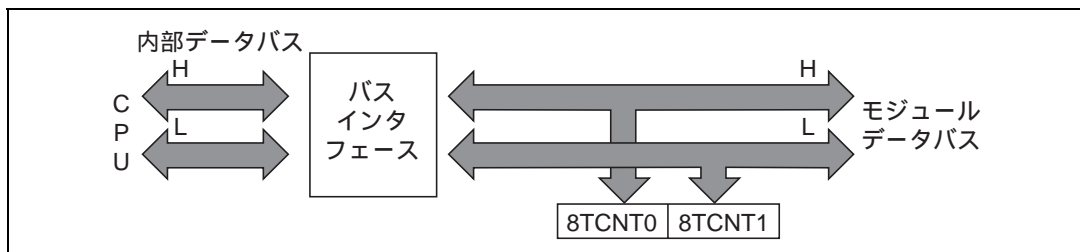
図 10.2 8TCNT のアクセス動作 [CPU 8TCNT (ワード)]
