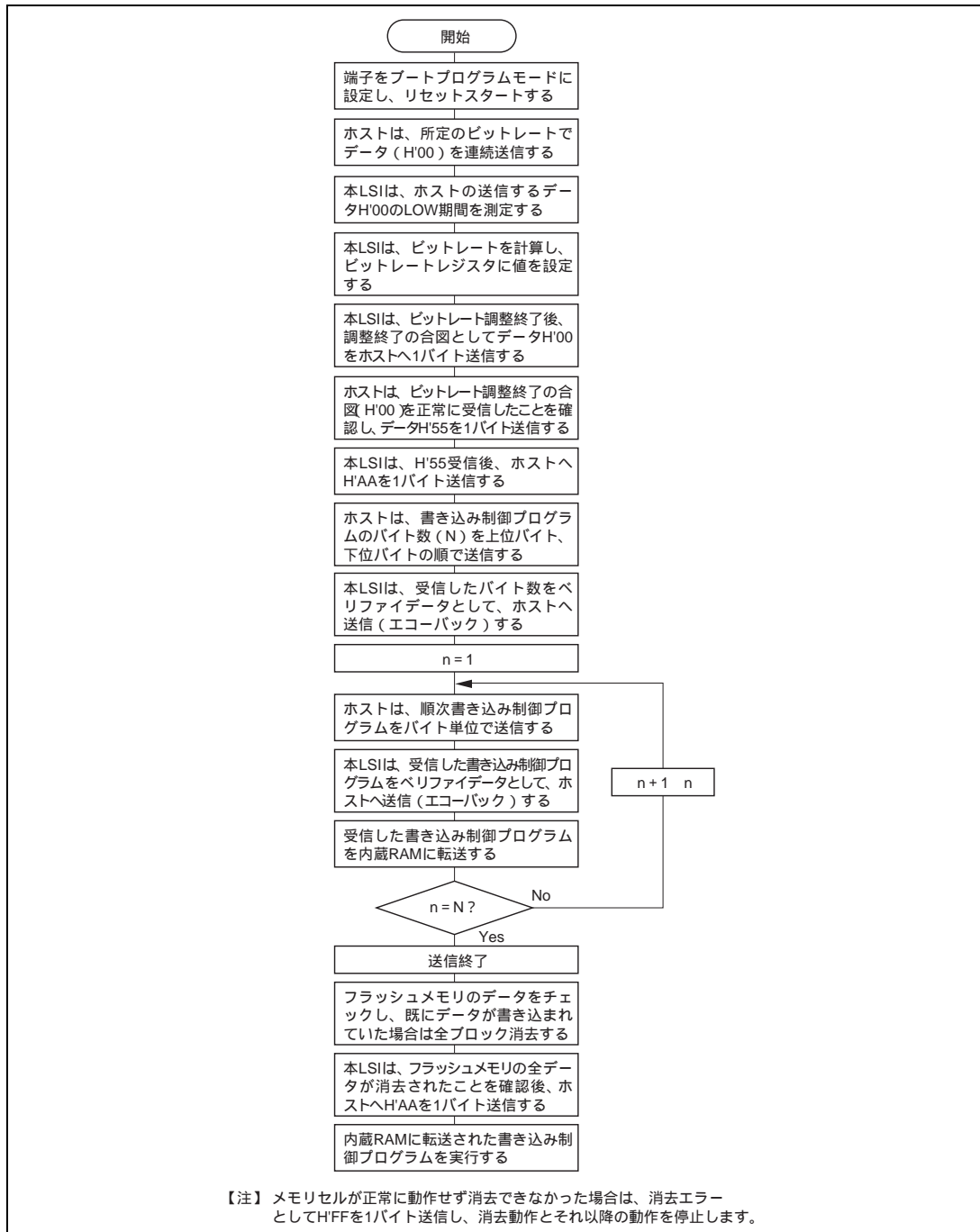
図 18.6 ブートモード実行手順
