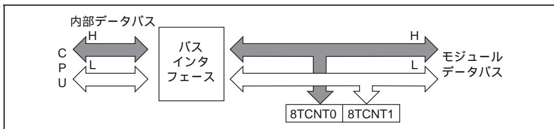
図 10.4 8TCNTH のアクセス動作 [CPU 8TCNTH (上位バイト)]
