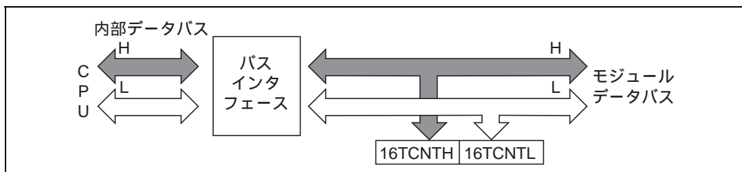
図 9.6 16TCNTH のアクセス動作 [ CPU 16TCNTH (上位バイト) ]
