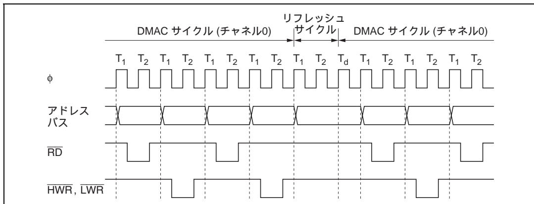
図 7.20 DRAM インタフェースと DMAC の動作タイミング
