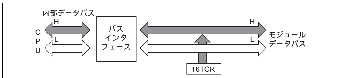
図 9.11 16TCR のアクセス動作 [ 16TCR CPU ]
