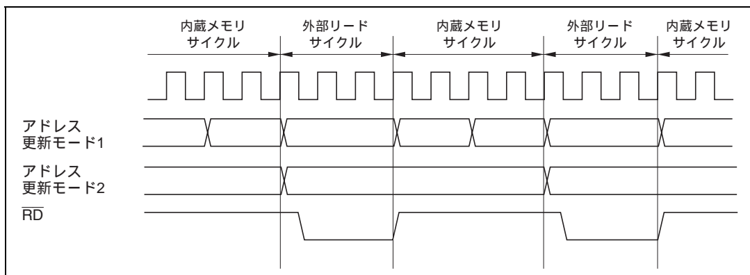
図 6.5 各アドレス更新モードにおけるアドレス出力例 （基本バスインタフェース、3 ステート空間の場合）
