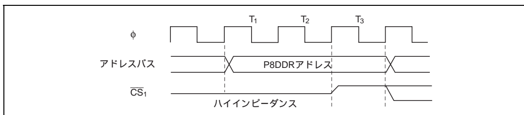
図 6.50 DDR ライトタイミング
