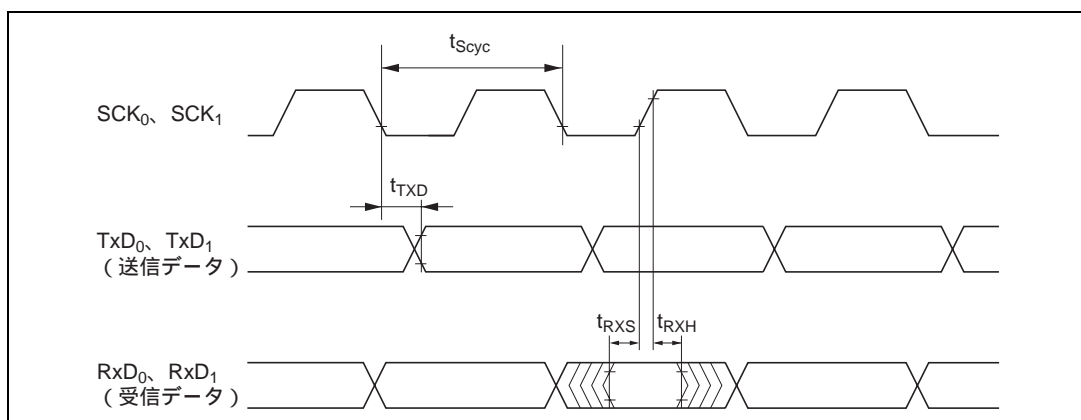
図 21.21 クロック同期式モード時の SCI 入出力タイミング
