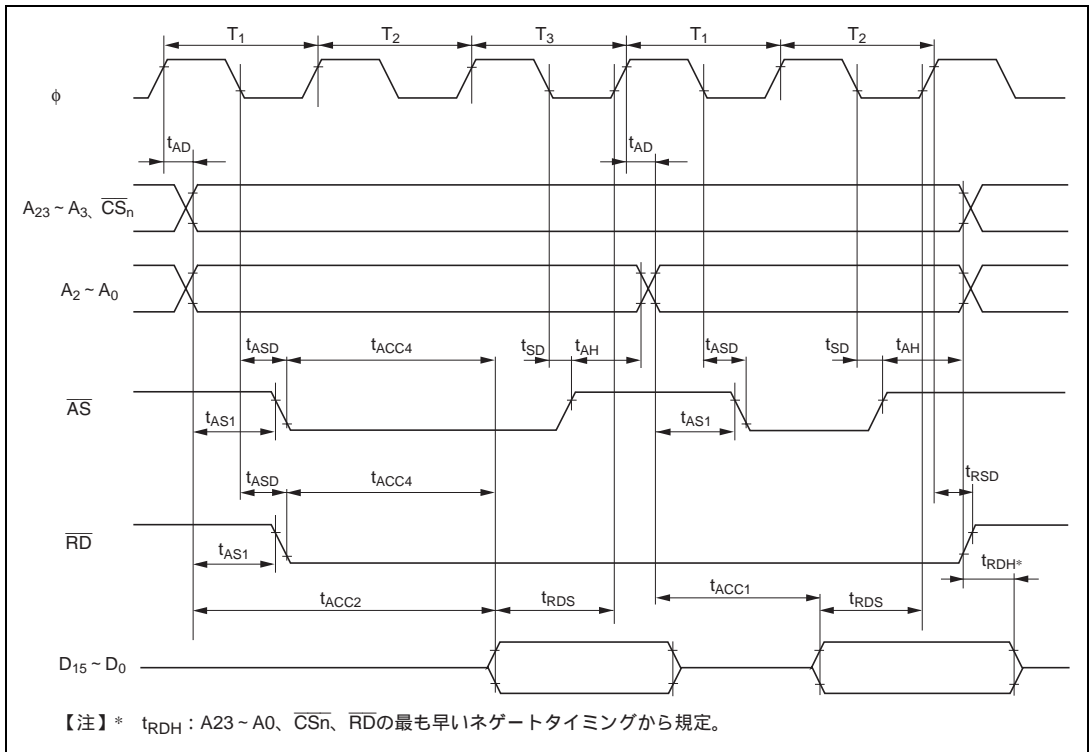
図 21.11 バースト ROM アクセスタイミング (バーストサイクル2 ステート)
