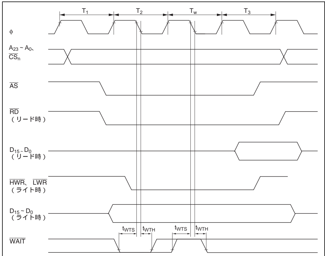
図 21.10 基本バスタイミング / 3 ステートアクセス 1 ウェイト
