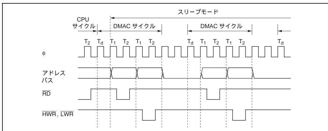
図 7.24 スリープモード中のサイクルスチールモードのタイミング
