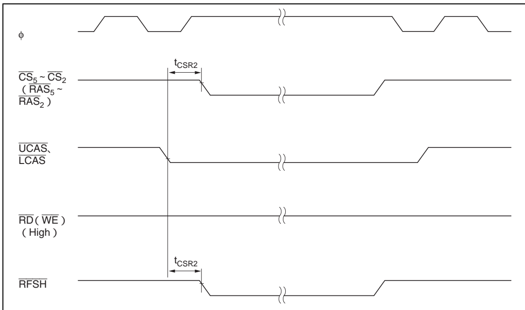
図 21.16 DRAM バスタイミング (セルフリフレッシュ)
