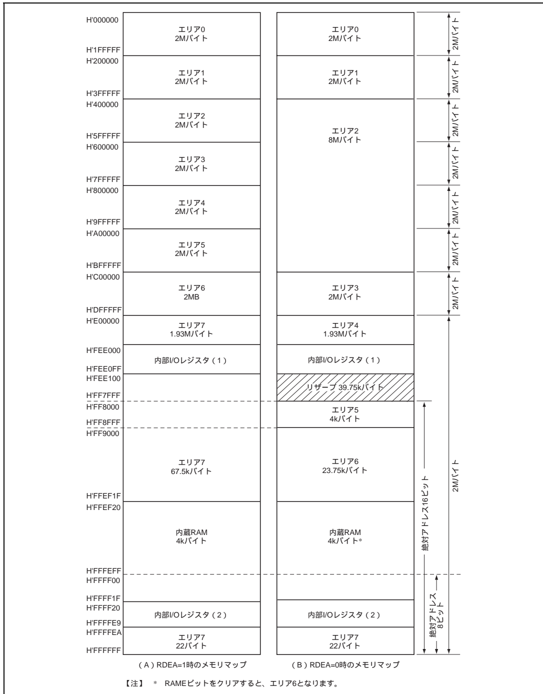
図 6.3 16M バイトモード時のメモリマップ
