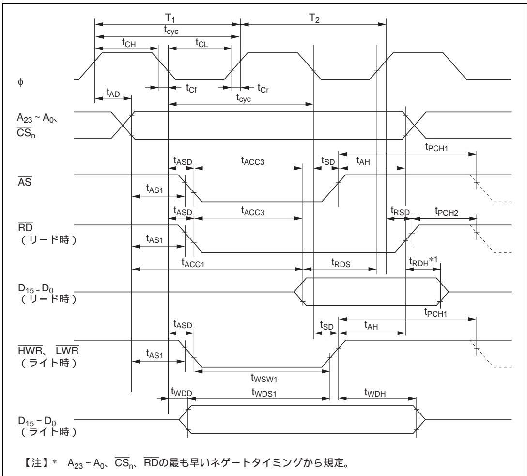
図 21.8 基本バスタイミング / 2ステートアクセス
