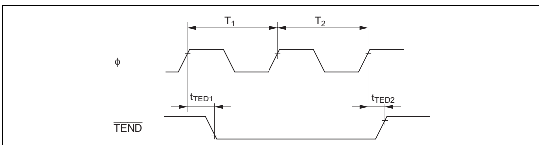
図 21.22 DMAC、 \overline{\text{TEND}} 出力タイミング / 2ステートアクセス
