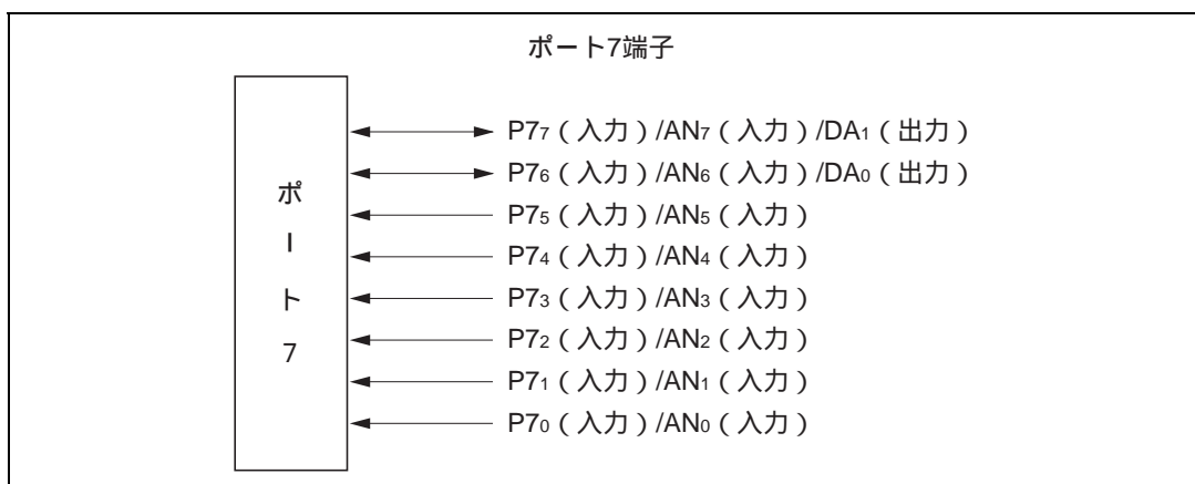
図 8.7 ポート 7 の端子構成
