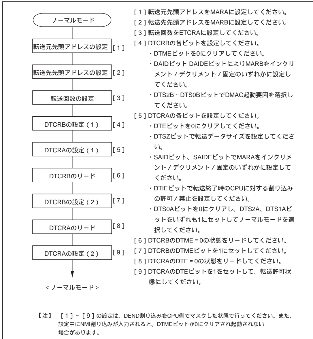
図 7.9 ノーマルモードの設定手順例
