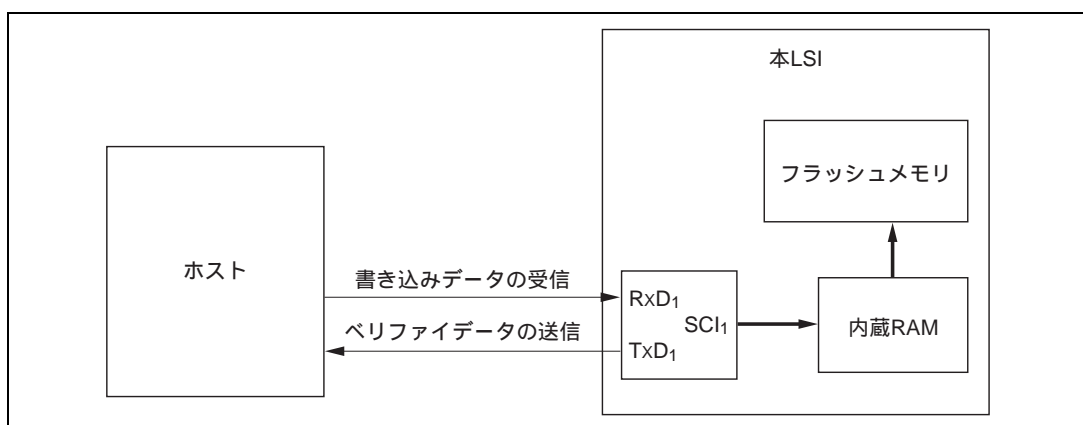
図 18.5 ブートモード時のシステム構成図
