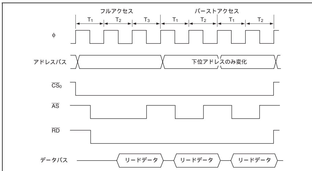
図 6.42 バースト ROM アクセスタイミング例
