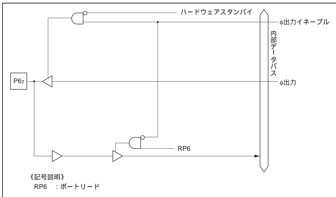
図 C.6 (g) ポート 6 ブロック図 (P6 7 端子)
