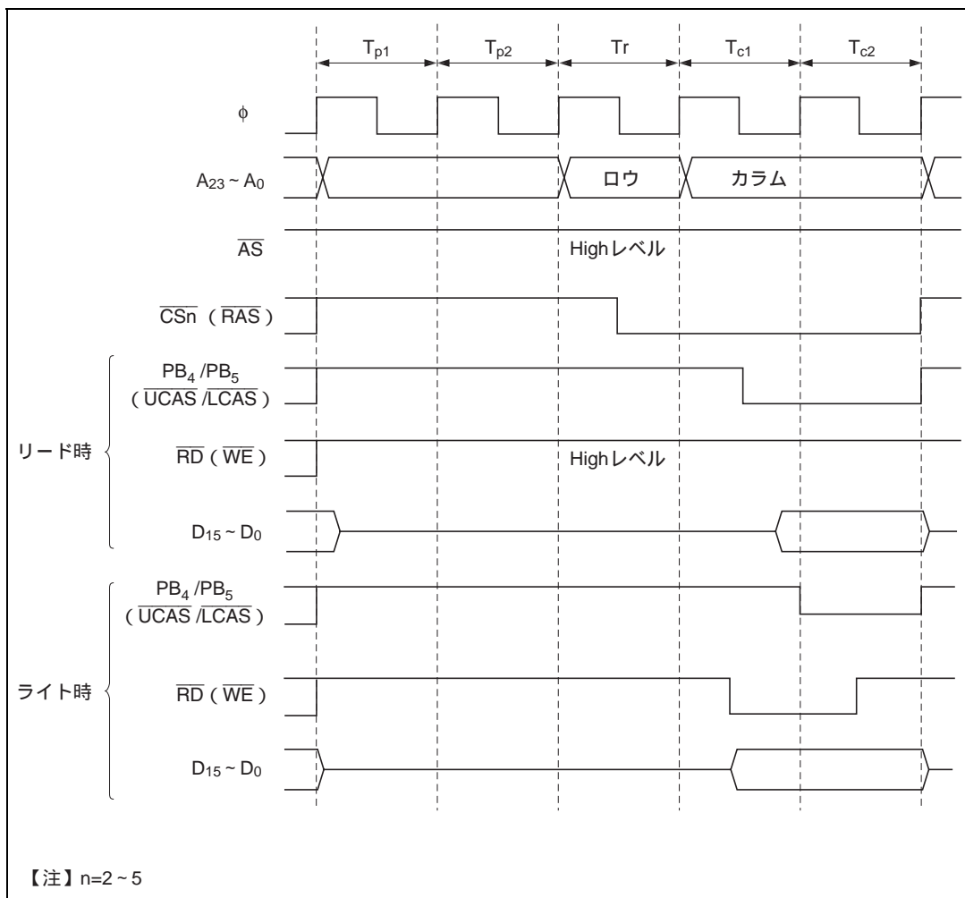
図 6.19 プリチャージサイクル 2 スタート時のタイミング (DRCRB の CSEL=0 の場合)
