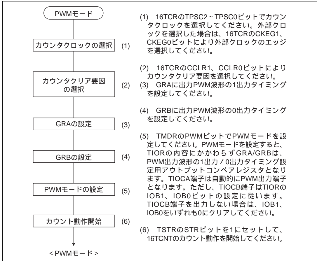
図9.26 PWMモードの設定手順
