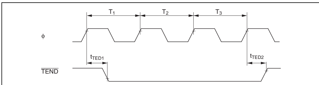
図 21.23 DMAC、 \overline{\text{TEND}} 出力タイミング / 3ステートアクセス
