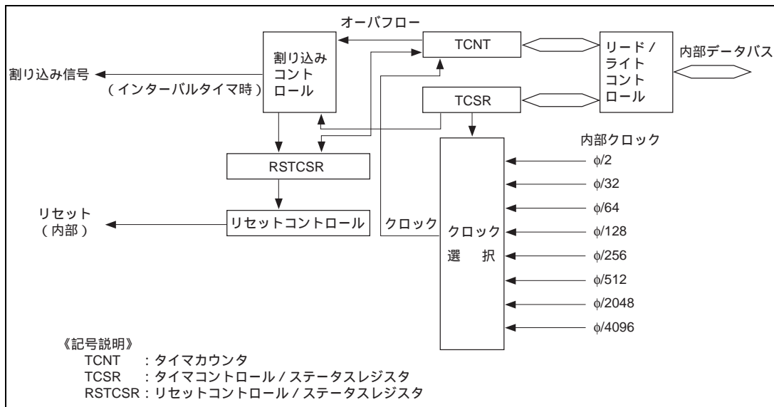
図 12.1 WDT のブロック図
