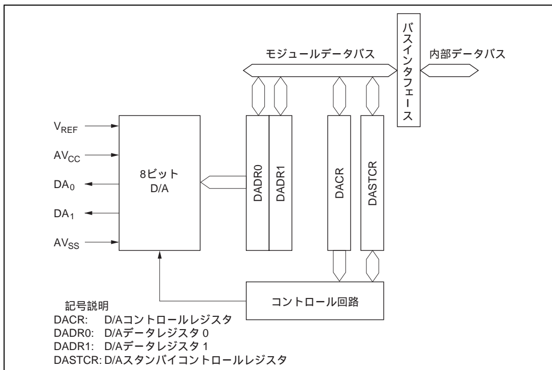
図 16.1 D/A 変換器のブロック図
