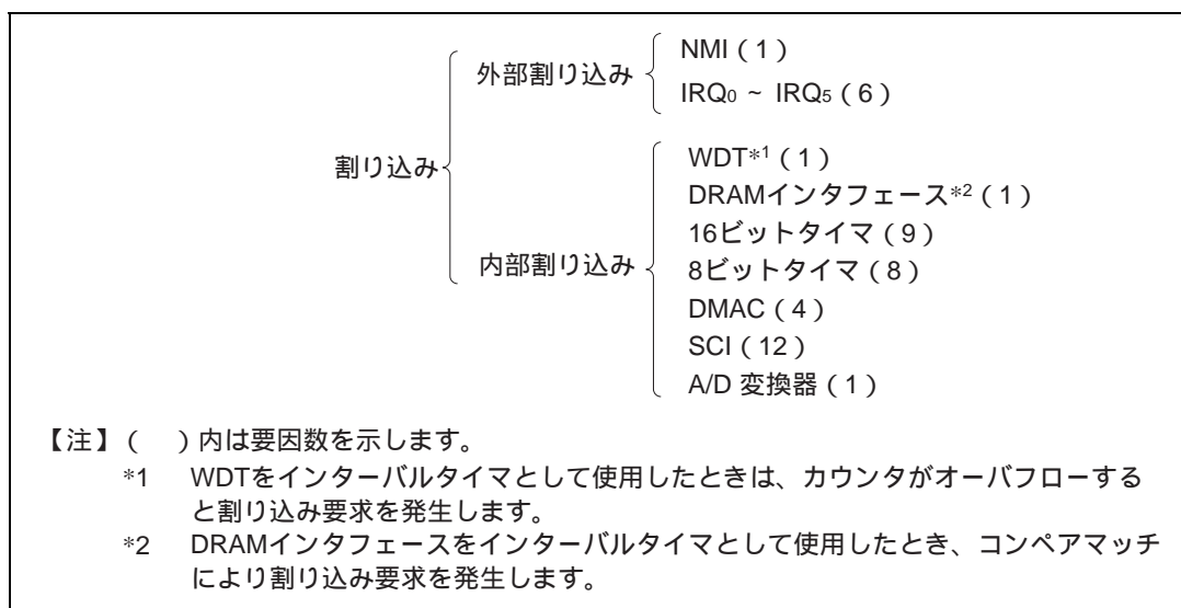
図 4.5 割り込み要因と要因数
