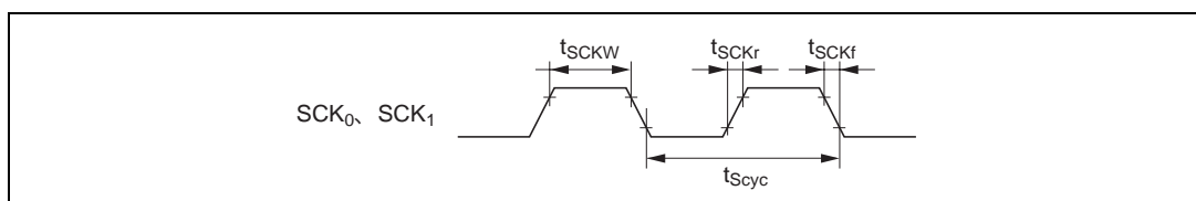
図 21.20 SCI 入力クロックタイミング
