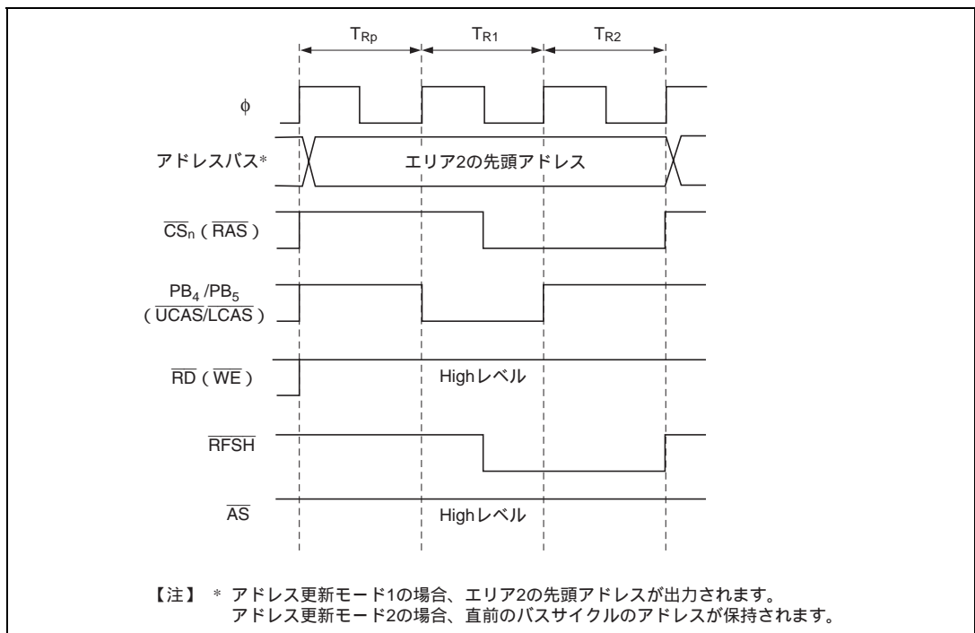
図 6.28 CBR リフレッシュタイミング (CSEL=0,TPC=0,RLW=0 の場合)
