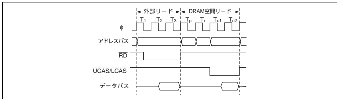
図 6.46 アイドルサイクル動作例 (4) (プリチャージサイクルが連続する場合)
