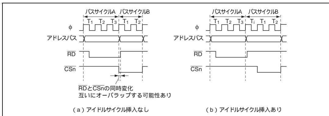
図 6.47 アイドルサイクル動作例 (5)
