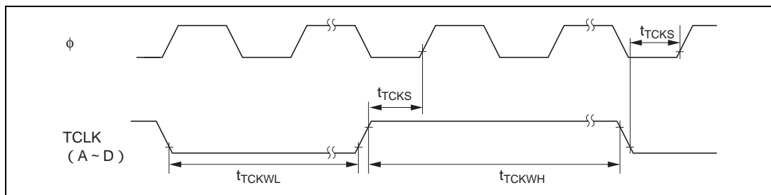
図 21.19 タイマ外部クロック入力タイミング
