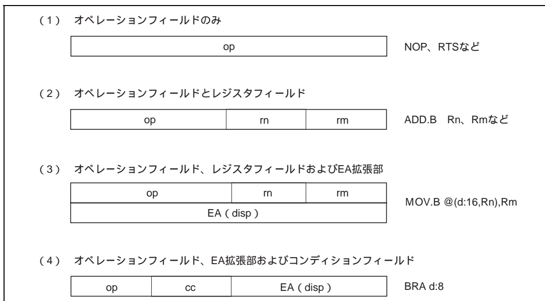
図 2.9 命令フォーマット
