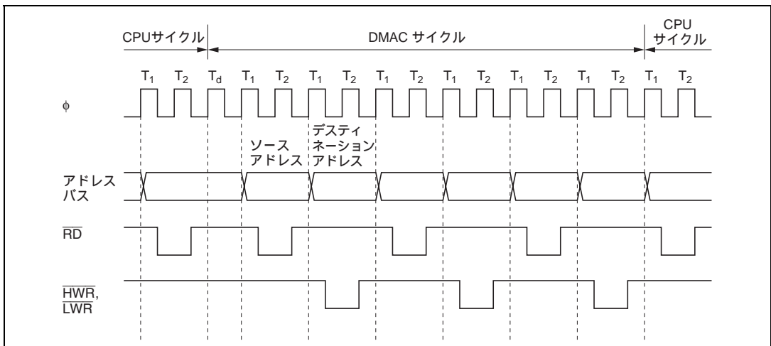
図 7.15 バーストモード DMA 転送バスタイミング
