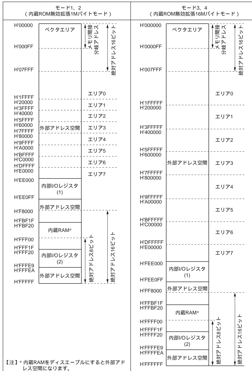
図 3.1 H8/3068F の各動作モードにおけるメモリマップ (EMC ビット=1 のとき) (1)
