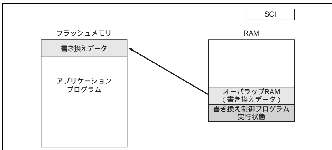
図 18.4 ユーザプログラムモードのオーバーラップ RAM データの書き込み
