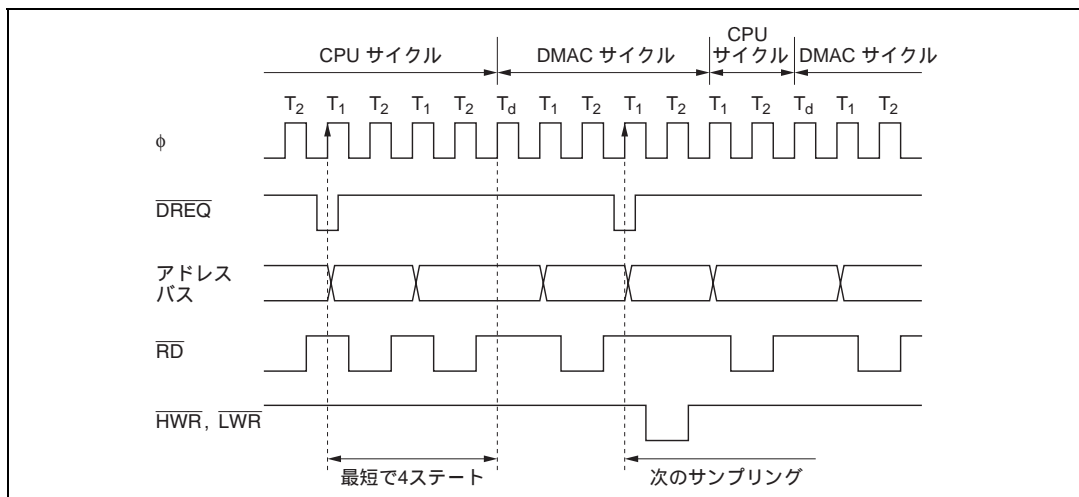
図 7.16 ノーマルモード時の \overline{\text{DREQ}} 端子の立ち下がりエッジで DMAC 起動タイミング
