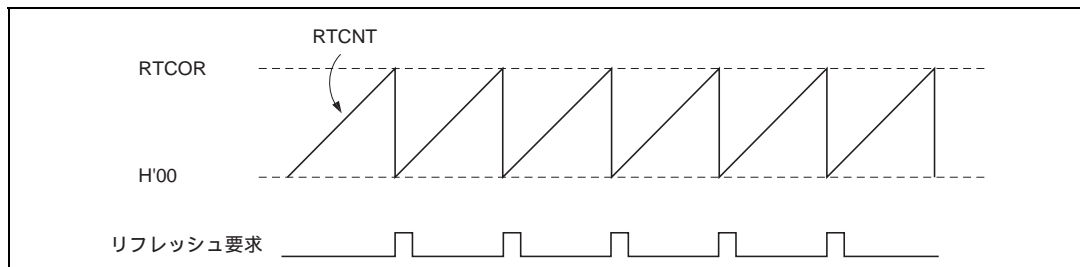
図 6.26 RTCNT の動作
