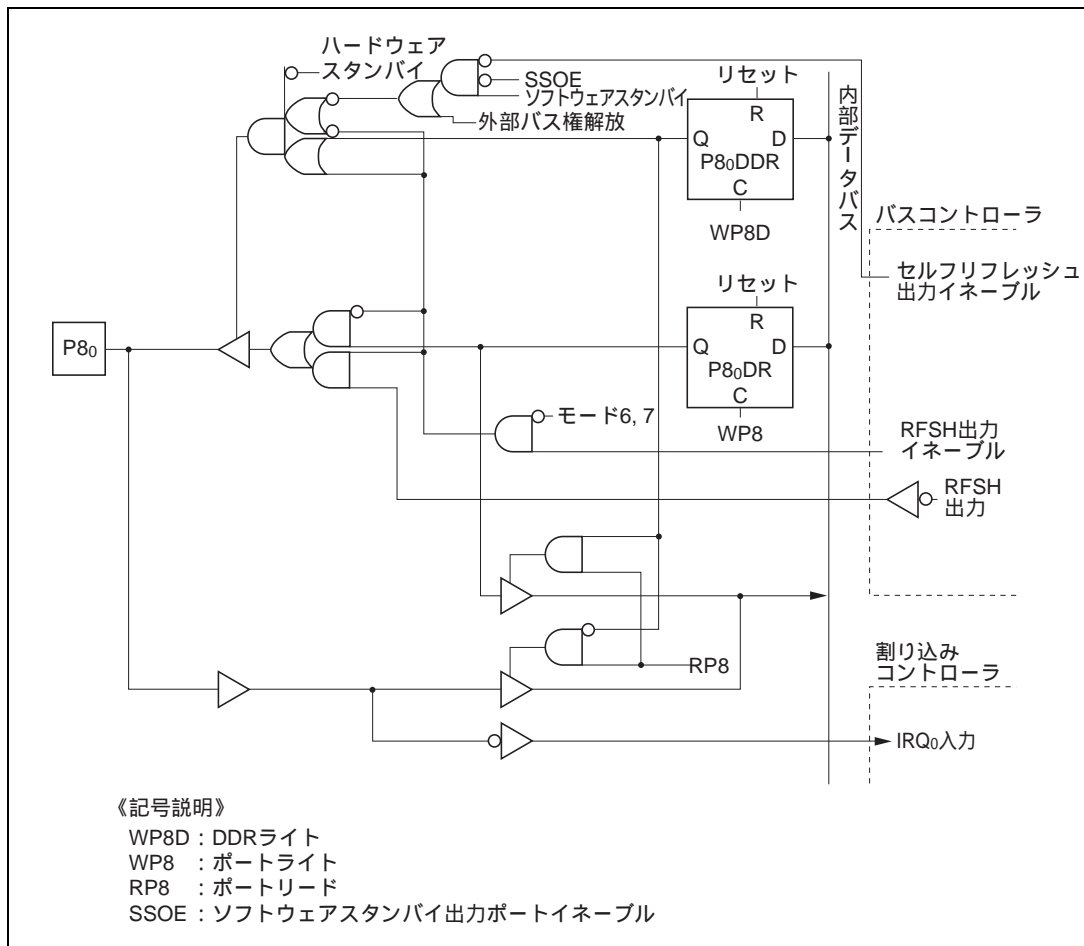
図 C.8 (a) ポート 8 ブロック図 (P8 0 端子)
