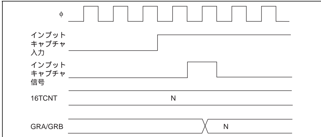
図 9.23 インพุットキャプチャ入力信号タイミング
