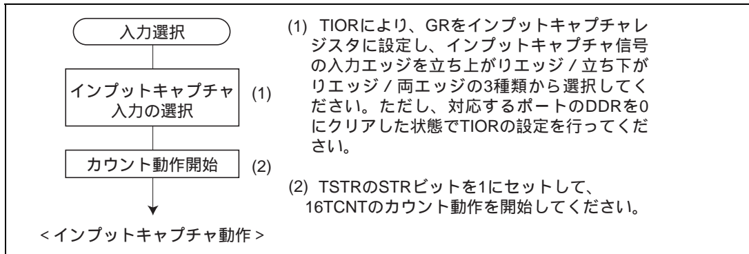
図 9.21 インットキャプチャ動作の設定手順例
