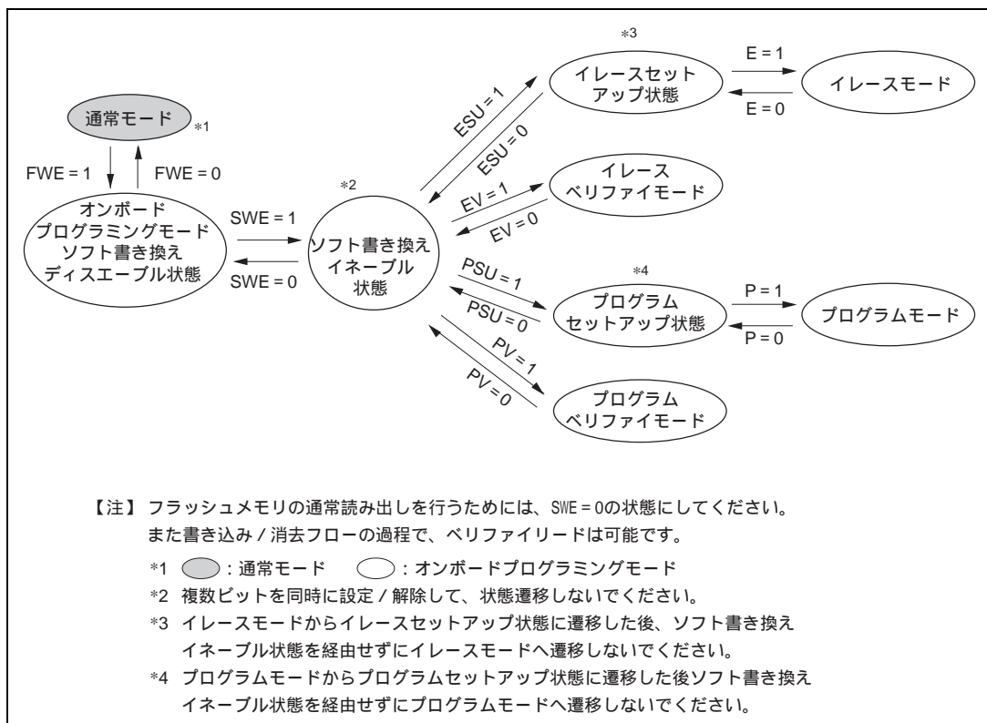
図 18.9 FLMCR1 の各ビット設定による状態遷移
