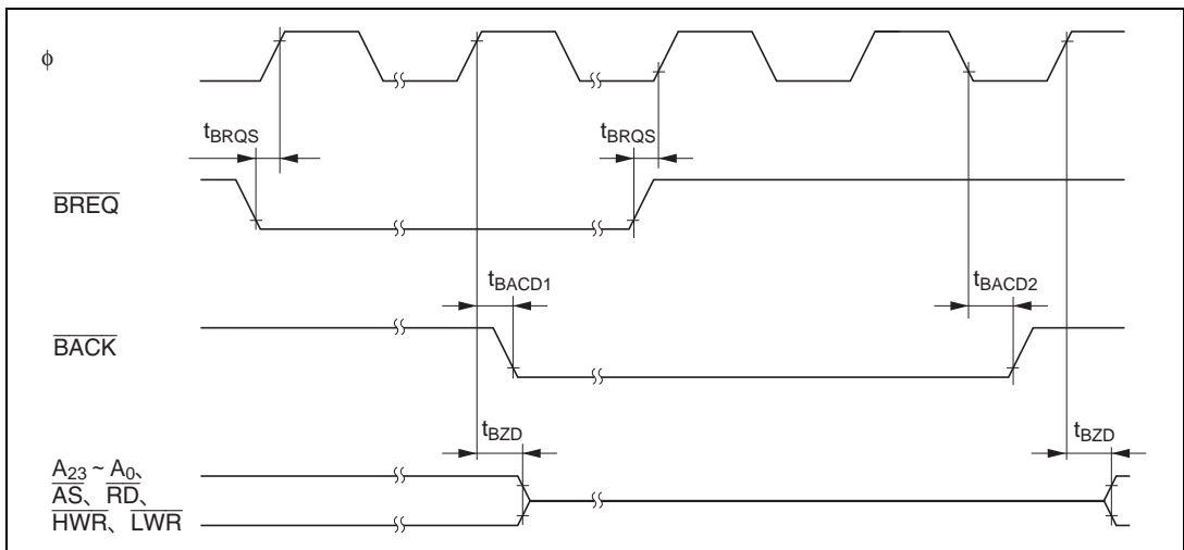
図 21.13 バスリリースモードタイミング
