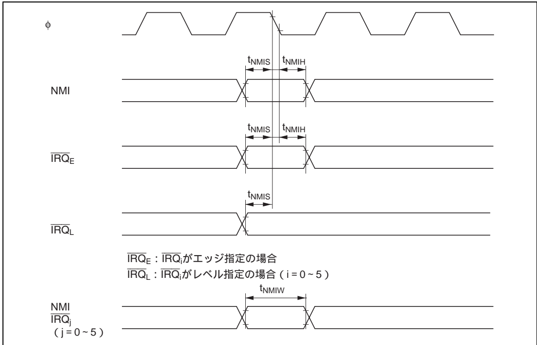
図 21.7 割り込み入力タイミング
