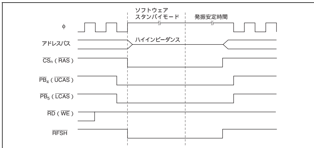
図 6.30 セルフリフレッシュタイミング (CSEL=0 の場合)
