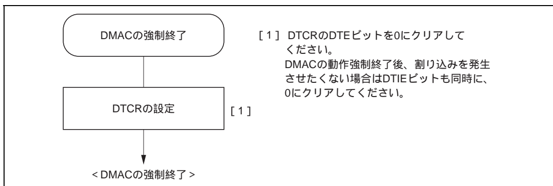
図 7.22 DMAC 動作の強制終了手順
