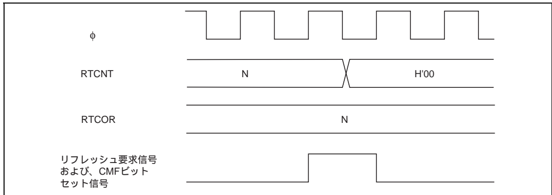
図 6.27 コンペアマッチのタイミング
