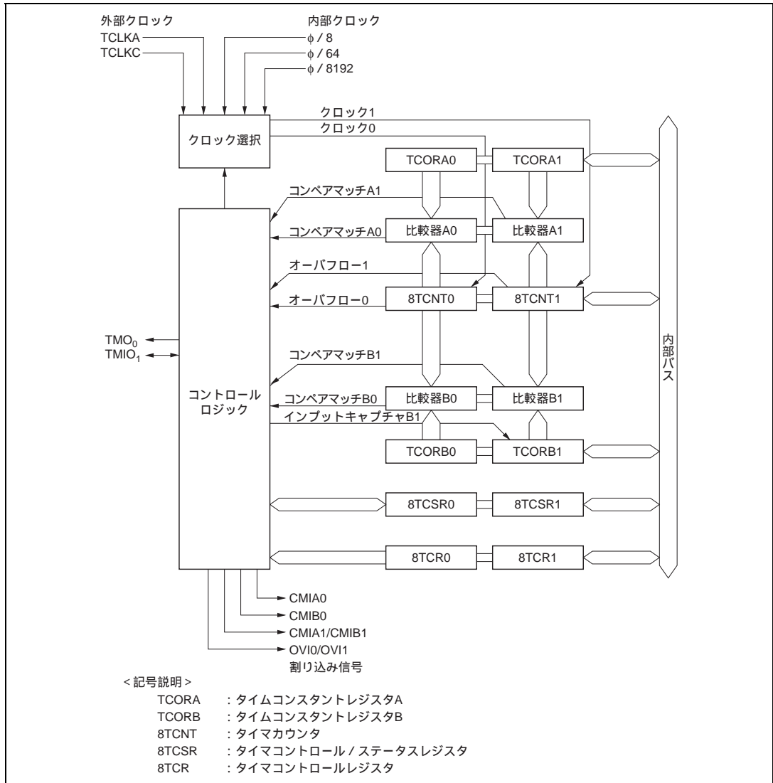
図 10.1 8ビットタイマのブロック図(2チャンネル分:グループ0)
