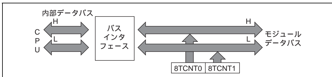
図 10.3 8TCNT のアクセス動作 [8TCNT CPU (ワード)]
