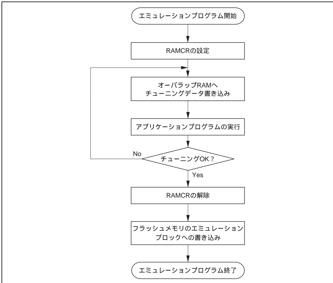
図 18.13 RAM によるエミュレーションフロー
