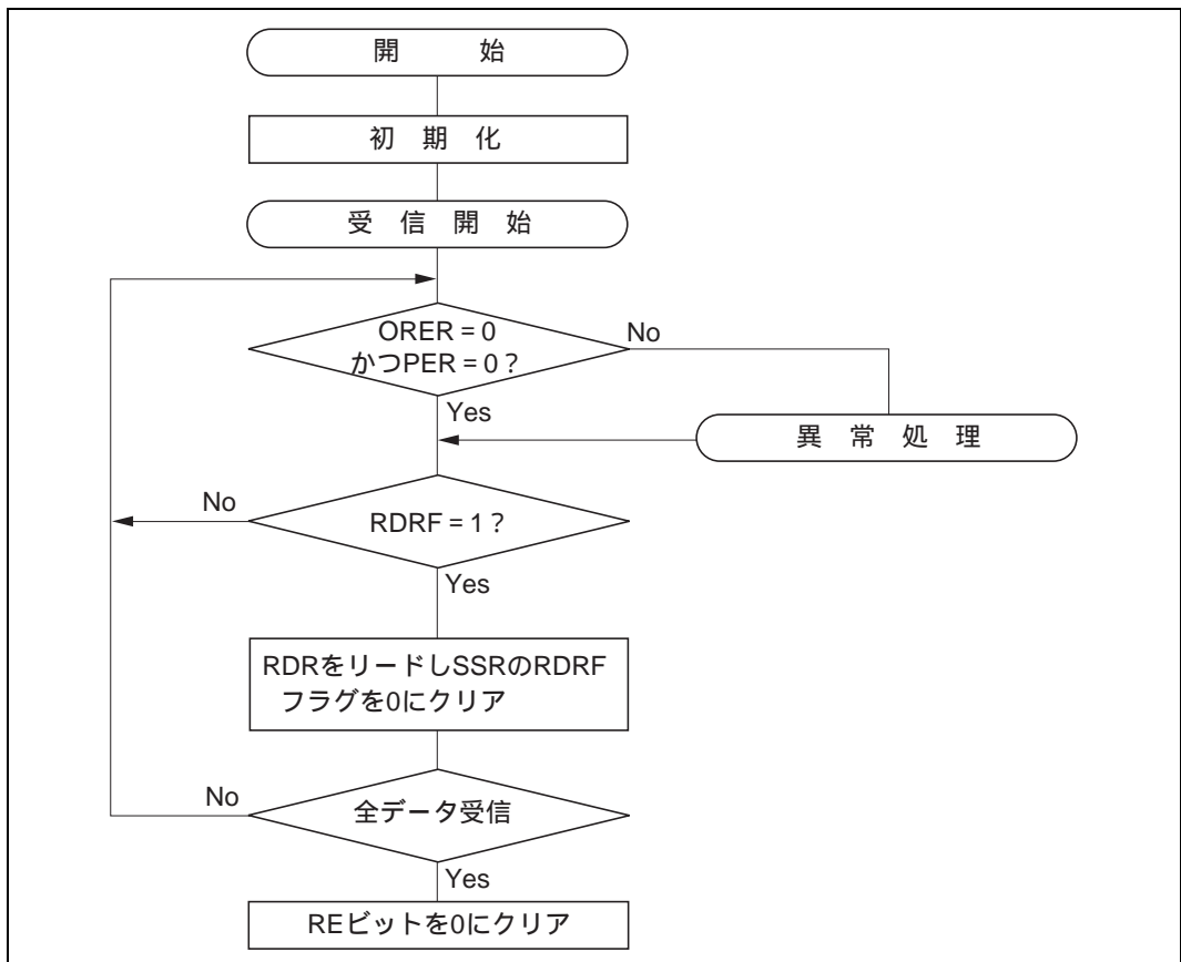
図 14.8 受信処理フローの例
