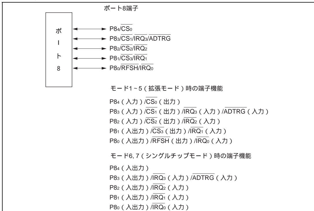
図 8.8 ポート 8 の端子構成
