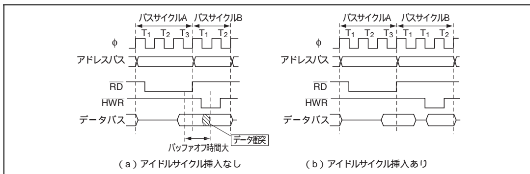
図 6.44 アイドルサイクル動作例 (2) (ICIS0=1 のとき)
