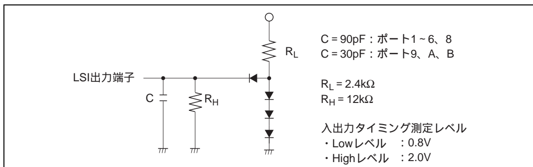
図 21.3 出力負荷回路
