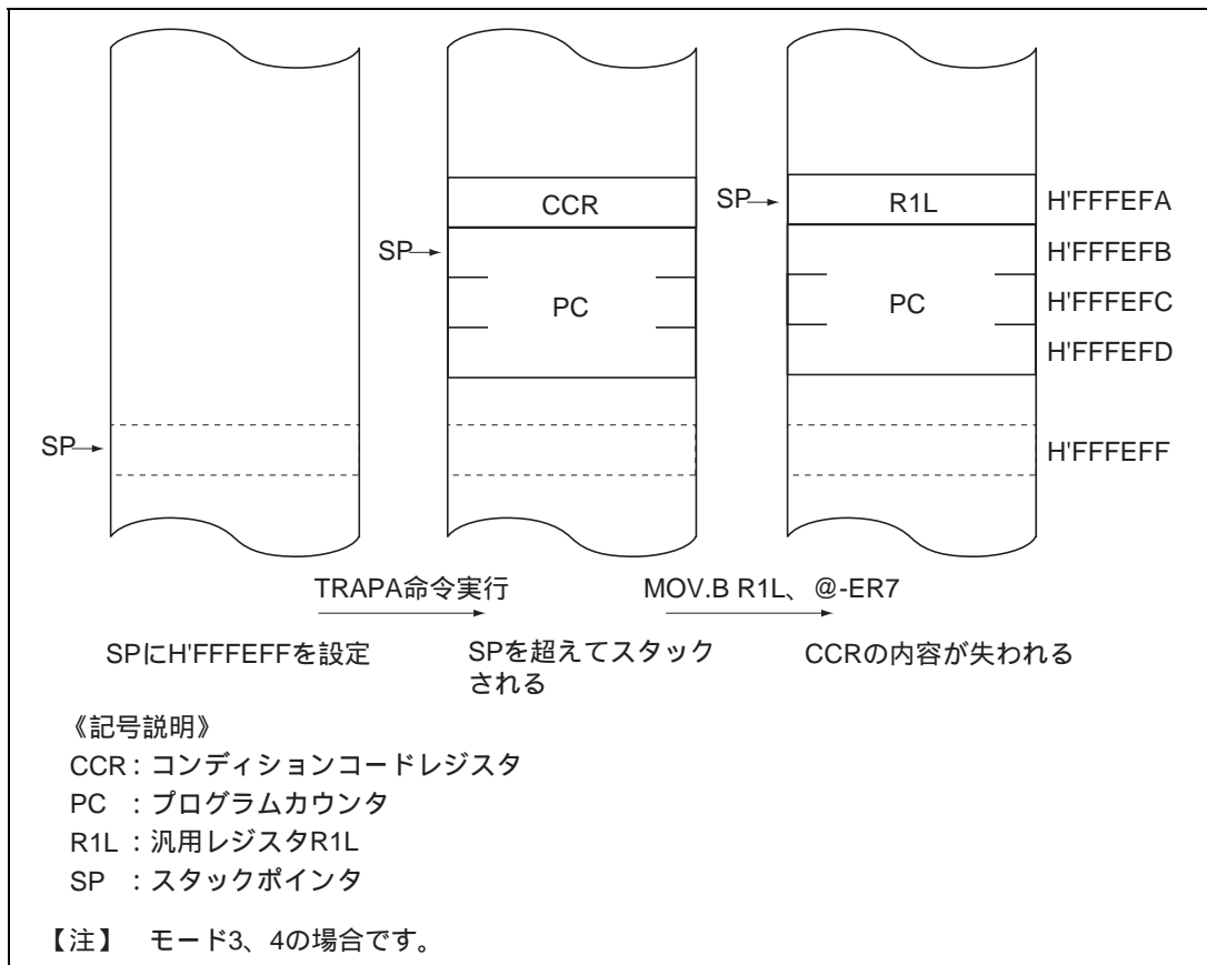
図 4.7 SP を奇数に設定したときの動作
