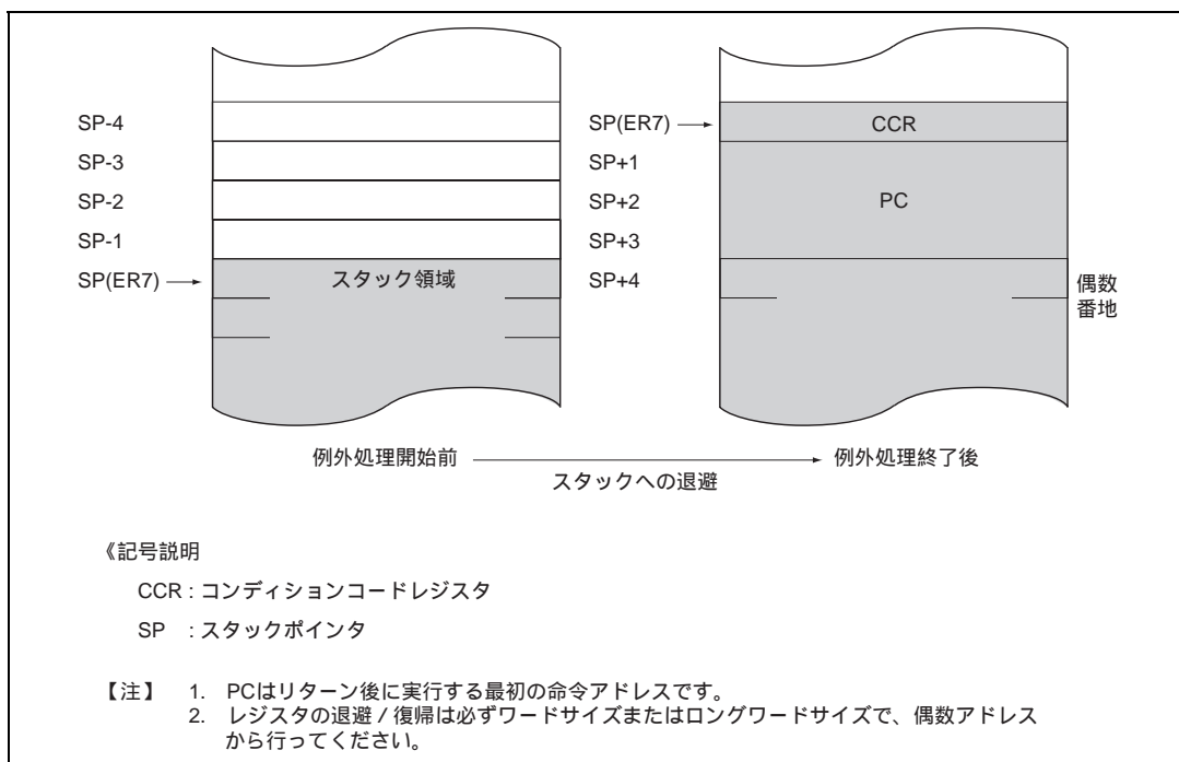
図 2.14 例外処理終了後のスタック状態
