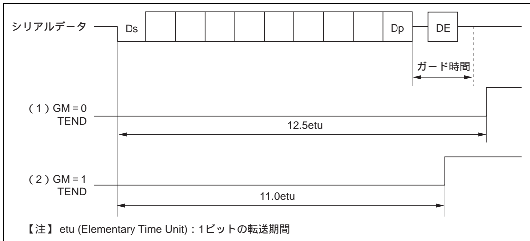
図 14.4 TEND フラグセットタイミング
