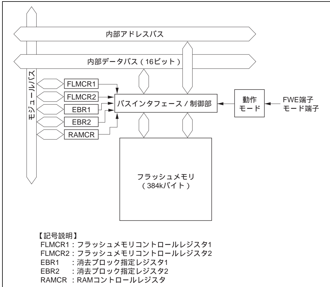
図 18.1 フラッシュメモリのブロック図
