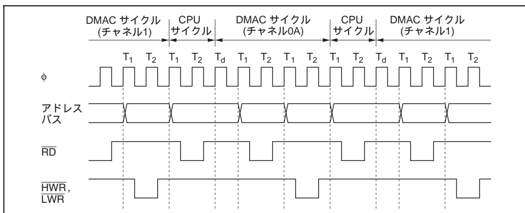
図 7.19 複数チャンネルの動作タイミング
