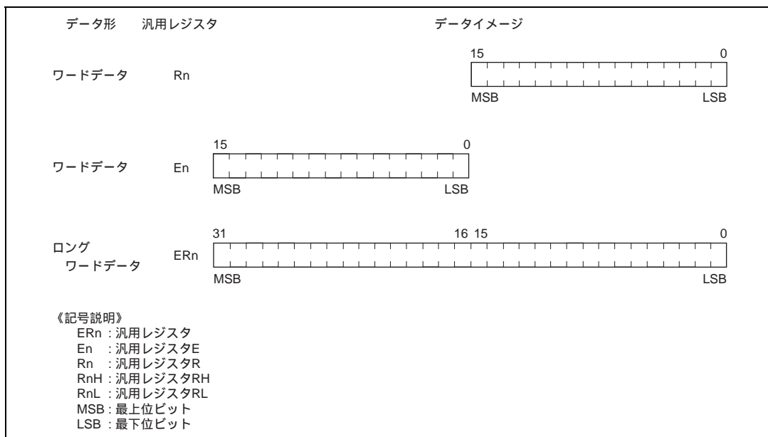
図 2.7 汎用レジスタのデータ構成 (2)
