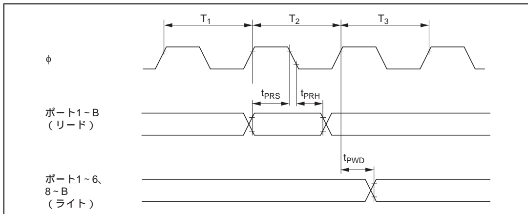
図 21.17 TPC、I/Oポート入出力タイミング
