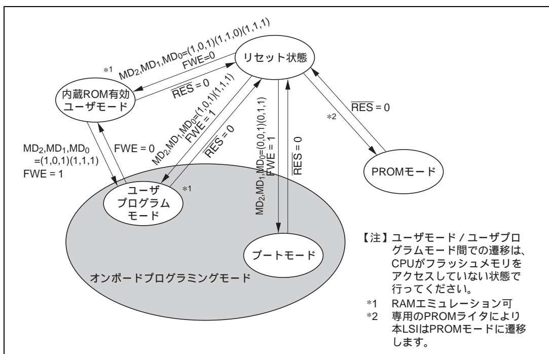
図 18.2 フラッシュメモリに関する状態遷移
