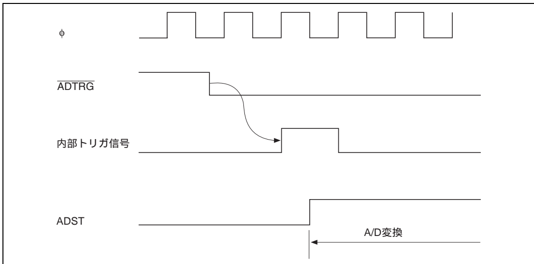
図 15.6 外部トリガ入力タイミング
