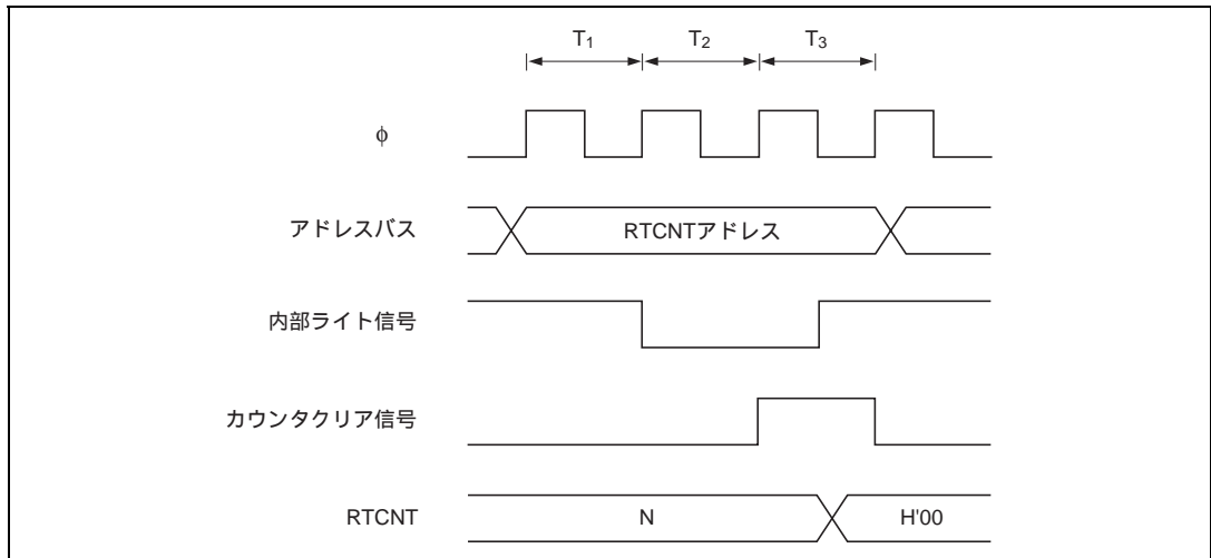
図 6.39 RTCNT のライトとクリアの競合
