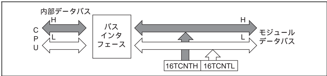
図 9.8 16TCNTH のアクセス動作 [ 16TCNTH CPU (上位バイト) ]
