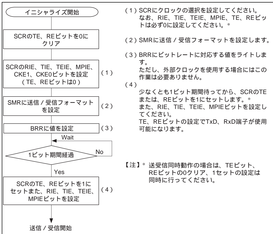
図 13.15 SCI のイニシャライズフローチャートの例
