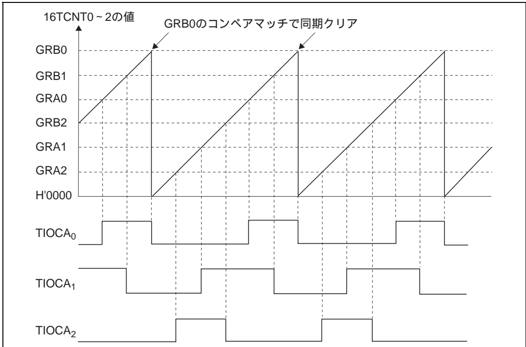
図 9.25 同期動作例
