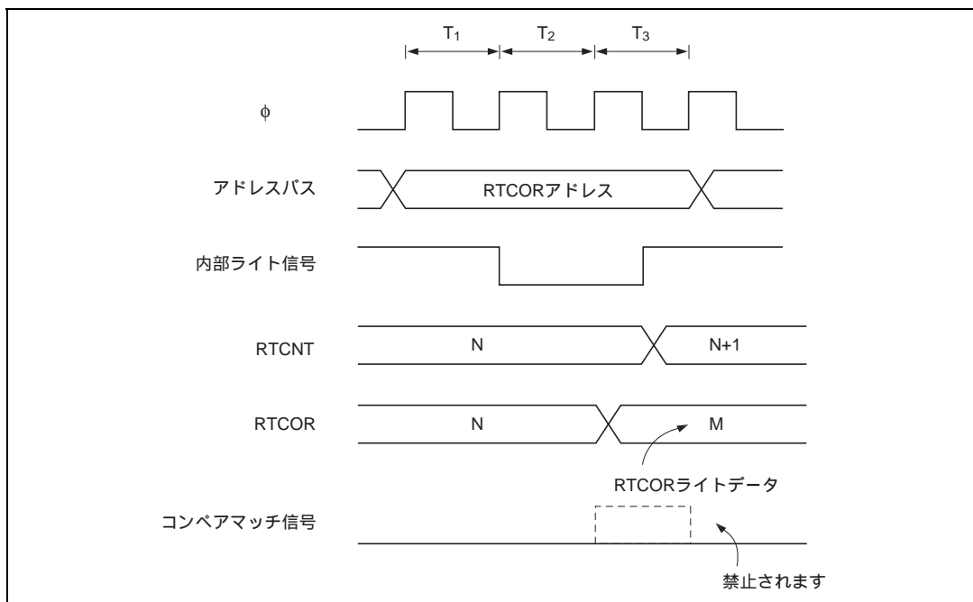
図 6.41 RTCOR のライトとコンペアマッチの競合
