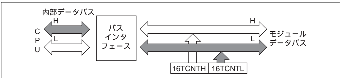
図 9.9 16TCNTL のアクセス動作 [ 16TCNTL CPU (下位バイト) ]
