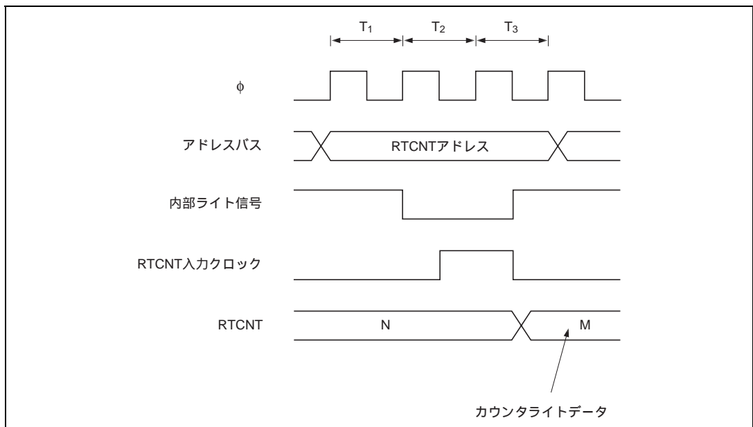
図 6.40 RTCNT のライトとカウントアップの競合
