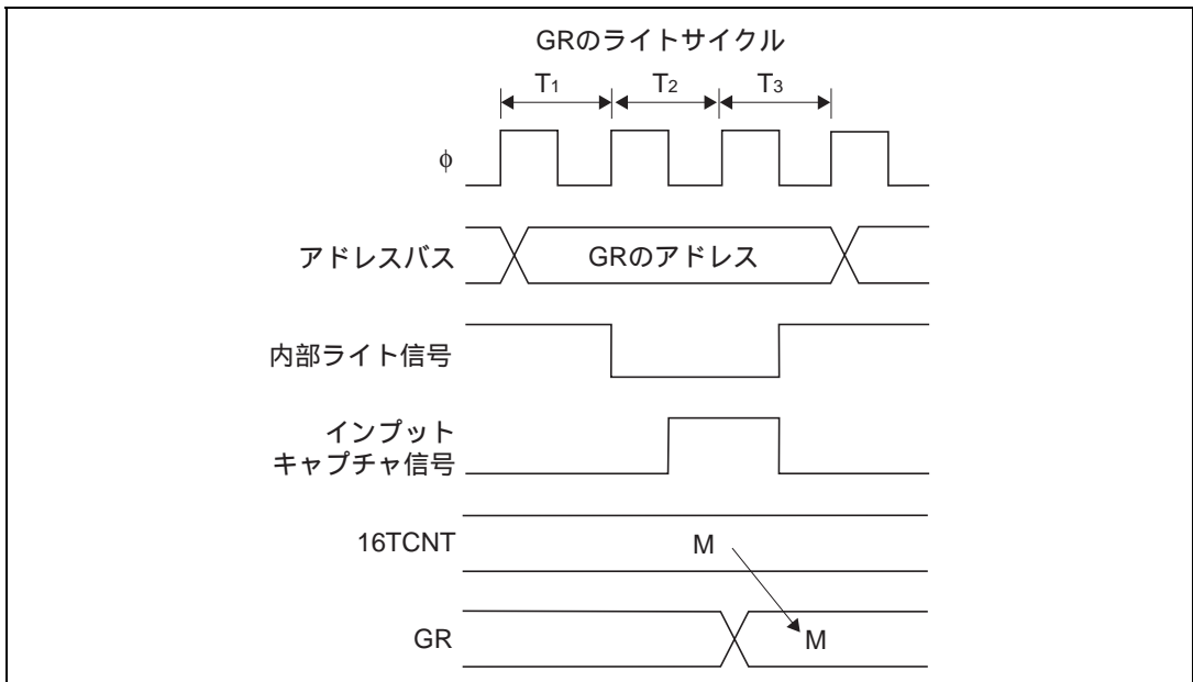
図 9.44 GRのライトと入力キャプチャの競合
