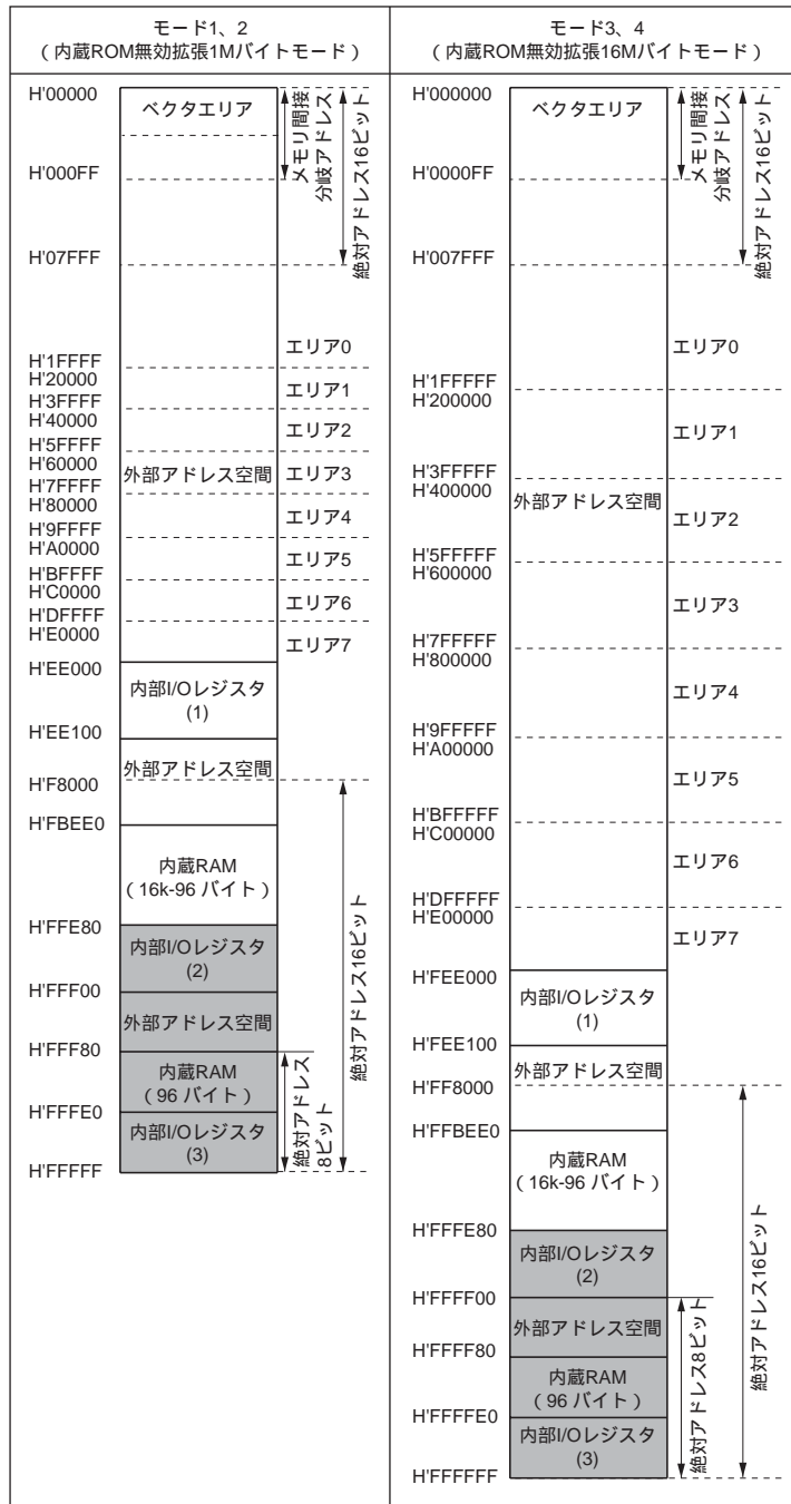
図 3.2 H8/3068F の各動作モードにおけるメモリマップ (EMC ビット=0 のとき) (1)
