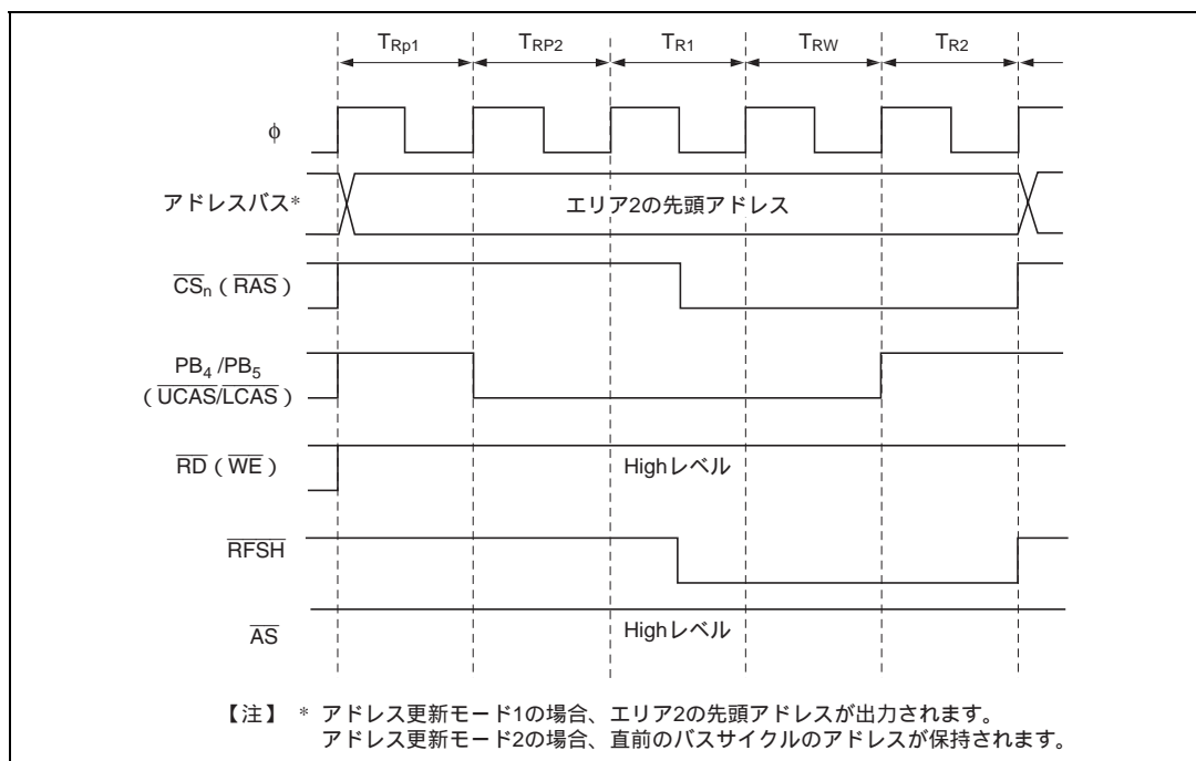
図 6.29 CBR リフレッシュタイミング (CSEL=0、TPC=1、RLW=1 の場合)
