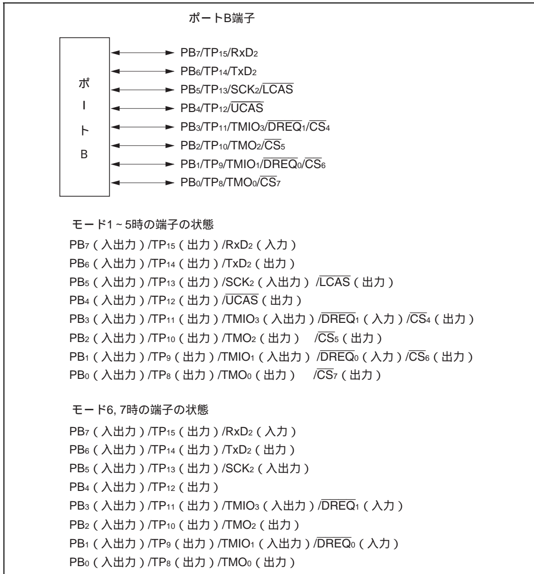
図 8.11 ポート B の端子構成
