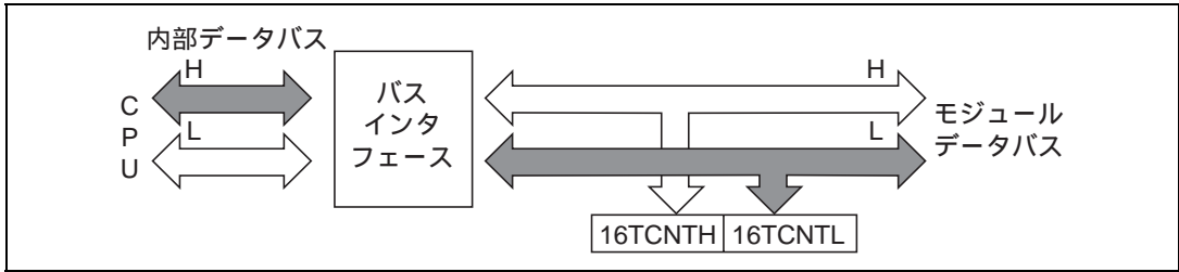
図 9.7 16TCNTL のアクセス動作 [ CPU 16TCNTL (下位バイト) ]
