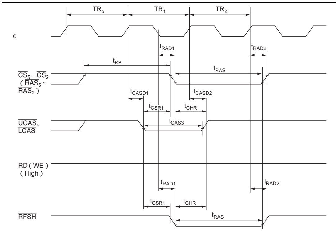
図 21.15 DRAM バスタイミング (CAS ビフォア RAS リフレッシュ)
