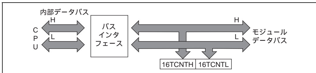
図 9.4 16TCNT のアクセス動作 [ CPU 16TCNT (ワード) ]
