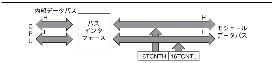
図 9.5 16TCNT のアクセス動作 [ 16TCNT CPU (ワード) ]
