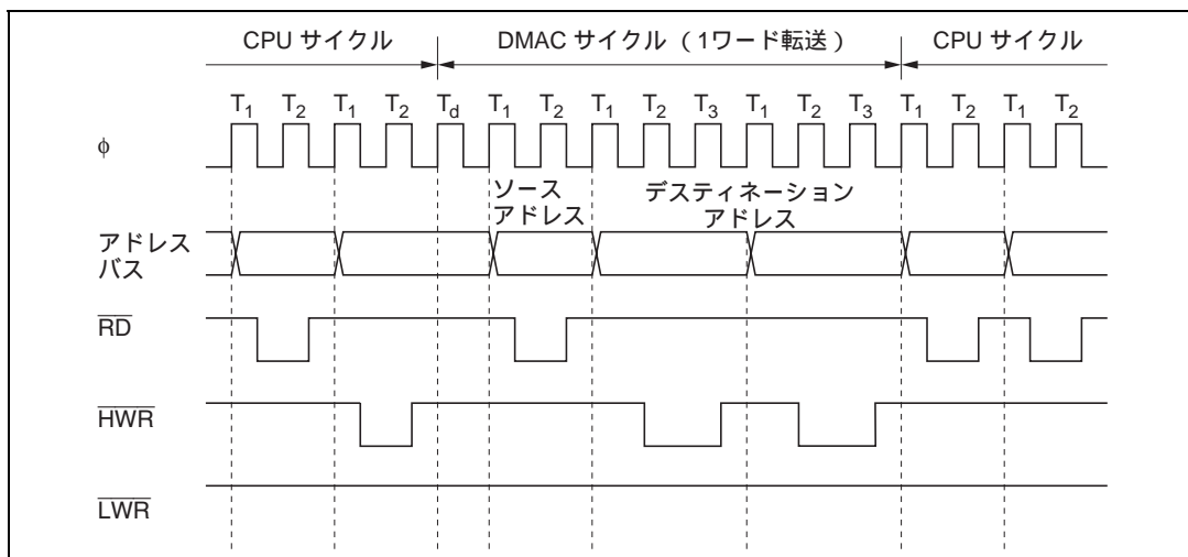
図 7.13 DMA 転送バスタイミング例
