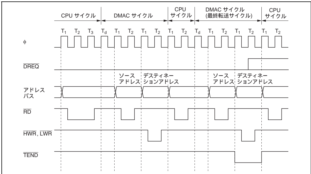
図 7.14 DREQ 端子 Low レベル入力選択時の DMAC 転送バスタイミング
