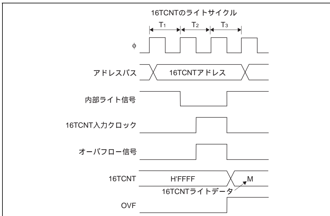
図 9.41 16TCNT のライトとオーバーフローの競合
