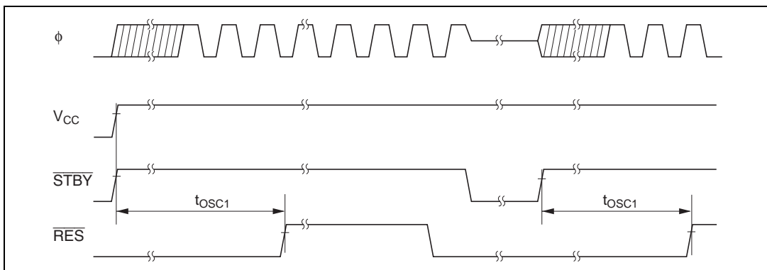
図 21.4 発振安定時間タイミング
