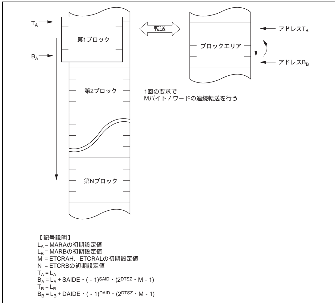
図 7.10 ブロック転送モードの動作
