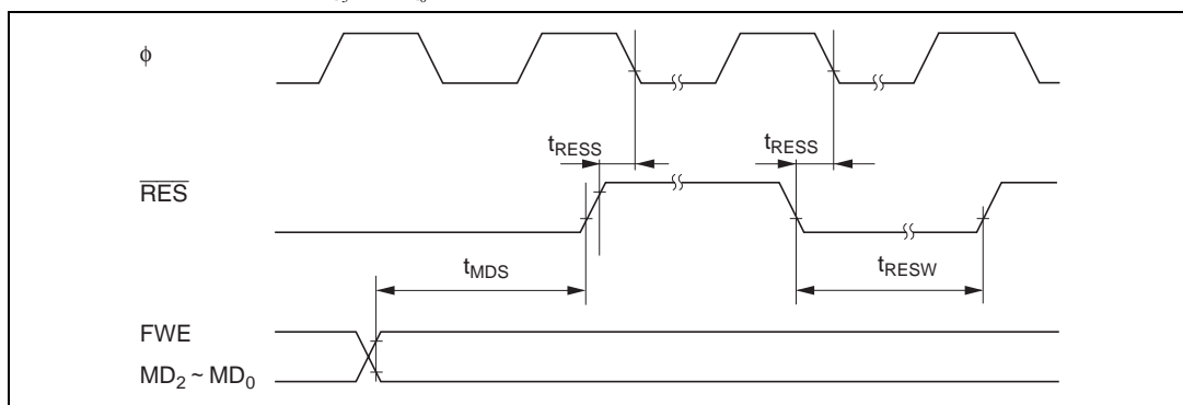
図 21.5 リセット入力タイミング
