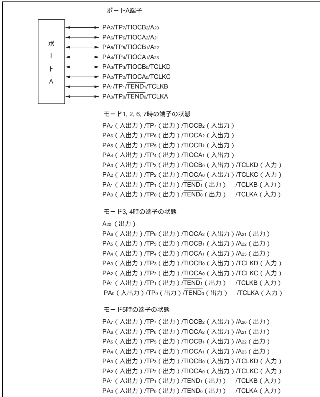
図 8.10 ポート A の端子構成
