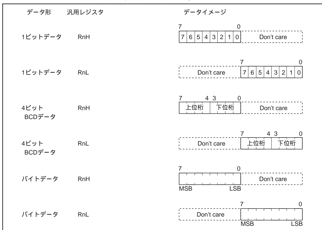
図 2.6 汎用レジスタのデータ構成 (1)
