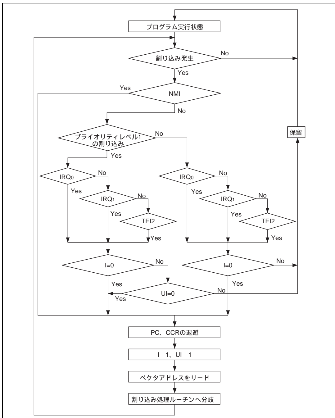
図 5.6 UE = 0 の場合の割り込み受け付けまでのフロー
