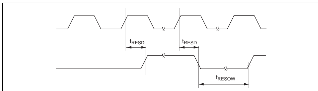
図 21.6 リセット出力タイミング*
