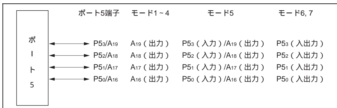
図 8.5 ポート 5 の端子構成
