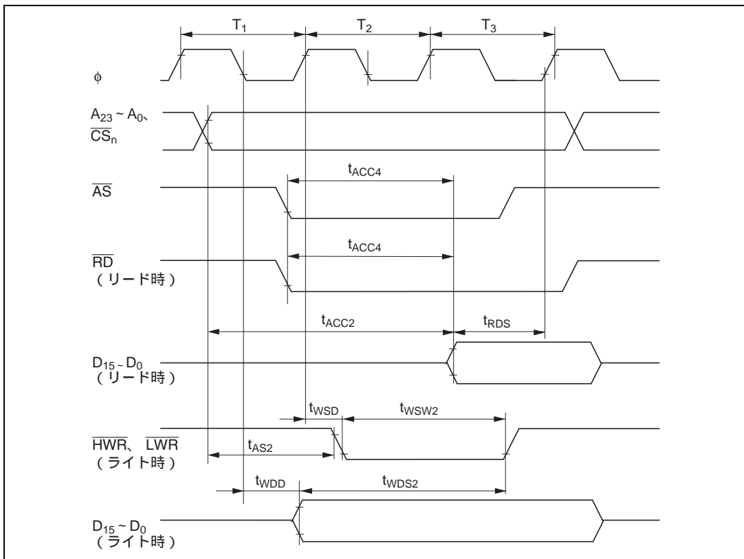
図 21.9 基本バスタイミング / 3 ステートアクセス
