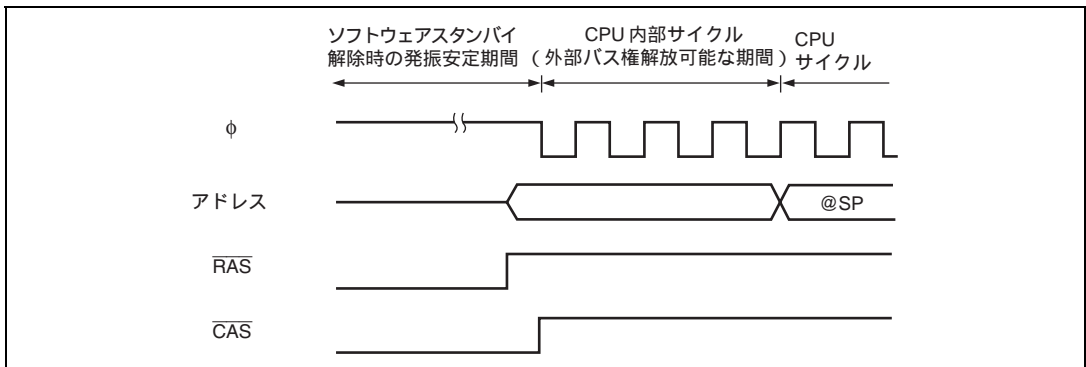
図 6.37 セルフリフレッシュの解除
