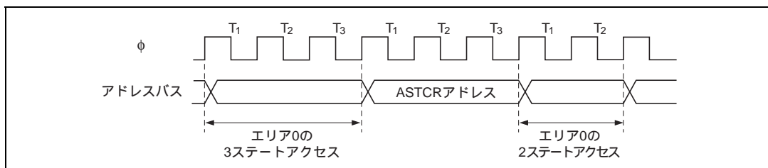
図 6.49 ASTCR ライトタイミング
