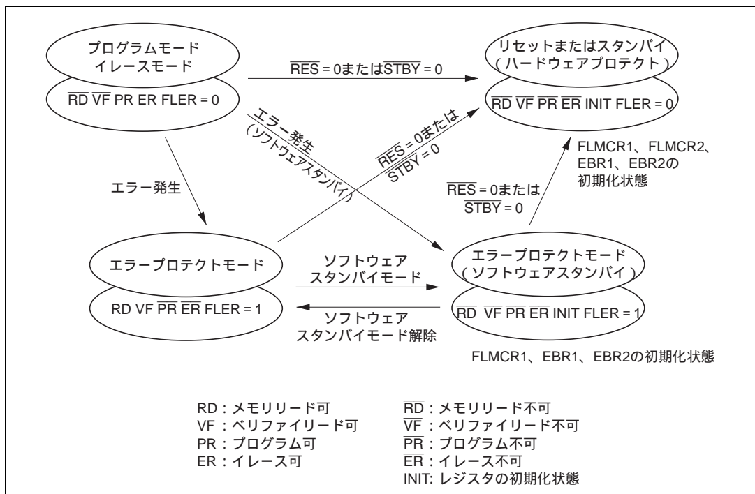
図 18.12 フラッシュメモリの状態遷移図 (モード 5、7 (内蔵 ROM が有効) で FWE 端子に High レベル印加時)
