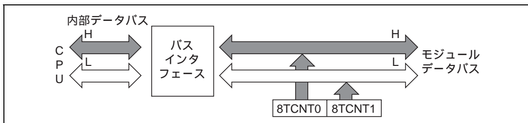
図 10.6 8TCNT0 のアクセス動作 [ 8TCNT0 CPU (上位バイト) ]
