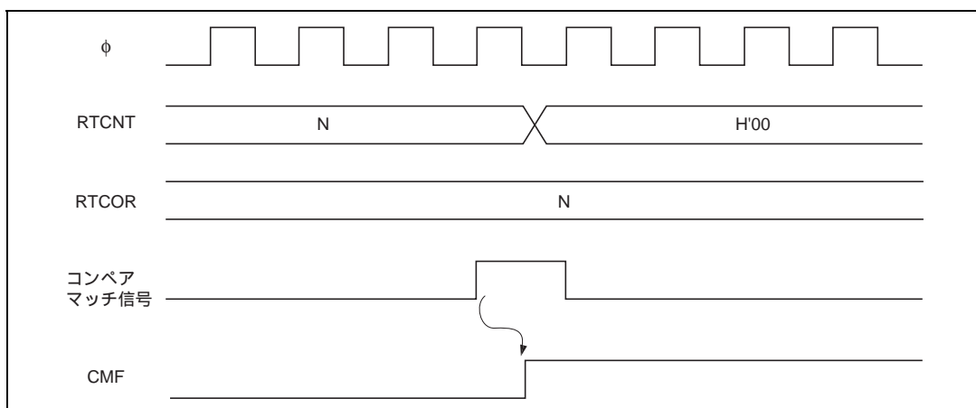
図 6.38 CMF フラグセットタイミング
