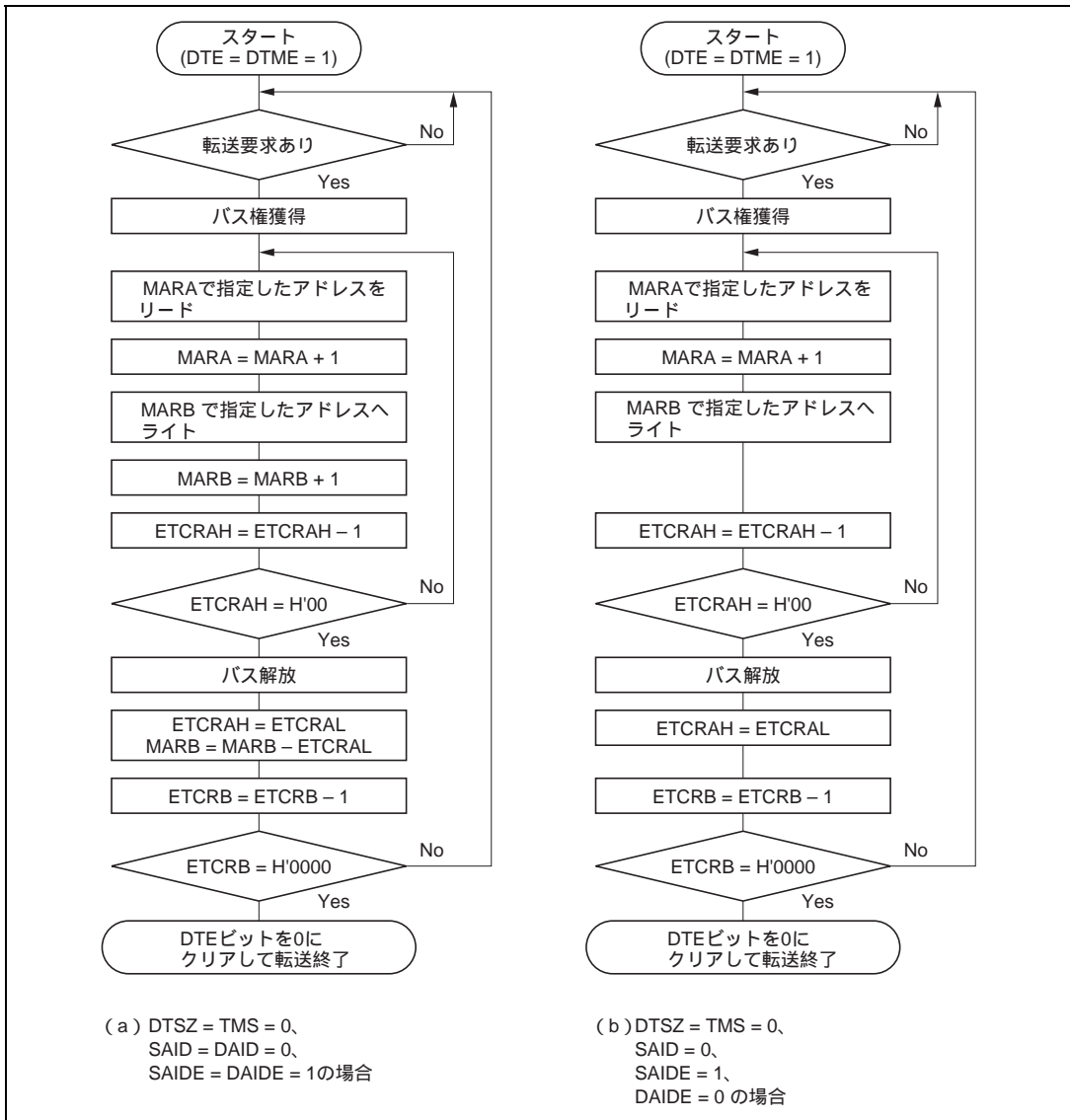
図 7.11 ブロック転送モードの動作フロー
