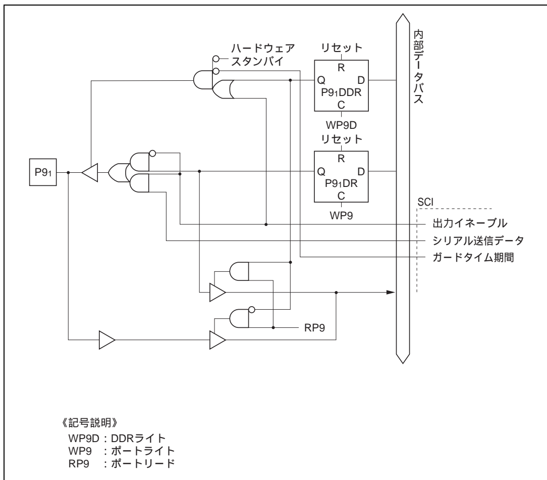
図 C.9 (b) ポート 9 ブロック図 (P9, 端子)
