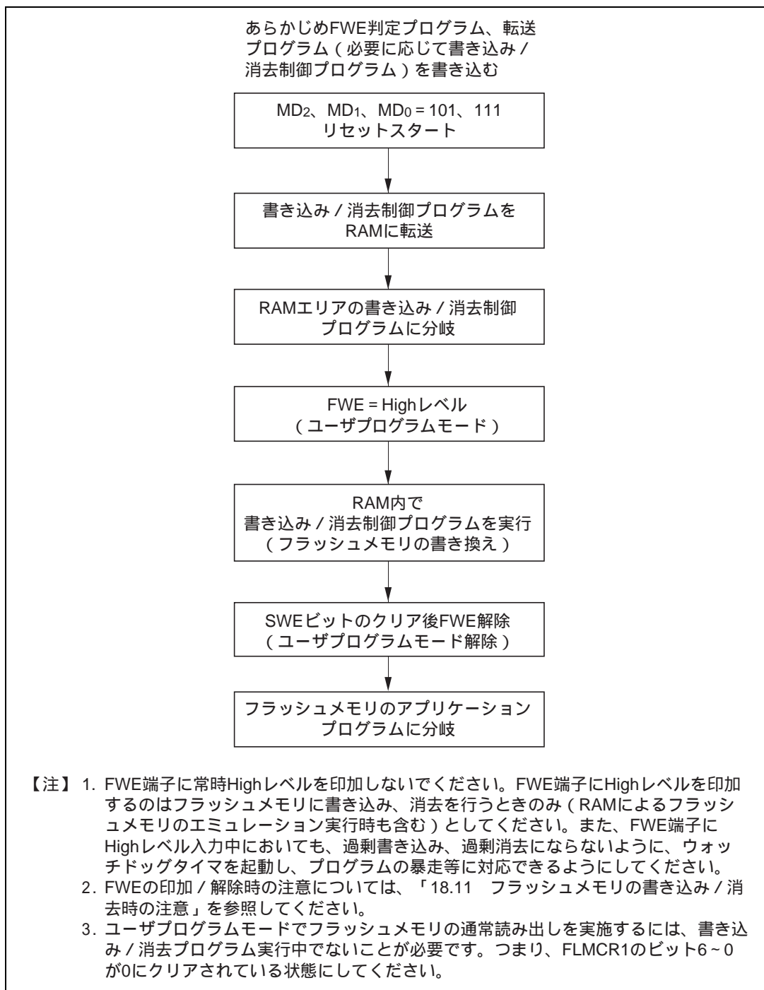
図 18.8 ユーザプログラムモードの実行手順例
