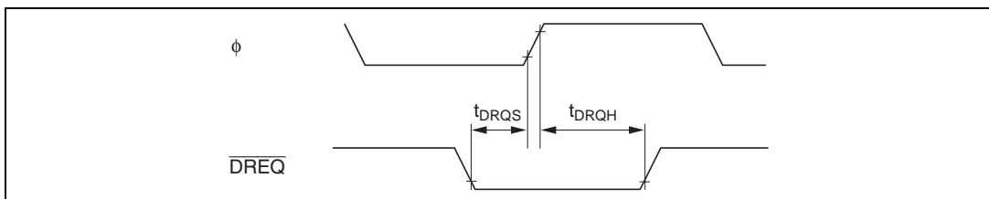
図 21.24 DMAC、 \overline{\text{DREQ}} 入力タイミング
