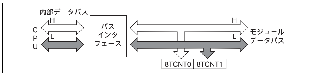
図 10.5 8TCNT1 のアクセス動作 [ CPU 8TCNT1 (下位バイト) ]
