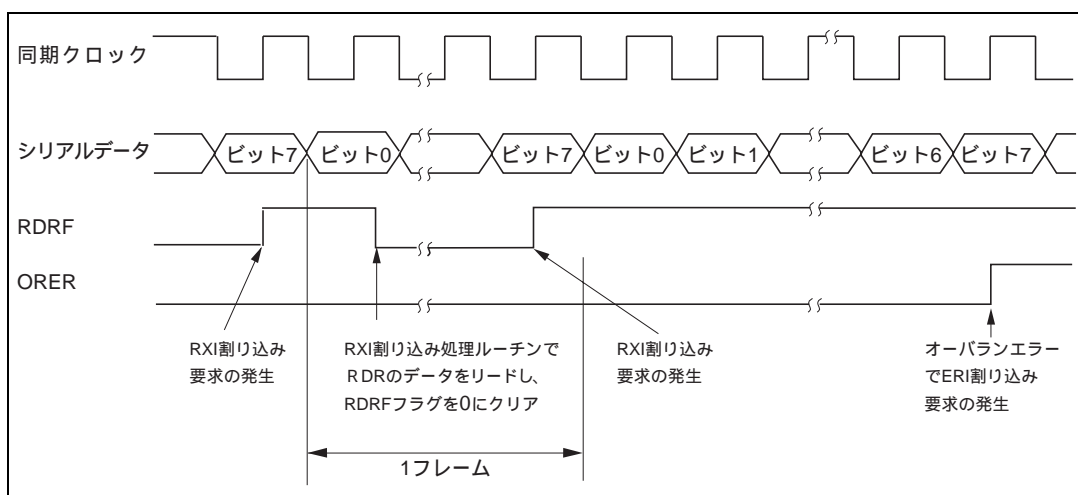
図 13.19 SCI の受信時の動作例
