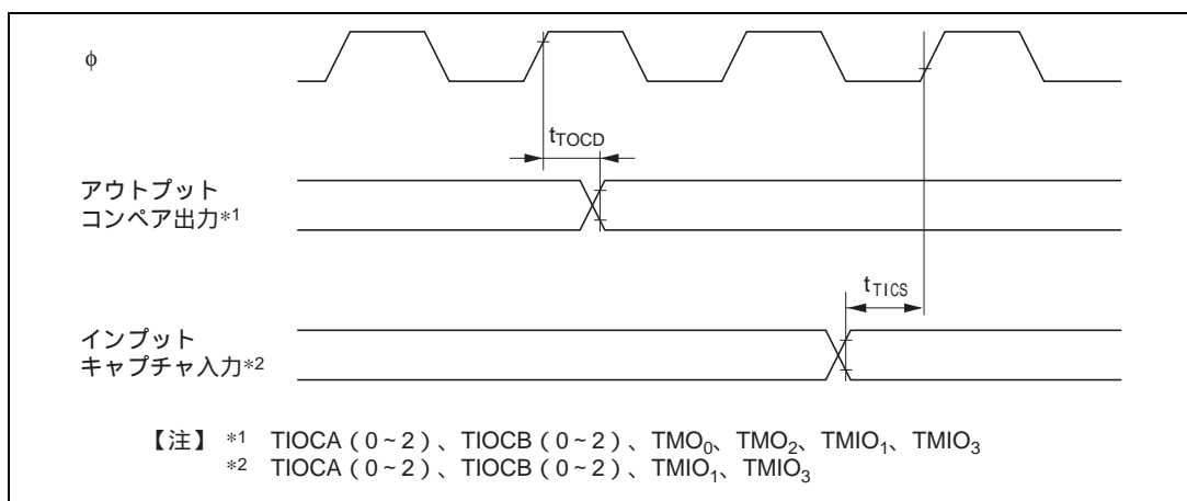
図 21.18 タイマ入出力タイミング
