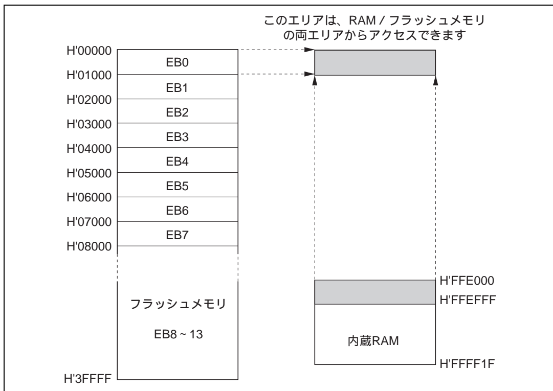
図 18.14 RAM のオーバーラップ動作例
