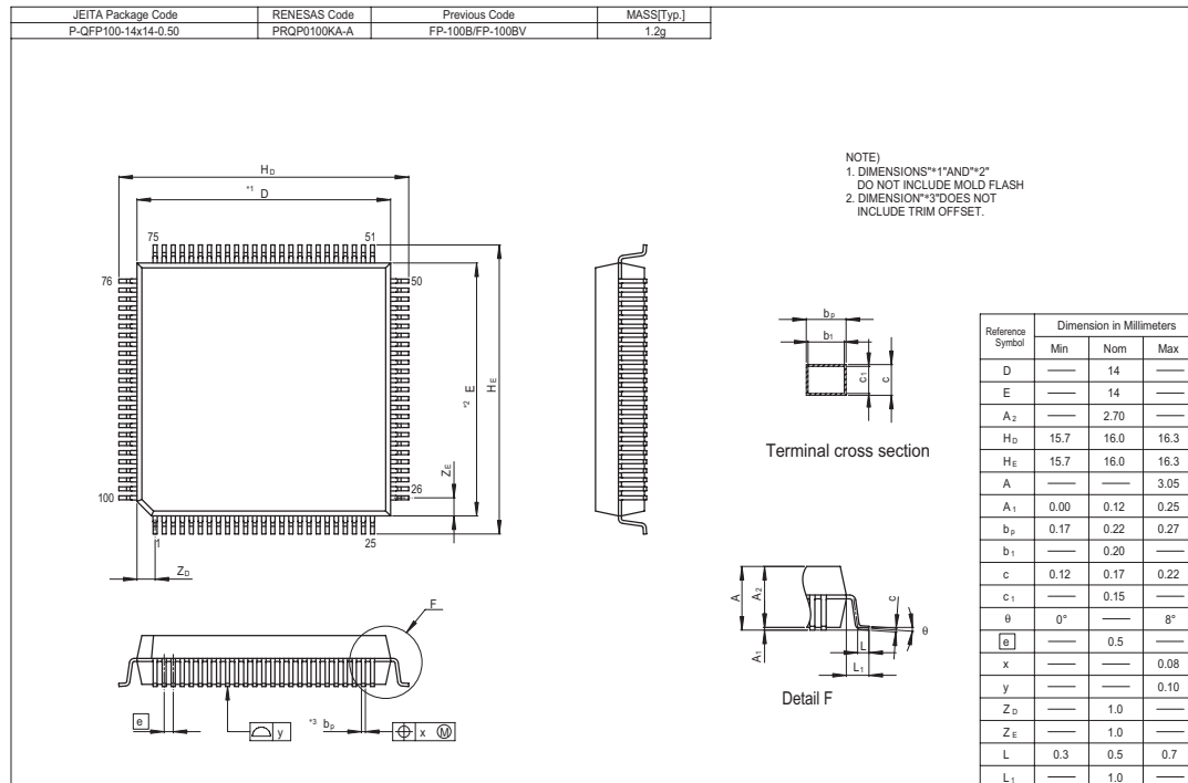
図 G.1 外形寸法図 (FP-100B) 単位 : mm
