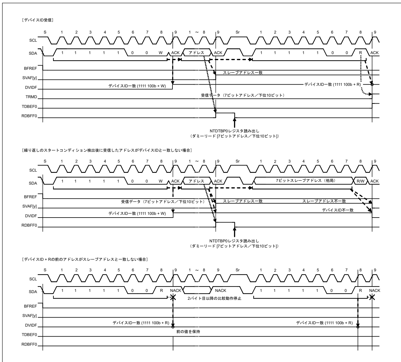
図 25.63 デバイス ID 受信時の SVAF[y]、DVIDF フラグのセット/クリアタイミング
