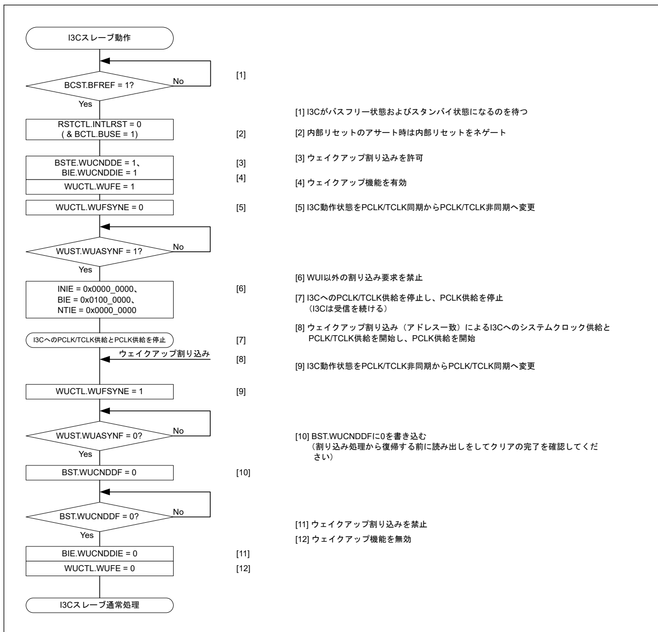
図 25.130 I3C スレーブウェイクアップの使用例 (スレーブアドレス一致に起因するウェイクアップ割り込みによるウェイクアップリカバリの場合)
