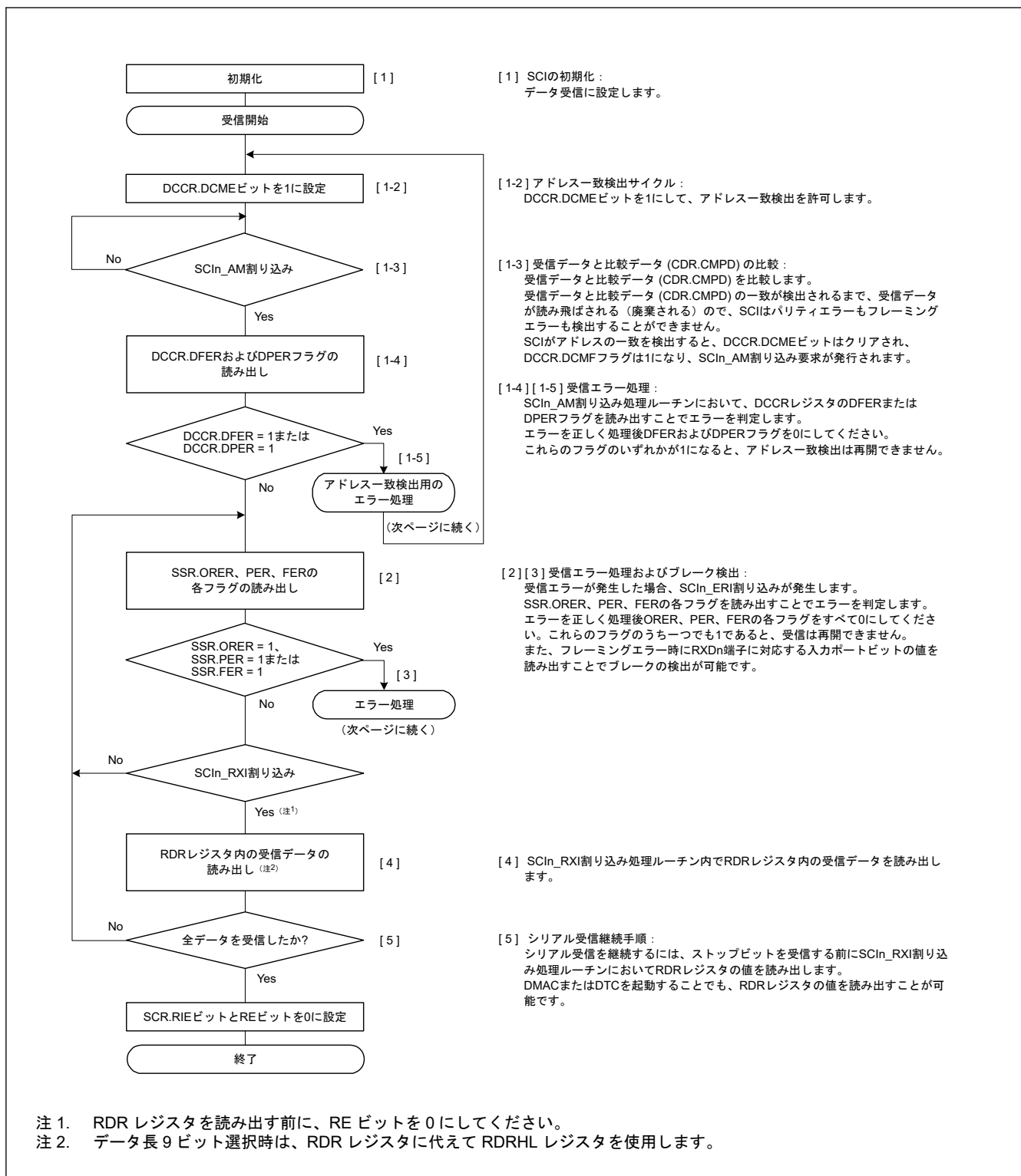
図 24.19 調歩同期式モードにおけるシリアル受信のフローチャート例（非 FIFO 選択、アドレス一致検出有効時） (1)
