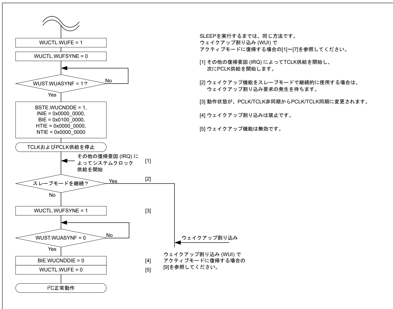
図 25.100 ノーマル WU モード 1 および 2 の使用例 (他のリカバリ要因 (IRQ) によるウェイクアップリカバリの場合)
