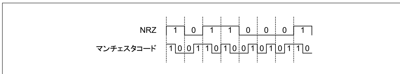
図 24.46 マンチェスタエンコードの例
