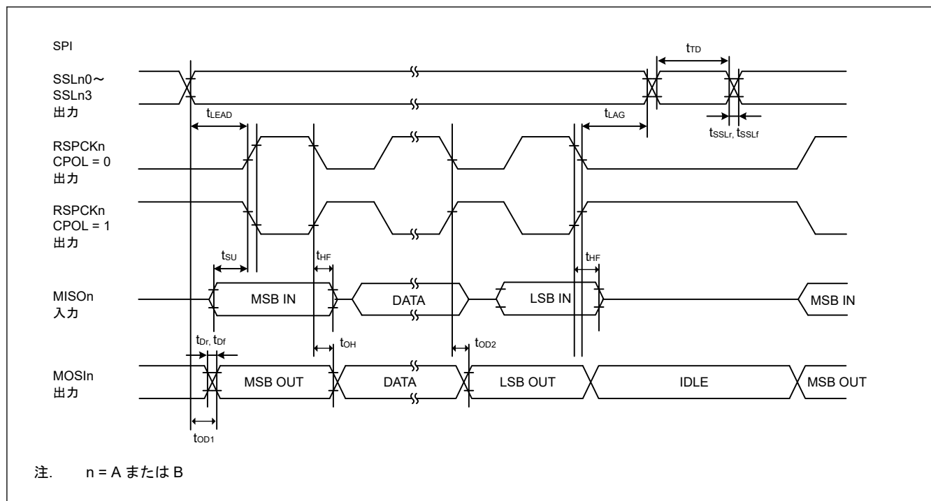
図 41.36 CPHA = 0 で、PCLKA/2 にビットレートが設定されている場合におけるマスタの SPI タイミング
