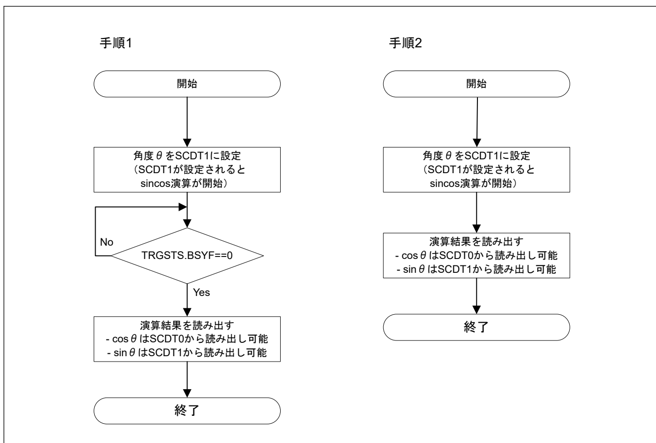
図 30.3 TFU の使用手順 (sincos 演算)
