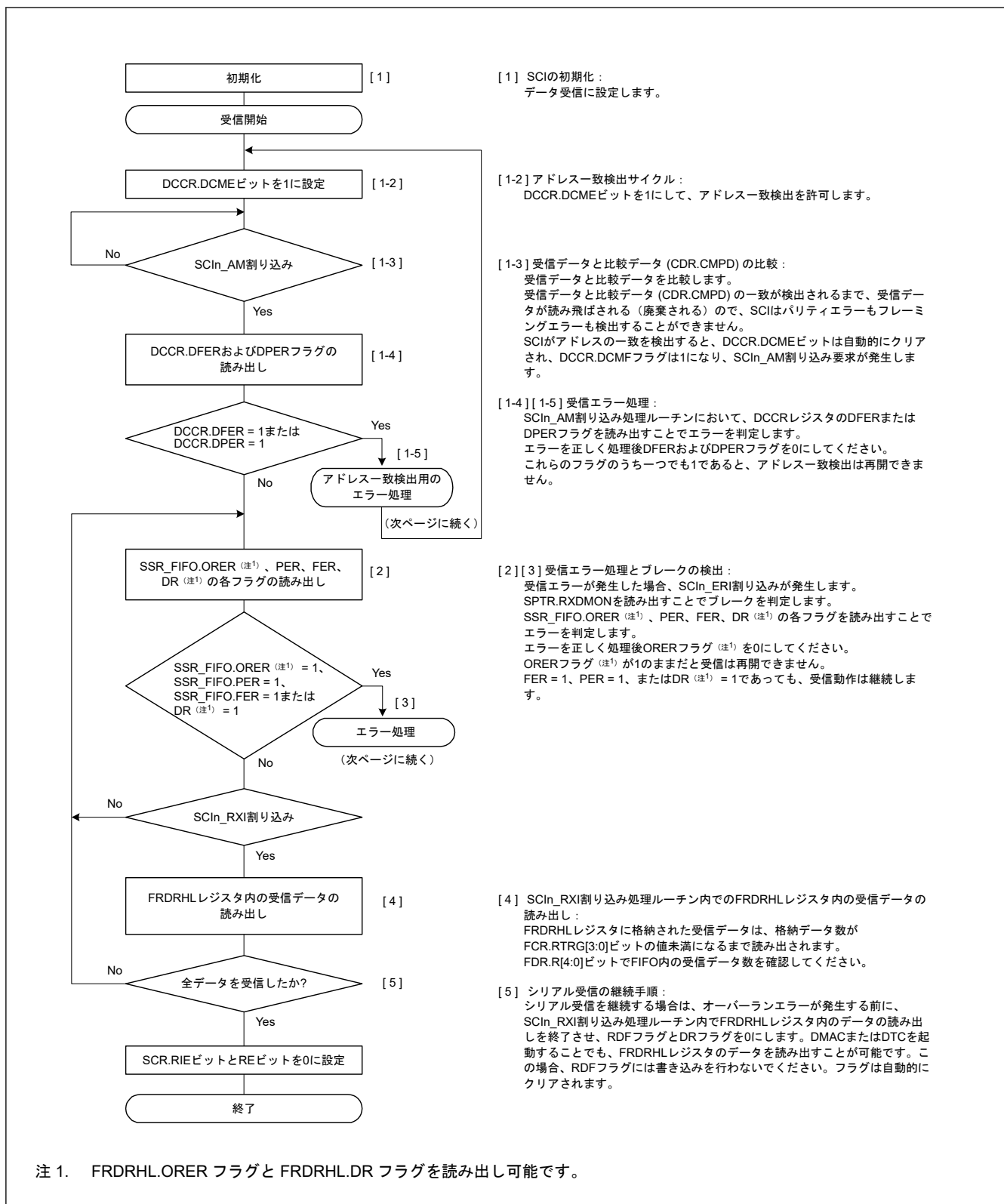
図 24.25 調歩同期式モードにおけるシリアル受信のフローチャート例 (FIFO 選択、アドレス一致検出有効時) (1)
