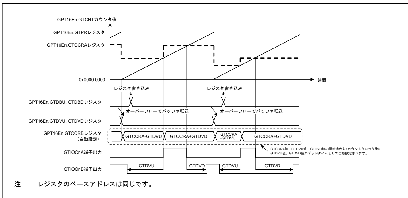
図 20.27 デッドタイム自動設定機能の動作例 (のこぎり波ワンショットパルスモード、アップカウント、GTDVU/GTDVD レジスタはバッファ動作、アクティブ High の場合)
