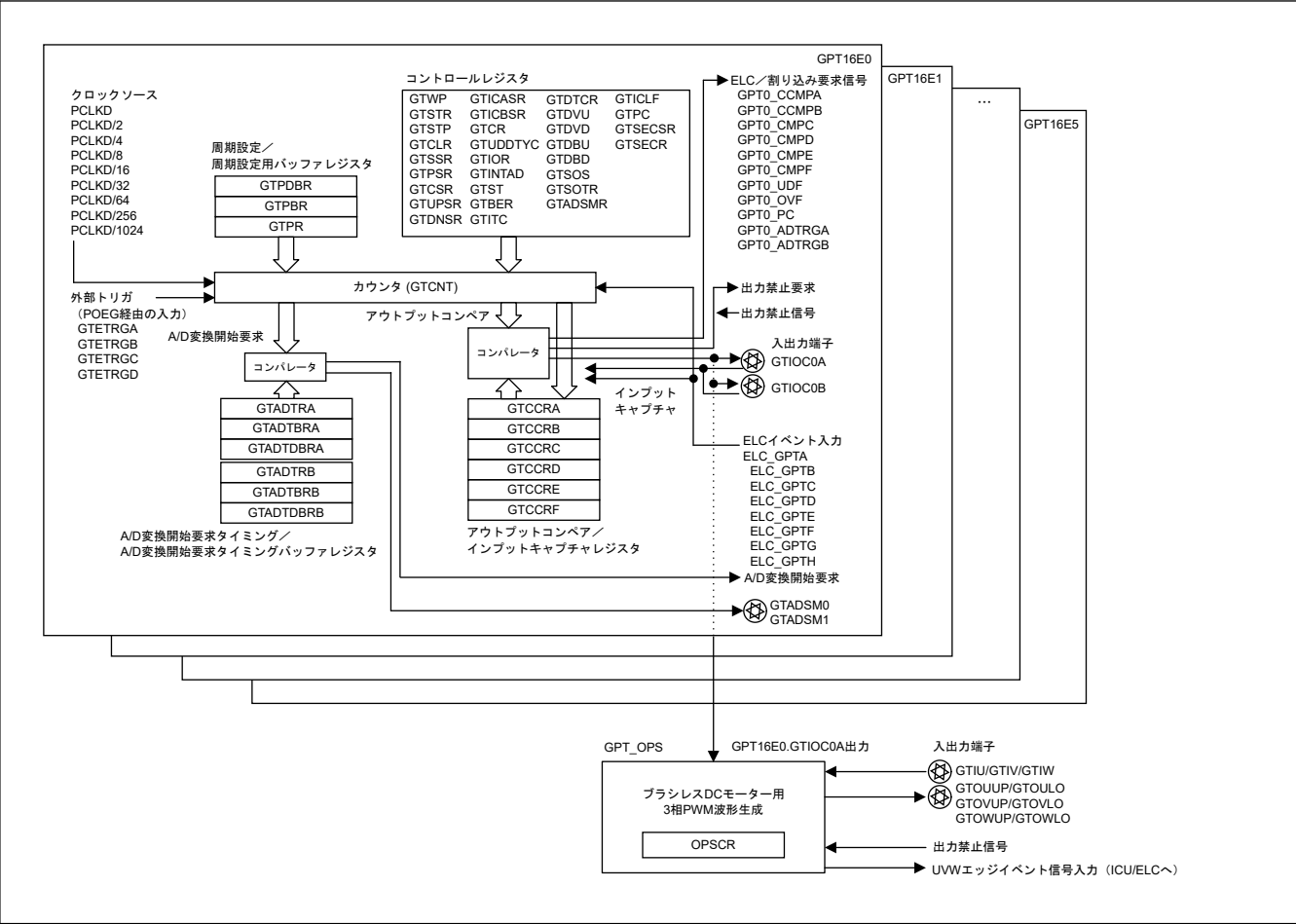
図 20.1 GPT のブロック図
