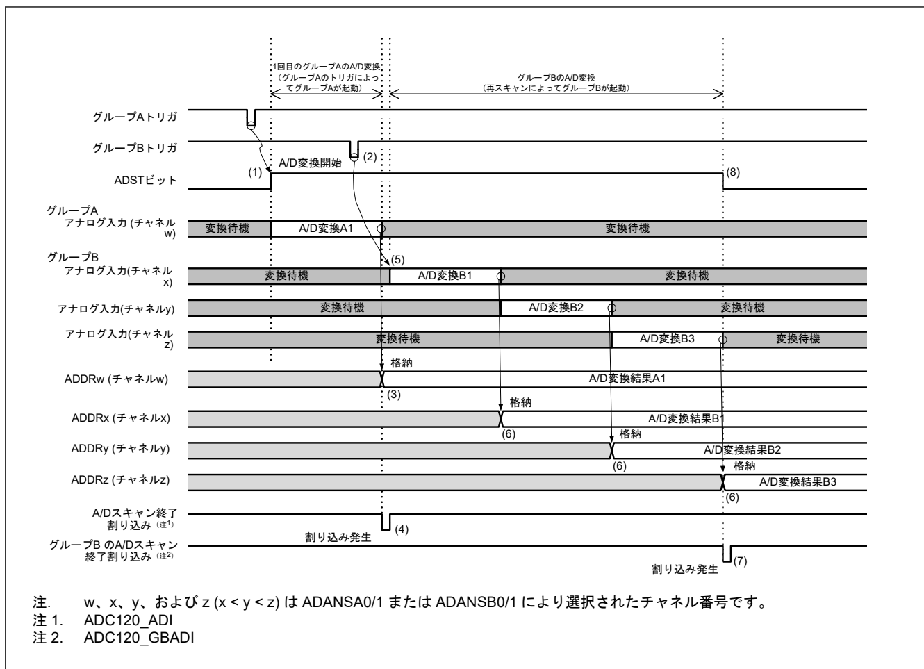
図 32.28 グループ優先動作の例 1-3：グループ A スキャン中のグループ B トリガ入力、再スキャンあり (ADGSPCR.GBRSCN = 1、ADGSPCR.GBRP = 0、および ADGSPCR.LGRRS = 0 の場合)
