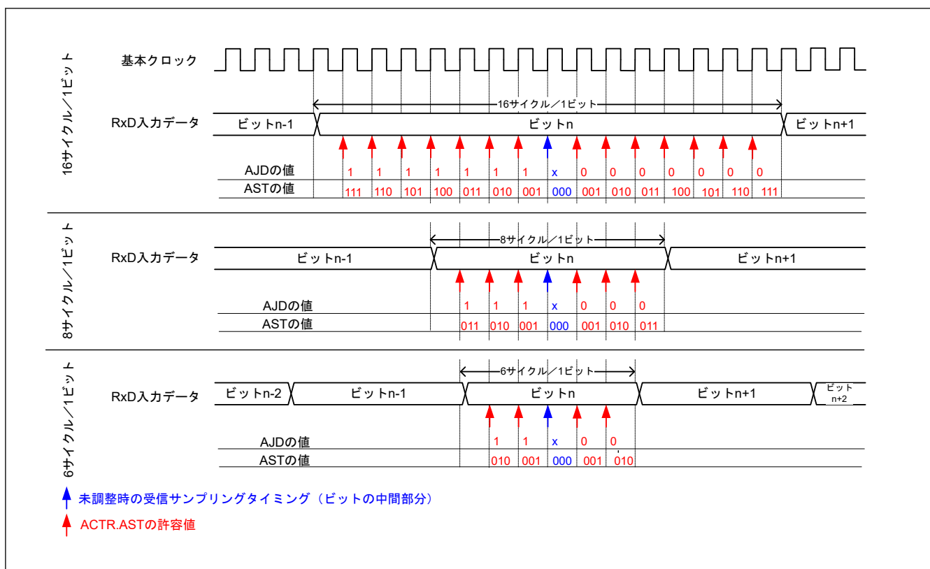
図 24.31 受信サンプリングタイミングの調整動作の概要（内部クロックを使用した調歩同期式モード）
