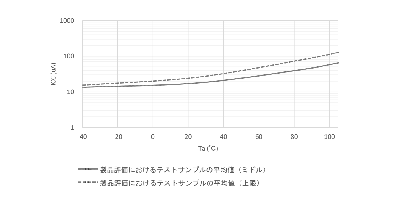
図 41.3 ディープソフトウェアスタンバイモード時の温度依存性、DPSBYCR.DEEPCUT[1:0] = 00b (参考データ)
