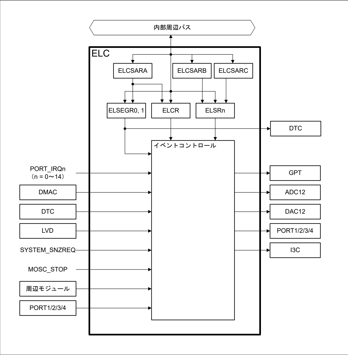
図 17.1 ELC のブロック図
