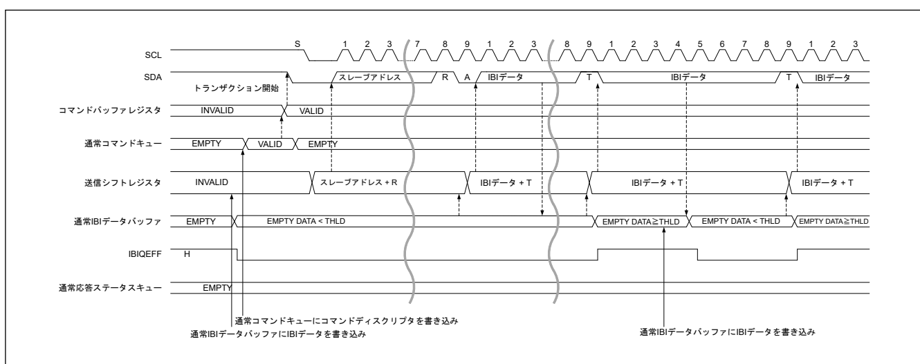
図 25.43 I3C スレーブ IBI 転送タイミング (1/2)
