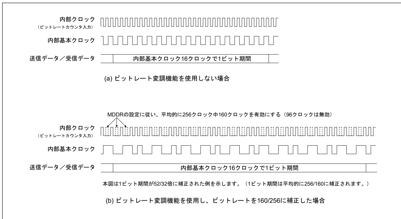
図 24.97 ビットレート変調機能使用時の内部基本クロックの例
