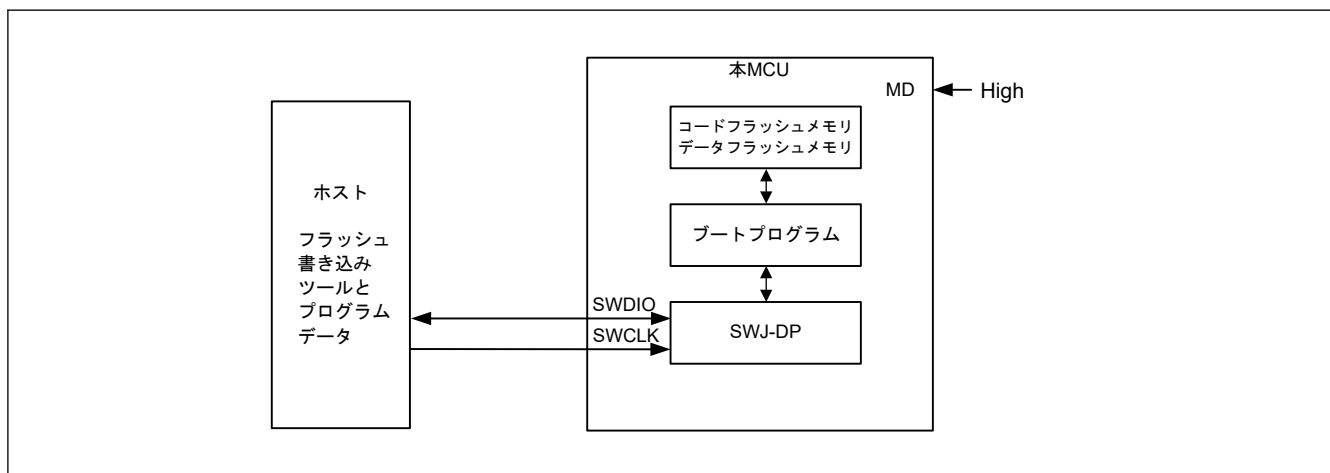
図 38.38 フラッシュメモリ関連モジュールのブロック図
