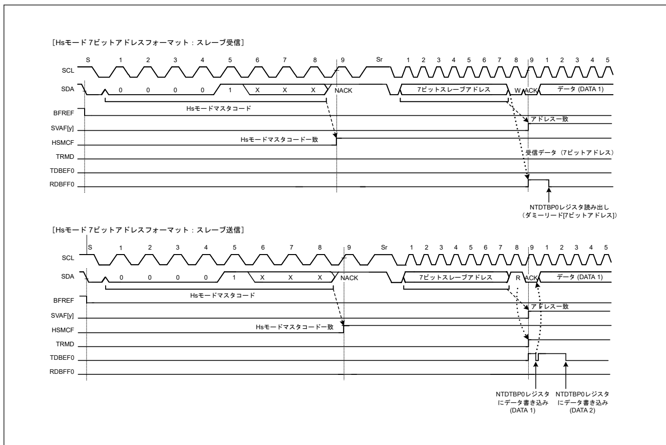
図 25.65 Hs モードマスタコード受信時に SVAf[y]、HSMCF フラグが1になるタイミング
