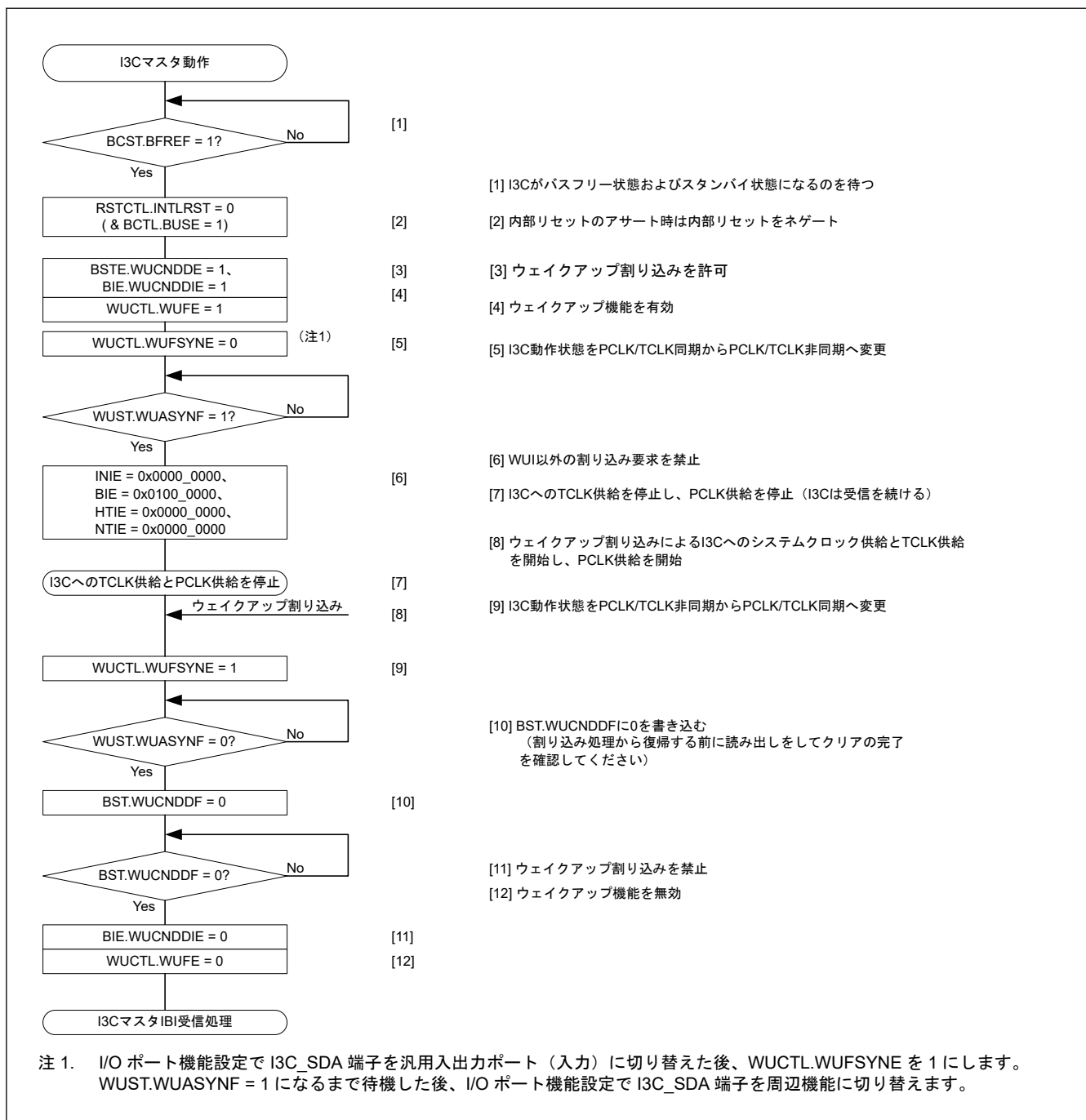
図 25.124 I3C マスタウェイクアップの使用例
