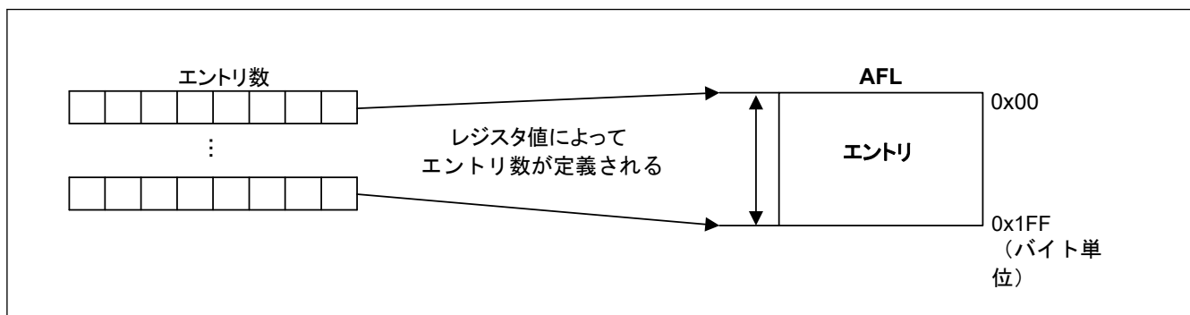
図 26.24 各チャンネルの AFL の構成
