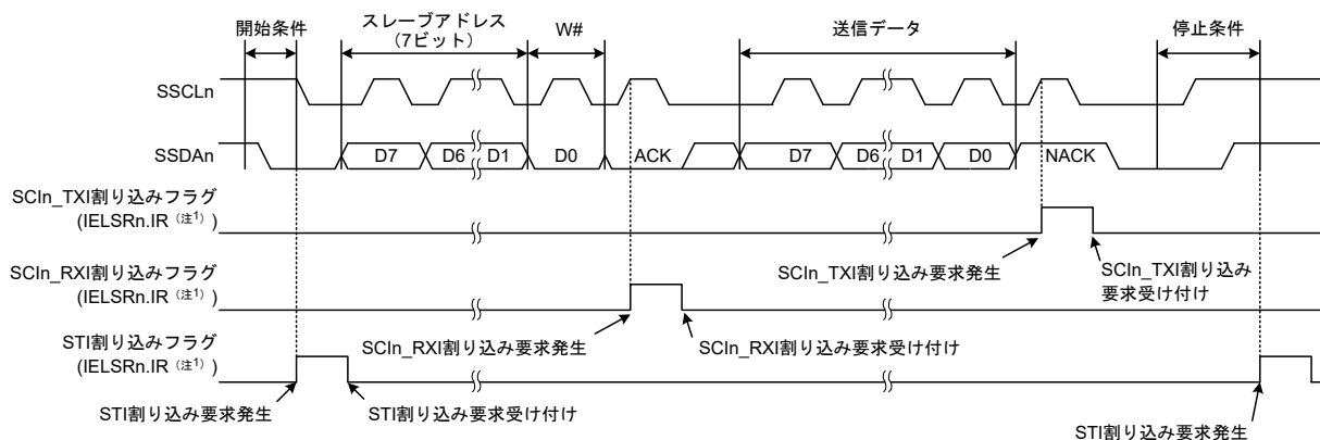
図 24.91 簡易 IIC モードにおけるマスタ送信の動作例 2 (7 ビットスレーブアドレス、ACK 割り込み、NACK 割り込み使用時)
