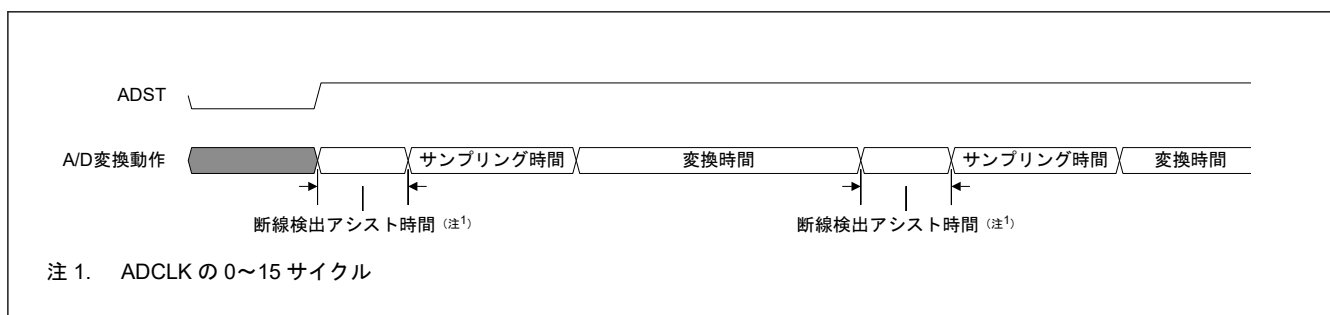
図 32.36 断線検出アシスト機能を使用した場合の A/D 変換動作図
