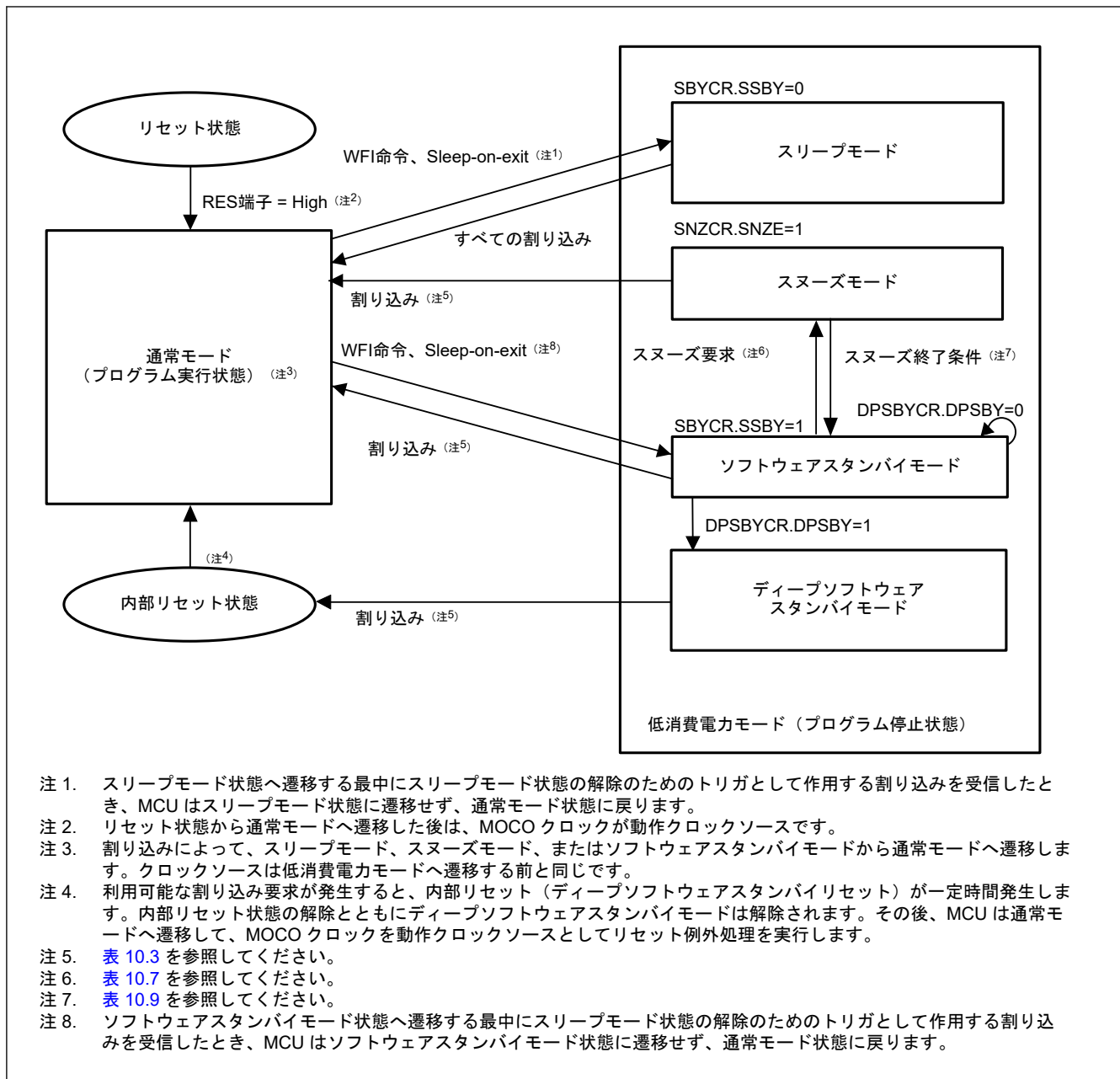
図 10.1 モード遷移
