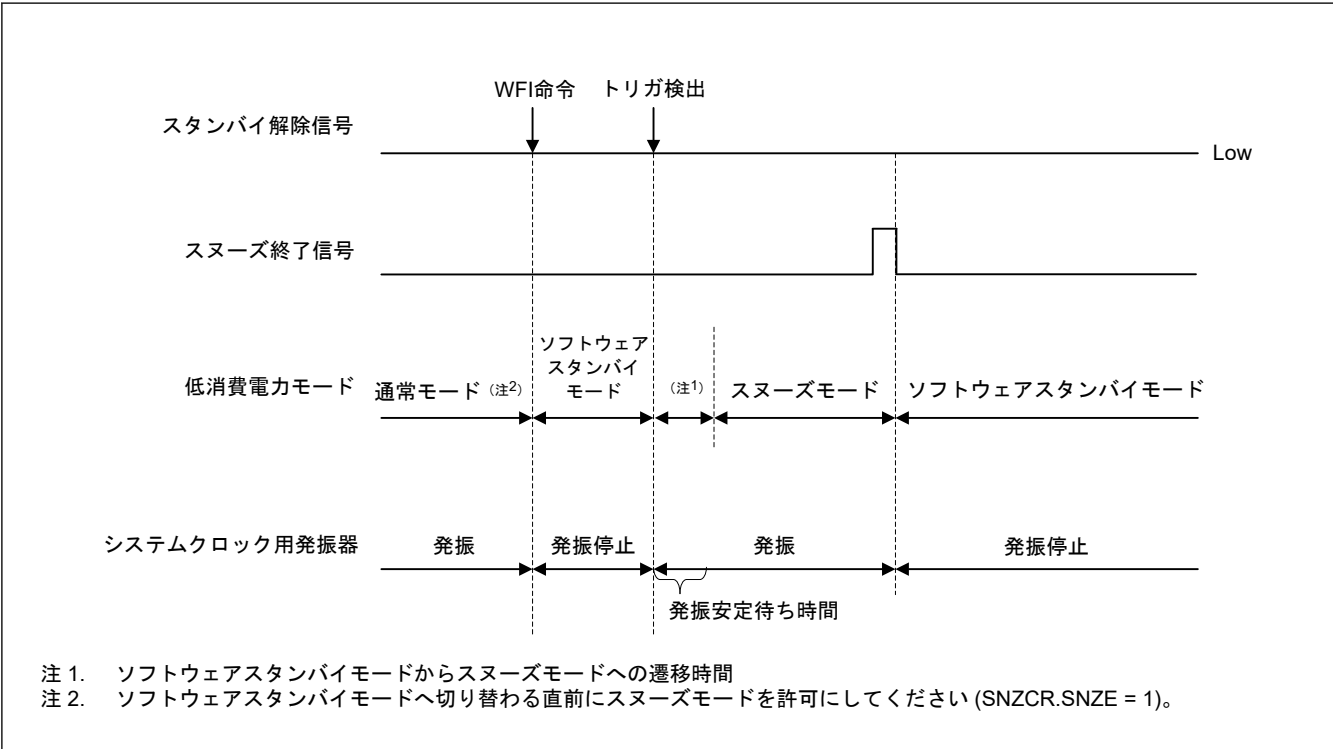
図 10.5 割り込み要求信号が発生しない場合のスヌーズモードの解除
