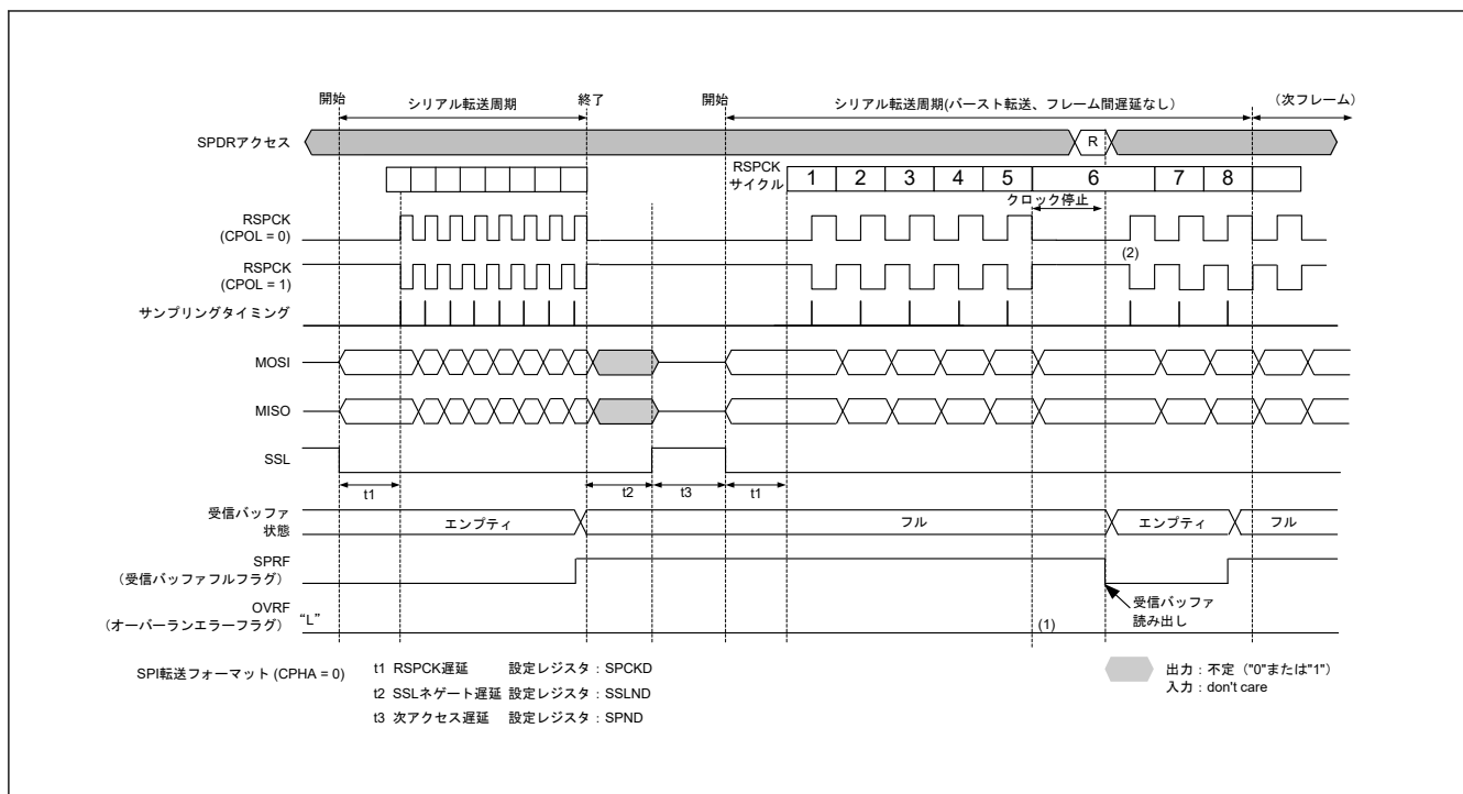
図 28.41 マスタモードの受信バッファフル状態でシリアル転送が継続する場合のクロック停止波形(パースト転送でフレーム間遅延なし、CPHA = 0)
