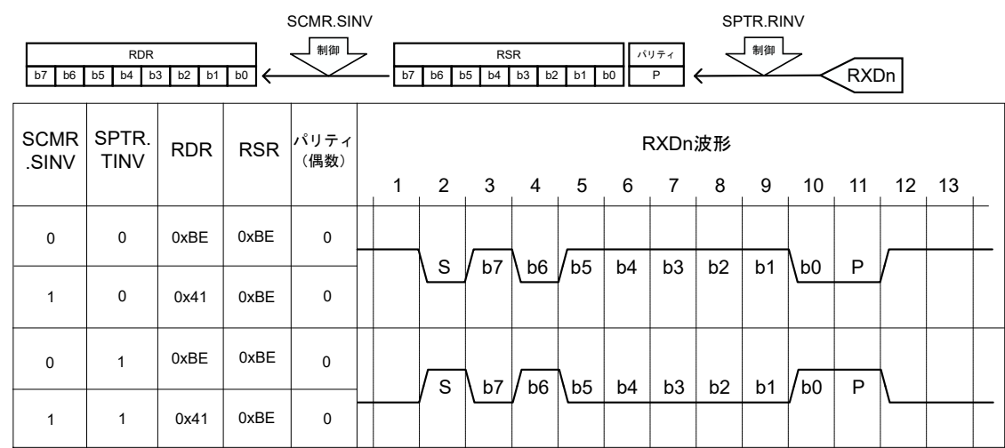
図 24.2 受信/送信データ制御の例
