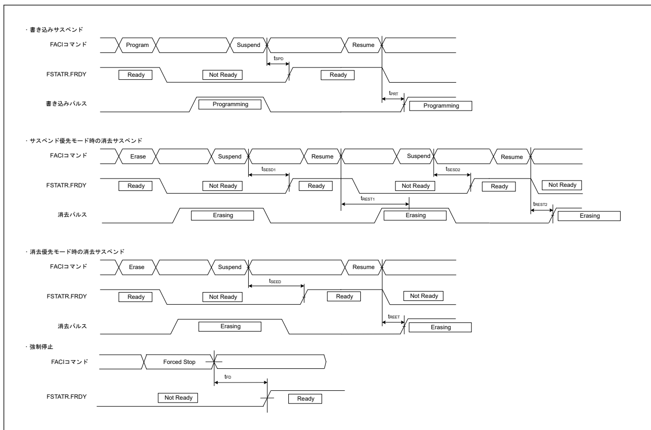
図 41.59 フラッシュメモリのプログラム／イレースのサスペンドタイミングと強制停止タイミング
