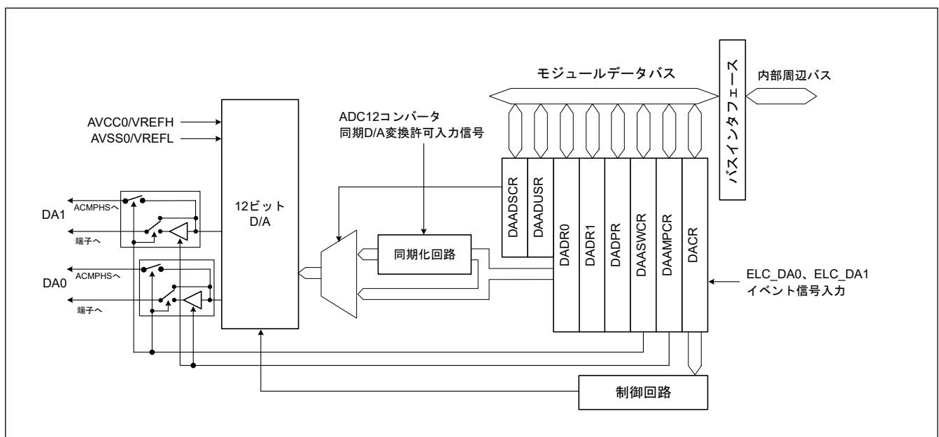
図 33.1 DAC12 のブロック図
