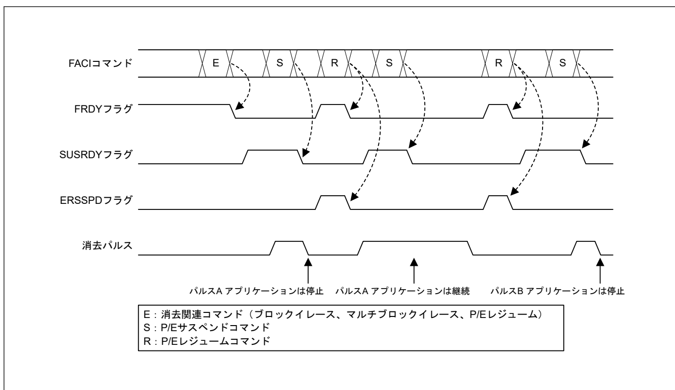
図 38.18 消去中のサスペンド（サスペンド優先モード）
