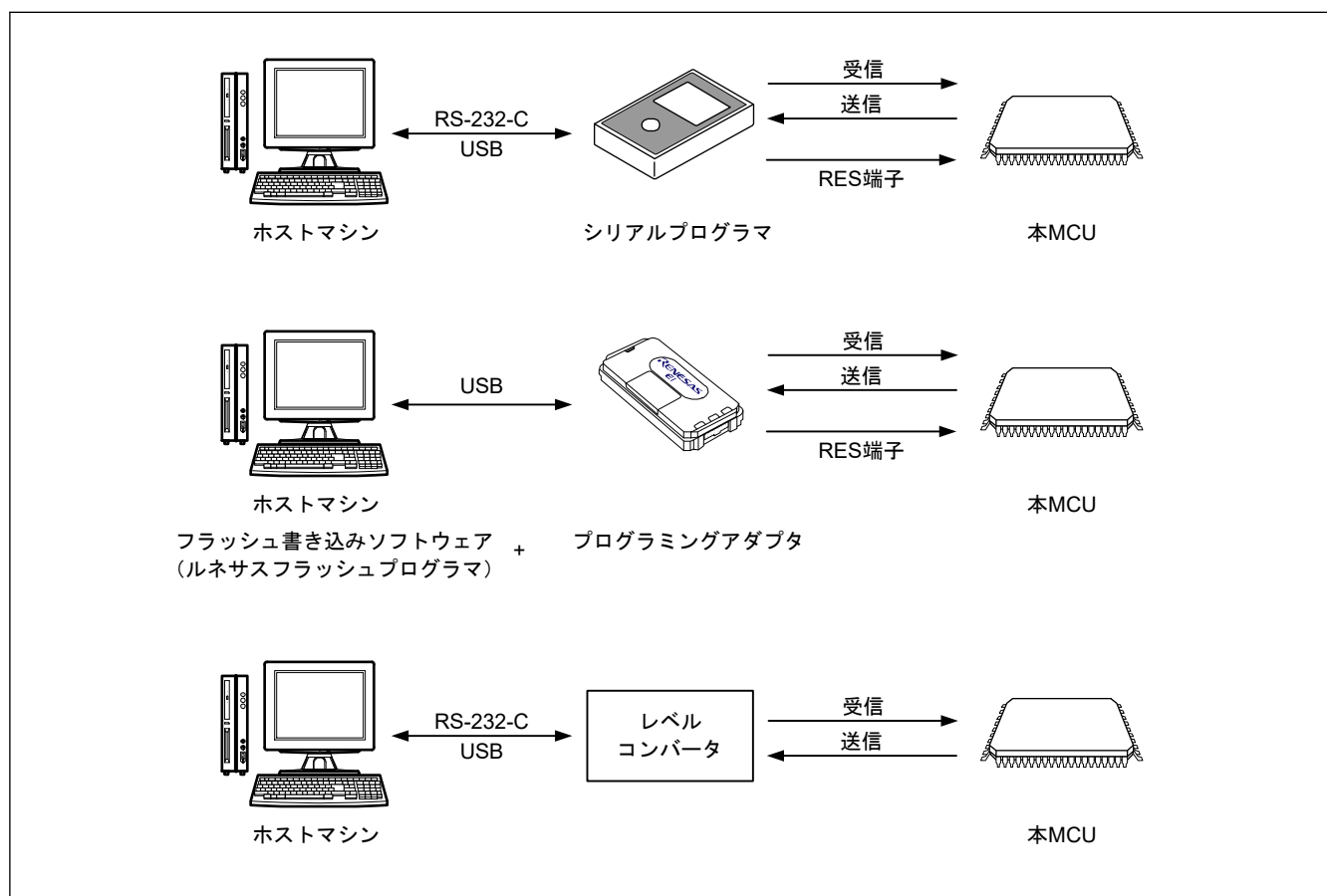
図 38.39 フラッシュメモリを書き換えるための環境
