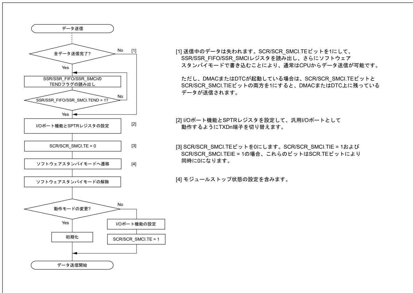
図 24.99 送信中にソフトウェアスタンバイモードへ遷移する場合のフローチャート例
