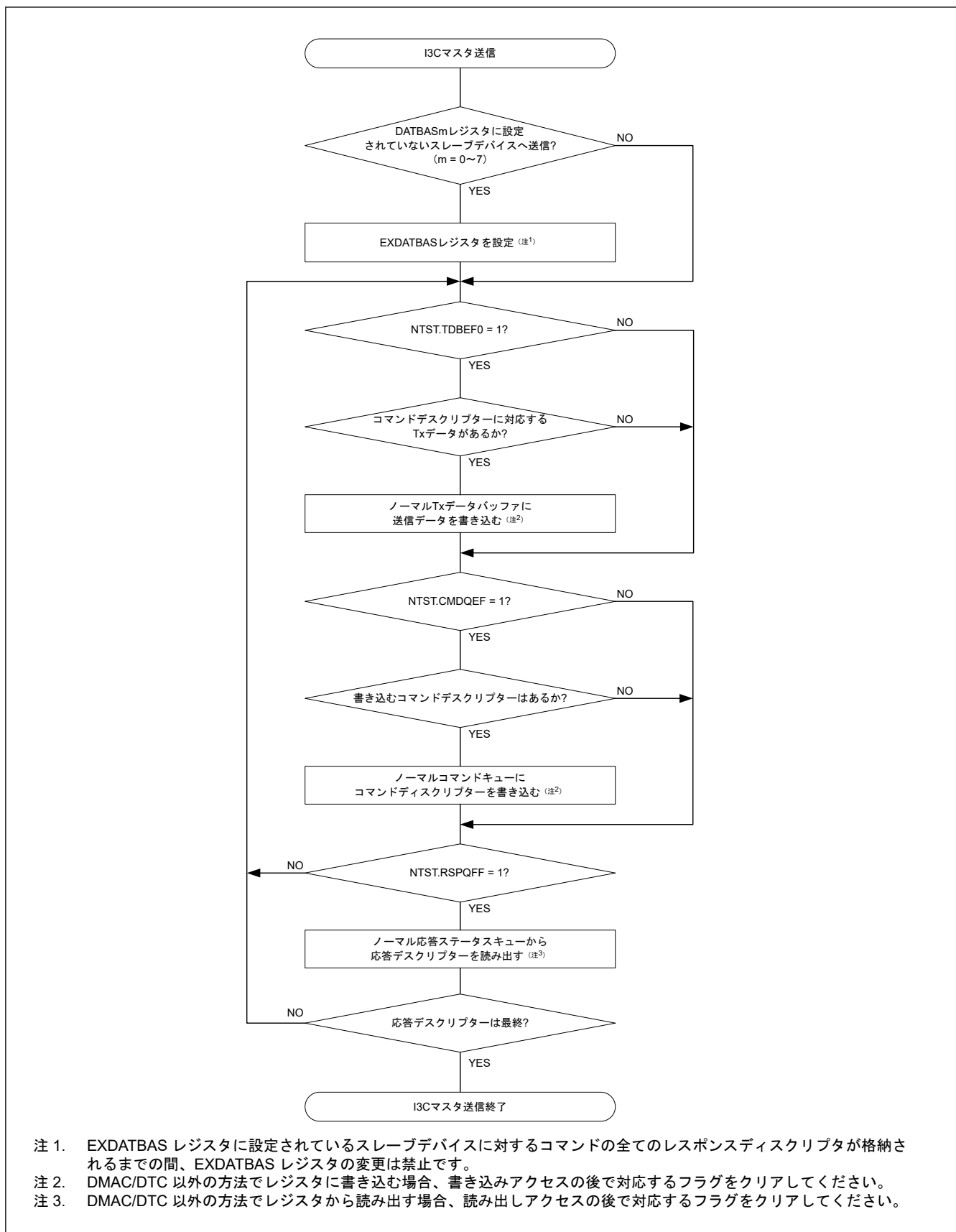
図 25.119 I3C マスタ送信のフローチャート例 (通常 FIFO バッファ転送)
