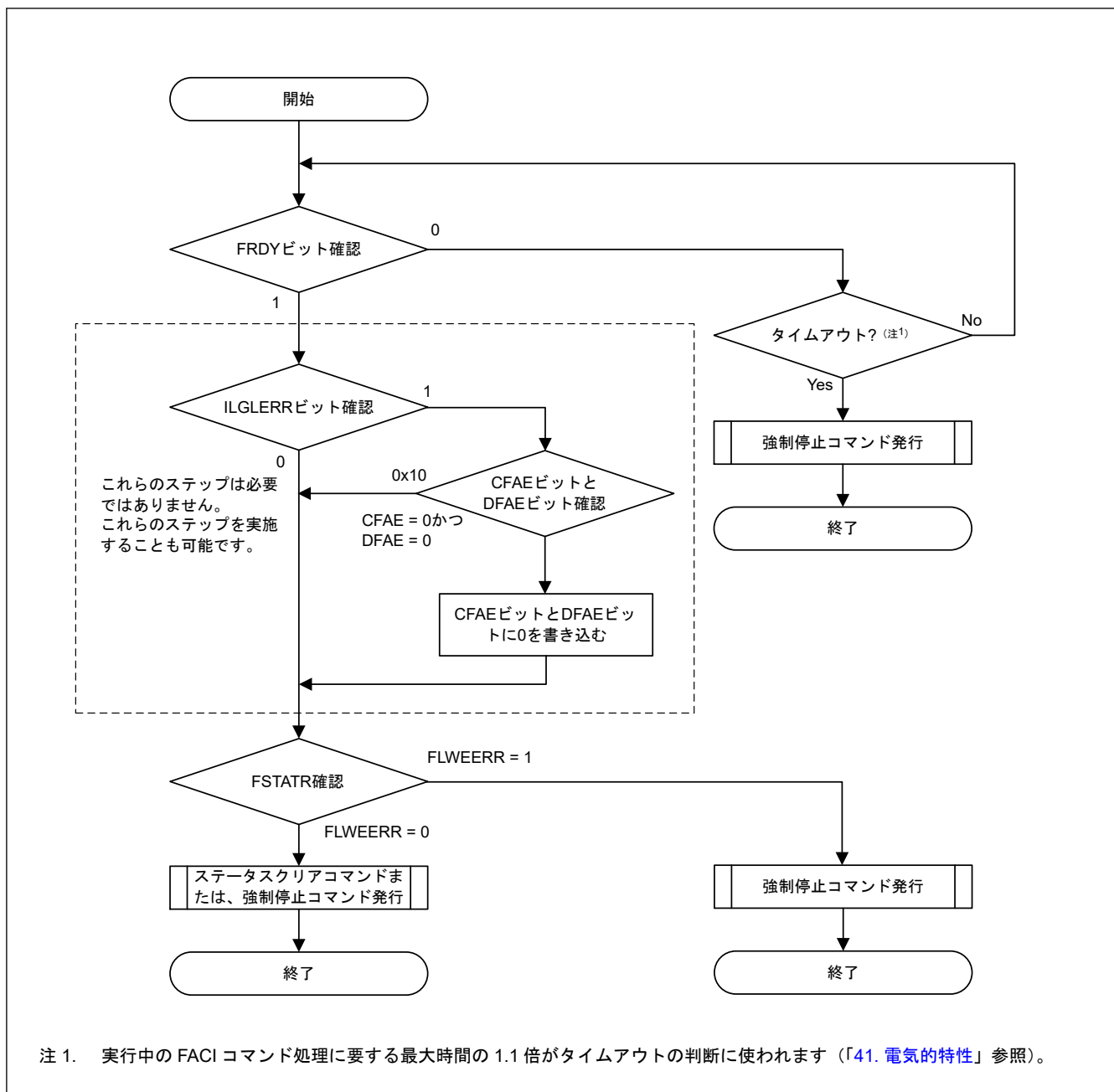
図 38.12 コマンドロック状態からの復帰フロー
