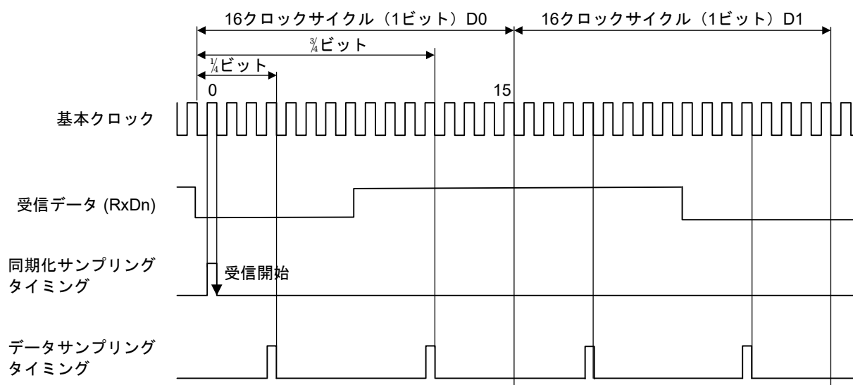
図 24.56 マンチェスタモードでのデータ受信サンプリングタイミング
