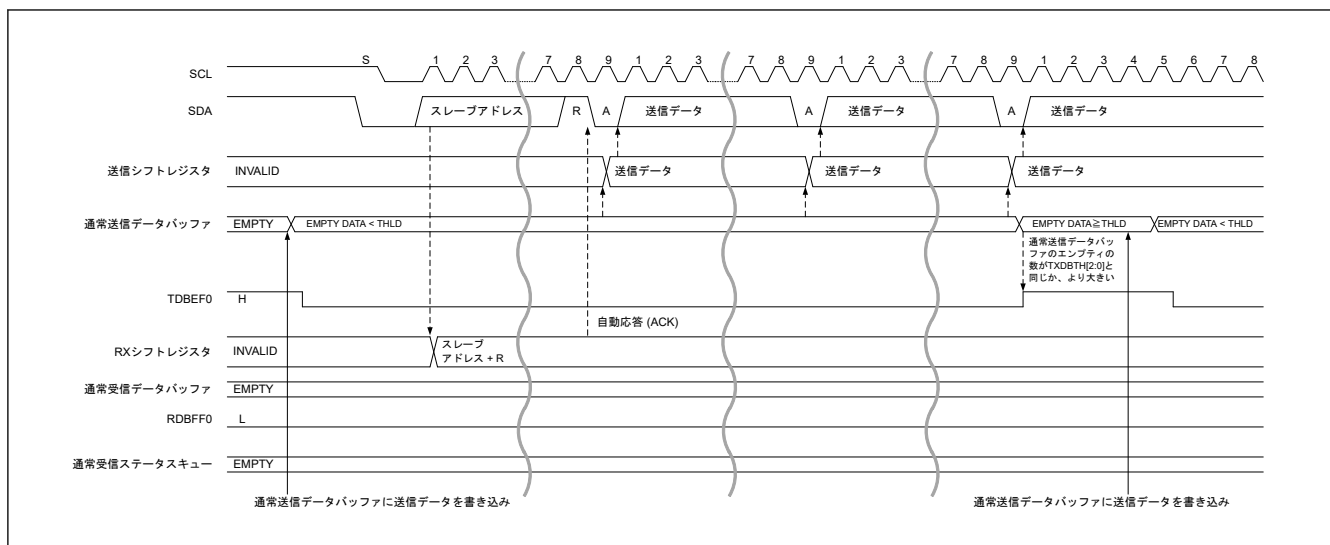
図 25.41 レガシー I2C メッセージデータ読み出し転送タイミング (1/2)
