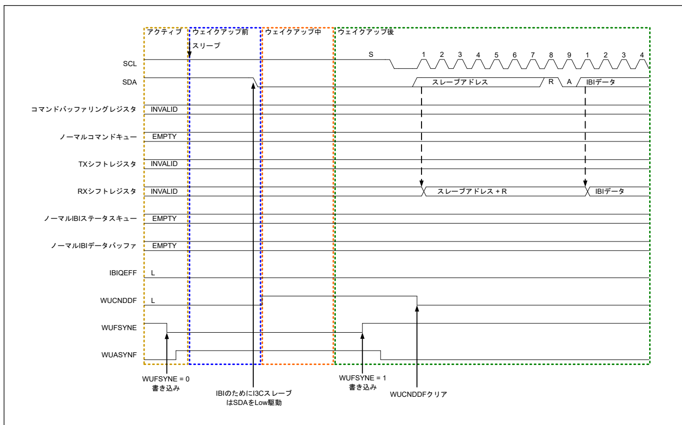
図 25.107 I3C マスタウェイクアップ動作
