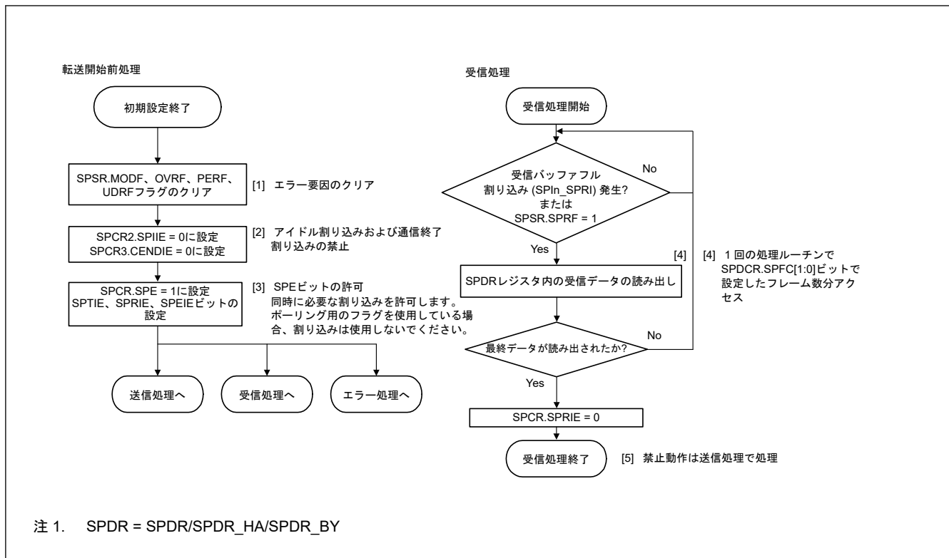
図 28.50 マスタモードでの受信フロー
