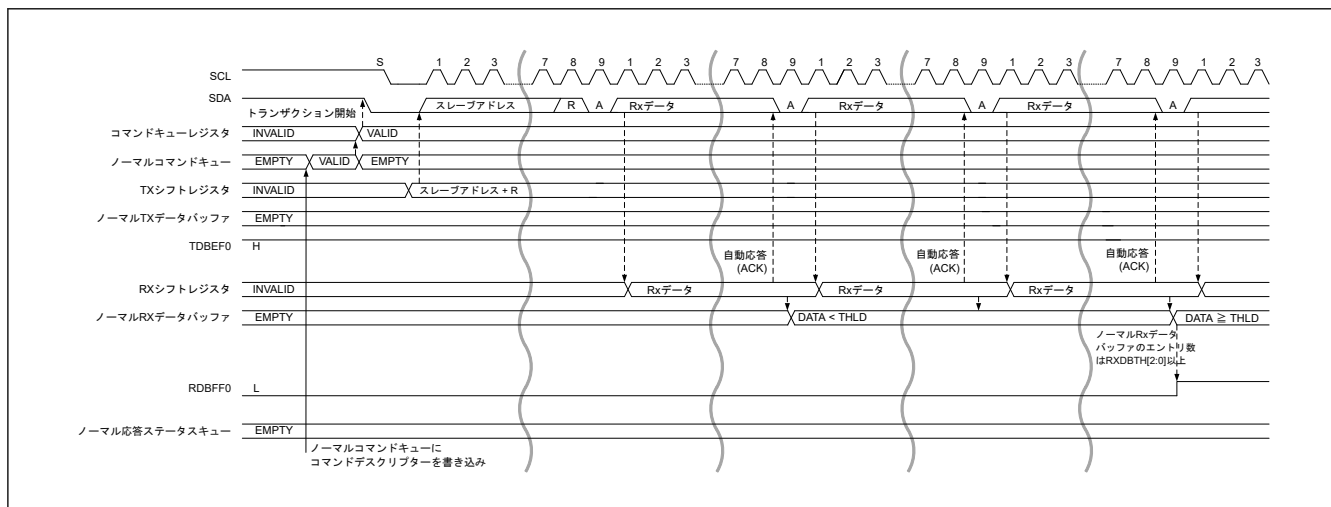
図 25.20 SDR データ読み出し転送タイミング (1/2)
