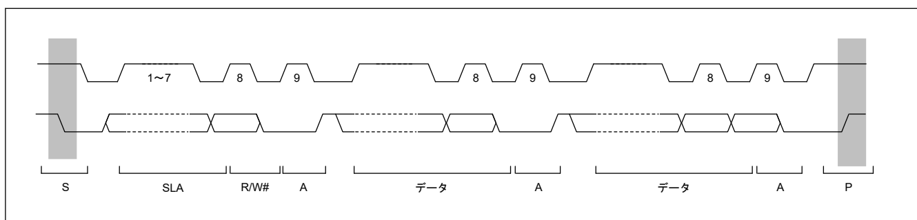
図 25.50 I 2 C バスタイミング (SLA = 7 ビットの場合)
