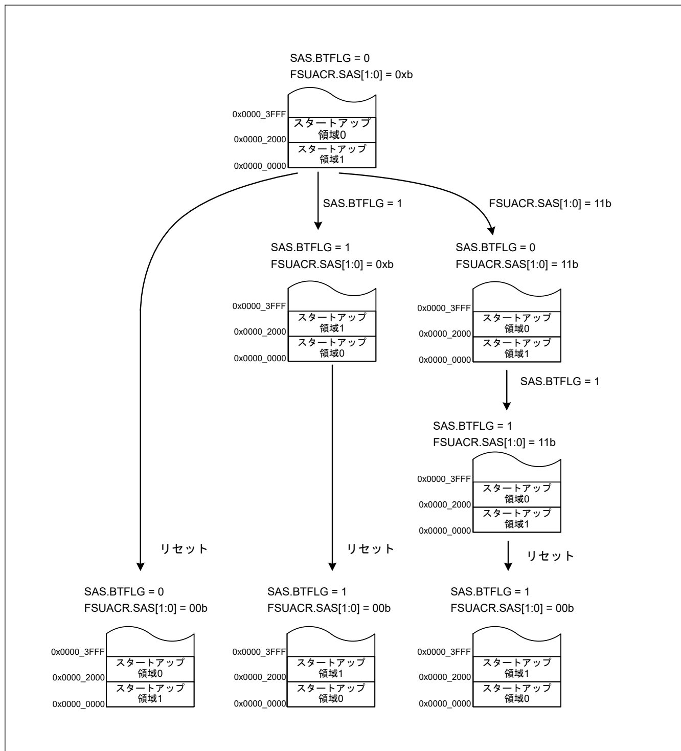
図 38.27 スタートアッププログラムプロテクション設定の遷移例 2
