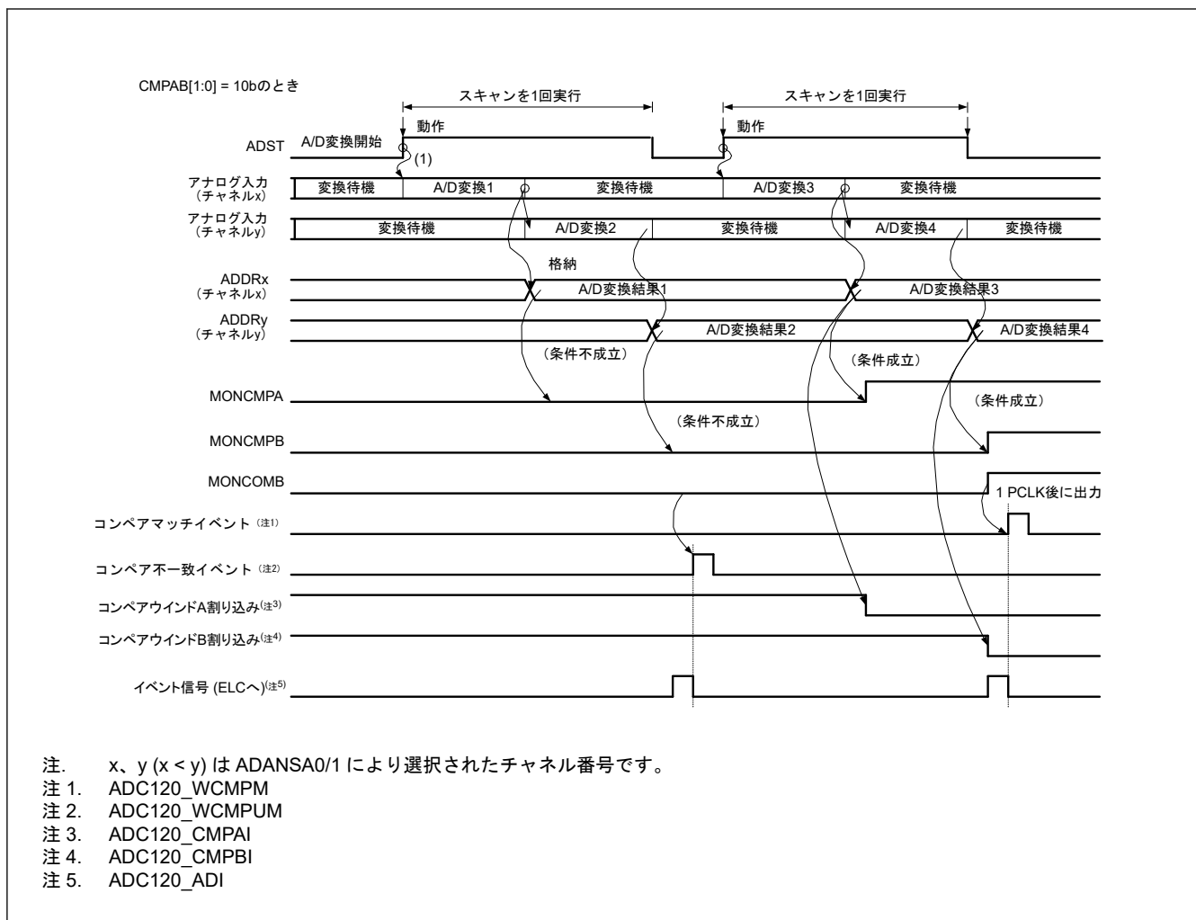
図 32.33 コンペア機能のイベント出力の動作例（アナログ入力（チャンネル x、y）を比較）
