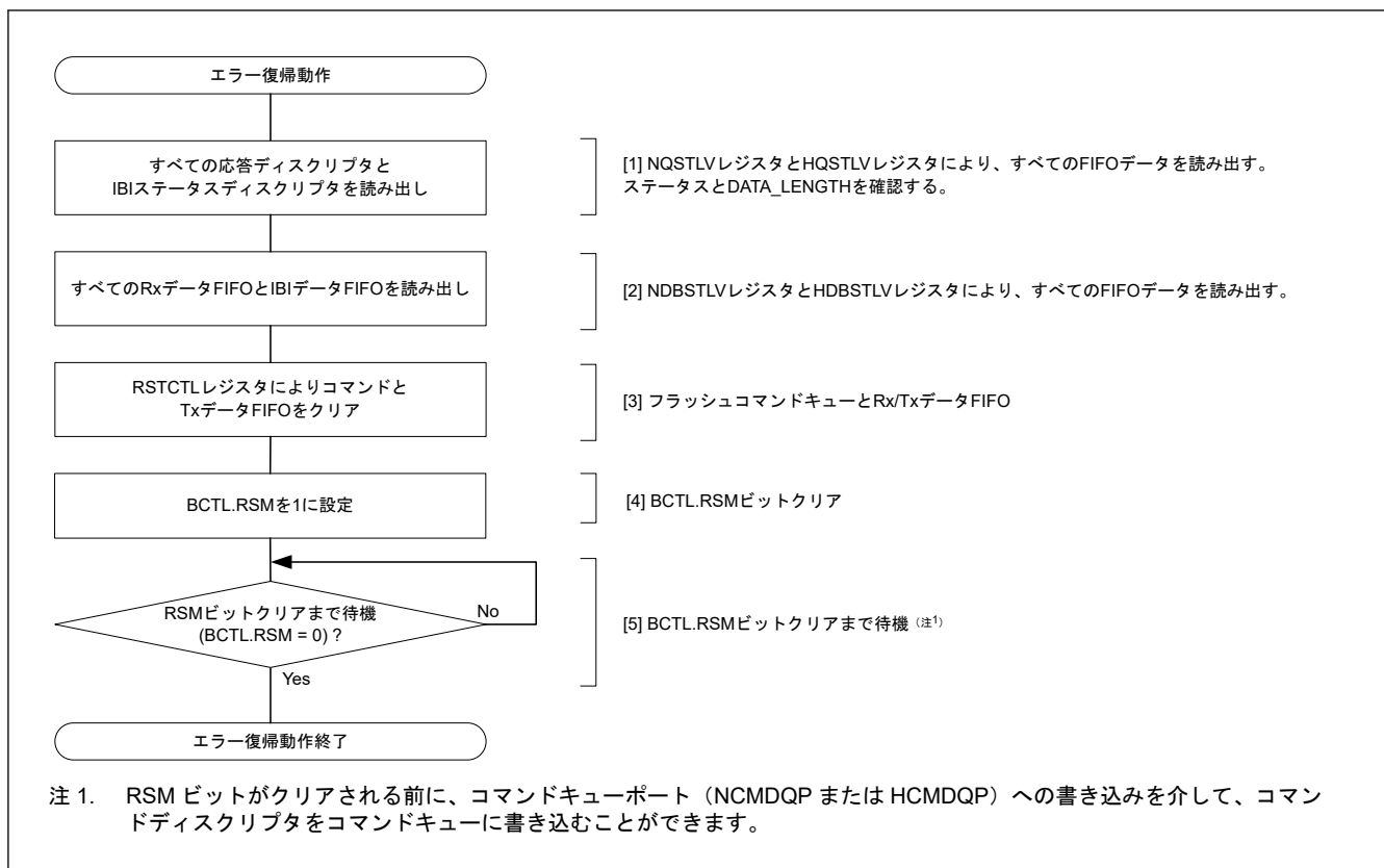
図 25.95 I3C マスタのエラー復帰動作フローの例
