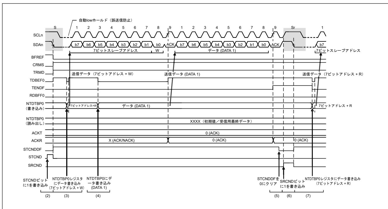
図 25.57 マスタ送信後の繰り返しのスタートコンディション発行タイミング
