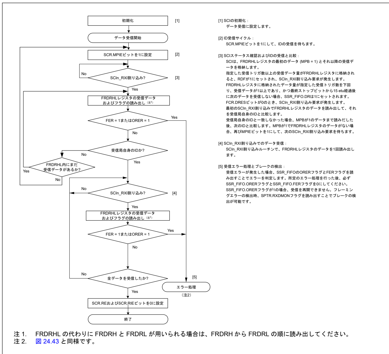
図 24.45 マルチプロセッサモードにおけるシリアル受信のフローチャート例 (FIFO 選択時)
