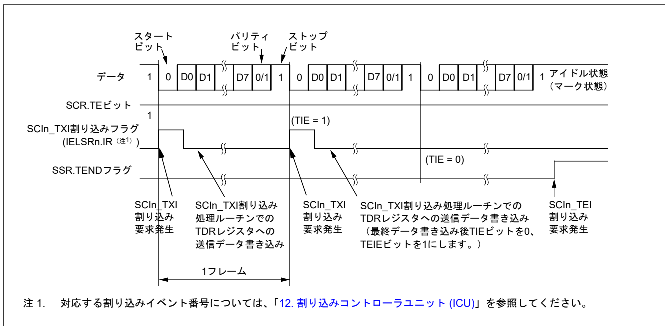
図 24.10 調歩同期式モードにおけるシリアル送信の動作例 (3) (8 ビットデータ/パリティあり/1ストップビット/CTS 機能不使用/送信中～送信終了時)
