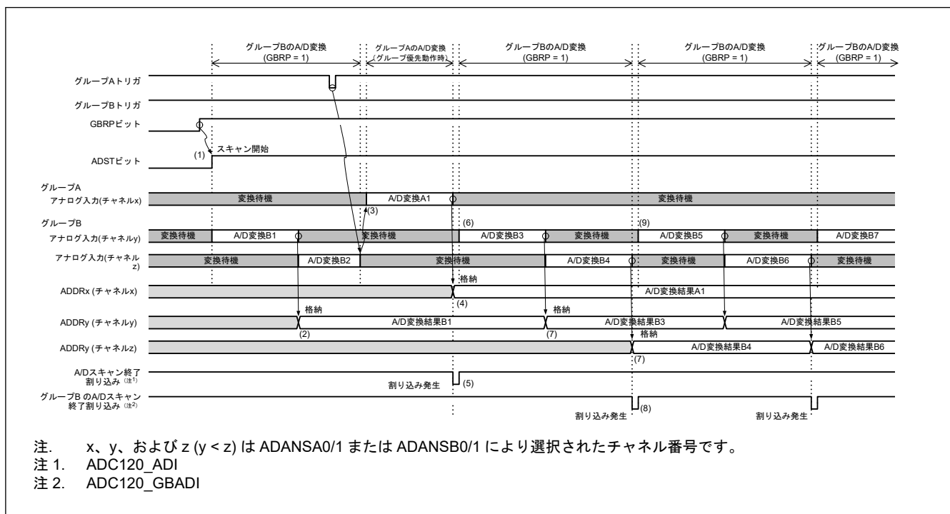
図 32.30 グループ優先動作の例 1-5 : グループ B のシングルスキャン連続動作 (ADGSPCR.GBRP = 1、ADGSPCR.LGRRS = 0 の場合)
