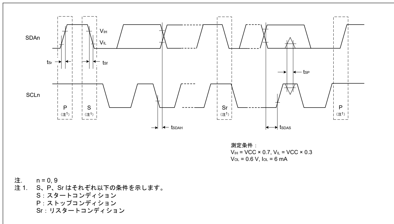
図 41.33 SCI 簡易 IIC モードタイミング
