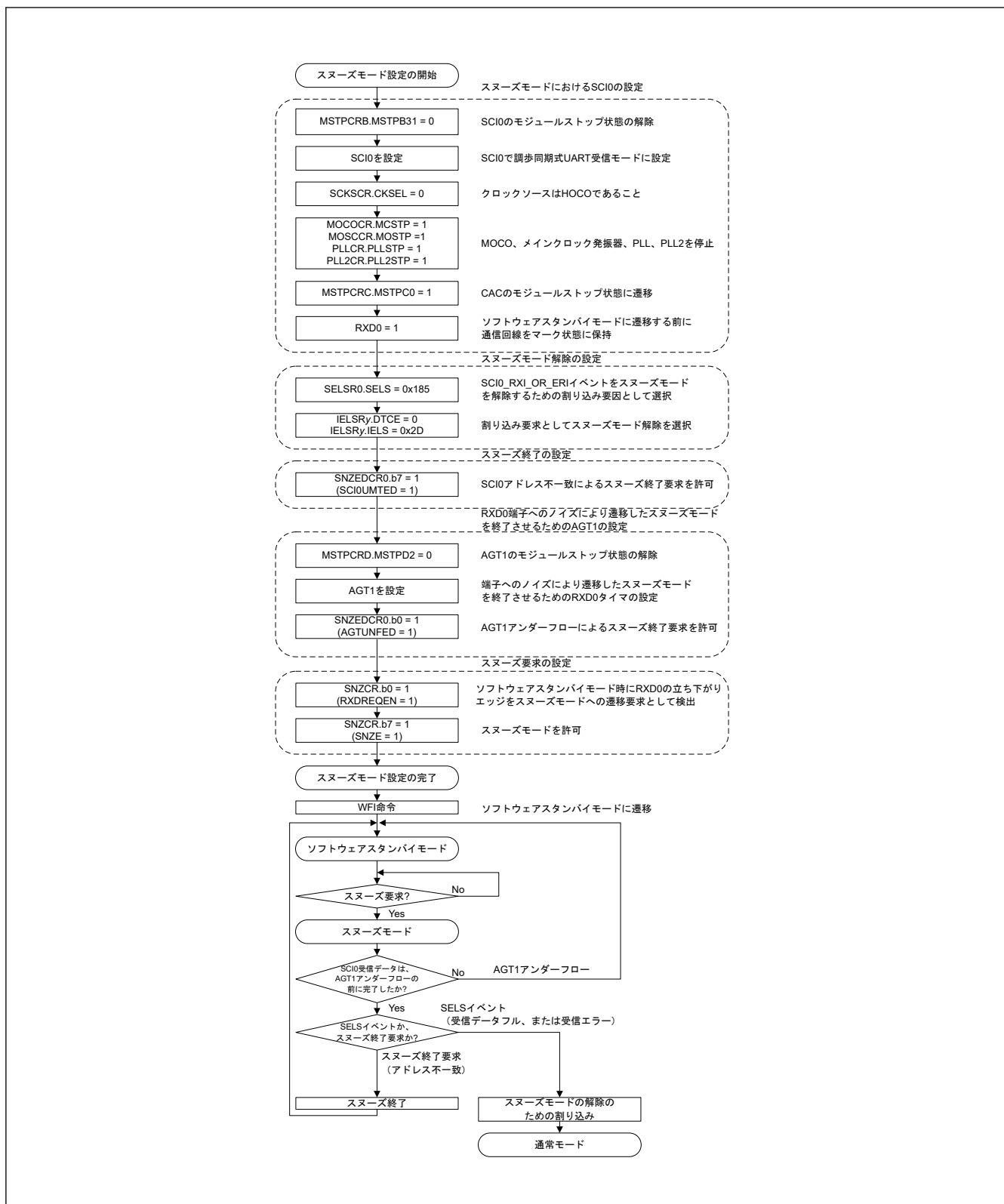
図 10.7 スヌーズモードエントリで SCI0 を使用する場合の設定例
