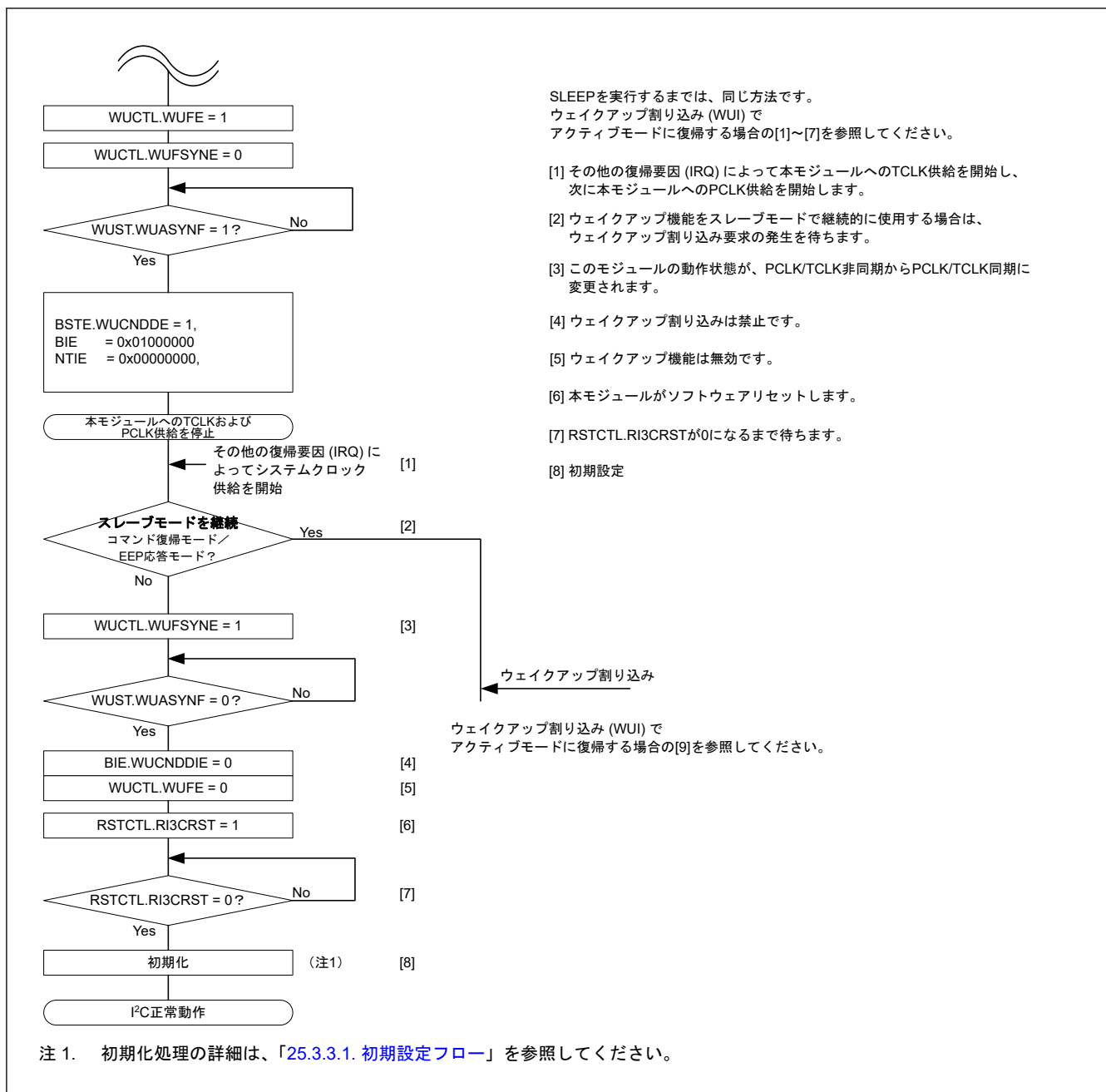
図 25.105 コマンドリカバリモードと EEP 応答モードの使用例 (他のリカバリ要因 (IRQ) によるウェイクアップリカバリの場合)
