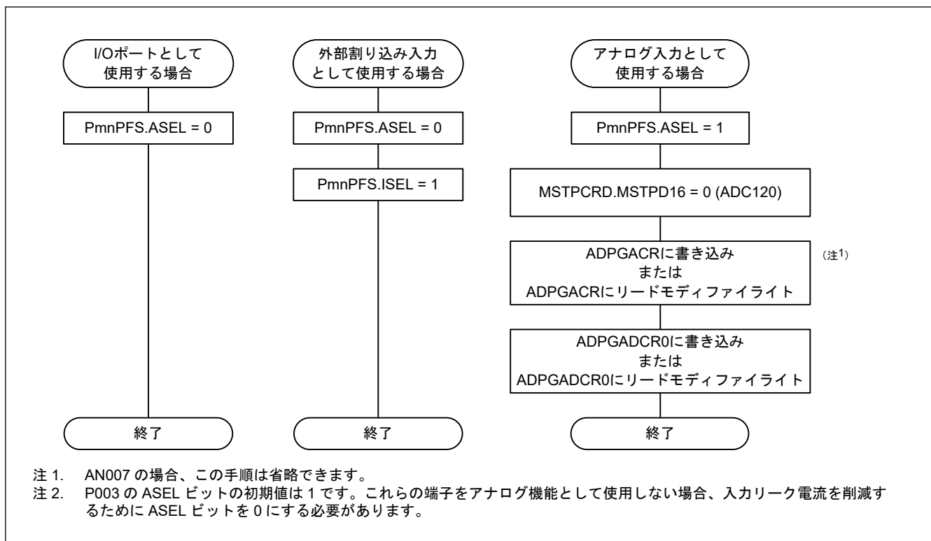
図 32.42 レジスタ設定手順
