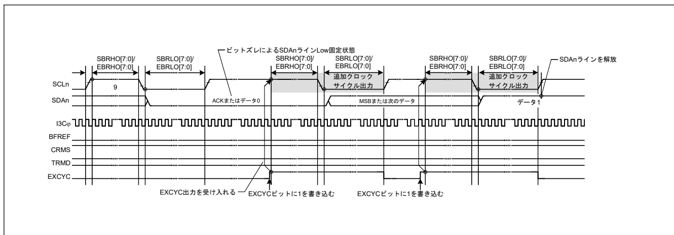
図 25.90 SCL クロック追加出力機能 (EXCYC ビット)
