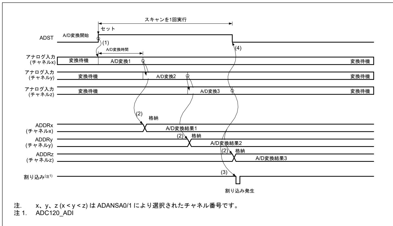
図 32.7 シングルスキャンモードの基本動作例（アナログ入力（チャンネル x~z）選択）
