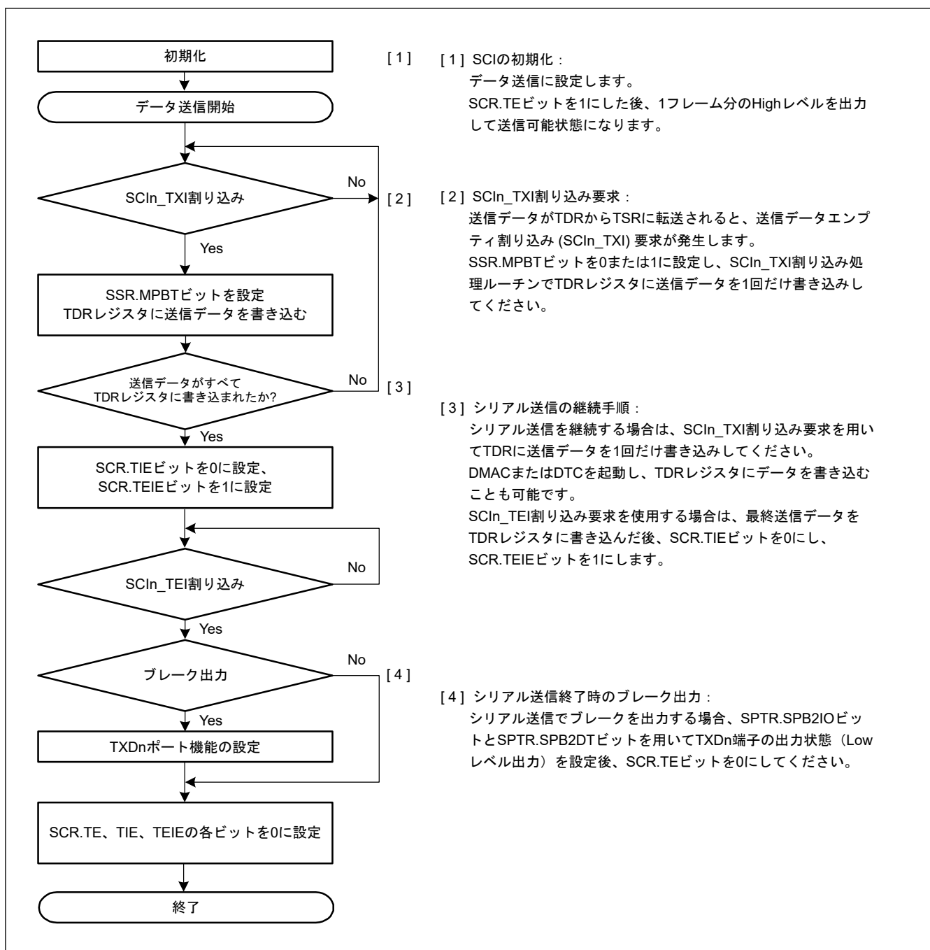
図 24.38 マルチプロセッサシリアル送信のフローチャート例 (非 FIFO 選択時)
