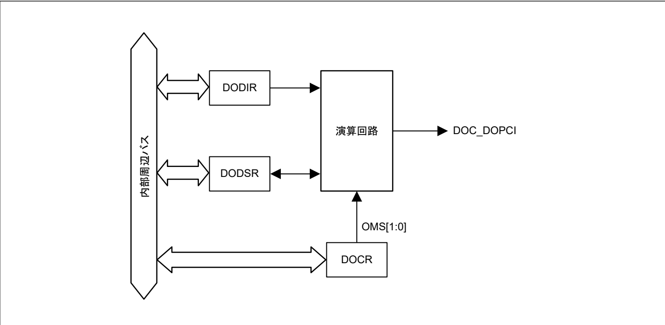
図 36.1 DOC のブロック図
