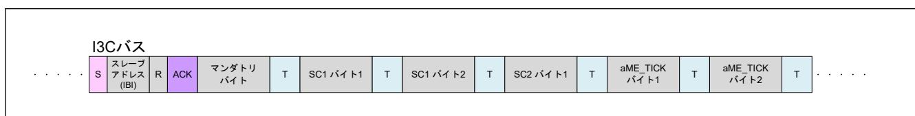
図 25.89 非同期モード 1 のタイムスタンプデータ転送動作例
