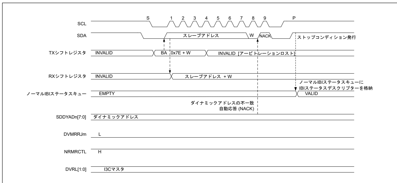
図 25.83 バス権要求 : NACK (DAT.DVDYAD[7:0]ビットが一致しない) かつ NRMRCTL が 1 の場合
