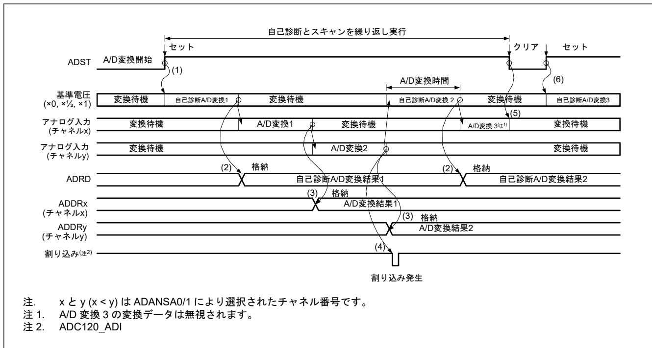
図 32.19 連続スキャンモードの基本動作例（アナログ入力（チャンネル x、y）選択+自己診断）
