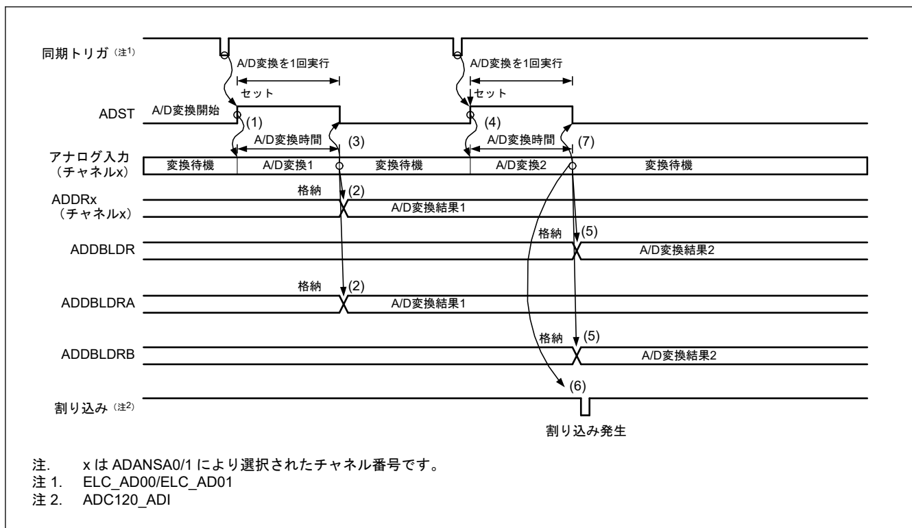
図 32.15 アナログ入力 (チャンネル x) と ELC_AD00/ELC_AD01 の重複選択時のダブルトリガモード拡張動作例
