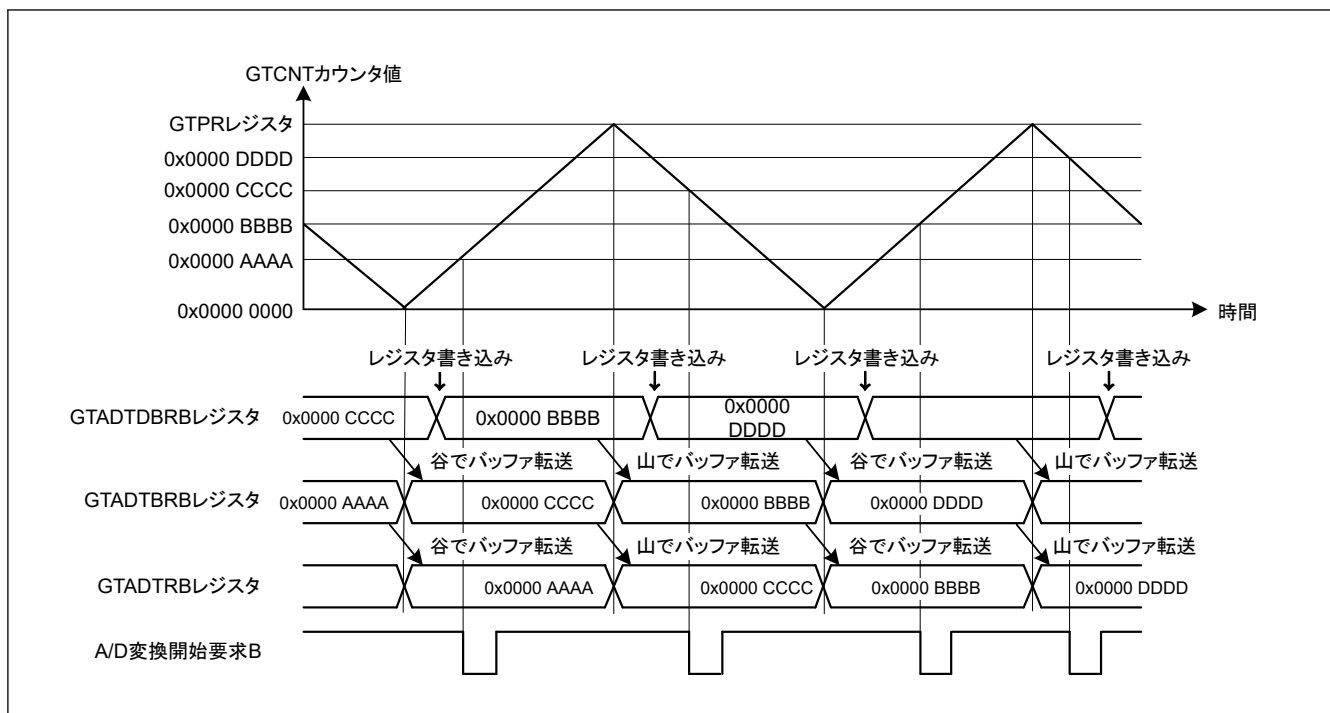
図 20.21 GTADTRA および GTADTRB レジスタのダブルバッファ動作例 (三角波、谷と山の両方でバッファ転送、アップカウントとダウナカウントの両方で A/D 変換開始要求発生の場合)
