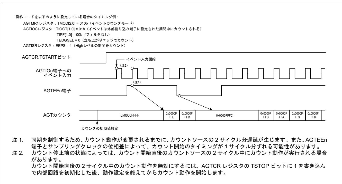
図 21.10 イベントカウンタモードでの動作例 2
