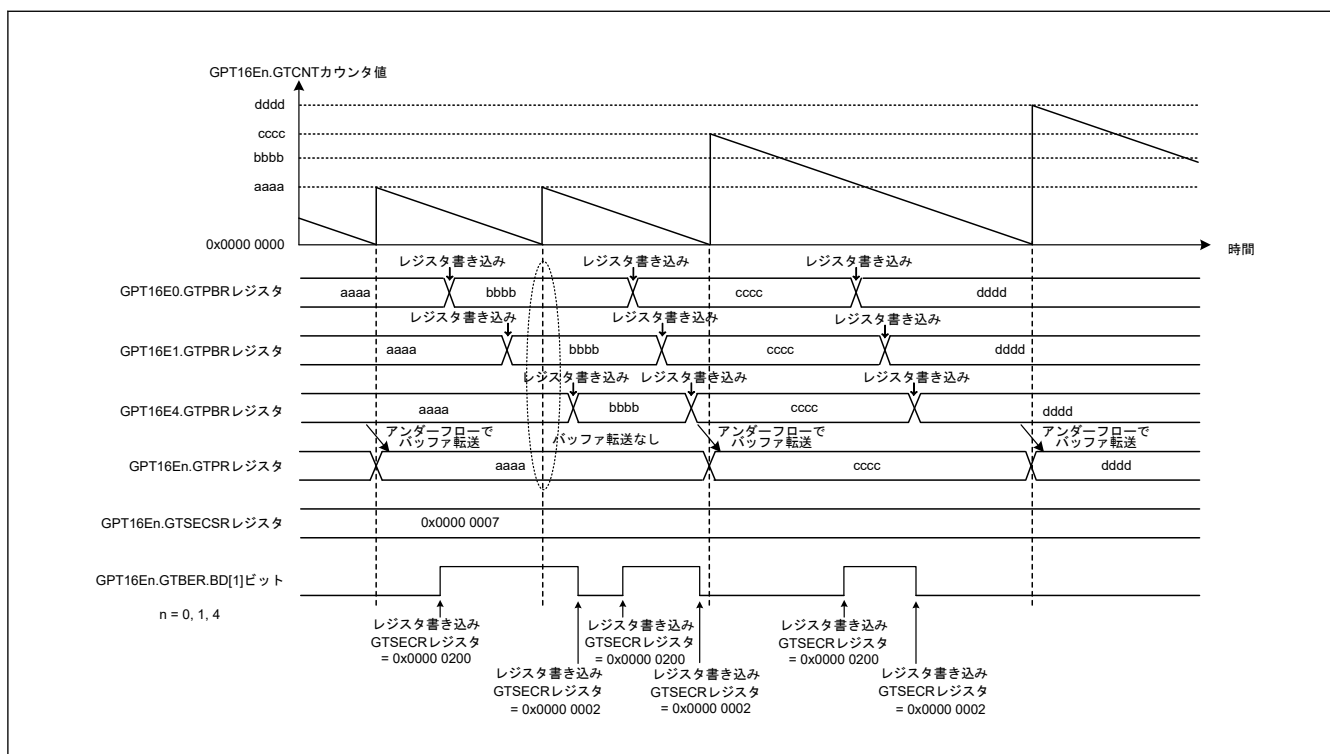
図 20.80 バッファ動作禁止の複数チャネルの動作例 (のこぎり波、シングルバッファ動作)
