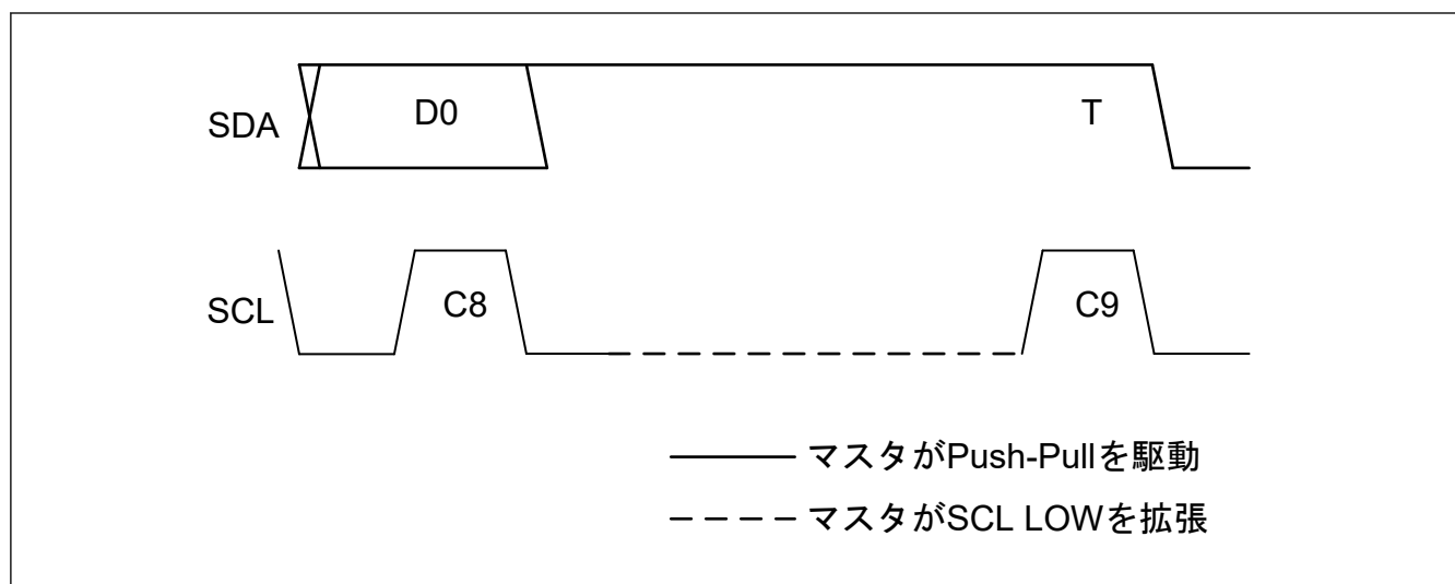
図 25.74 書き込みパリティビットのマスタクロックストール
