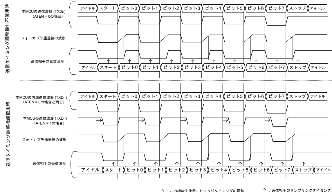
図 24.34 フォトカプラを経由する送信波形の説明
