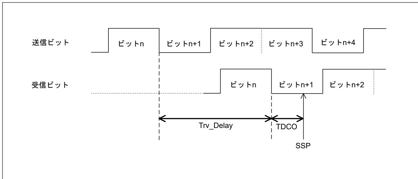
図 26.20 セカンダリサンプルポイントの位置
