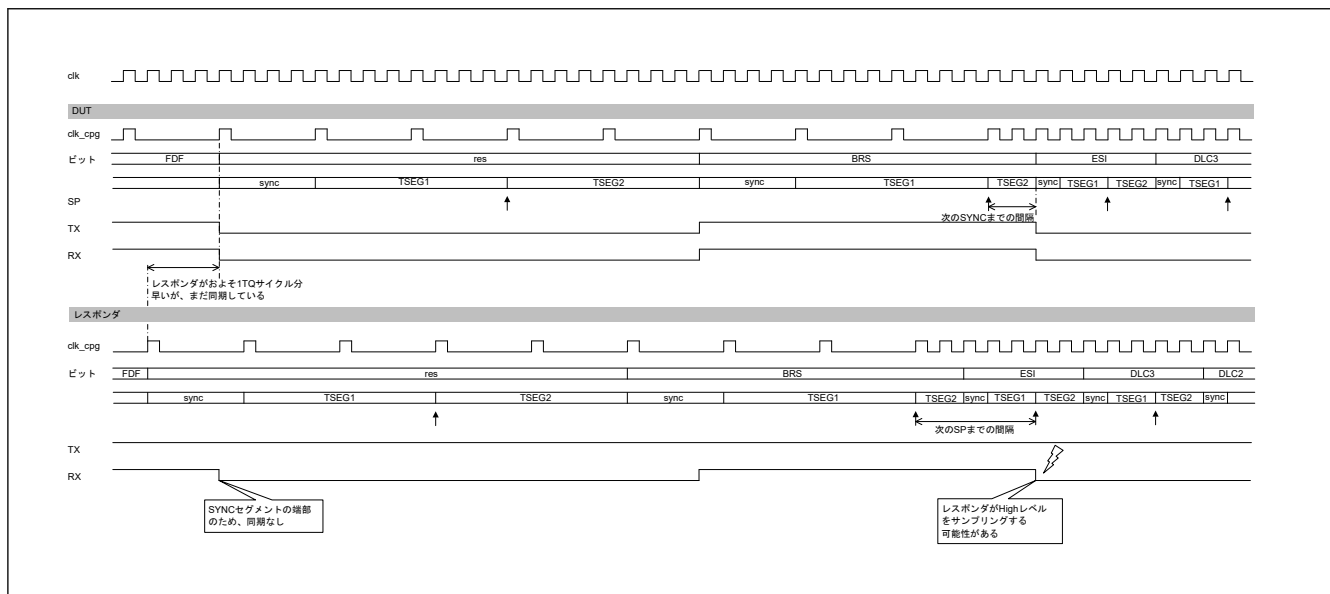
図 26.21 2 つの CAN ノード間の同期ズレ
