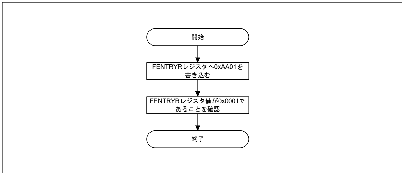
図 38.9 コードフラッシュ P/E モードへの遷移手順
