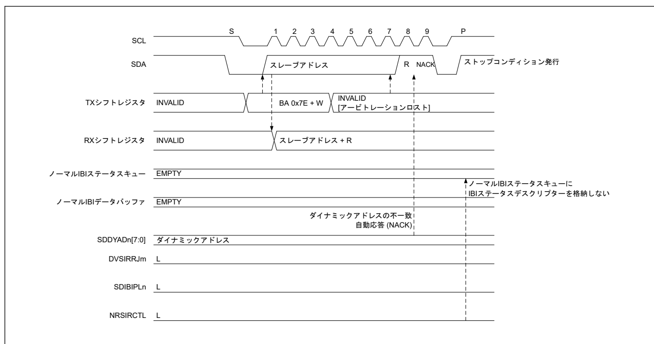
図 25.79 スレーブ割り込み要求 : NACK (DAT.SDDYAD[7:0]ビットが一致しない) かつ NRSIRCTL が 0 の場合
