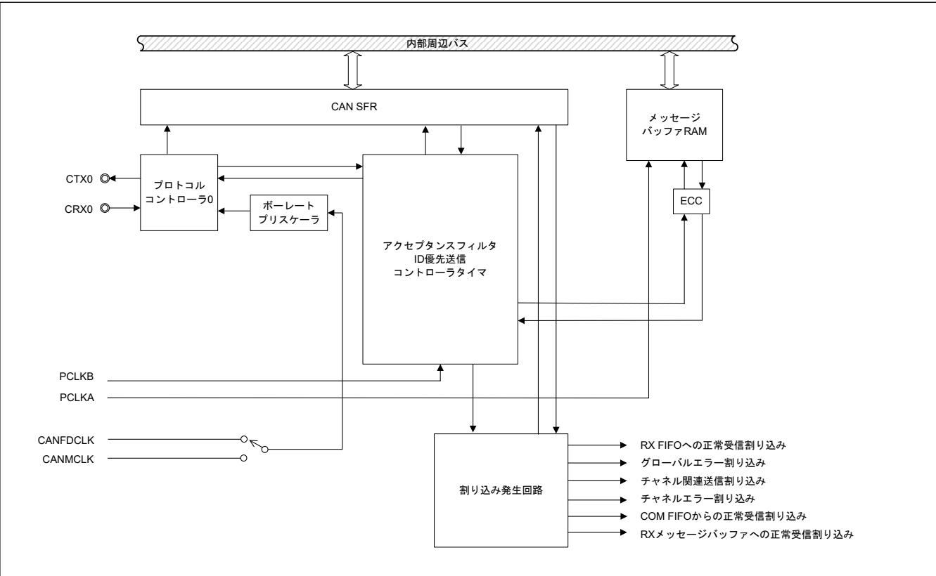
図 26.1 CANFD モジュールの概要
