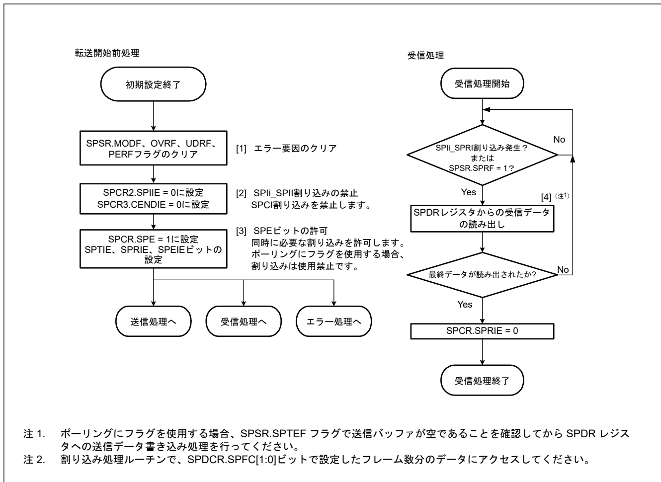
図 28.54 スレーブモードでの受信フロー
