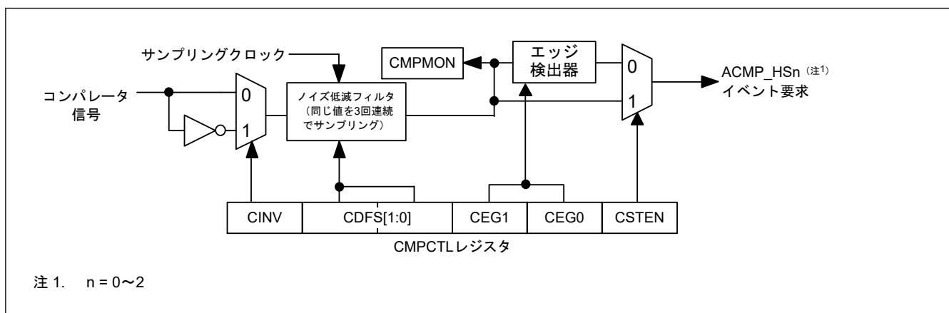
図 35.3 ノイズフィルタとエッジ検出回路の構成
