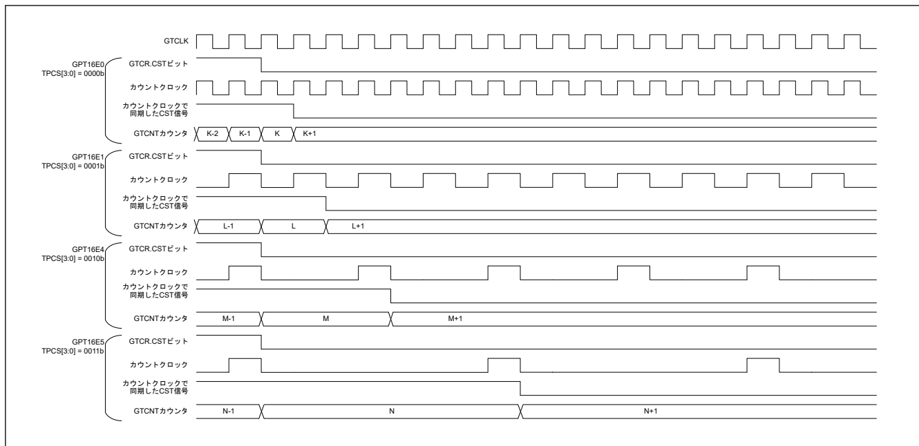
図 20.42 ソフトウェアによる同時ストップの動作例（異なるカウント周期）
