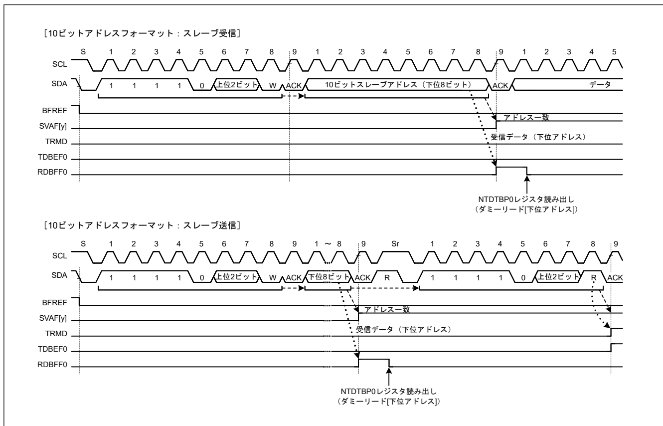
図 25.60 SVA[y]フラグが1になるタイミング (10ビットアドレスフォーマット選択時)
