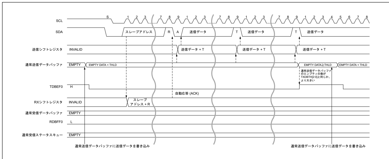
図 25.39 SDR データ読み出し転送タイミング (1/2)
