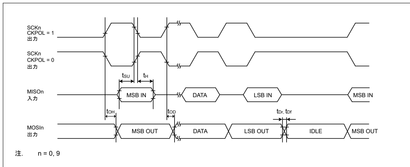
図 41.30 CKPH = 0 の場合におけるマスタの SCI 簡易 SPI モードタイミング
