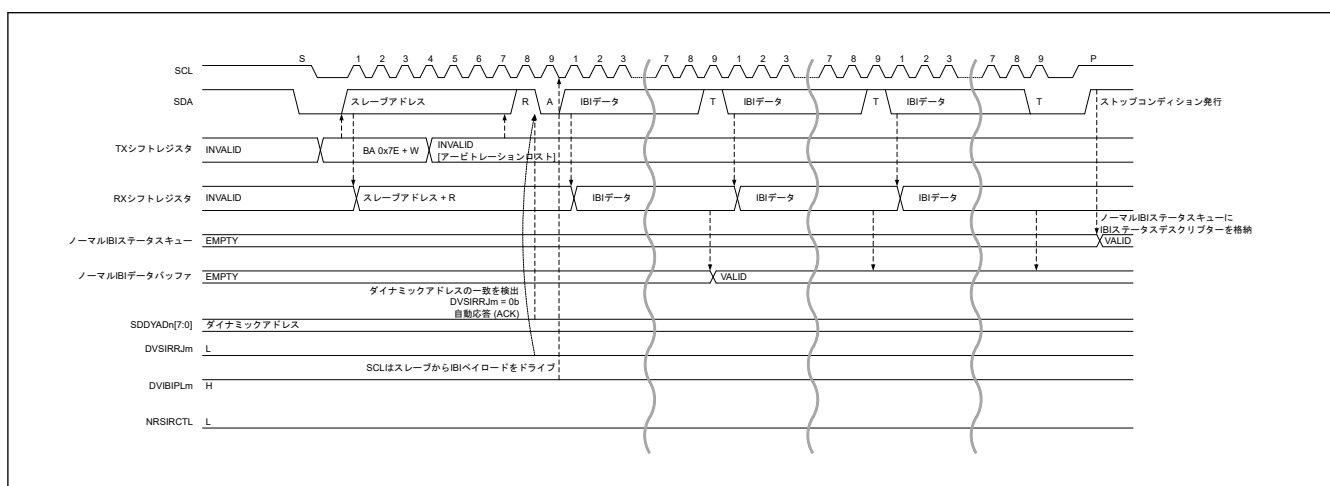
図 25.77 スレーブ割り込み要求：ACK かつ DVIBIPL が 1 の場合
