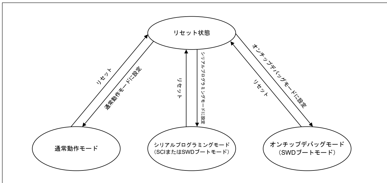
図 38.5 フラッシュメモリに関するモード遷移図
