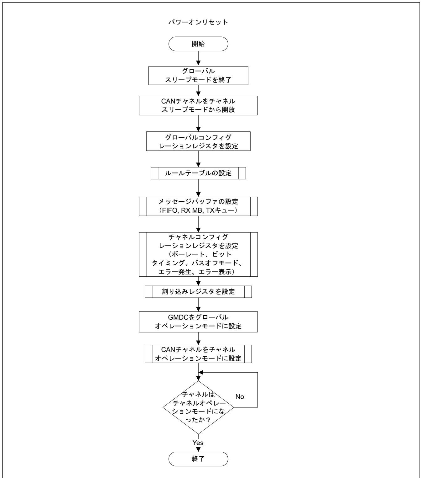
図 26.23 ハードウェアリセット後の構成手順
