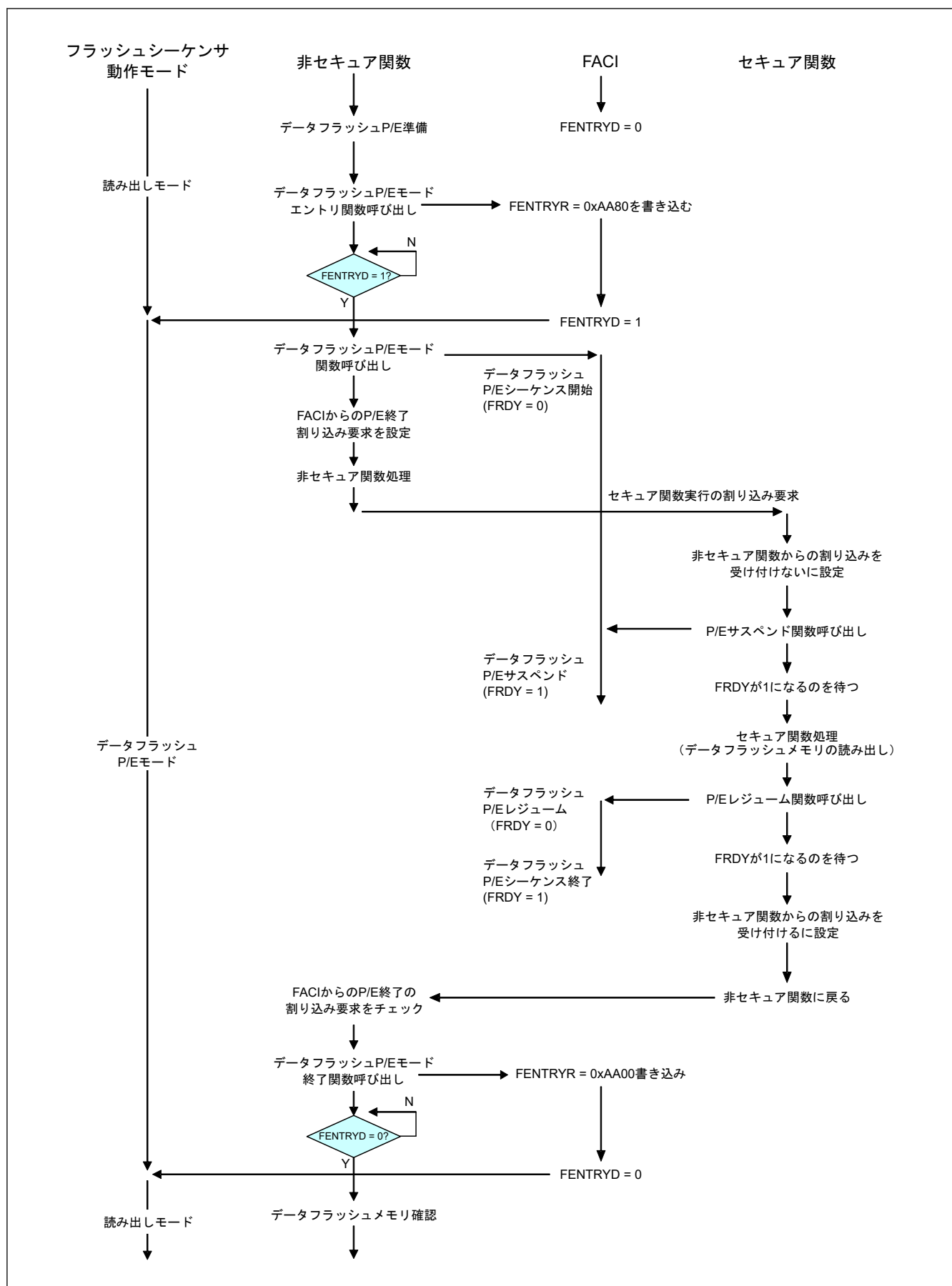
図 38.35 セキュア関数のデータフラッシュ P/E サスペンド例 (P/E 終了を検出するには割り込み要求を確認)
