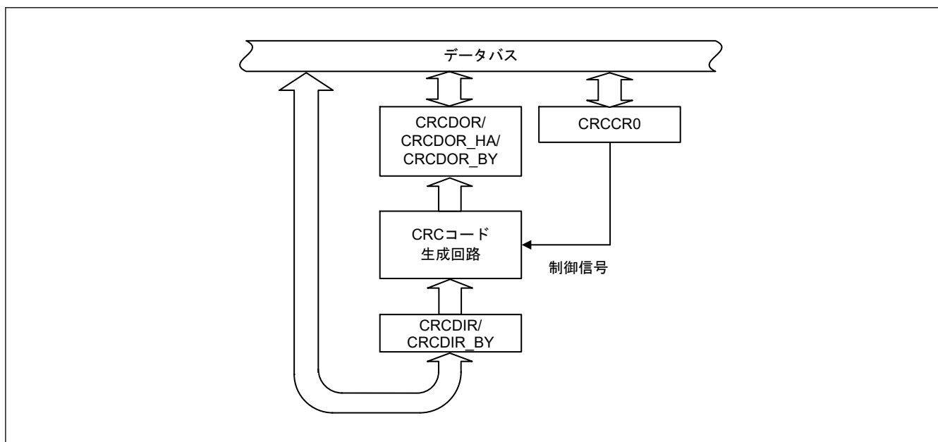
図 29.1 CRC 演算器のブロック図
