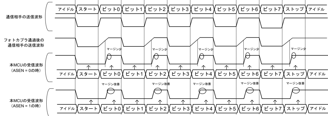
図 24.30 受信サンプリングタイミング調整機能による受信マージン向上の例
