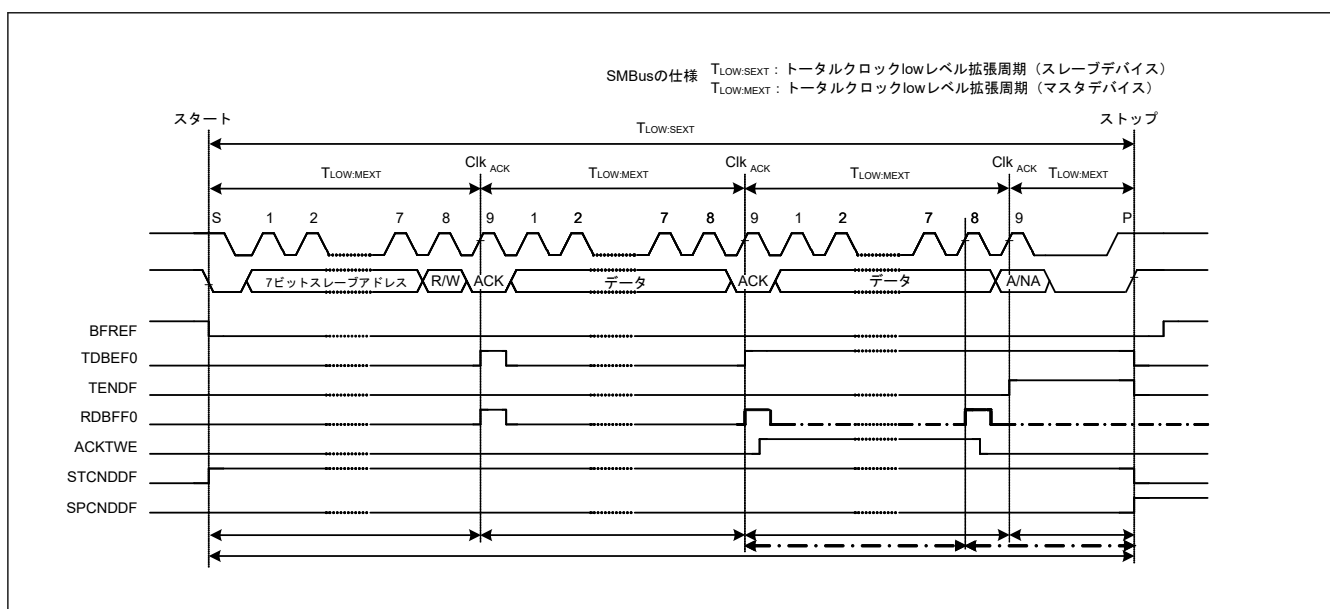
図 25.91 SMBus タイムアウト測定
