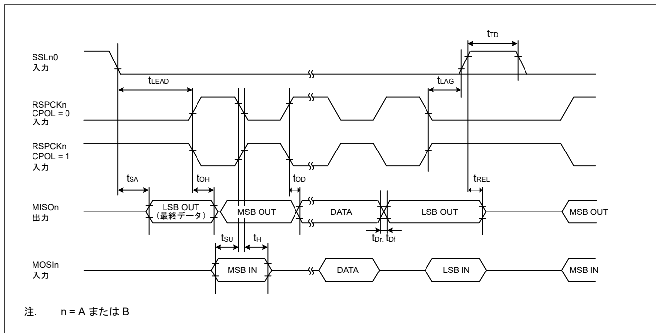
図 41.40 CPHA = 1 の場合におけるスレーブの SPI タイミング
