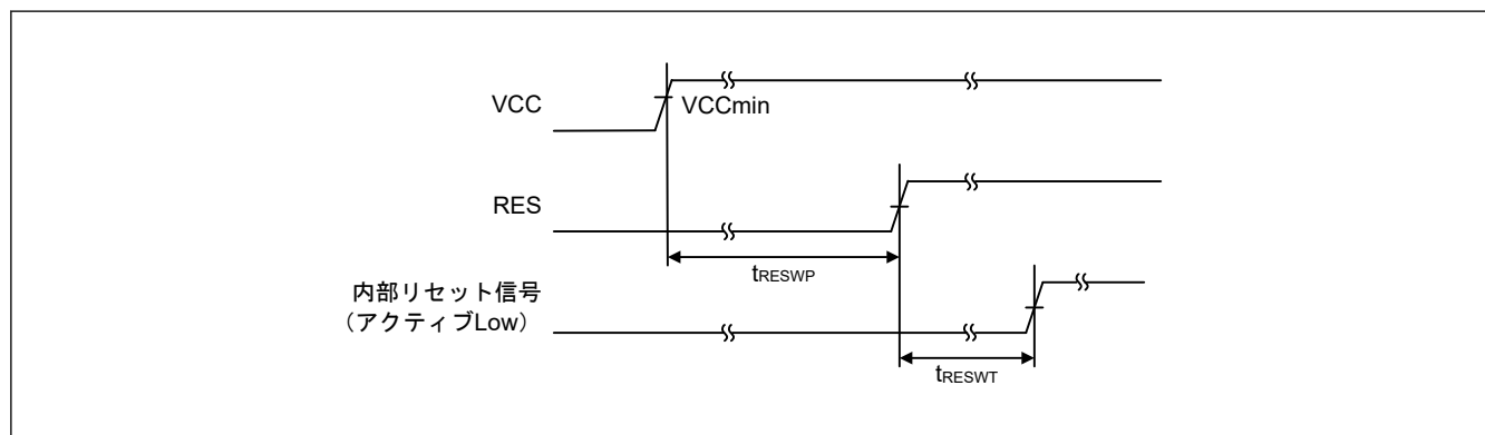
図 41.12 VCC が V_{POR} 電圧しきい値を超える条件下での RES 端子入力タイミング
