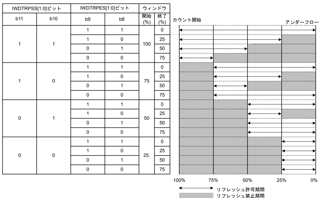
図 23.2 IWDRPSS[1:0]およびIWDRPES[1:0]ビットとリフレッシュ許可期間
