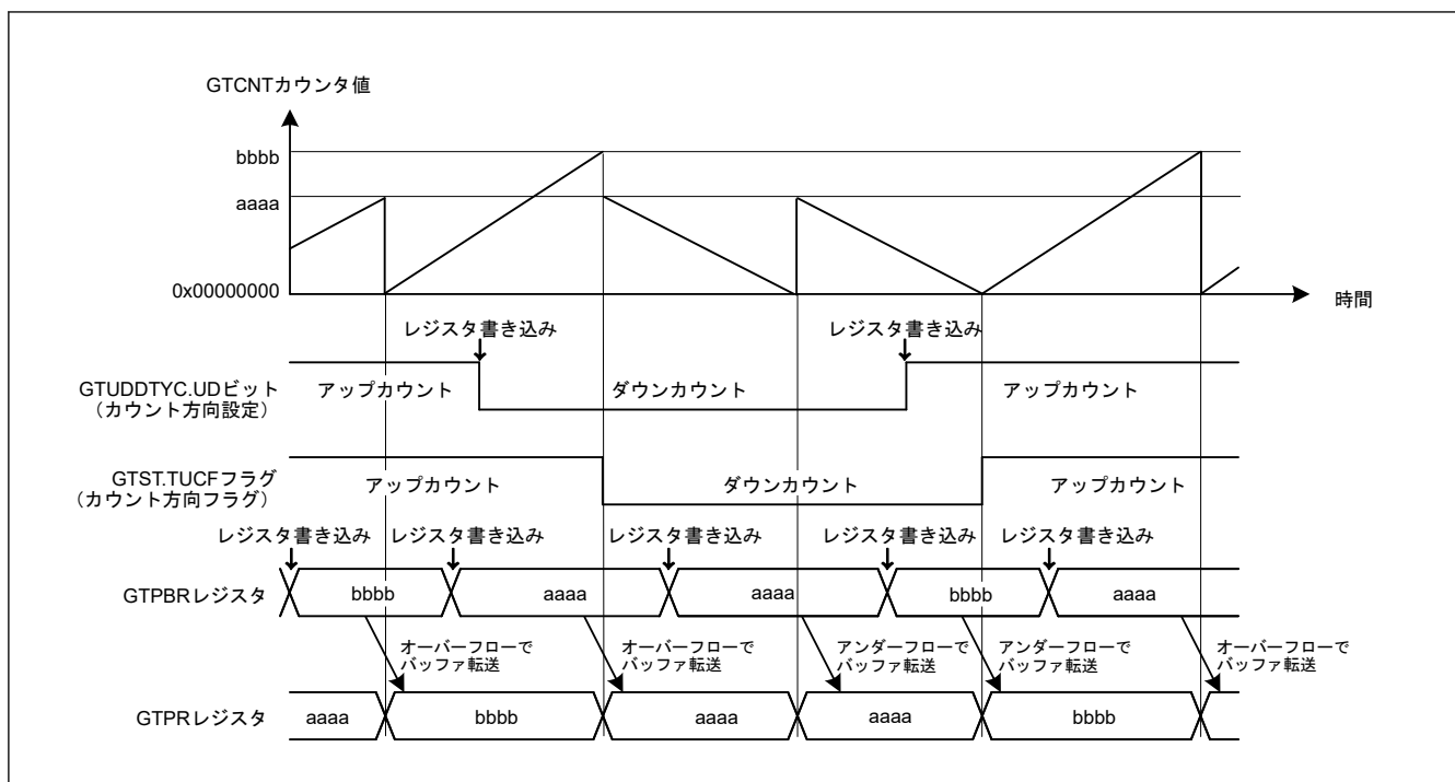
図 20.31 カウント方向切り替え機能の動作例 (バッファ動作時)
