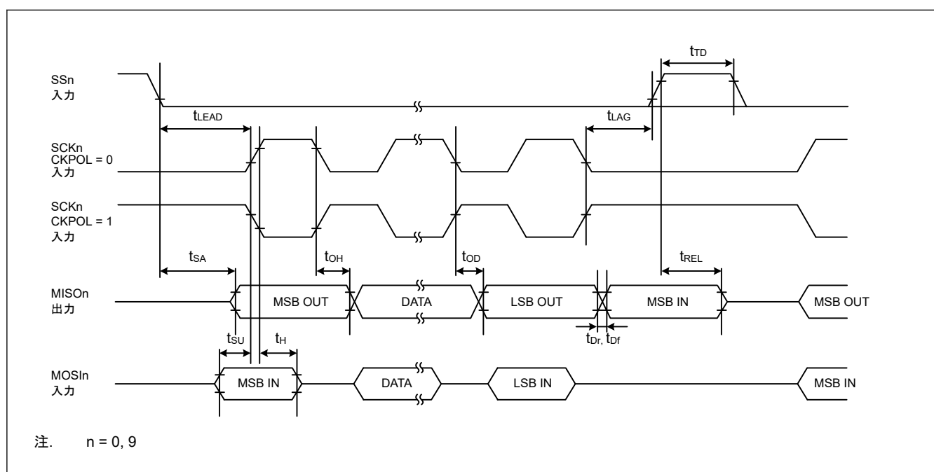
図 41.31 CKPH = 1 の場合におけるスレーブの SCI 簡易 SPI モードタイミング
