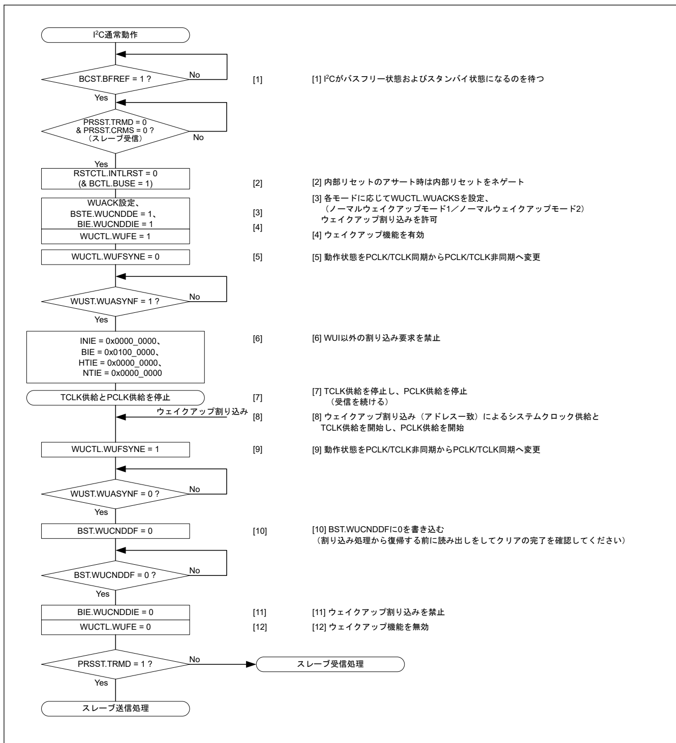
図 25.99 ノーマル WU モード 1 の使用例 (スレーブアドレス一致に起因するウェイクアップ割り込みによるウェイクアップリカバリの場合)
