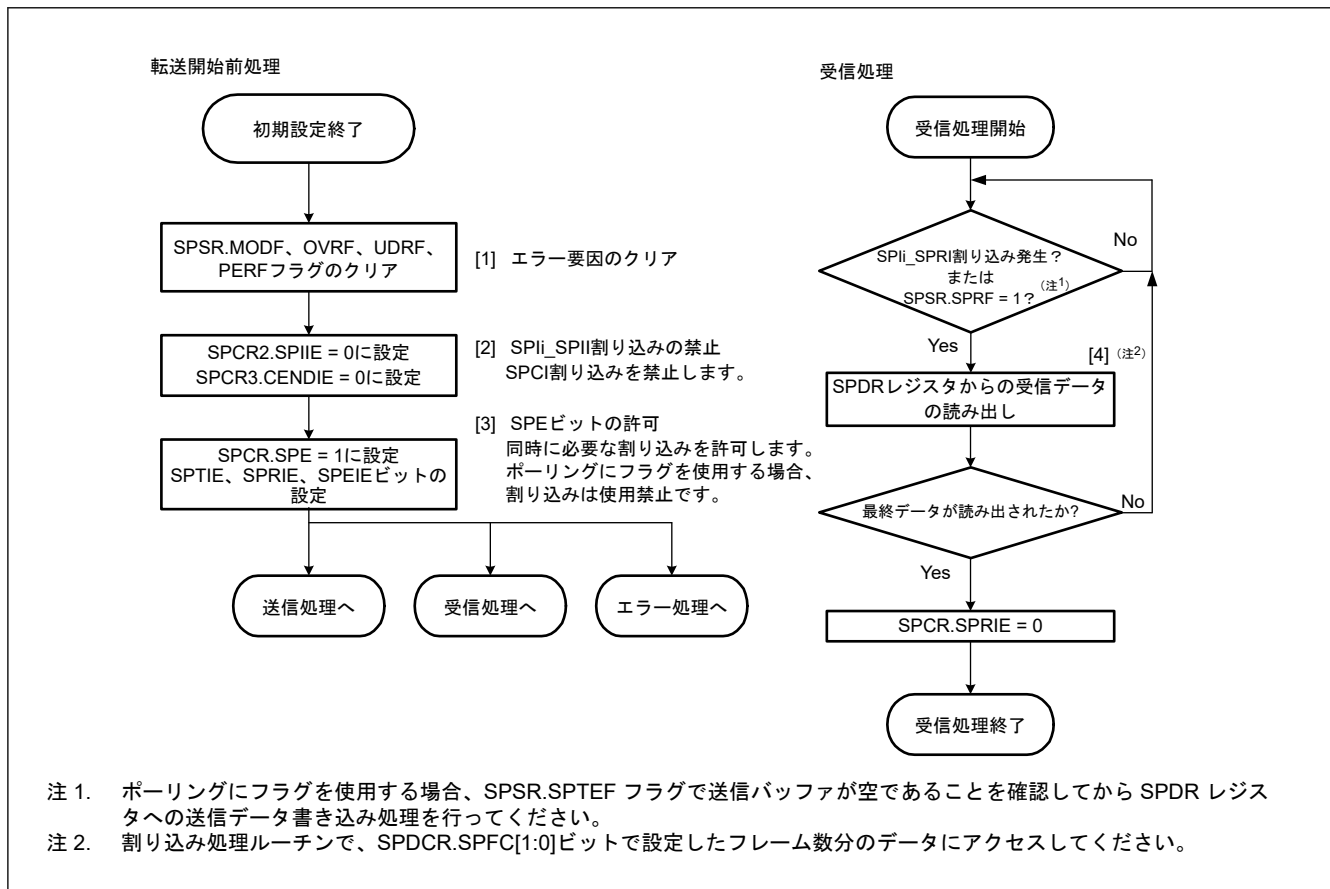
図 28.53 スレープモードでの送信フロー
