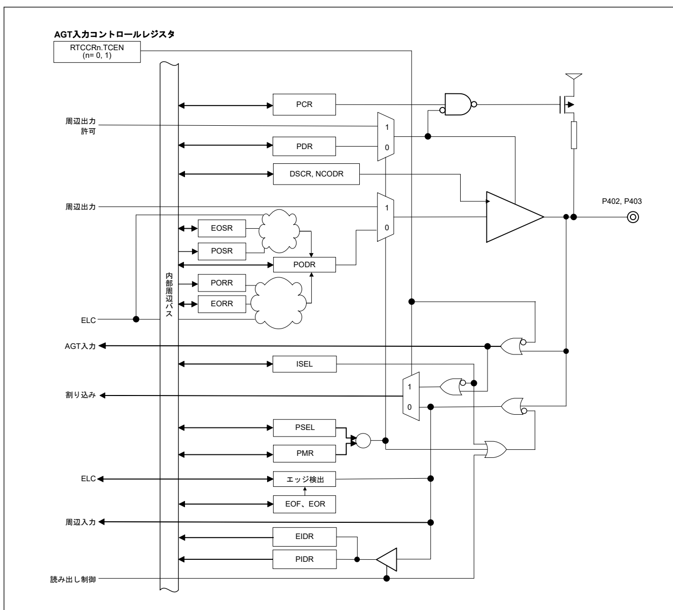
図 18.5 P402 および P403 の接続図
