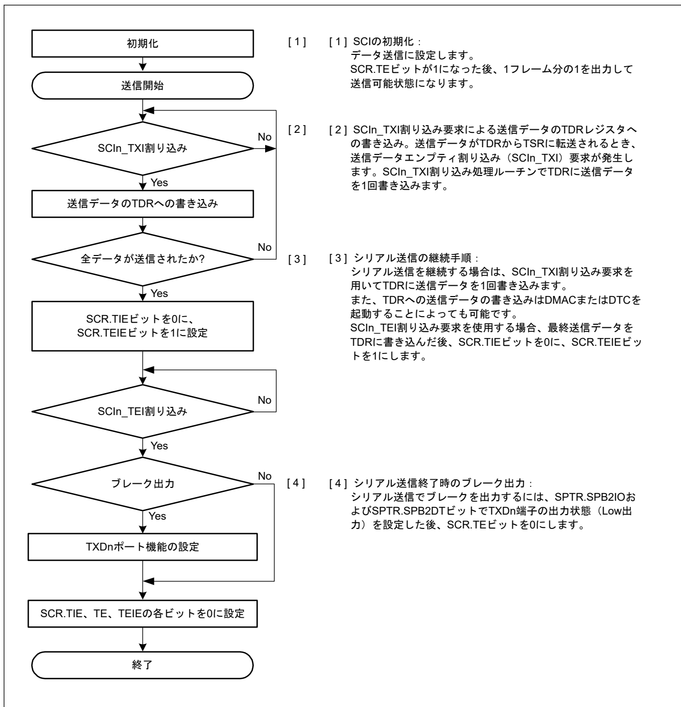
図 24.12 調歩同期式モードにおけるシリアル送信のフローチャート例（非 FIFO 選択時）
