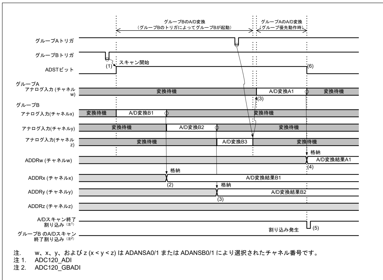
図 32.29 グループ優先動作の例 1-4 : グループ B スキャン中のグループ A トリガ入力、再スキャンなし (ADGSPCR.GBRSCN = 0、ADGSPCR.GBRP = 0、および ADGSPCR.LGRRS = 0 の場合)
