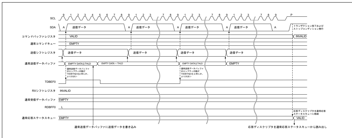
図 25.19 レガシー I2C メッセージデータ書き込みタイミング (2/2)
