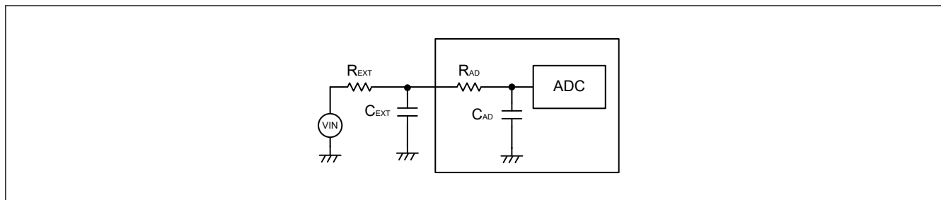
図 32.44 サンプル&amp;ホールド回路の簡略図
