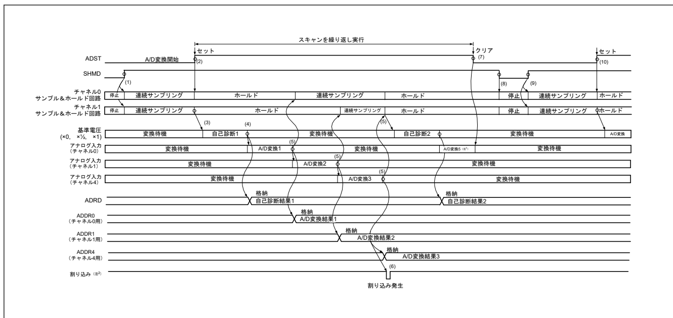
図 32.21 連続スキャンモードの動作例（チャンネル専用サンプル&ホールド回路を使用し、自己診断で AN000、AN001、AN004 を選択し、連続サンプリングを有効にした場合）
