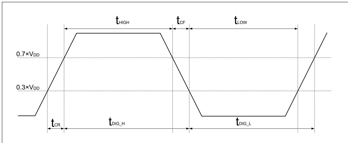
図 41.43 t_{DIG\_H} 、 t_{DIG\_L}
