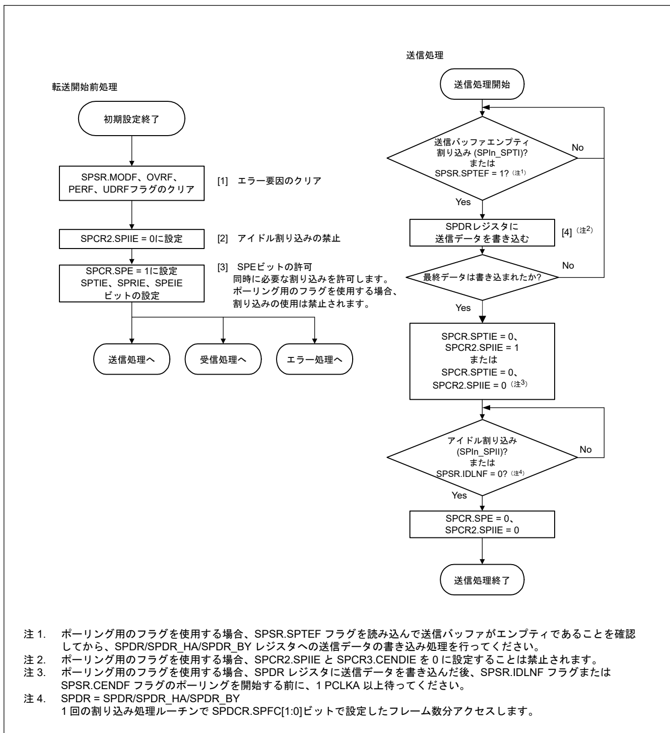
図 28.49 マスタモードでの送信フロー
