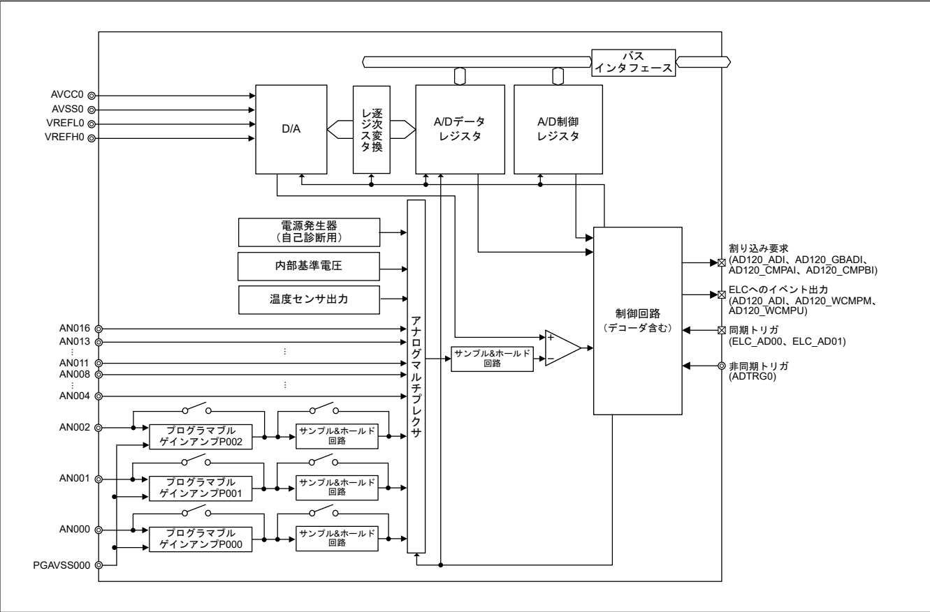
図 32.1 ADC12 のブロック図
