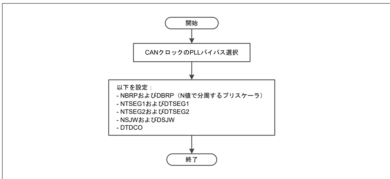
図 26.17 CAN のビットタイミングとボーレートを設定する手順
