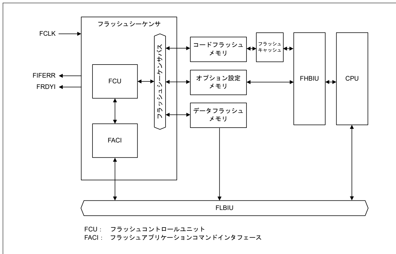
図 38.1 フラッシュメモリ関連モジュールのブロック図
