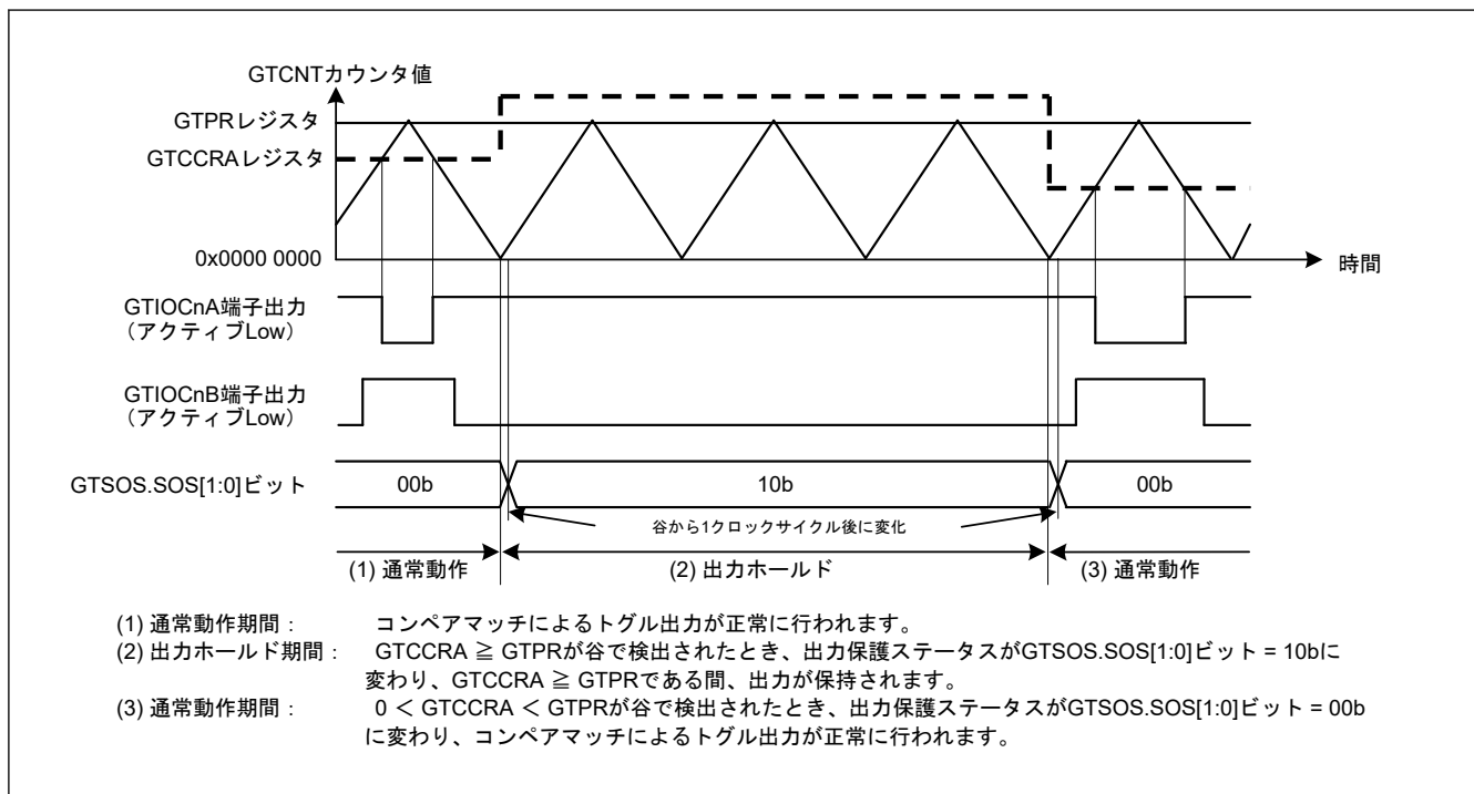
図 20.87 谷でのバッファ転送中に GTCCRA \geq GTPR となったときの出力保護機能の動作例 (谷でのバッファ転送中に 0 < \text{GTCCRA} < \text{GTPR} に復帰、アクティブレベルは Low) ( n = 0 \sim 5 )
