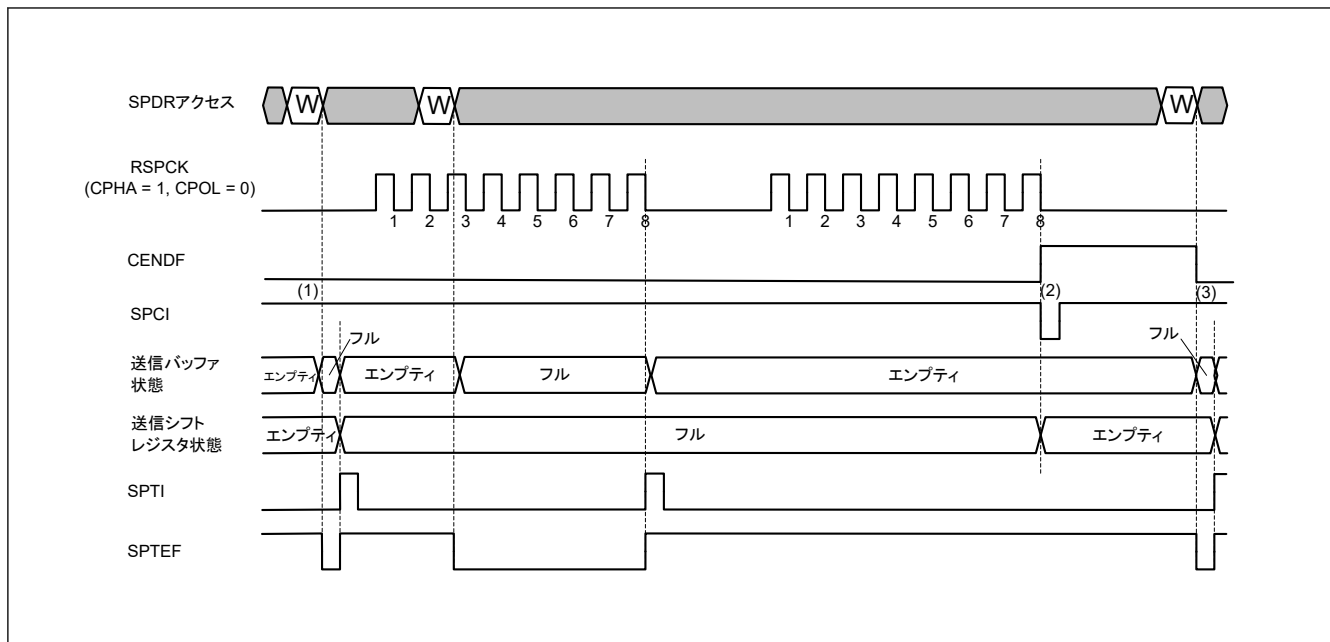
図 28.34 通信終了割り込み動作例（クロック同期式動作時の送受信／送信スレーブモード）
