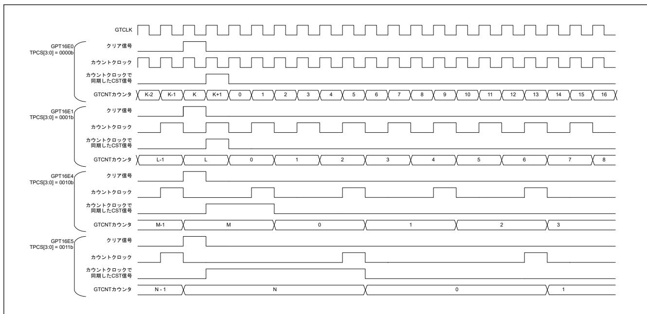
図 20.43 ソフトウェアによる同時クリアの動作例（異なるカウント周期）
