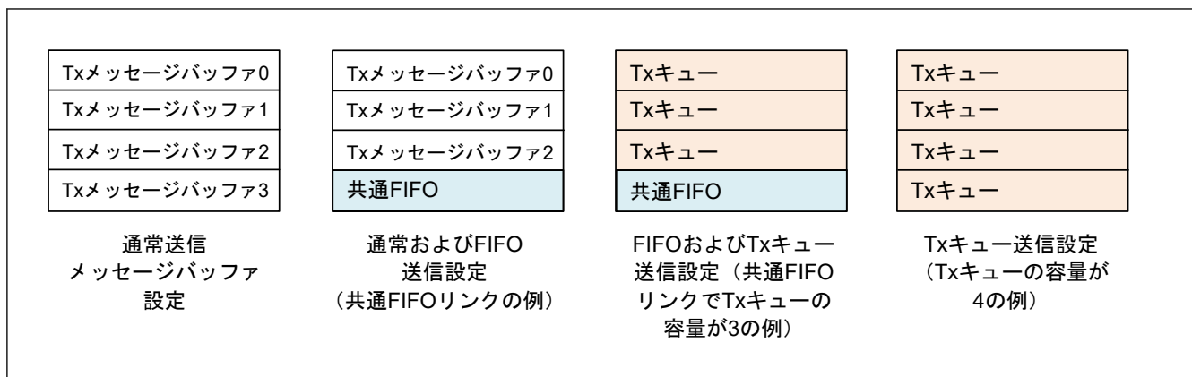
図 26.41 チャネル送信メッセージバッファの構成
