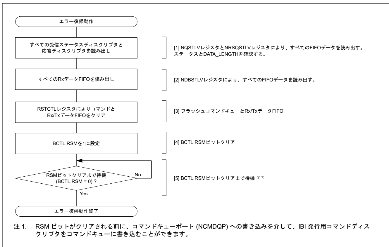
図 25.96 I3C スレーブでのエラー復帰動作フローチャート例
