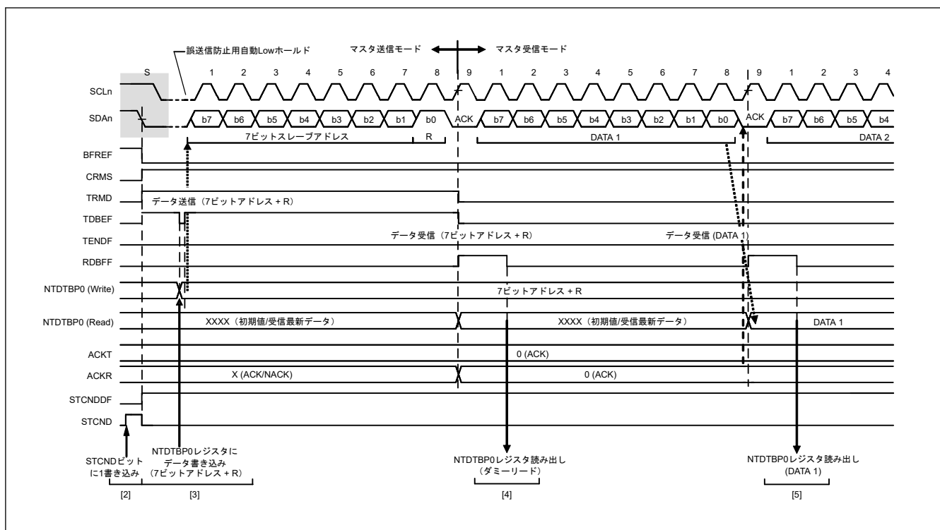
図 25.9 マスタ受信の動作タイミング (1) (7 ビットアドレスフォーマットで ACKTWE = 0 の場合)
