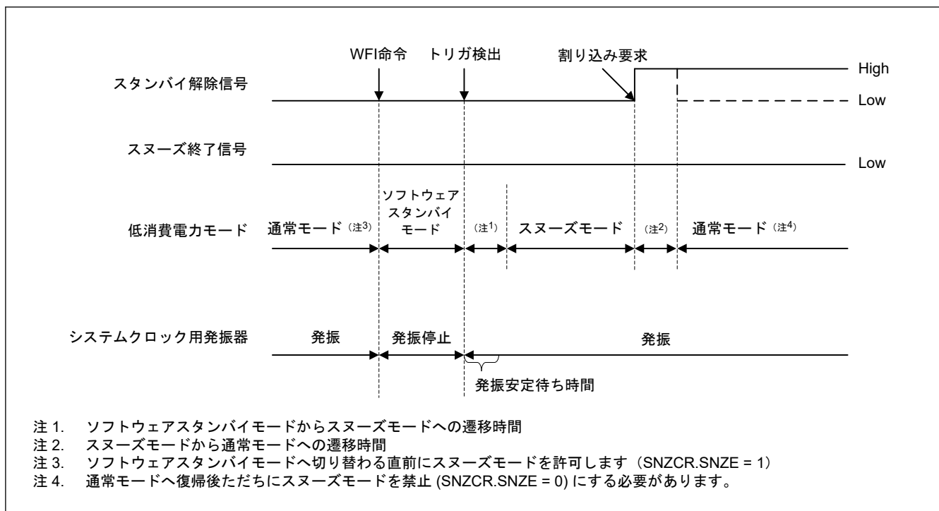
図 10.4 割り込み要求信号が発生する場合のスリープモードの解除
