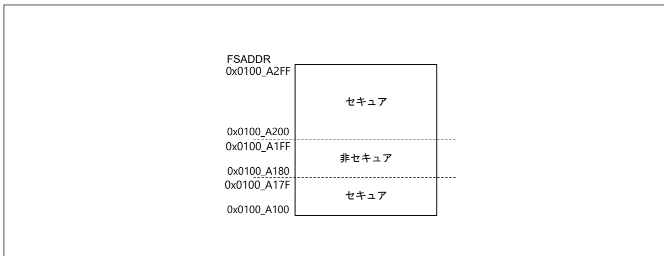
図 38.32 オプション設定メモリのセキュア／非セキュア領域
