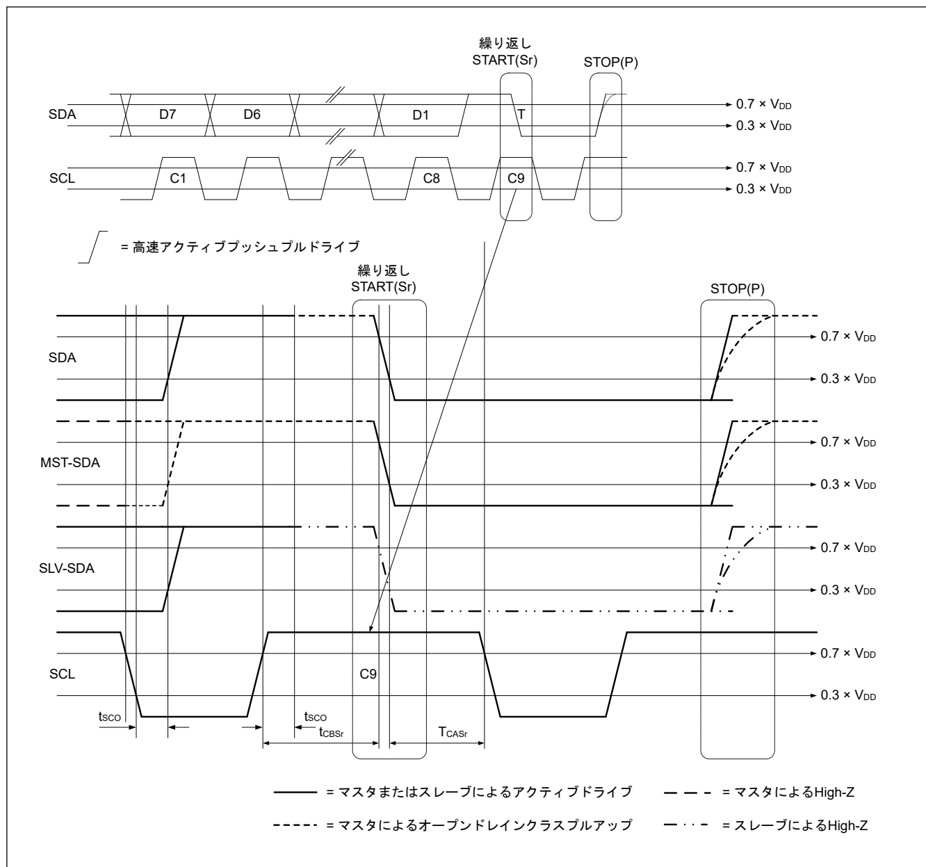
図 41.50 繰り返しのスタートコンディションおよびストップコンディションでのマスタ終了時の T ビット読み出し
