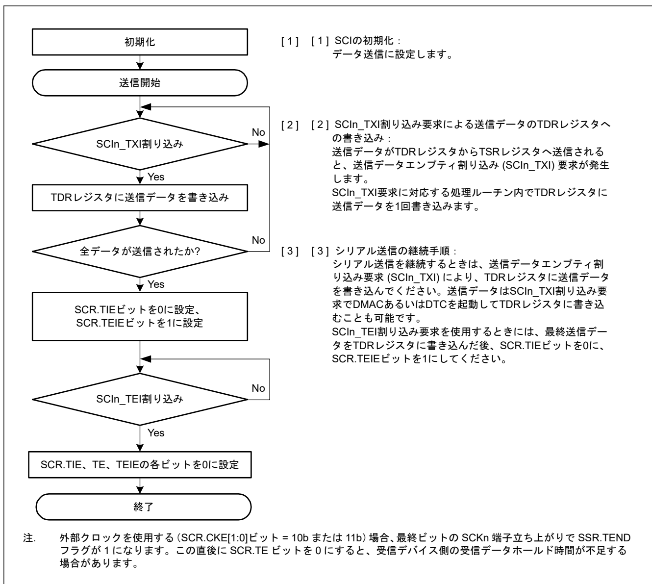
図 24.66 クロック同期式モードにおけるシリアル送信のフローチャート例 (非 FIFO 選択時)
