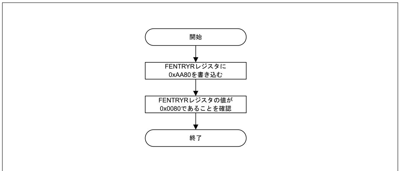
図 38.10 データフラッシュ P/E モードへの遷移手順
