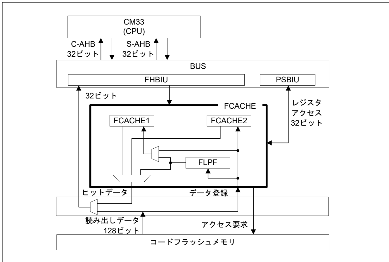
図 38.4 FCACHE のブロック図
