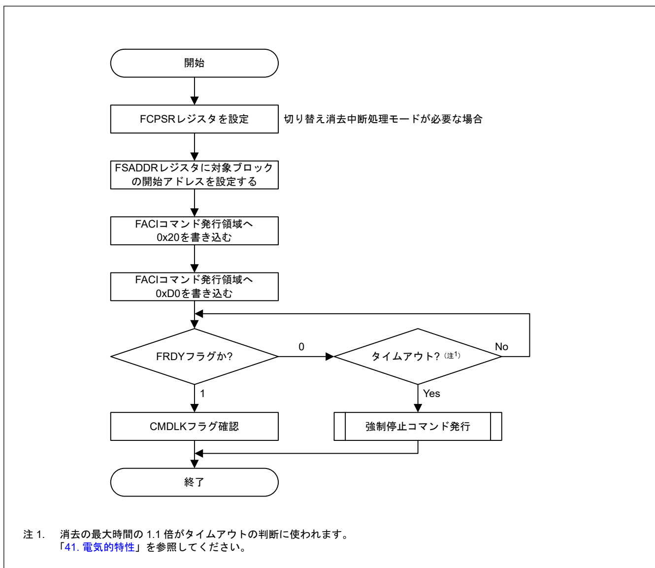
図 38.14 ブロックイレースコマンドの使用フロー
