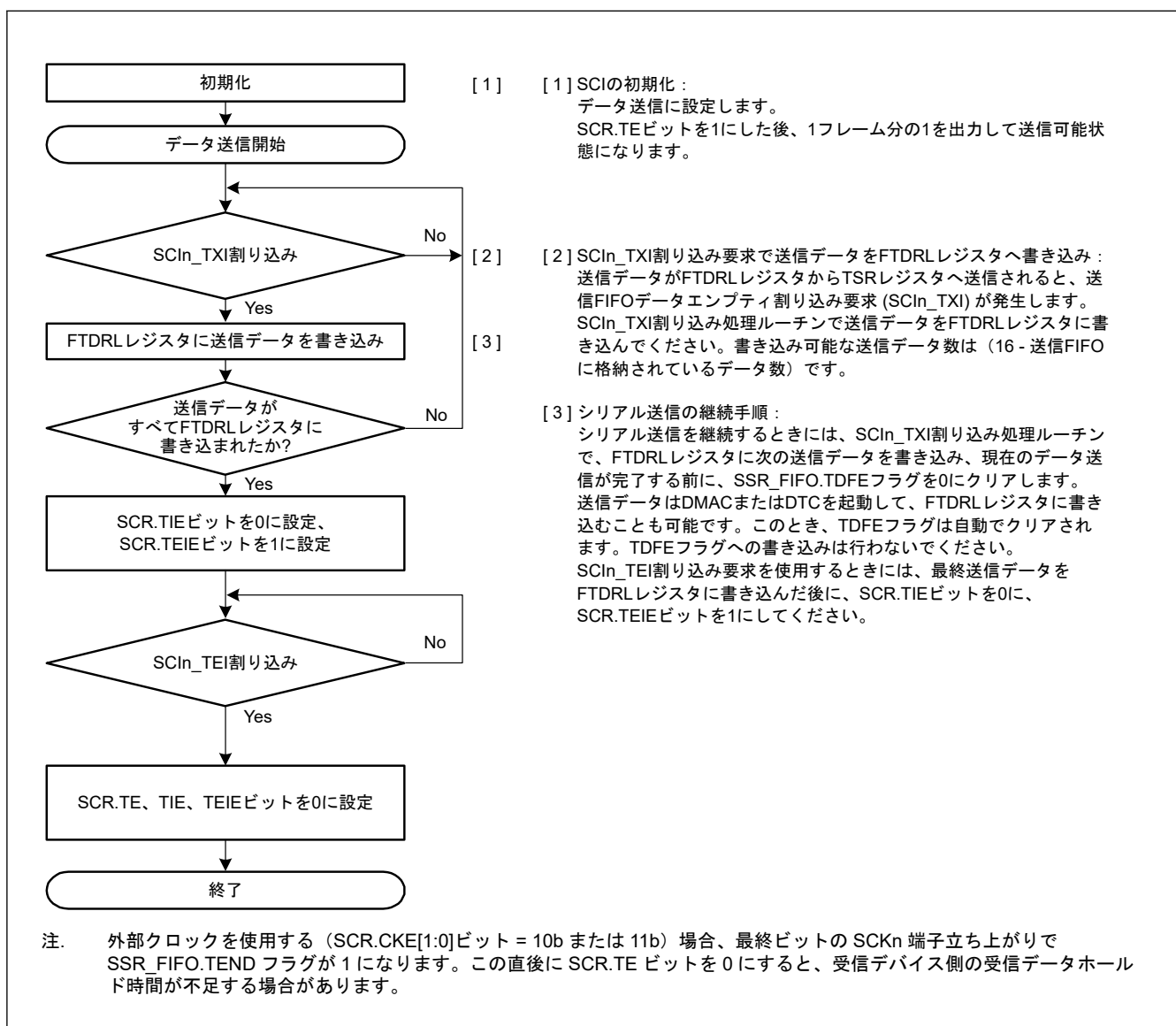
図 24.67 クロック同期式モードにおけるシリアル送信のフローチャート例 (FIFO 選択時)
