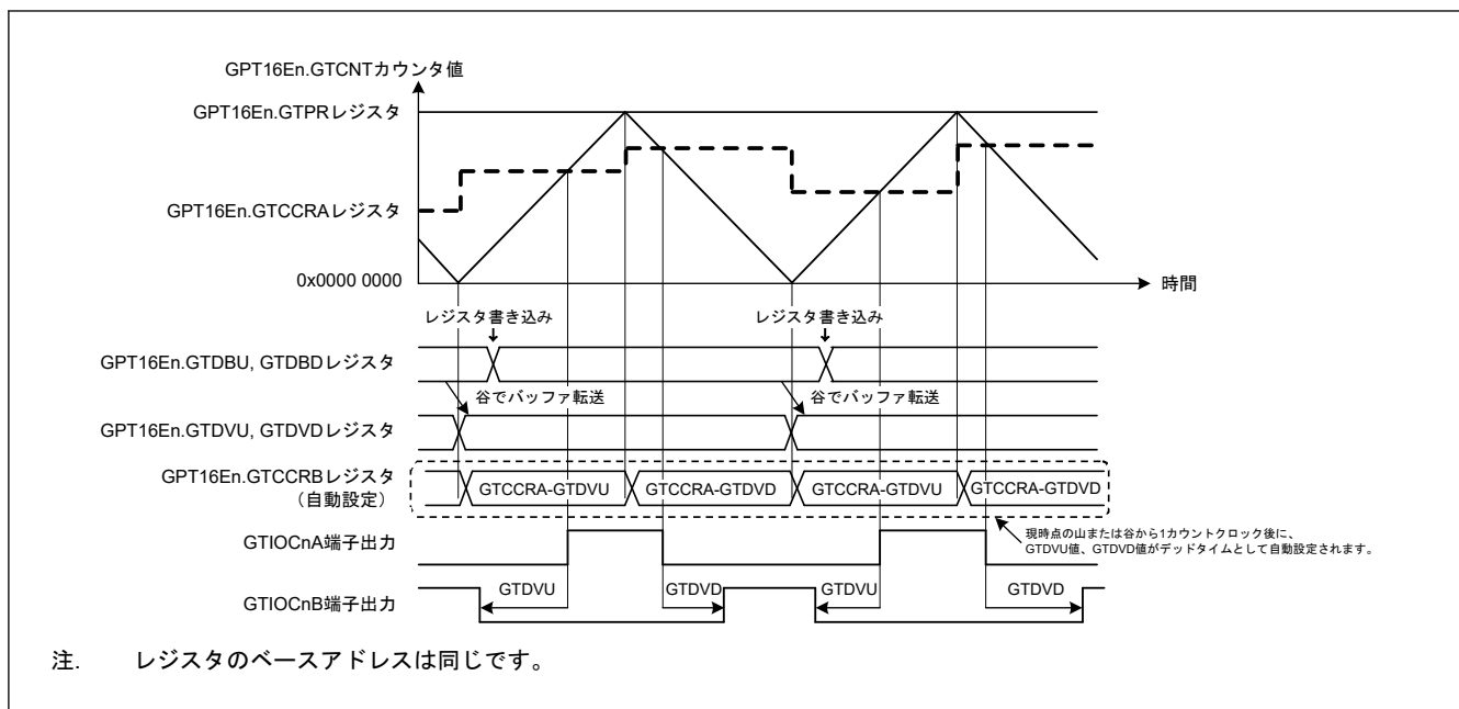
図 20.30 デッドタイム付きコンペアマッチ値の自動設定機能の動作例（三角波 PWM モード 2 または 3、GTDVU/GTDDVD レジスタはバッファ動作、アクティブ High の場合）
