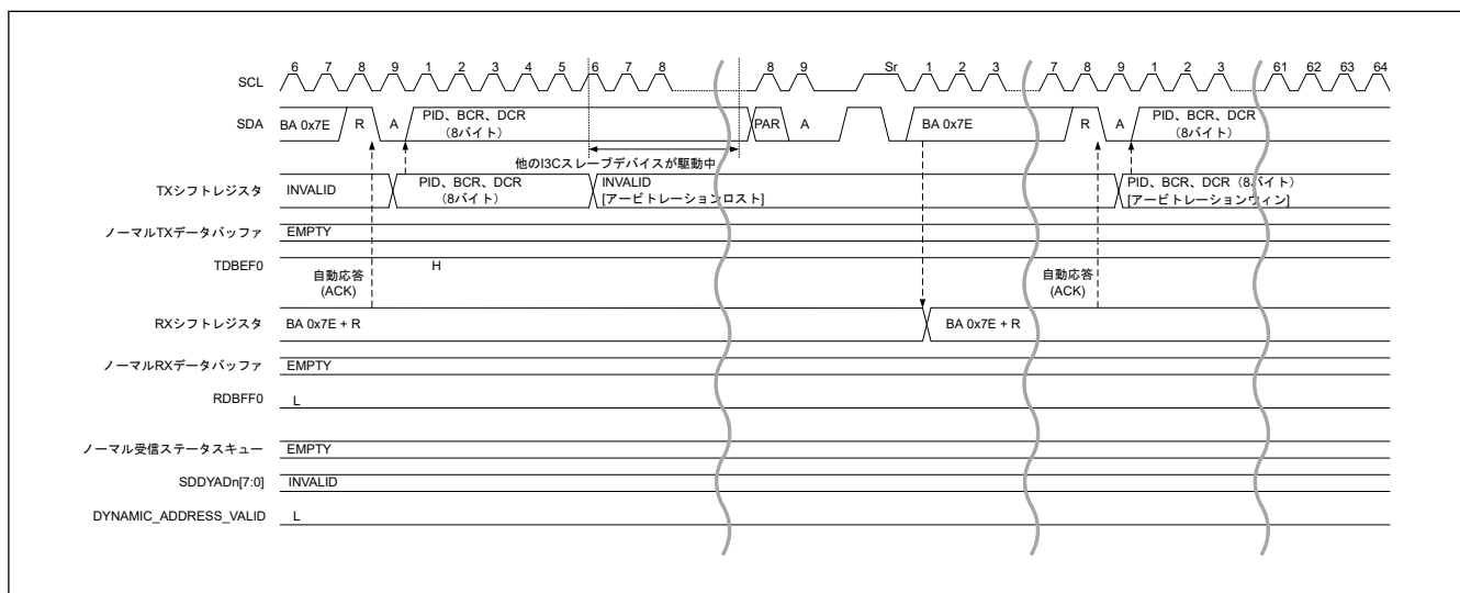
図 25.32 ダイナミックアドレス配置手順 (ENTDAA CCC) タイミング (2/3)
