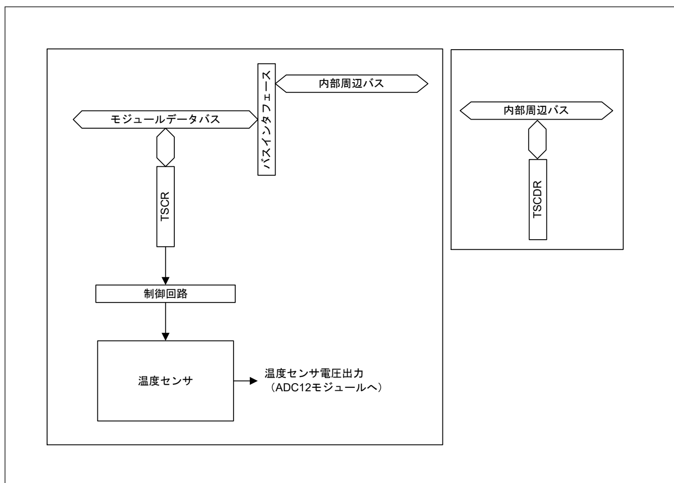
図 34.1 TSN のブロック図
