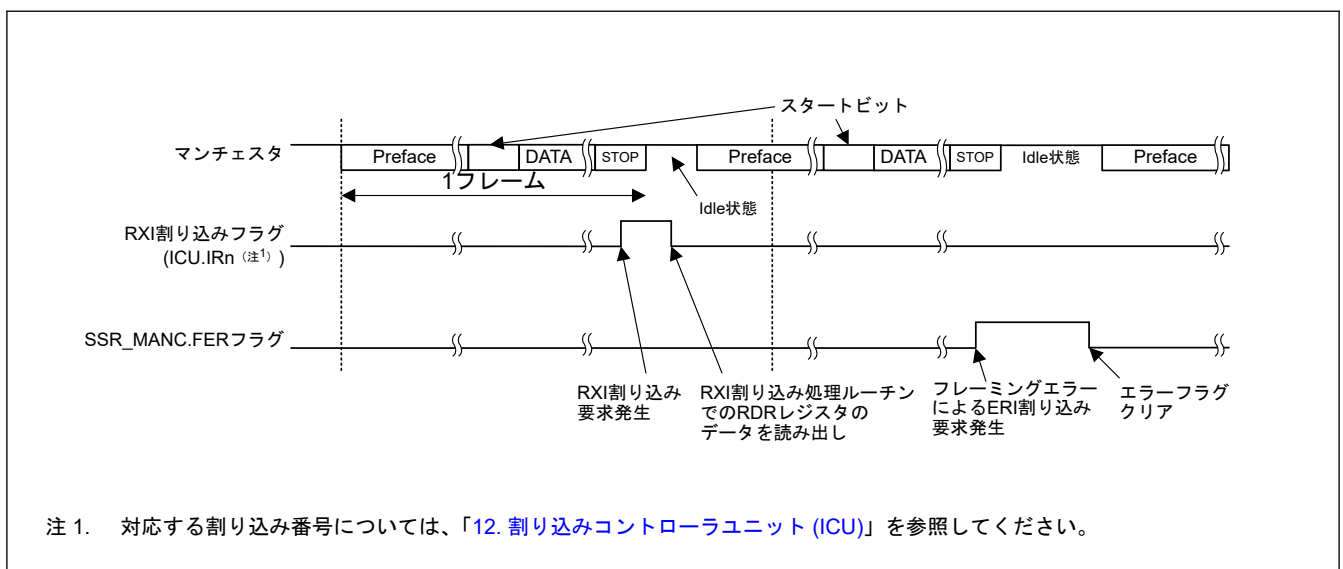
図 24.57 マンチェスタモードにおけるシリアルデータ受信の動作例 (プレフィスあり)
