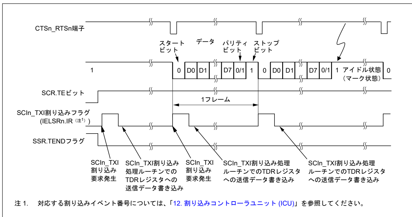
図 24.9 調歩同期式モードにおけるシリアル送信の動作例 (2) (8 ビットデータ/パリティあり/1 ストップビット /CTS 機能使用/送信開始時)
