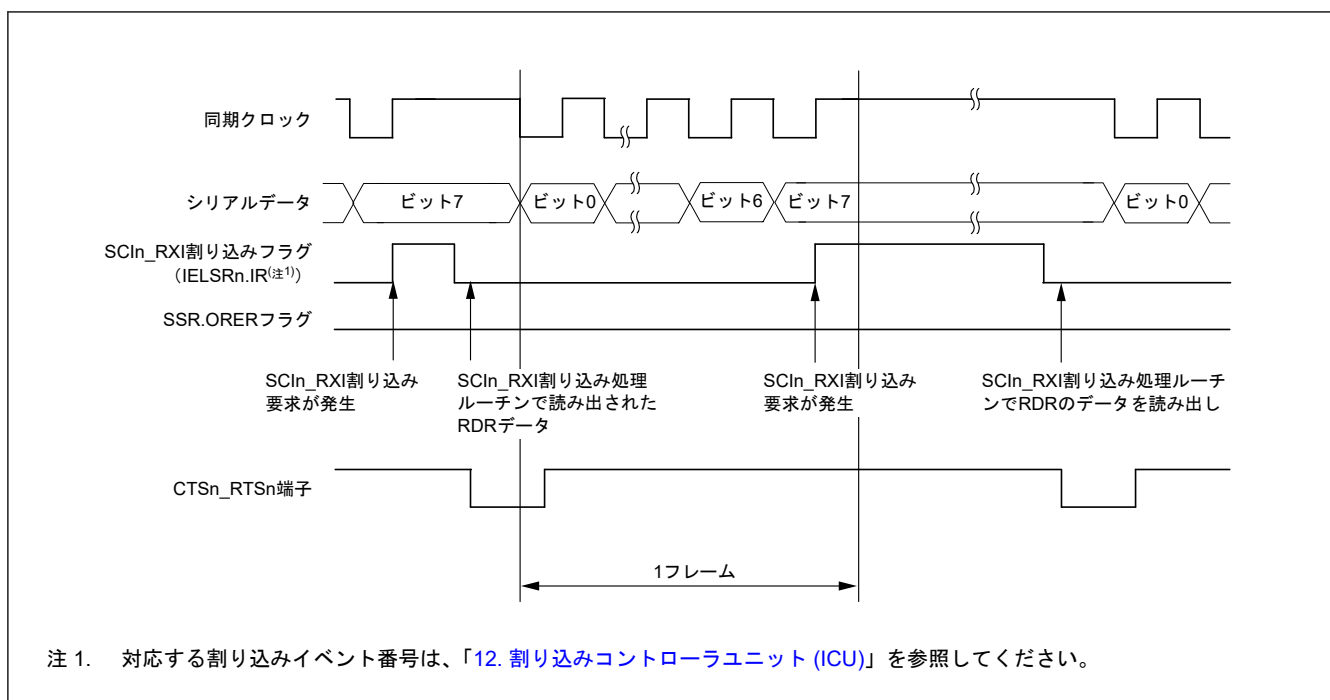
図 24.69 クロック同期式モードにおけるシリアル受信の動作例 (2) (RTS 機能を使用する場合)
