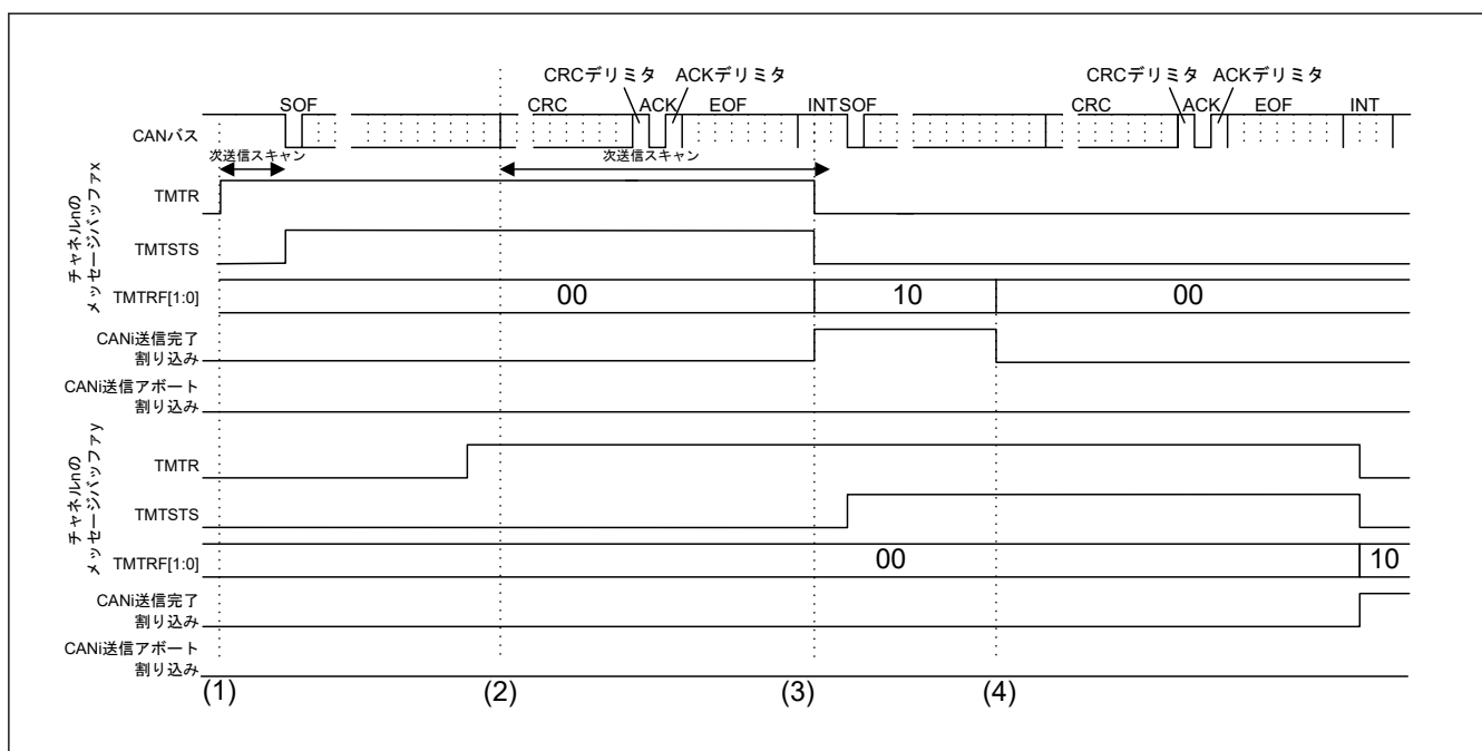
図 26.44 正常送信の要求およびフラグビットのタイミング
