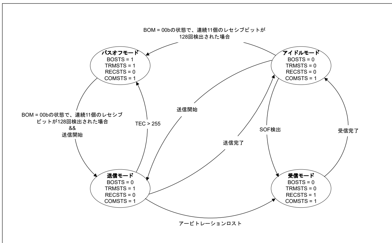
図 26.12 CAN チャンネルオペレーションモードのサブモード (BOM = 00b のときのみ)
