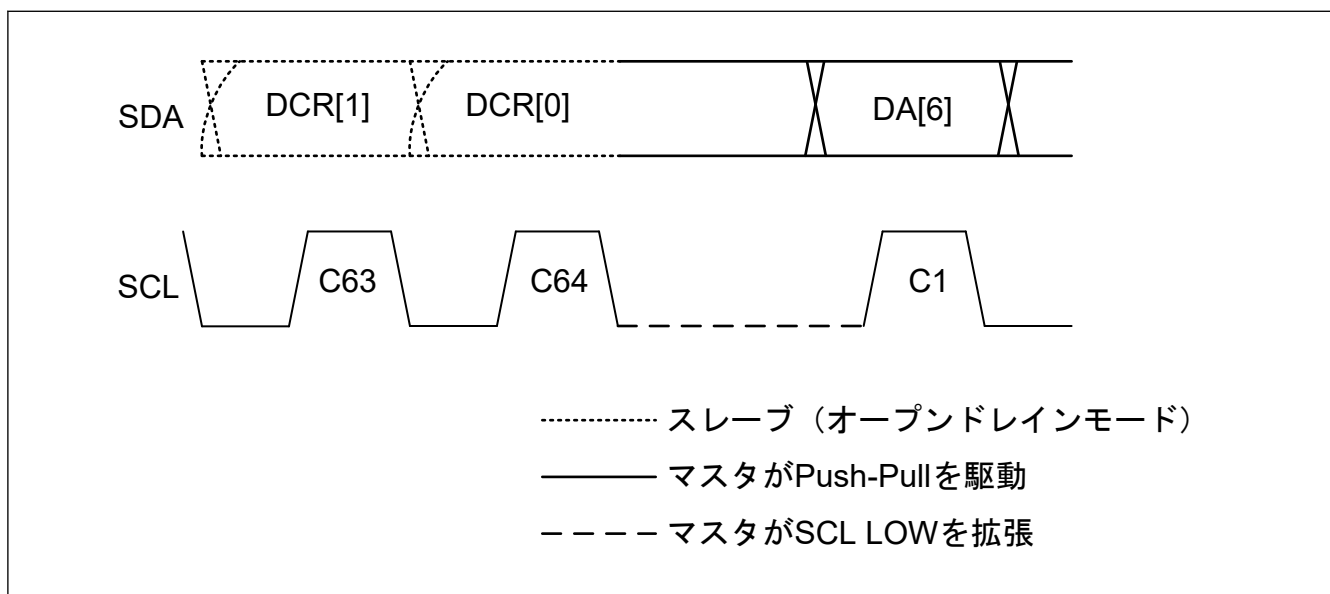
図 25.76 ダイナミックアドレスの最初のビットでのマスタクロックストール
