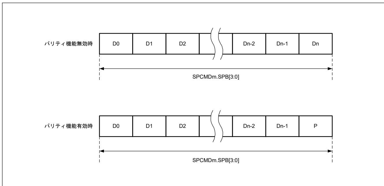
図 28.13 パリティ機能無効時と有効時のデータフォーマット
