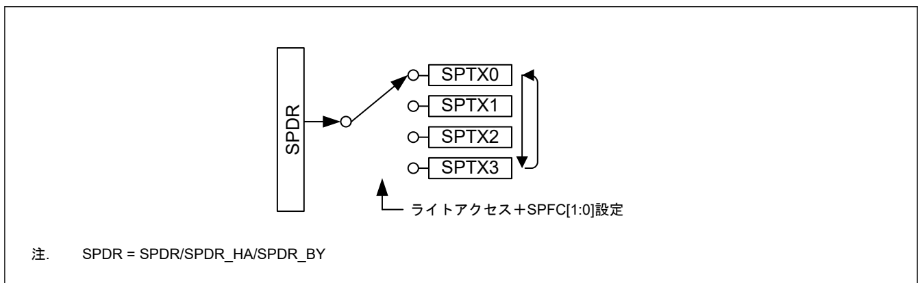
図 28.3 書き込み時の SPDR/SPDR_HA/SPDR_BY レジスタの構成図
