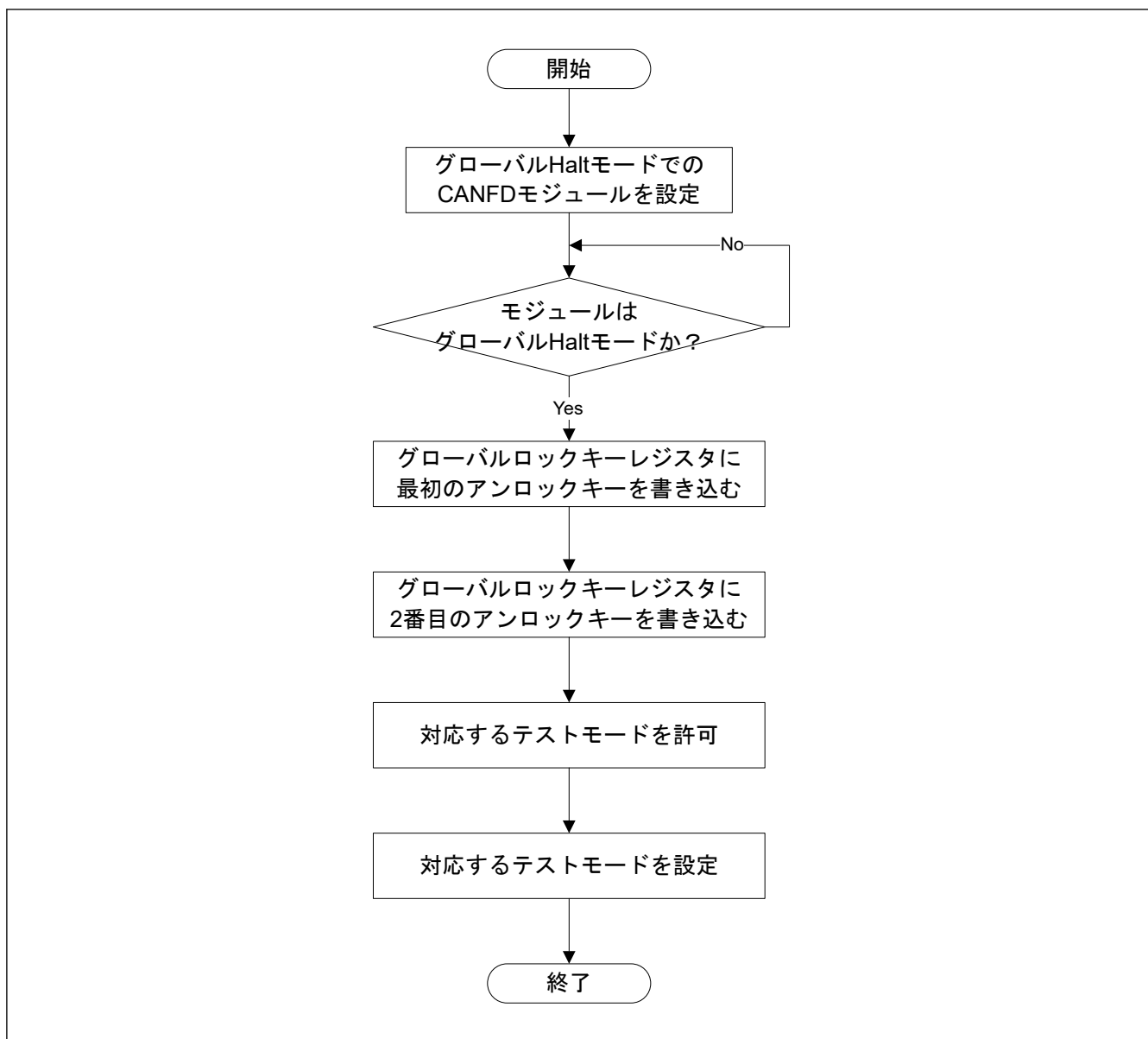
図 26.52 ソフトウェア保護のロック解除ルーチン
