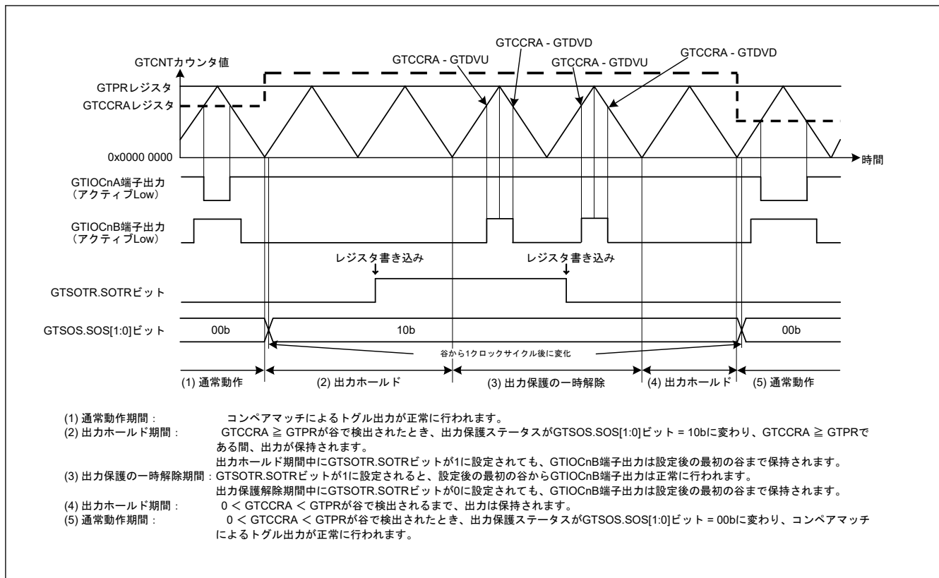
図 20.91 谷でのバッファ転送中に GTCCRA \geq GTPR となった場合の出力保護の一時解除の例（谷でのバッファ転送中に 0 < GTCCRA < GTPR に復帰、アクティブレベルは Low）（ n = 0 \sim 5 ）
