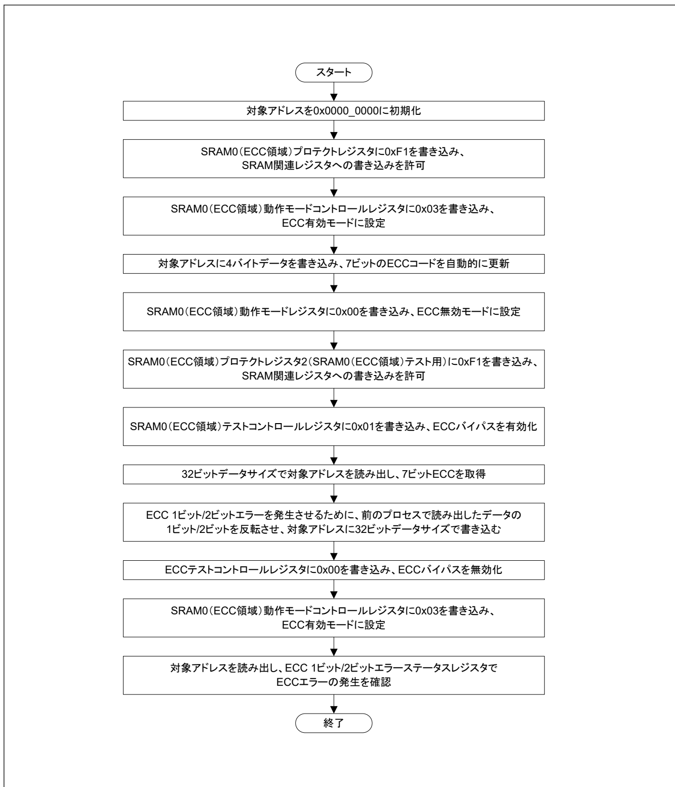
図 37.1 ECC デコーダのテスト方法
