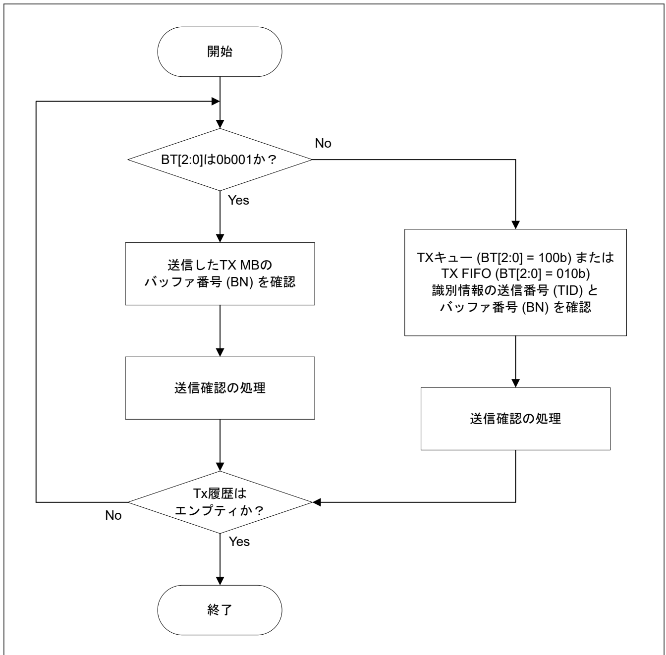
図 26.51 TX 履歴リストの処理手順
