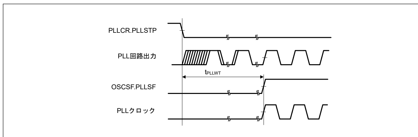
図 41.10 PLL クロック発振開始タイミング
