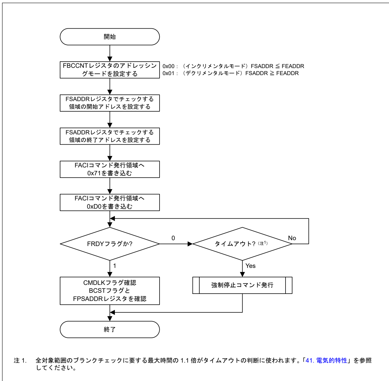
図 38.23 ブランクチェックコマンドの使用フロー
