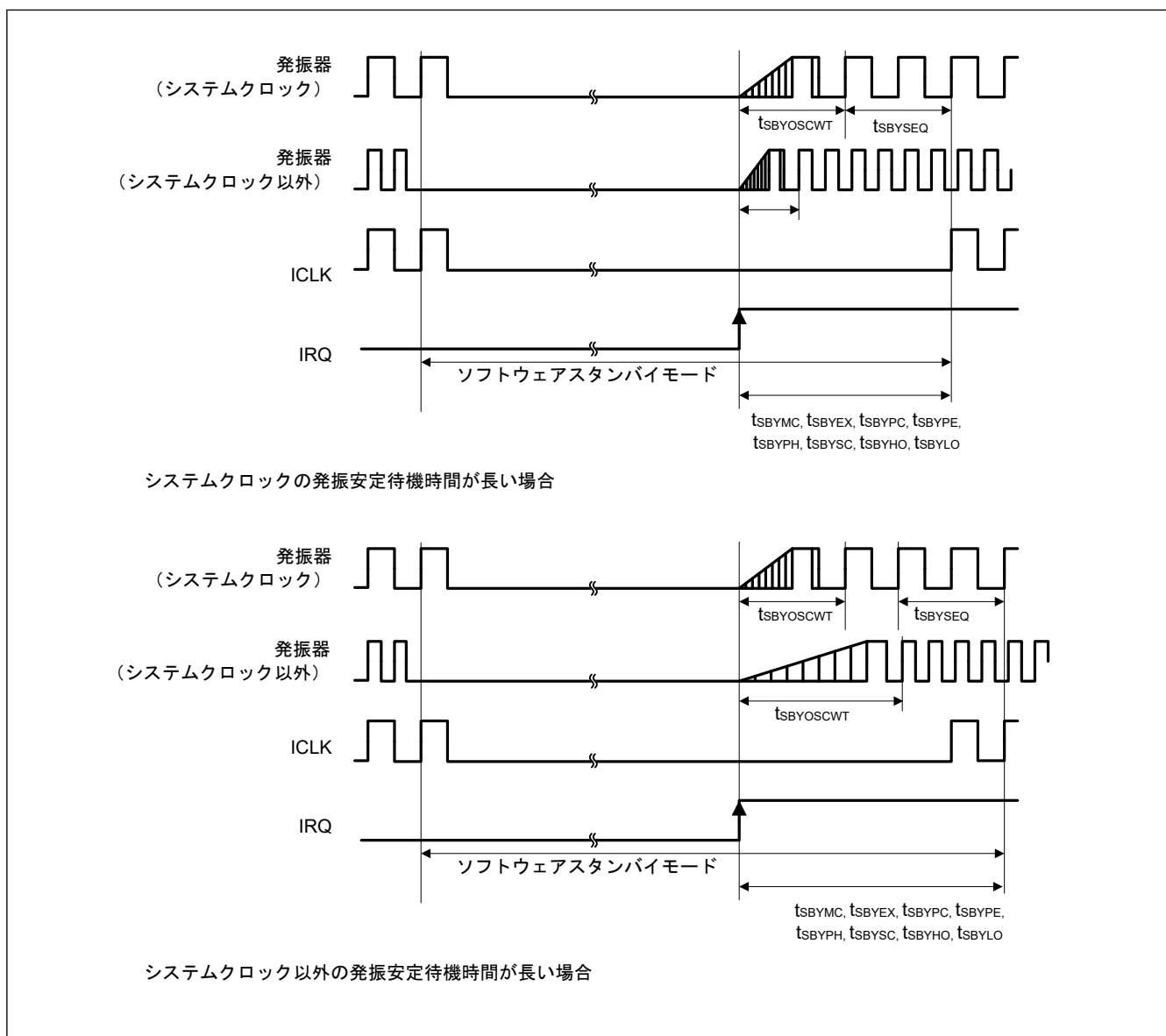
図 41.14 ソフトウェアスタンバイモード解除タイミング
