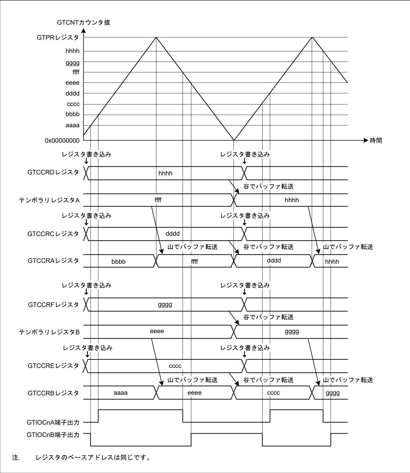
図 20.26 三角波 PWM モード 3 の動作例 (カウントスタート時に GTIOCnA 端子= Low 出力、および GTIOCnB 端子= High 出力、GTCCRA/GTCCRB レジスタのコンペアマッチ時にトグル出力、周期の終わりで出力保持の場合)
