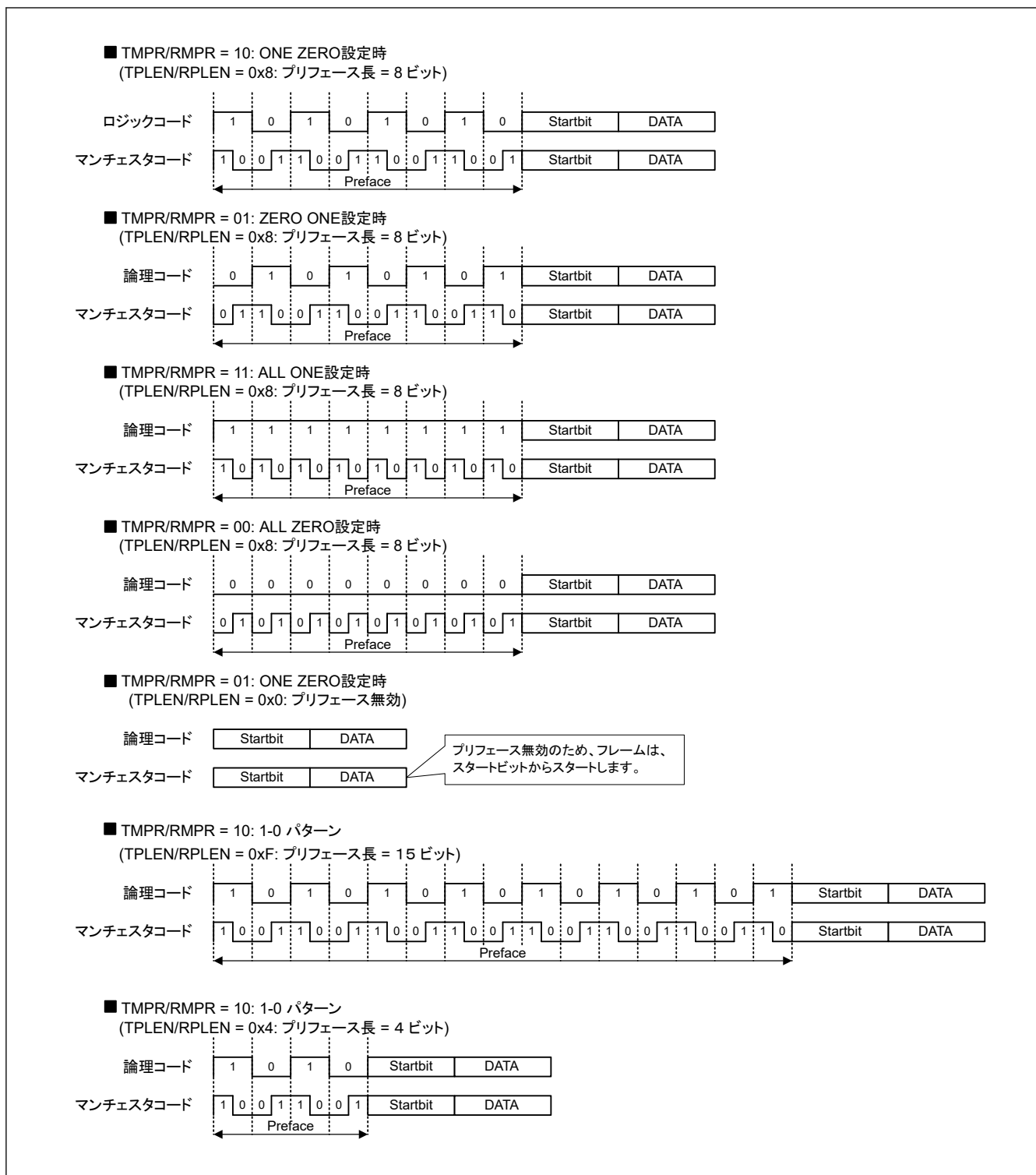
図 24.48 プレフィスパターンの設定例
