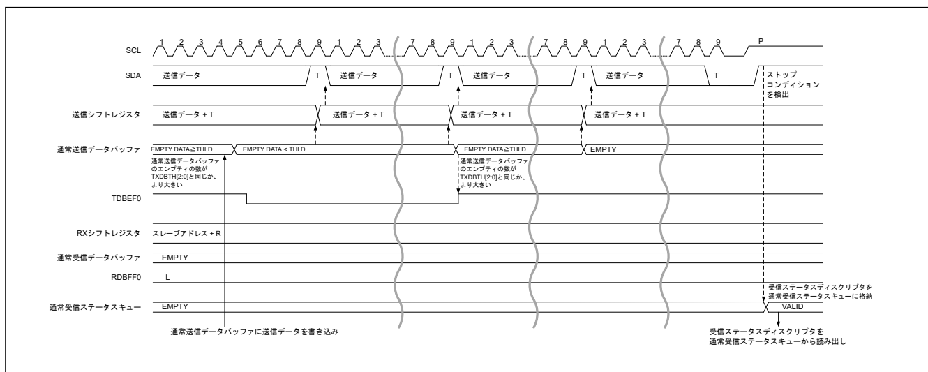
図 25.40 SDR データ読み出し転送タイミング (2/2)
