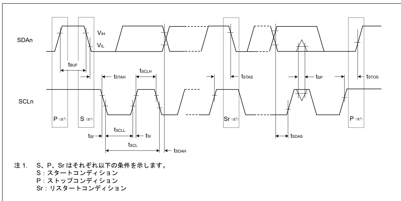
図 41.41 I 2 C バスインタフェース入出力タイミング
