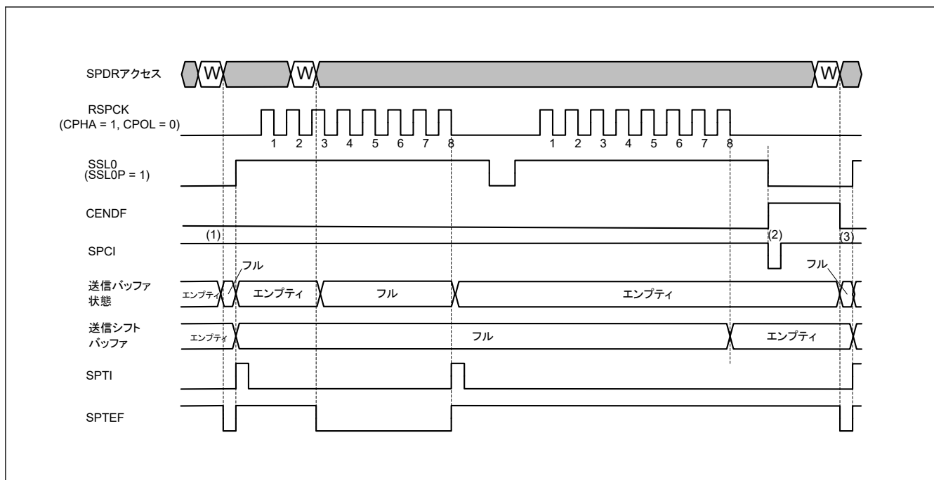
図 28.32 通信終了割り込み動作例 (SPI 動作時の送受信/送信スレーブモード)
