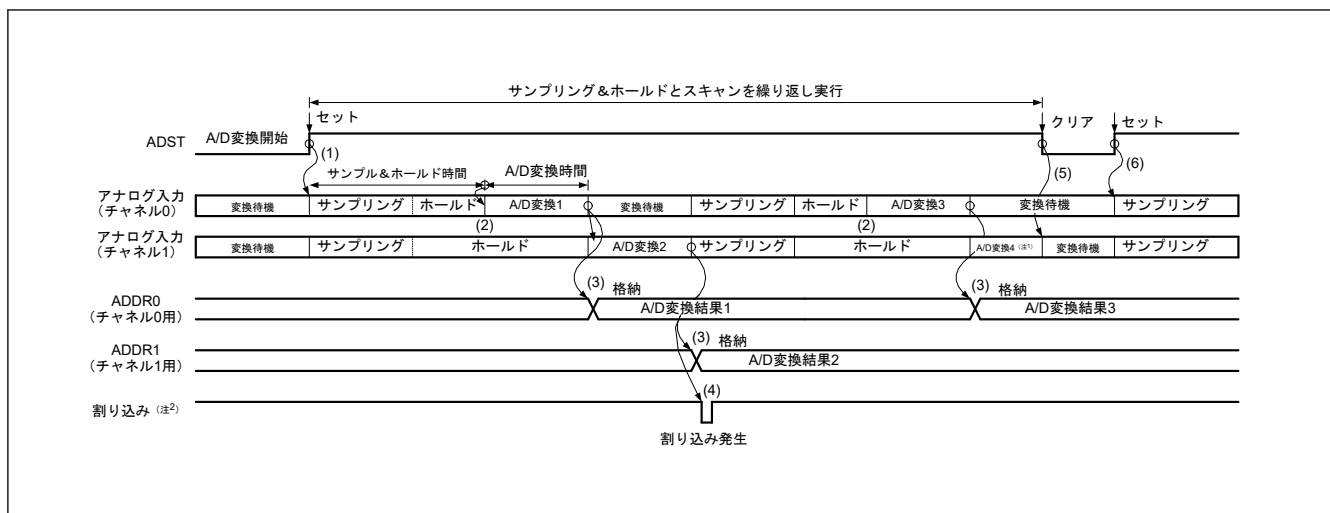
図 32.17 連続スキャンモードの動作例（チャンネル専用サンプル&ホールド回路を使用し、AN000 と AN001 を選択した場合）
