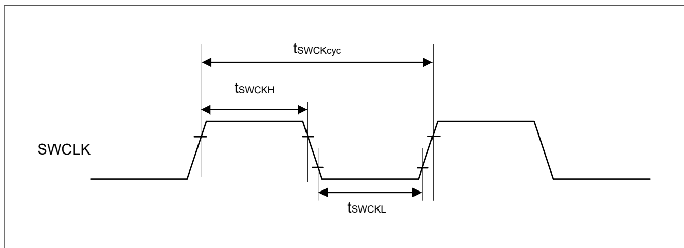
図 41.60 SWD SWCLK タイミング
