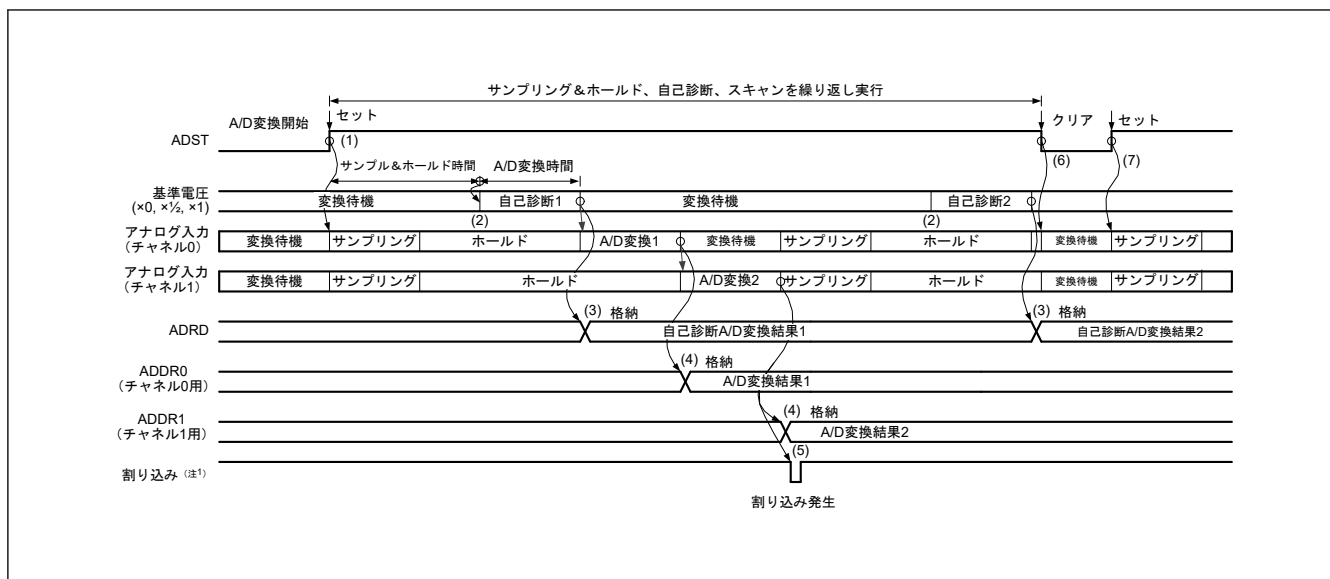
図 32.20 連続スキャンモードの動作例（チャンネル専用サンプル&ホールド回路を使用し、自己診断で AN000 と AN001 を選択した場合）
