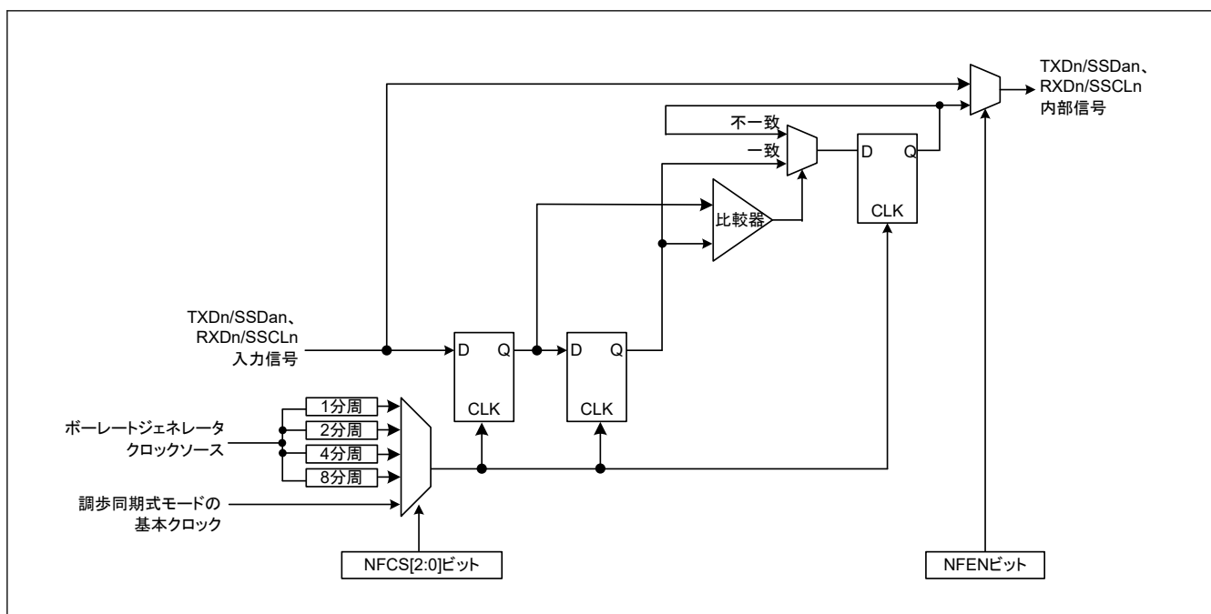
図 24.98 デジタルノイズフィルタ回路のブロック図
