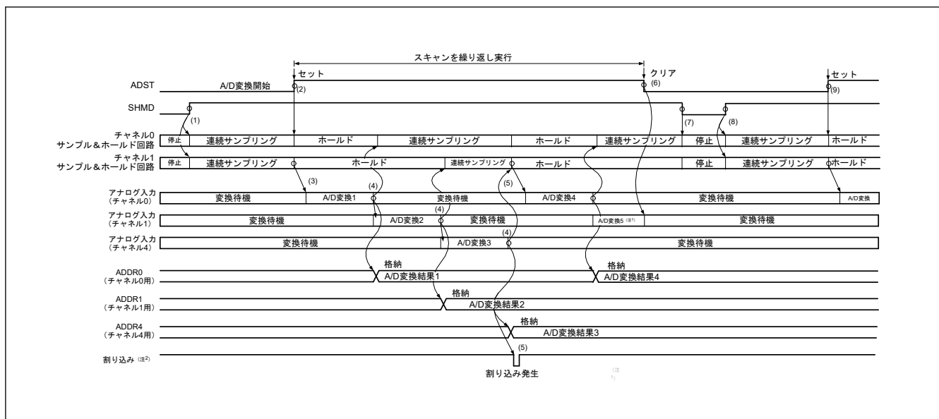
図 32.18 連続スキャンモードの動作例 (チャンネル専用サンプル&ホールド回路を使用し、AN000、AN001、AN004 を選択し、連続サンプリングを有効にした場合)
