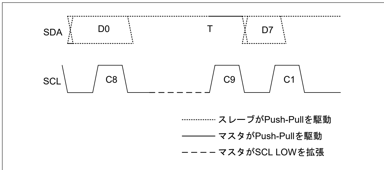
図 25.75 次の読み出しデータの前の T ビットでのマスタクロックストール
