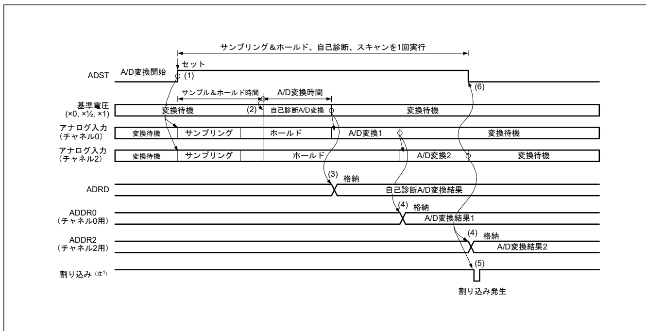
図 32.11 シングルスキャンモードの動作例（チャンネル専用サンプル&ホールド回路を使用し、自己診断で AN000 と AN002 を選択し、連続サンプリングを無効にした場合）
