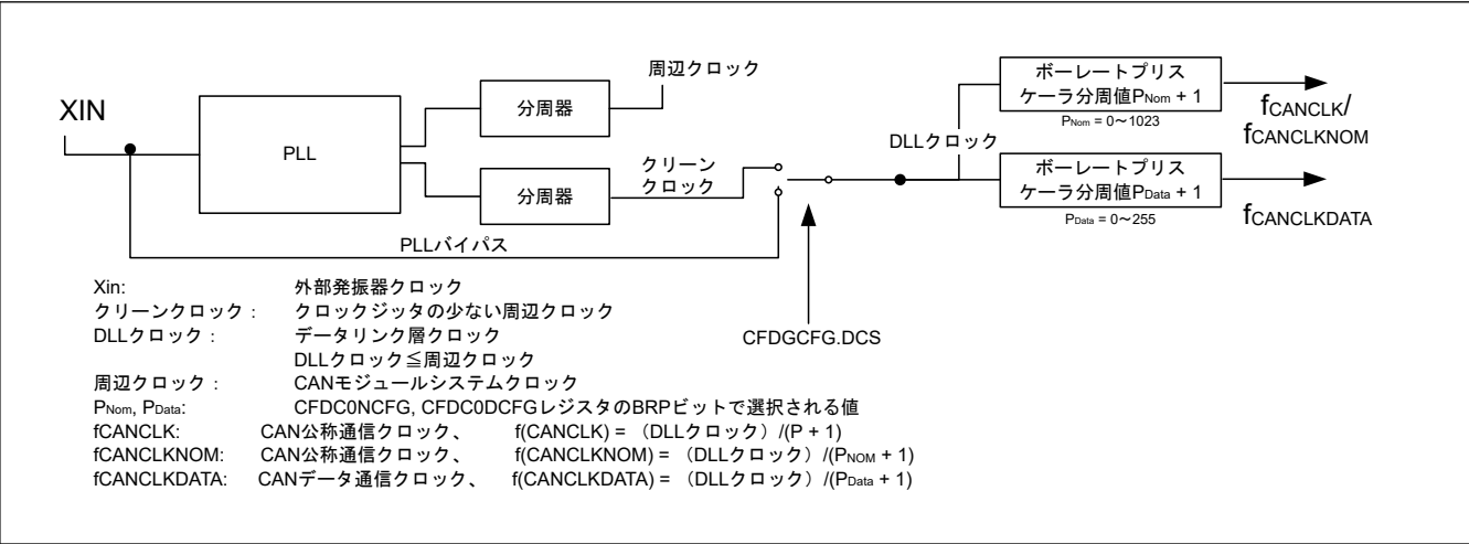
図 26.16 CAN チャネルの通信クロックを生成する回路のブロック図
