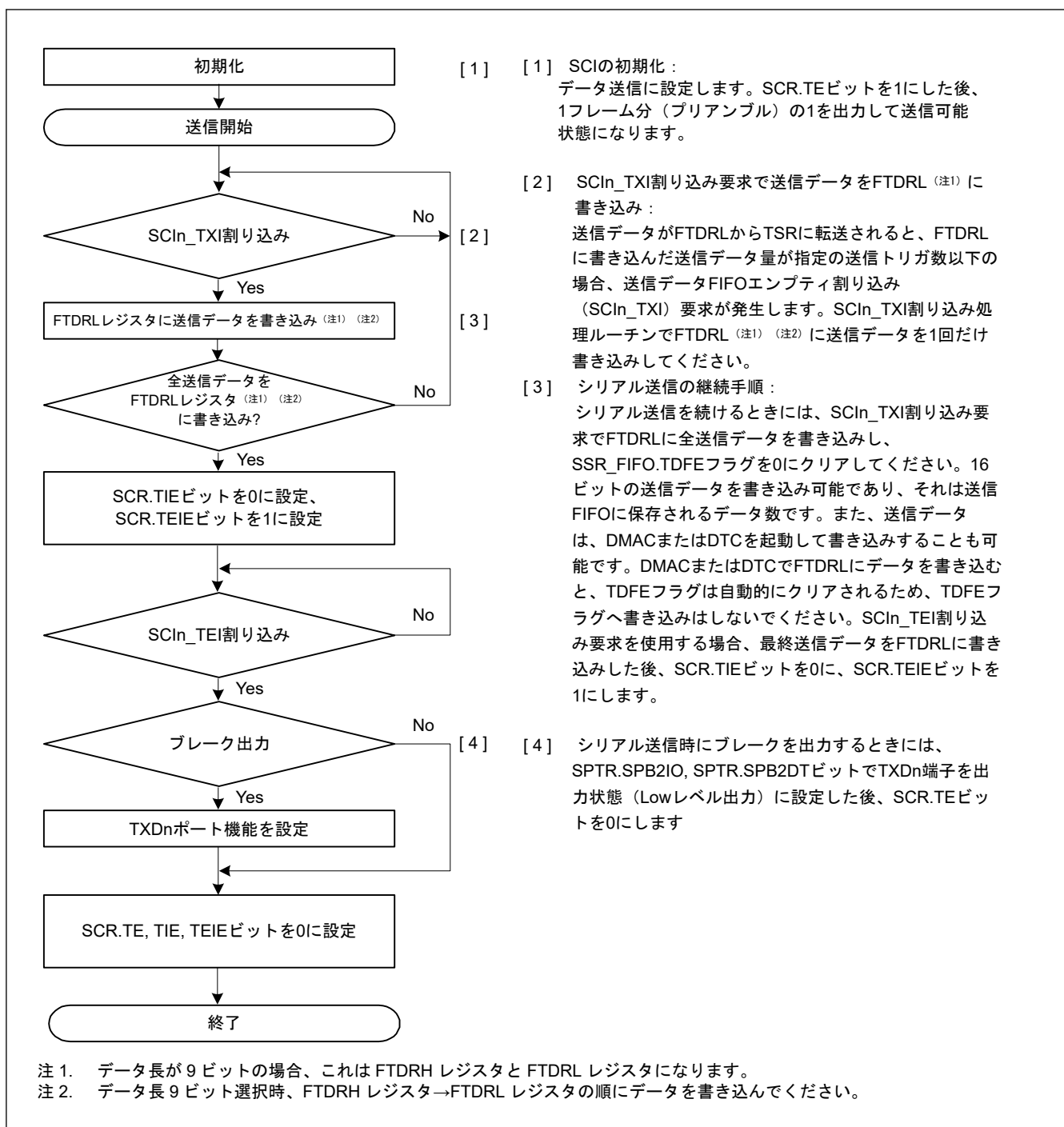
図 24.14 調歩同期式モードにおけるシリアル送信のフローチャート例（FIFO 選択時）
