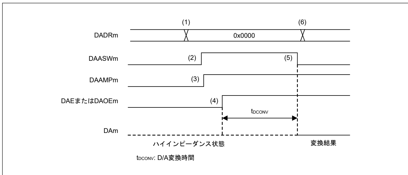
図 33.5 出力アンプを使用した DAC12 の初期化フロー例
