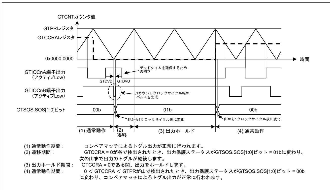
図 20.86 山でのバッファ転送中に GTCCRA が 0 になったときの出力保護機能の動作例 (山でのバッファ転送中に 0 < \text{GTCCRA} < \text{GTPR} に復帰、アクティブレベルは Low) ( n = 0 \sim 5 )
