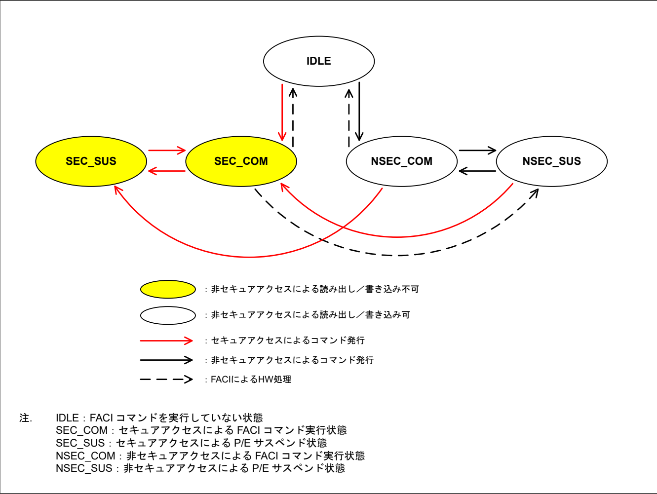
図 38.33 FACI コマンド動作中の保護状態
