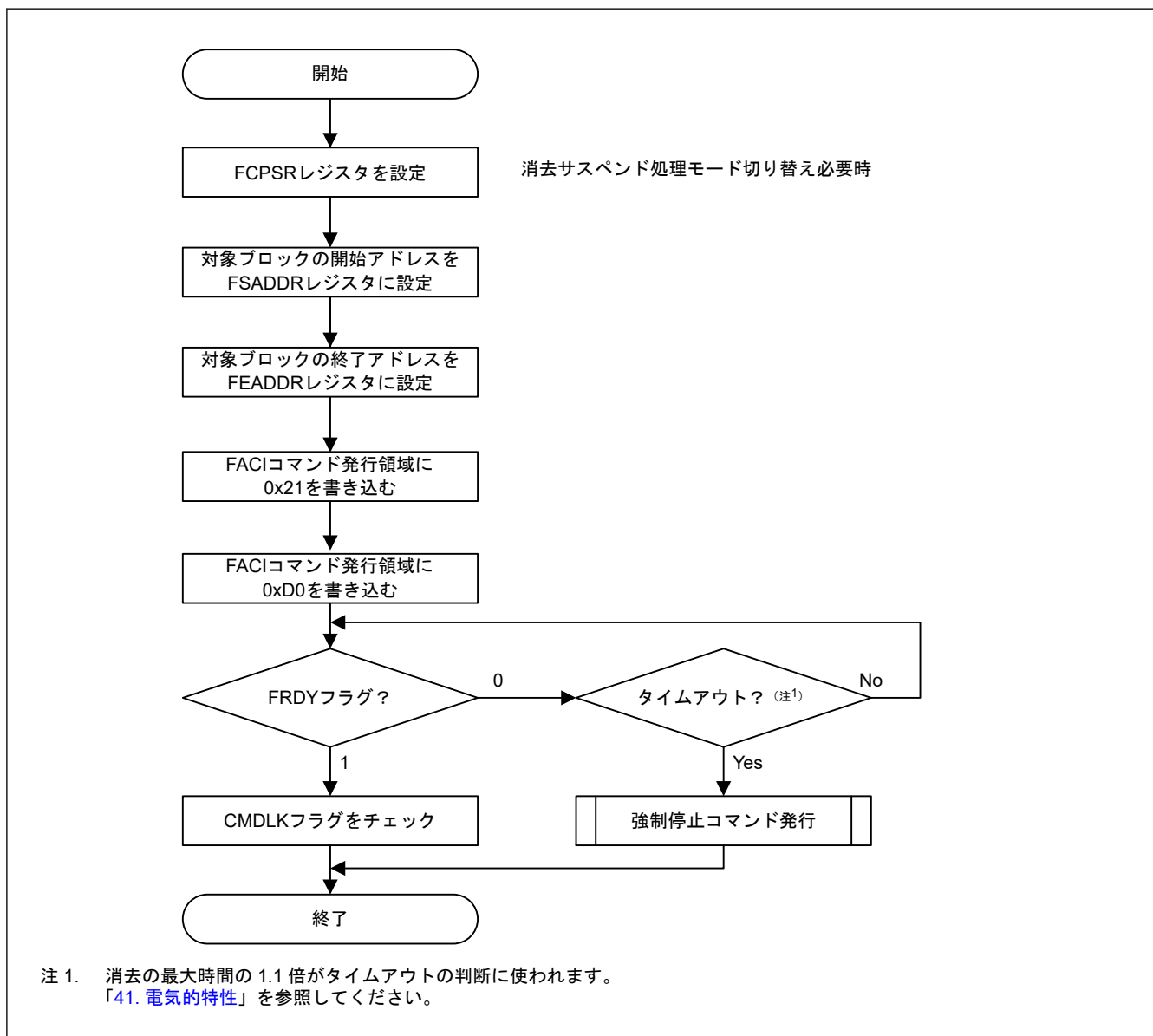
図 38.15 マルチブロックコマンドの使用フロー
