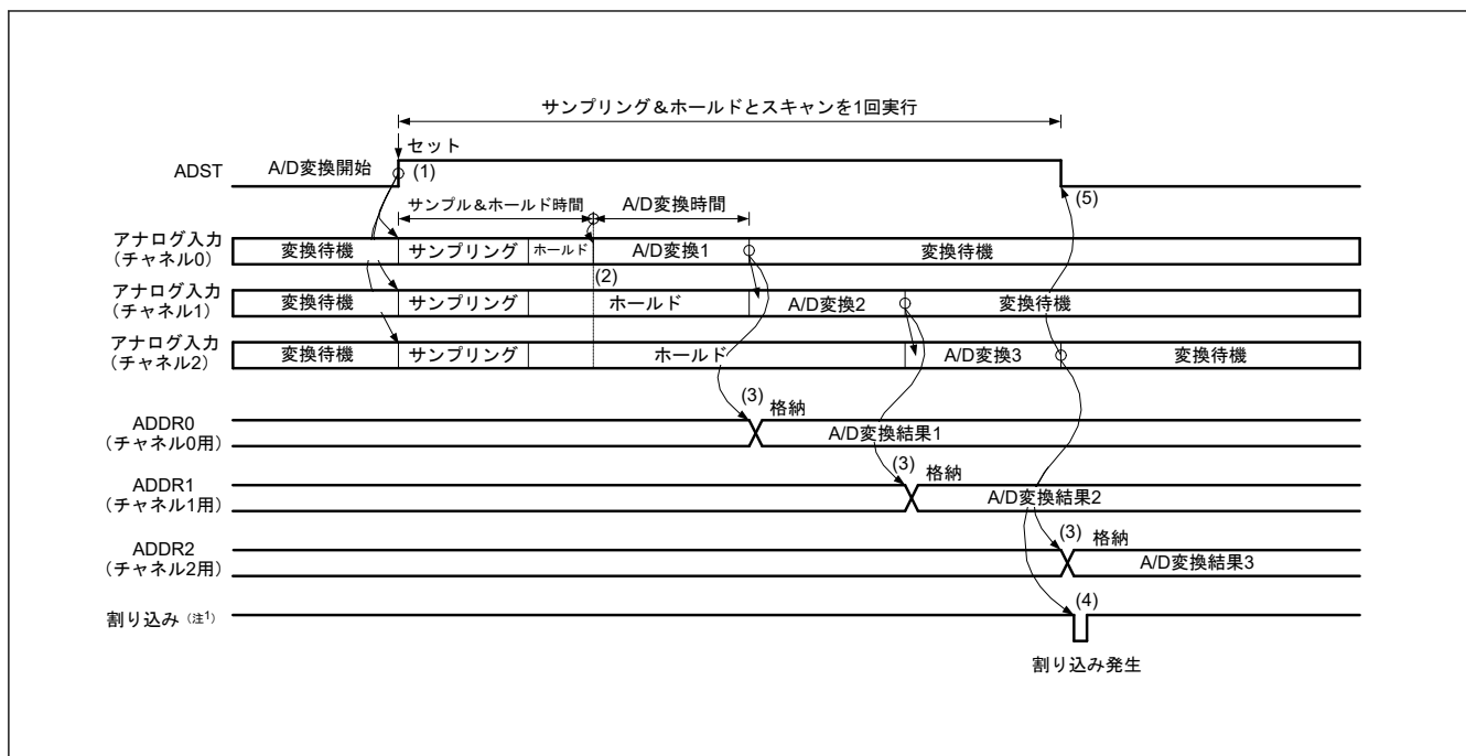
図 32.8 シングルスキャンモードの動作例 (チャンネル専用サンプル&ホールド回路を使用し、AN000～AN002 を選択した場合)
