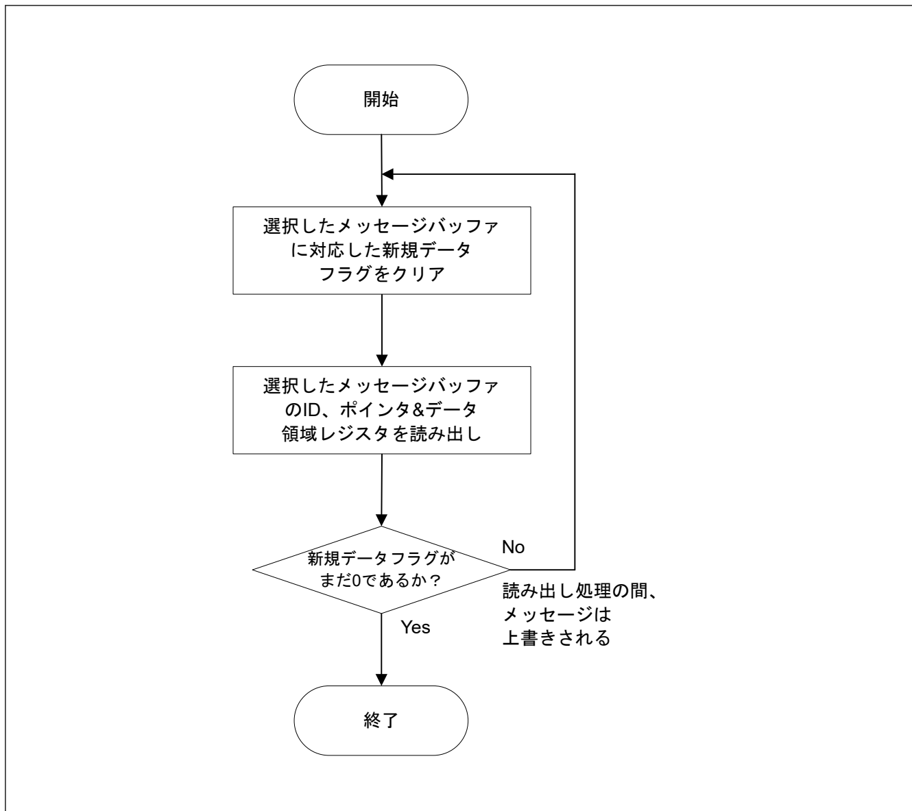
図 26.38 RX メッセージバッファの読み出しフロー
