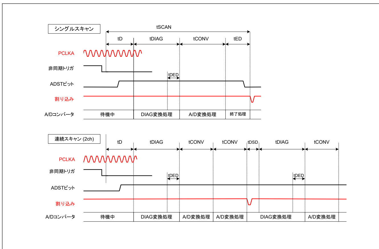
図 32.35 スキャン変換のタイミング (非同期トリガ入力 (ADTRG0) 起動の場合)
