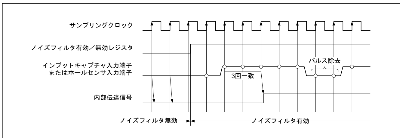
図 20.77 ノイズフィルタのタイミング
