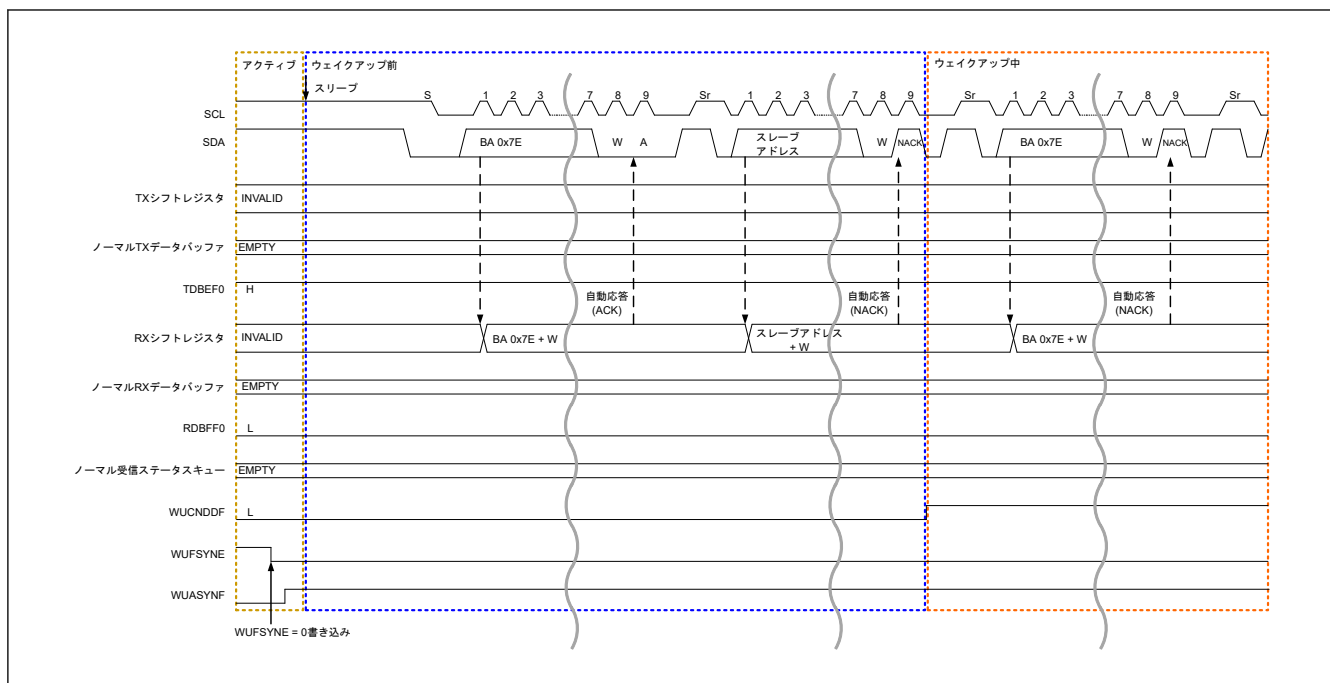
図 25.108 I3C スレーブウェイクアップ動作 (1/2)
