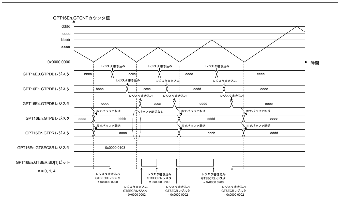
図 20.79 バッファ動作禁止の複数チャネルの動作例 (三角波、ダブルバッファ動作)
