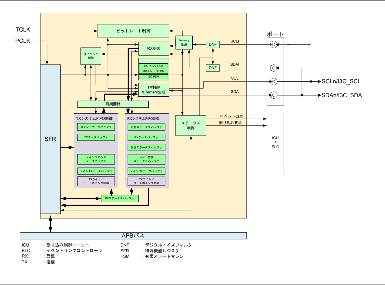
図 25.1 I3C ブロック図
