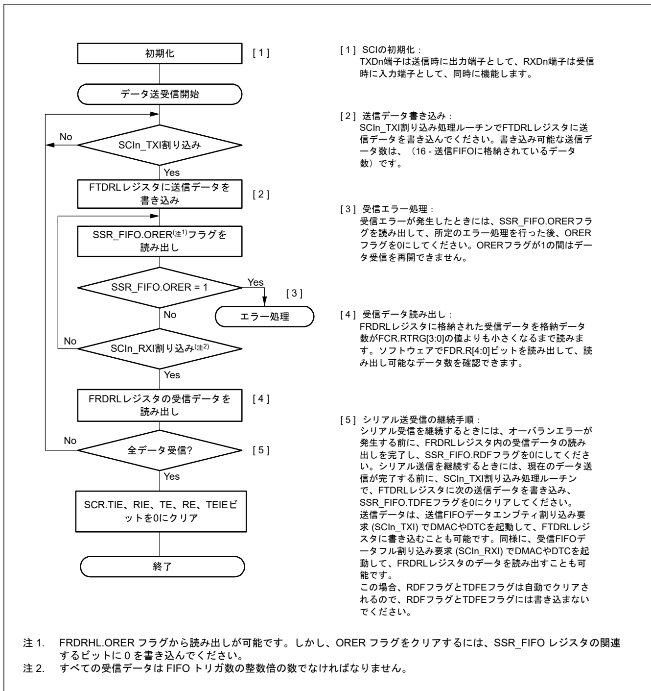
図 24.73 クロック同期式モードにおけるシリアル同時送受信動作のフローチャート例 (FIFO 選択時)
