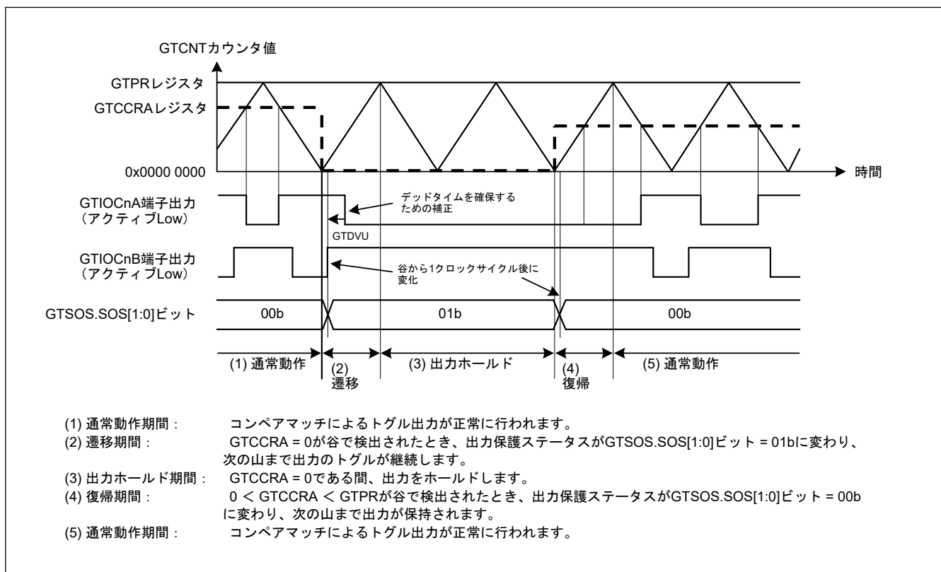
図 20.83 谷でのバッファ転送中に GTCCRA が 0 になったときの出力保護機能の動作例（谷でのバッファ転送中に 0 &lt; GTCCRA &lt; GTPR に復帰、アクティブレベルは Low）(n = 0~5)
