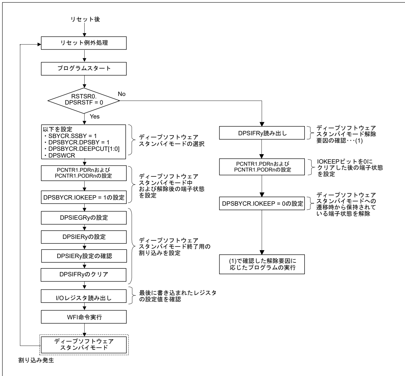
図 10.9 ディープソフトウェアスタンバイモード使用時のフローチャート例
