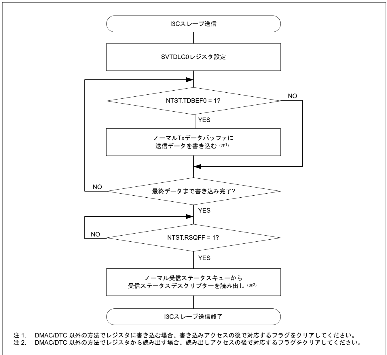
図 25.127 I3C スレーブ送信のフローチャート例 (通常 FIFO バッファ転送)
