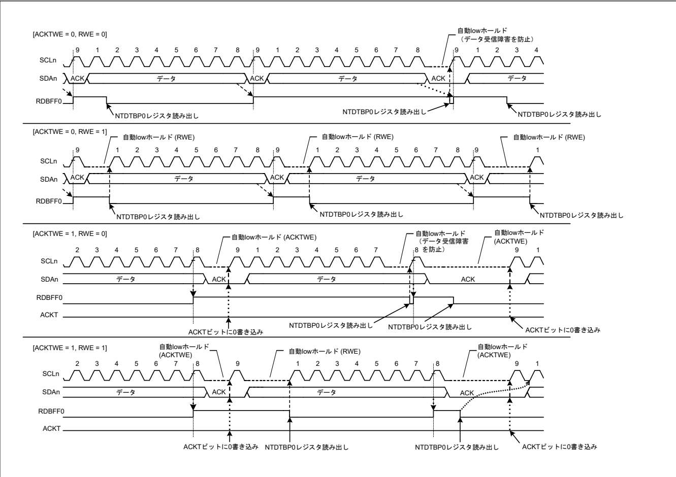
図 25.72 受信モード時の自動 Low ホールド動作（ACKTWE および RWE ビットを使用）
