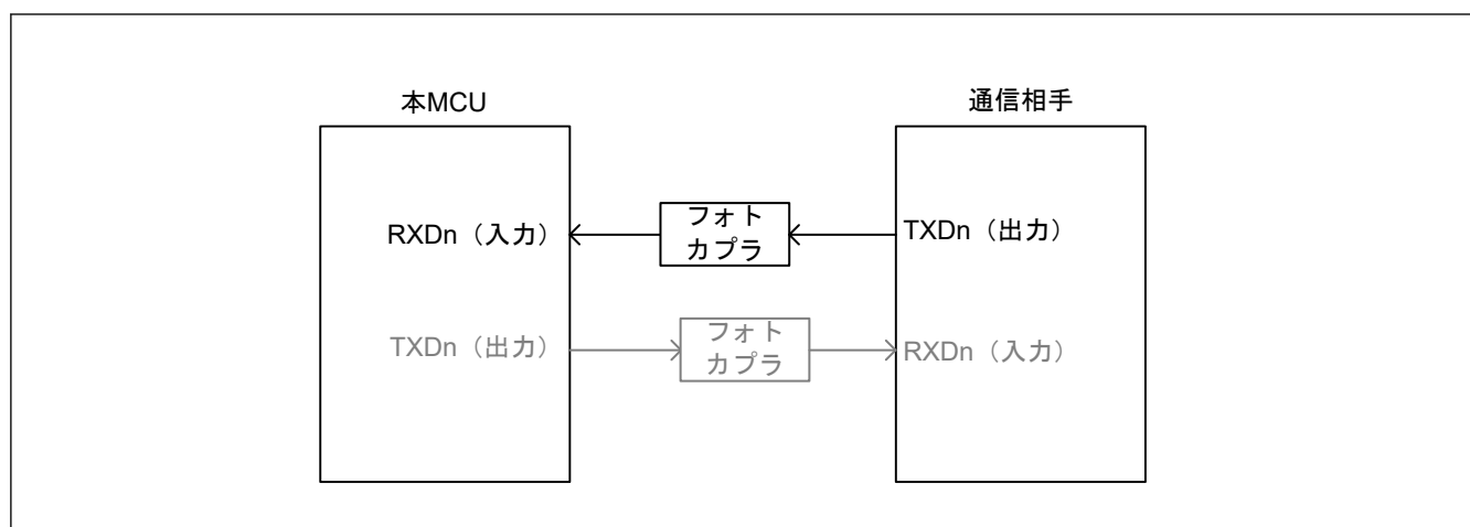
図 24.28 フォトカプラを通過する受信のブロック図イメージ
