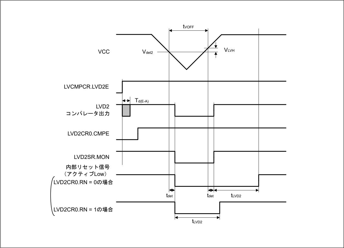
図 41.58 電圧検出回路タイミング ( V_{det2} )
