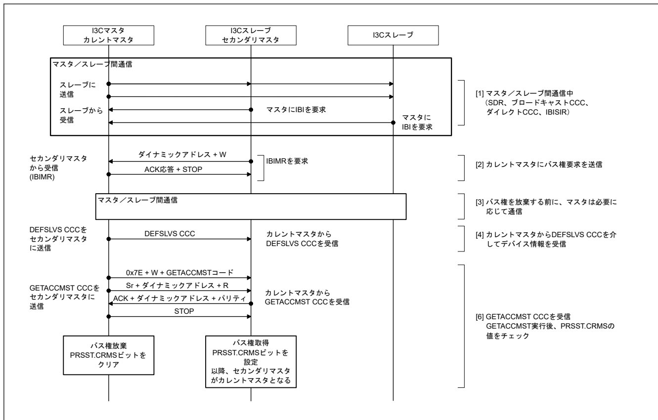
図 25.45 I3C スレーブバス権処理フロー
