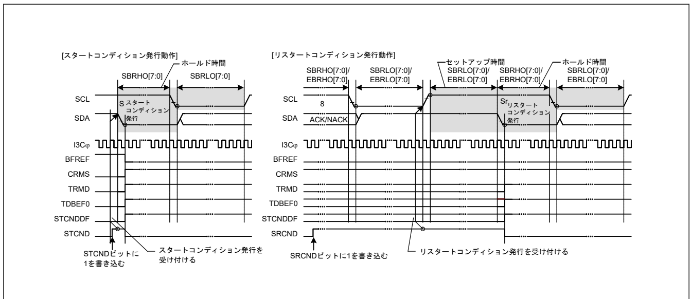
図 25.56 スタートコンディション／繰り返しのスタートコンディション発行動作タイミング (STCND、SRCND ビット)
