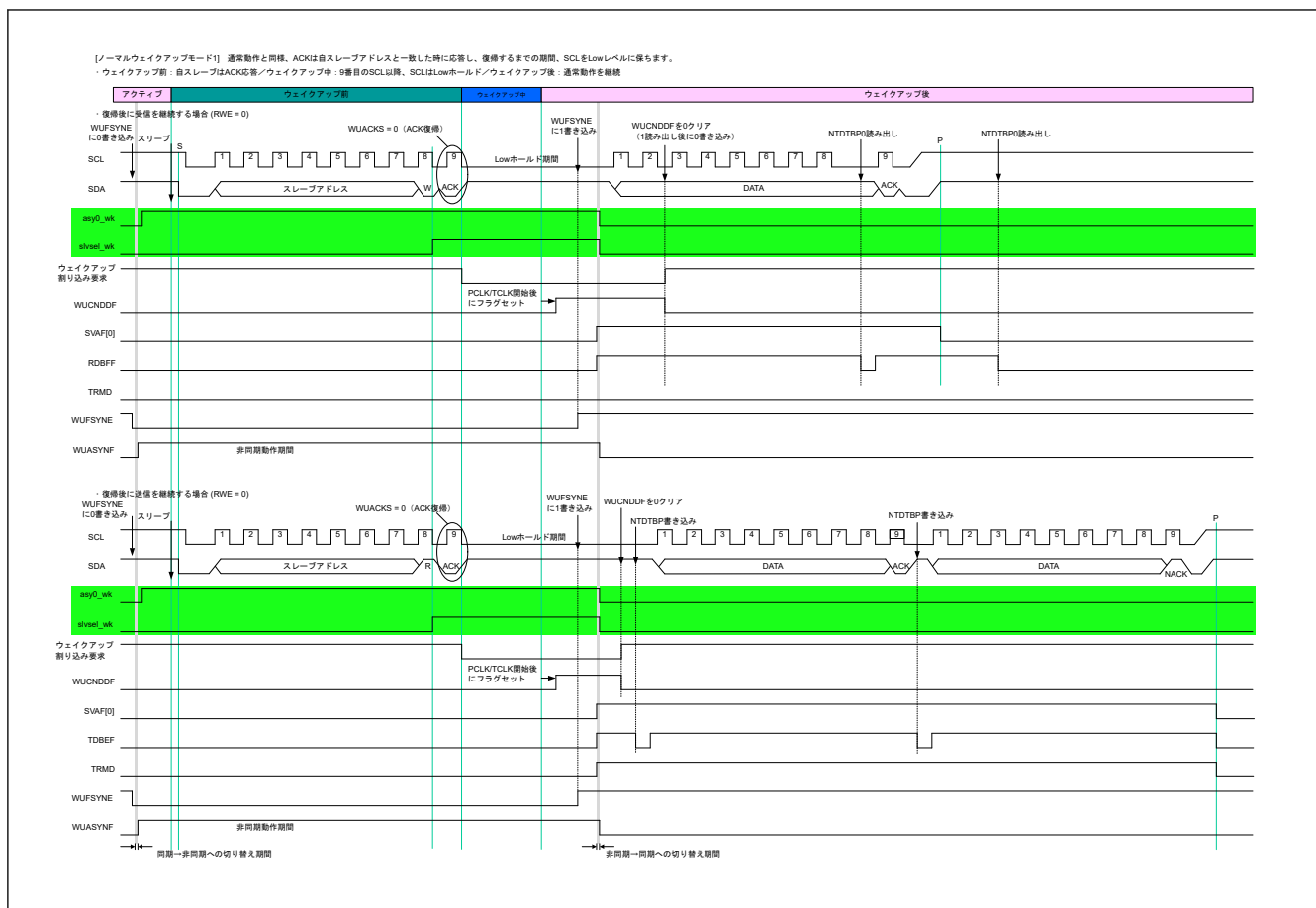
図 25.101 ノーマル WU モード1のタイミング
