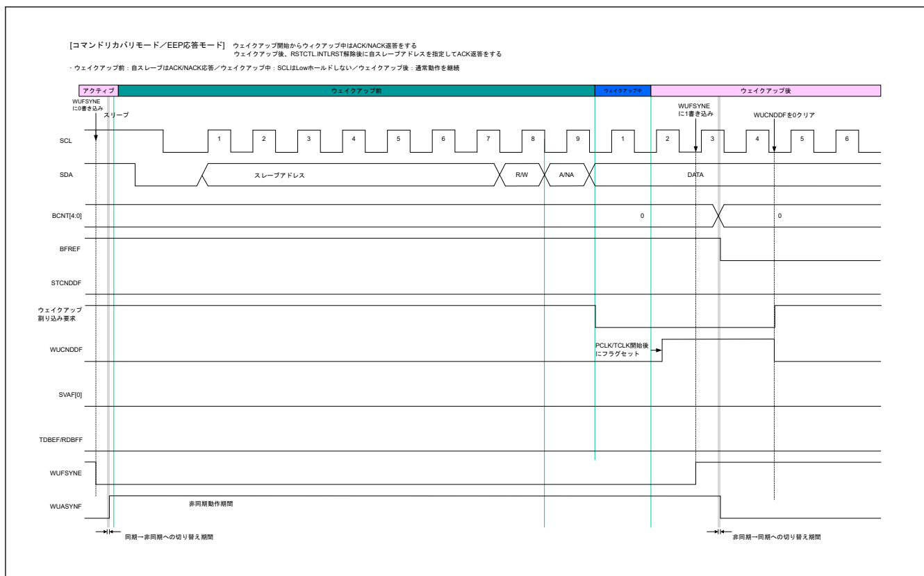
図 25.106 コマンドリカバリモードと EEP 応答モードのタイミング
