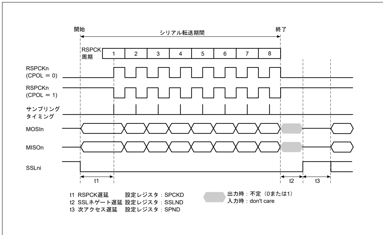
図 28.24 SPI 転送フォーマット (CPHA = 0 の場合)
