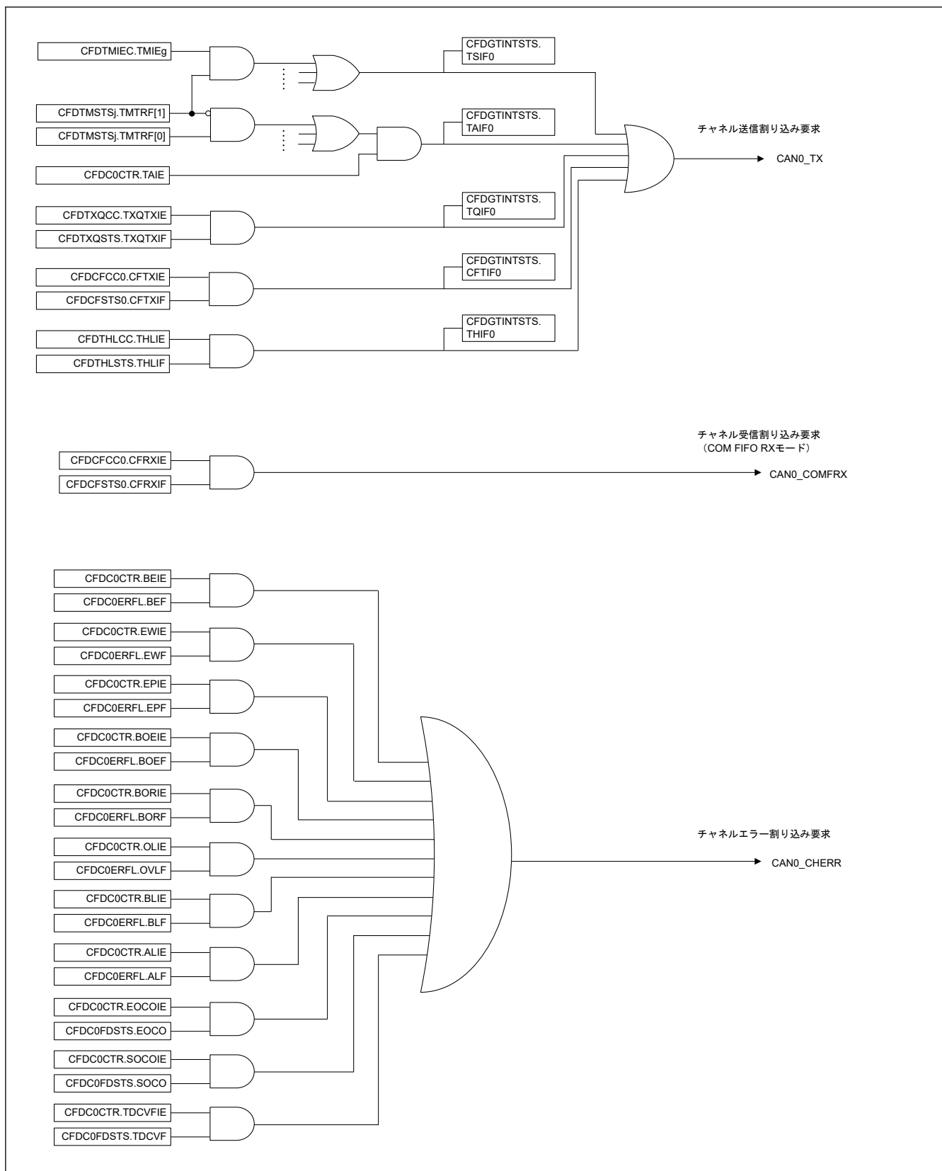
図 26.32 チャンネル割り込みのブロック図
