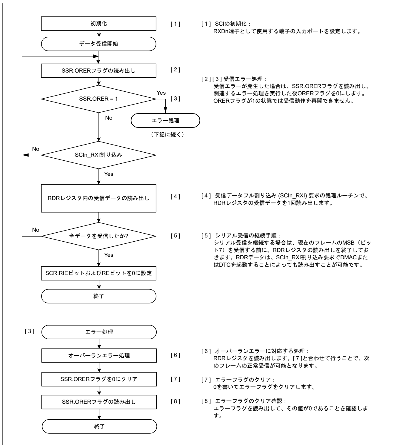
図 24.70 クロック同期式モードにおけるシリアル受信のフローチャート例 (非 FIFO 選択時)
