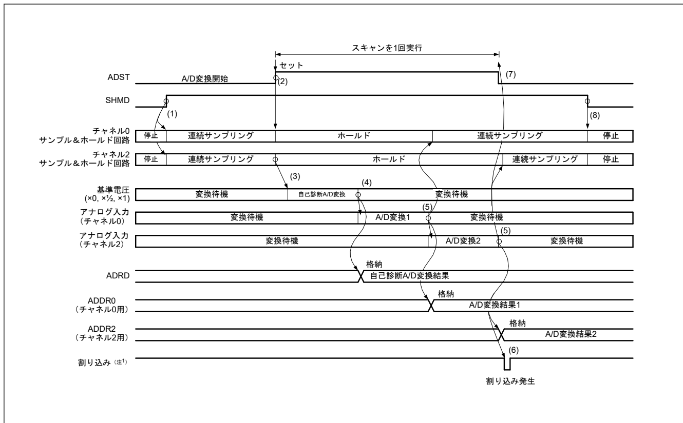
図 32.12 シングルスキャンモードの動作例（チャンネル専用サンプル&ホールド回路を使用し、自己診断で AN000 ~AN002 を選択し、連続サンプリングを有効にした場合）
