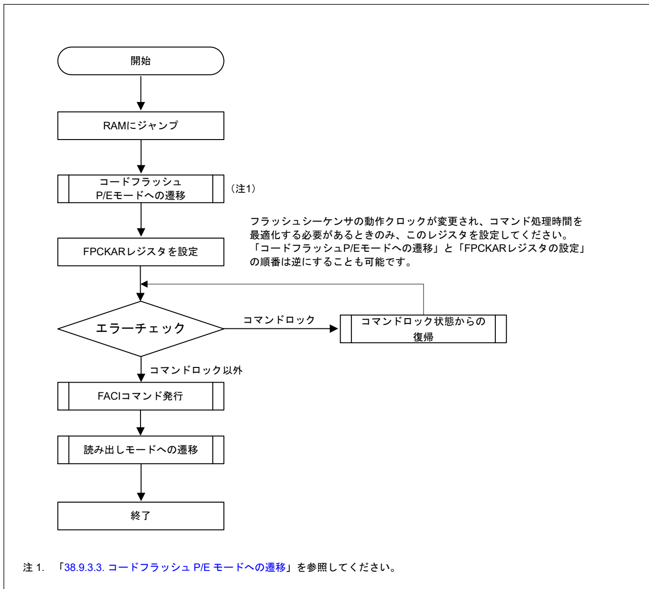
図 38.7 コードフラッシュ P/E モードでのコマンド使用概要
