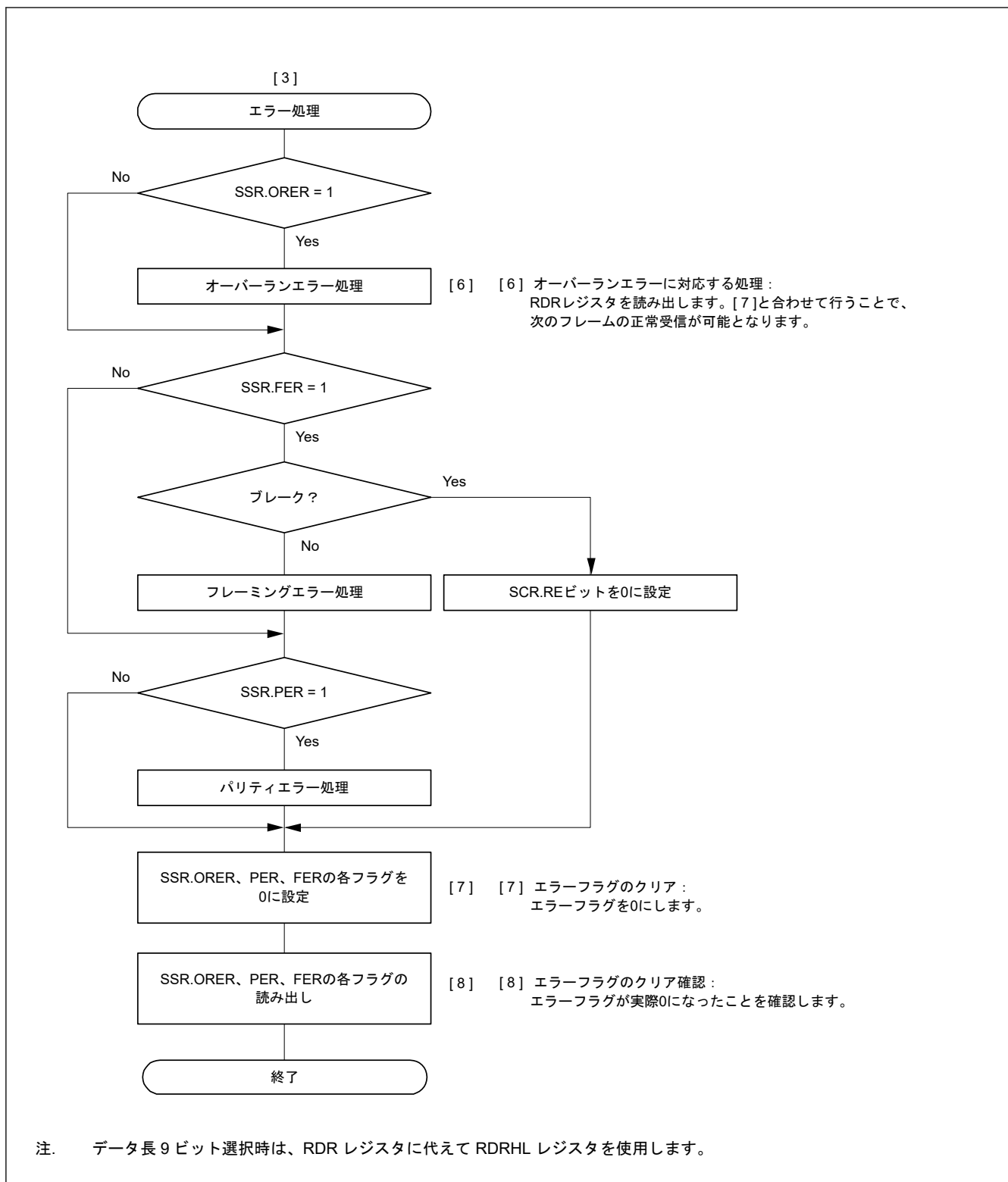
図 24.21 調歩同期式モードにおけるシリアル受信のフローチャート例（非 FIFO 選択、アドレス一致検出有効時） (3)
