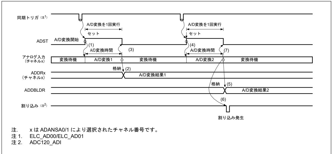
図 32.14 シングルスキャンモードの動作例 (ダブルトリガモード選択、アナログ入力 (チャンネル x) を 2 重化)
