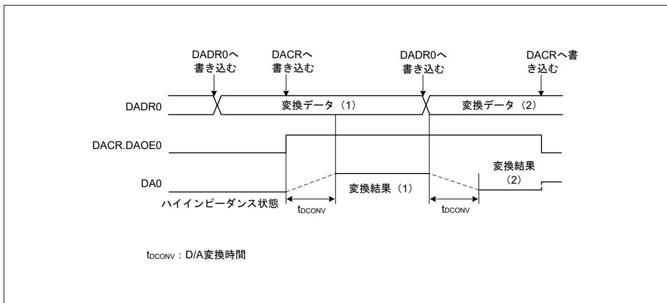
図 33.2 DAC12 の動作例
