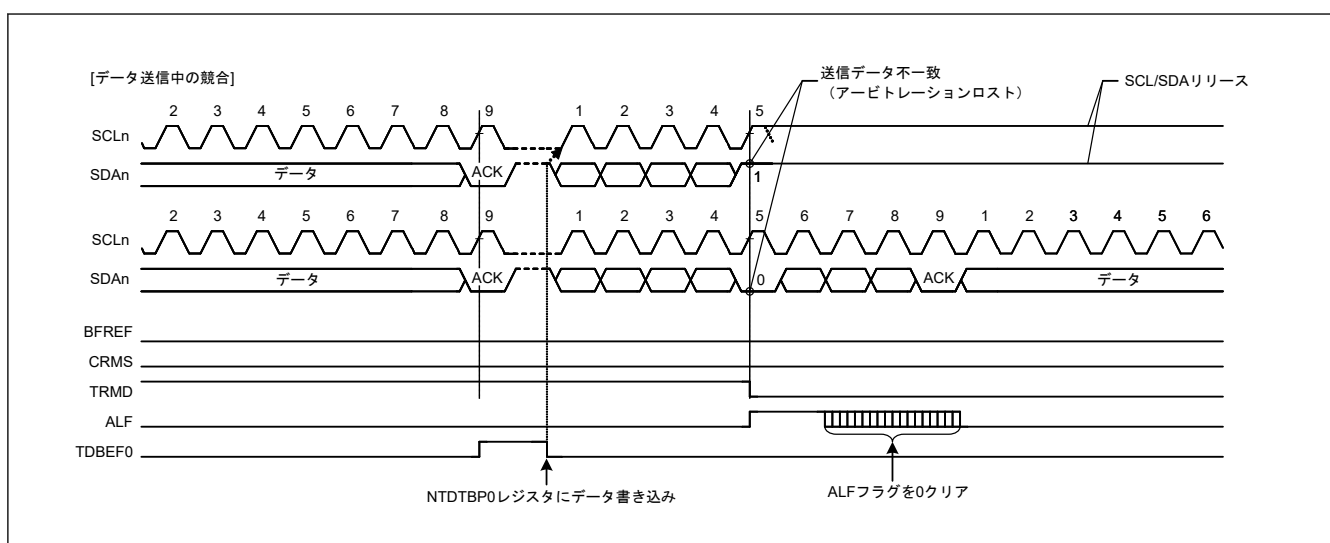
図 25.69 スレーブアービトレーションロスト検出動作例 (SALE = 1 の場合)
