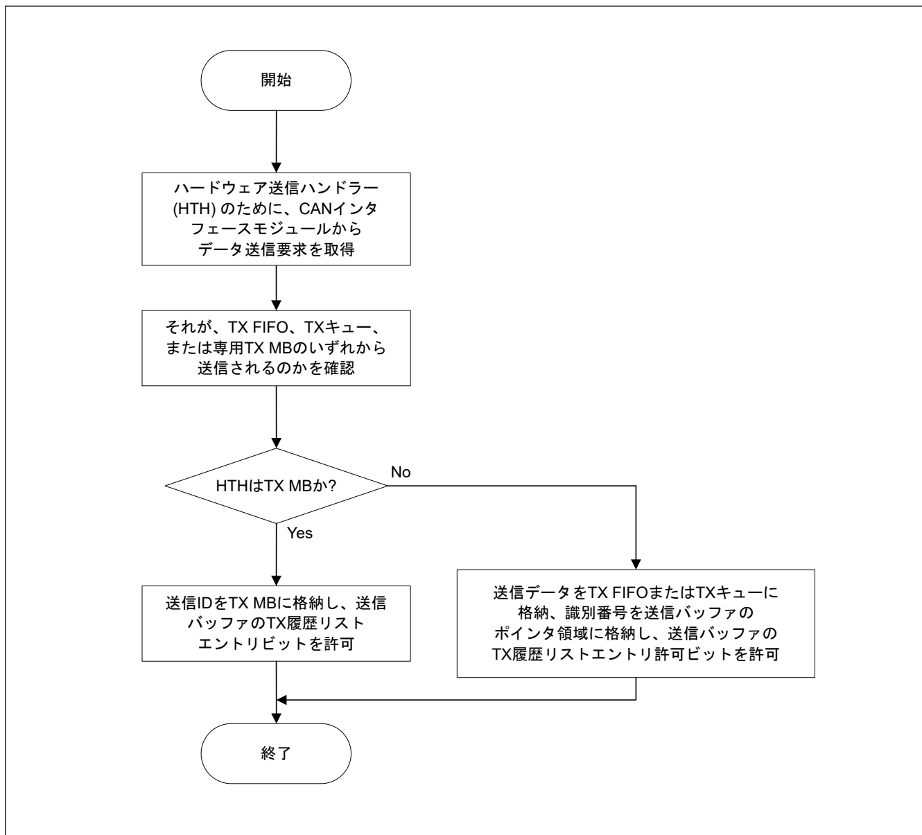
図 26.50 TX 履歴リストの準備手順
