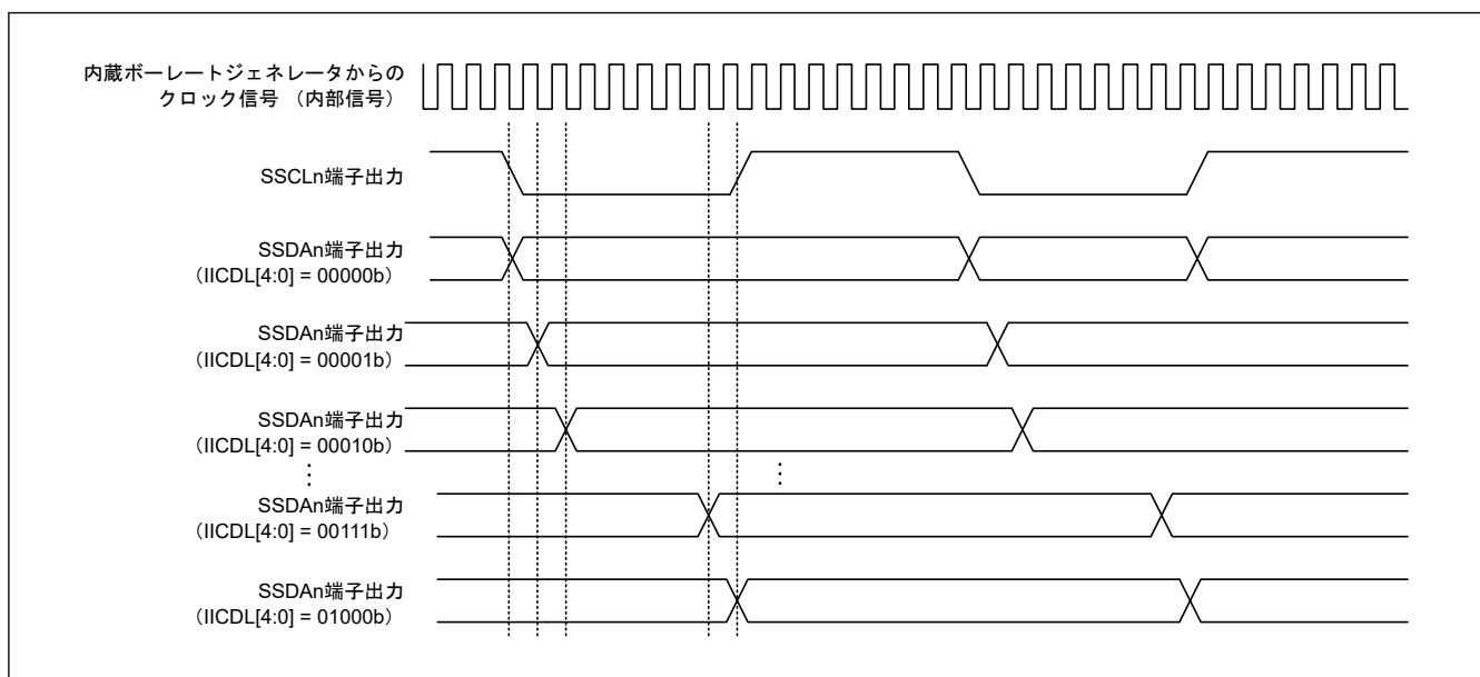
図 24.89 SDAn 出力遅延のタイミング
