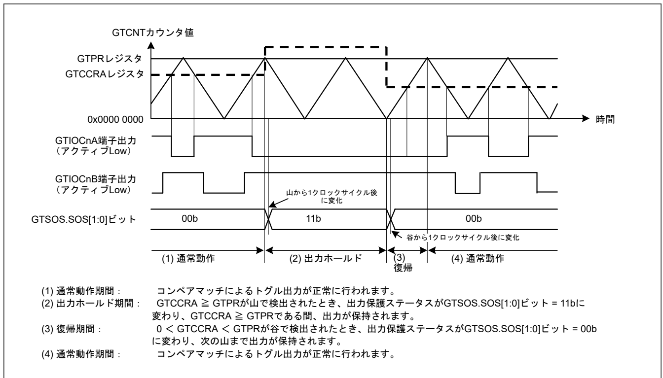
図 20.90 山でのバッファ転送中に GTCCRA \geq GTPR となったときの出力保護機能の動作例（谷でのバッファ転送中に 0 < GTCCRA < GTPR に復帰、アクティブレベルは Low）（ n = 0 \sim 5 ）
