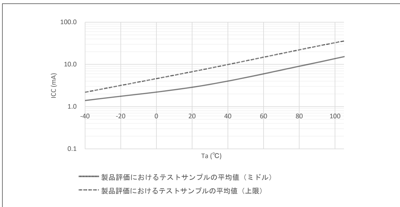
図 41.2 ソフトウェアスタンバイモード時の温度依存性 (参考データ)
