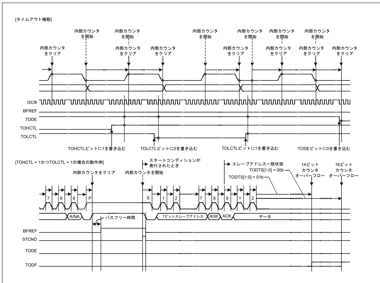
図 25.92 タイムアウトエラー検出機能 (TODE、TODTS[1:0]、TOHCTL、TOLCTL ビットの使用)
