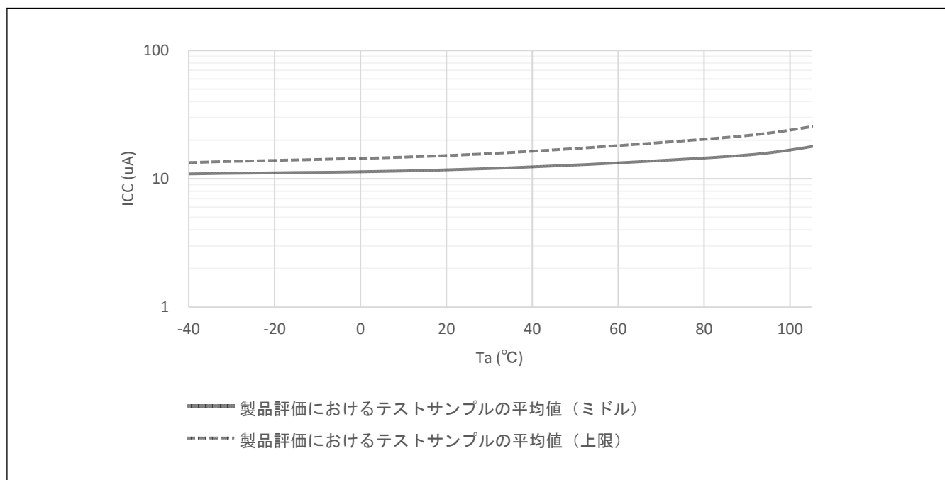
図 41.4 ディープソフトウェアスタンバイモード時の温度依存性、DPSBYCR.DEEPCUT[1:0] = 01b (参考データ)
