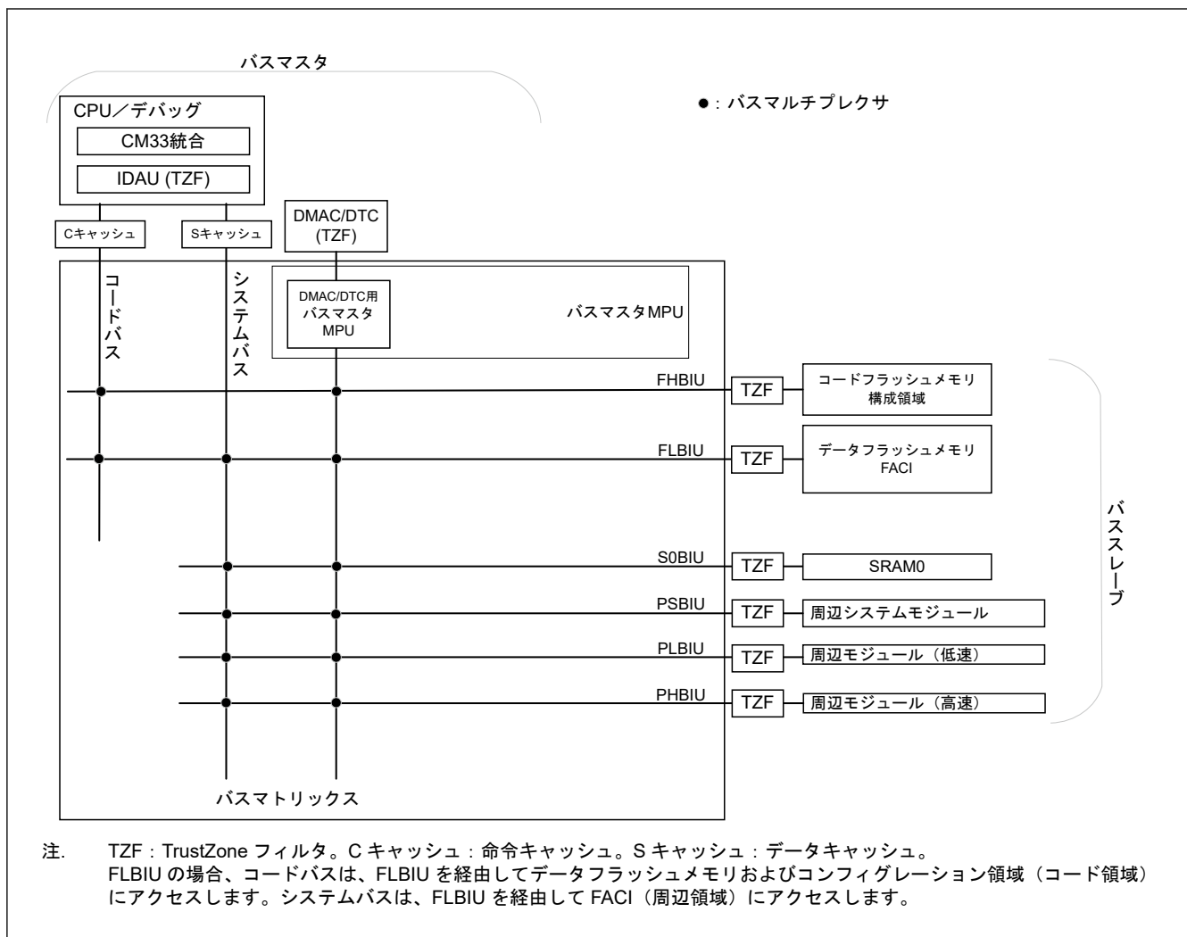
図 13.1 バス接続
