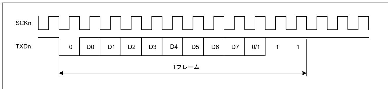
図 24.5 調歩同期式モードにおける出力クロックと送信データの位相関係 (SMR.CHR = 0、PE = 1、MP = 0、および STOP = 1 の場合)
