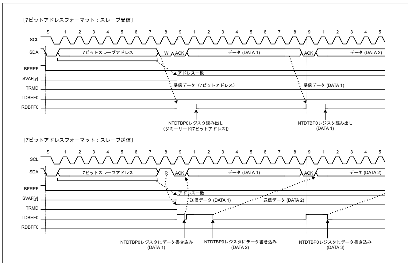
図 25.59 SVA[y]フラグが1になるタイミング (7ビットアドレスフォーマット選択時)
