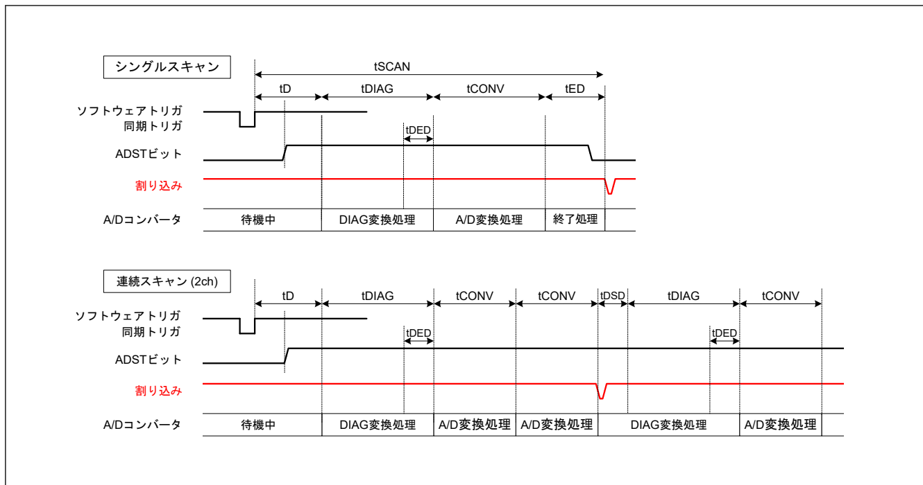
図 32.34 スキャン変換のタイミング (ソフトウェア起動または同期トリガ入力 (ELC) 起動の場合)
