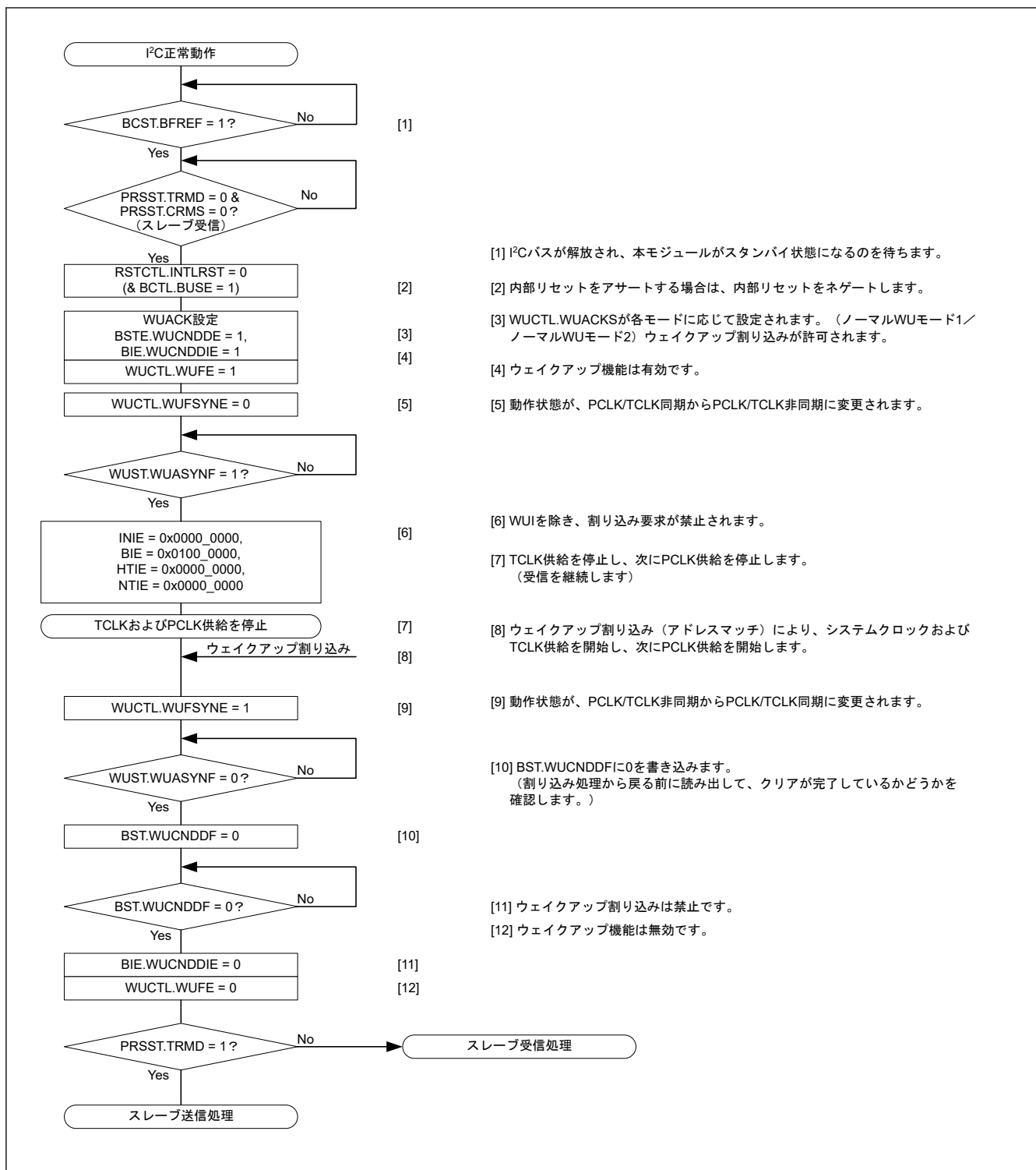
図 25.102 ノーマル WU モード 2 の使用例 (スレーブアドレス一致に起因するウェイクアップ割り込みによるウェイクアップリカバリの場合)
