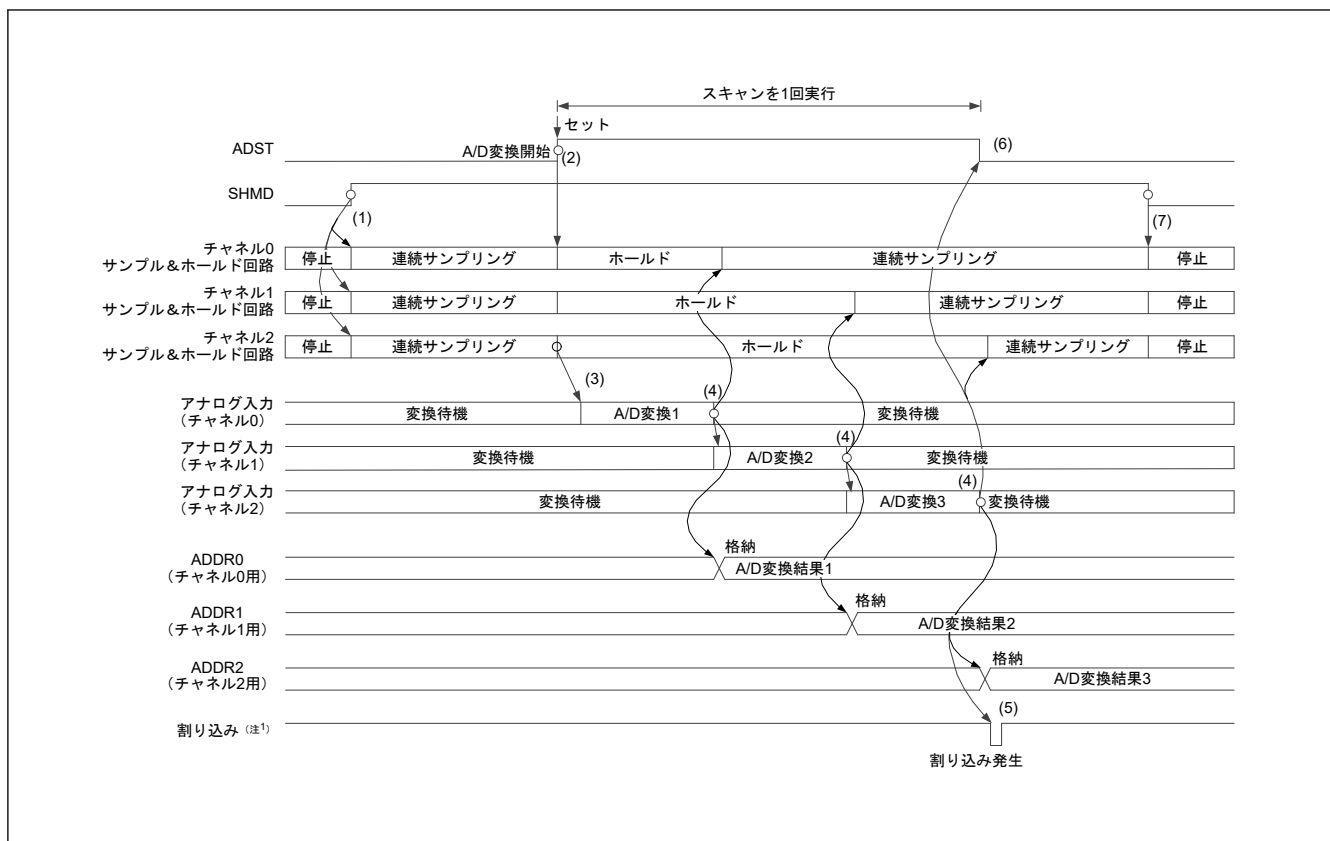
図 32.9 シングルスキャンモードの動作例 (チャンネル専用サンプル&ホールド回路を使用し、AN000~AN002 を選択し、連続サンプリングを有効にした場合)
