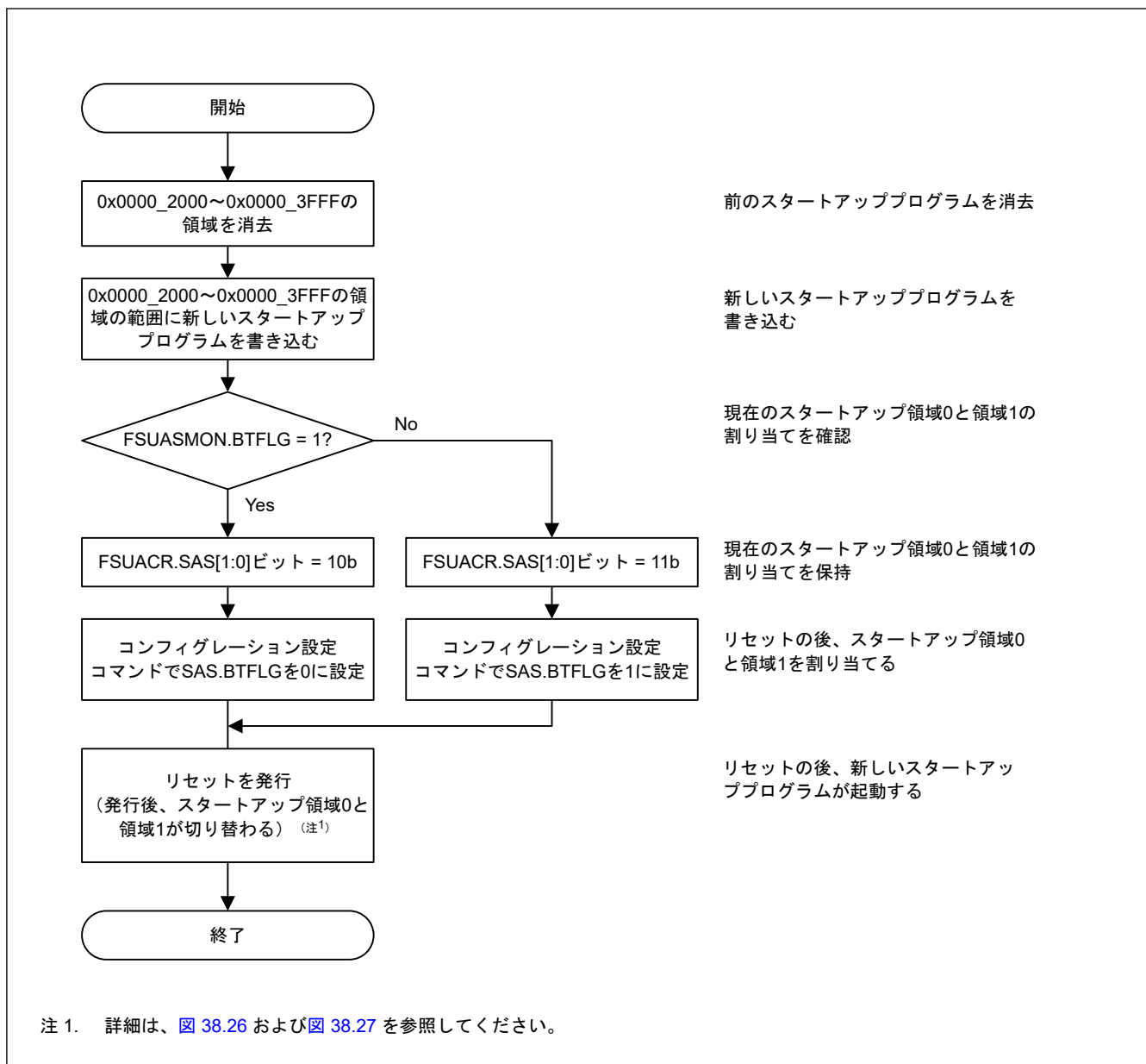
図 38.28 スタートアッププログラムプロテクションの概念
