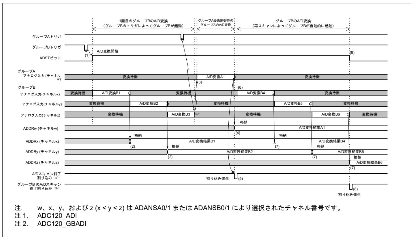
図 32.26 グループ優先動作の例 1-1: グループ B スキャン中のグループ A トリガ入力、再スキャンあり (ADGSPCR.GBRSCN = 1、ADGSPCR.GBRP = 0、および ADGSPCR.LGRRS = 0 の場合)
