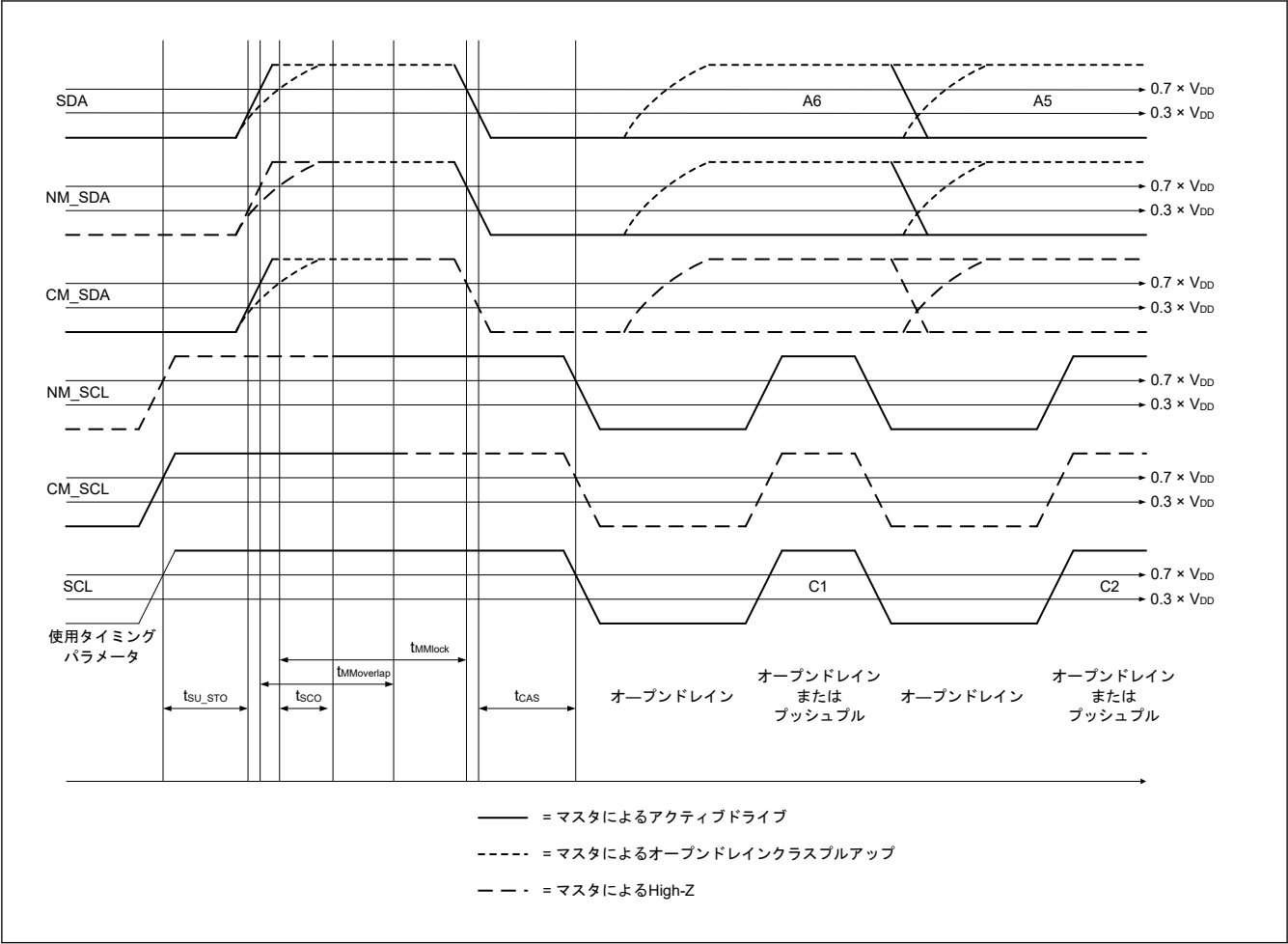
図 41.51 I3C タイミング (オープンドレインタイミングパラメータ)
