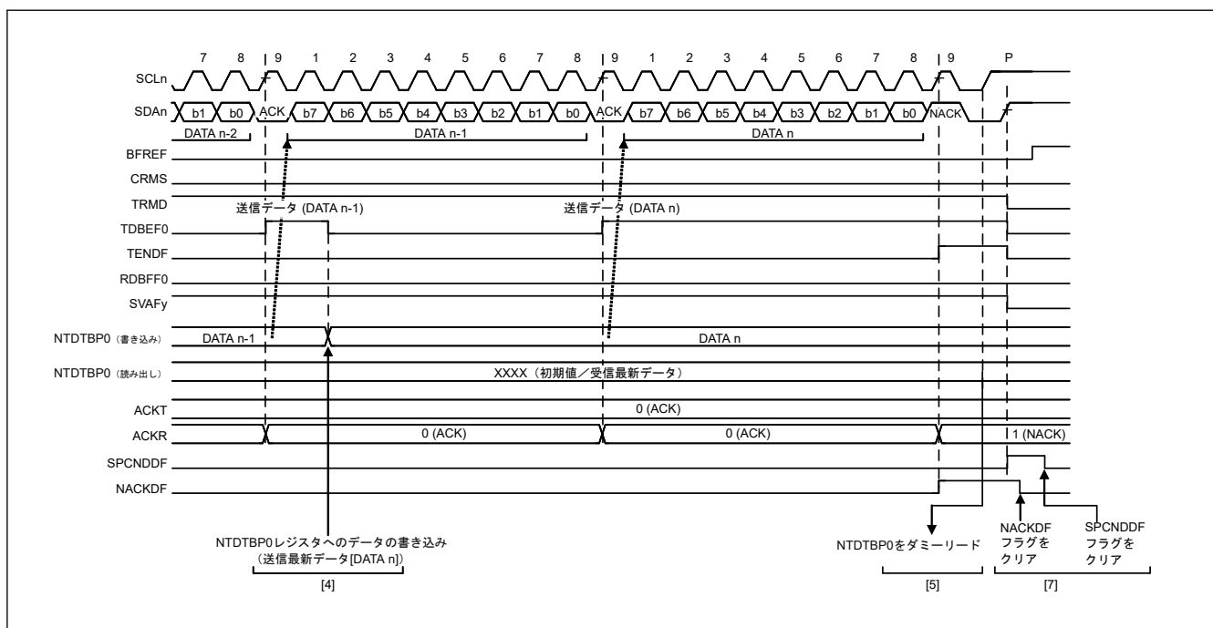
図 25.30 スレーブ送信の動作タイミング (2)
