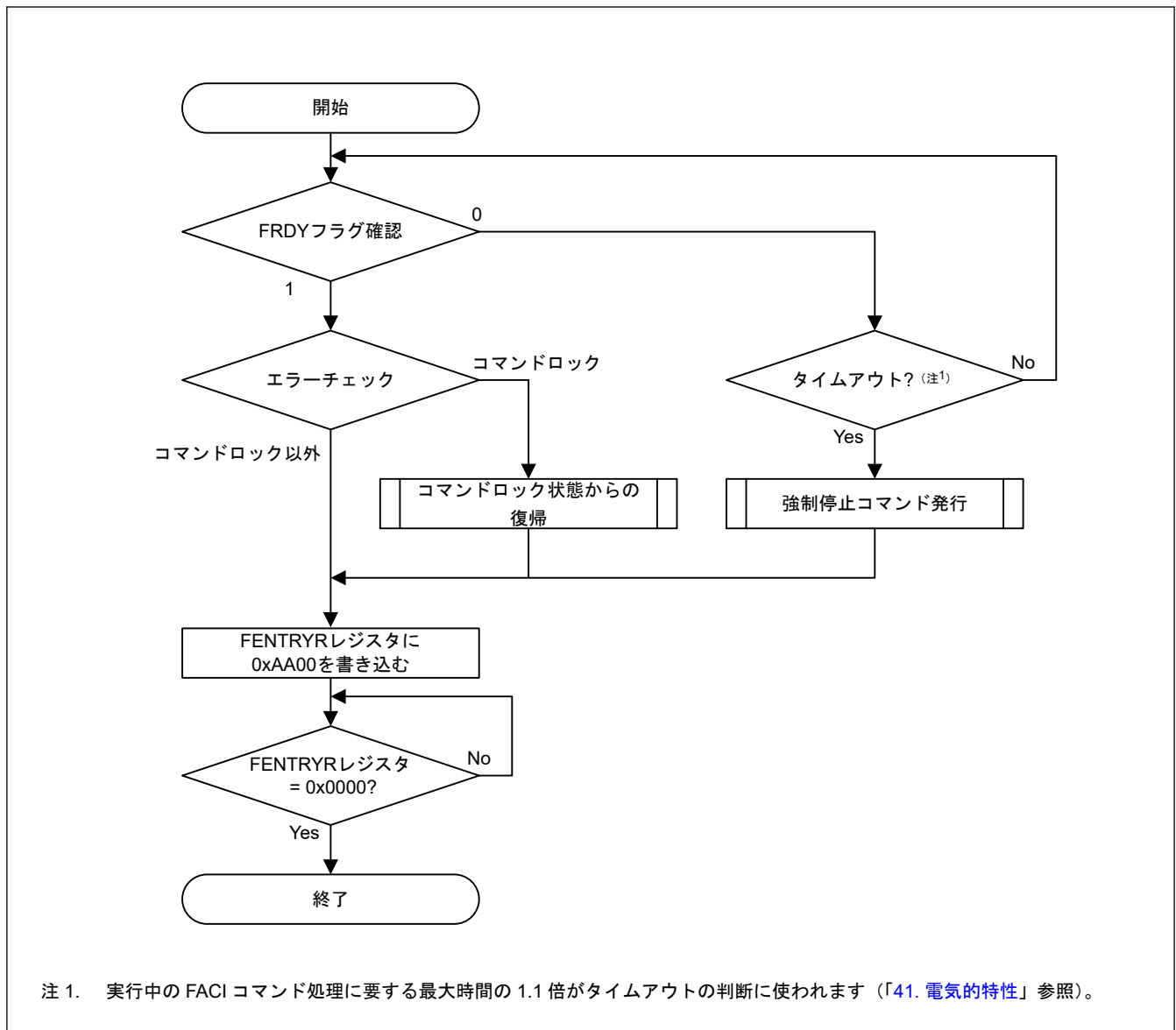
図 38.11 読み出しモードへの遷移手順
