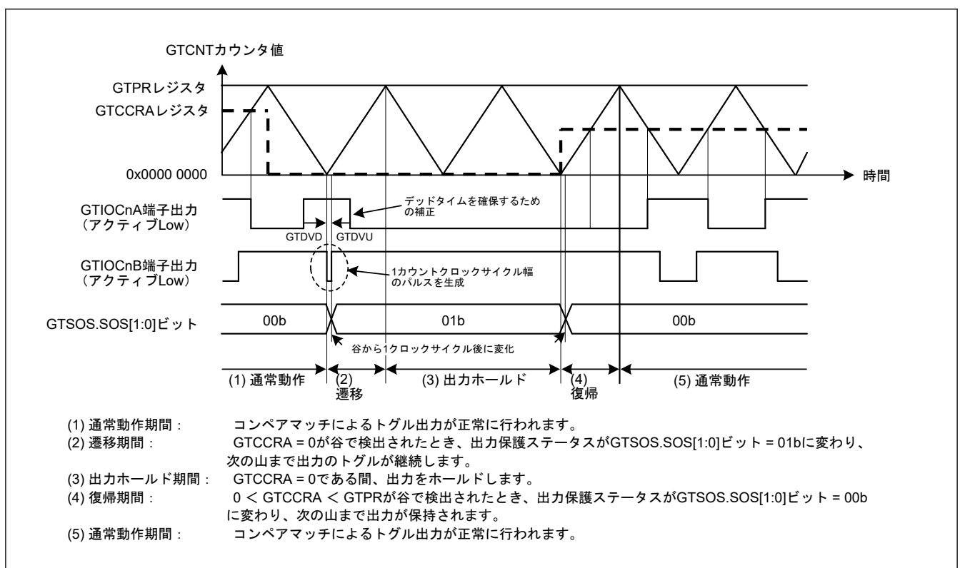
図 20.85 山でのバッファ転送中に GTCCRA が 0 になったときの出力保護機能の動作例 (谷でのバッファ転送中に 0 < GTCCRA < GTPR に復帰、アクティブレベルは Low) ( n = 0 \sim 5 )
