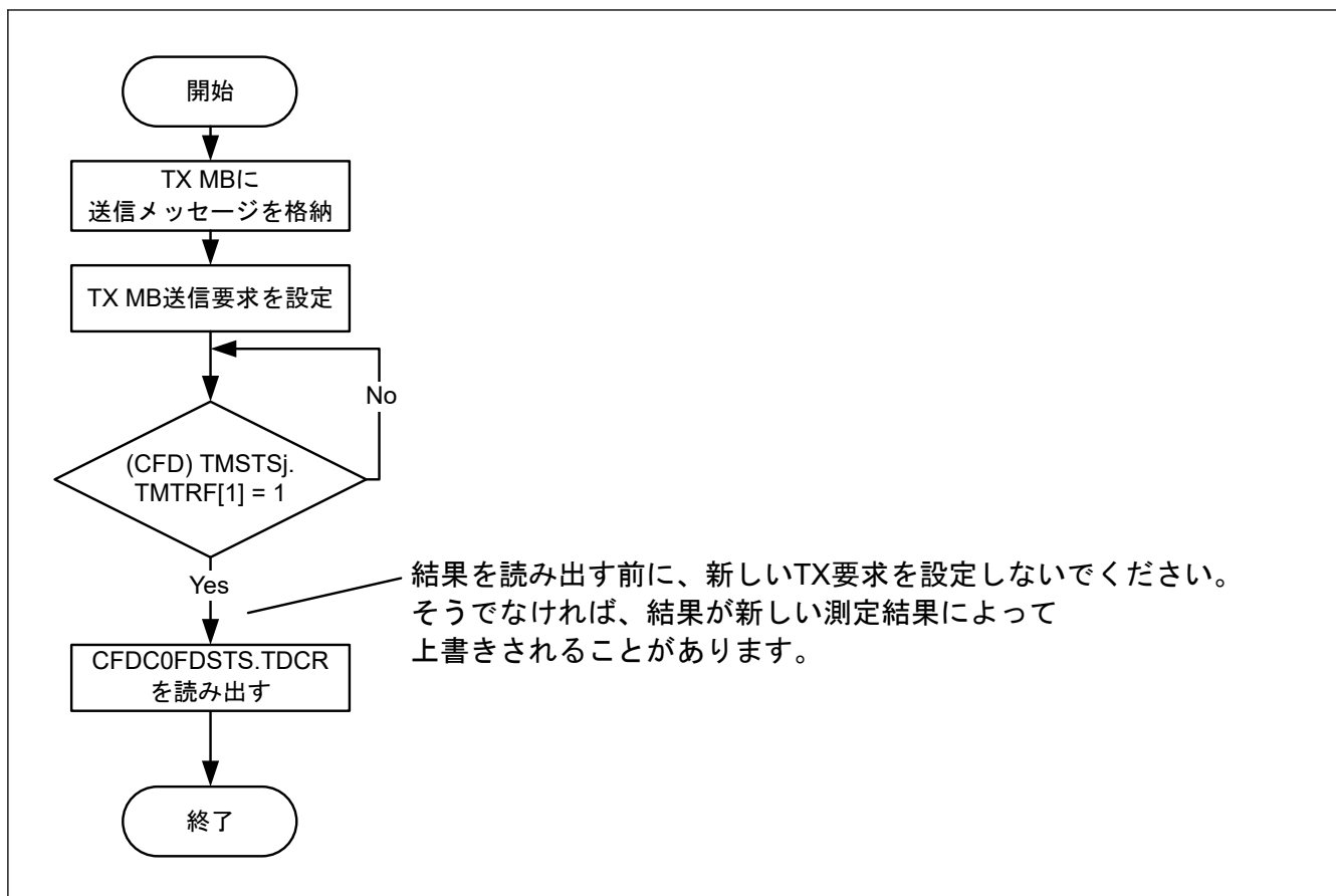
図 26.22 TDC 結果読み出しフロー
