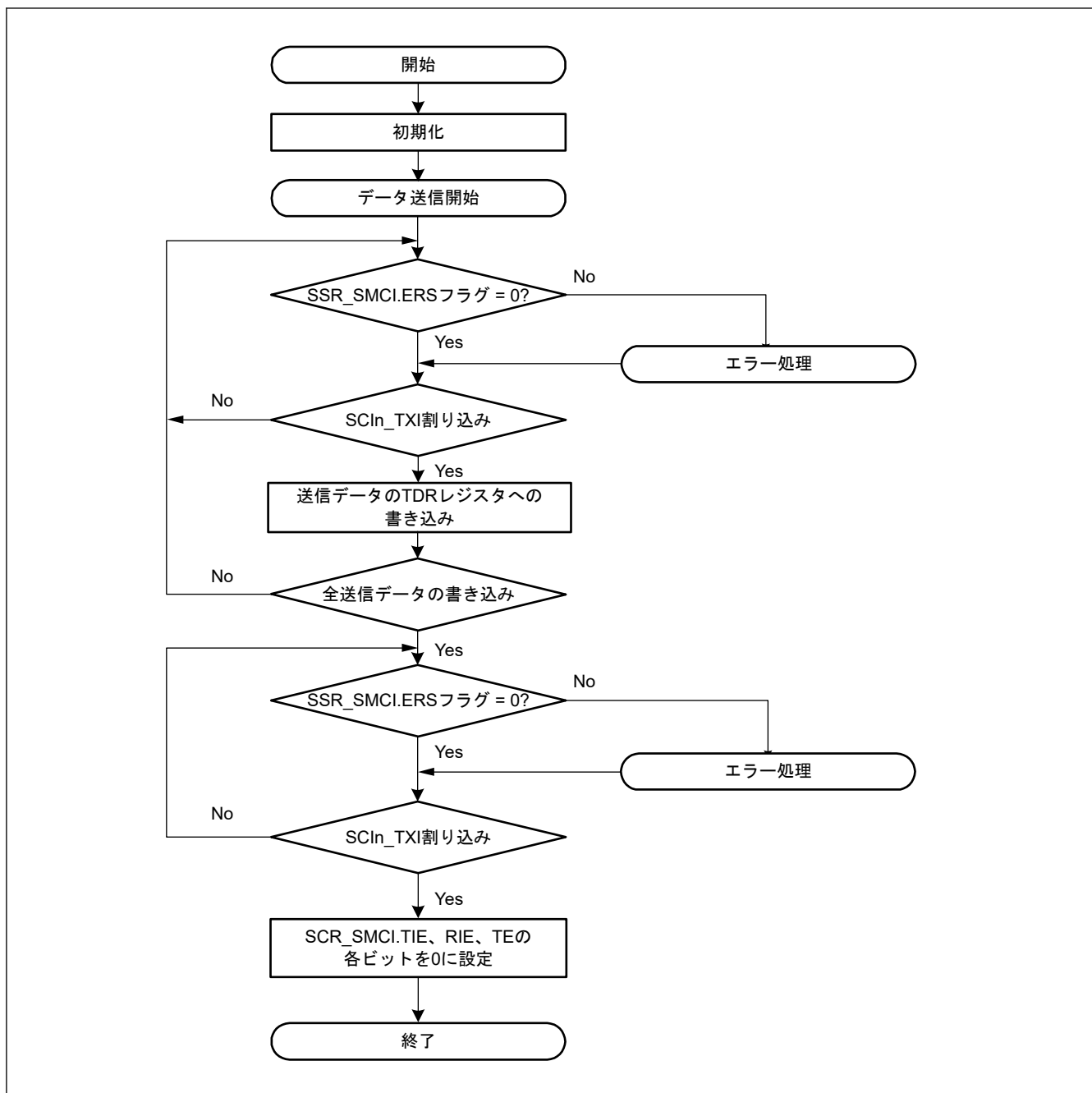
図 24.81 スマートカードインタフェース送信のフローチャート例
