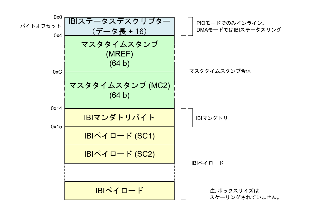
図 25.87 IBI イベント用のマスタタイムスタンプカウンタ
