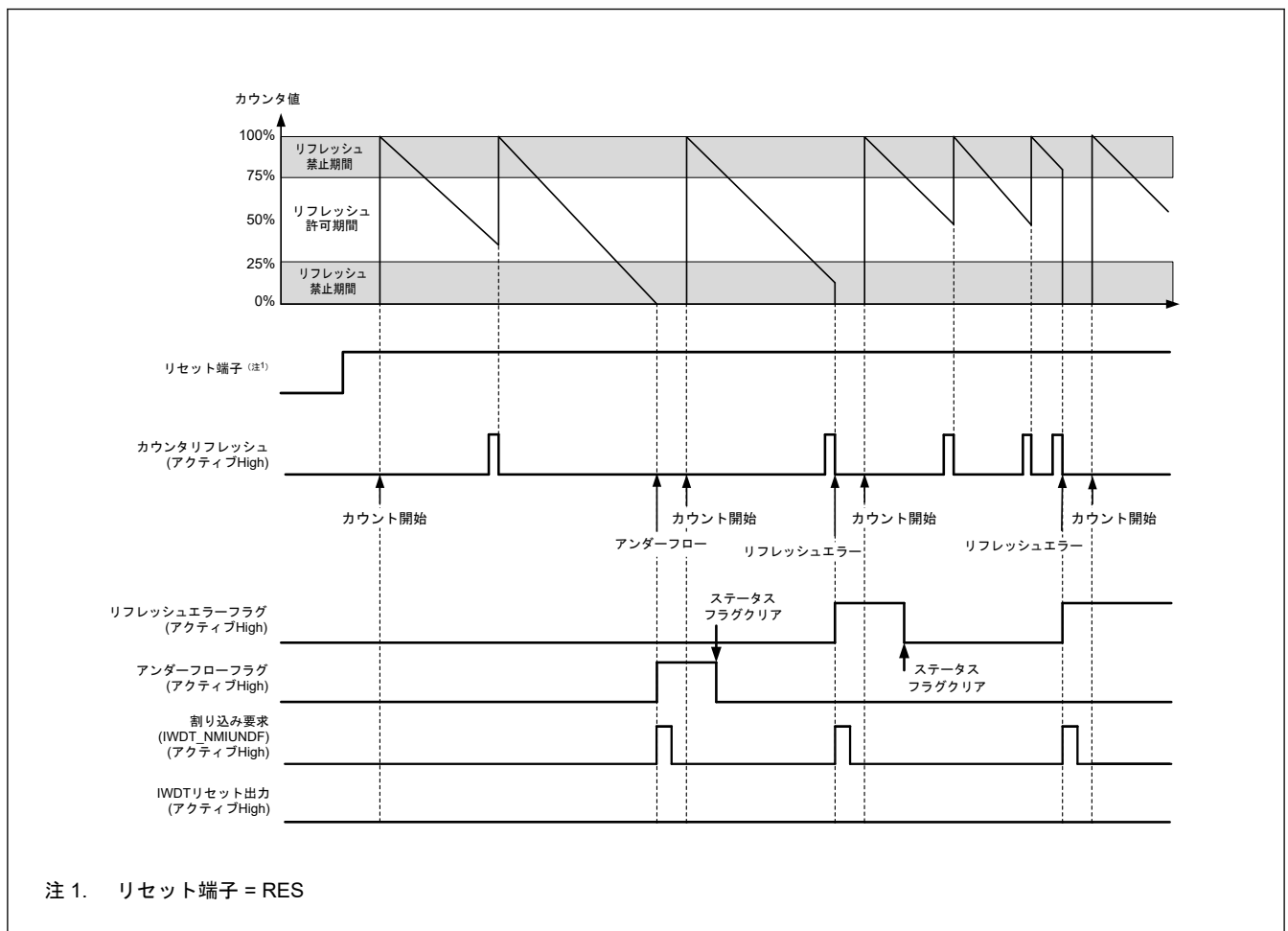
図 23.3 オートスタートモードでの動作例
