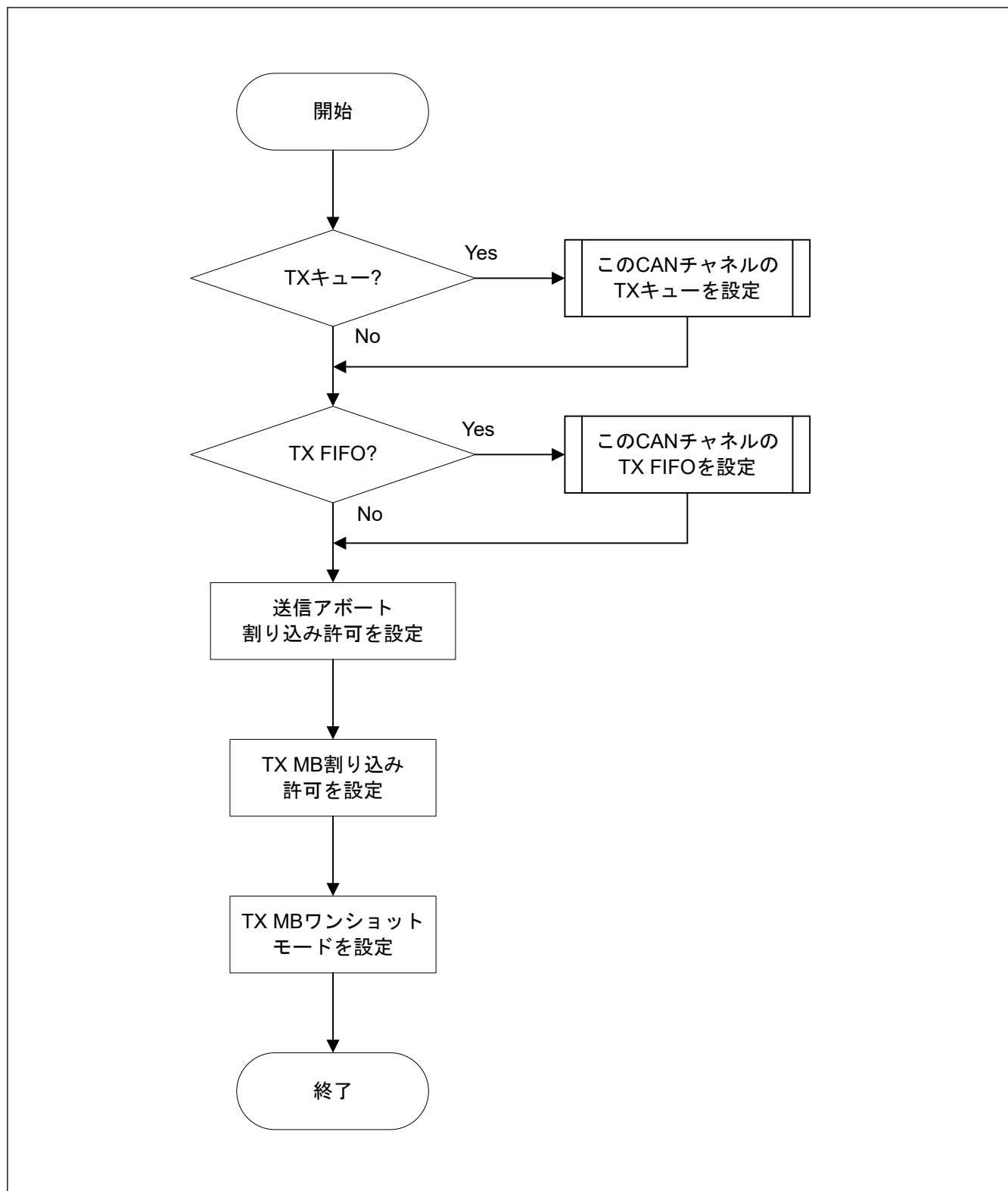
図 26.42 送信構成フロー
