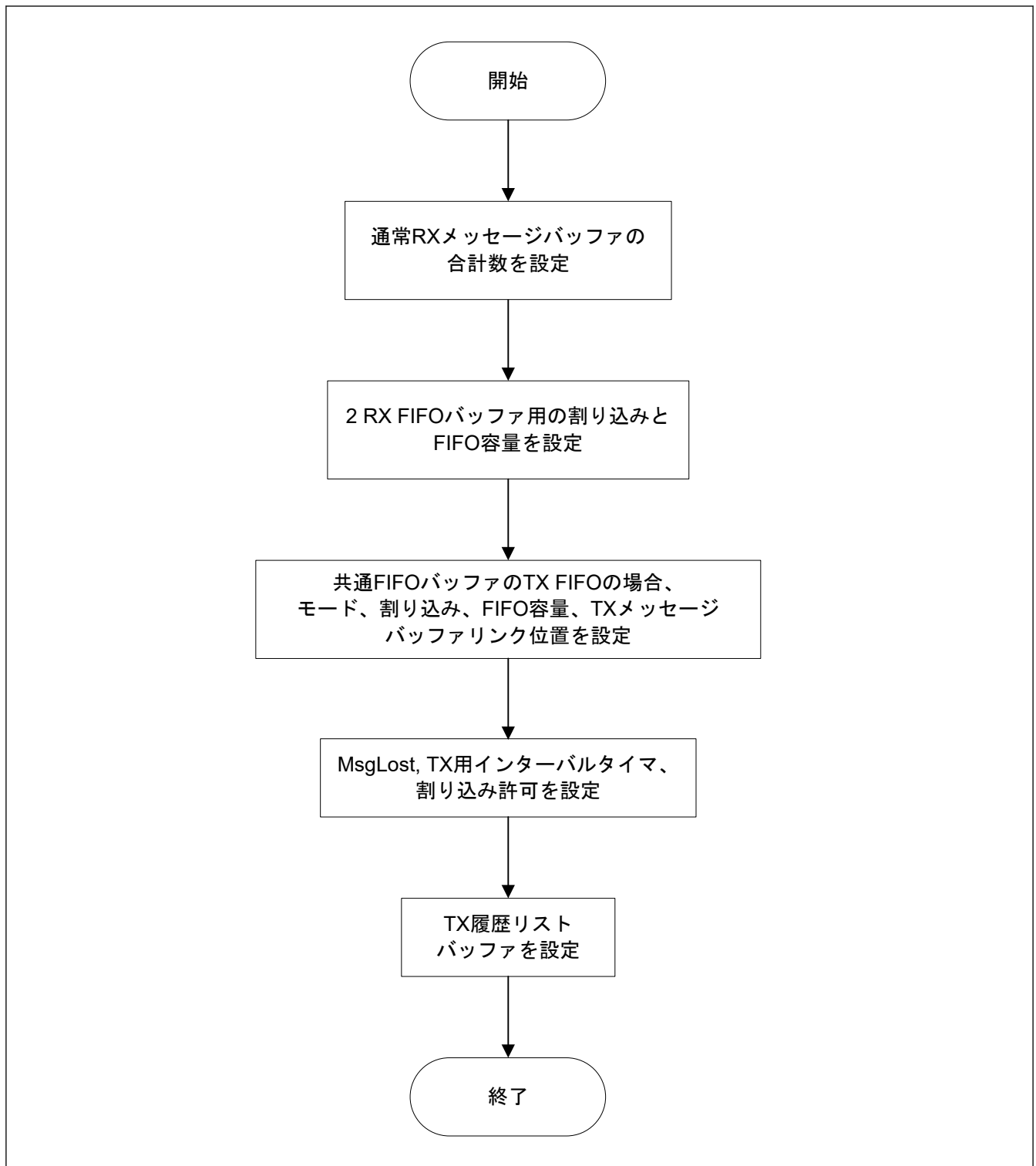
図 26.30 CANFD モジュールにおける FIFO バッファの構成フロー
