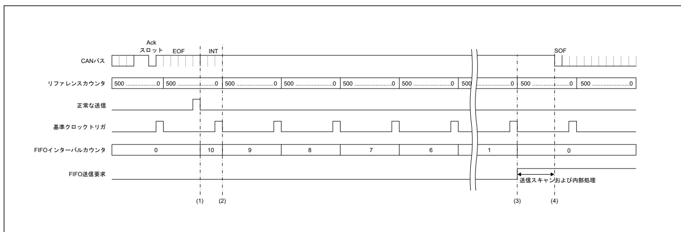
図 26.47 インターバル処理時間の例
