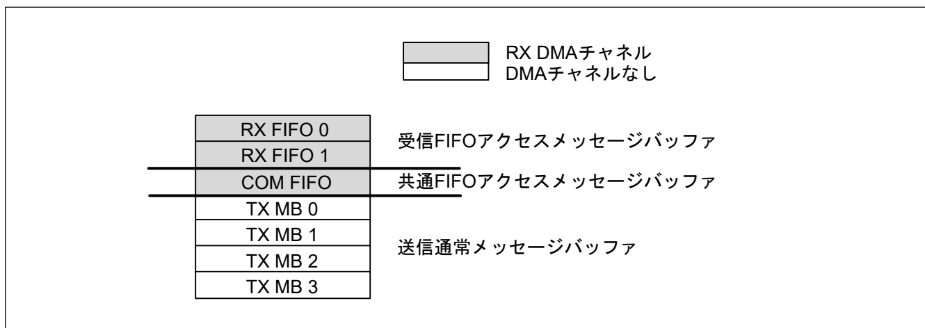
図 26.33 DMA チャンネルに接続可能なメッセージバッファ
