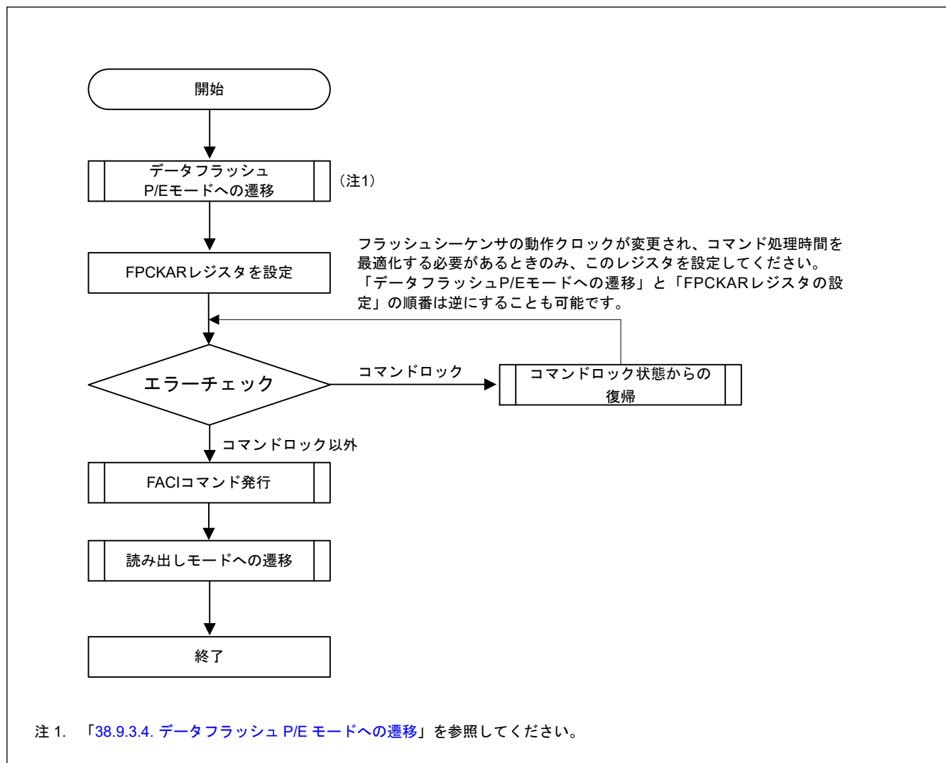
図 38.8 データフラッシュ P/E モードでのコマンド使用概要
