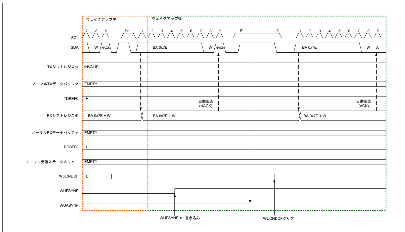
図 25.109 I3C スレーブウェイクアップ動作 (2/2)
