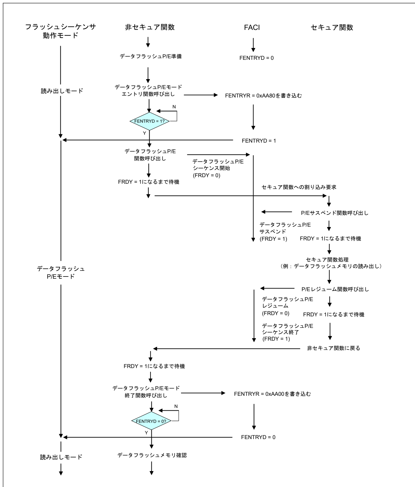
図 38.34 セキュア関数のデータフラッシュ P/E サスペンド例 (P/E 終了を検出するには FRDY ビットを確認)
