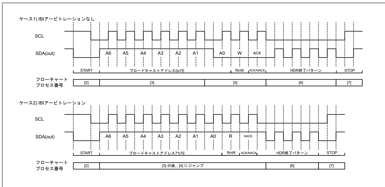
図 25.98 I3C マスタの I3C エスカレーション処理タイミングチャート
