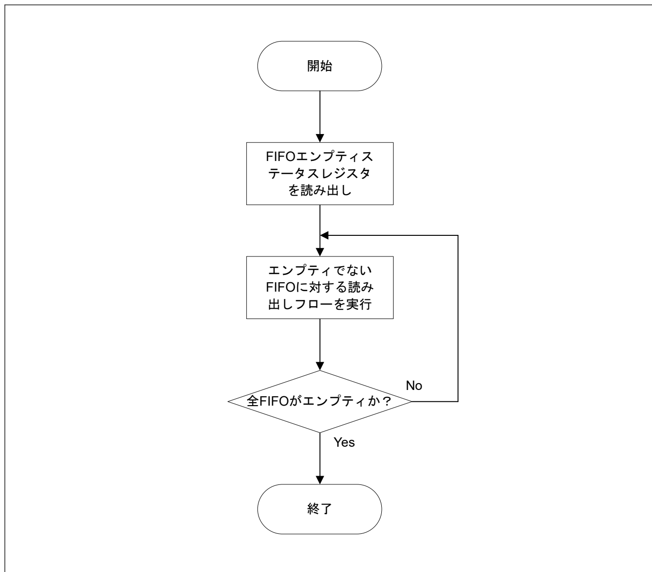
図 26.39 FIFO バッファのメッセージアクセスフロー (ポーリングの場合の例)
