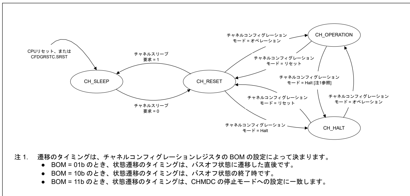
図 26.11 CAN チャンネルモード間の遷移
