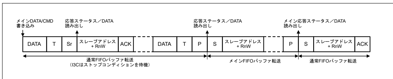
図 25.48 優先 FIFO バッファ転送のデータハンドラ
