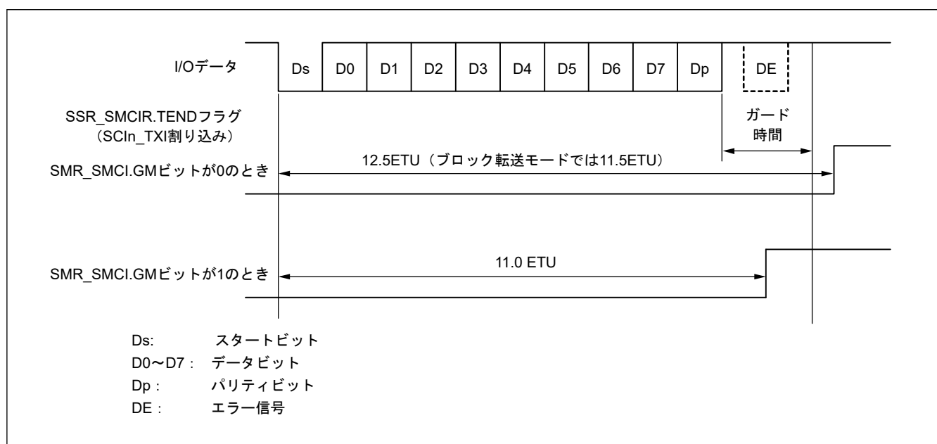
図 24.80 送信中の SSR.TEND フラグの発生タイミング
