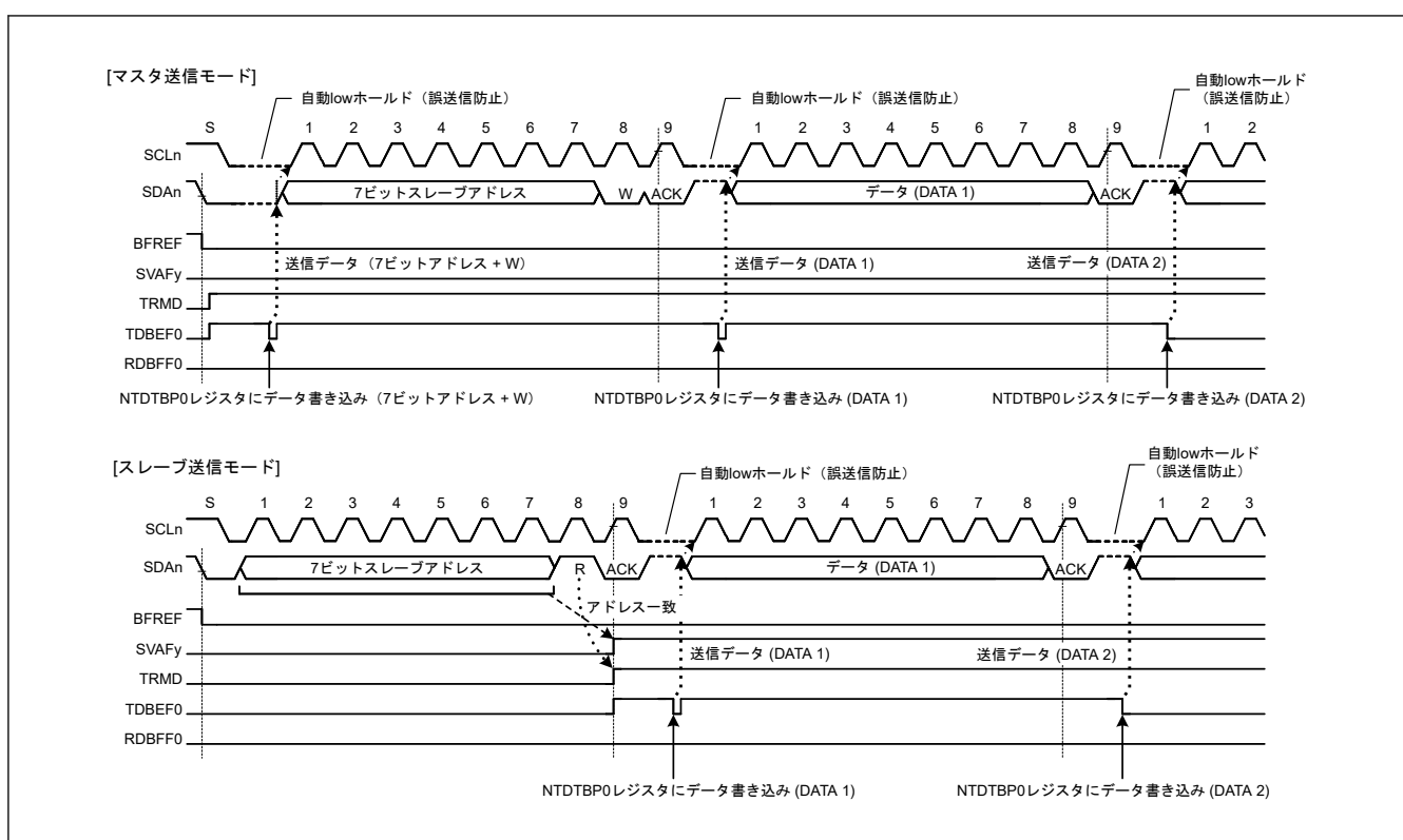
図 25.70 送信モード時の自動 Low ホールド動作
