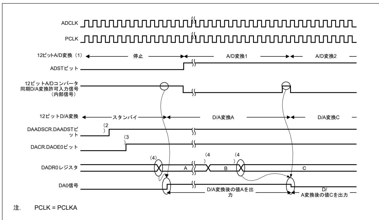
図 33.3 DAC12 を次に同期して変換する例 : ADC12
