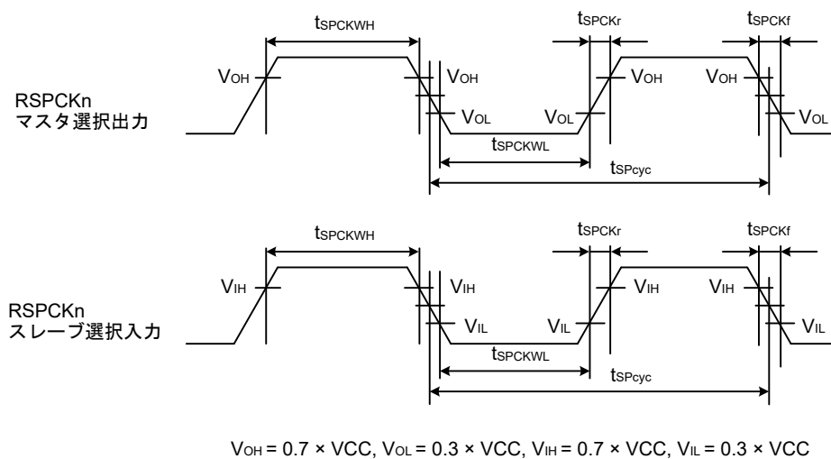
図 41.34 SPI クロックタイミング
