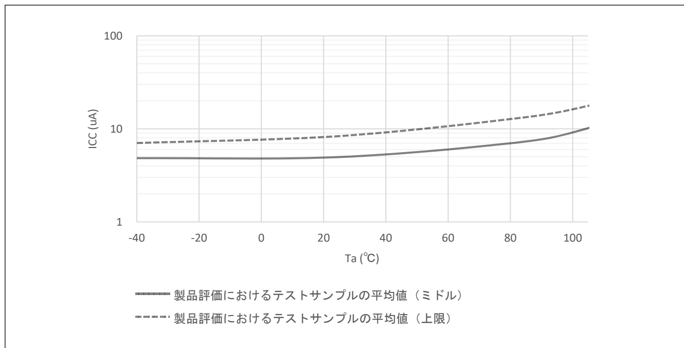
図 41.5 ディープソフトウェアスタンバイモード時の温度依存性、DPSBYCR.DEEPCUT[1:0] = 11b (参考データ)
