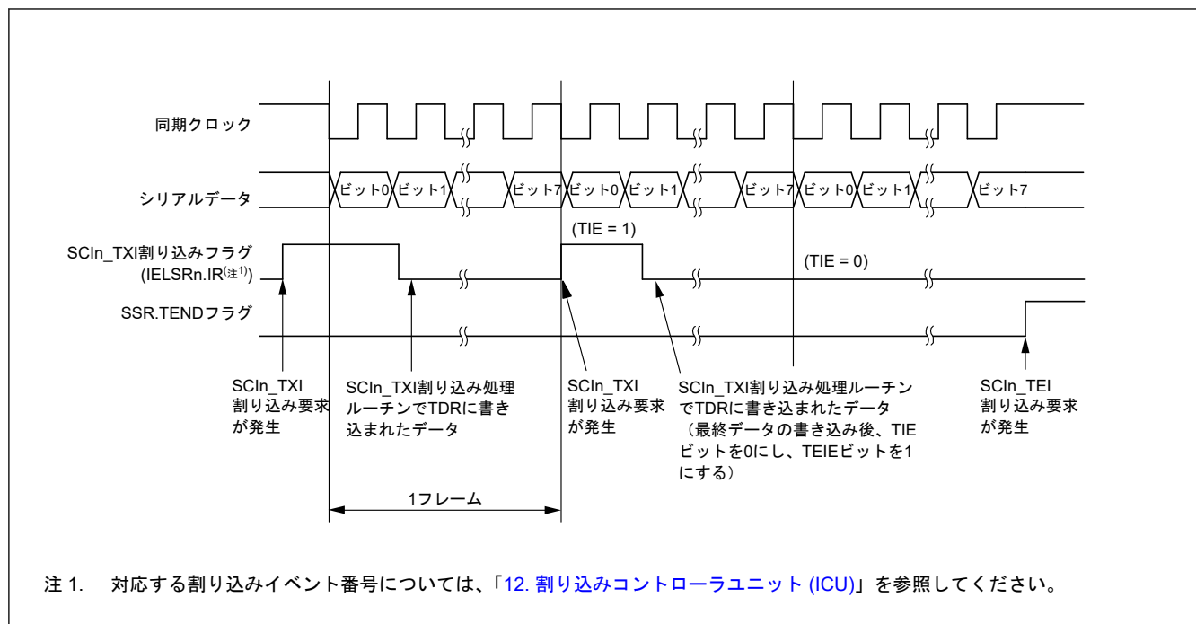
図 24.65 クロック同期式モードにおけるシリアル送信の動作例 (送信中～送信終了時)
