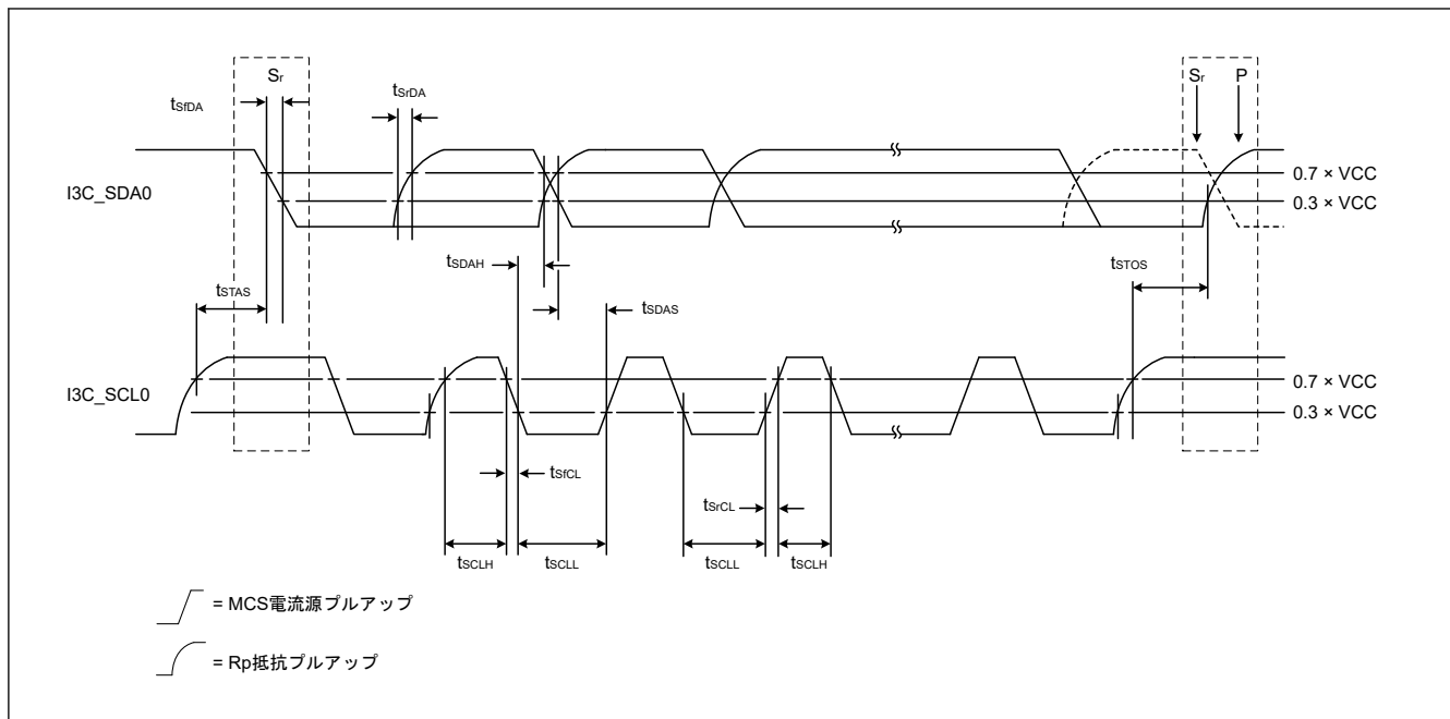
図 41.42 I 2 C バスインタフェース入出力タイミング (Hs モード)
