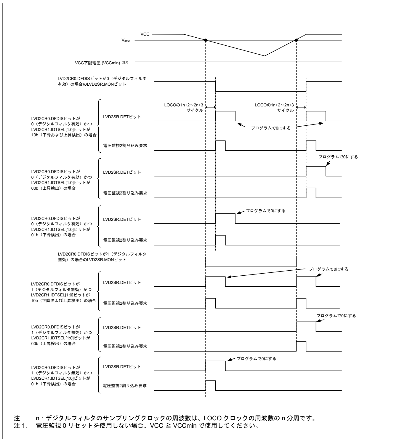
図 7.6 電圧監視 2 割り込みの動作例
