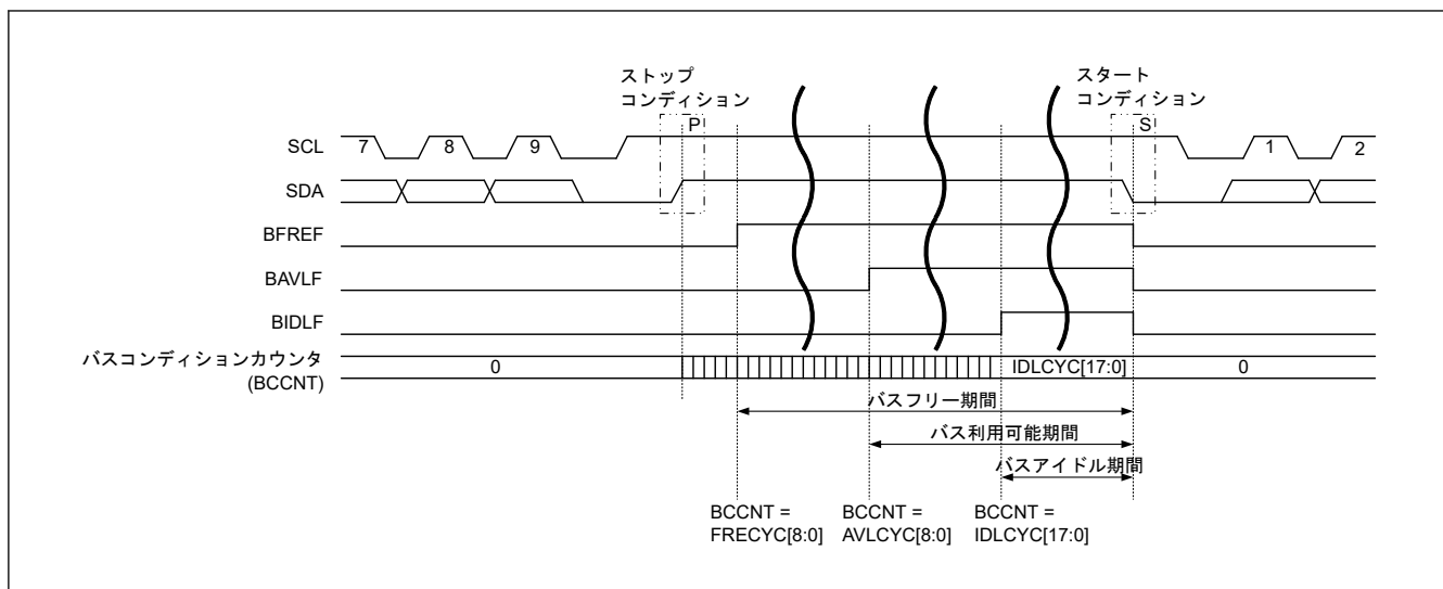
図 25.55 バス状態
