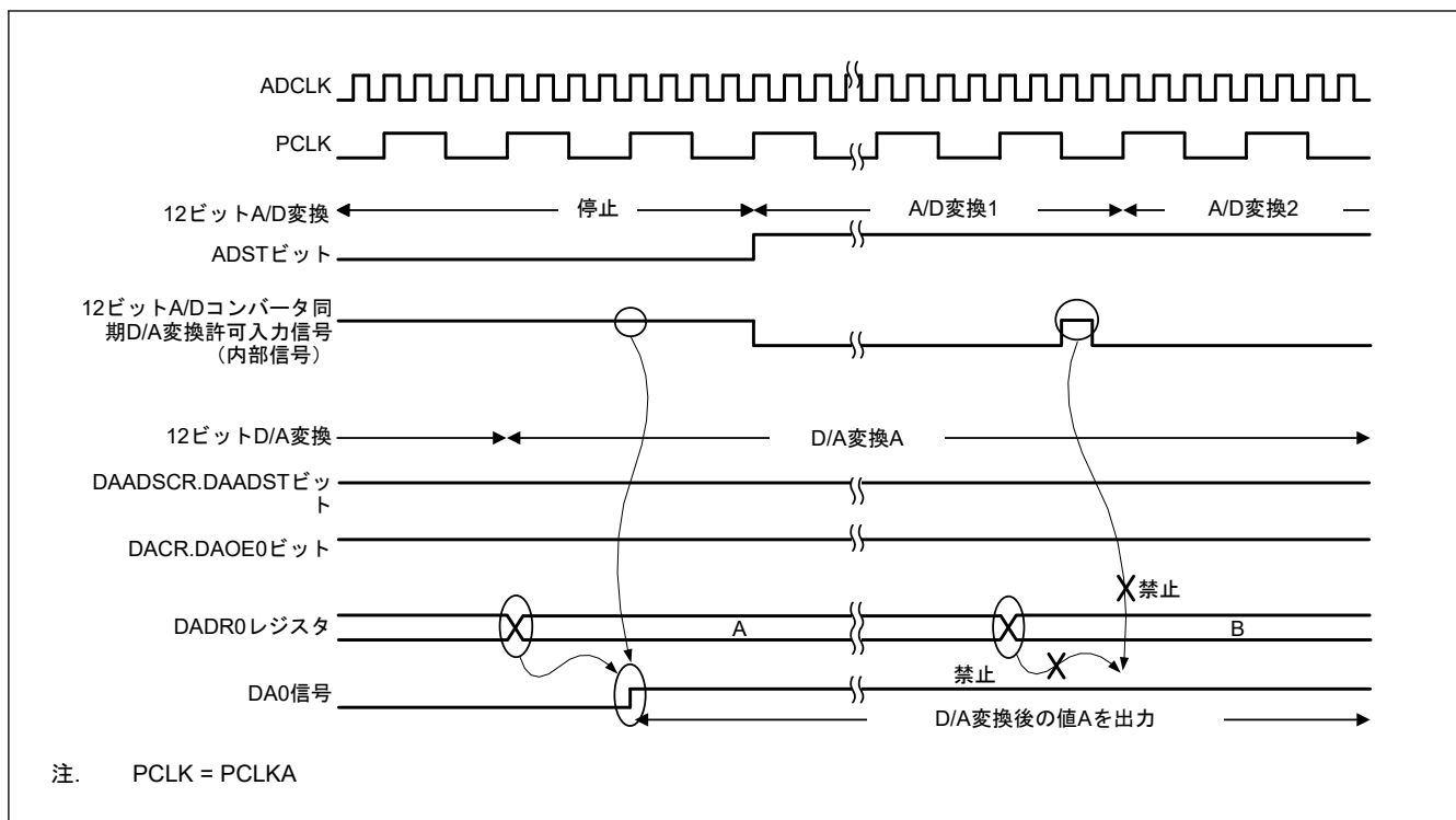
図 33.4 DAC12 が次からの同期 D/A 変換許可入力信号を取り込めない場合の例：ADC12
