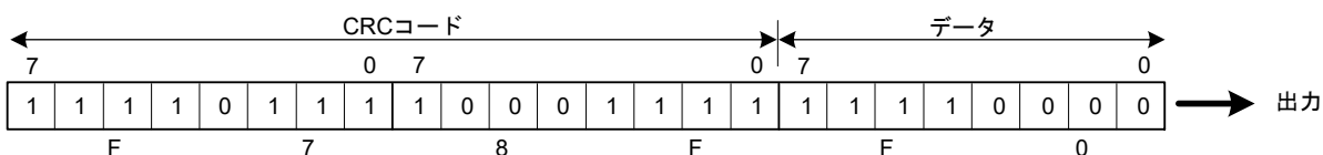
図 29.2 LSB ファーストのデータ送信
