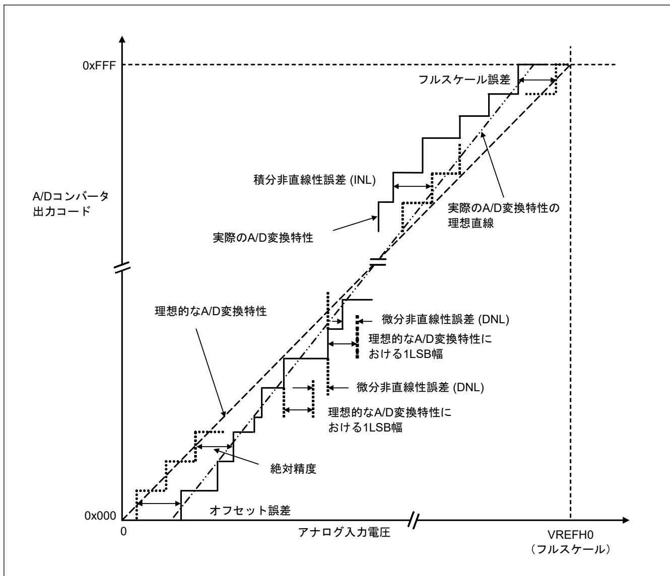
図 41.53 ADC12 特性用語の解説図
