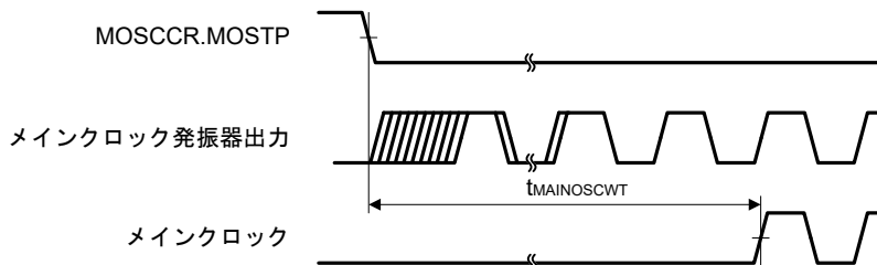
図 41.8 メインクロック発振開始タイミング
