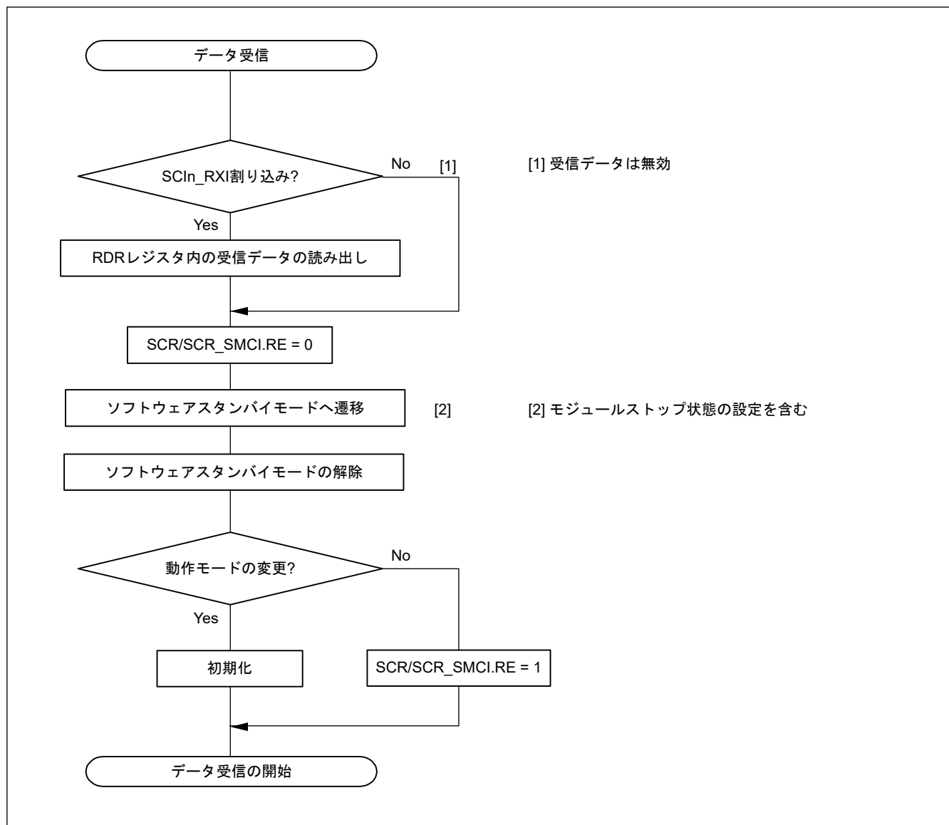
図 24.102 受信中にソフトウェアスタンバイモードへ遷移する場合のフローチャート例
