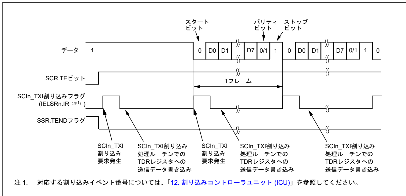
図 24.8 調歩同期式モードにおけるシリアル送信の動作例 (1) (8 ビットデータ/パリティあり/1 ストップビット /CTS 機能不使用/送信開始時)
