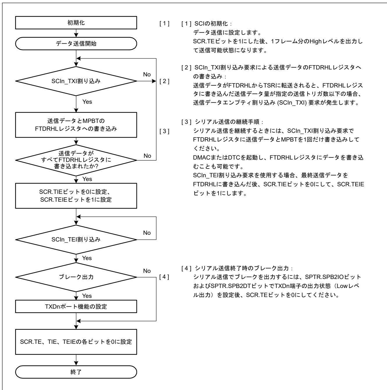
図 24.40 マルチプロセッサモードにおけるシリアル送信のフローチャート例 (FIFO 選択時)
