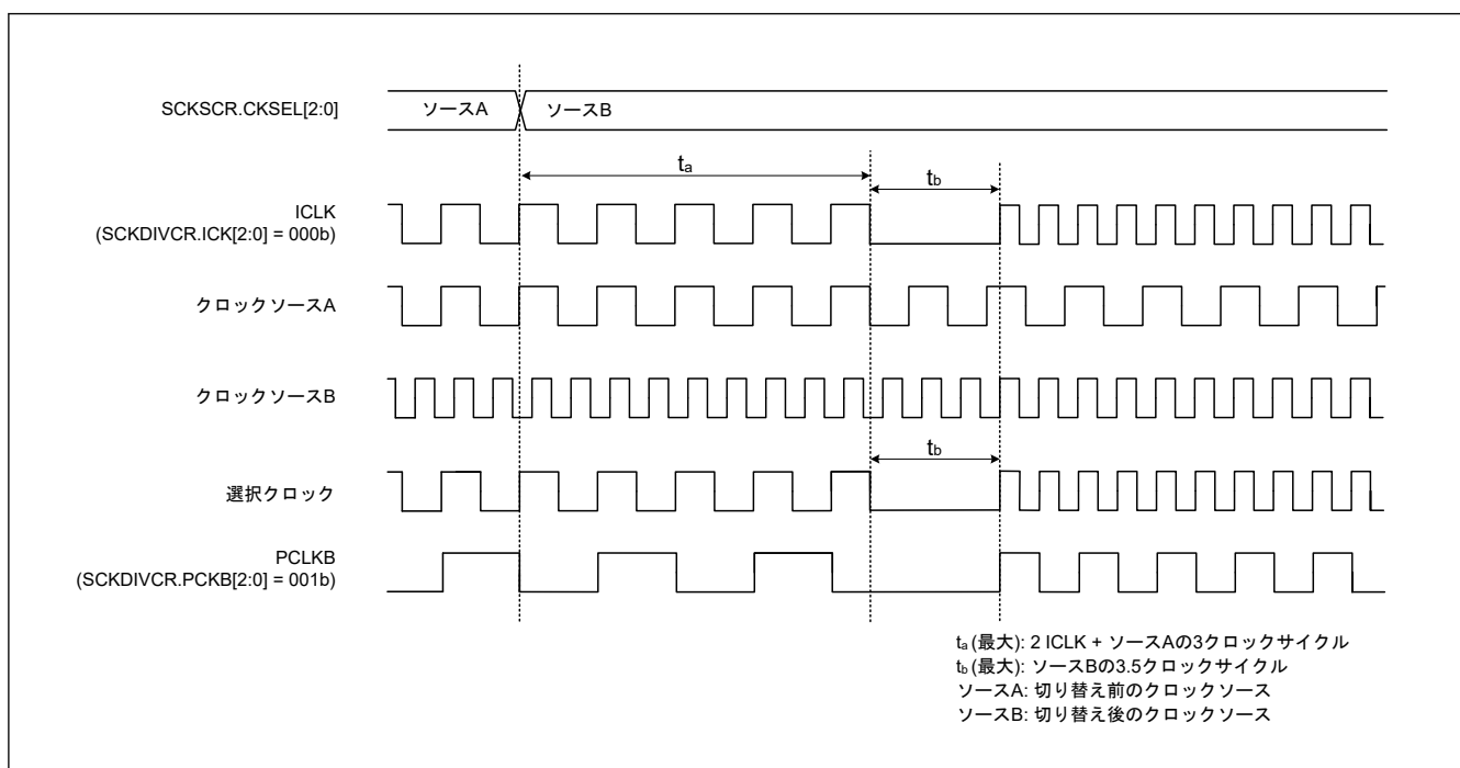
図 8.10 クロックソース切り替えのタイミング
