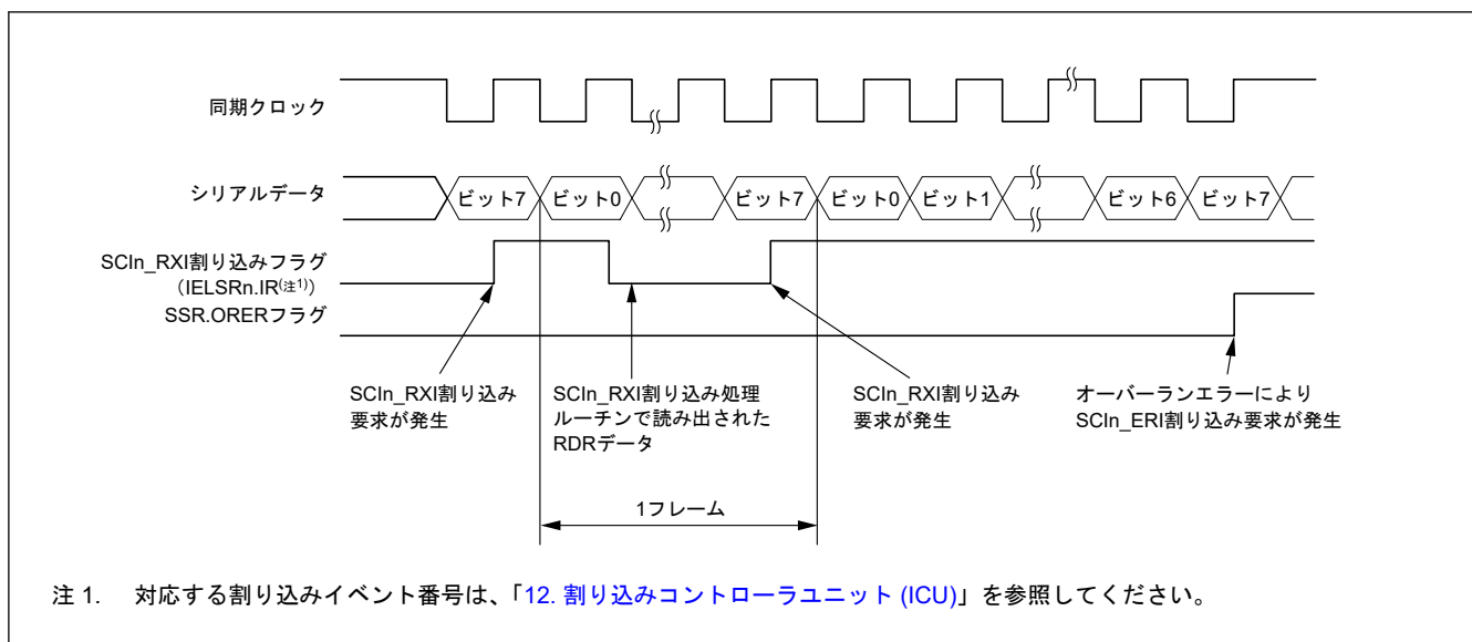
図 24.68 クロック同期式モードにおけるシリアル受信の動作例 (1) (RTS 機能を使用しない場合)
