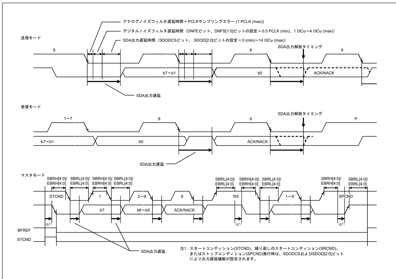
図 25.111 SDA 出力遅延機能
