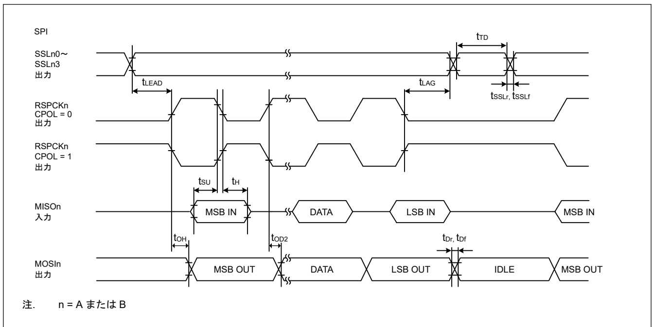
図 44.37 CPHA = 1 の場合におけるマスタの SPI タイミング
