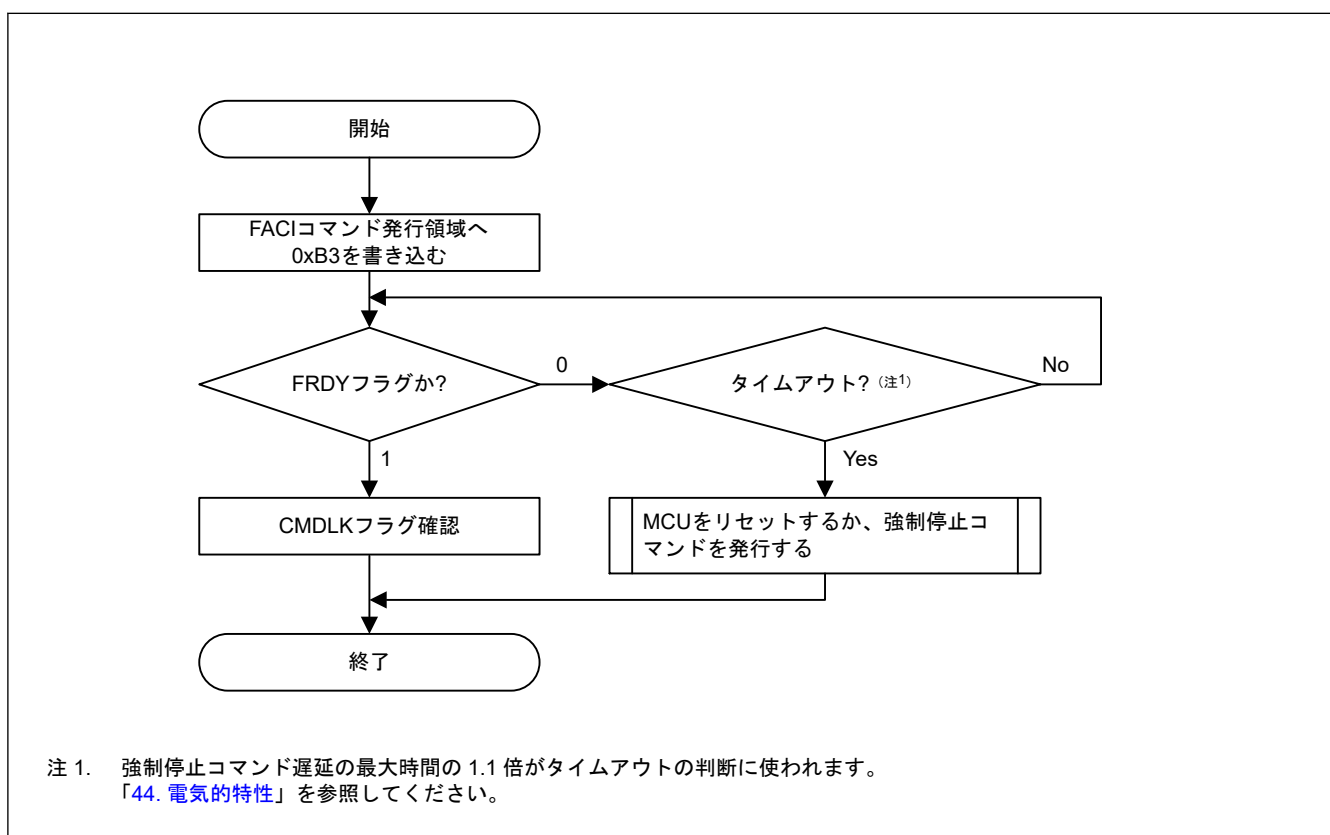
図 41.22 強制停止コマンドの使用フロー
