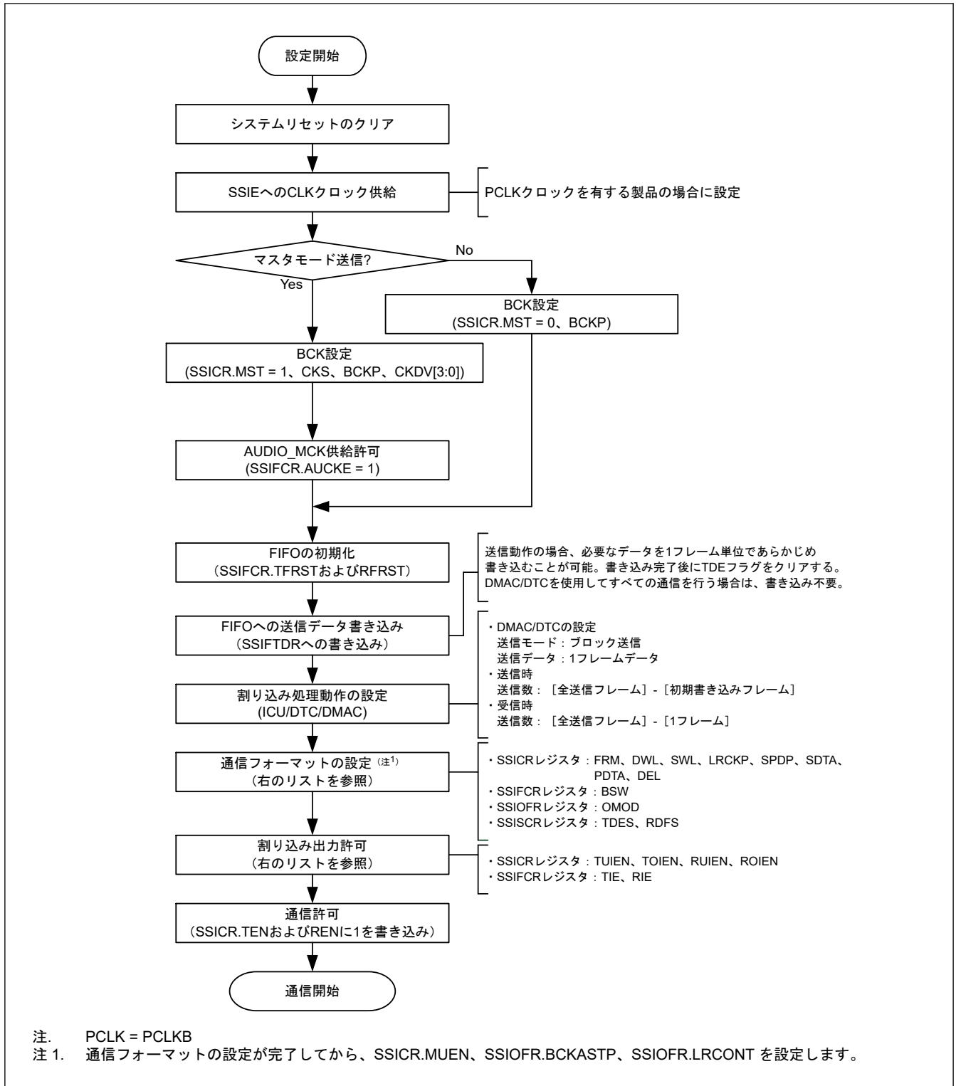
図 32.53 通信開始手順 (CPU 動作手順)
