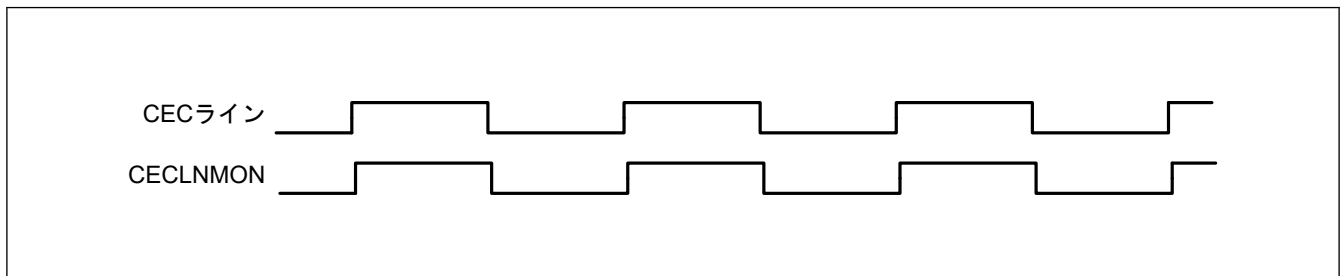
図 31.31 CECLNMON ビットのタイミング
