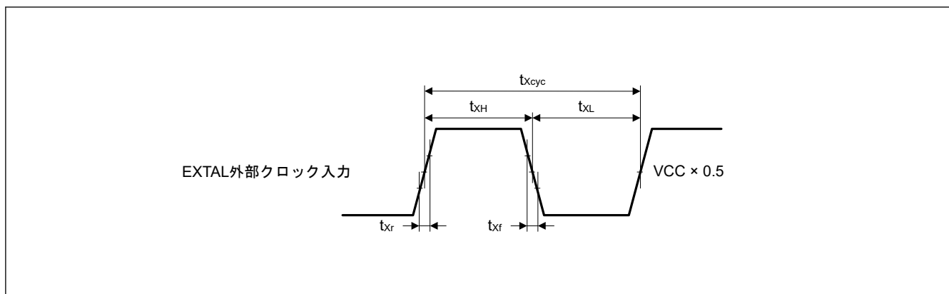
図 44.7 EXTERNAL 外部クロック入力タイミング
