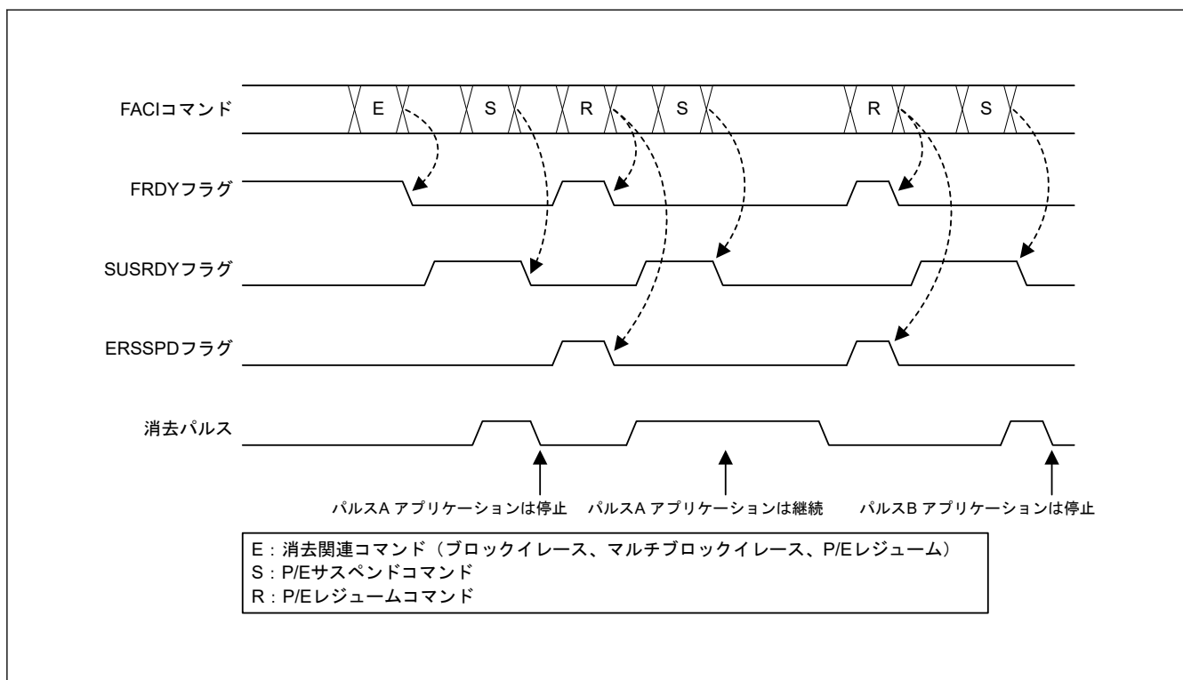
図 41.18 消去中のサスペンド (サスペンド優先モード)
