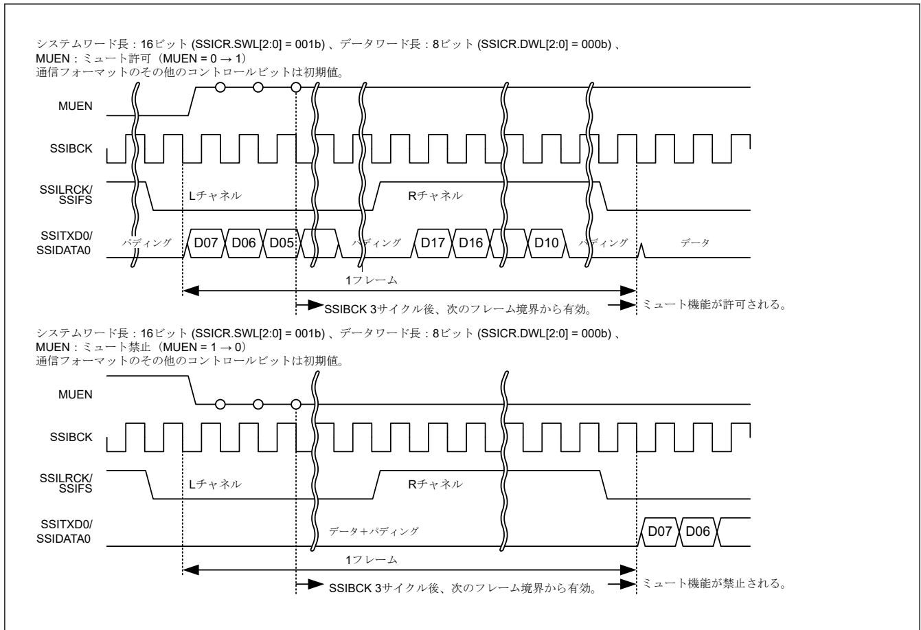
図 32.5 ミュート機能設定時のデータ送信
