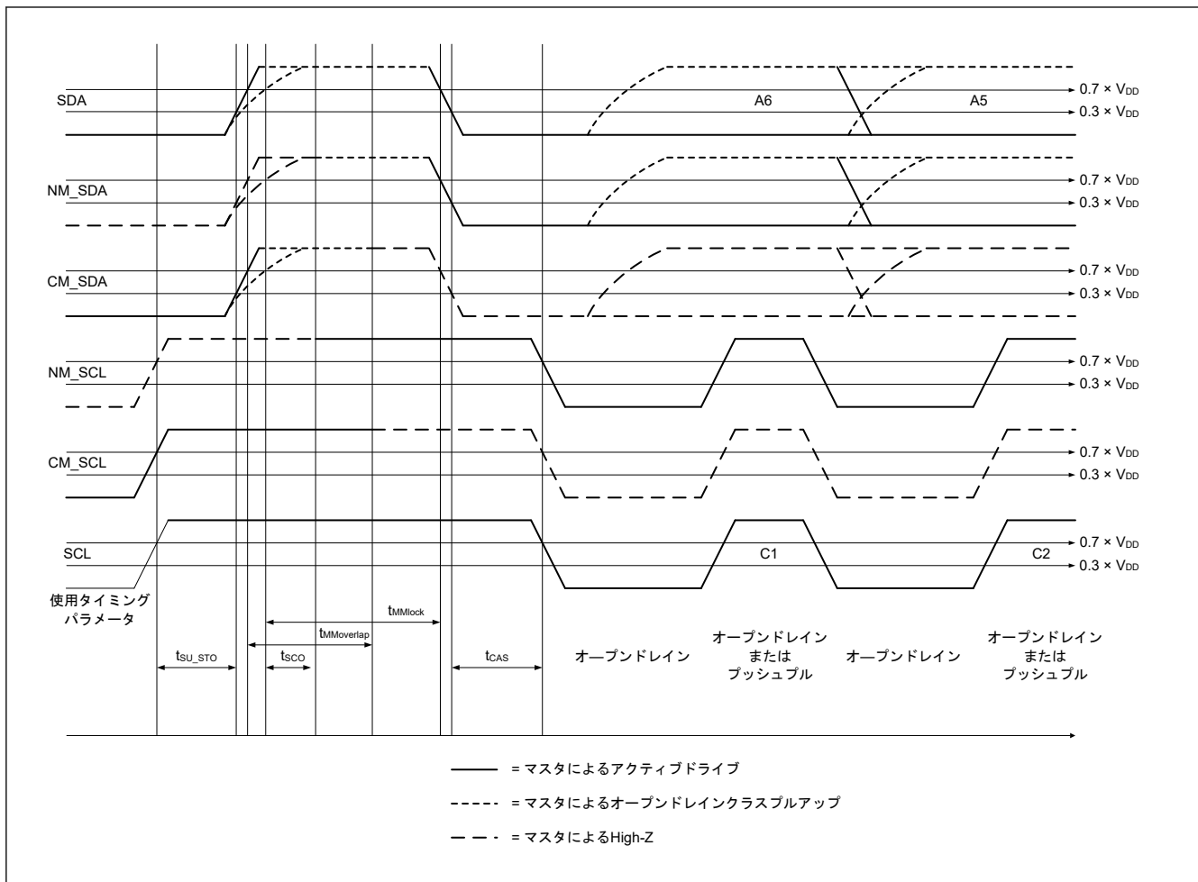
図 44.51 I3C タイミング (オープンドレインタイミングパラメータ)
