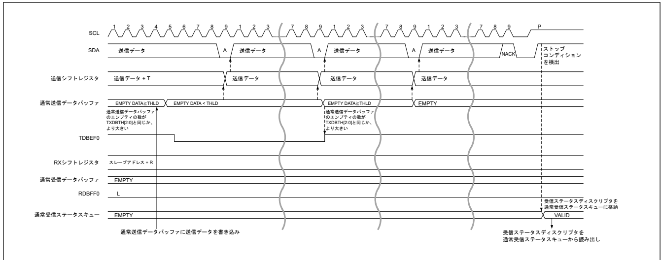
図 27.42 レガシー I 2 C メッセージデータ読み出し転送タイミング (2/2)
