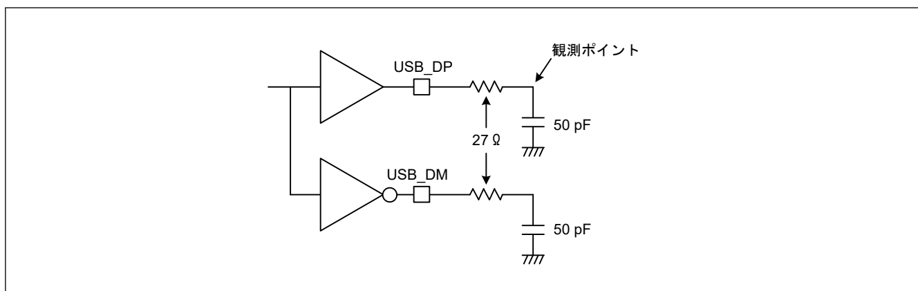
図 44.59 フルスピードモードにおける測定回路
