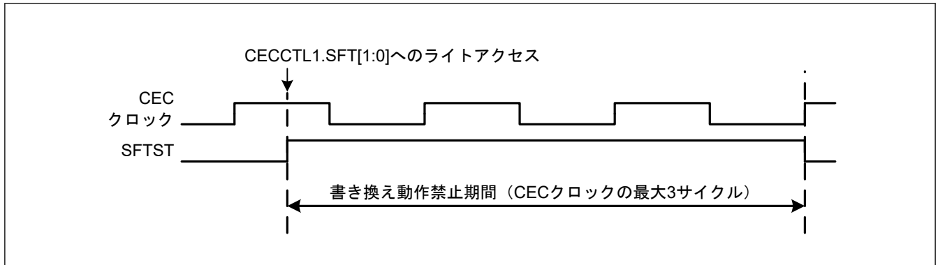
図 31.30 SFTST ビットのタイミング
