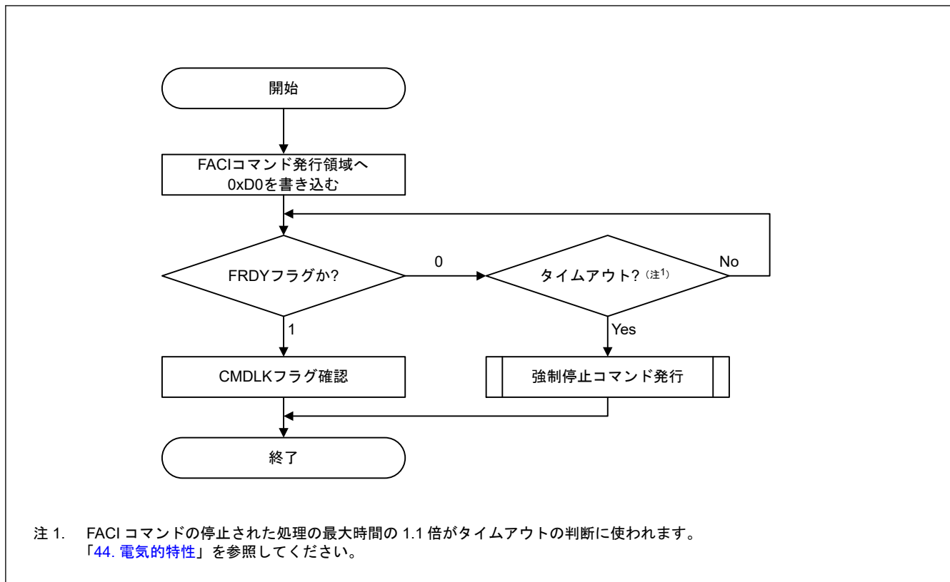
図 41.20 P/E レジュームコマンドの使用フロー
