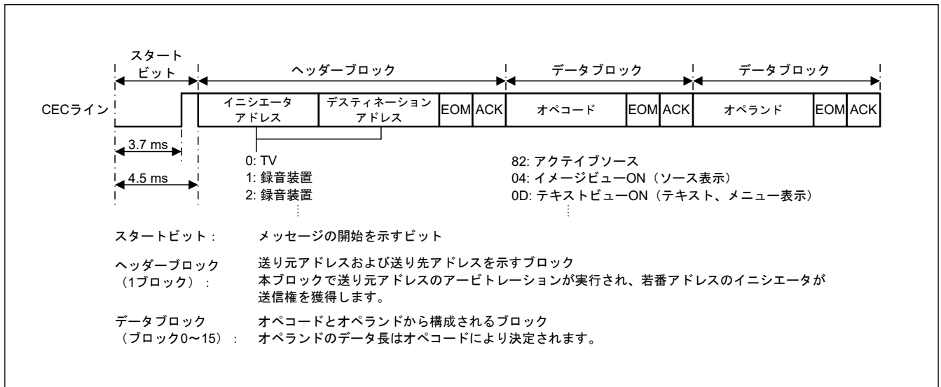
図 31.5 CEC 通信フォーマット
