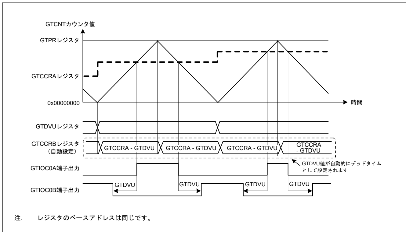
図 20.29 デッドタイム付きコンペアマッチ値の自動設定機能の動作例(三角波 PWM モード 1、GTDVU/GTDDVD レジスタはバッファ動作、アクティブ High の場合)
