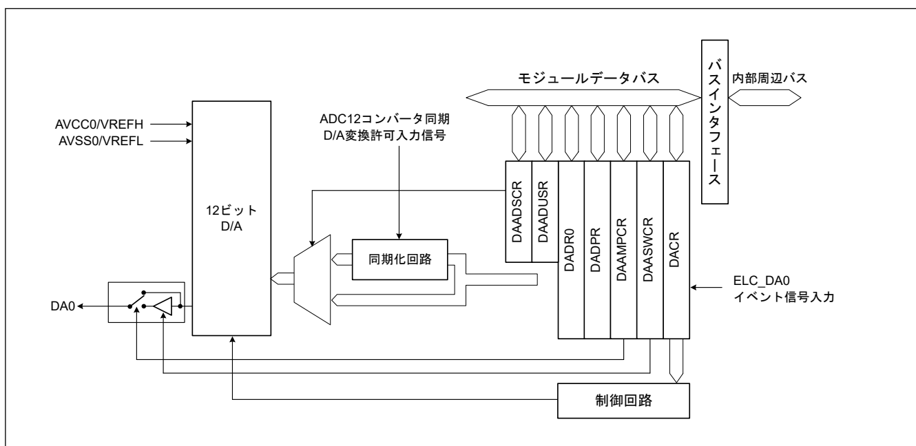
図 36.1 DAC12 のブロック図
