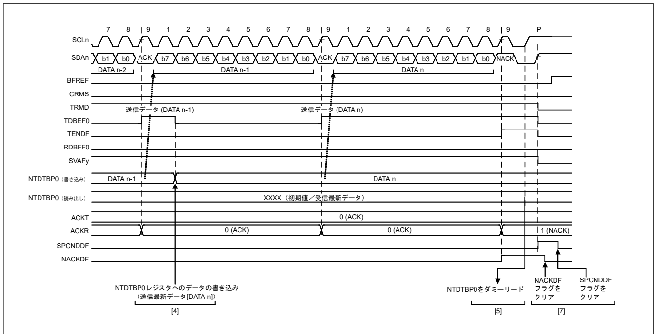
図 27.30 スレーブ送信の動作タイミング (2)
