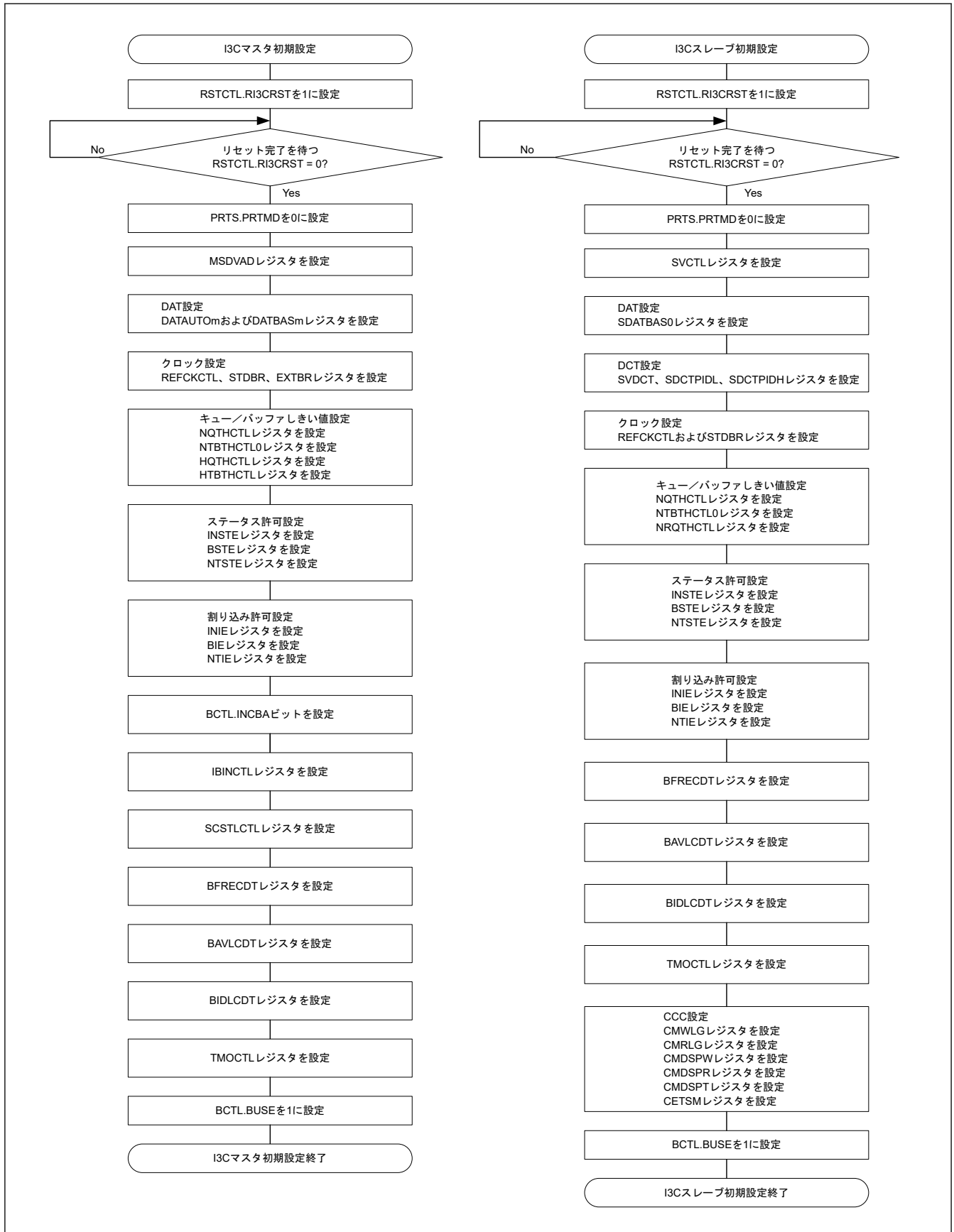
図 27.114 I3C の初期化フローチャート例
