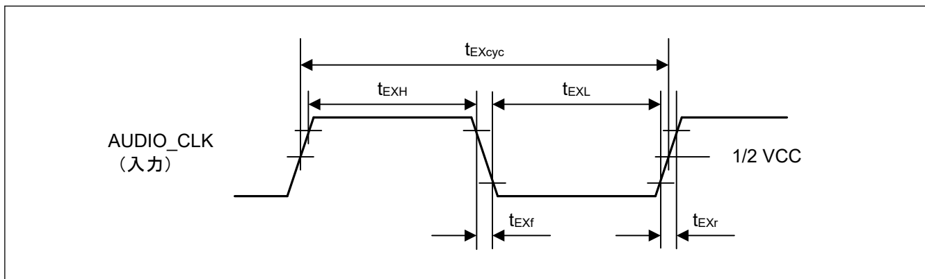
図 44.53 クロック入力タイミング
