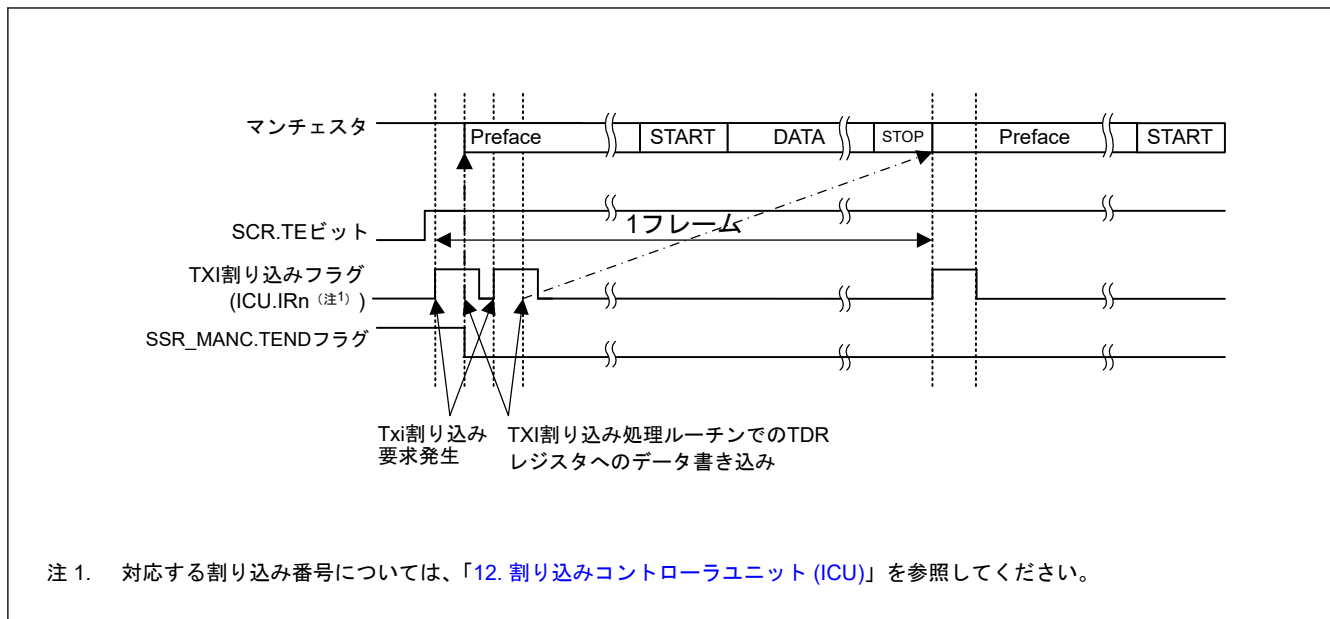
図 26.53 マンチェスタモードにおけるシリアル送信の送信開始動作の例 (プレフィスあり、CTS 機能なし)
