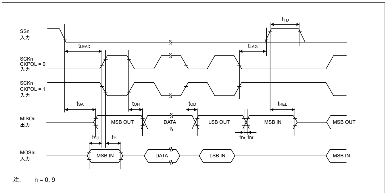
図 44.31 CKPH = 1 の場合におけるスレーブの SCI 簡易 SPI モードタイミング
