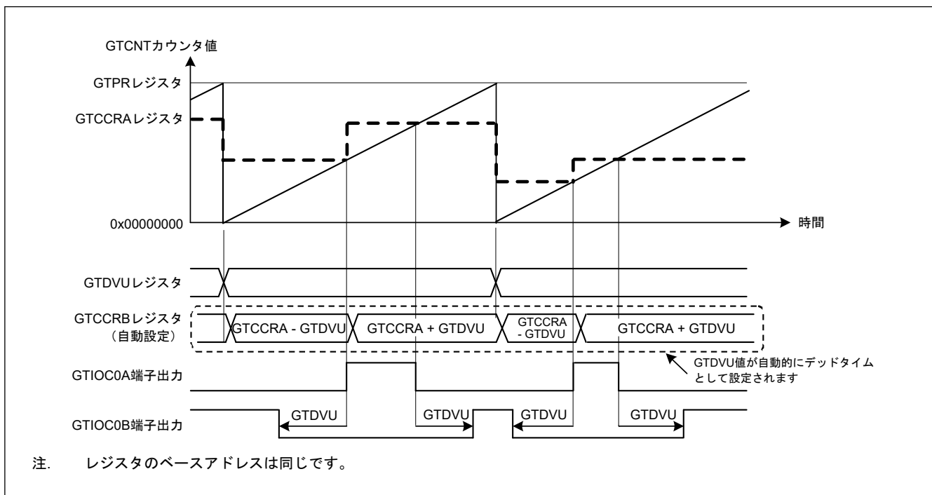
図 20.27 デッドタイム自動設定機能の動作例(のこぎり波ワンショットパルスモード、アップカウント、GTDVU/GTDVD レジスタはバッファ動作、アクティブ High の場合)
