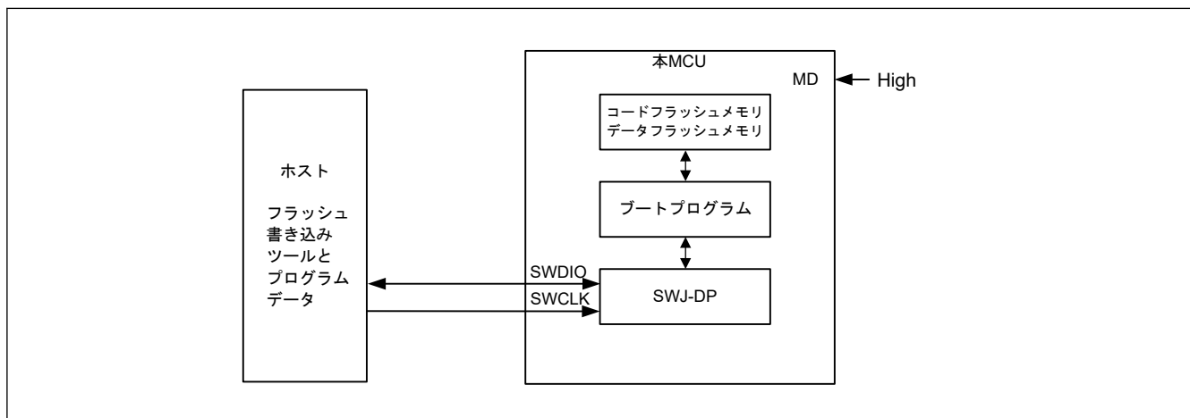
図 41.39 フラッシュメモリ関連モジュールのブロック図
