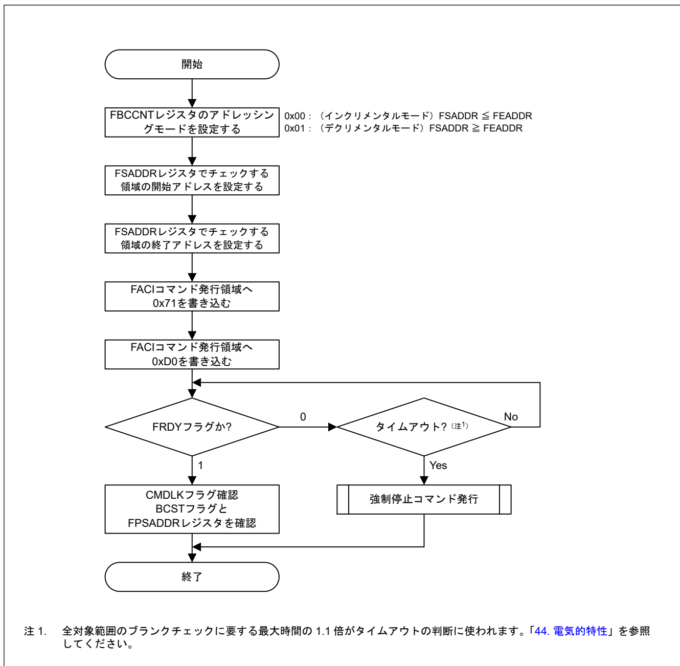
図 41.23 ブランクチェックコマンドの使用フロー
