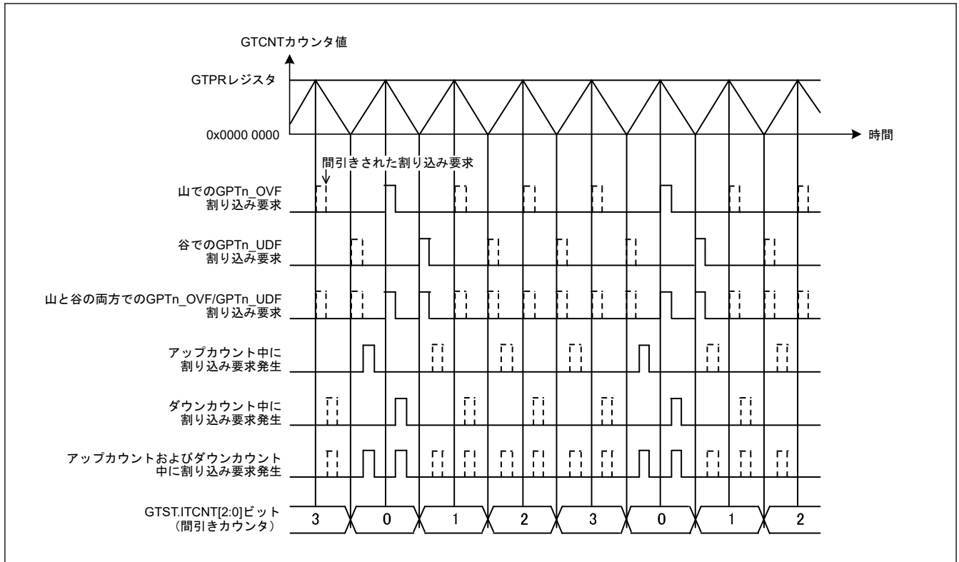
図 20.70 割り込み間引き機能の動作例 (三角波、谷をカウントして間引き、間引き回数 3 の場合)
