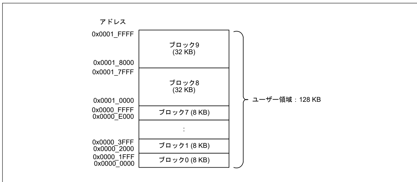
図 41.2 コードフラッシュメモリのマップ
