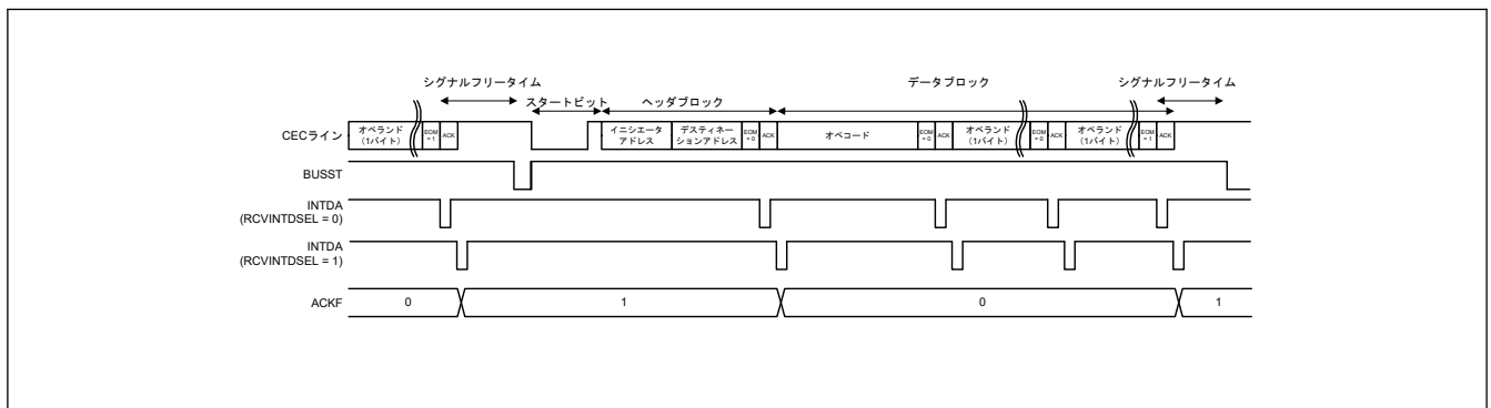
図 31.32 ACKF ビットのタイミング
