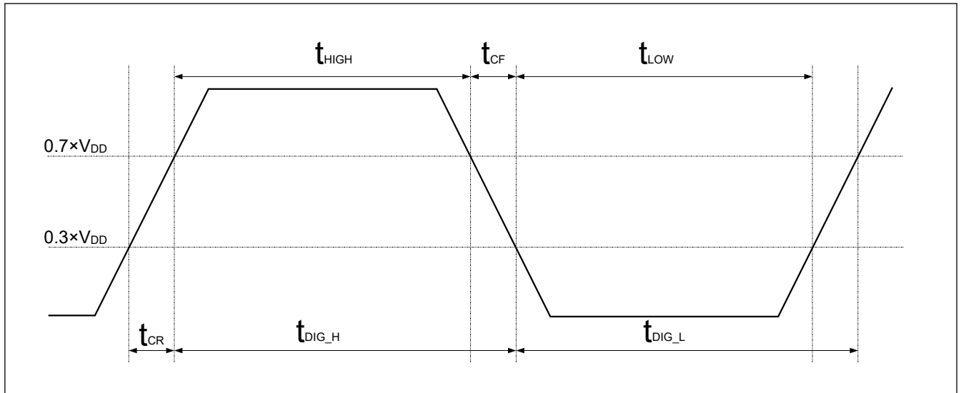
図 44.43 t_{DIG\_H} 、 t_{DIG\_L}
