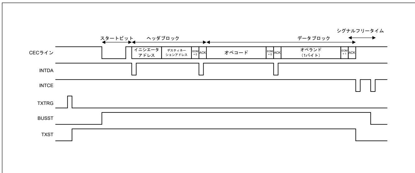
図 31.26 通常送信動作中の送信ステータスフラグのタイミング
