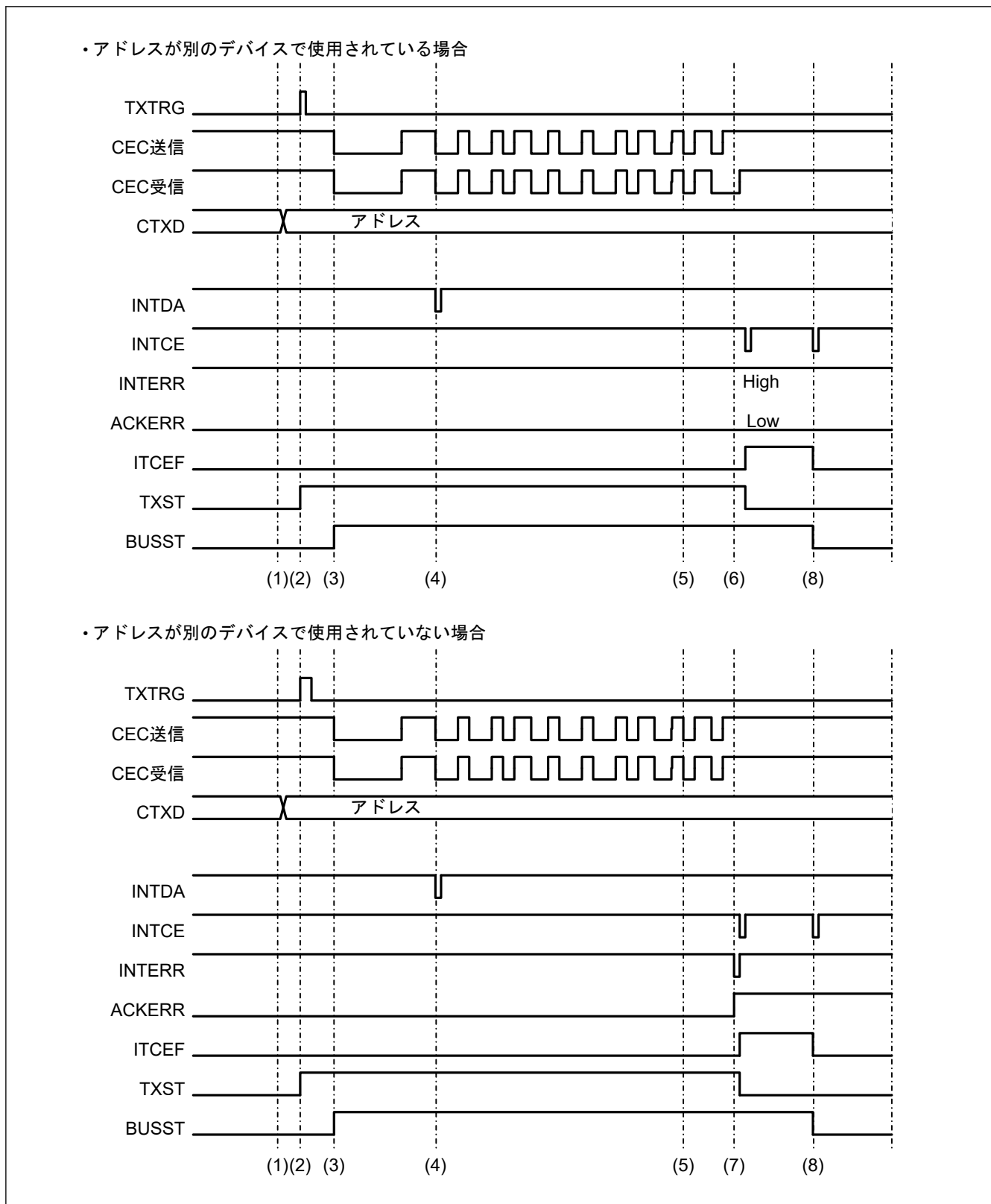
図 31.15 ロジカルアロケーション (CECCTL1.CESEL[1:0] = 00b のとき)
