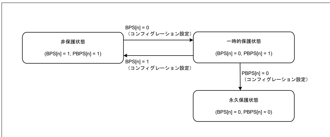
図 41.29 BPS[n]ビットおよび PBPS[n]ビットによるフラッシュシーケンサの状態遷移
