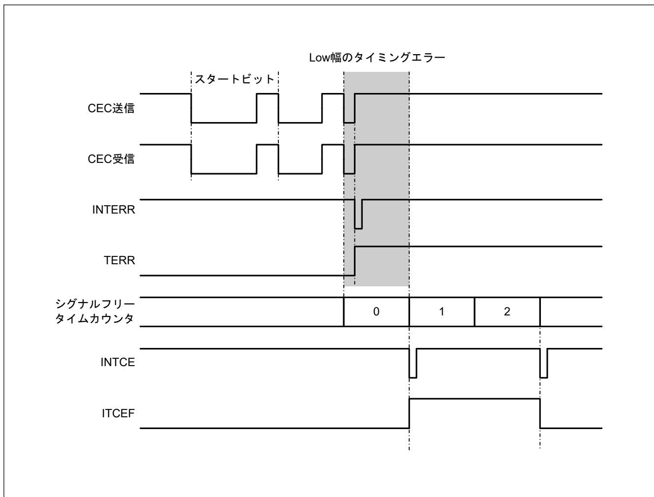
図 31.40 イニシエータ動作時のタイミングエラー
