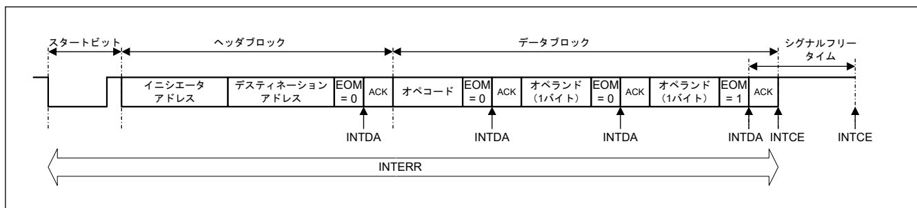
図 31.21 受信割り込みタイミング基本タイミング
