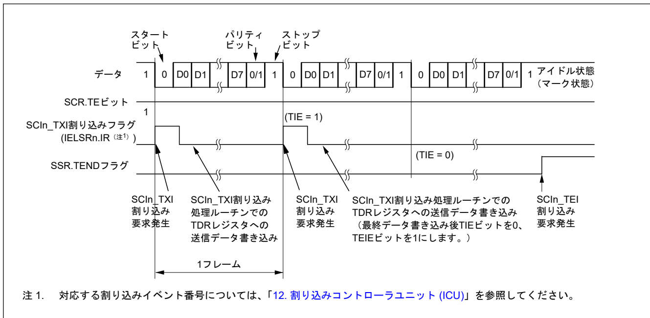
図 26.10 調歩同期式モードにおけるシリアル送信の動作例 (3) (8 ビットデータ/パリティあり/1ストップビット/CTS 機能不使用/送信中~送信終了時)
