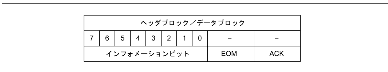
図 31.8 ヘッダブロック、データブロックのフォーマット
