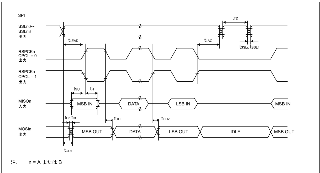
図 44.35 CPHA = 0 の場合におけるマスタの SPI タイミング
