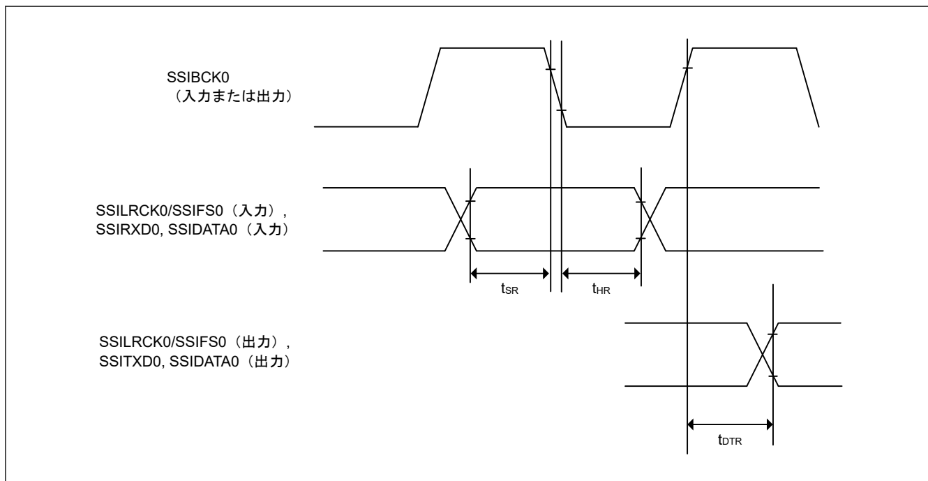
図 44.55 SSICR.BCKP = 1 の場合の SSIE データ送受信タイミング
