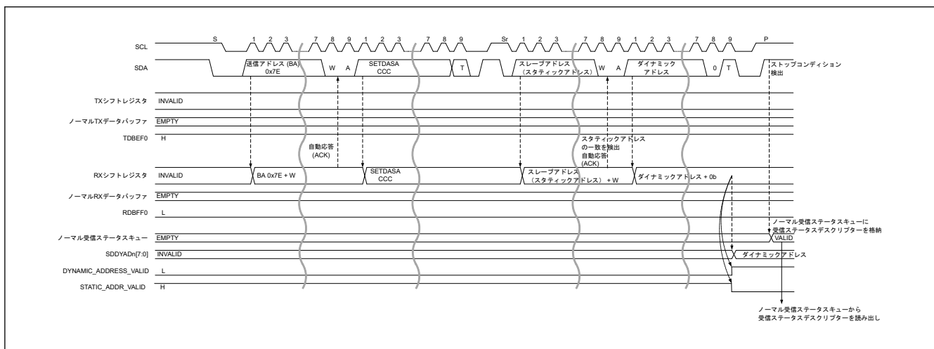
図 27.34 ダイナミックアドレス配置手順 (SETDASAs CCC) タイミング
