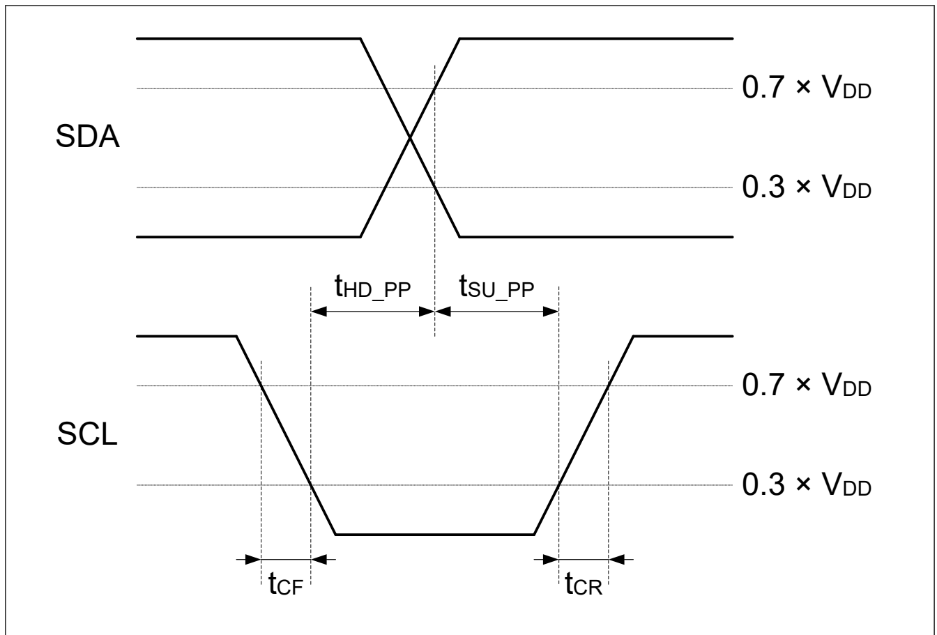
図 44.47 I3C マスタ出カタイミング
