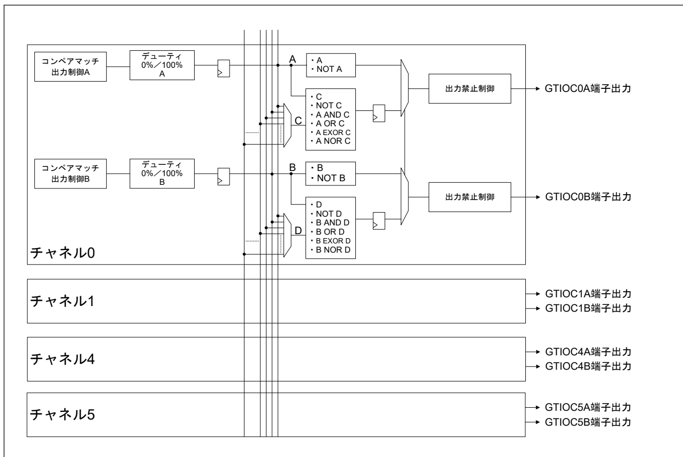
図 20.67 チャンネル間論理演算のブロック図
