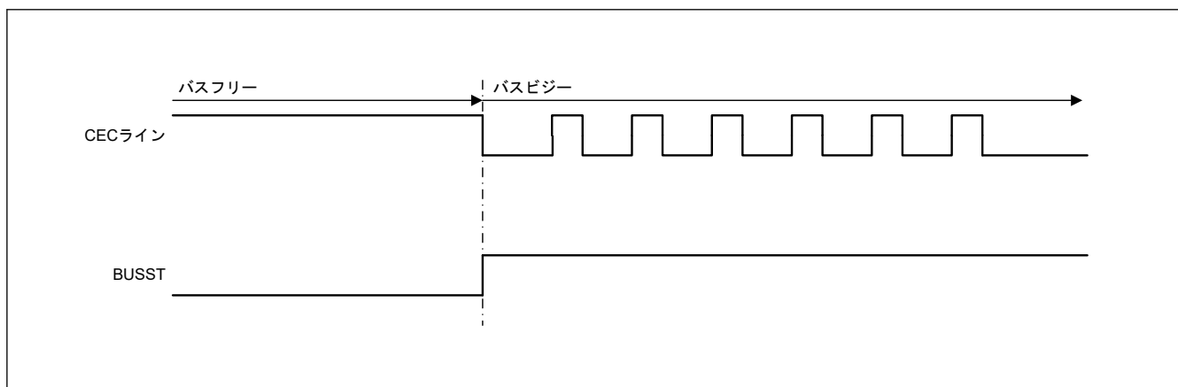
図 31.24 CEC ラインの立ち下がり検出タイミング
