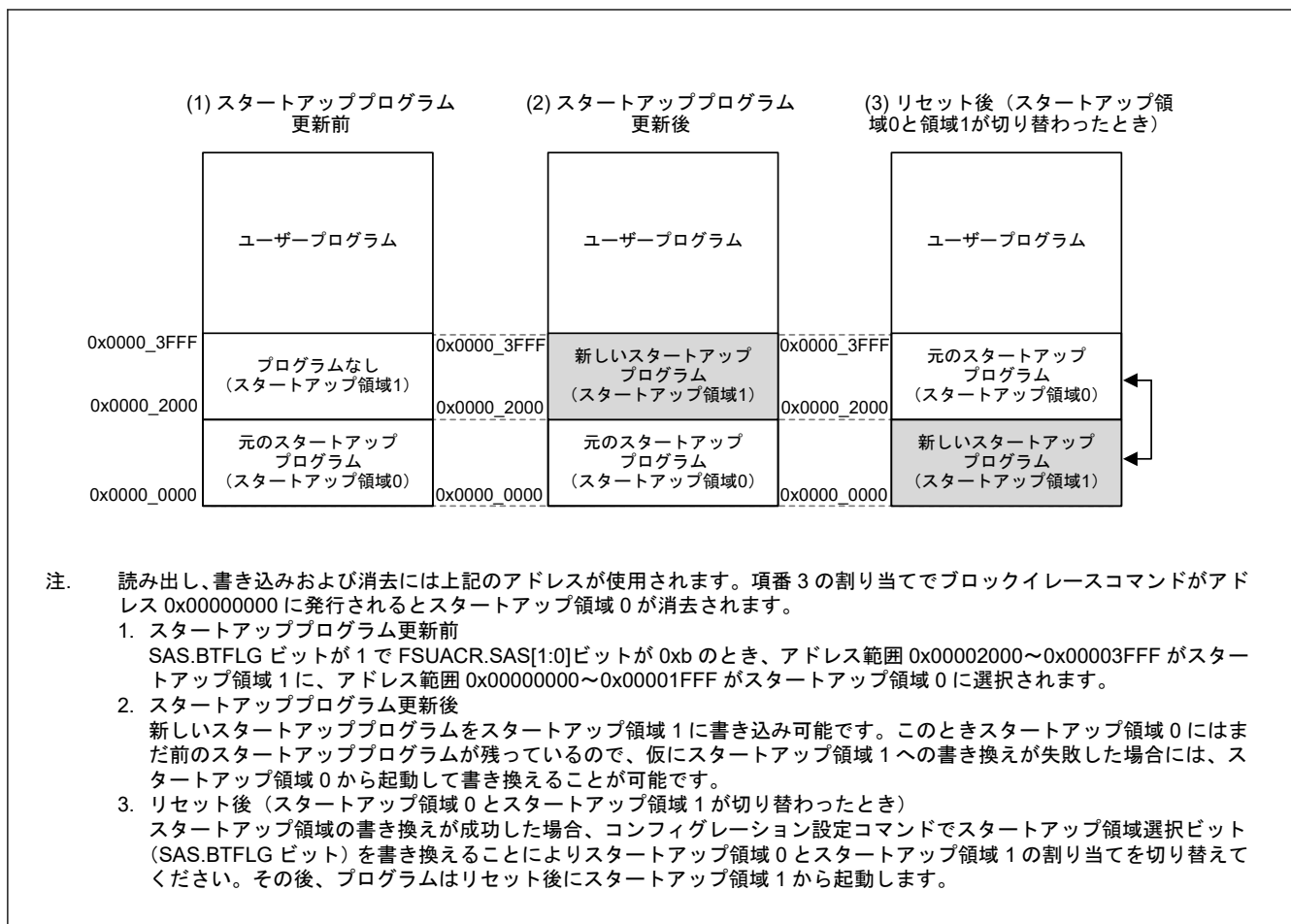
図 41.25 スタートアッププログラムプロテクションの概念
