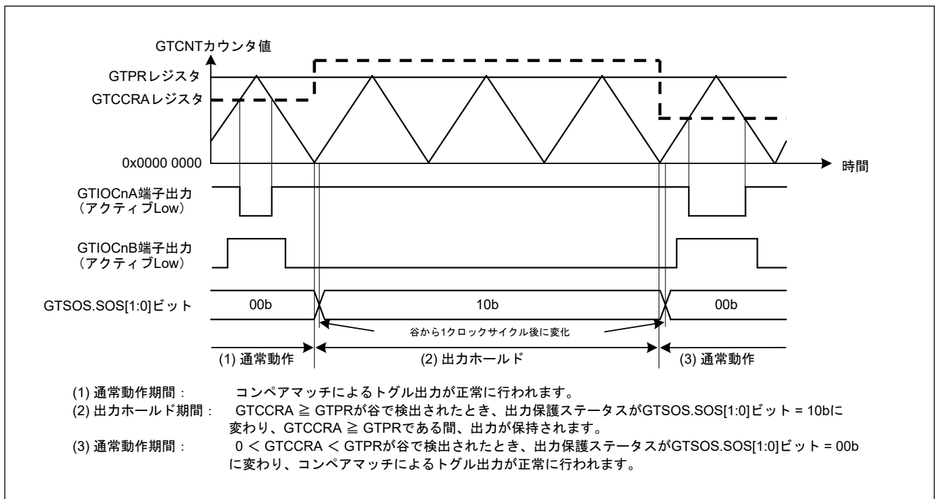
図 20.87 谷でのバッファ転送中に GTCCRA \geq GTPR となったときの出力保護機能の動作例 (谷でのバッファ転送中に 0 < GTCCRA < GTPR に復帰、アクティブレベルは Low) ( n = 0, 1, 4, 5 )
