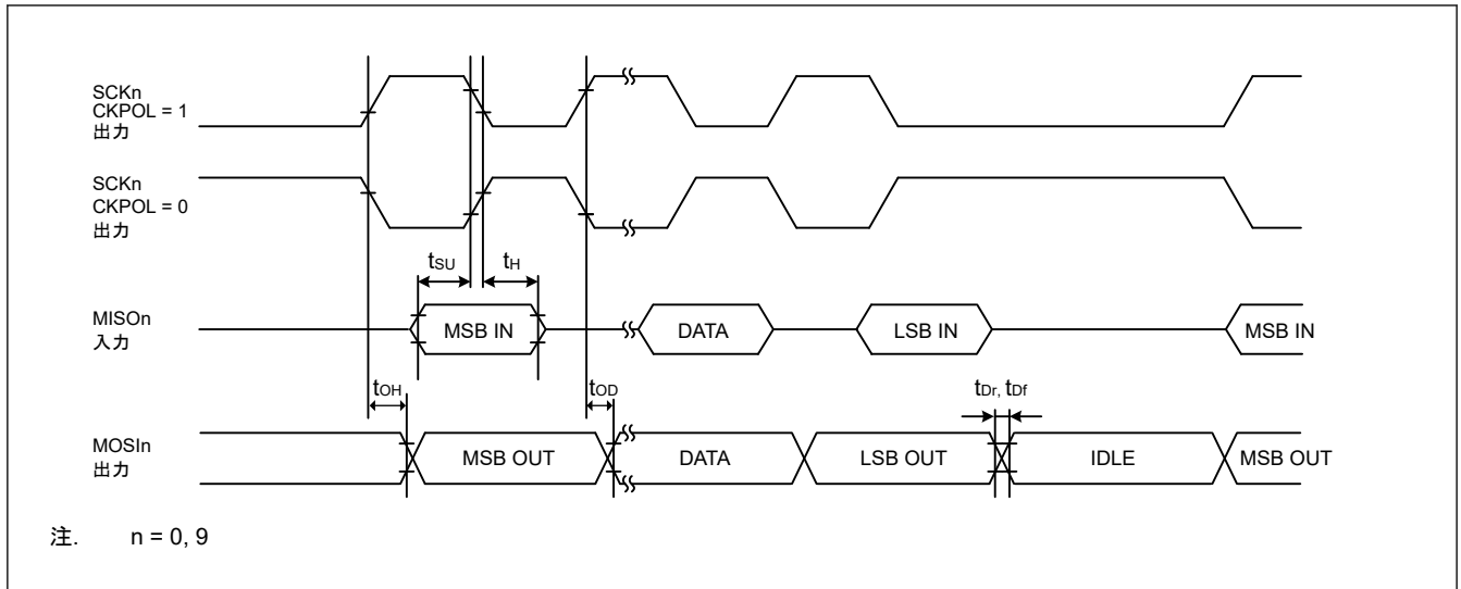
図 44.30 CKPH = 0 の場合におけるマスタの SCI 簡易 SPI モードタイミング
