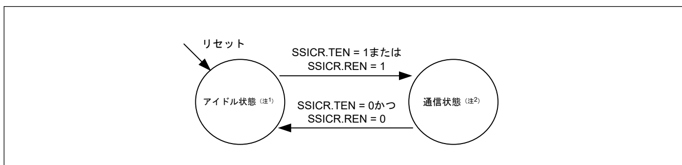
図 32.43 SSIE の状態遷移
