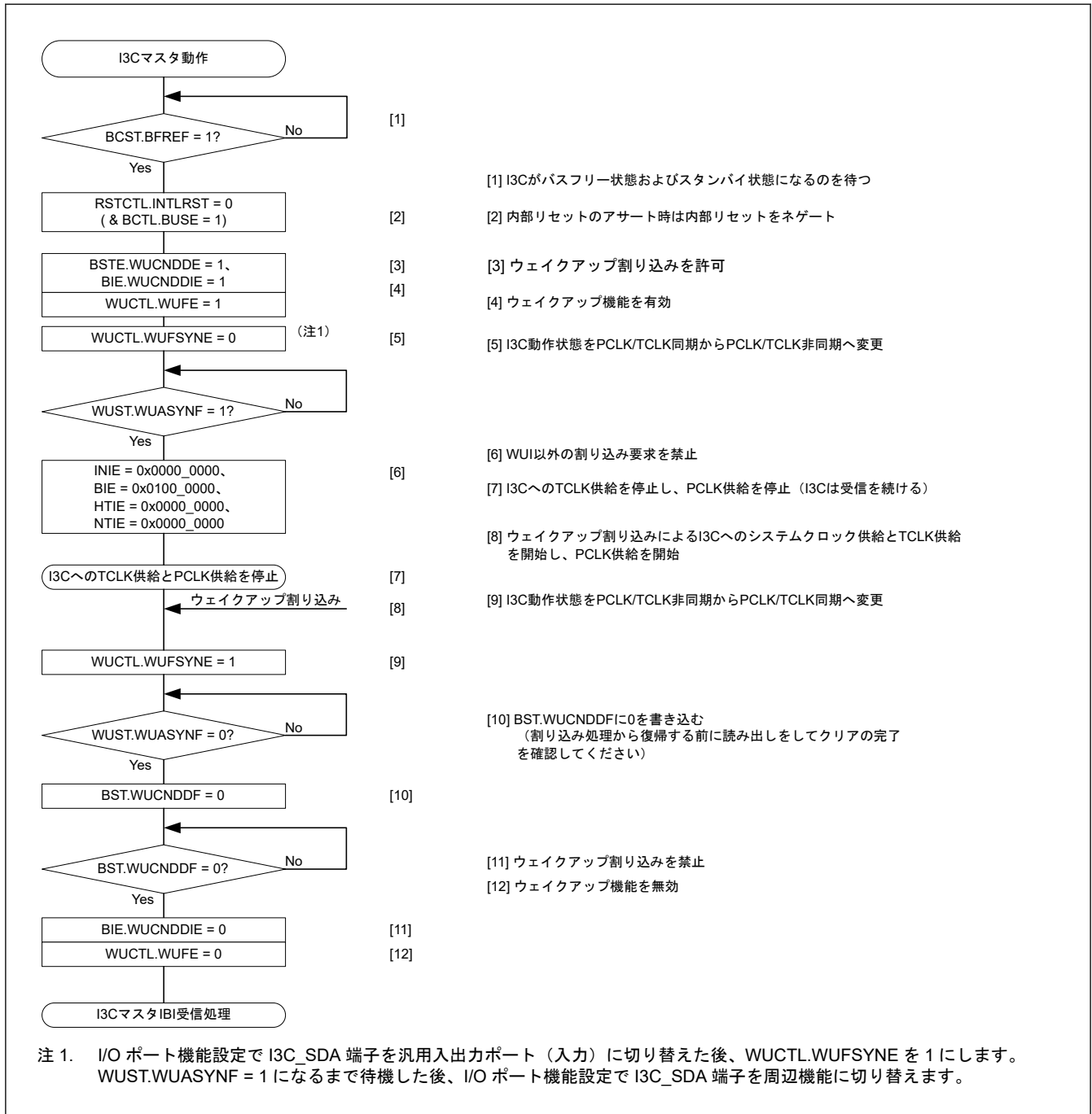
図 27.124 I3C マスタウェイクアップの使用例
