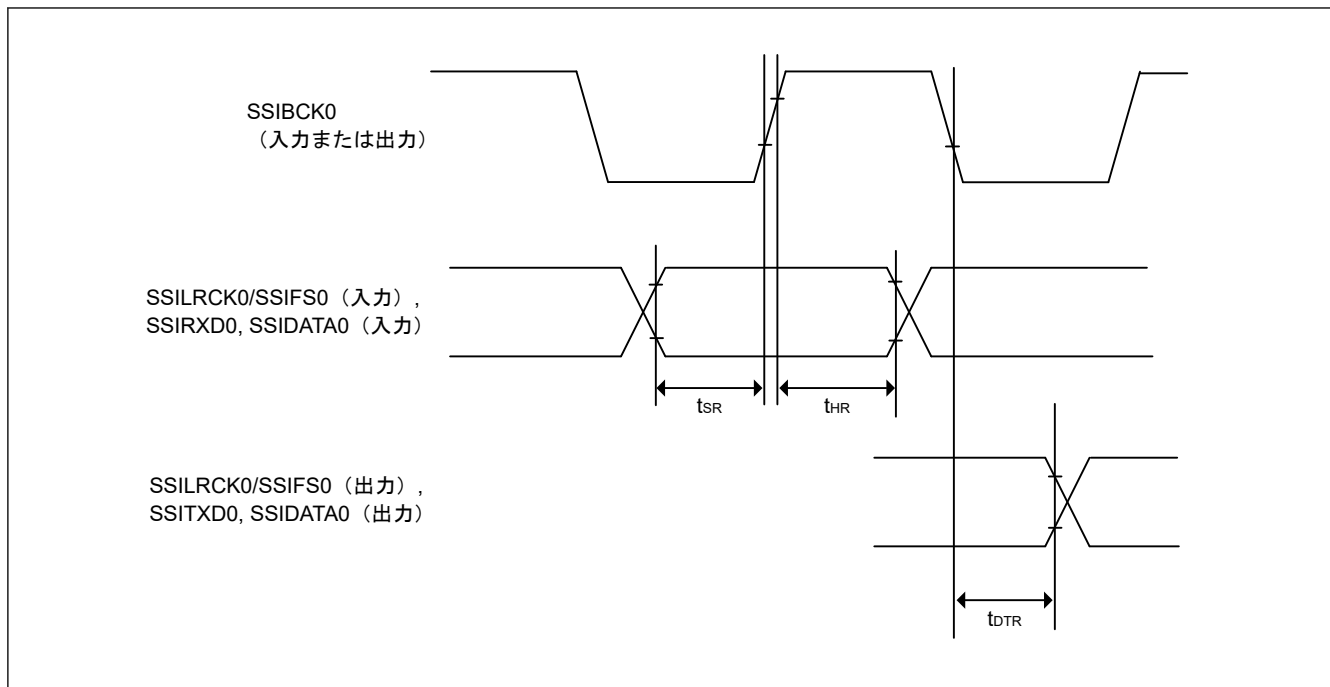
図 44.54 SSICR.BCKP = 0 の場合の SSIE データ送受信タイミング
