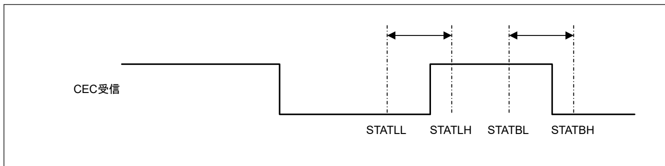
図 31.12 スタートビットの受信タイミング
