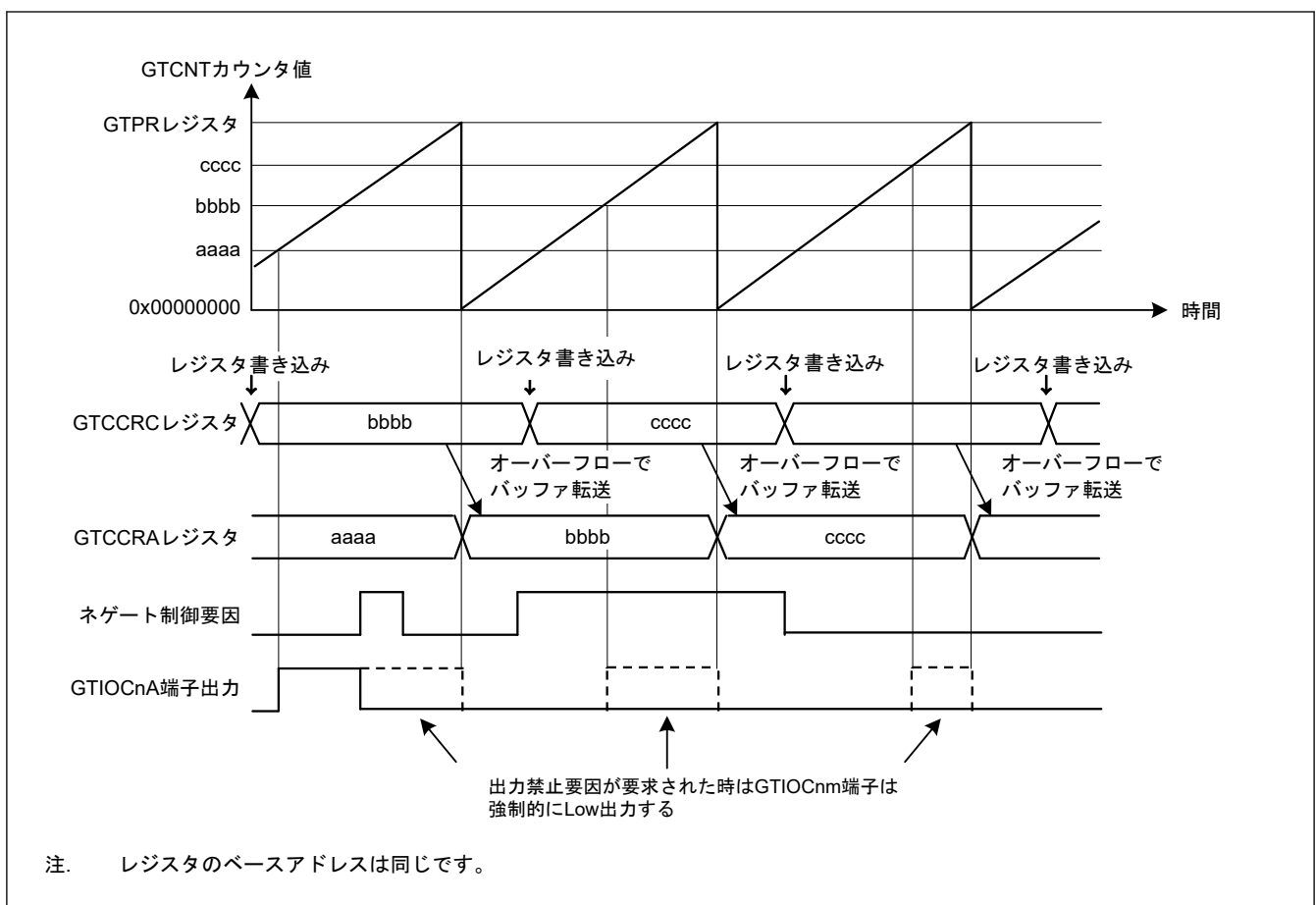
図 20.81 GTIOCnm 端子出力禁止制御動作例 (のこぎり波でアップカウント、バッファ動作、アクティブレベル 1、GTCCRA レジスタのコンペアマッチで High 出力、周期の終わりで Low 出力、出力禁止で Low 出力の場合) (n = 0, 1, 4, 5, m = A, B)
