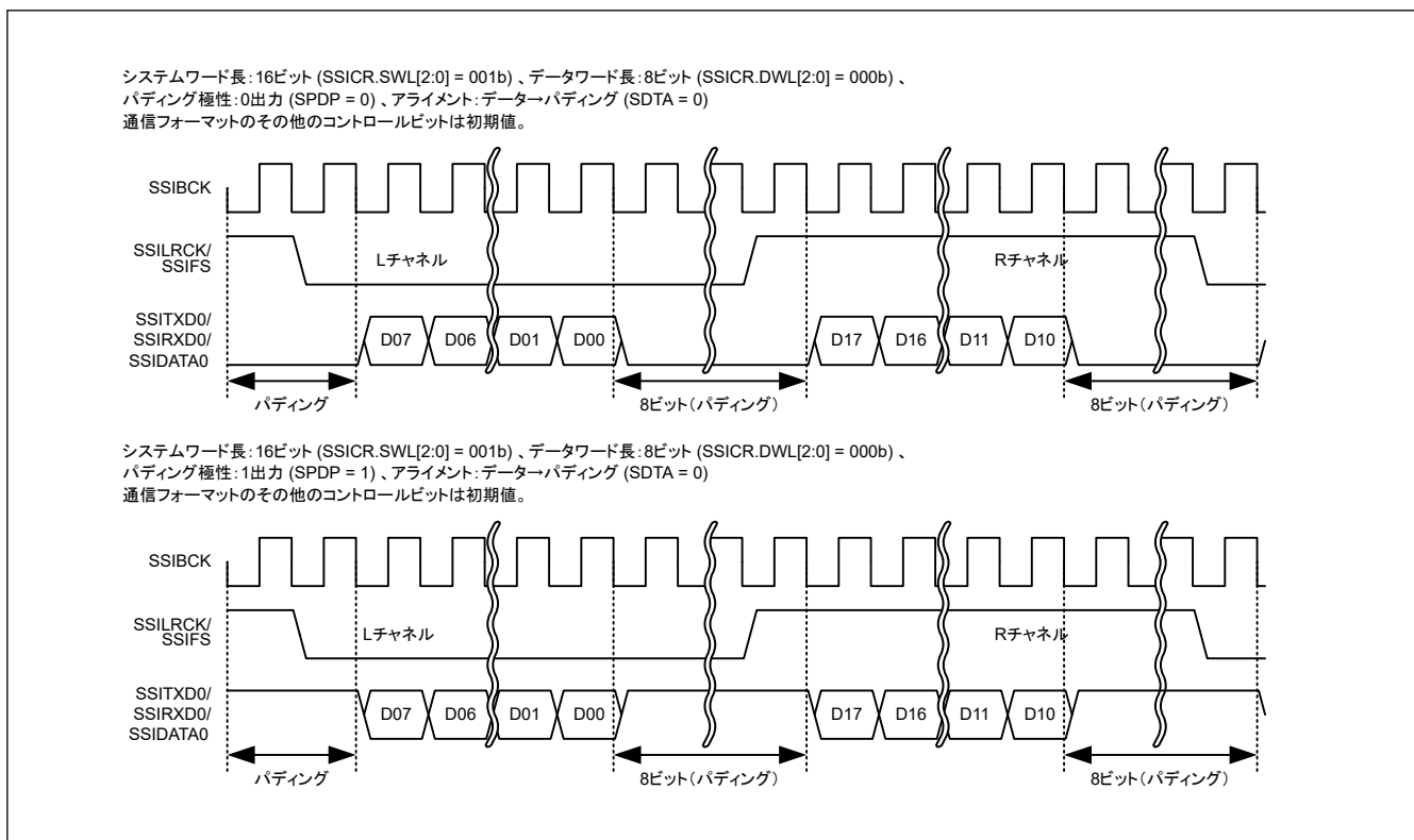
図 32.11 パディングビットの極性
