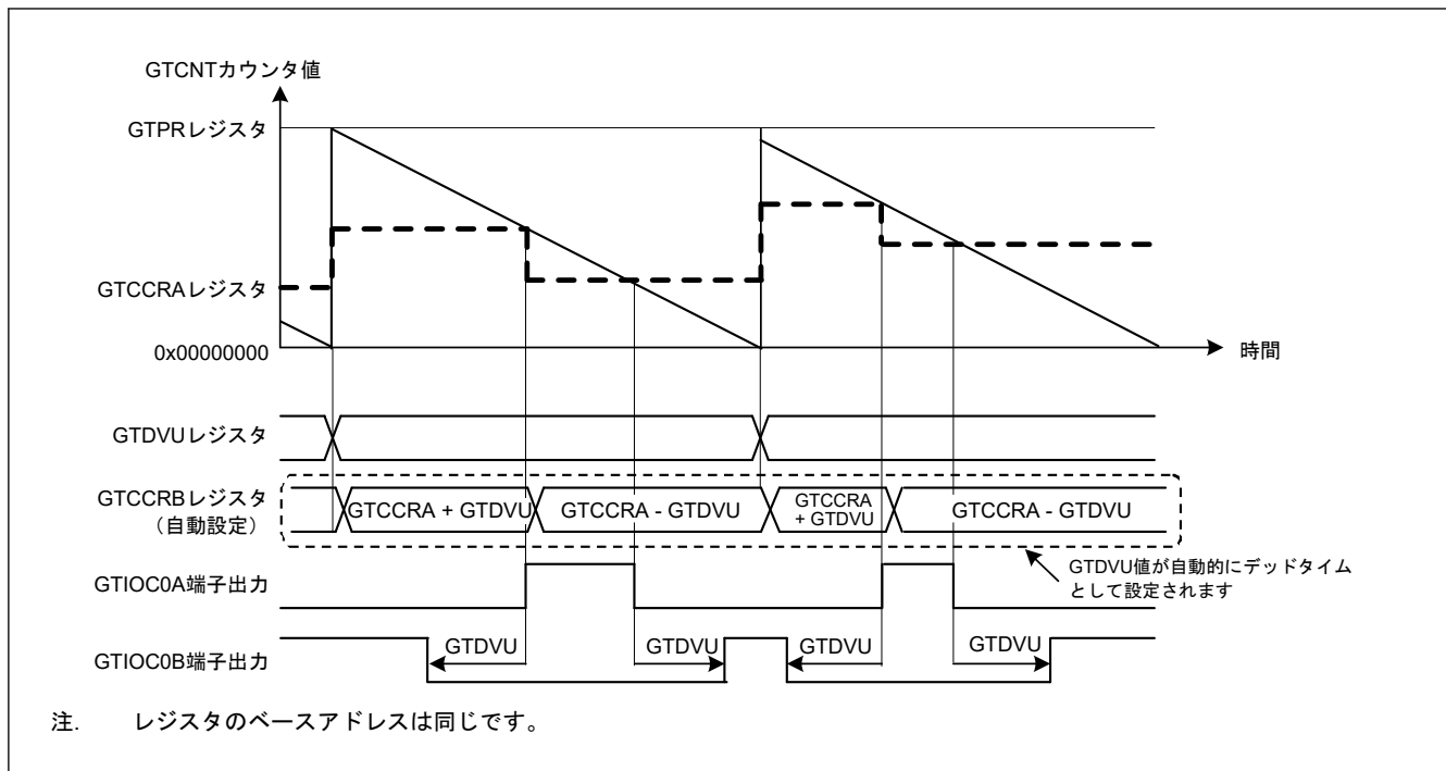
図 20.28 デッドタイム自動設定機能の動作例(のこぎり波ワンショットパルスモード、ダウンカウント、GTDVU/GTDDVD レジスタはバッファ動作、アクティブ High の場合)
