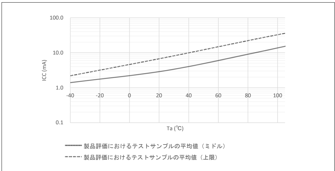
図 44.2 ソフトウェアスタンバイモード時の温度依存性 (参考データ)
