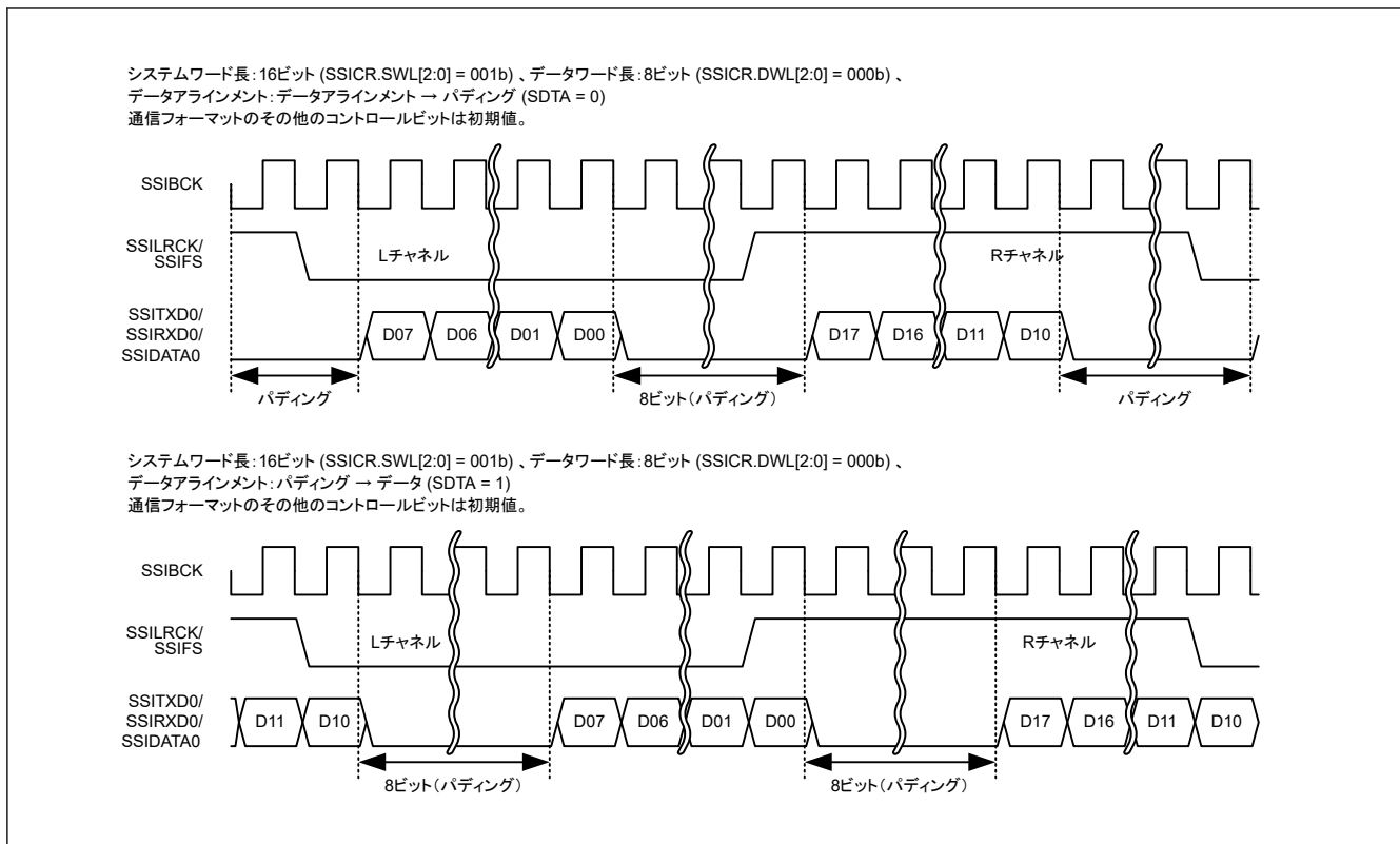
図 32.10 パディングビットを伴うシリアルデータのアライメント設定
