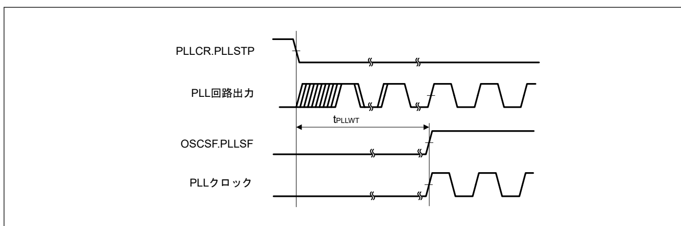
図 44.10 PLL クロック発振開始タイミング
