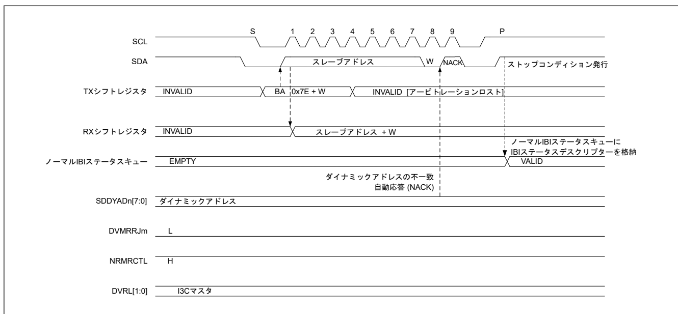
図 27.83 バス権要求 : NACK (DAT.DVDYAD[7:0]ビットが一致しない) かつ NRMRCTL が 1 の場合
