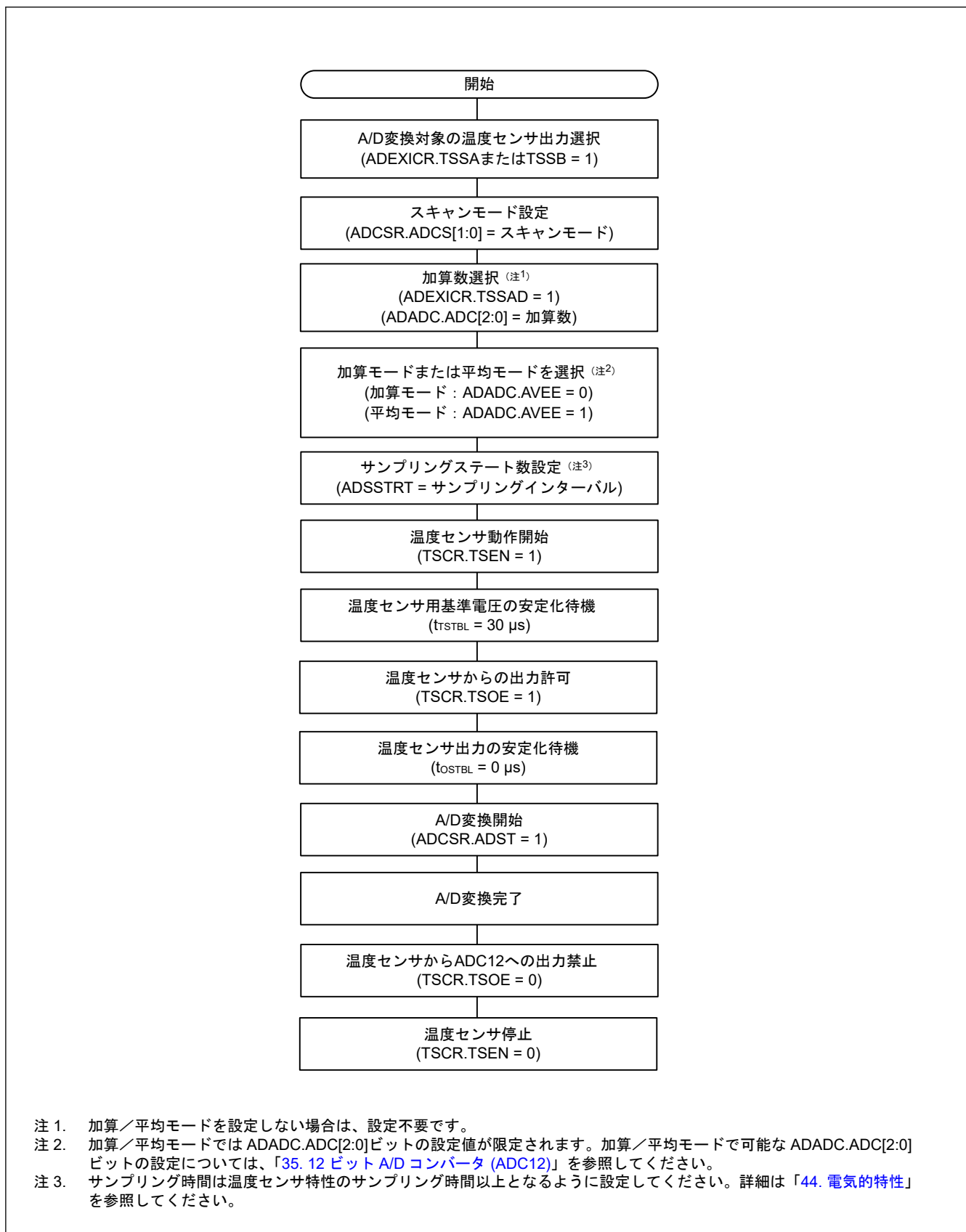
図 37.2 TSN の使用手順例
