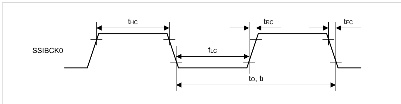
図 44.52 SSIE クロック入出力タイミング
