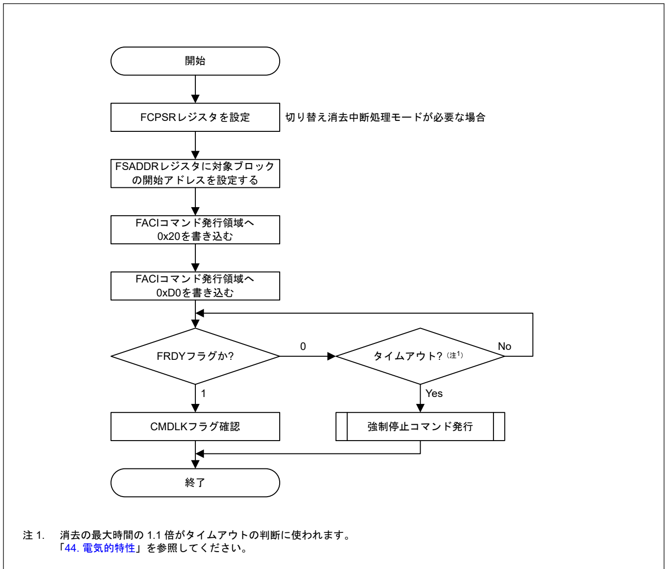
図 41.14 ブロックイレースコマンドの使用フロー
