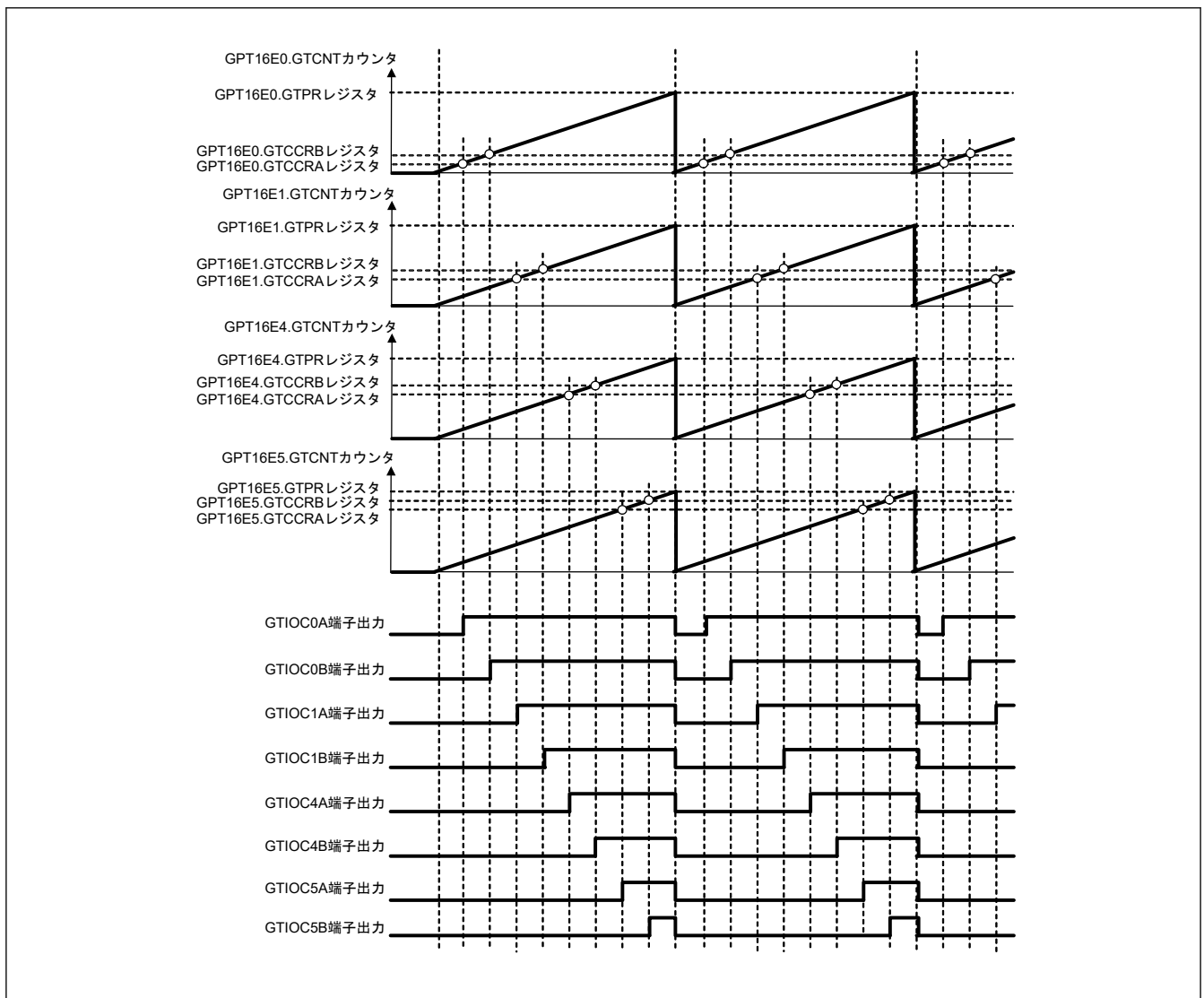
図 20.45 同期 PWM 出力例
