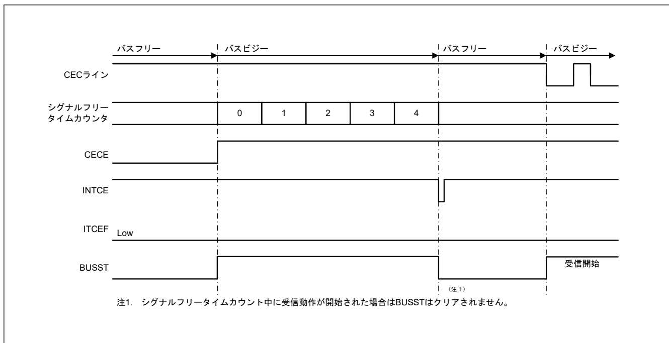
図 31.23 CECE = 1 時の受信開始時のタイミング
