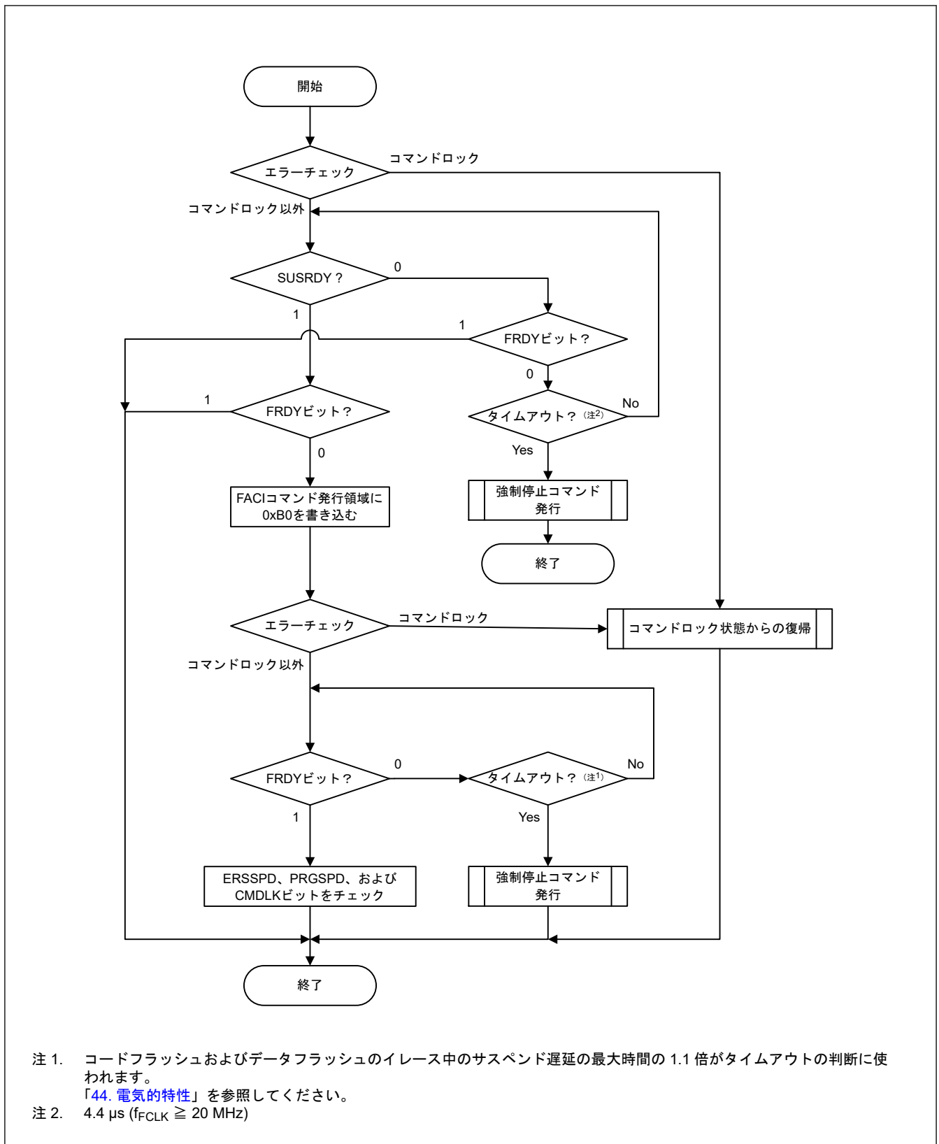
図 41.16 P/E サスペンドコマンドの使用フロー
