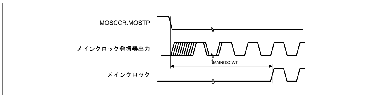
図 44.8 メインクロック発振開始タイミング
