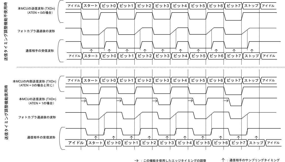
図 26.34 フォトカプラを経由する送信波形の説明
