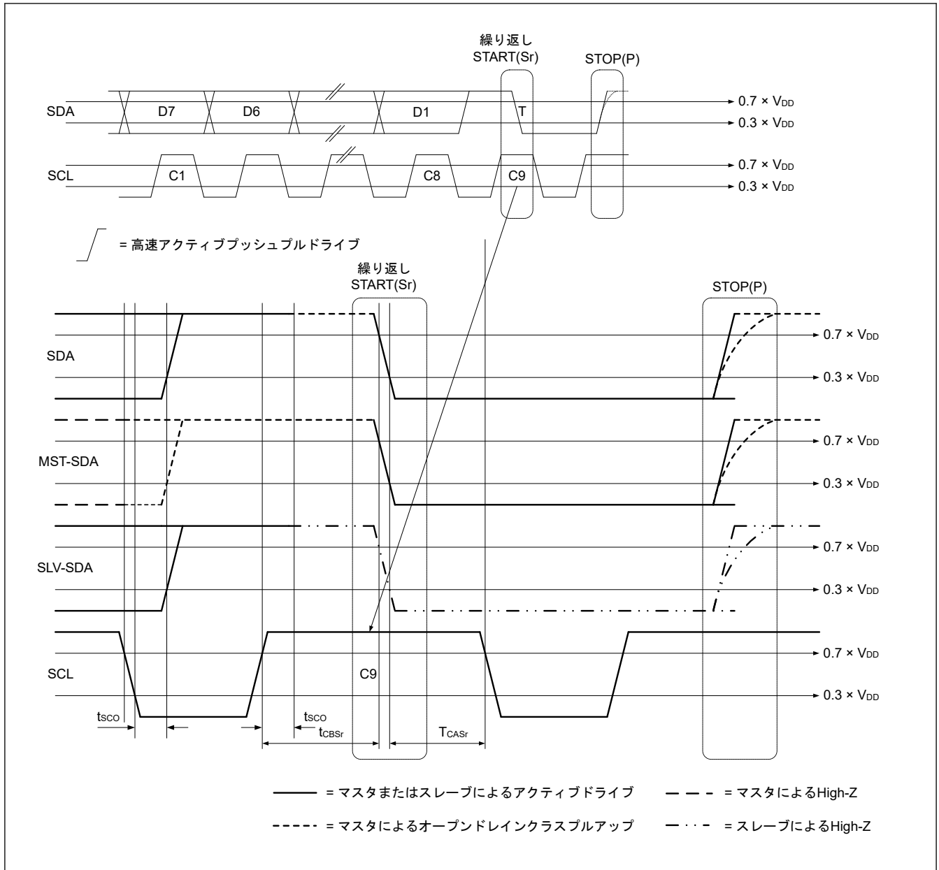
図 44.50 繰り返しのスタートコンディションおよびストップコンディションでのマスタ終了時のTビット読み出し
