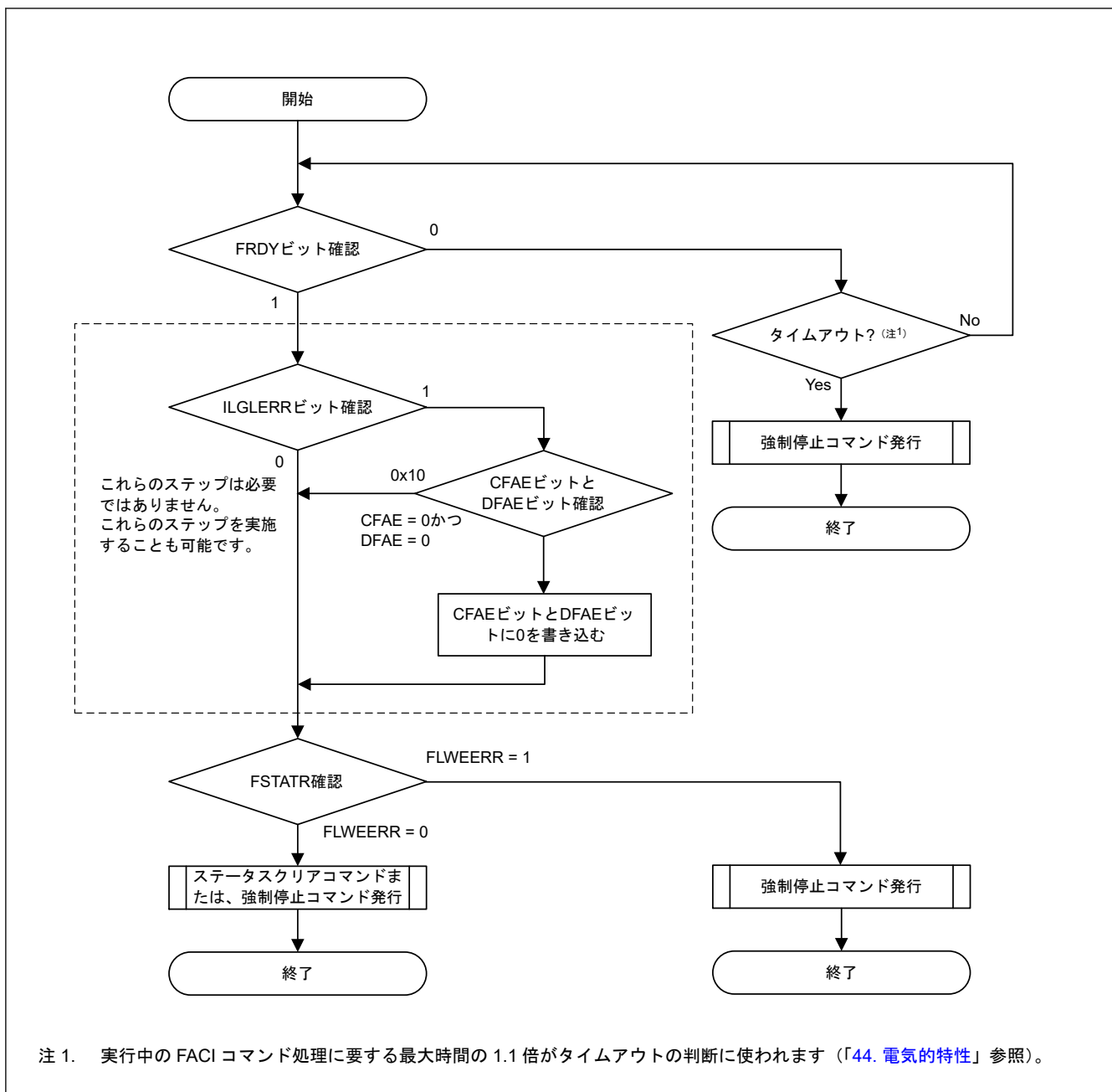
図 41.12 コマンドロック状態からの復帰フロー
