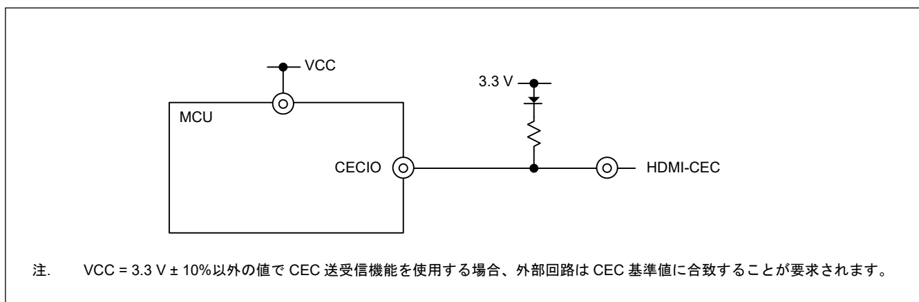
図 31.2 外部回路への I/O 端子の接続例 (VCC = 3.3 V ± 10%の場合)
