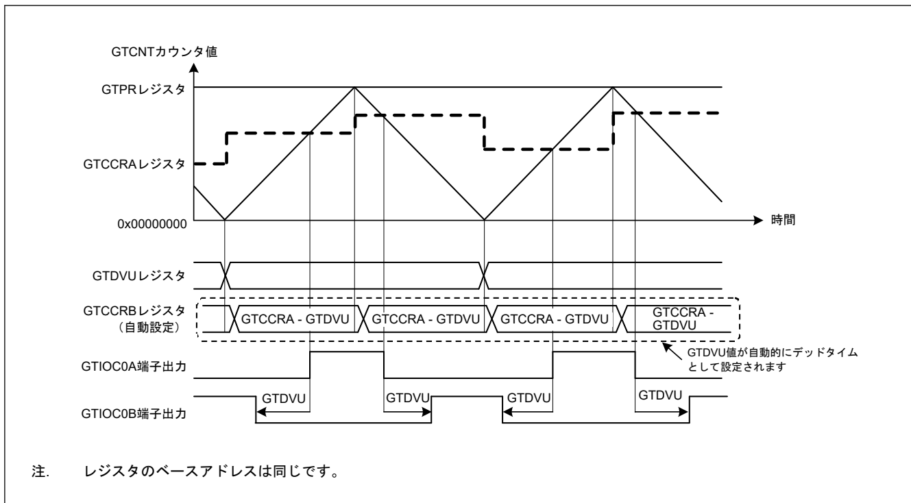
図 20.30 デッドタイム付きコンペアマッチ値の自動設定機能の動作例 (三角波 PWM モード 2 または 3、GTDVU/GTDVD レジスタはバッファ動作、アクティブ High の場合)
