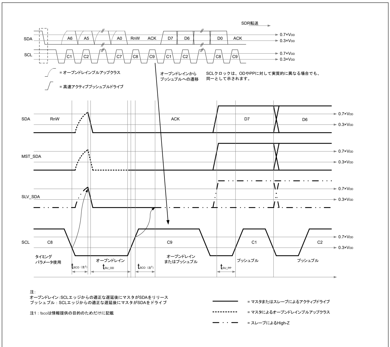
図 44.44 I3C データ転送 - スレーブによる ACK
