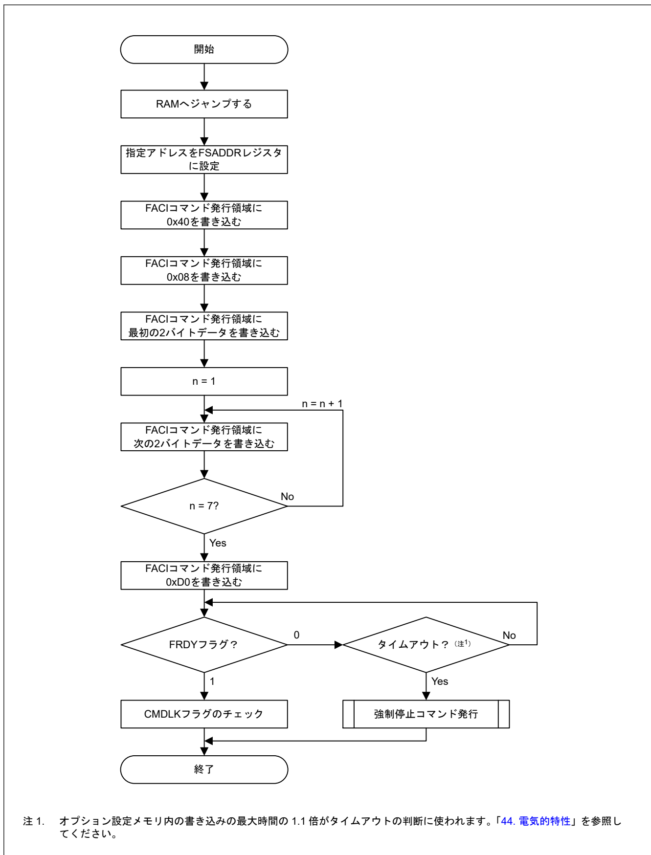
図 41.24 コンフィグレーション設定コマンドの使用フロー
