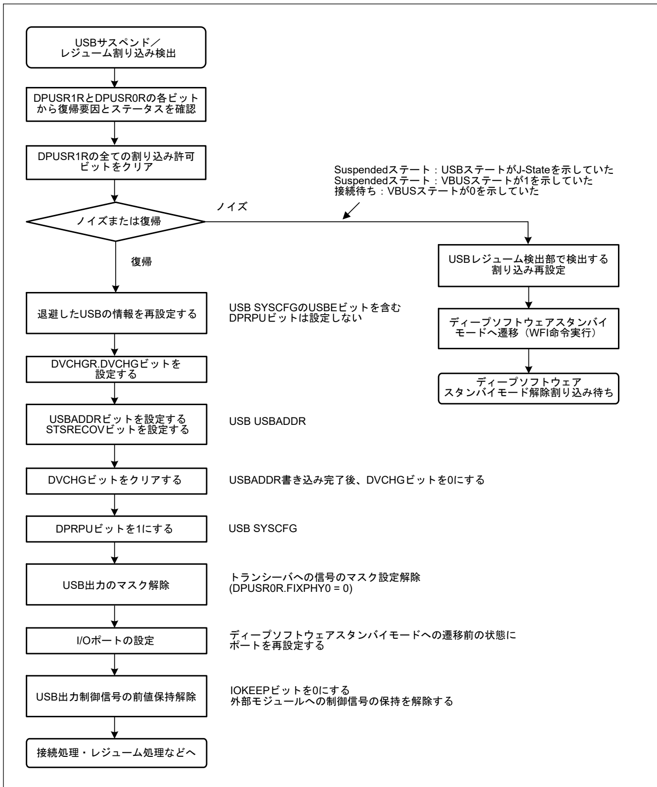
図 25.6 ディープソフトウェアスタンバイモード解除時の USBFS 設定フロー
