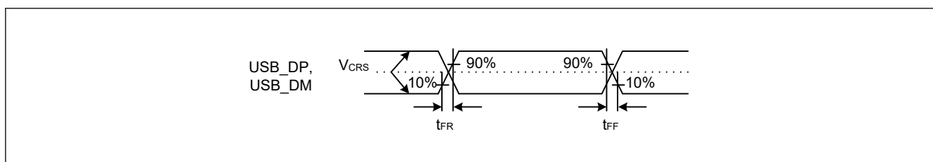
図 44.58 フルスピードモードにおける USB_DP、USB_DM の出カタイミング
