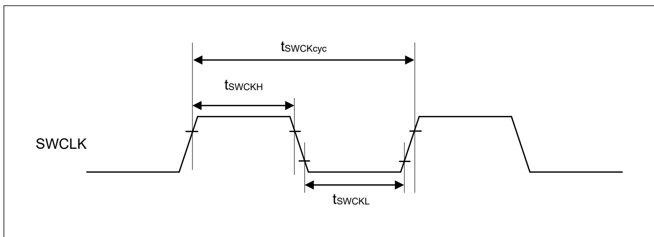
図 44.67 SWD SWCLK タイミング
