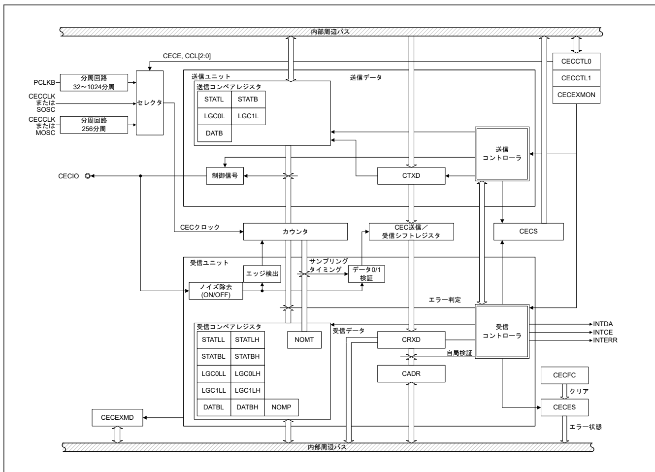
図 31.1 CEC のブロック図
