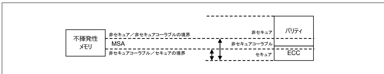
図 39.4 SRAM メモリ用 TrustZone フィルタ
