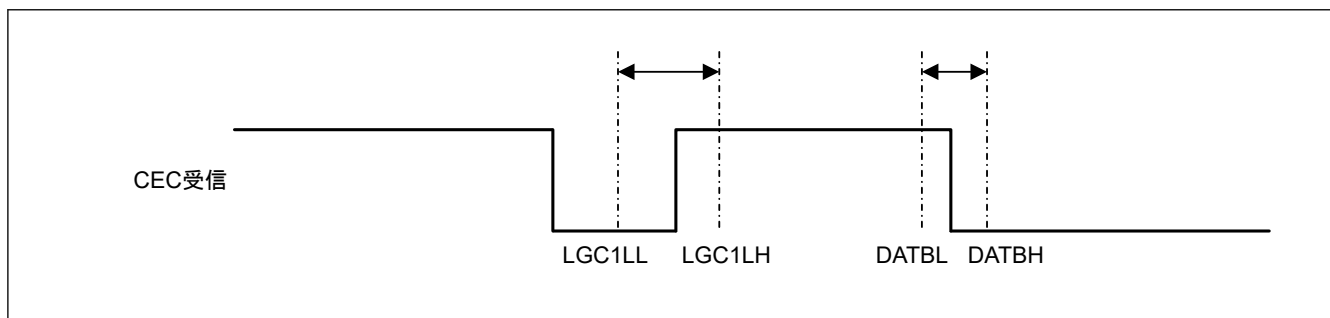
図 31.14 データビット (ロジカル 1) の受信タイミング
