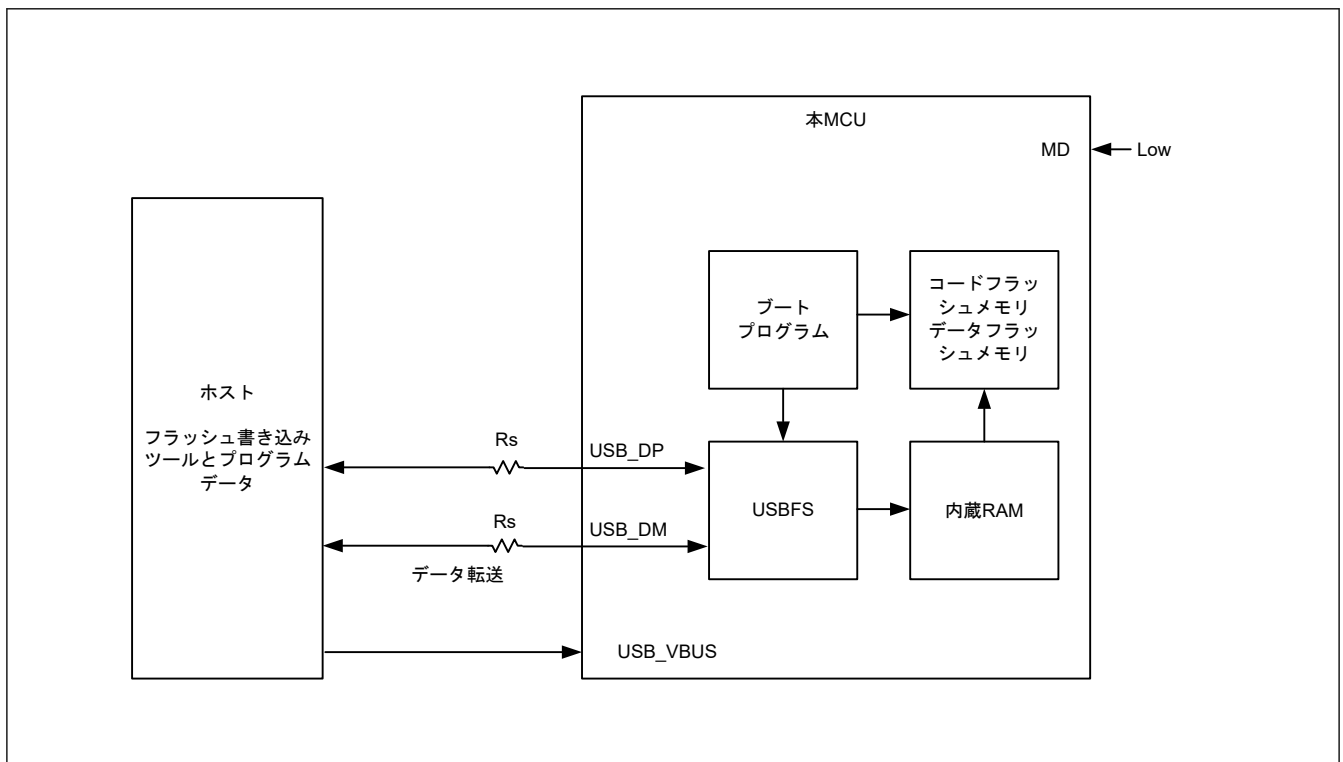
図 41.38 ブートモード (USB インタフェース) のシステム構成図
