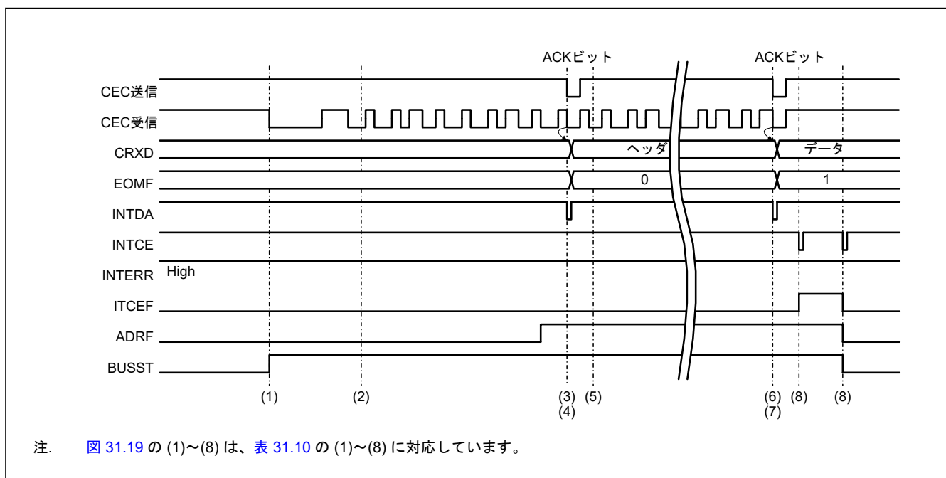
図 31.19 受信基本タイミング (1) (ダイレクトアドレス受信、CECCTL1.CESEL[1:0] = 00b のとき)
