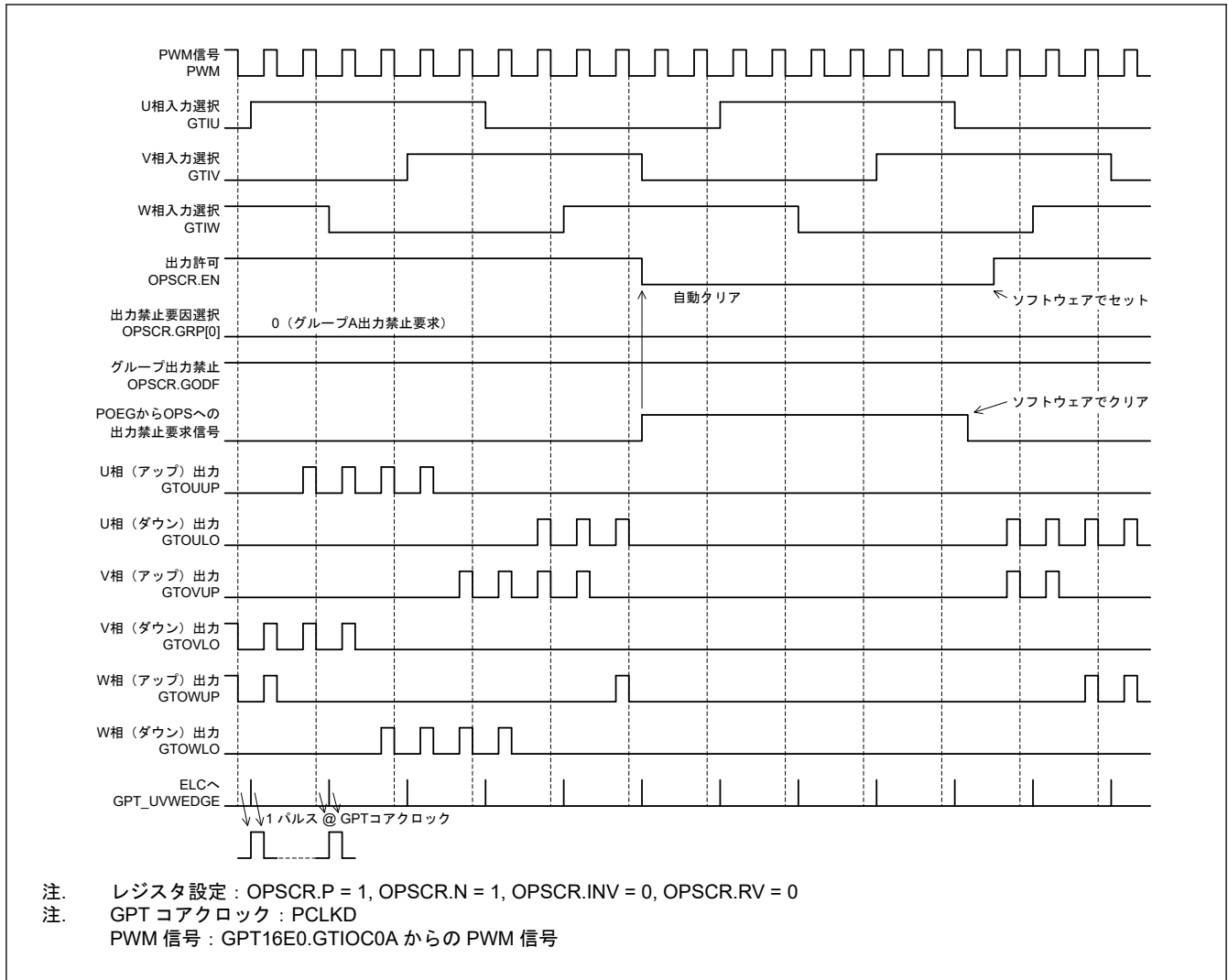
図 20.66 グループ出力禁止制御動作例
