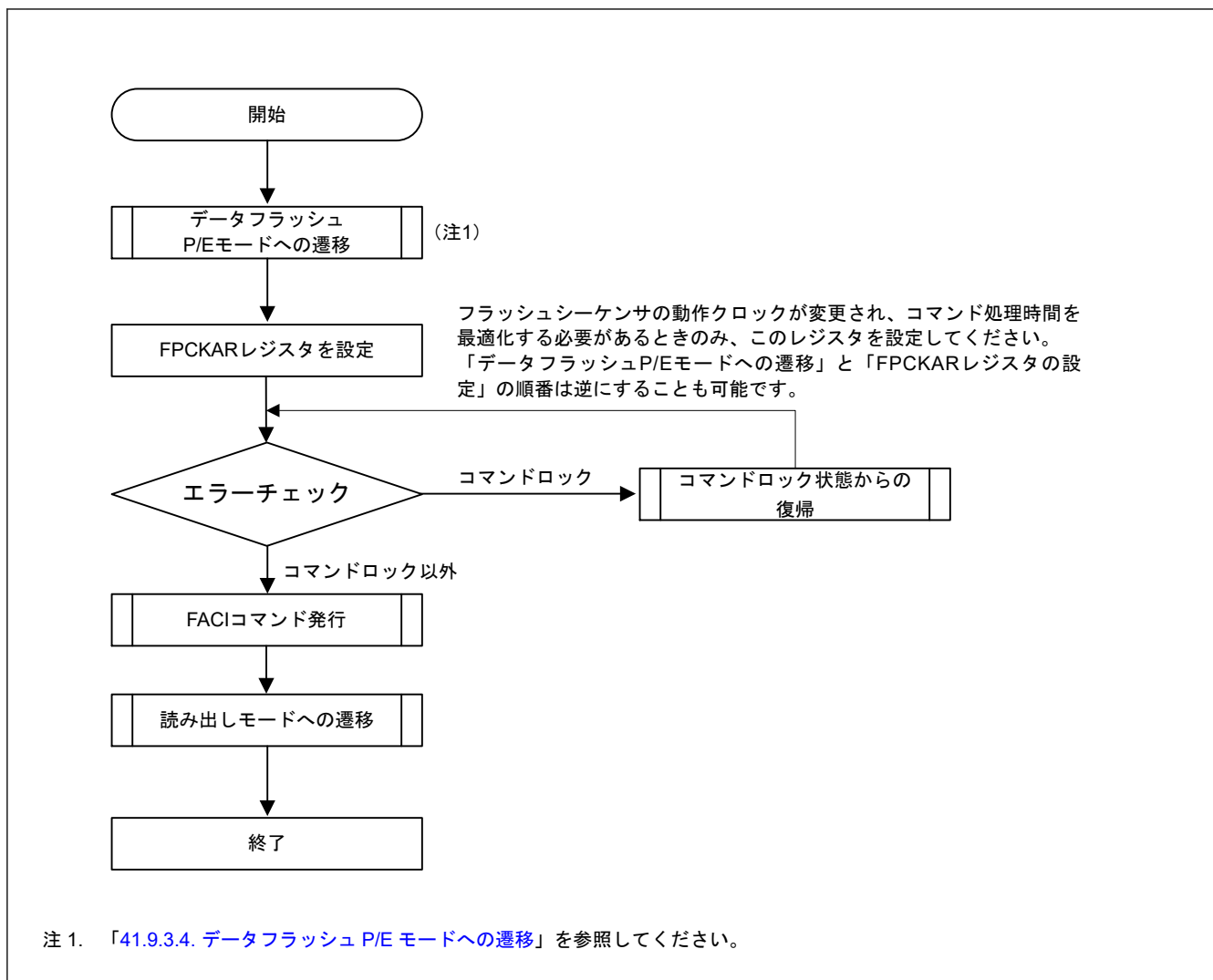
図 41.8 データフラッシュ P/E モードでのコマンド使用概要
