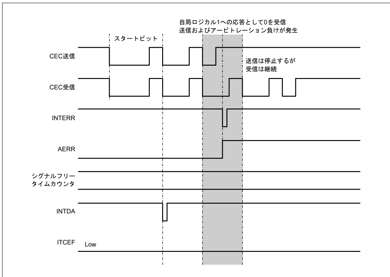
図 31.38 アービトレーションタイミング
