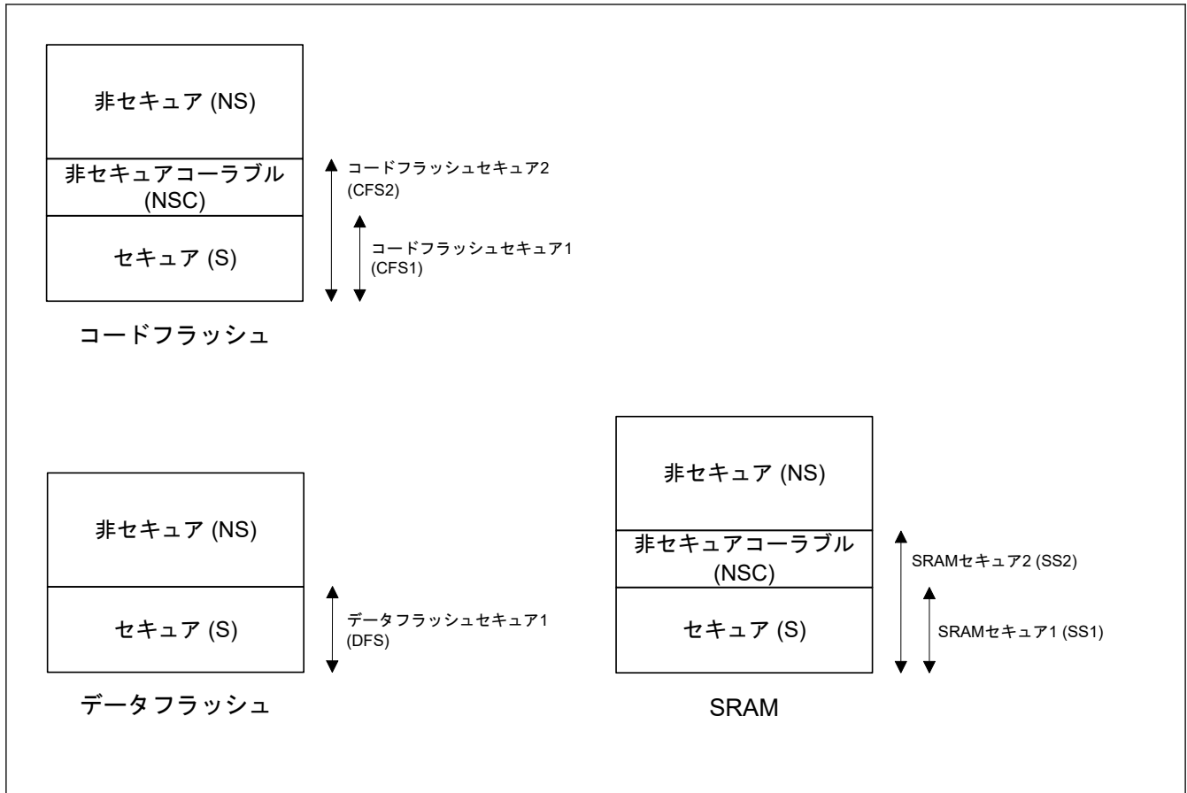
図 43.1 メモリマッピング
