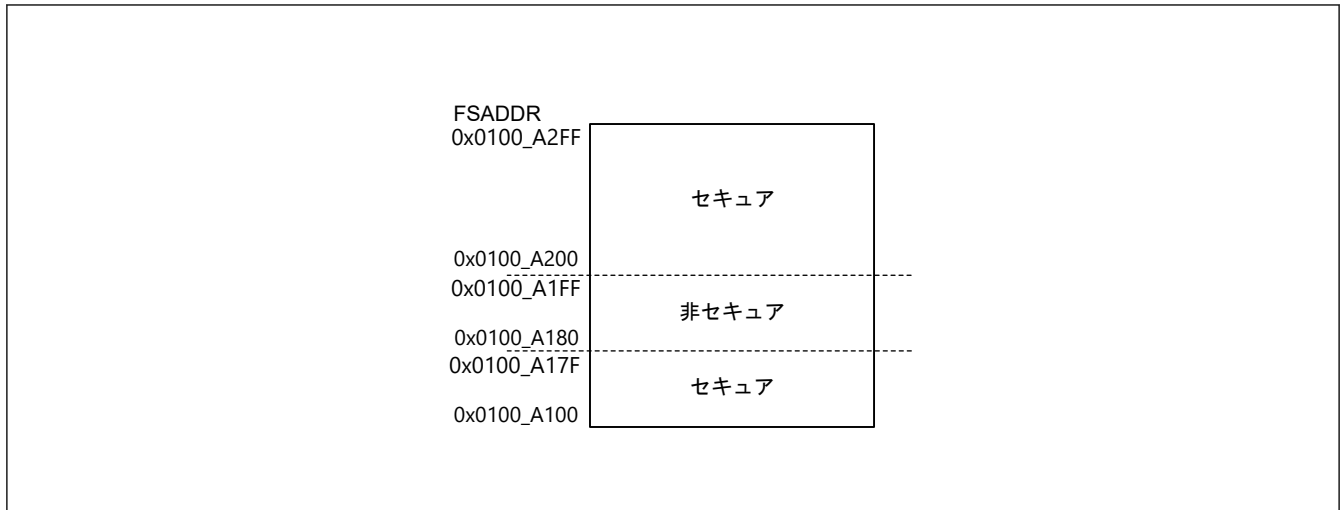
図 41.32 オプション設定メモリのセキュア/非セキュア領域
