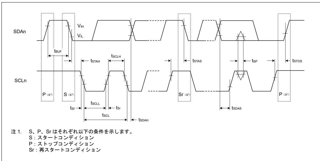
図 44.41 I2C バスインタフェース入出力タイミング
