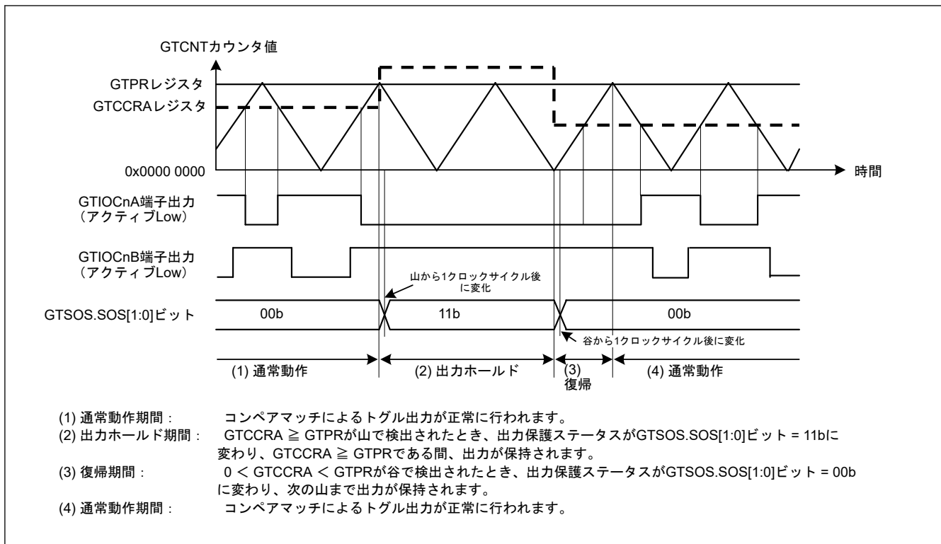
図 20.90 山でのバッファ転送中に GTCCRA \geq GTPR となったときの出力保護機能の動作例（谷でのバッファ転送中に 0 < GTCCRA < GTPR に復帰、アクティブレベルは Low）（ n = 0, 1, 4, 5 ）
