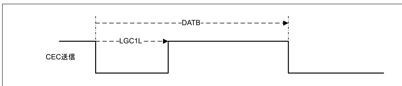
図 31.11 データビット (ロジカル 1) の出力波形
