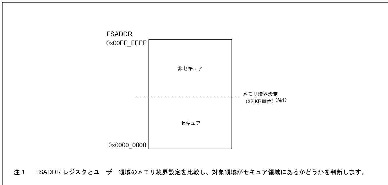
図 41.30 ユーザー領域のセキュア/非セキュア領域
