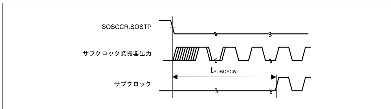
図 44.11 サブクロック発振開始タイミング
