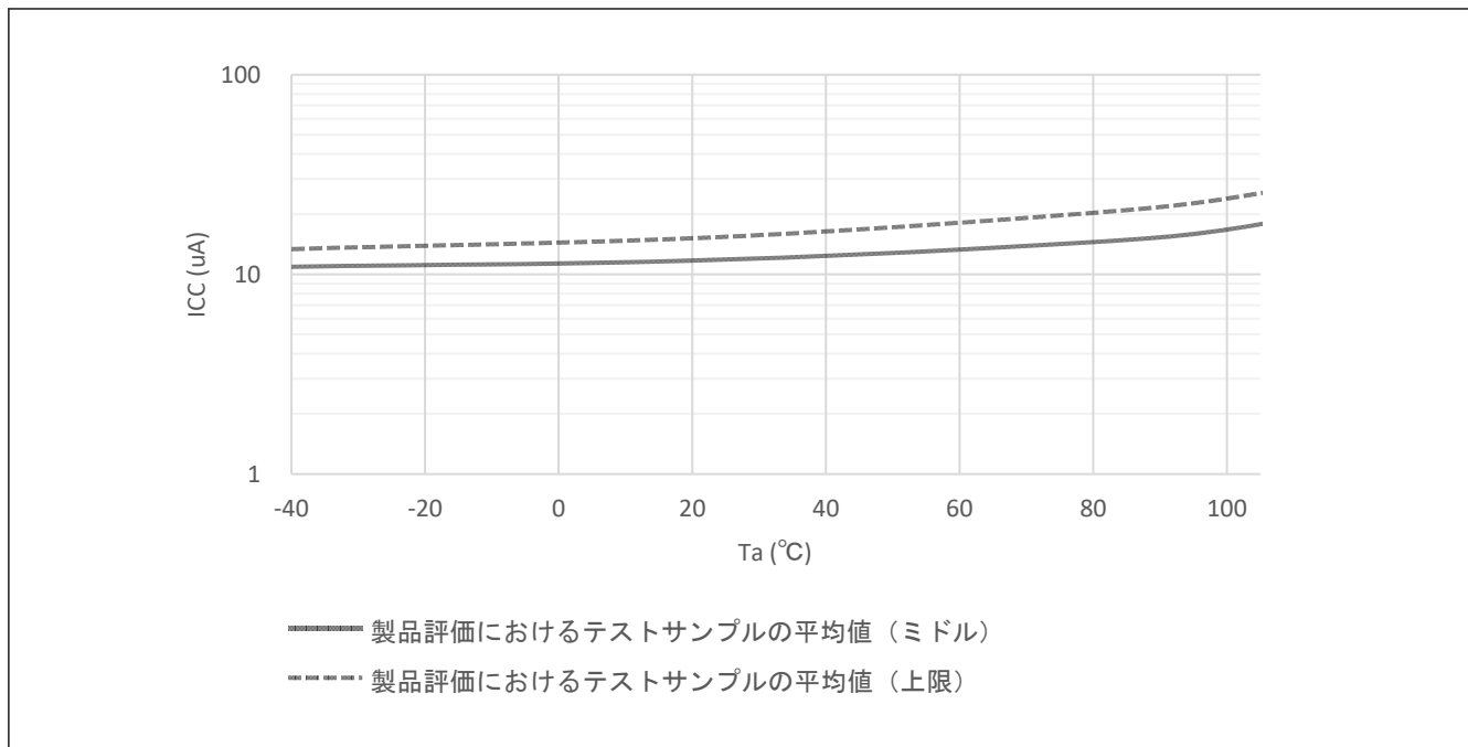
図 44.4 ディープソフトウェアスタンバイモード時の温度依存性、SRAM および USB レジューム検出部への電源供給なし、パワーオンリセット回路、低消費電力機能無効 (参考データ)
