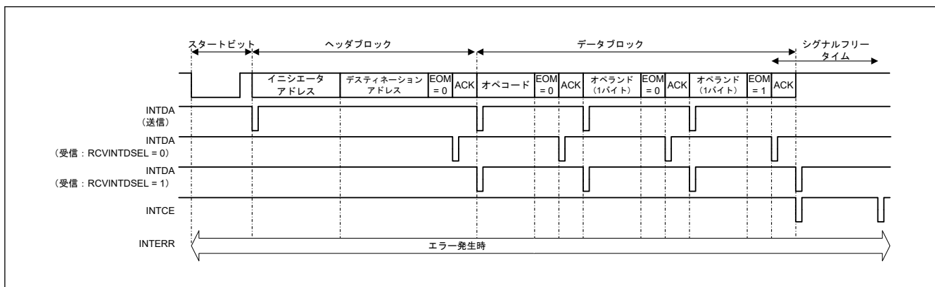
図 31.33 割り込みの発生タイミング
