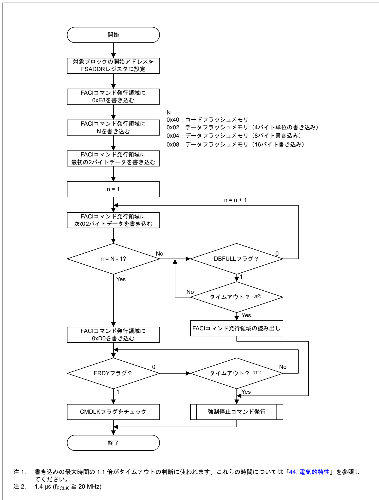
図 41.13 プログラムコマンドの使用フロー
