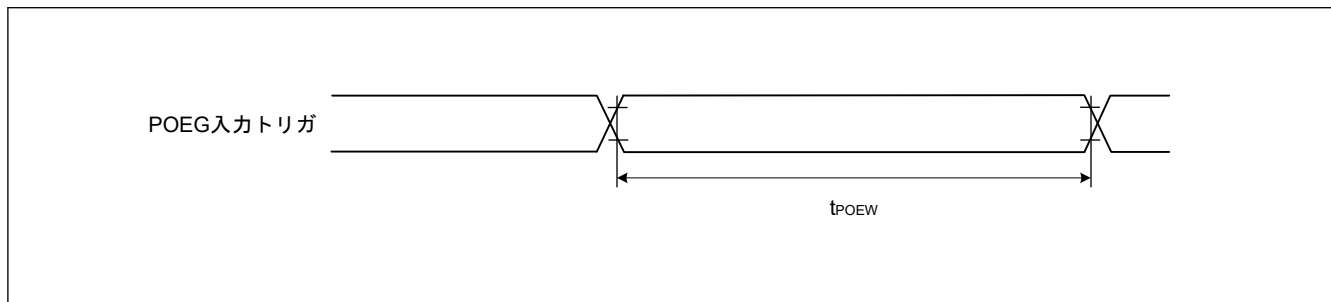
図 44.20 POEG 入力トリガタイミング
