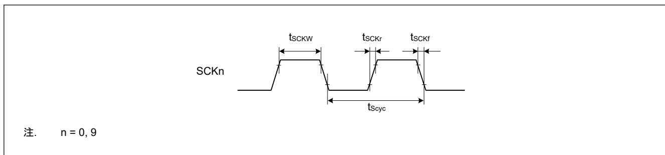
図 44.26 SCK クロック入出力タイミング
