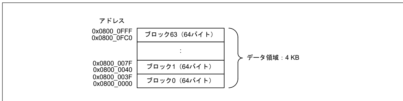
図 41.3 データフラッシュメモリのマップ
