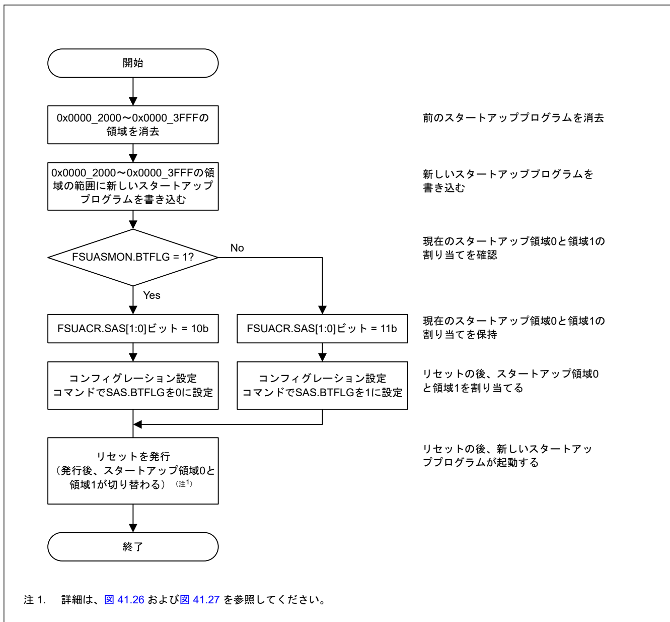
図 41.28 スタートアッププログラムプロテクションの概念
