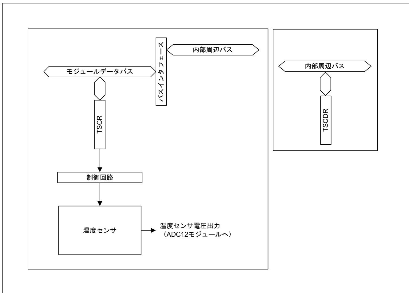
図 37.1 TSN のブロック図
