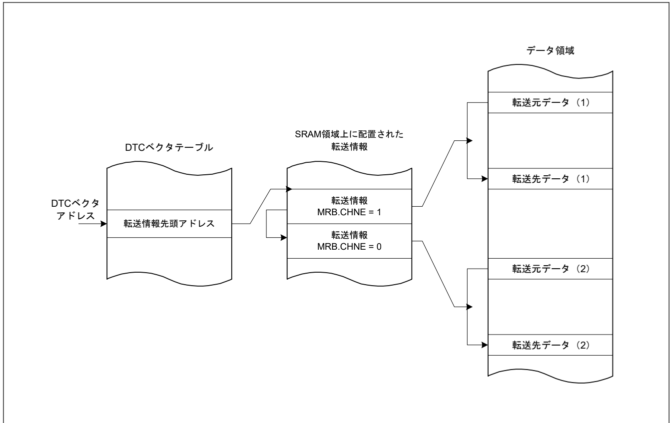
図 16.8 チェーン転送の動作
