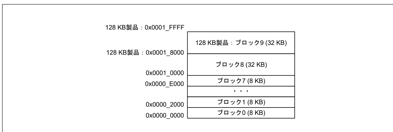
図 6.2 コードフラッシュのブロック構成
