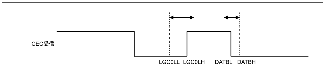
図 31.13 データビット (ロジカル 0) の受信タイミング
