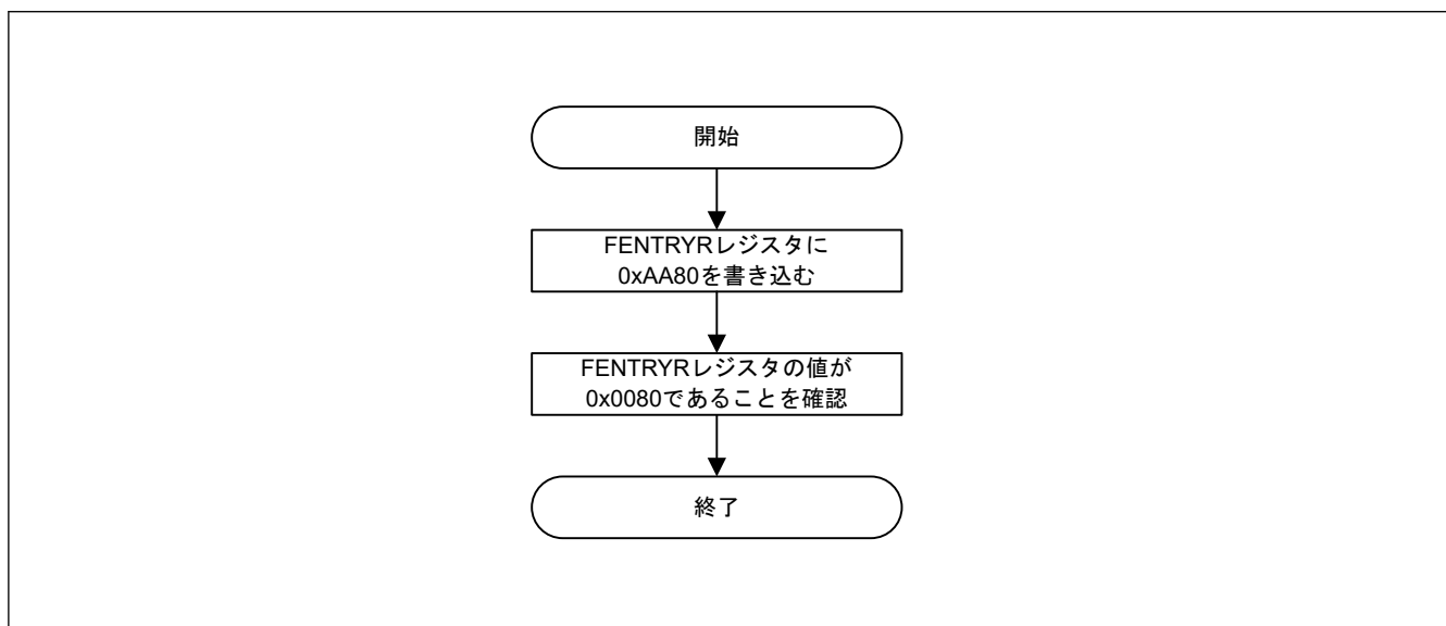
図 41.10 データフラッシュ P/E モードへの遷移手順
