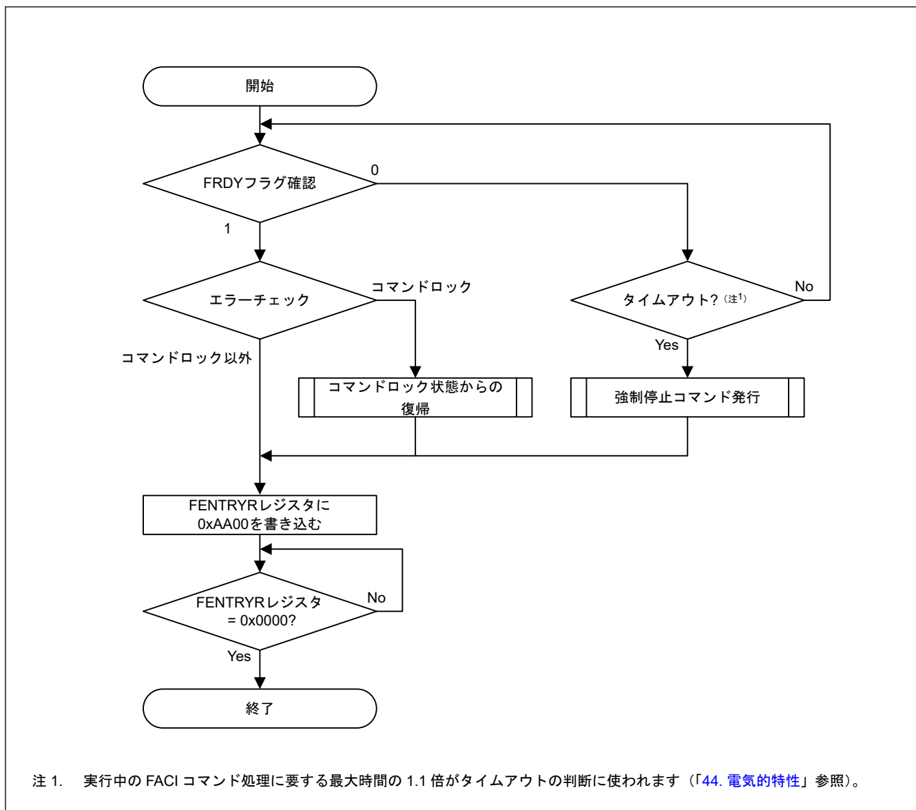
図 41.11 読み出しモードへの遷移手順
