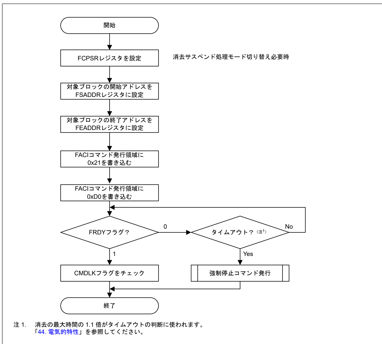
図 41.15 マルチブロックコマンドの使用フロー
