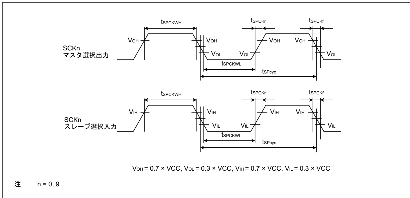
図 44.28 SCI 簡易 SPI モードクロックタイミング
