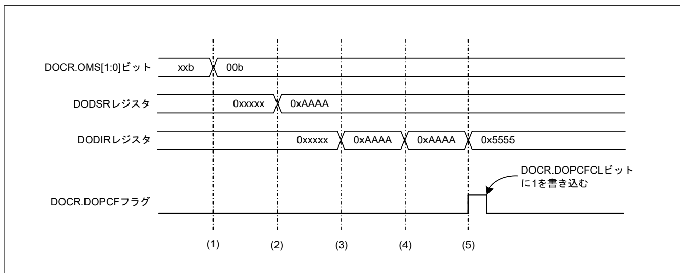
図 38.2 データ比較モードの動作例
