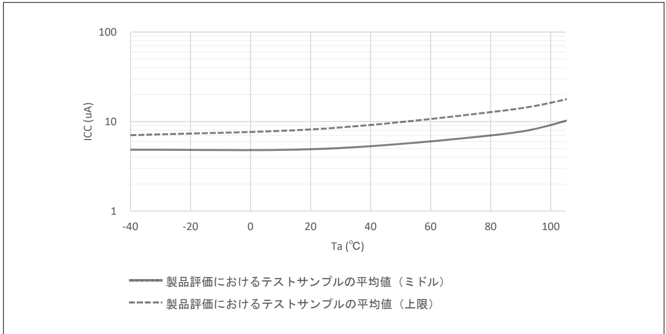
図 44.5 ディープソフトウェアスタンバイモード時の温度依存性、SRAM および USB レジューム検出部への電源供給なし、パワーオンリセット回路、低消費電力機能有効 (参考データ)
