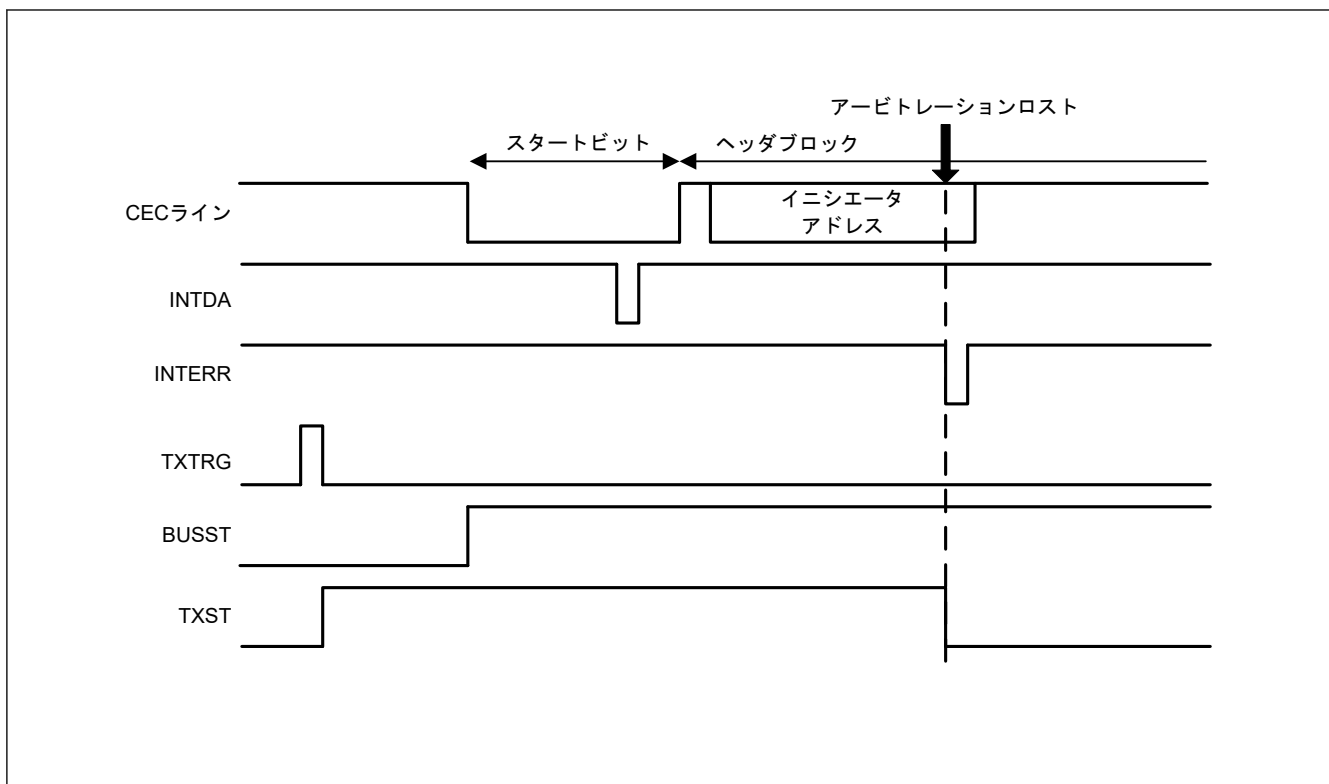
図 31.27 アービトレーションロスト発生時の送信ステータスフラグのタイミング
