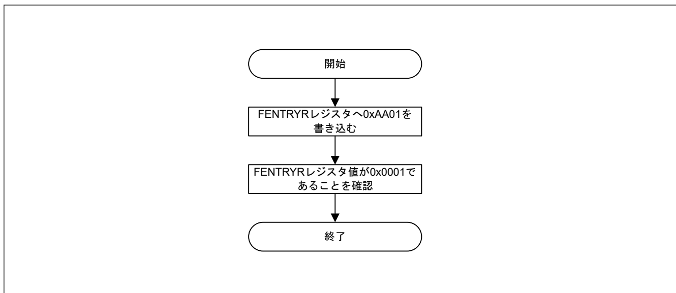
図 41.9 コードフラッシュ P/E モードへの遷移手順
