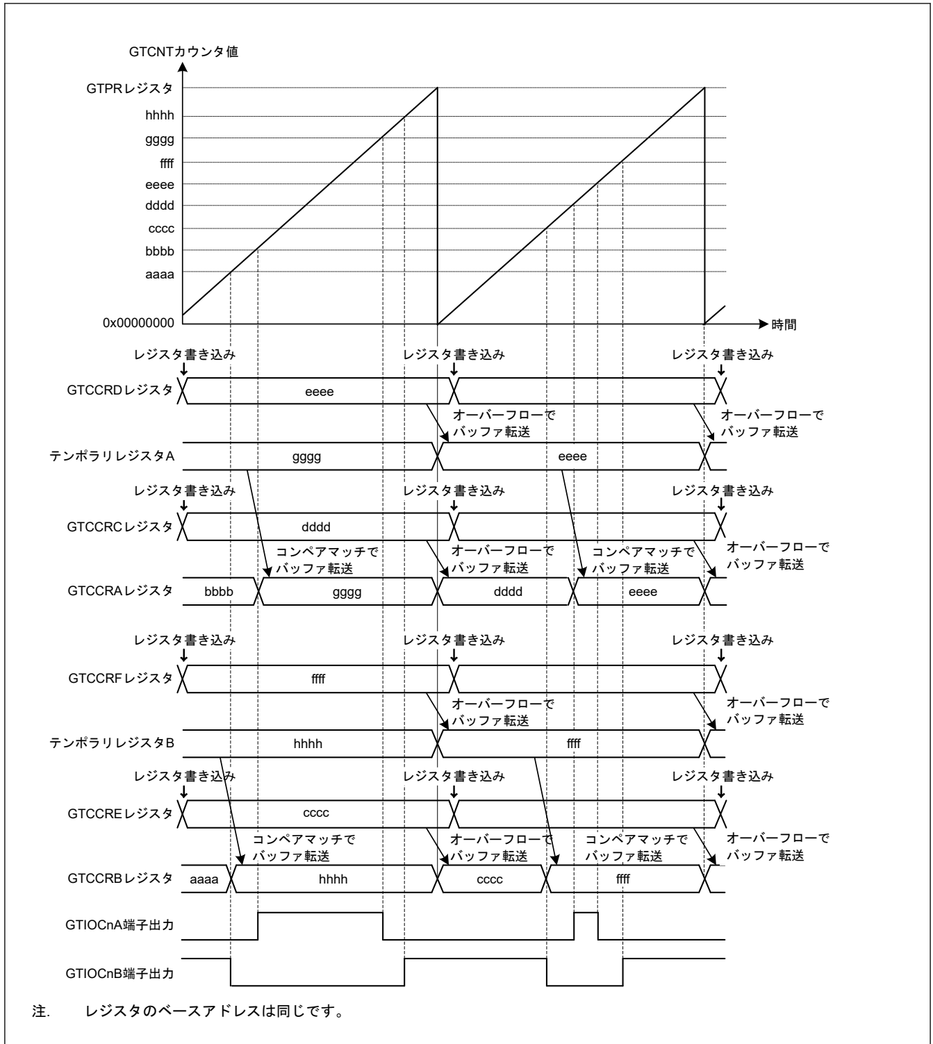
図 20.23 のこぎり波ワンショットパルスモードの動作例 (アップカウント、カウントスタート時に GTIOcNA 端子 = Low 出力 / GTIOcNB 端子 = High 出力、GTCCRA/GTCRCB レジスタのコンペアマッチ時に トグル出力、周期の終わりで出力保持の場合)
