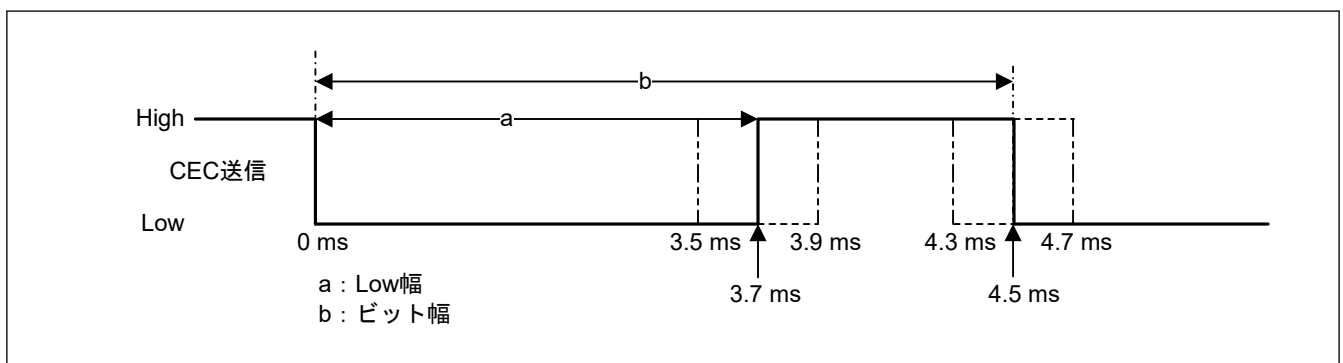
図 31.6 スタートビットのフォーマット例
