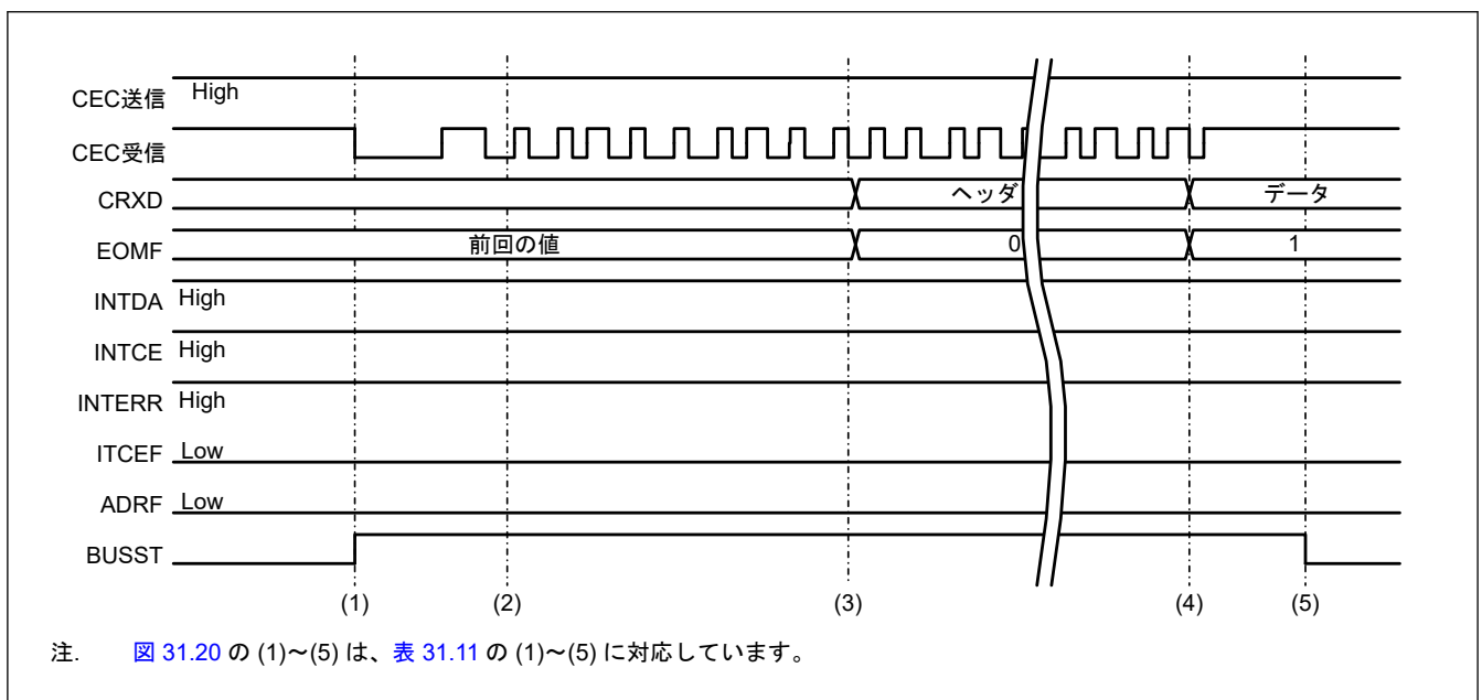
図 31.20 受信基本タイミング (2) (CECCTL0.CECRXEN = 1、ダイレクトアドレス、アドレス不一致、CECCTL1.CINTMK = 0)
