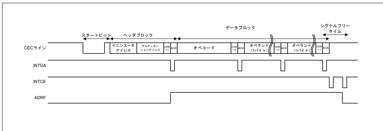
図 31.22 ADRF ビットの動作タイミング
