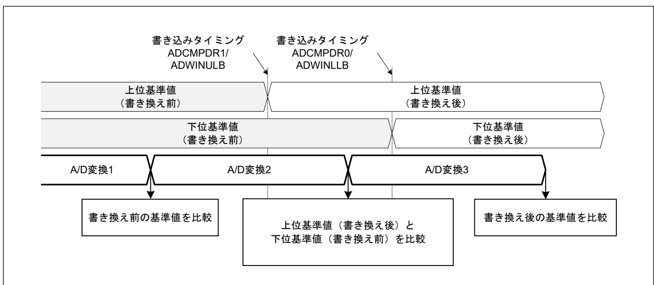
図 35.4 書き換え前後の上側基準値と下側基準値の比較
