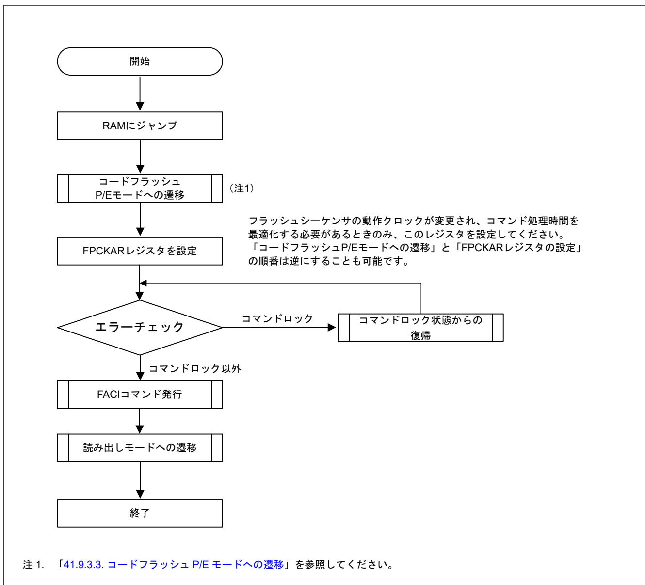
図 41.7 コードフラッシュ P/E モードでのコマンド使用概要
