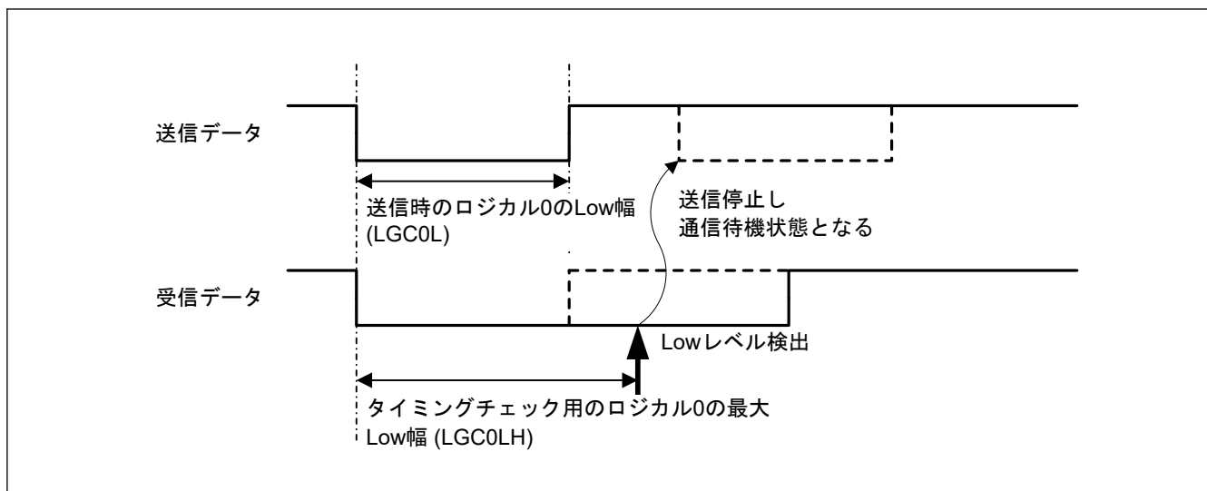
図 31.18 エラー処理パルス受信動作
