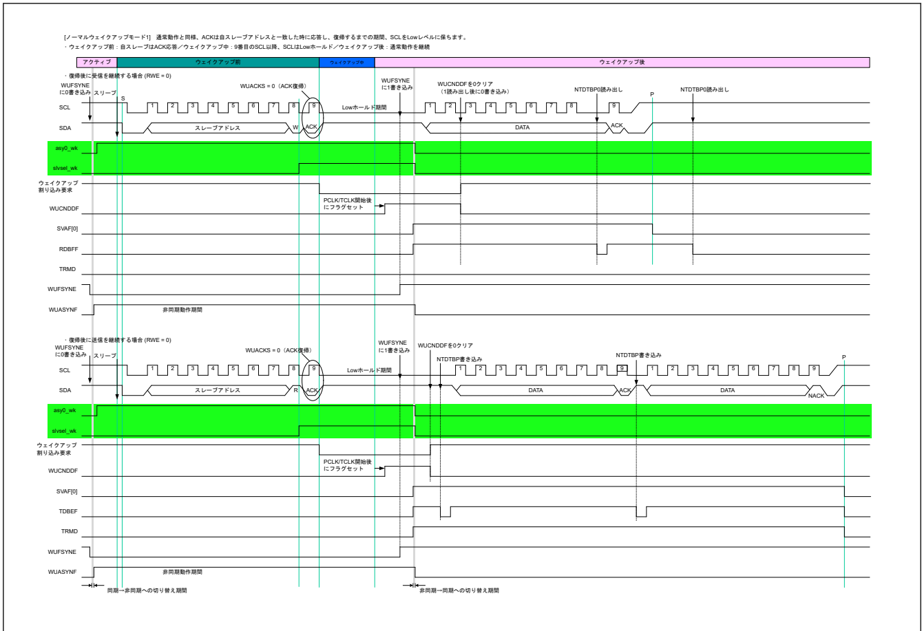
図 27.101 ノーマル WU モード 1 のタイミング
