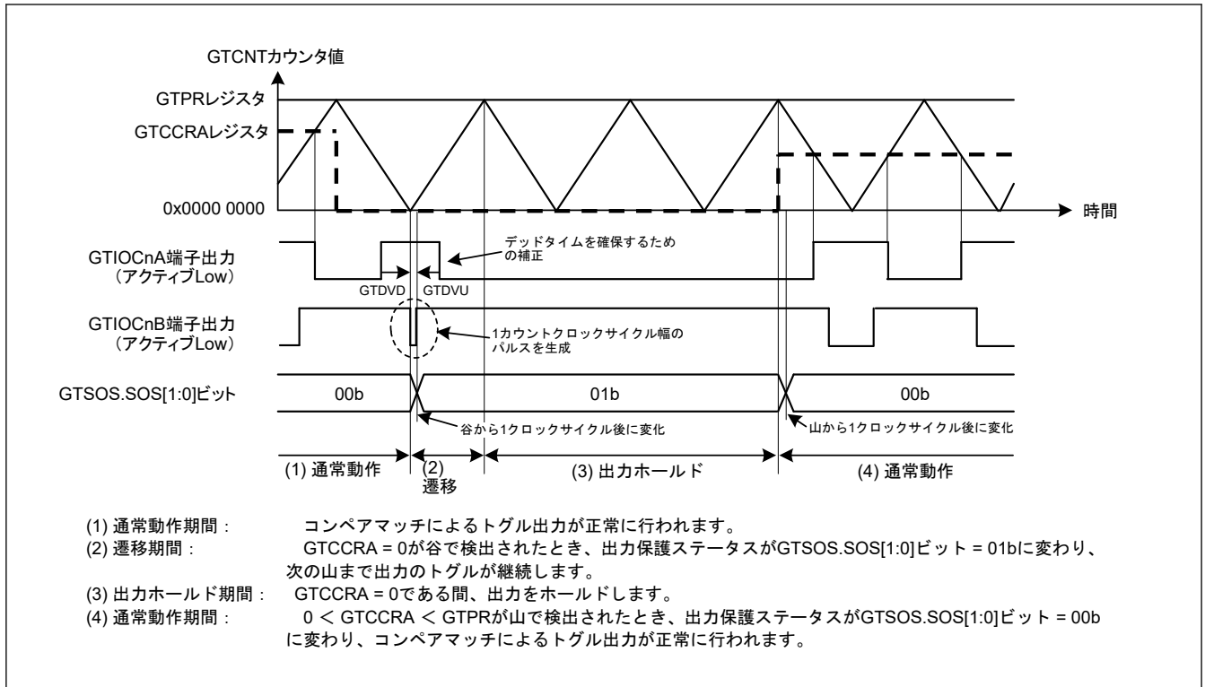
図 20.86 山でのバッファ転送中に GTCCRA が 0 になったときの出力保護機能の動作例 (山でのバッファ転送中に 0 < GTCCRA < GTPR に復帰、アクティブレベルは Low) ( n = 0, 1, 4, 5 )
