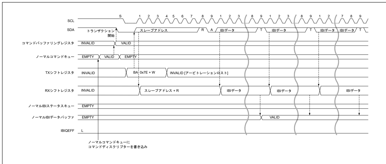
図 27.24 I3C マスタ IBI 転送タイミング (1/2)
