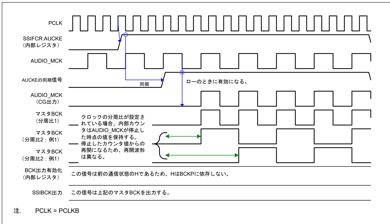
図 32.27 通信停止からマスタモード通信開始までの動作のタイミング図
