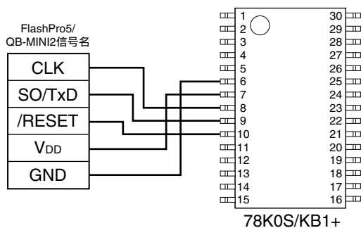
図19 - 3 FlashPro5/QB-MINI2との配線図 (30ピン製品の場合)
