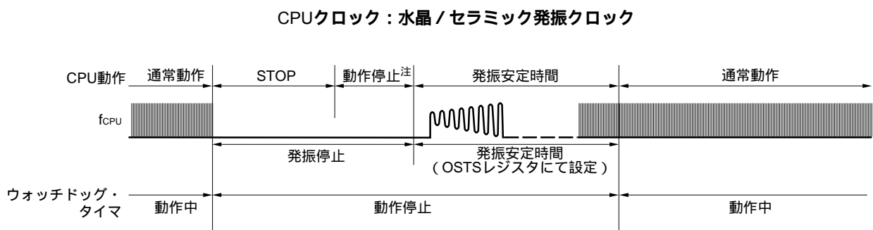
図9 - 6 STOPモード時の動作（WDT動作クロック：システム・クロック）
