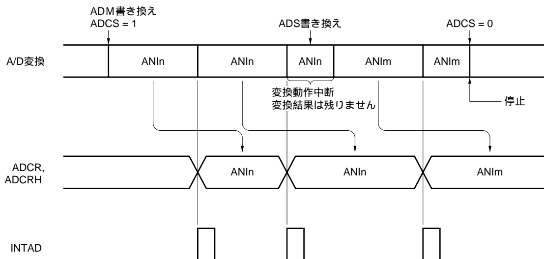
図10 - 12 A/D変換動作
