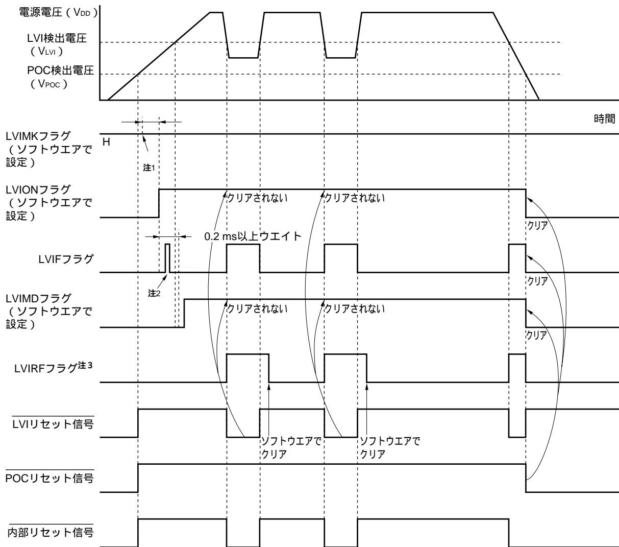
図17-4 低電圧検出回路の内部リセット信号発生タイミング
