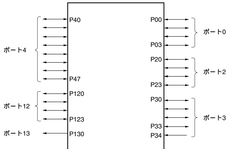
図4 - 1 ポートの機能
