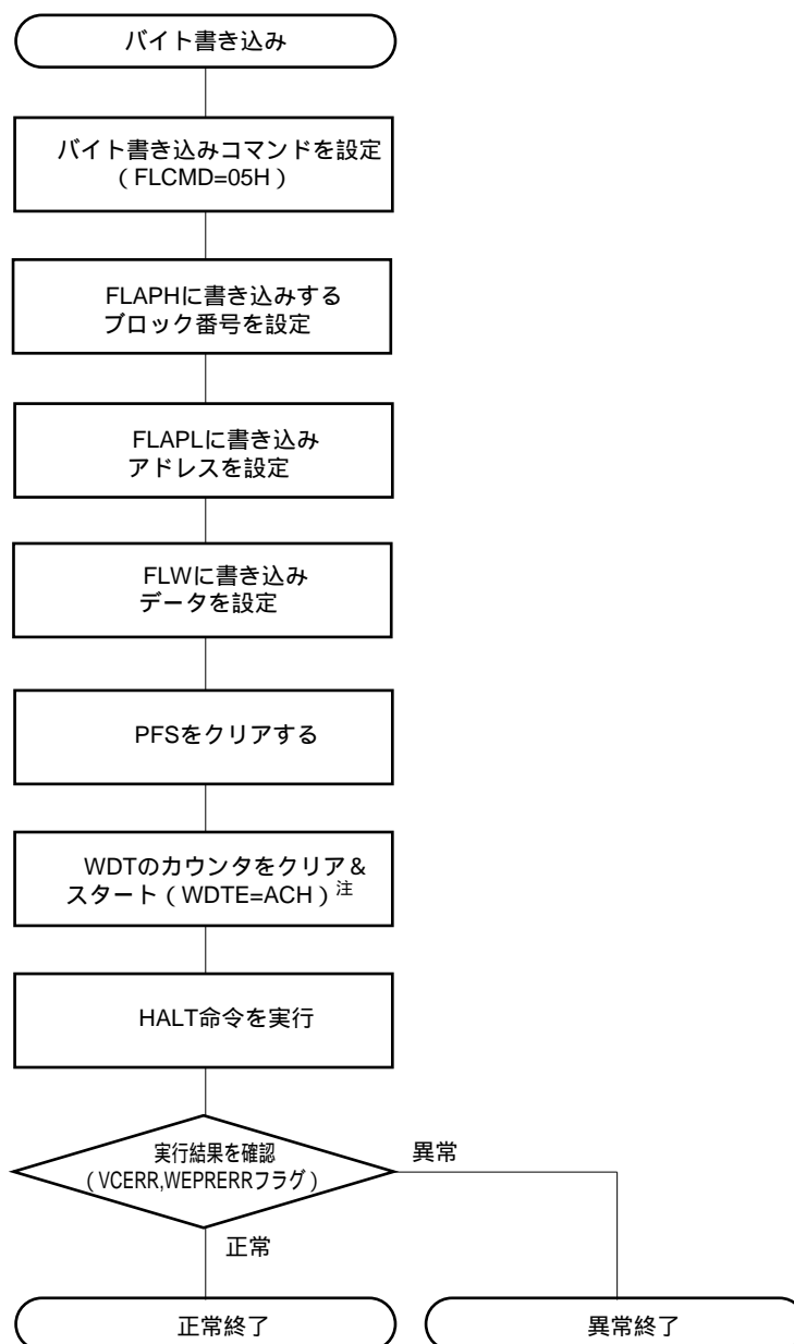
図19 - 22 セルフ・プログラミング・モードのバイト書き込み動作例
