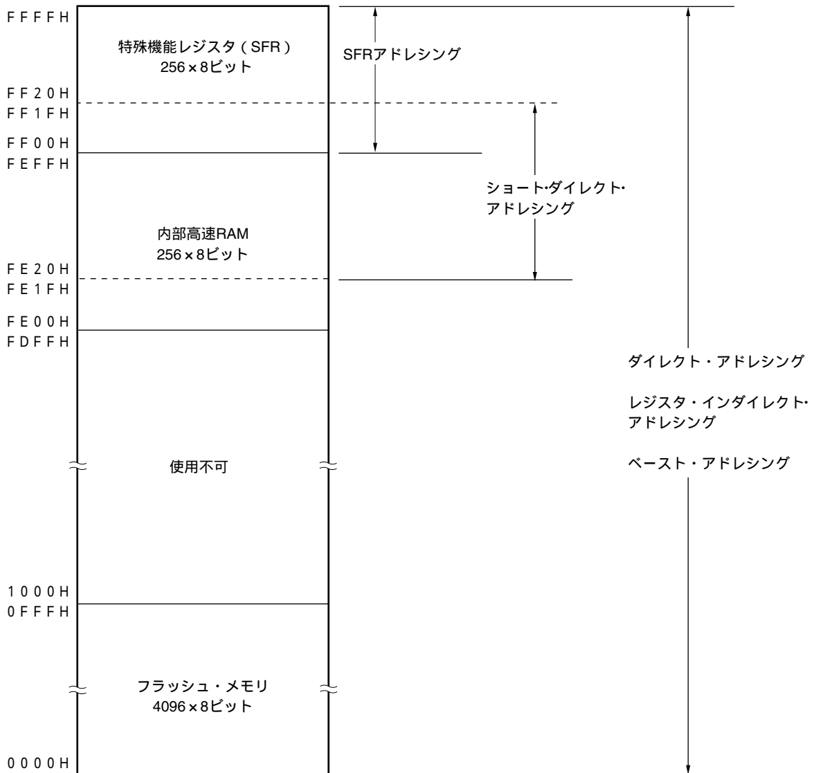
図3 - 3 データ・メモリのアドレッシング (μPD78F9232)
