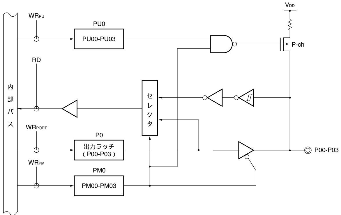
図4 - 2 P00-P03のブロック図
