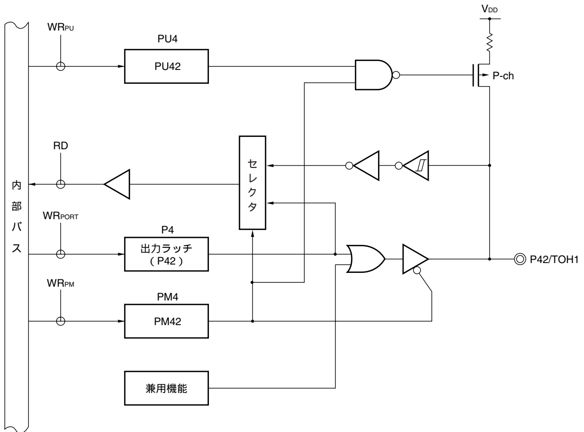
図4 - 10 P42のブロック図
