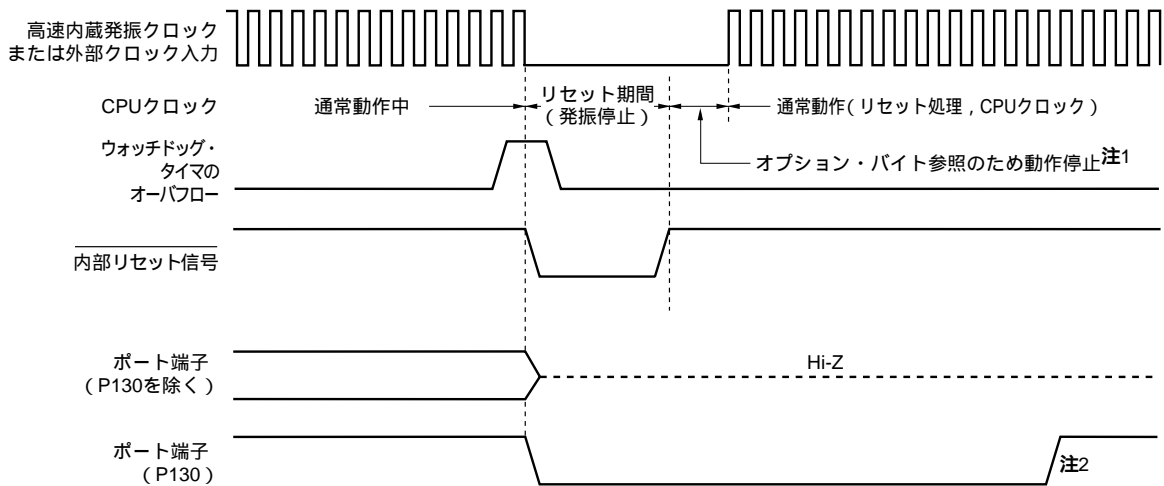
図15 - 3 ウォッチドッグ・タイマのオーバーフローによるリセット・タイミング
