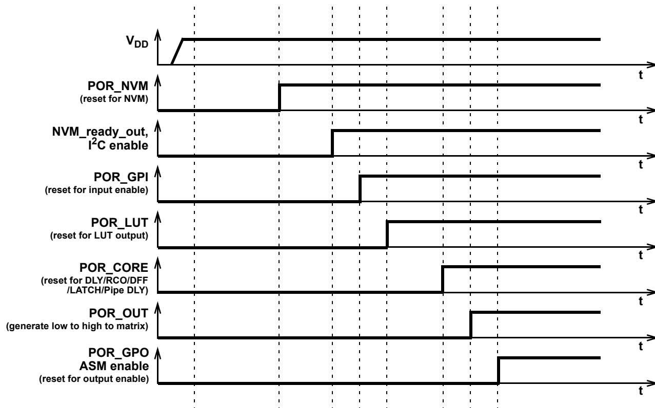
Figure 71: POR Sequence
