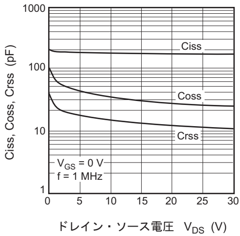
容量対ドレイン・ソース電圧特性
