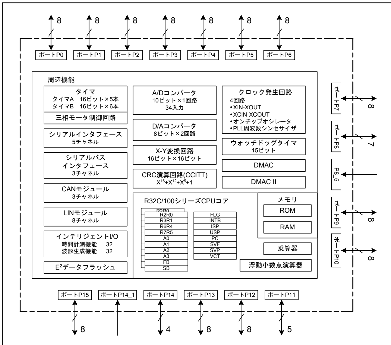
図 1.2 R32C/152グループのブロック図
