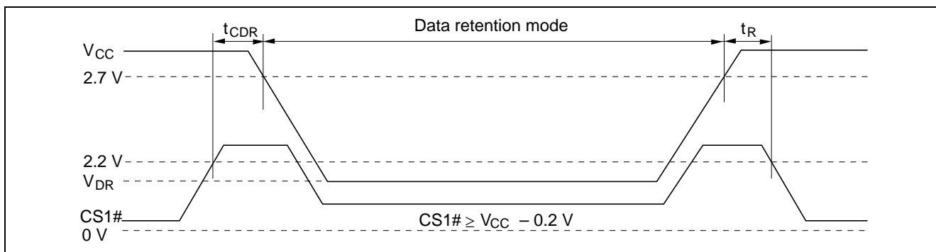
低電源電圧時データ保持タイミング波形(1) (CS1# Controlled)
