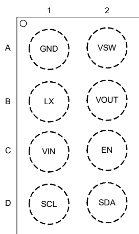
8 Bump WLCSP
