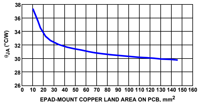
図 12. \theta_{JA} vs プリント基板上で EPAD が接する銅エリアの面積
