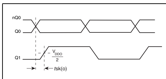
Output Skew
