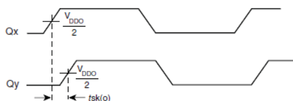
OUTPUT SKEW
