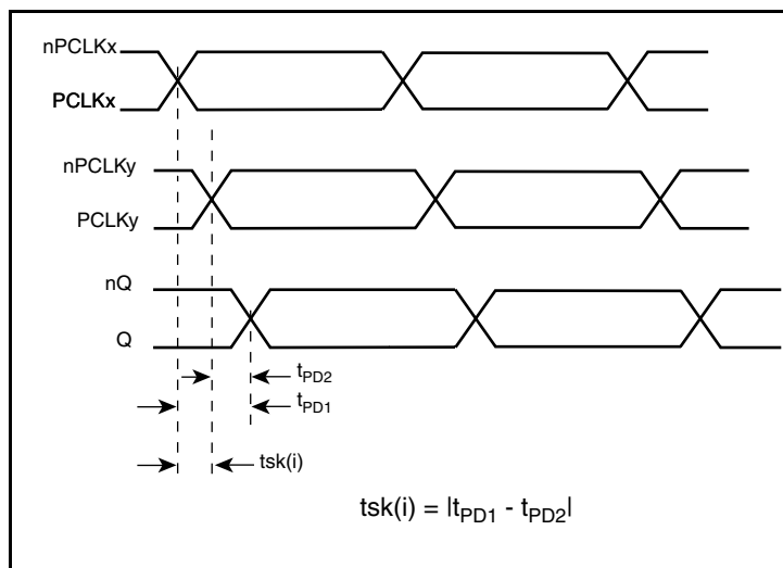
Input Skew
