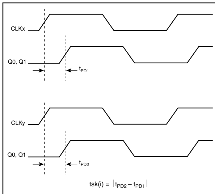
Input Skew
