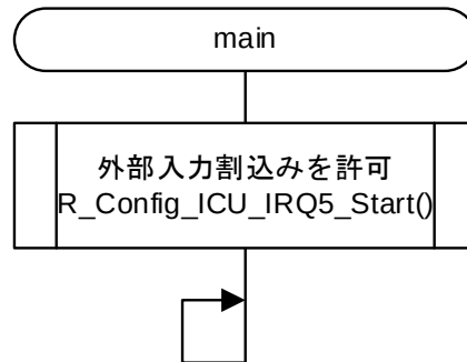
図 3.1 メイン処理
