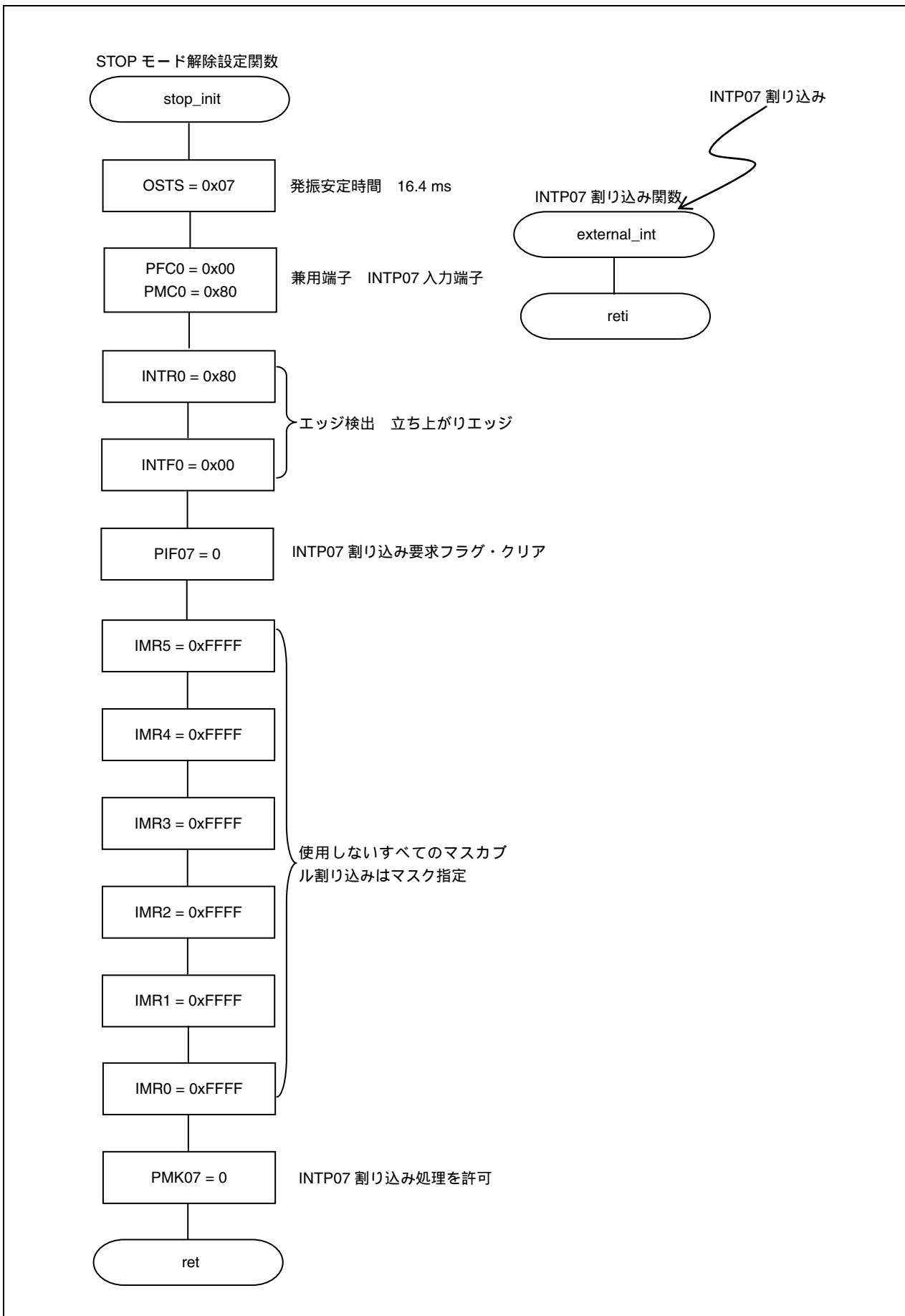
図3 - 1 STOPモード (2/3)
