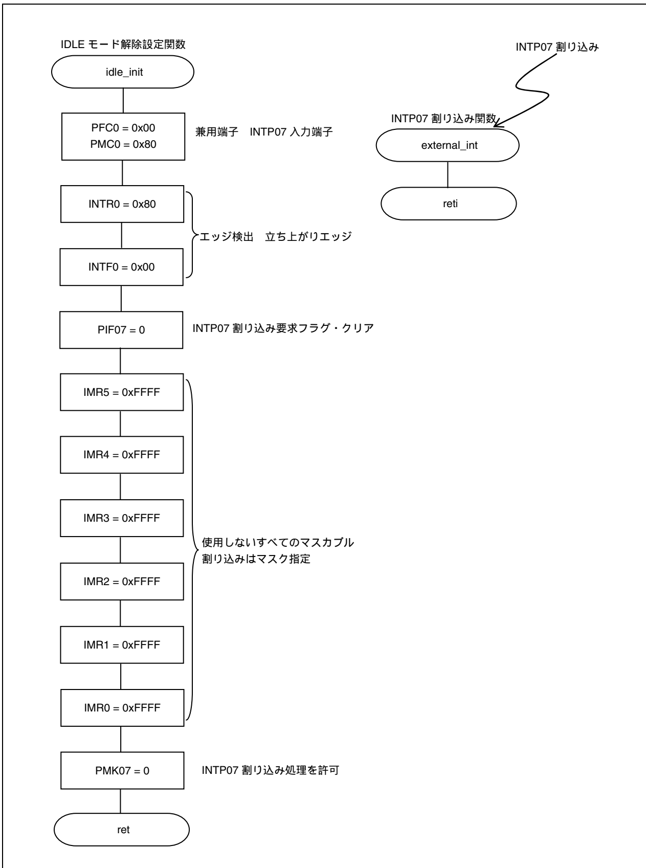
図2-1 IDLEモード (2/3)
