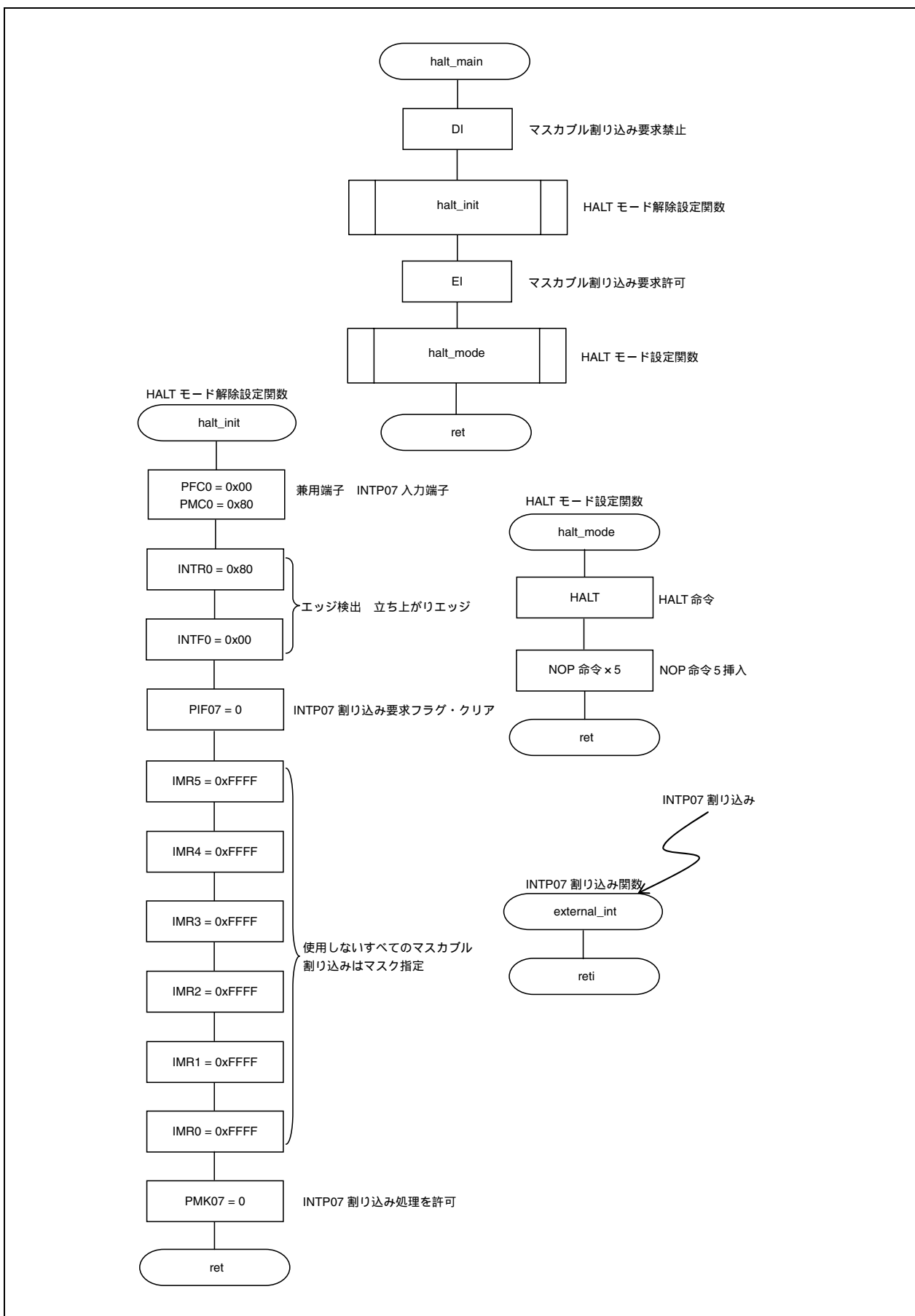
図1 - 1 HALTモード
