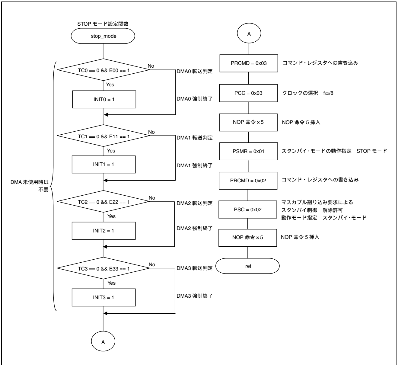
図3 - 1 STOPモード (3/3)
