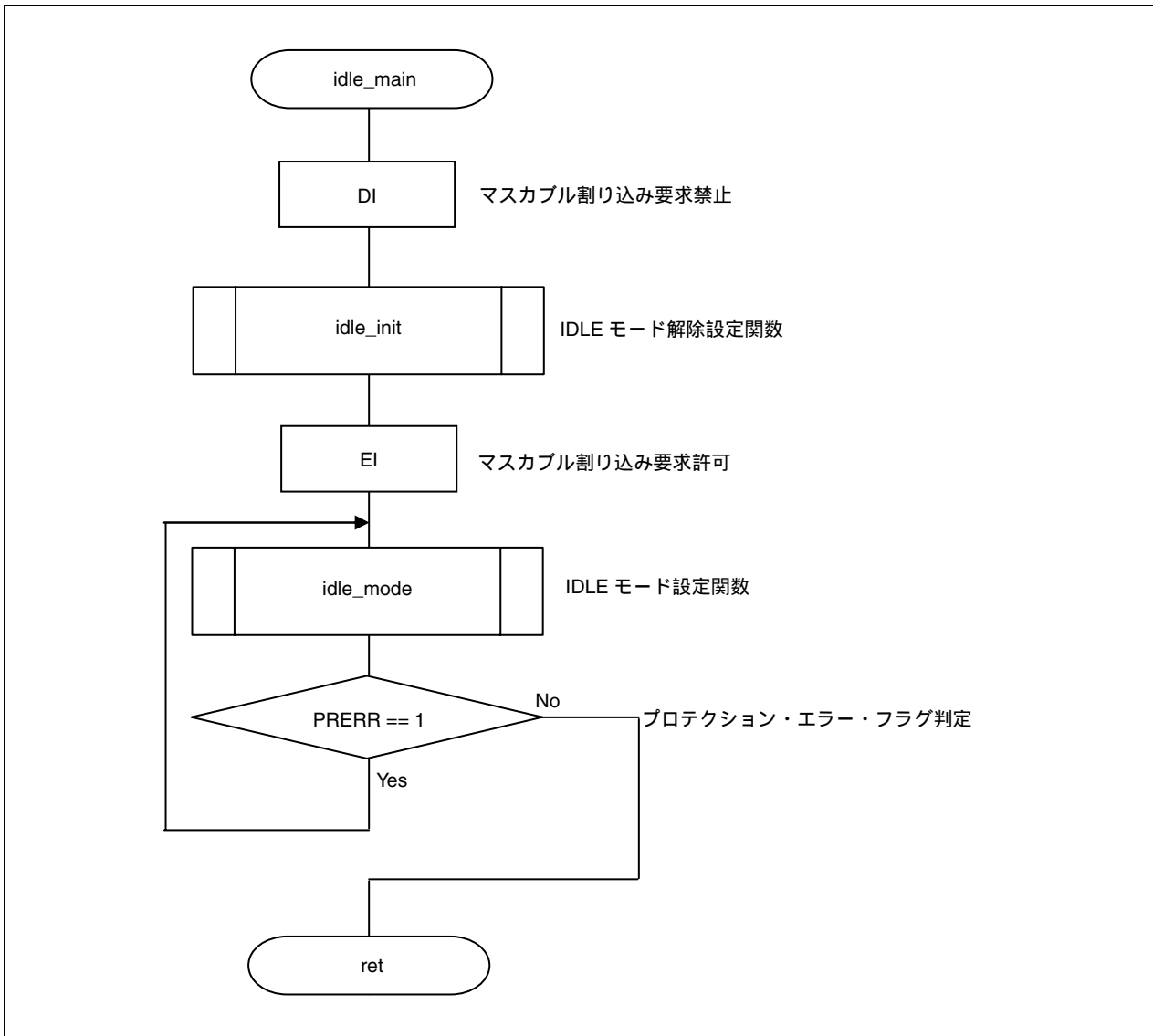
図2-1 IDLEモード (1/3)
