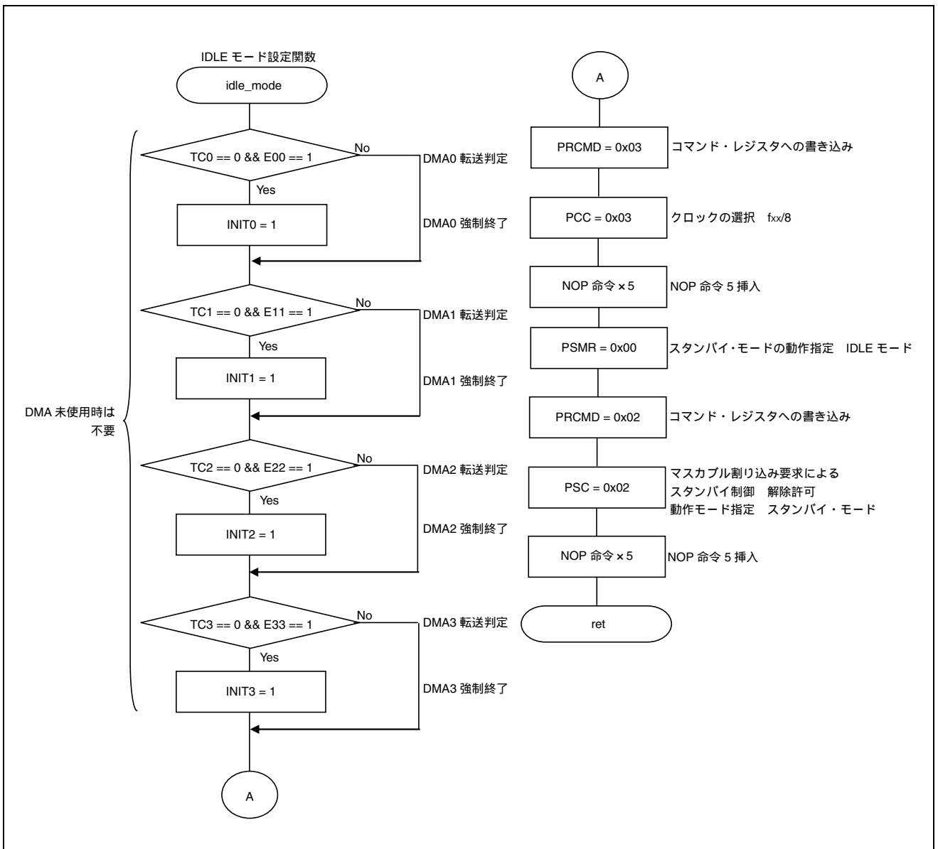
図2-1 IDLEモード (3/3)
