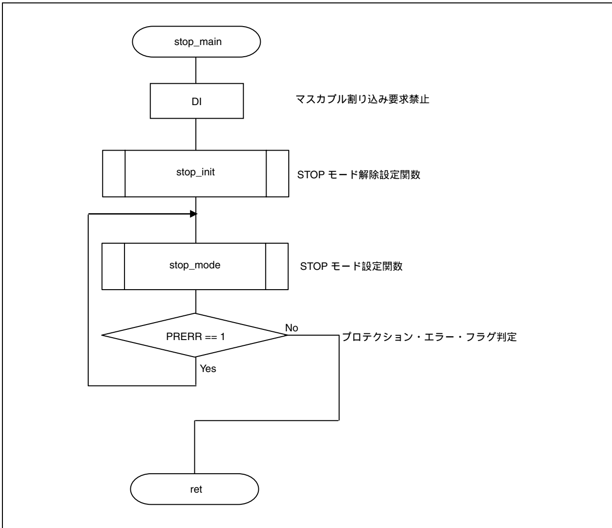
図3 - 1 STOPモード (1/3)
