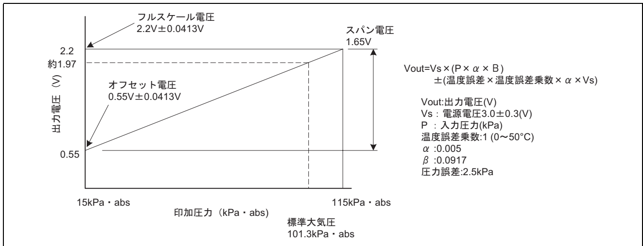
図 3 出力特性(参考)
