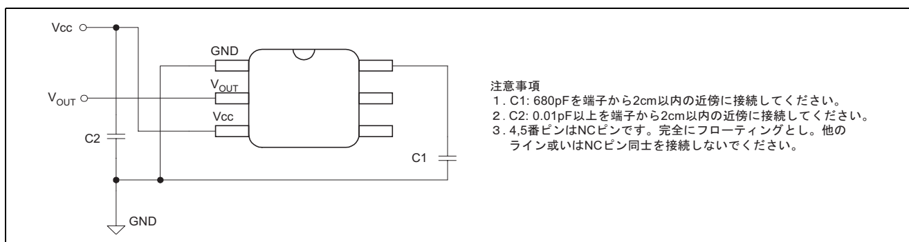
図 2 接続図(参考)
