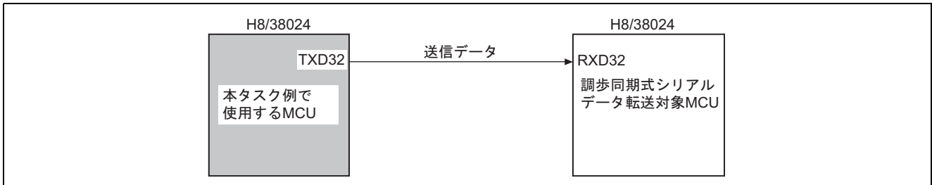
図 1 調歩同期式シリアルデータ送信
