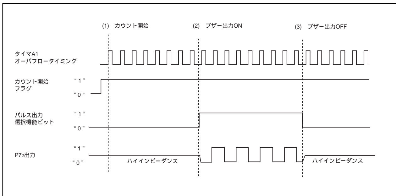
図1 ブザー出力の動作図
