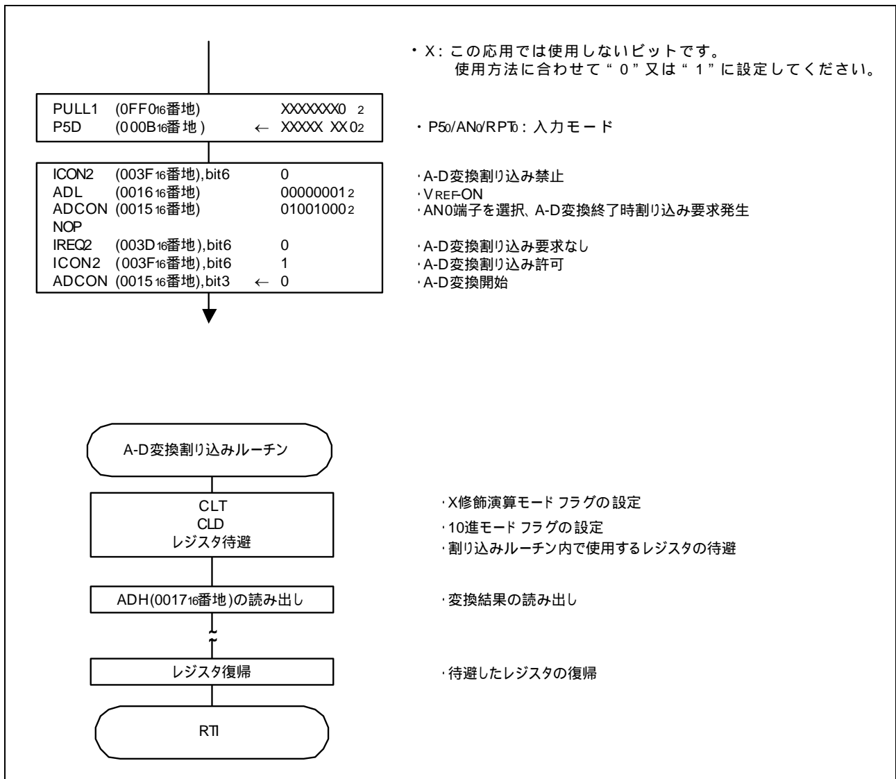
図 3.3 制御手順
