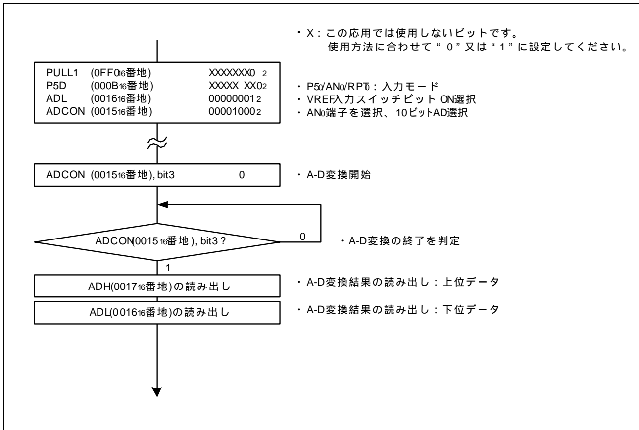
図 3.3 制御手順
