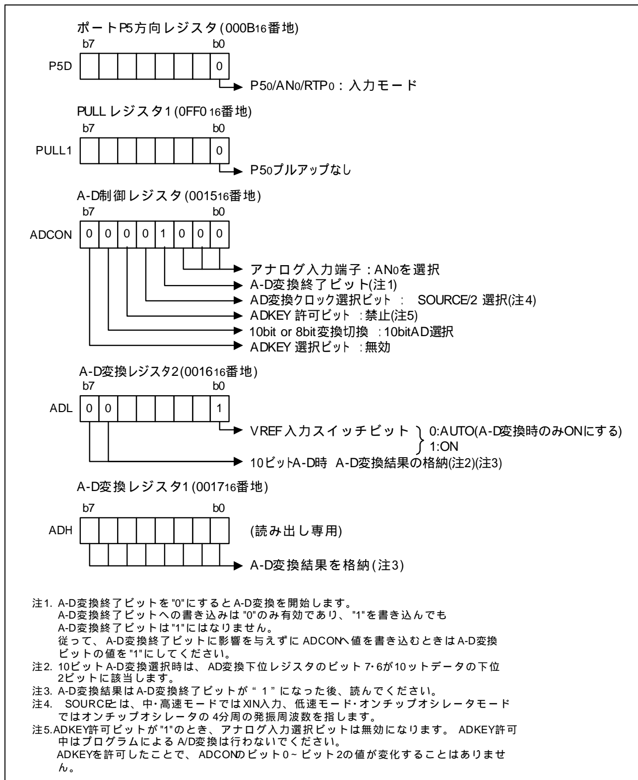
図 3.2 関連レジスタの設定
