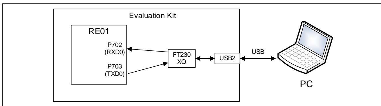
図 3.2 RE01 256KB グループ用サンプルコードシステム構成図
