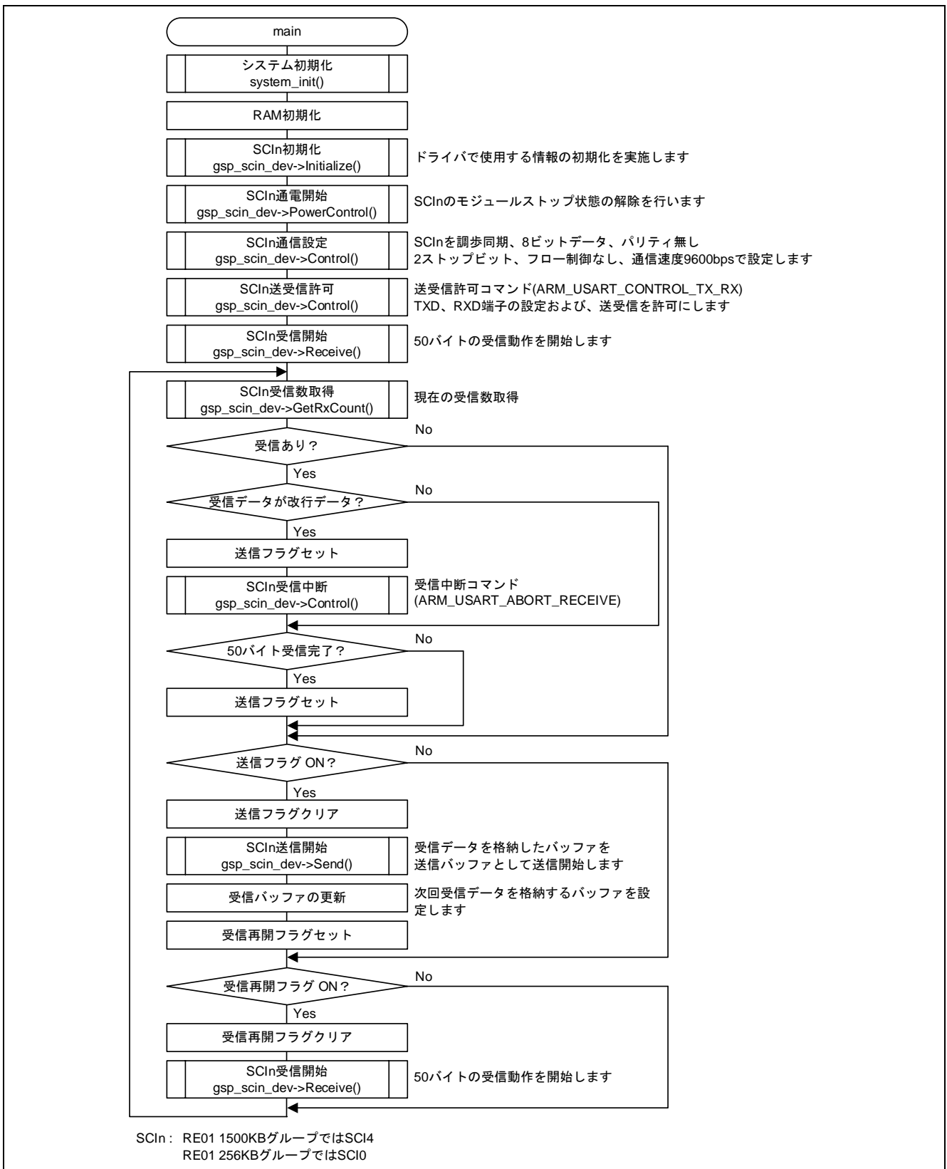
図 3.3 メイン処理
