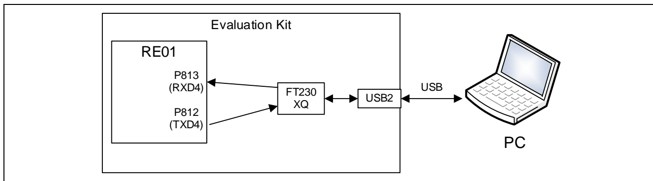
図 3.1 RE01 1500KB グループ用サンプルコードシステム構成図
