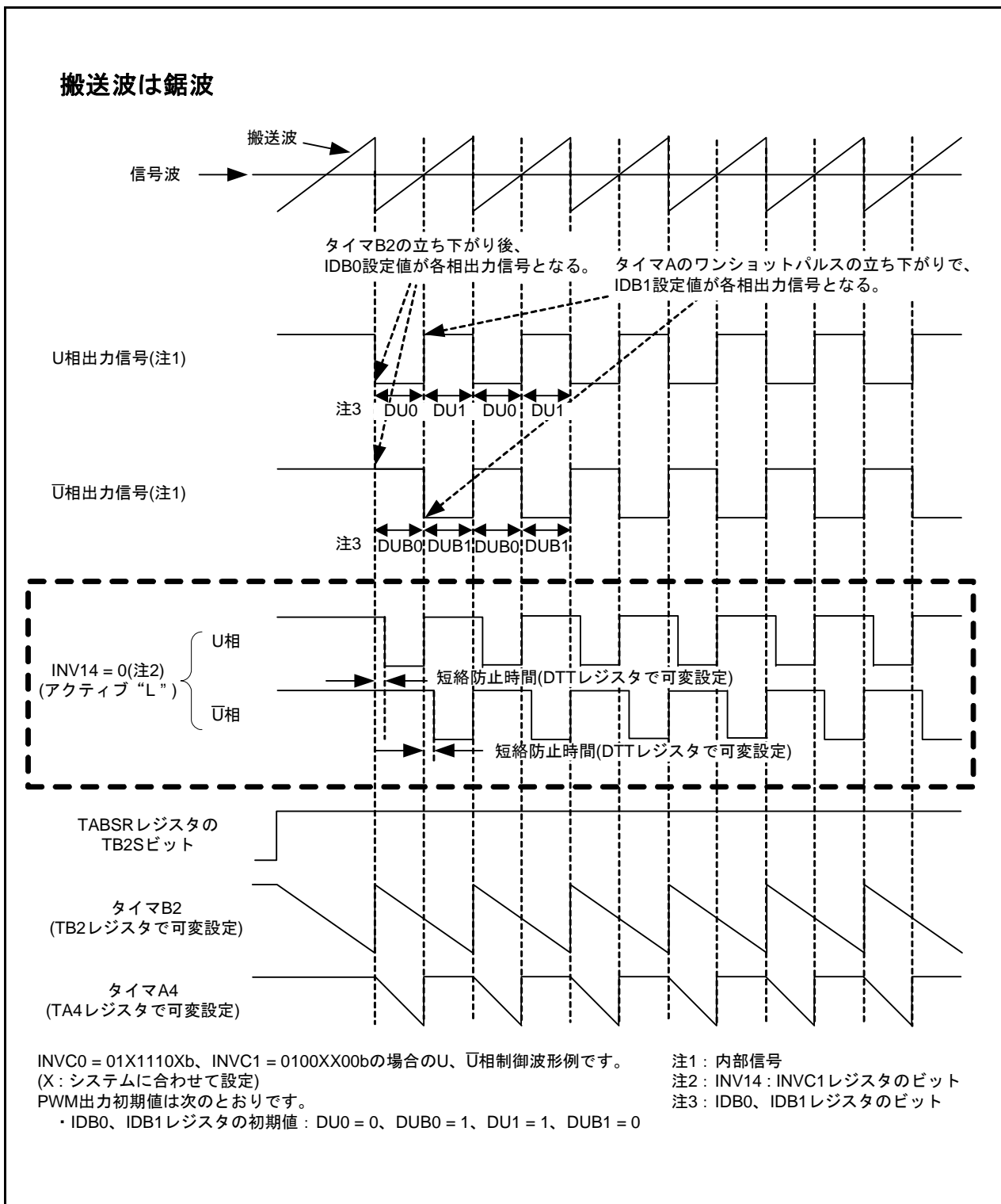
図 3.1 鋸波変調動作タイミング
