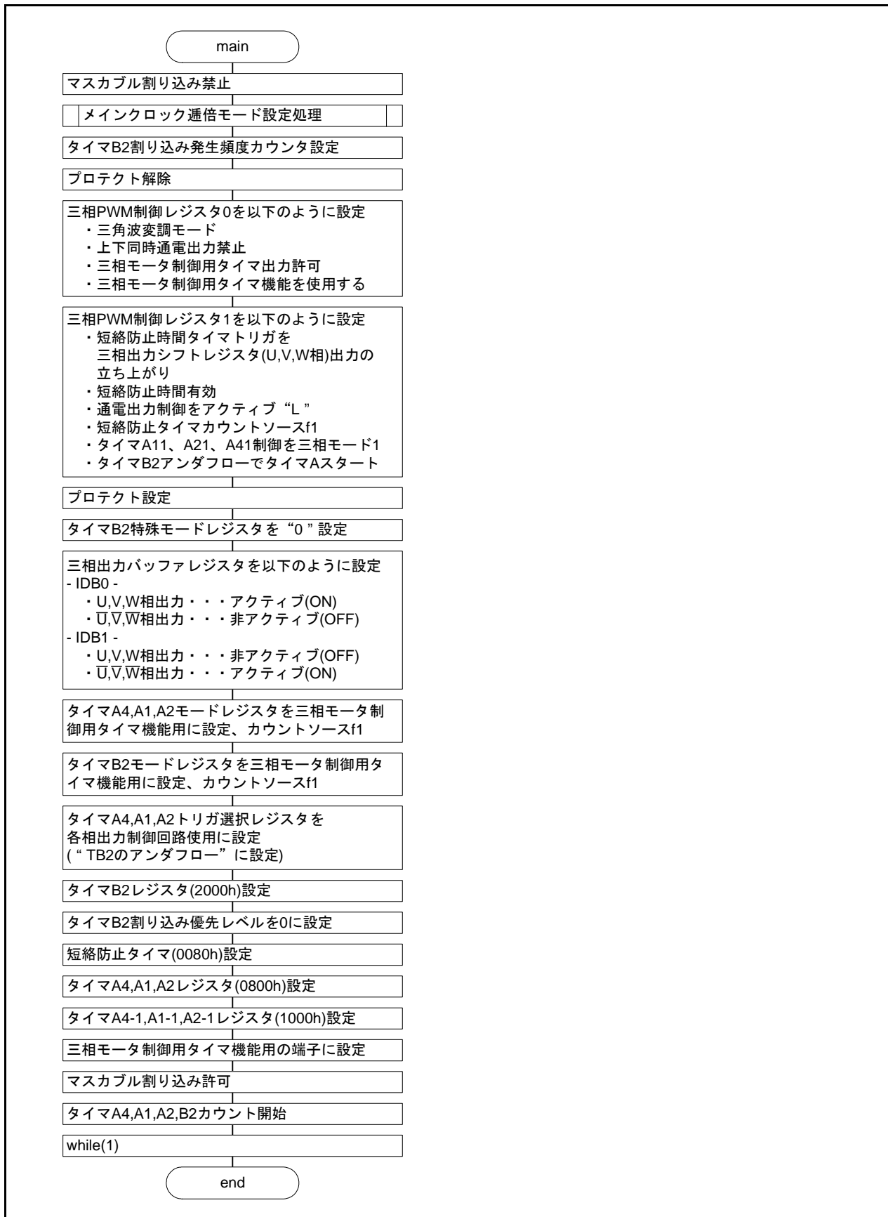
図 3.4 三角波変調(三相モード1)・フローチャート
