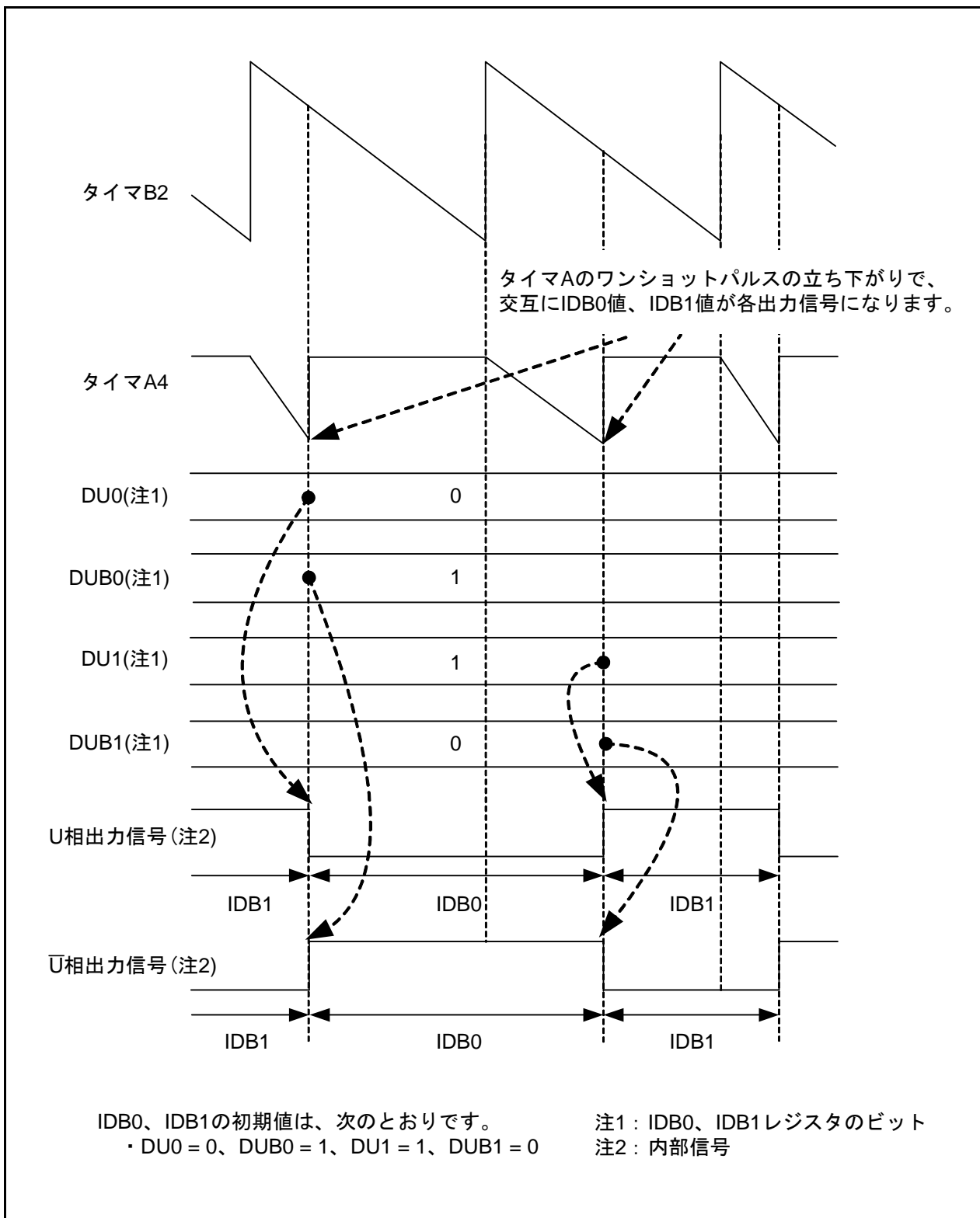
図 3.3 U相出力信号の動作例
