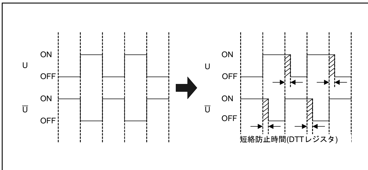
図 3.2 短絡防止時間(アクティブ“L”の場合)
