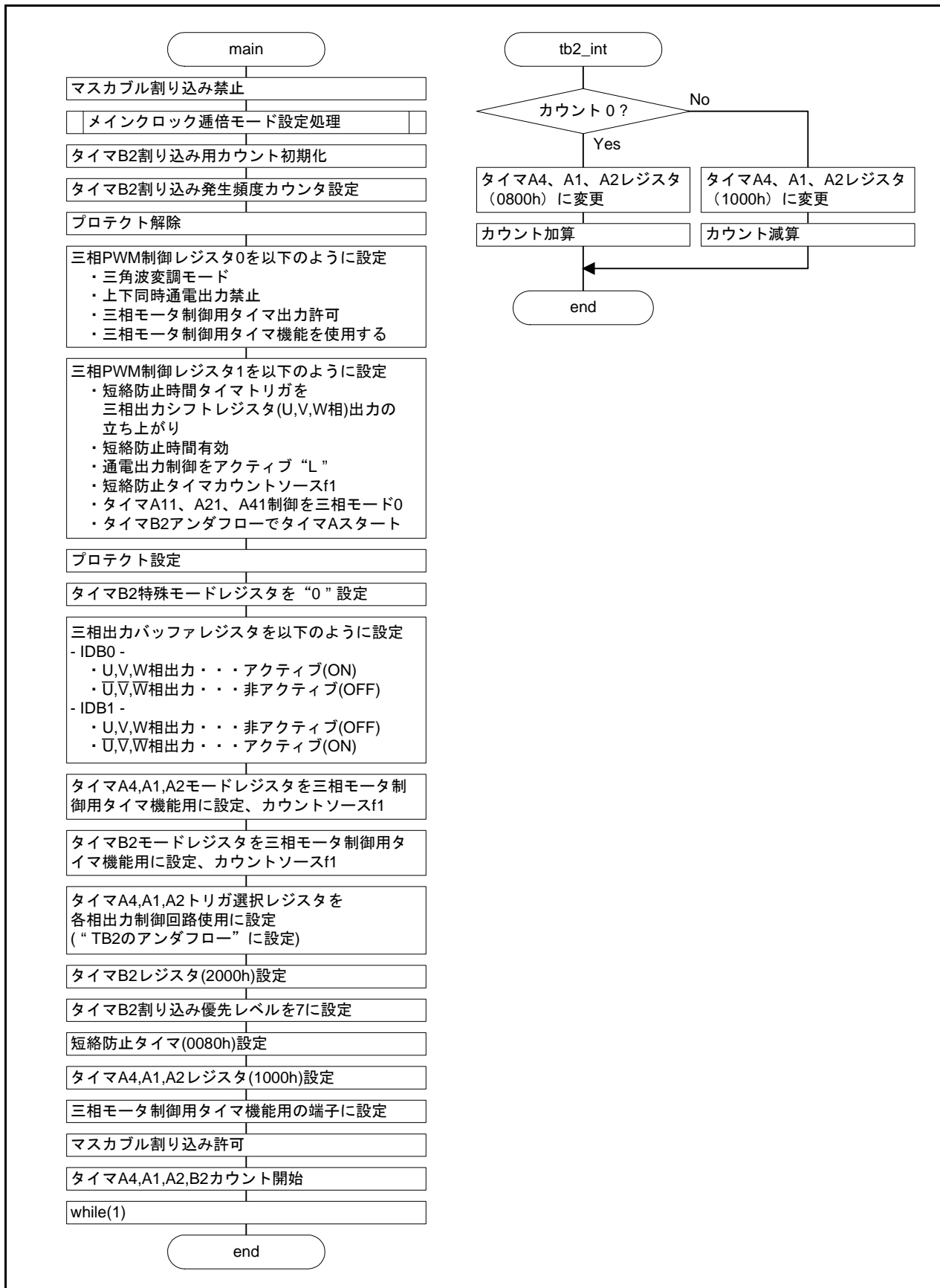
図 3.4 三角波変調(三相モード0)・フローチャート
