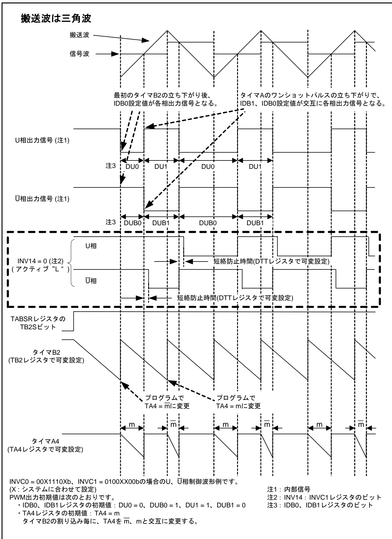
図 3.1 三角波変調(三相モード0)動作タイミング
