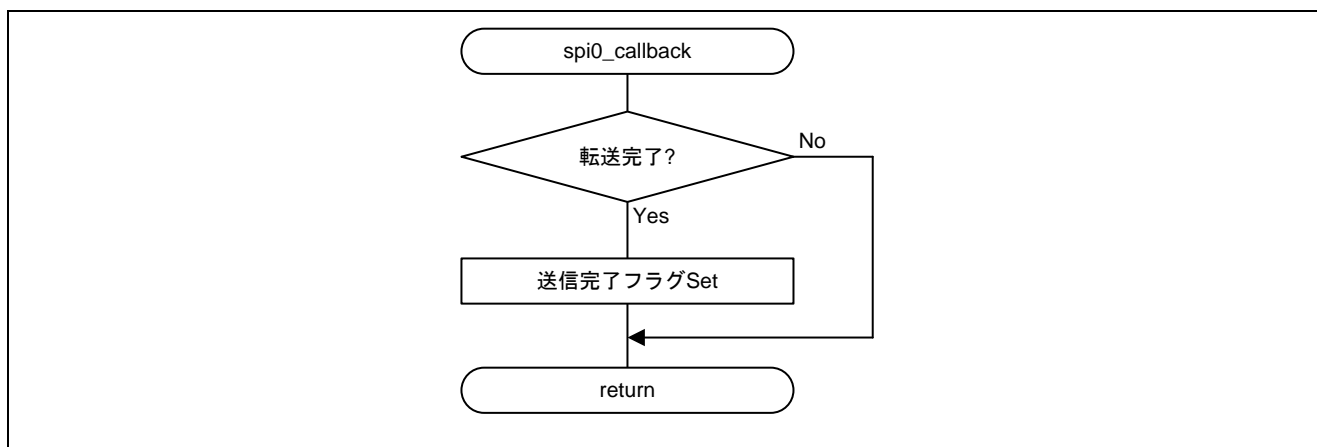
図 3.4 SPI0 転送完了コールバック処理
