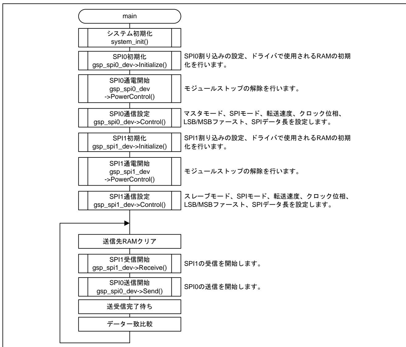
図 3.2 メイン処理
