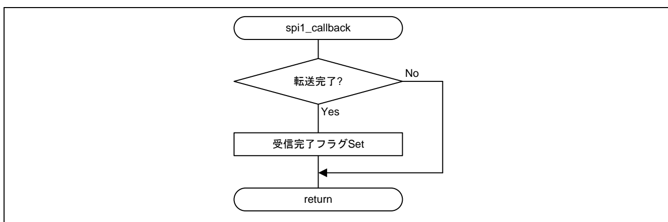
図 3.5 SPI1 転送完了コールバック処理
