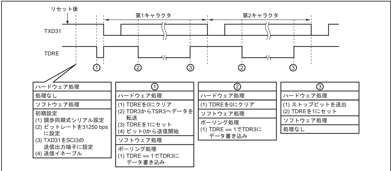
図4 調歩同期式モードシリアルデータ送信の動作説明
