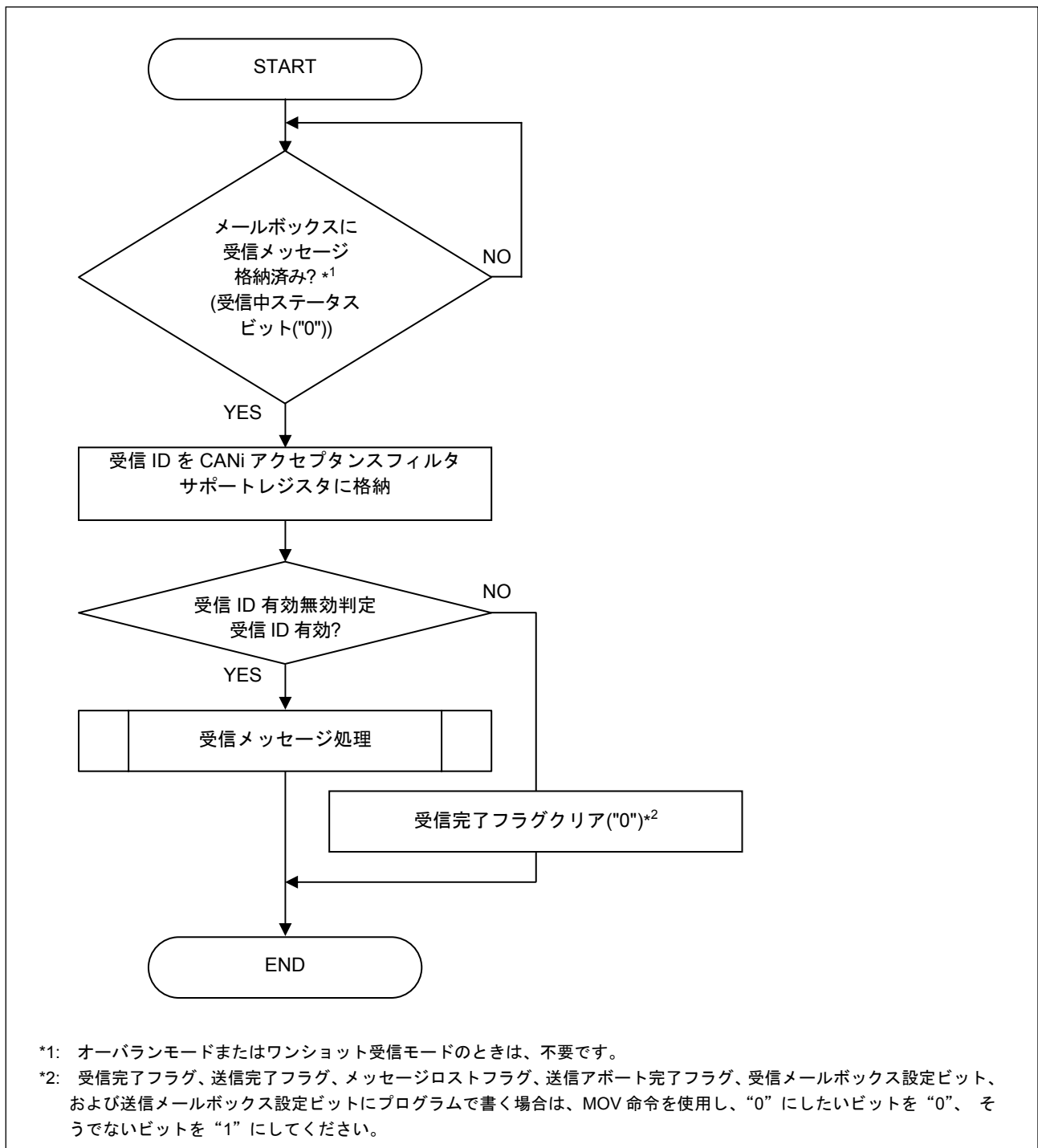
図7.7 アクセプタンスフィルタサポートユニット使用手順
