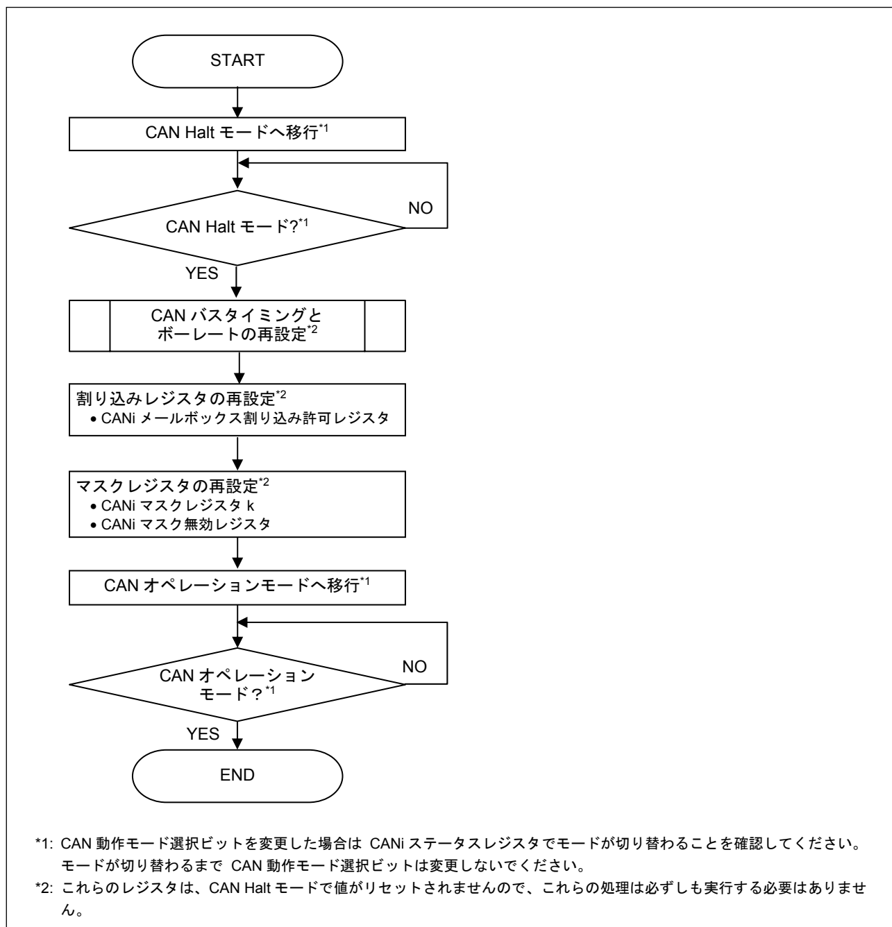
図2.3 CAN Halt モードへ移行した後に行う CAN コンフィグレーション手順
