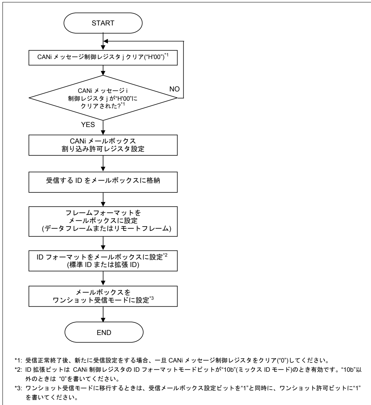
図2.13 ワンショット受信要求手順
