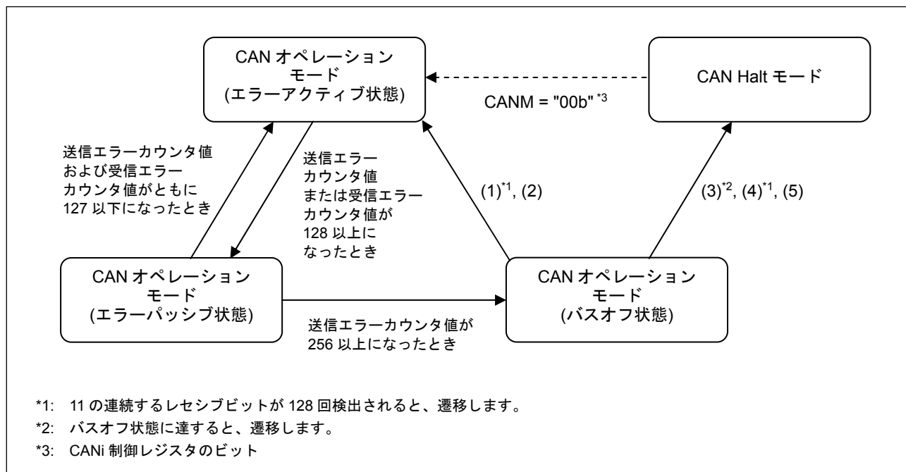
図6.1 バスオフ状態への遷移およびバスオフ状態からの復帰
