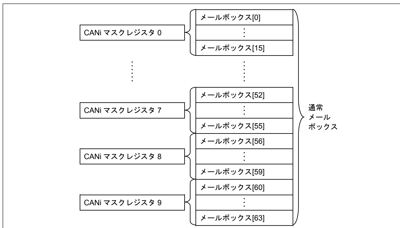
図3.1 通常メールボックスモードのメールボックス構造
