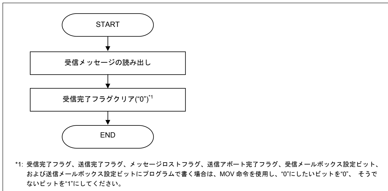
図2.14 ワンショット受信モードに設定したメールボックスの受信メッセージ処理手順
