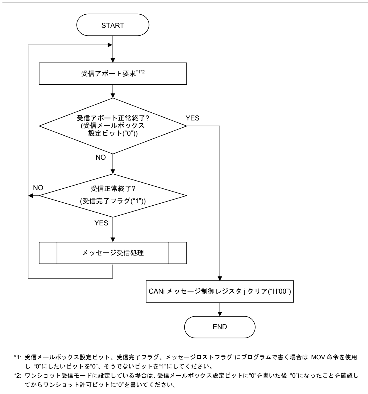
図2.15 受信アポート手順
