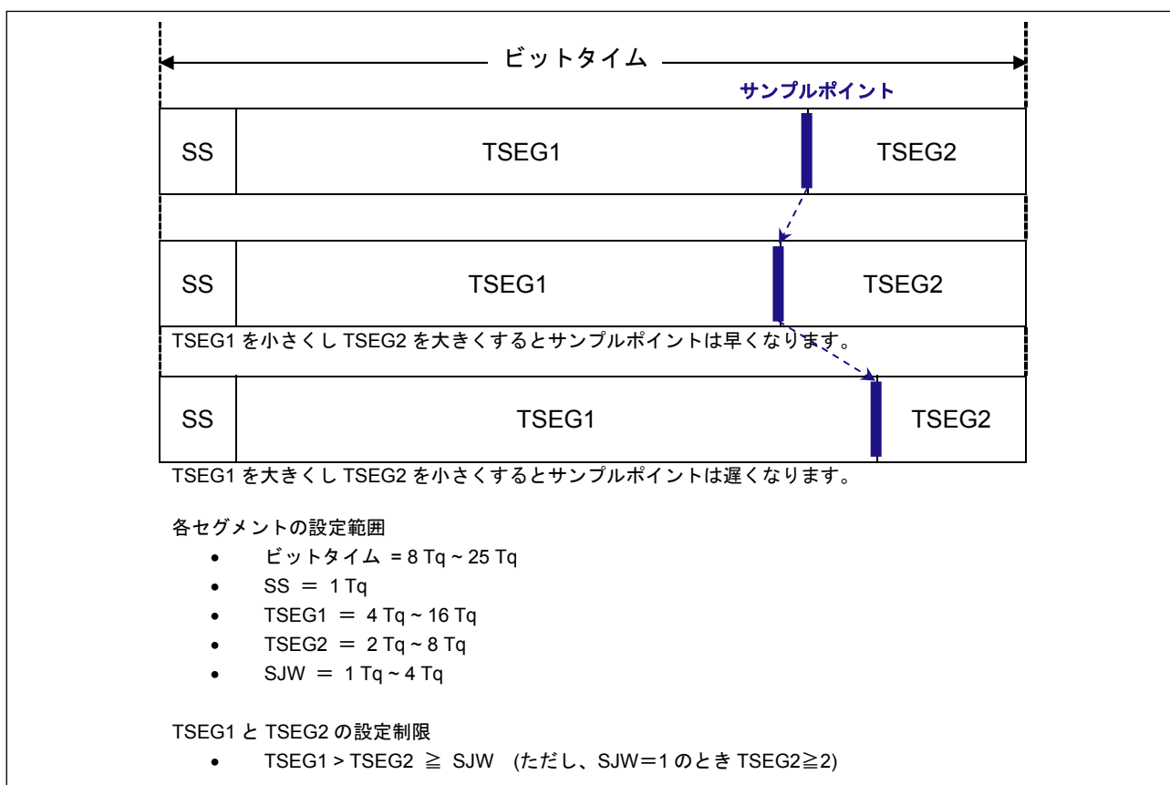
図 1.1 ビットのセグメント構成とサンプルポイント
