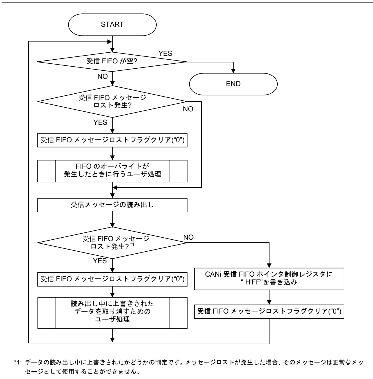
図3.6 FIFO メールボックスモードでの受信処理手順(オーバーライトモード)
