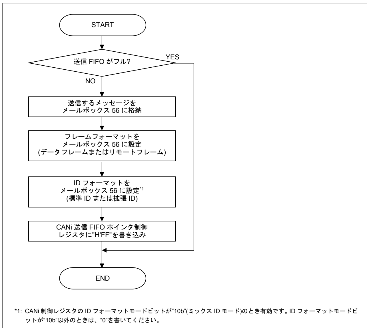
図3.5 FIFO メールボックスモードでの送信処理手順
