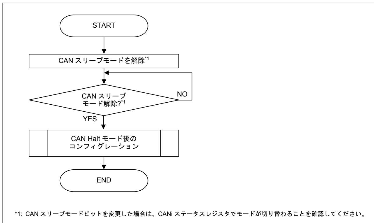
図8.4 CAN Halt モード時のCAN ウェイクアップ手順
