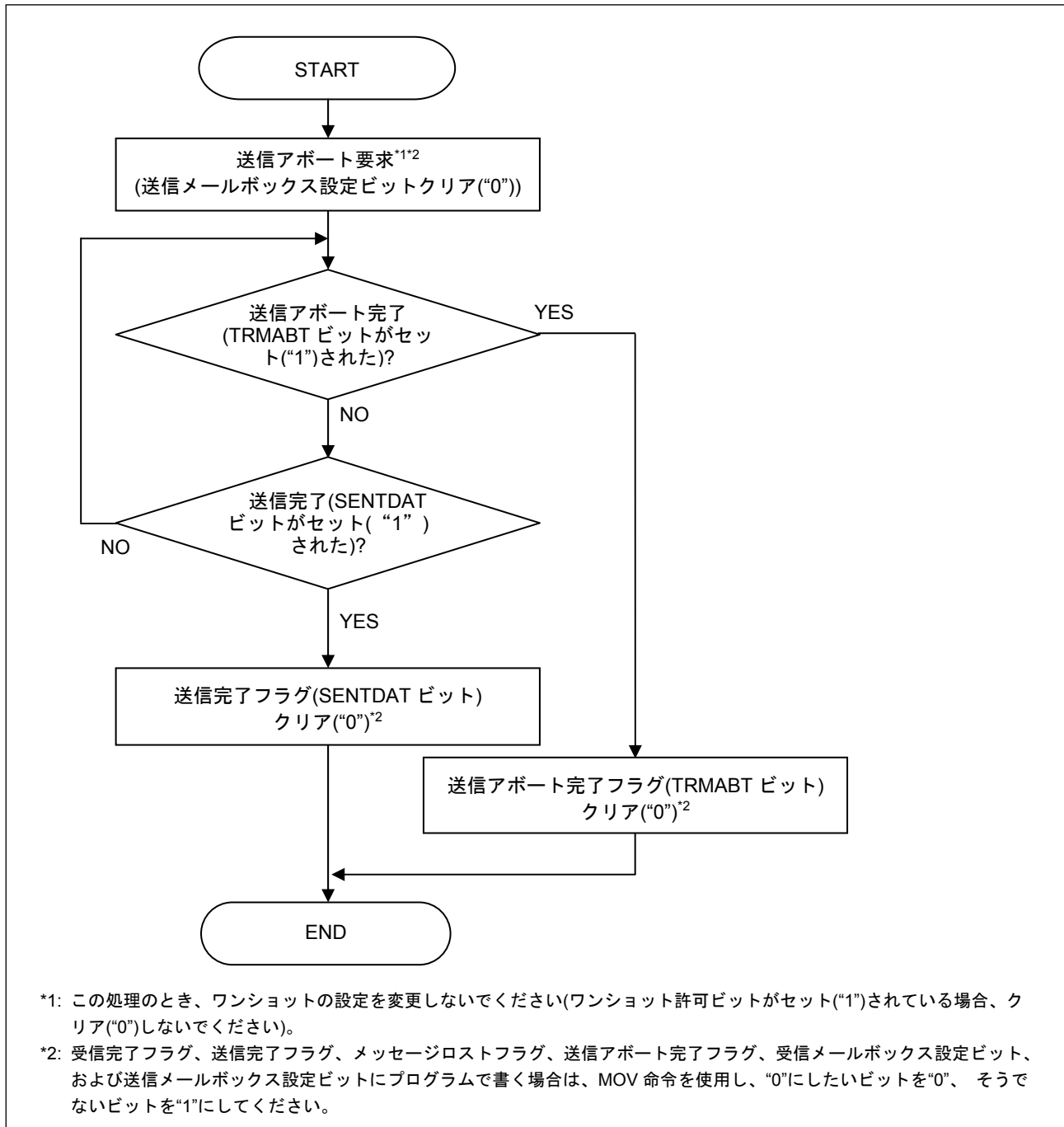
図2.9 送信アボート手順
