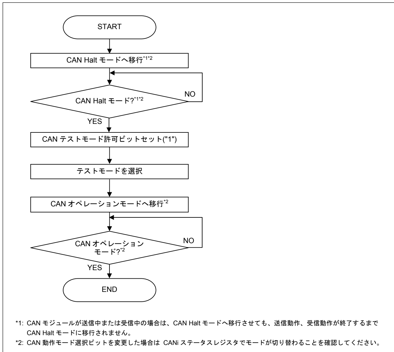
図9.1 テストモードの設定手順
