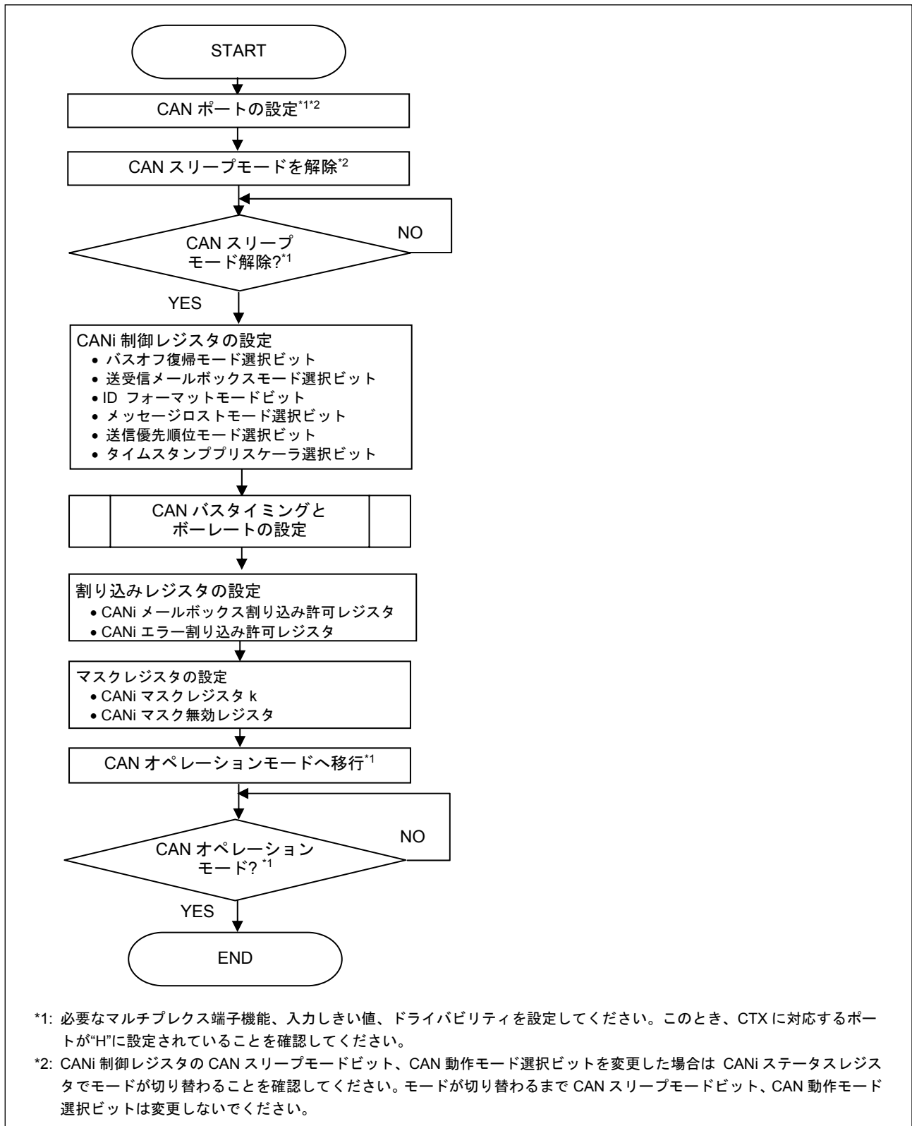
図2.1 ハードウェアリセット後に行う CAN コンフィグレーション手順
