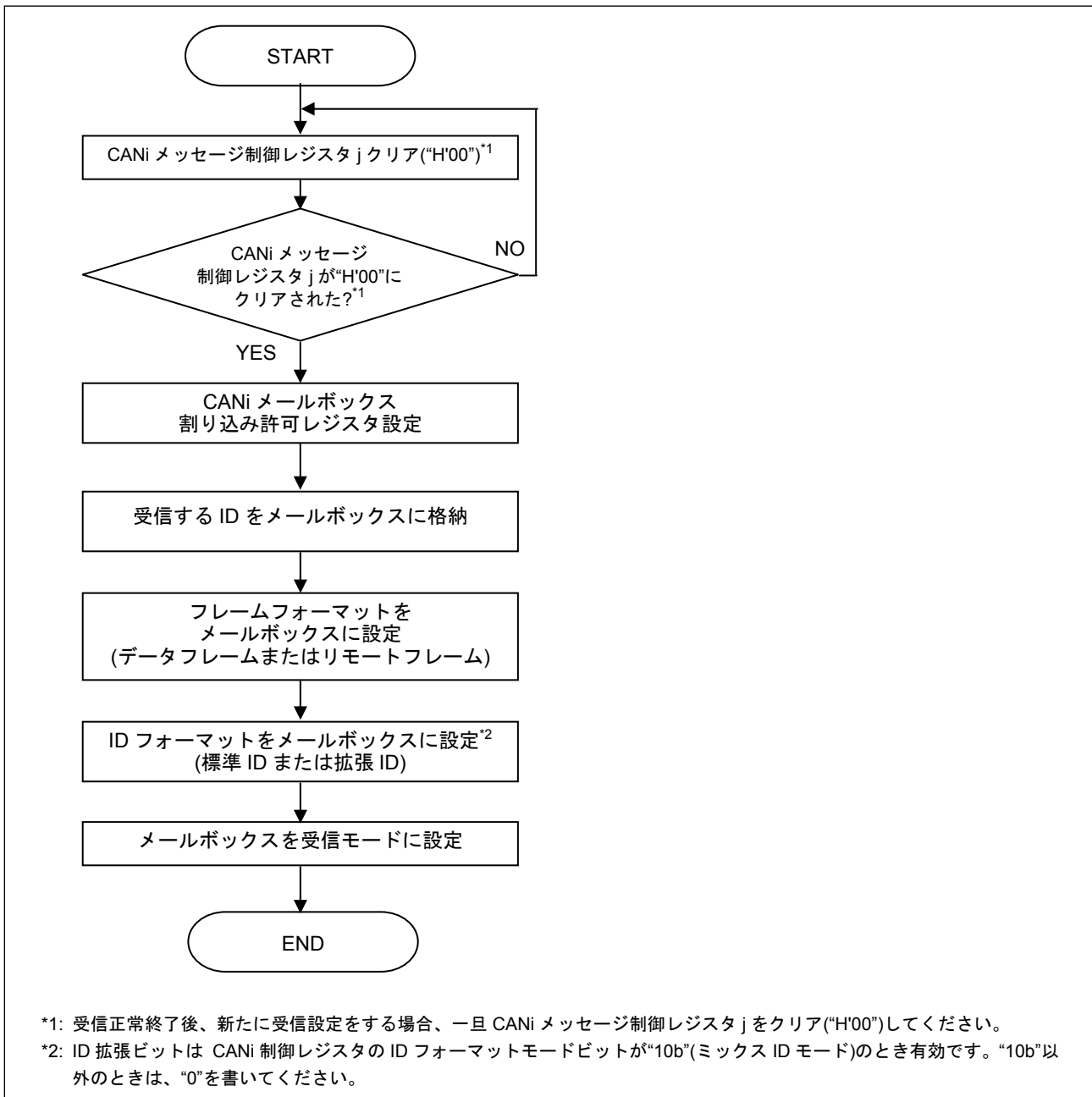
図2.10 受信要求手順
