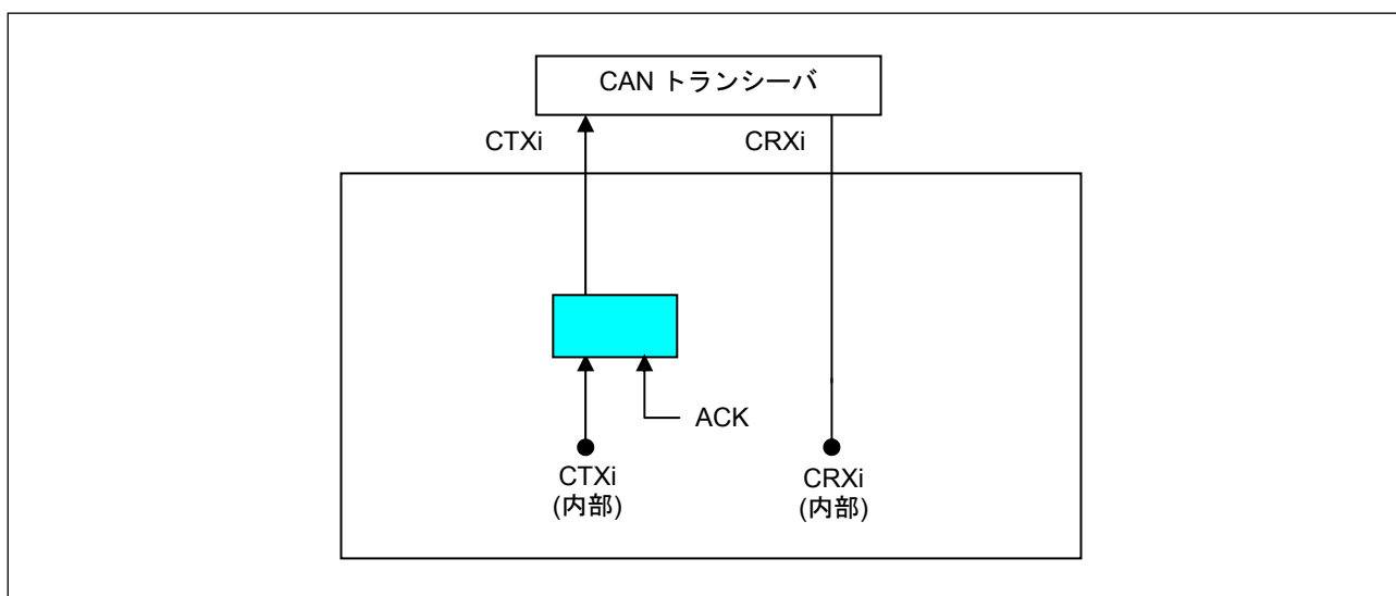
図9.3 セルフモード 0時の接続イメージ
