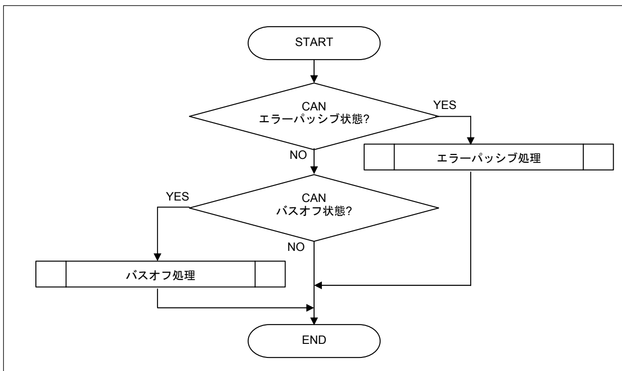
図5.1 CANi ステータスレジスタによる CAN エラー確認手順
