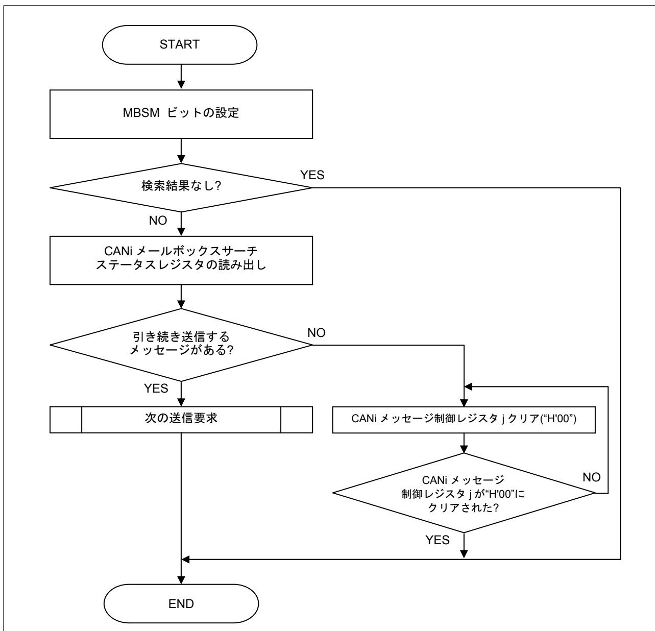
図4.3 送信メールボックス検索手順
