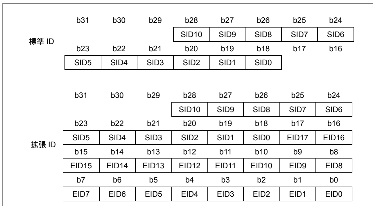
図7.1 標準 ID と拡張 ID のビットマップ
