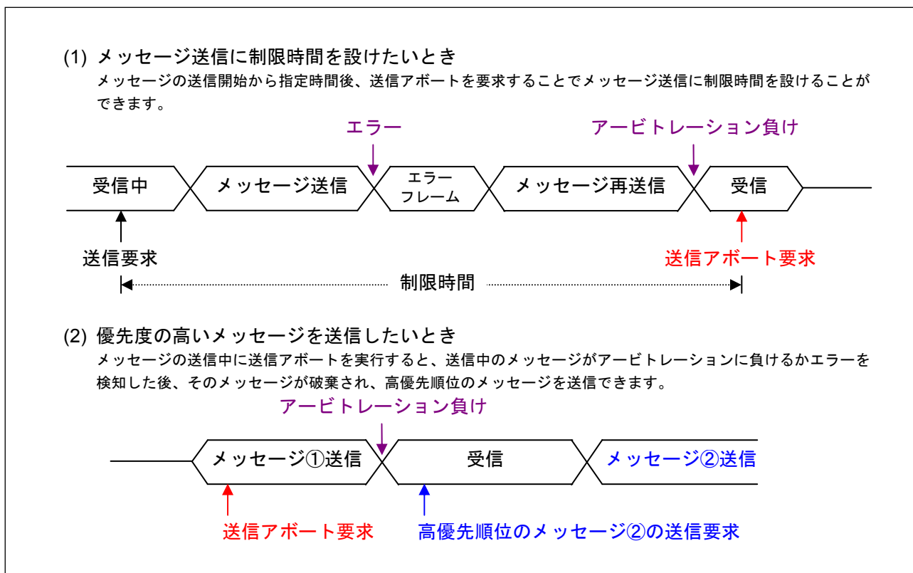
図2.8 送信アボート機能の応用例
