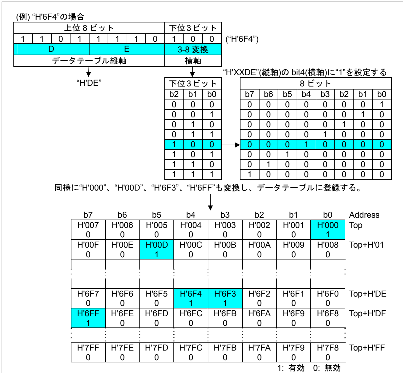
図7.5 データテーブル構成(データテーブル作成例)
