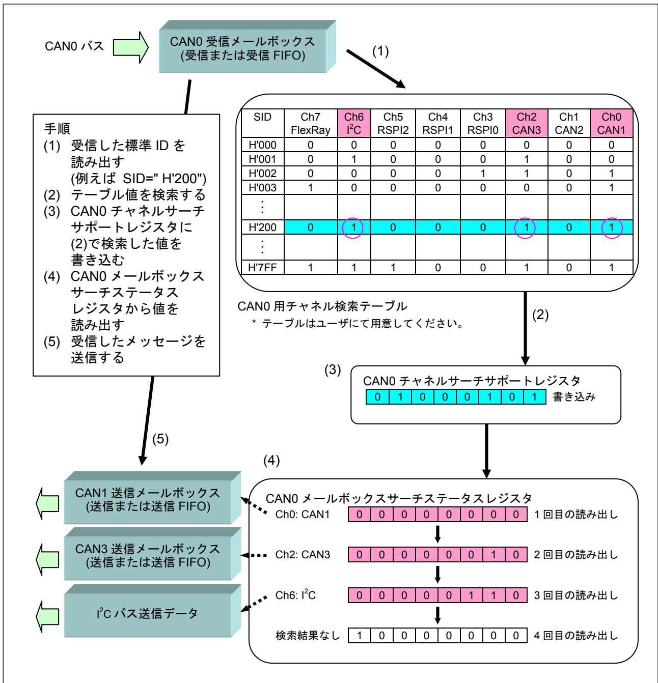
図4.5 チャネル検索モードの概略(CAN0 の場合)
