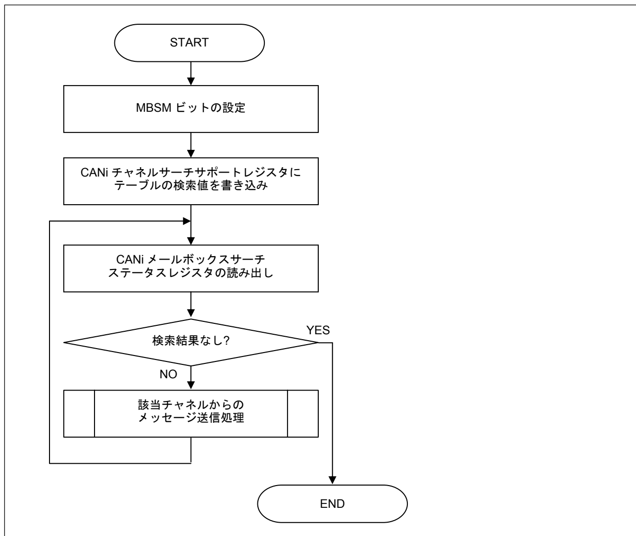
図4.6 チャンネル検索手順
