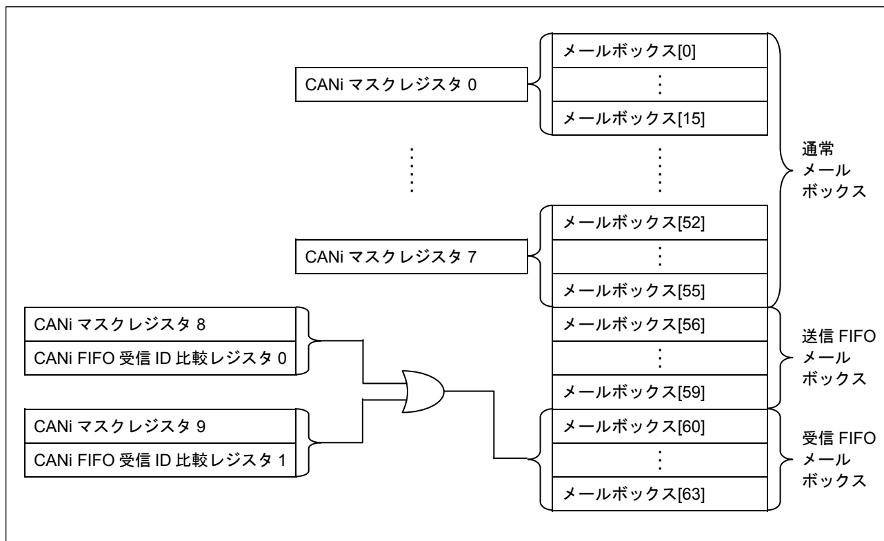
図3.2 FIFO メールボックスモードのメールボックス構造
