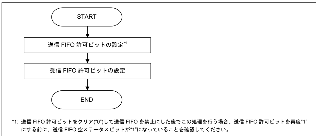
図3.4 CAN オペレーションモードの FIFO メールボックスモード設定手順
