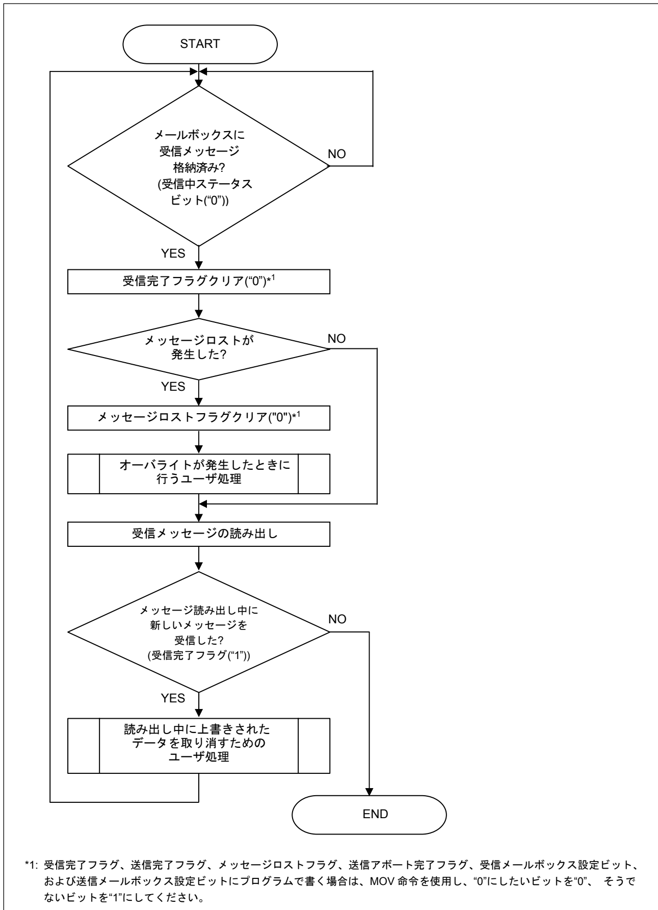
図2.11 受信モードに設定したメールボックスの受信メッセージ処理手順(オーバーライトモード)
