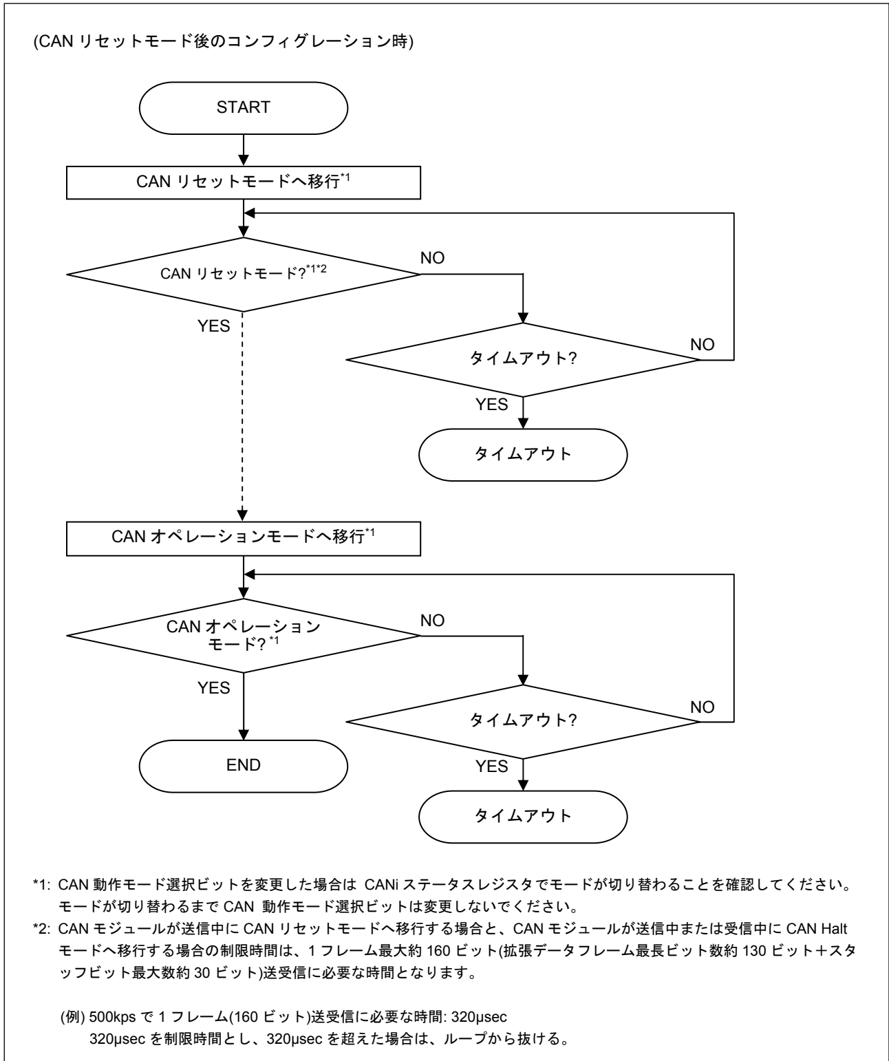
図10.1 ループの制限時間を持たせた場合の処理例
