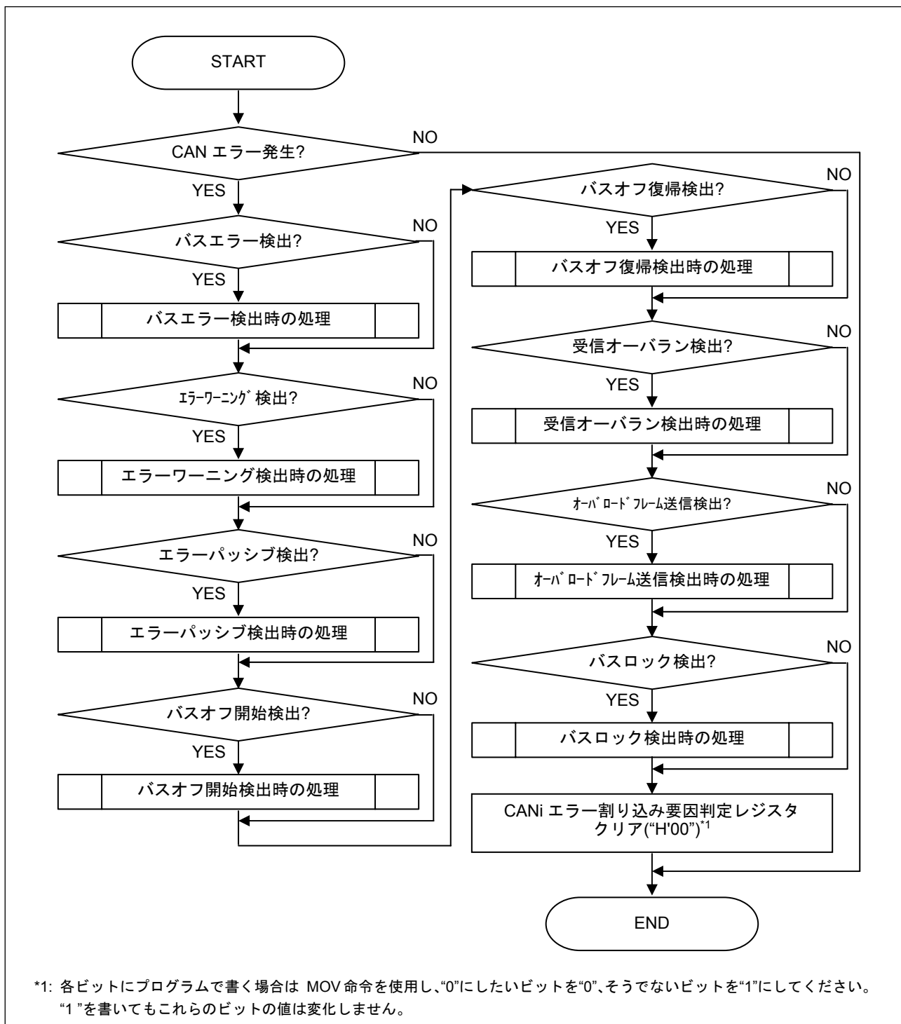
図5.2 CANi エラー割り込み要因判定レジスタによる CAN エラー確認手順
