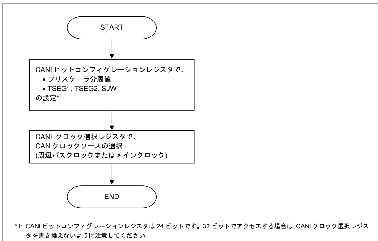
図1.4 CAN ビットタイミングと転送速度の設定手順
