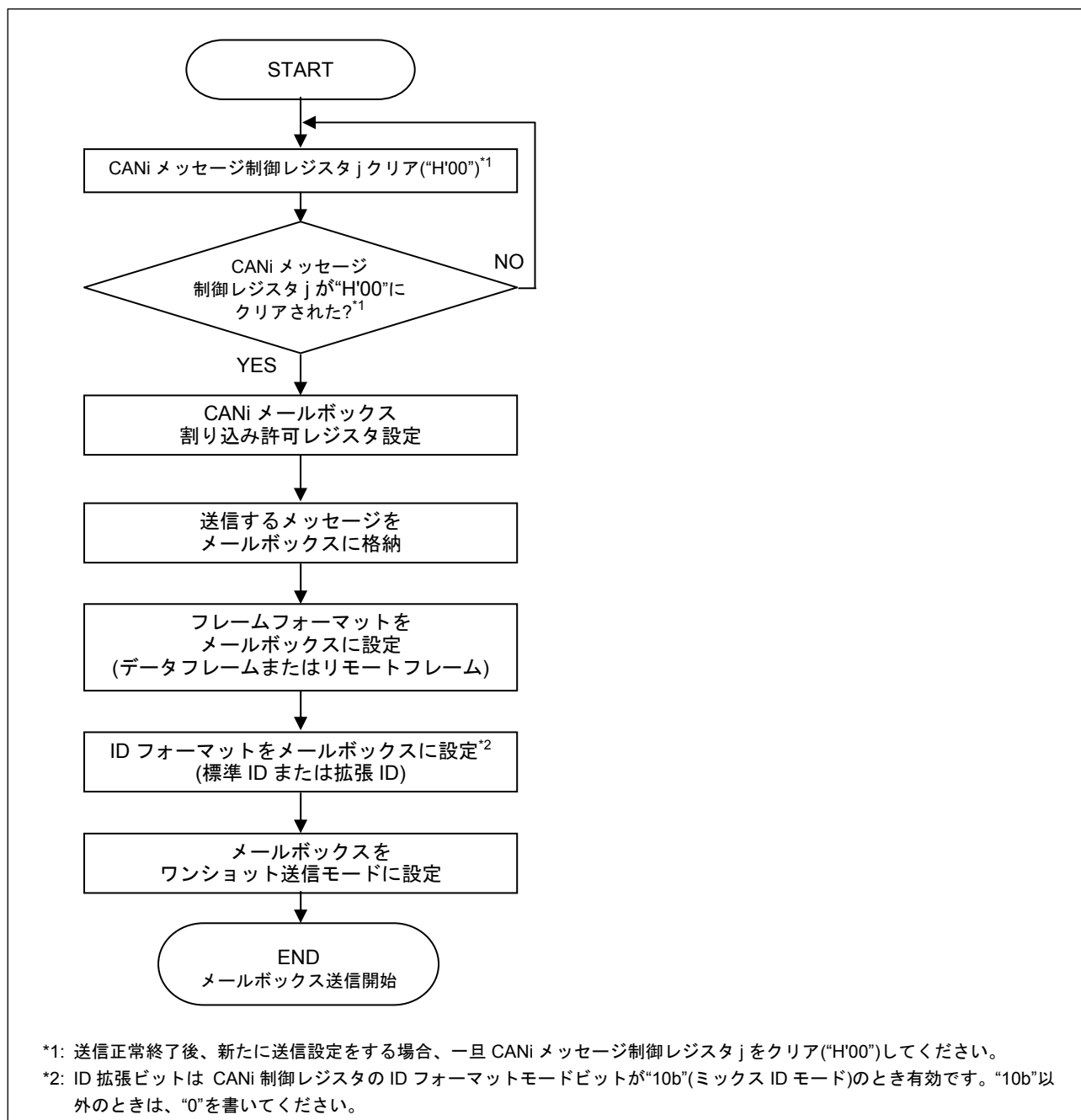
図2.6 ワンショット送信要求手順
