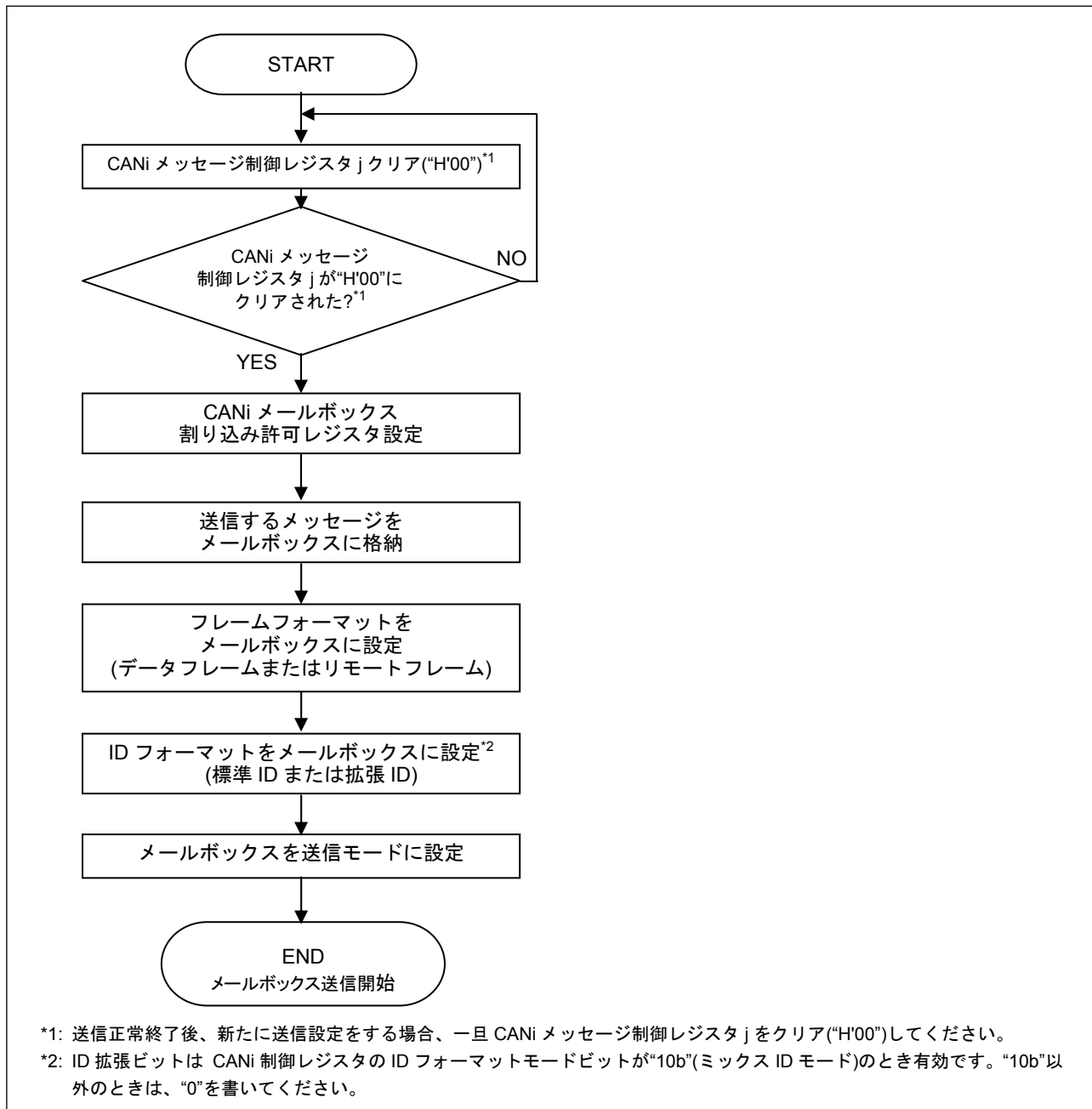
図2.4 送信要求手順
