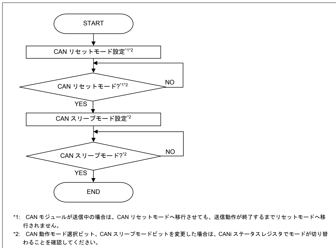
図8.1 CAN モジュールを CAN リセットモードへ移行してから CAN スリープモードへ移行させる手順
