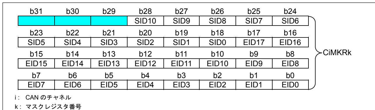
図7.3 ビットマップ
