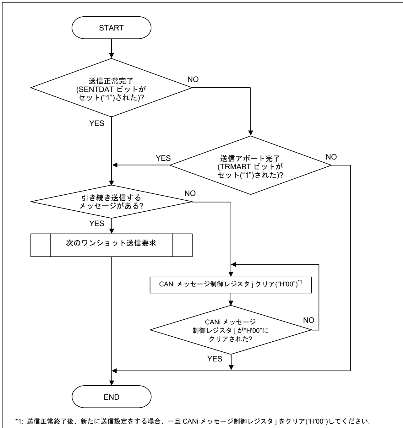
図2.7 ワンショット送信完了手順
