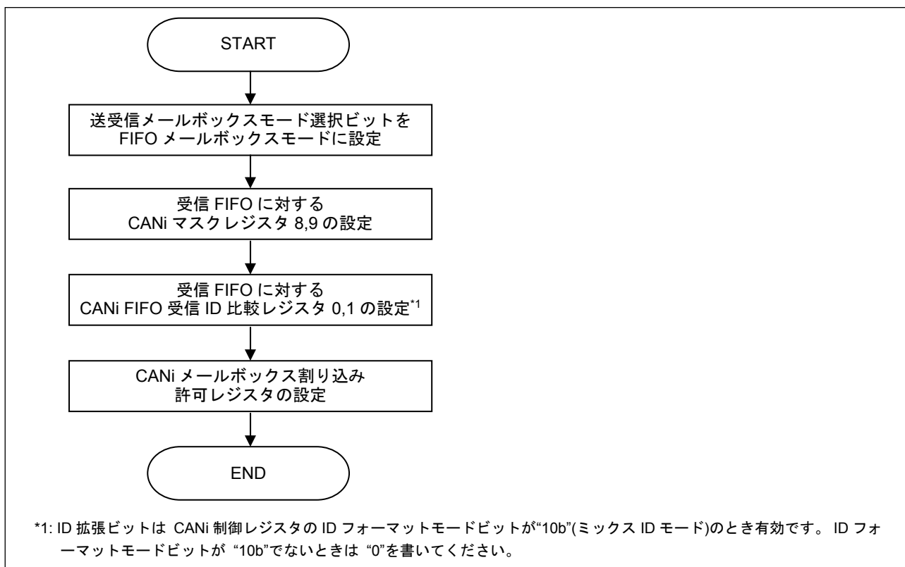
図3.3 CAN コンフィグレーションの FIFO メールボックスモード設定手順
