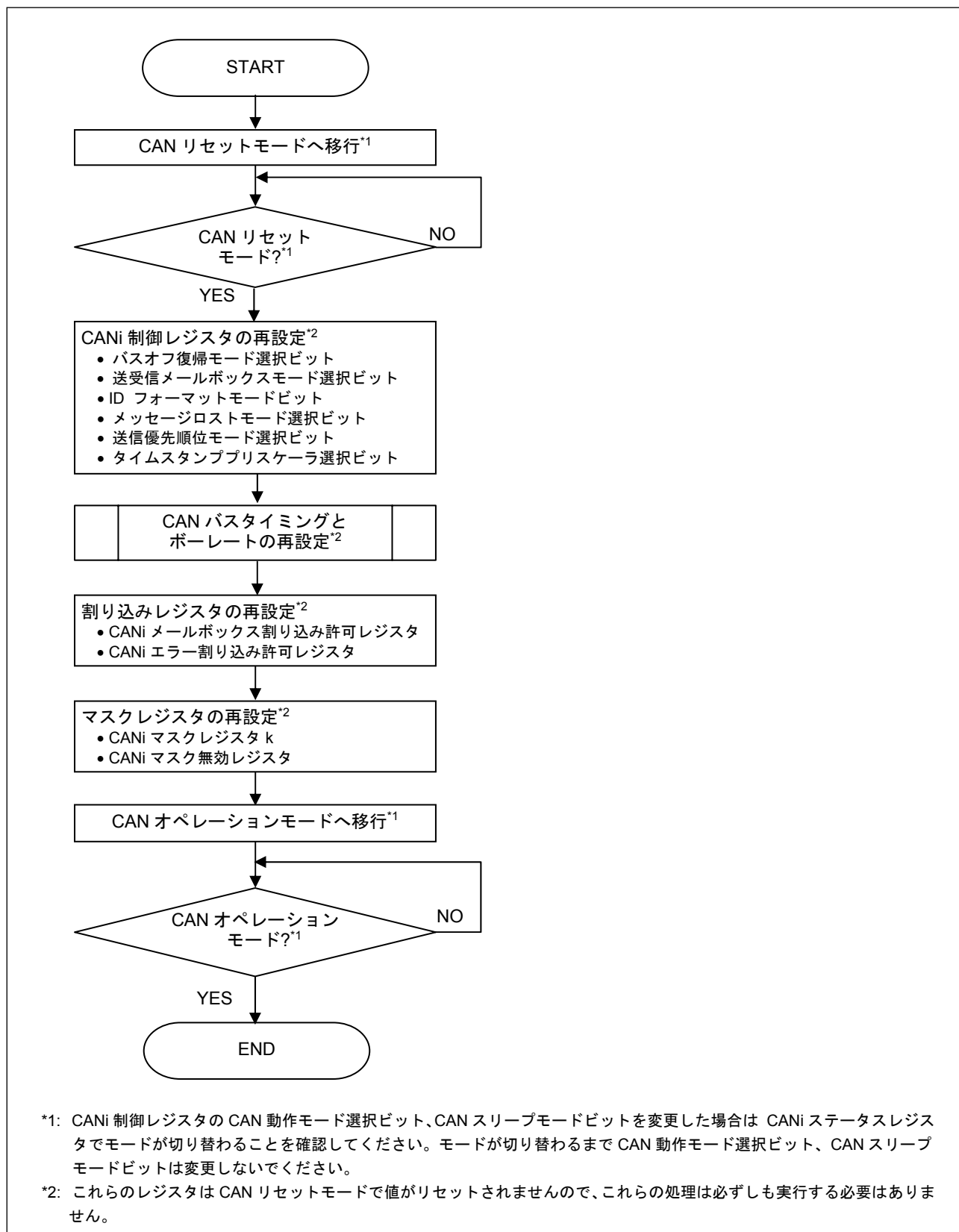
図2.2 CAN リセットモードへ移行した後に行う CAN コンフィグレーション手順
