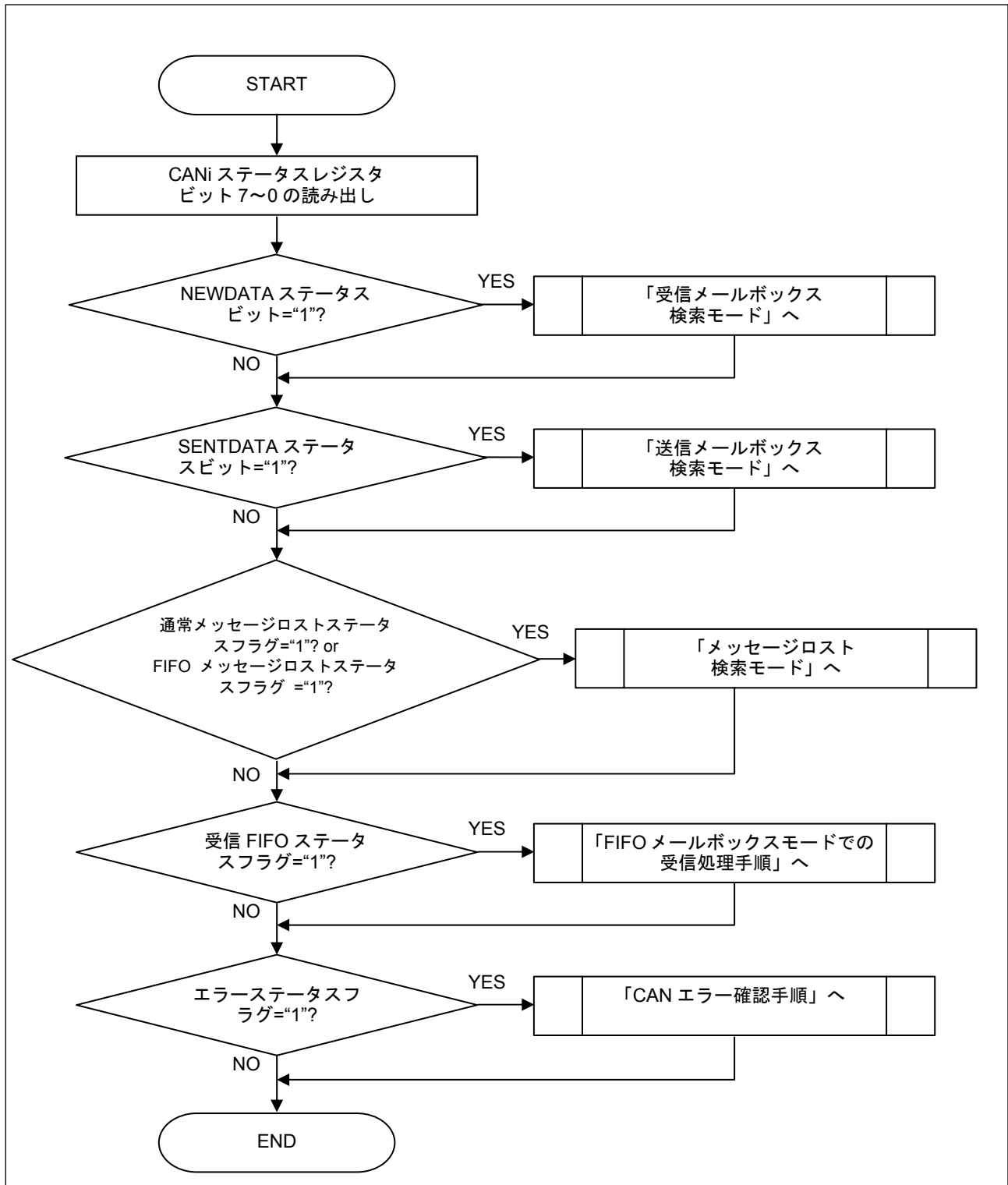
図4.1 CANi ステータスレジスタ確認例(ポーリング時)
