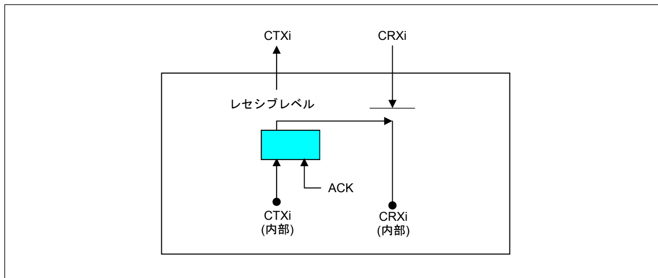
図9.4 セルフモード1時の接続イメージ
