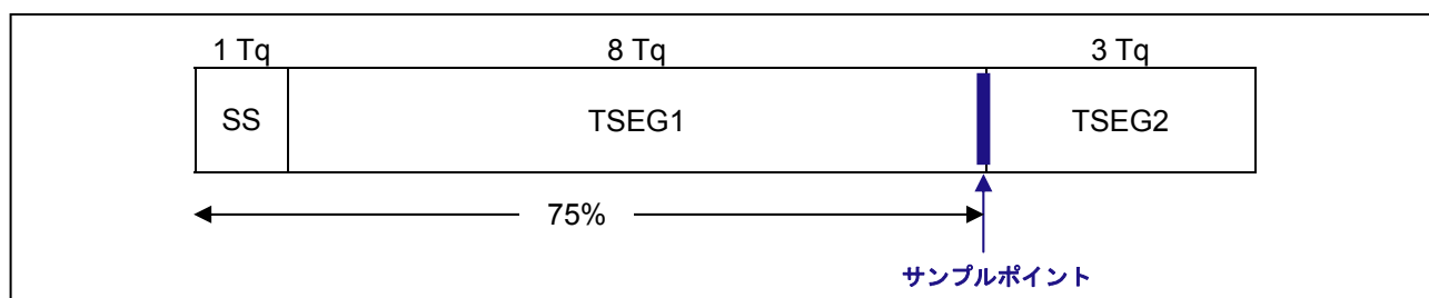
図1.2 サンプルポイントが75%のビットタイミングの設定例
