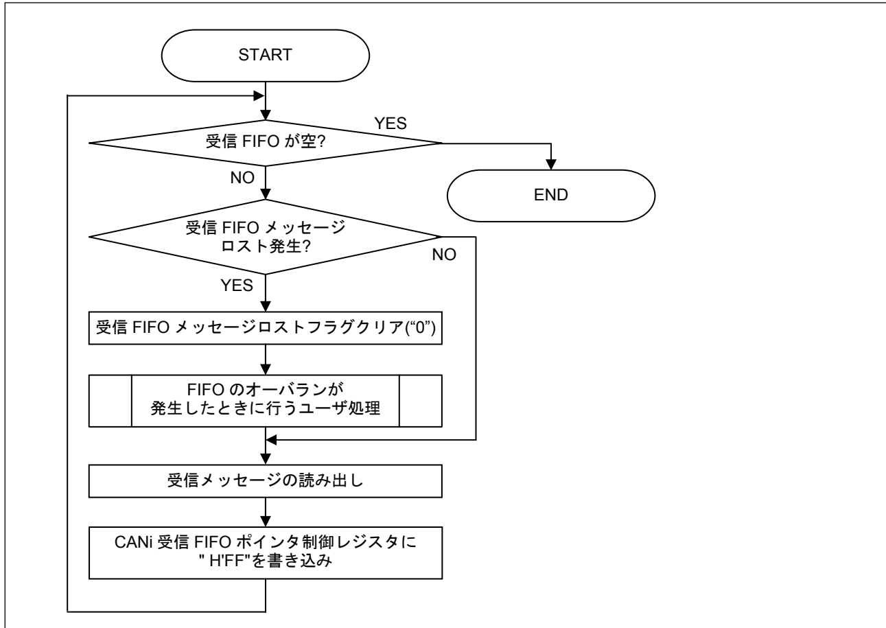
図3.7 FIFO メールボックスモードでの受信処理手順(オーバランモード)
