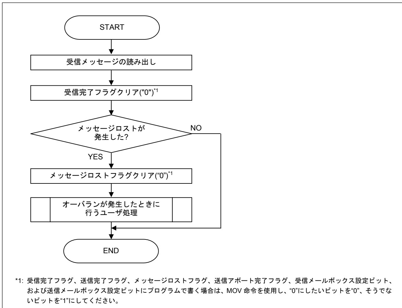
図2.12 受信モードに設定したメールボックスの受信メッセージ処理手順(オーバランモード)
