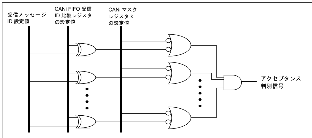
図7.4 FIFOi 受信 ID 比較レジスタと CANi マスクレジスタ k の構成
