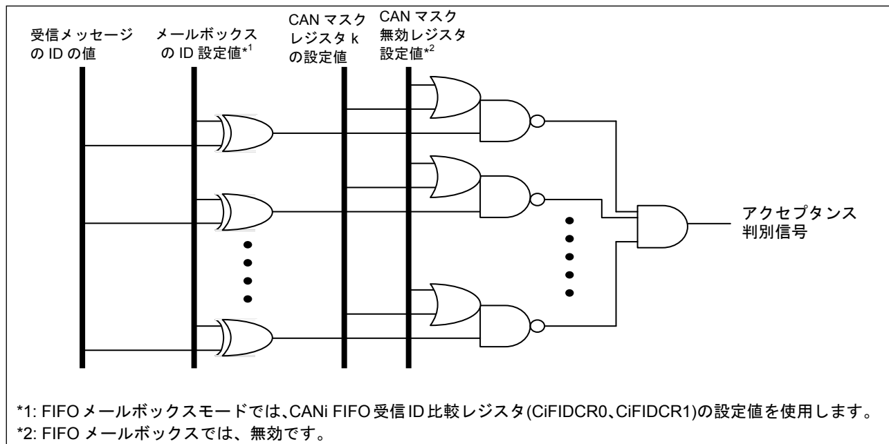
図7.2 IDとマスクレジスタの構成
