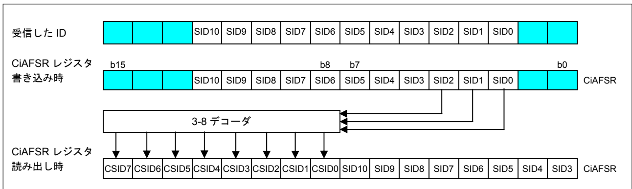
図7.6 CANi アクセプタンスフィルタサポートレジスタへの書き込み、読み出し時の状態
