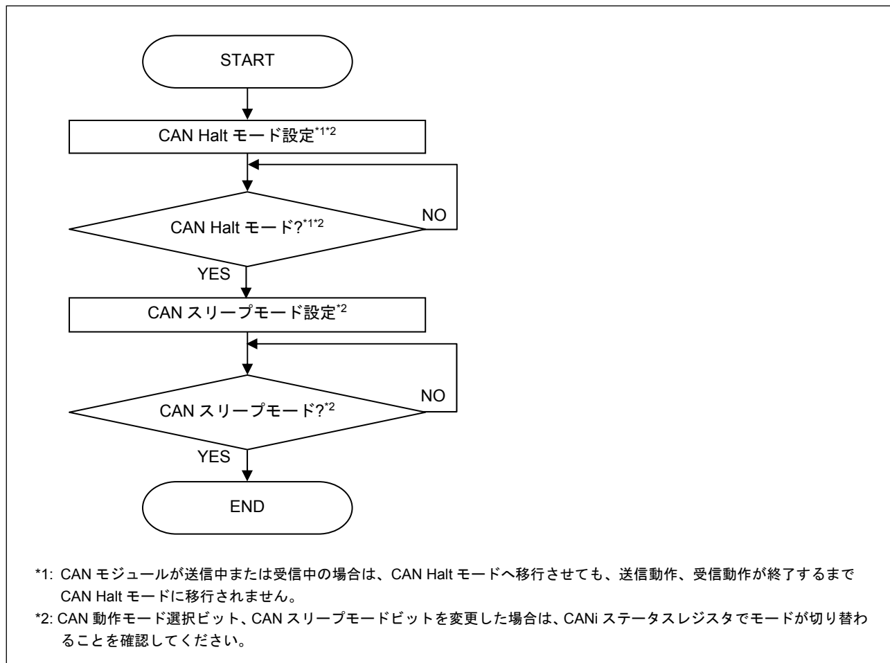
図8.2 CAN モジュールを CAN Halt モードへ移行してから CAN スリープモードへ移行させる手順
