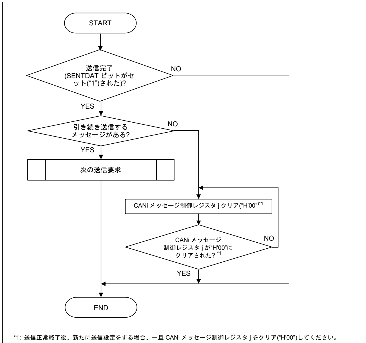
図2.5 送信完了手順
