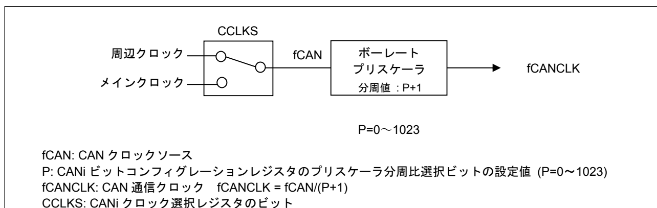
図1.3 CAN クロックの発生回路ブロック図
