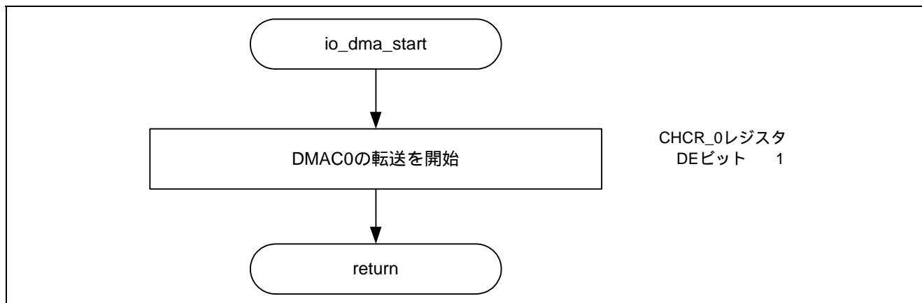
図5.6 DMA 転送の開始処理
