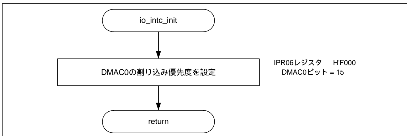
図5.4 INTC の初期設定
