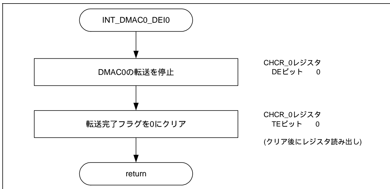
図5.7 DMA 転送完了割り込み処理
