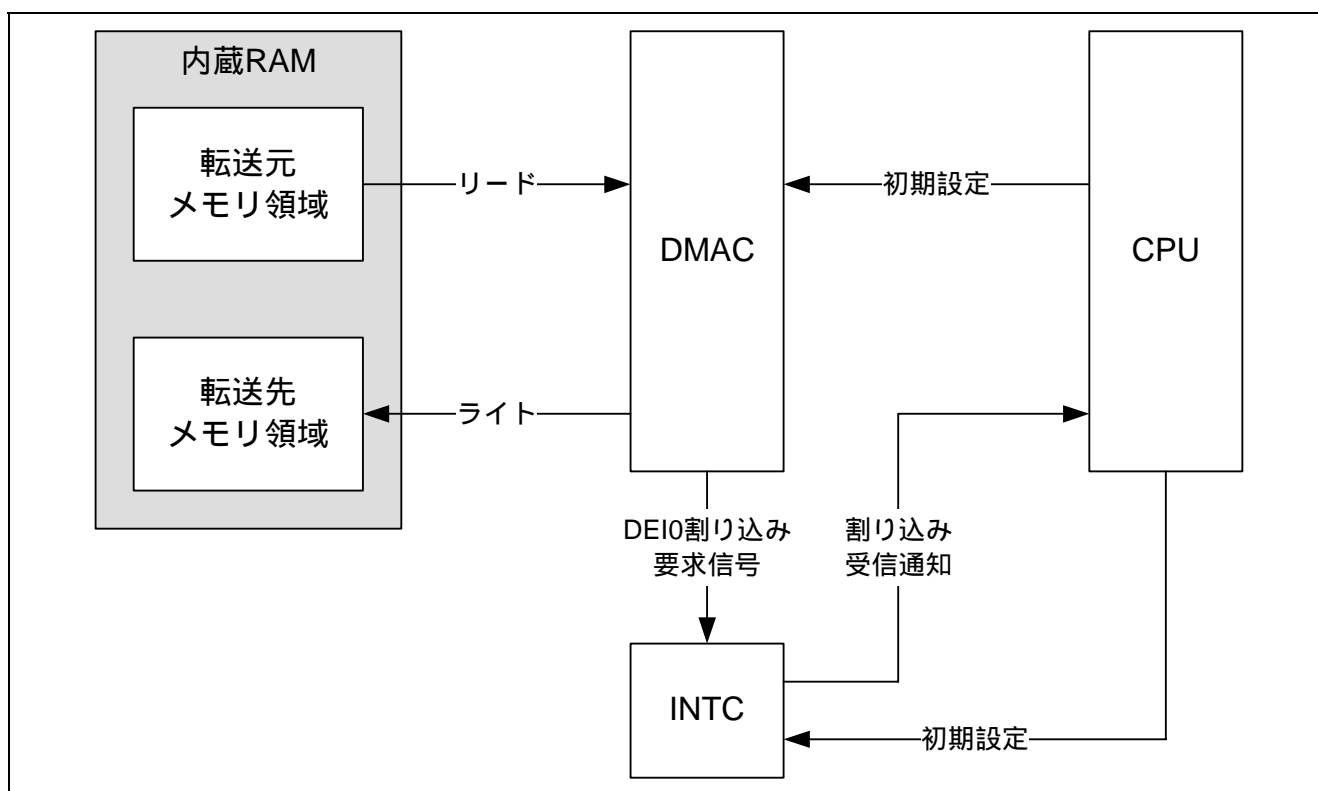
図1.1 使用する周辺機能のブロック図
