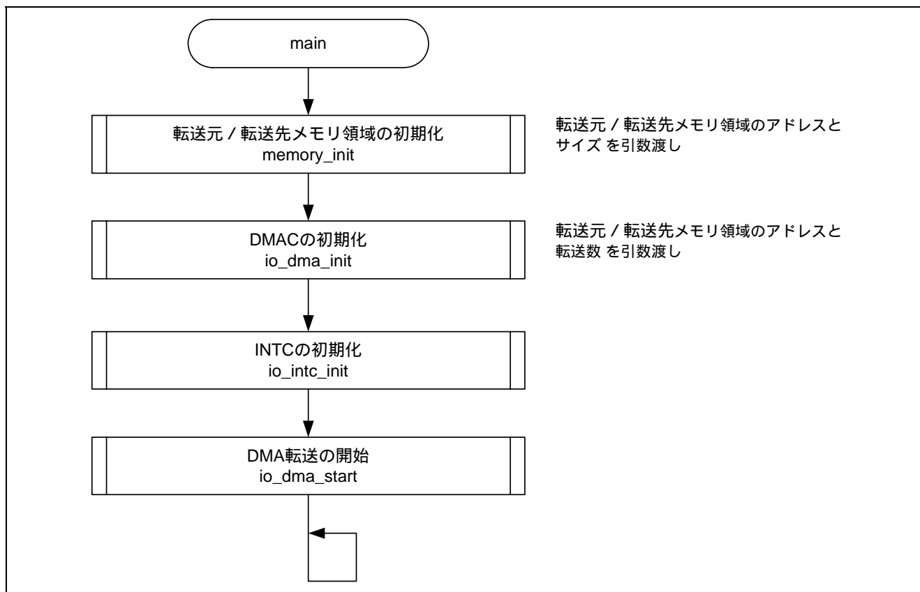
図5.2 メイン処理
