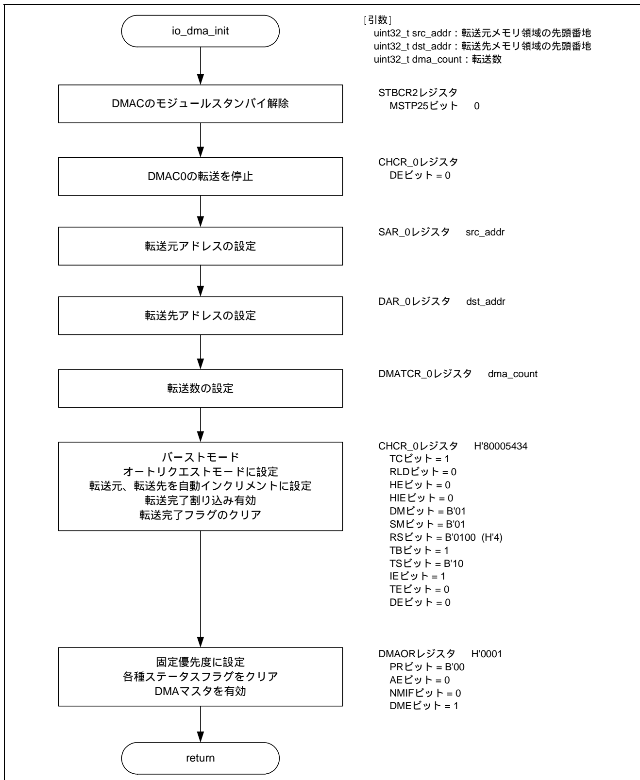
図5.5 DMAC の初期設定
