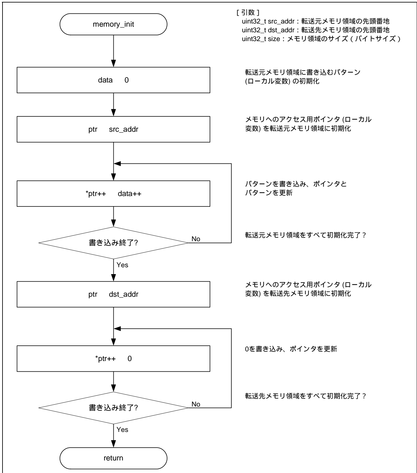
図5.3 転送元 / 転送先メモリ領域の初期化
