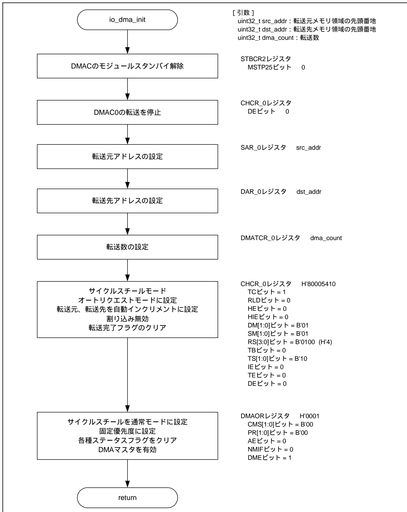
図5.4 DMAC の初期設定
