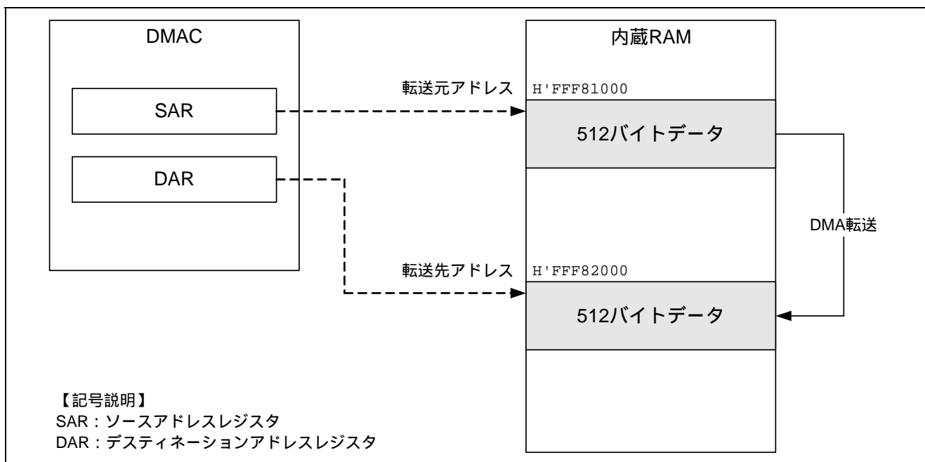
図5.1 動作イメージ
