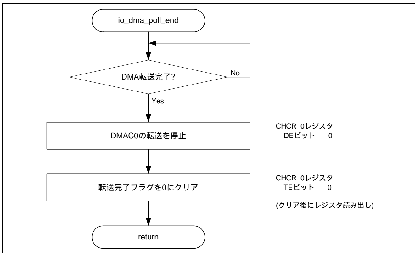
図5.6 DMA 転送の完了待ち処理
