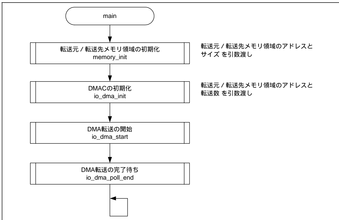
図5.2 メイン処理
