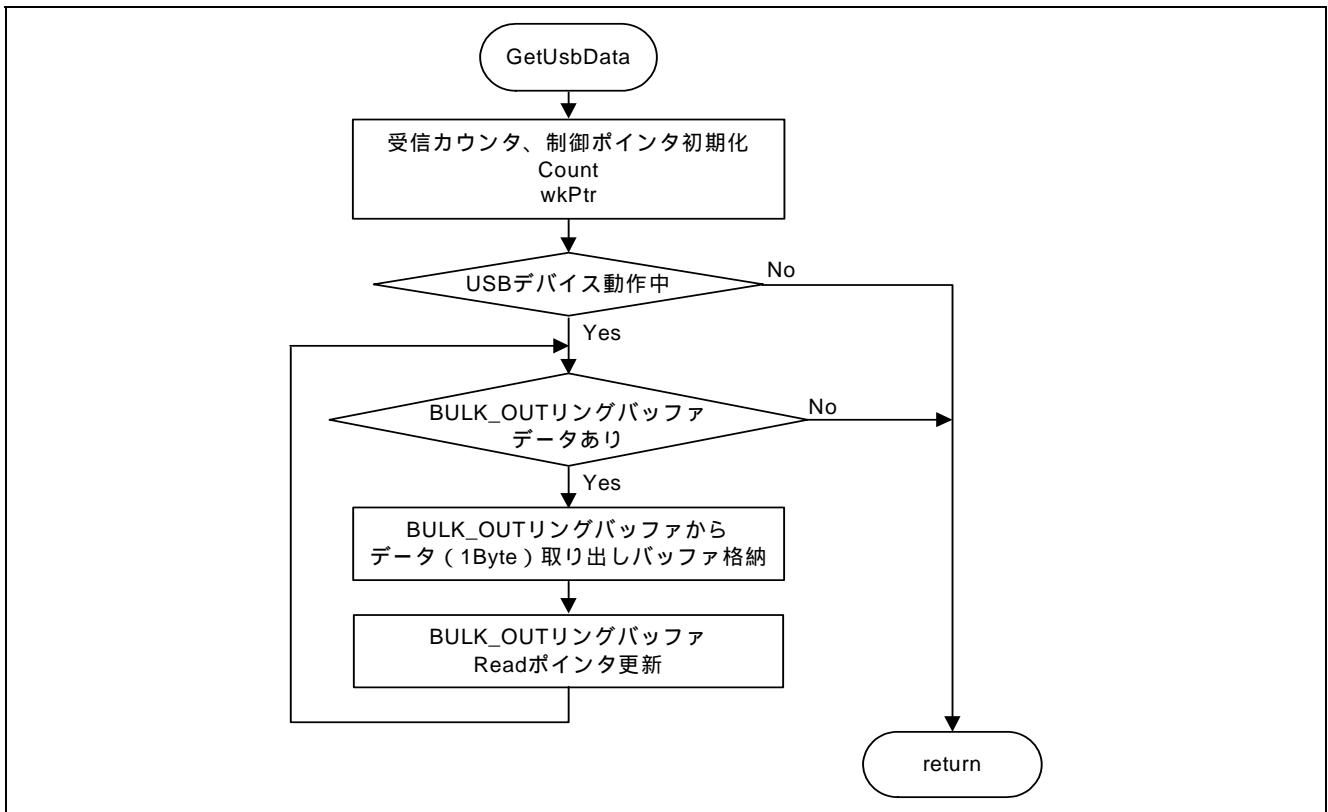
図4 USB 受信チェック処理フロー
