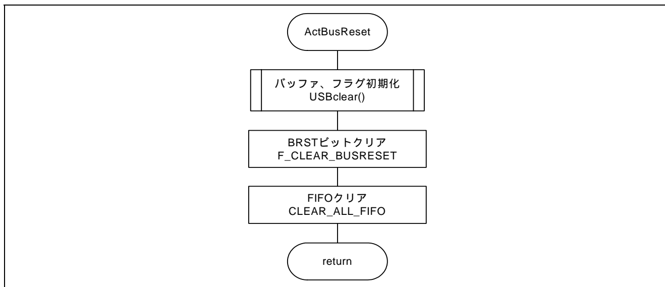
図6 ActBusReset 処理フロー
