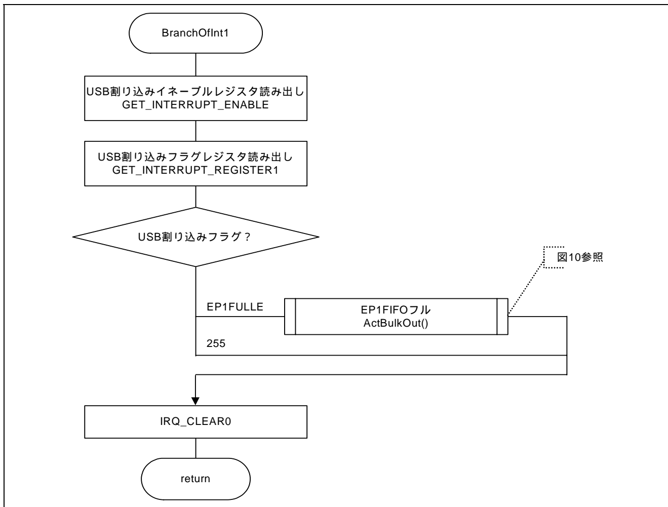
図13 BranchOfInt1 処理フロー
