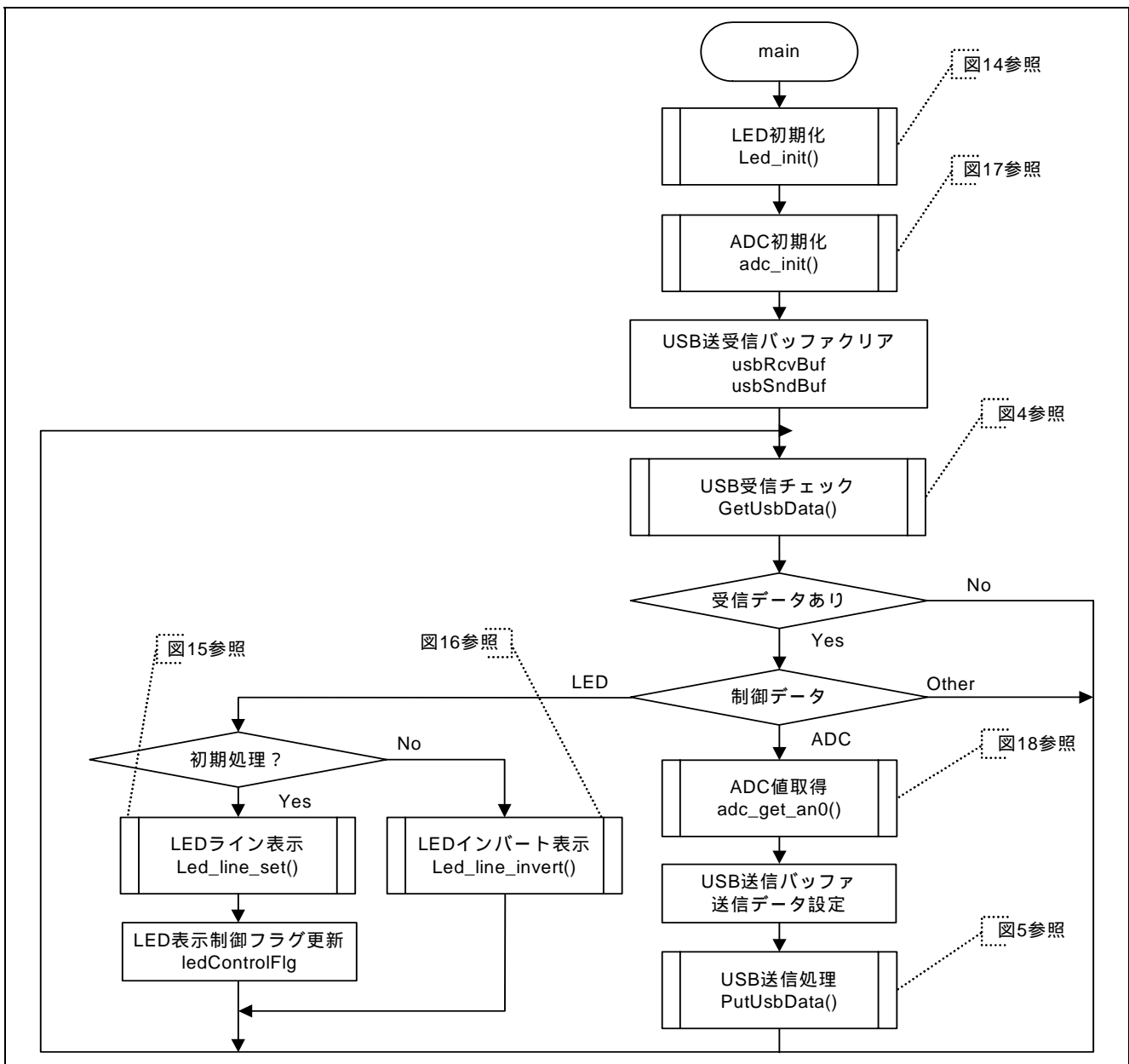
図3 メイン処理フロー
