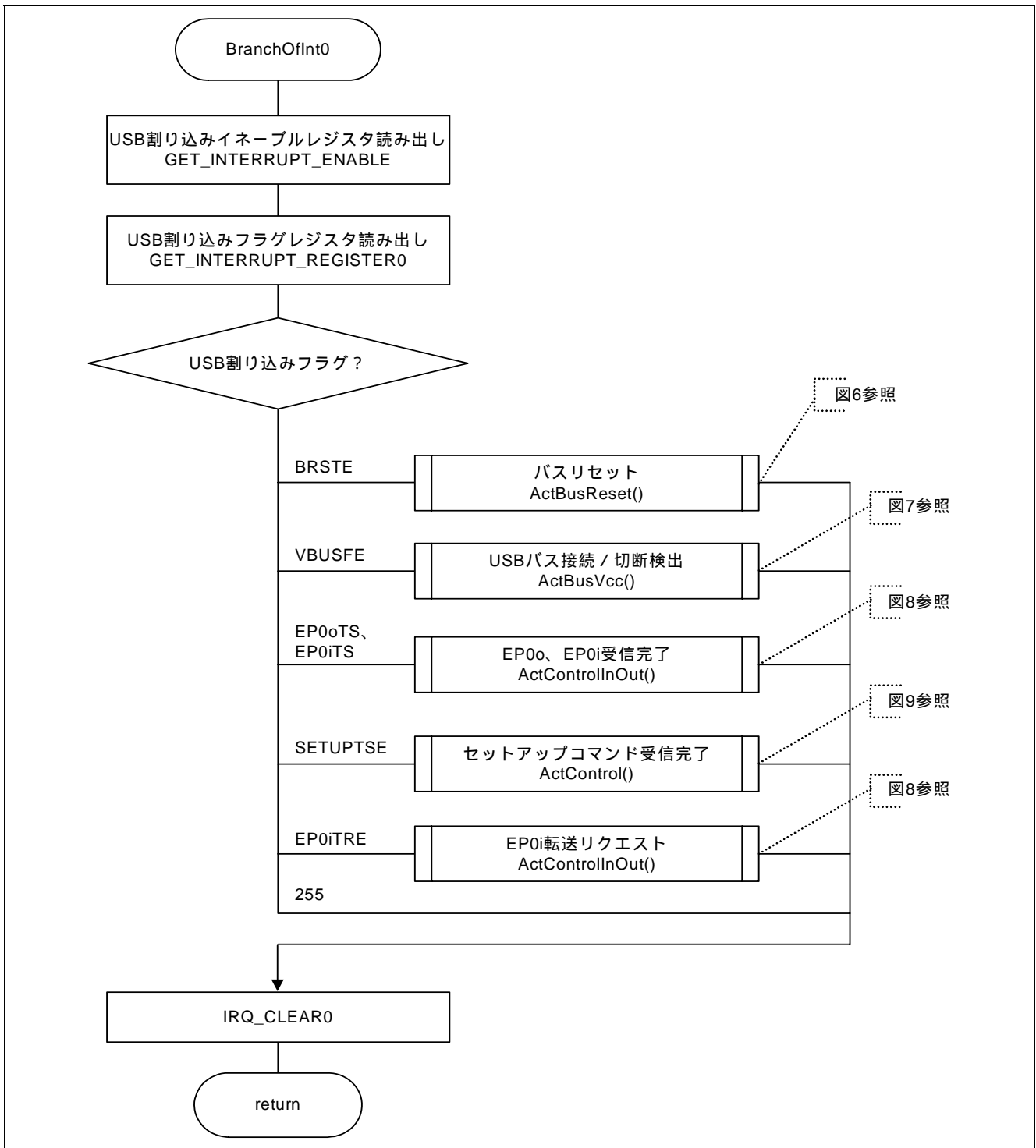
図12 BranchOfInt0 処理フロー
