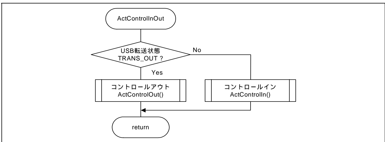
図8 ActControllnOut 処理フロー
