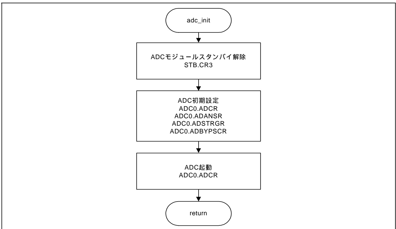
図17 adc_init 処理フロー
