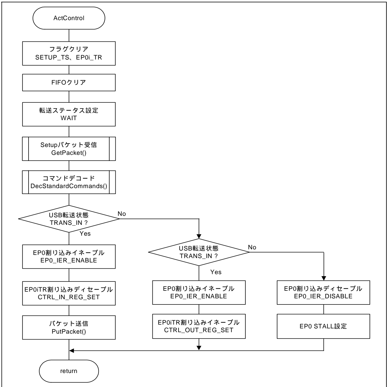
図9 ActControl 処理フロー
