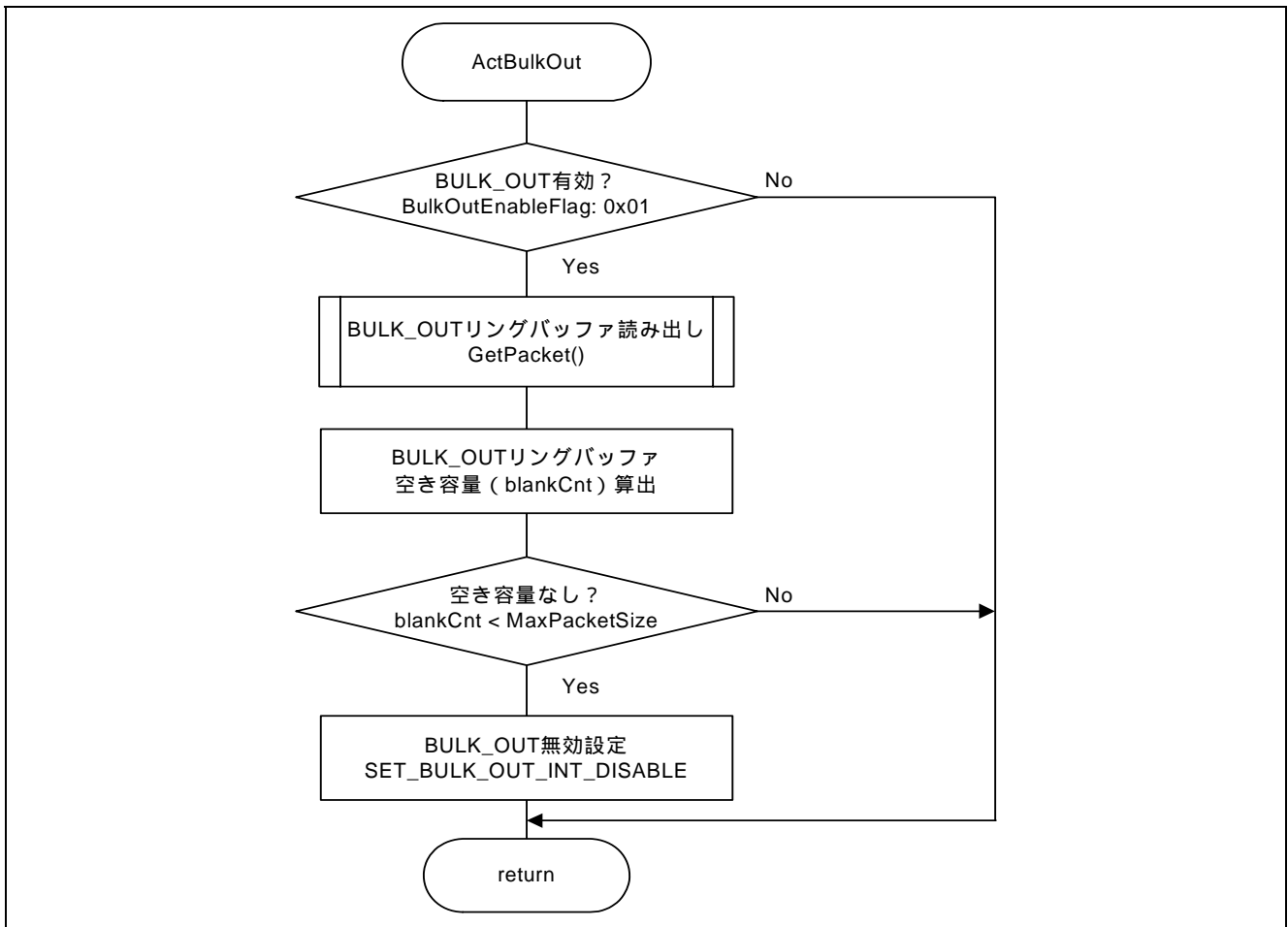
図10 ActBulkOut 処理フロー
