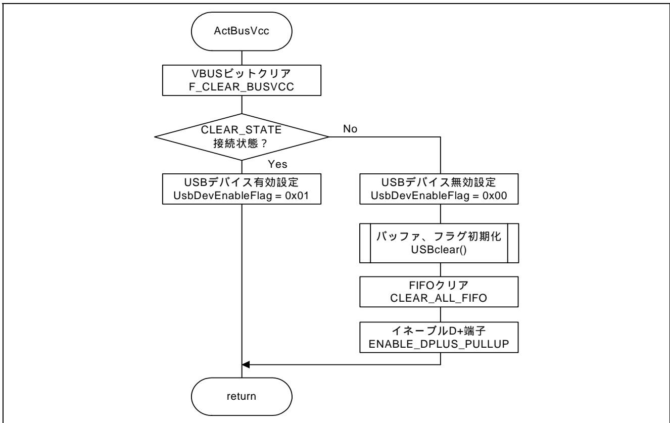
図7 ActBusVcc 処理フロー
