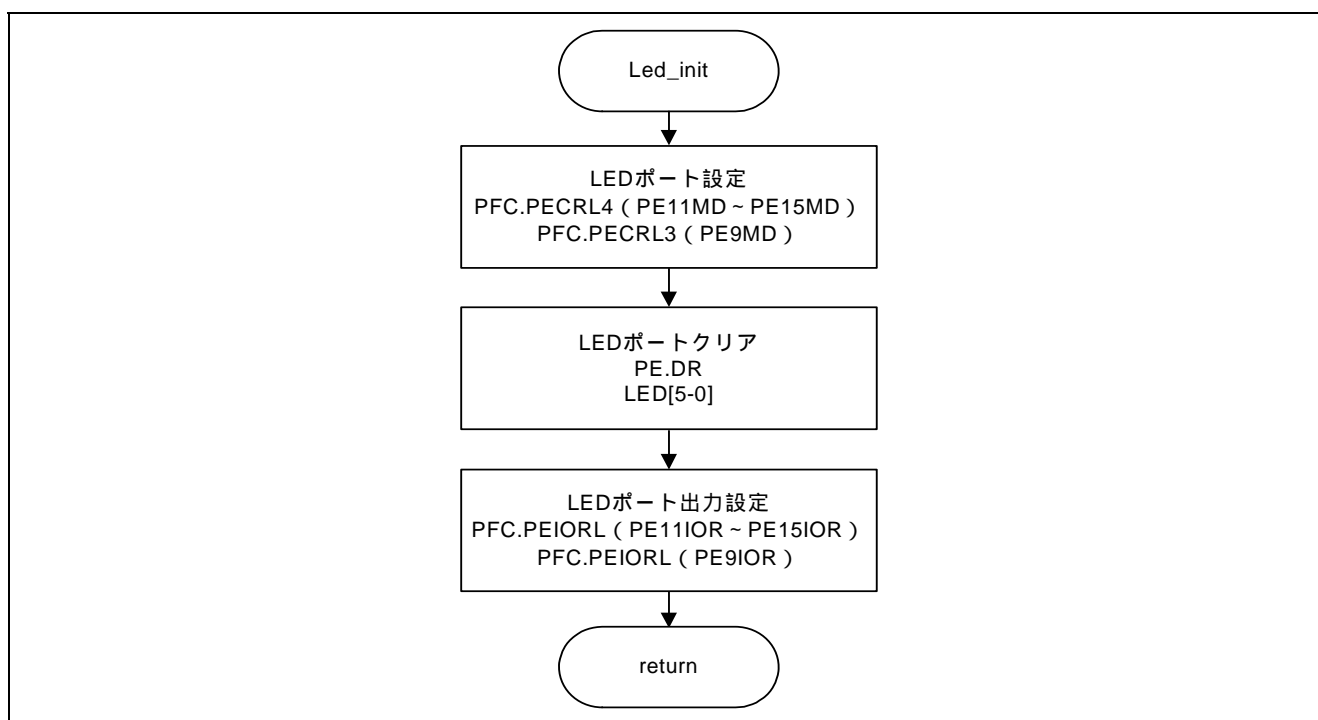
図14 Led_init 処理フロー
