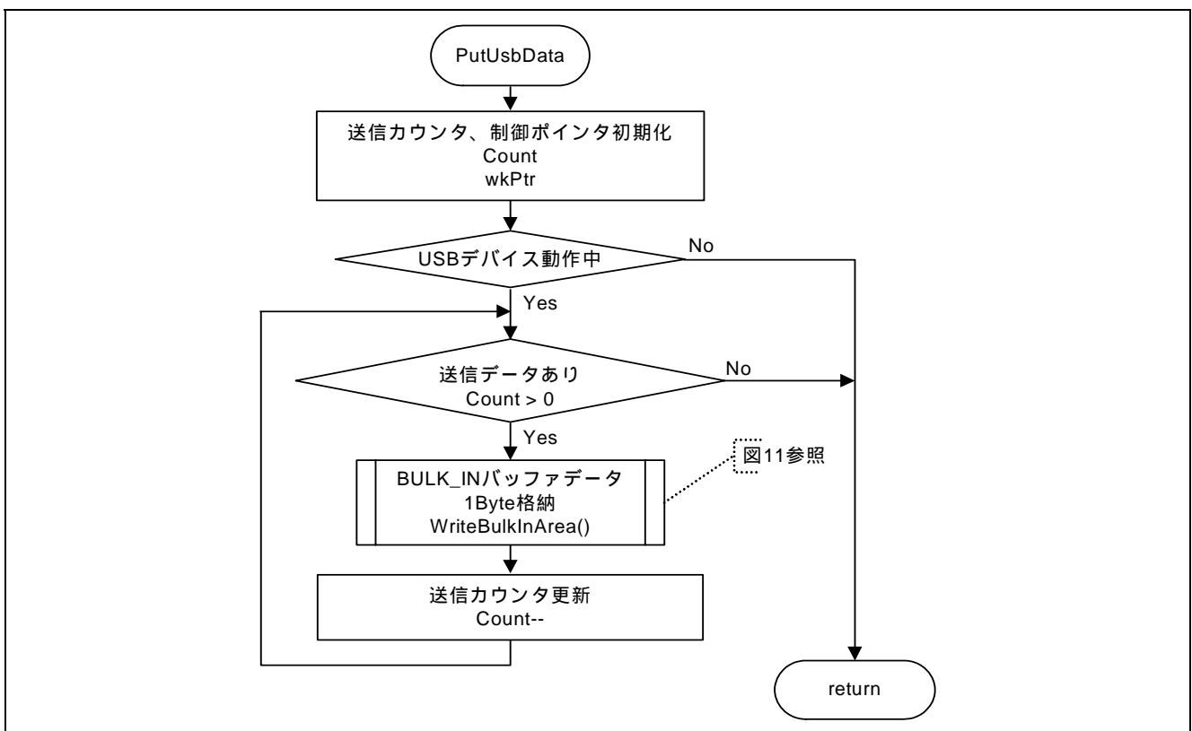
図5 USB 送信処理フロー
