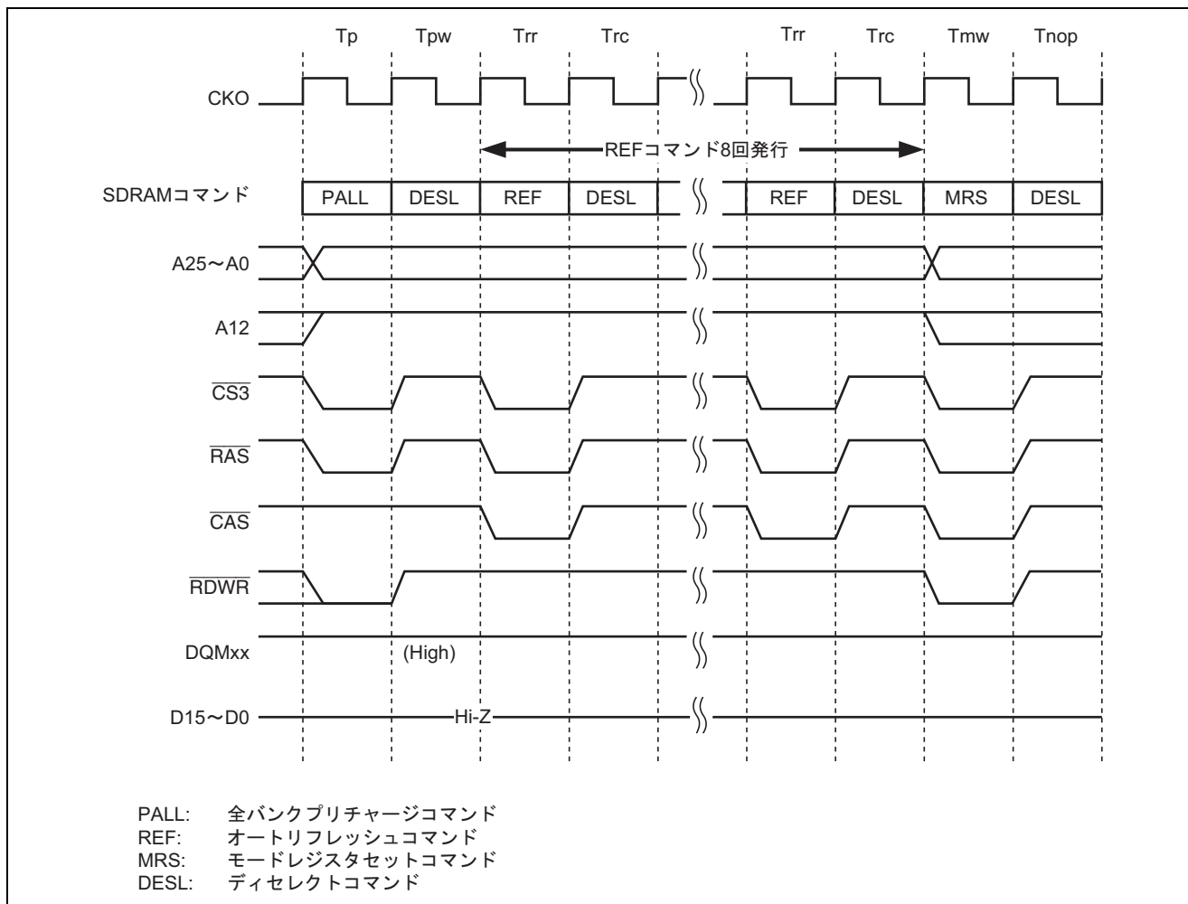
図 4 SDRAM モードレジスタ書き込みタイミング例
