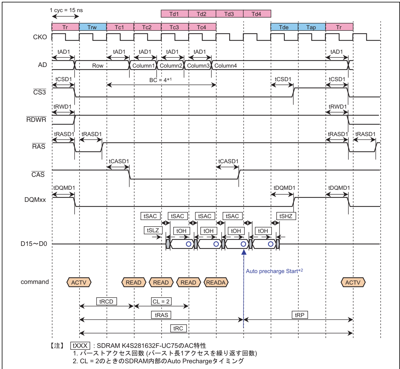
図 6 SDRAM バーストリードタイミング
