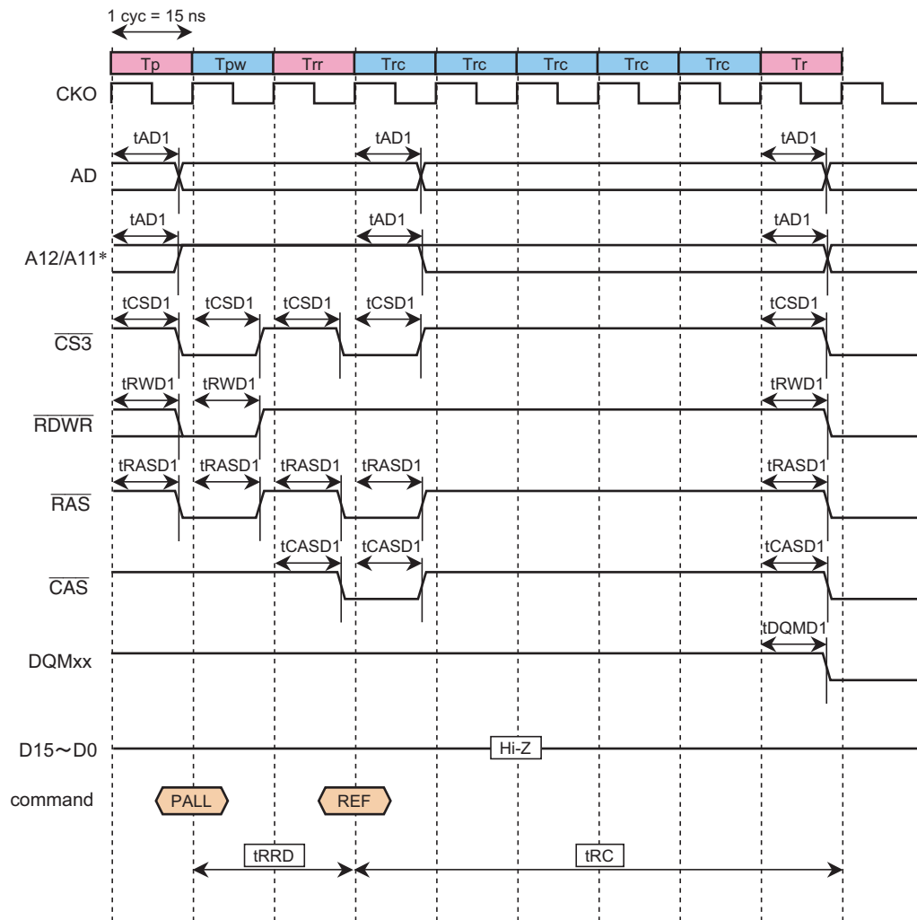
図9 SDRAM リフレッシュタイミング
