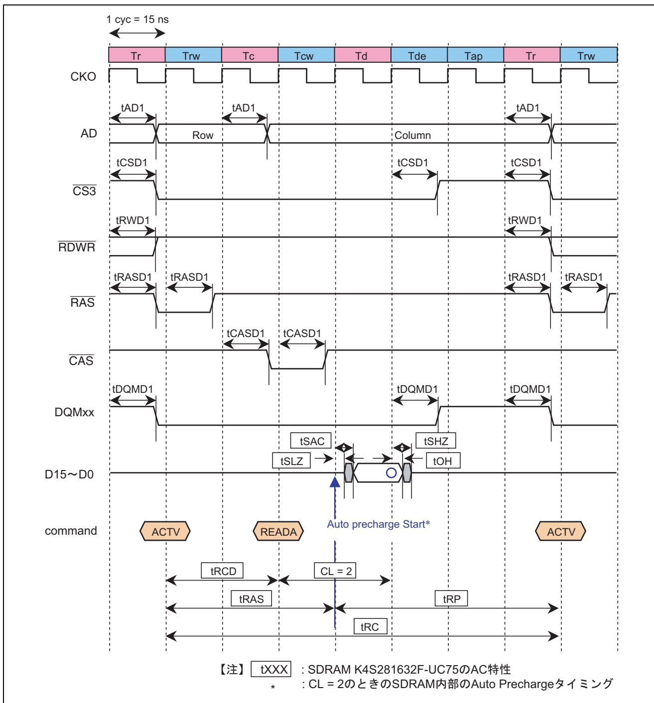
図 5 SDRAM シングルリードタイミング
