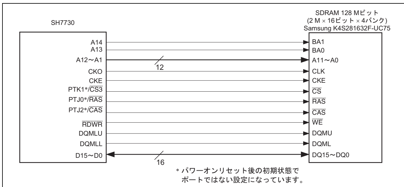
図 2 SDRAM 接続回路例 (128 M ビット × 1 個, 16 ビットバス)
