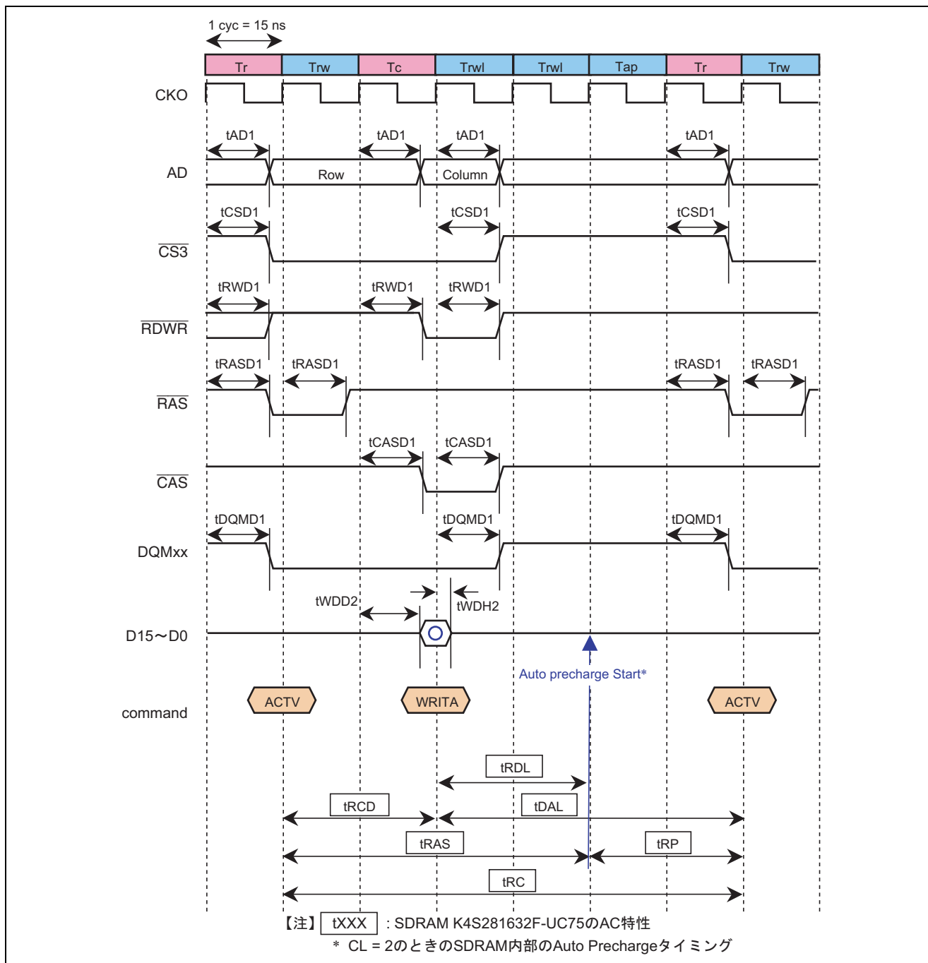
図 7 SDRAM シングルライトタイミング
