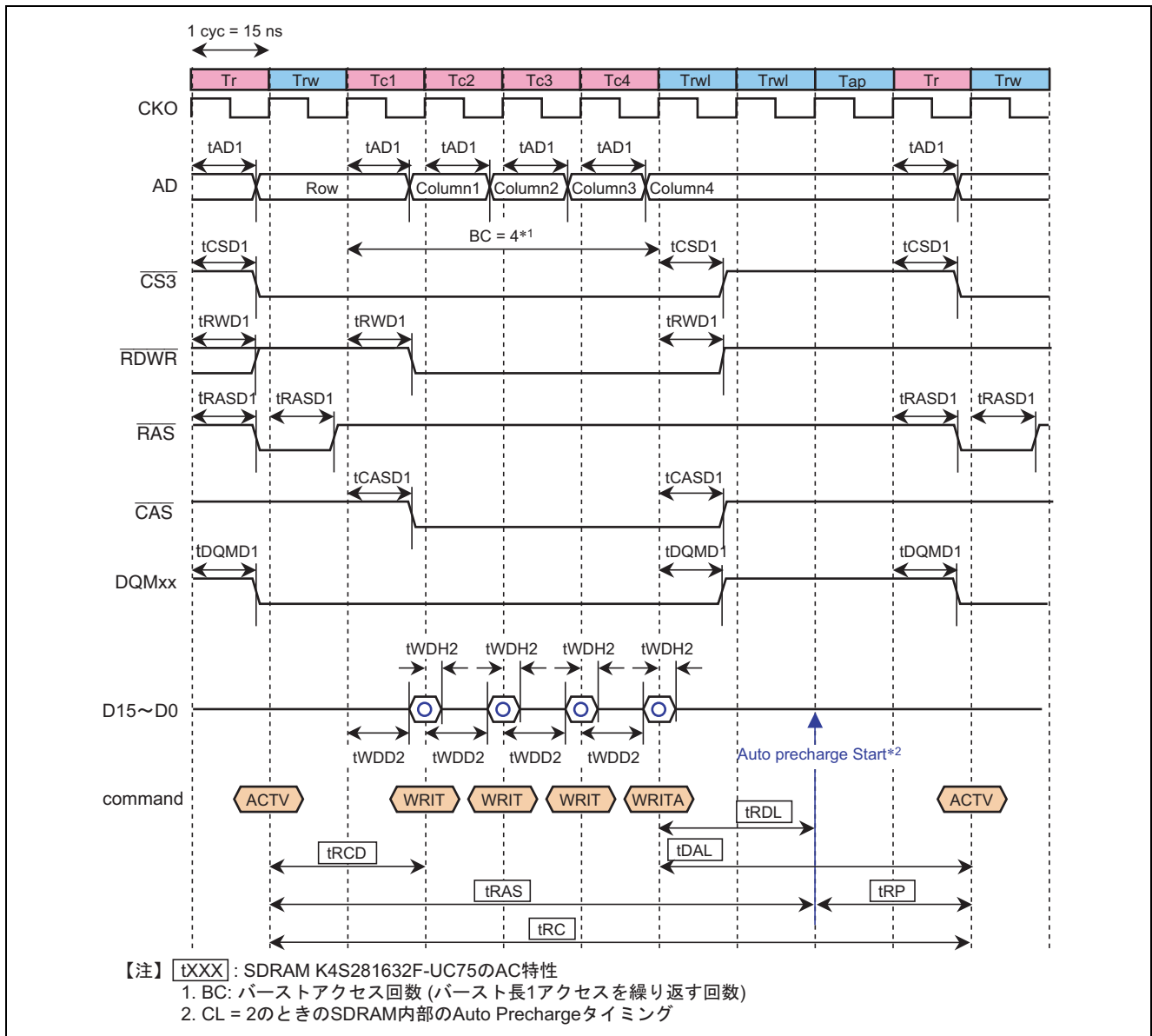
図 8 SDRAM バーストライトタイミング
