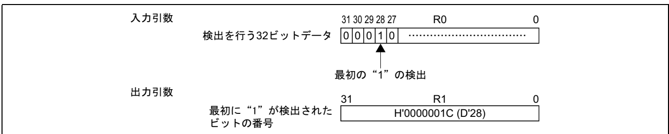
図 1 ソフトウェア FIND1 の実行例
