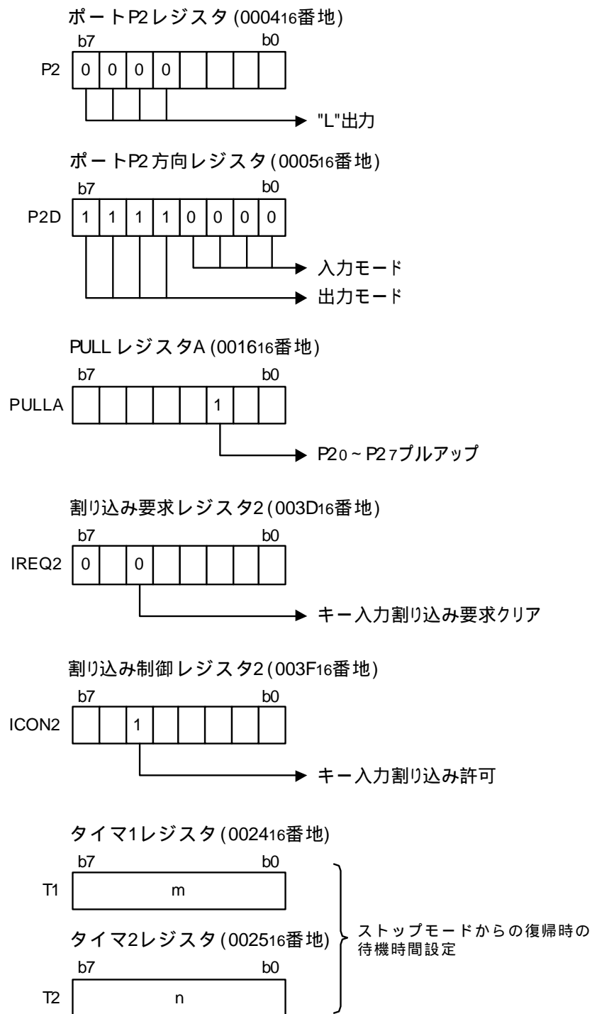
図 3.3 関連レジスタの設定
