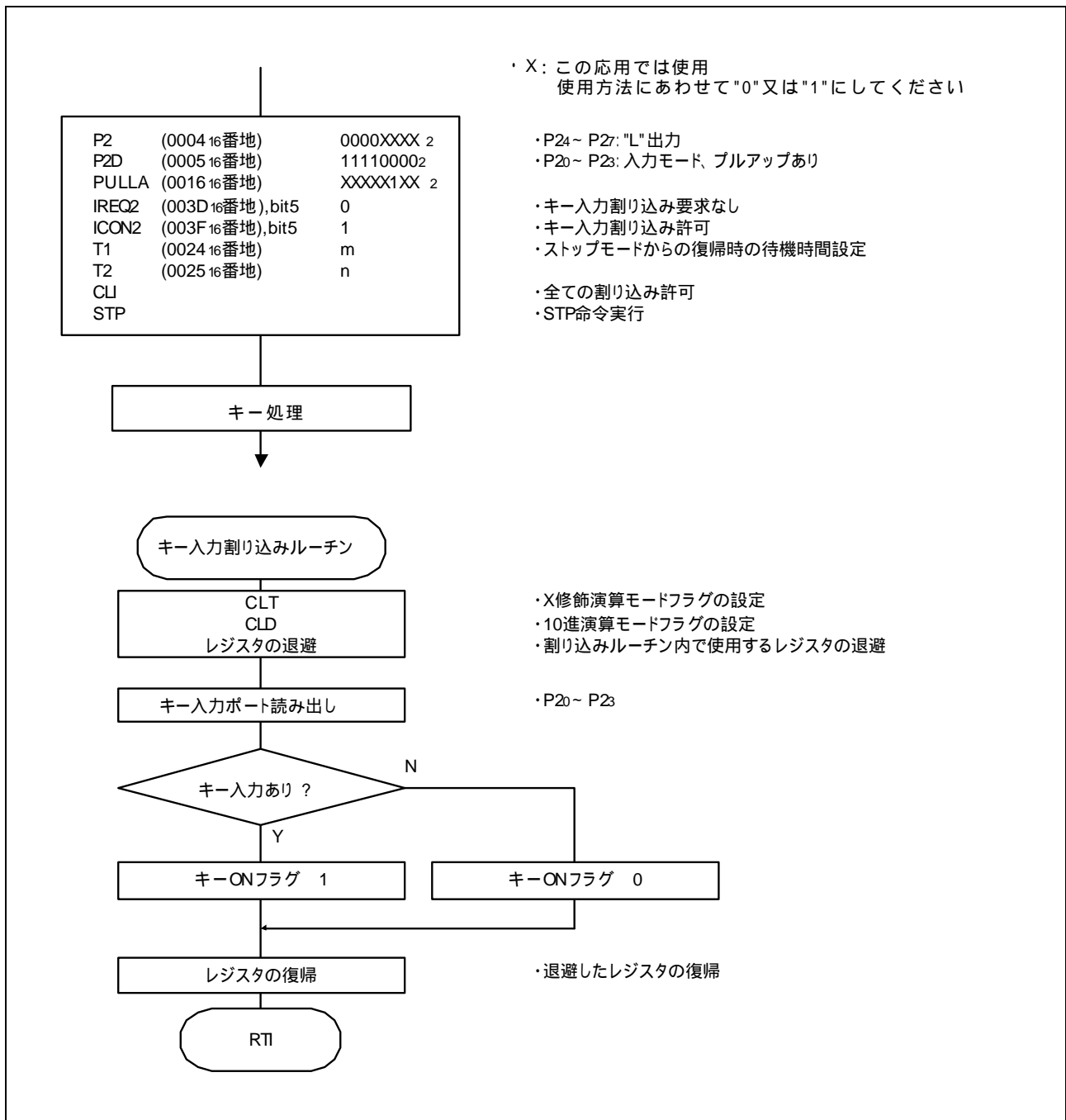
図 3.4 制御手順
