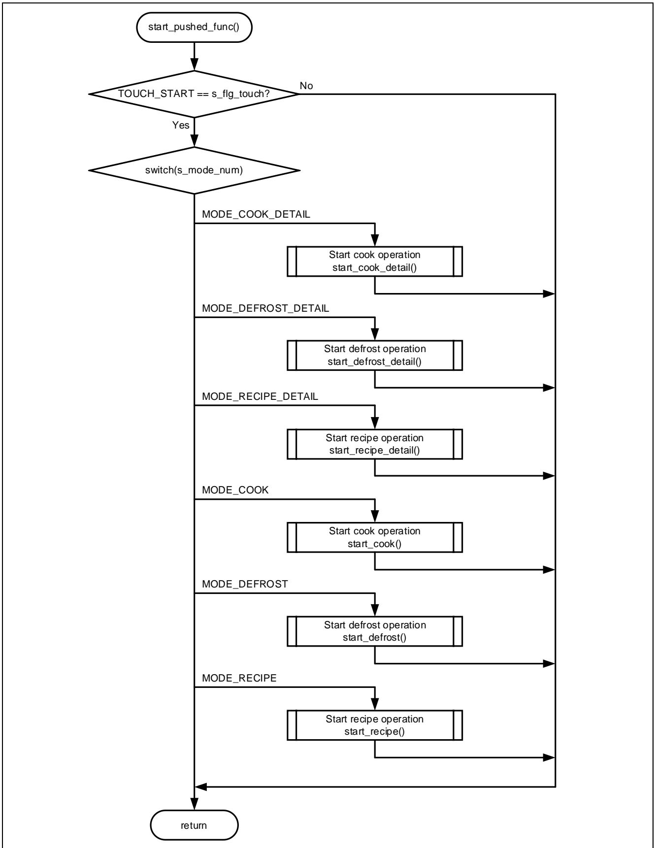
図 4-11 「2」 ボタンタッチ時のフローチャート
