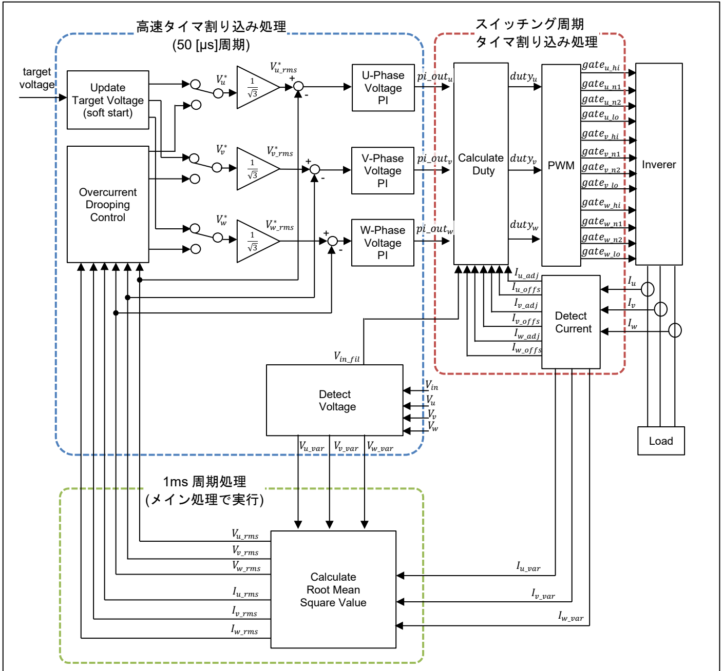
図 3-9 2 レベル及び 3 レベルインバータ制御概略ブロック図
