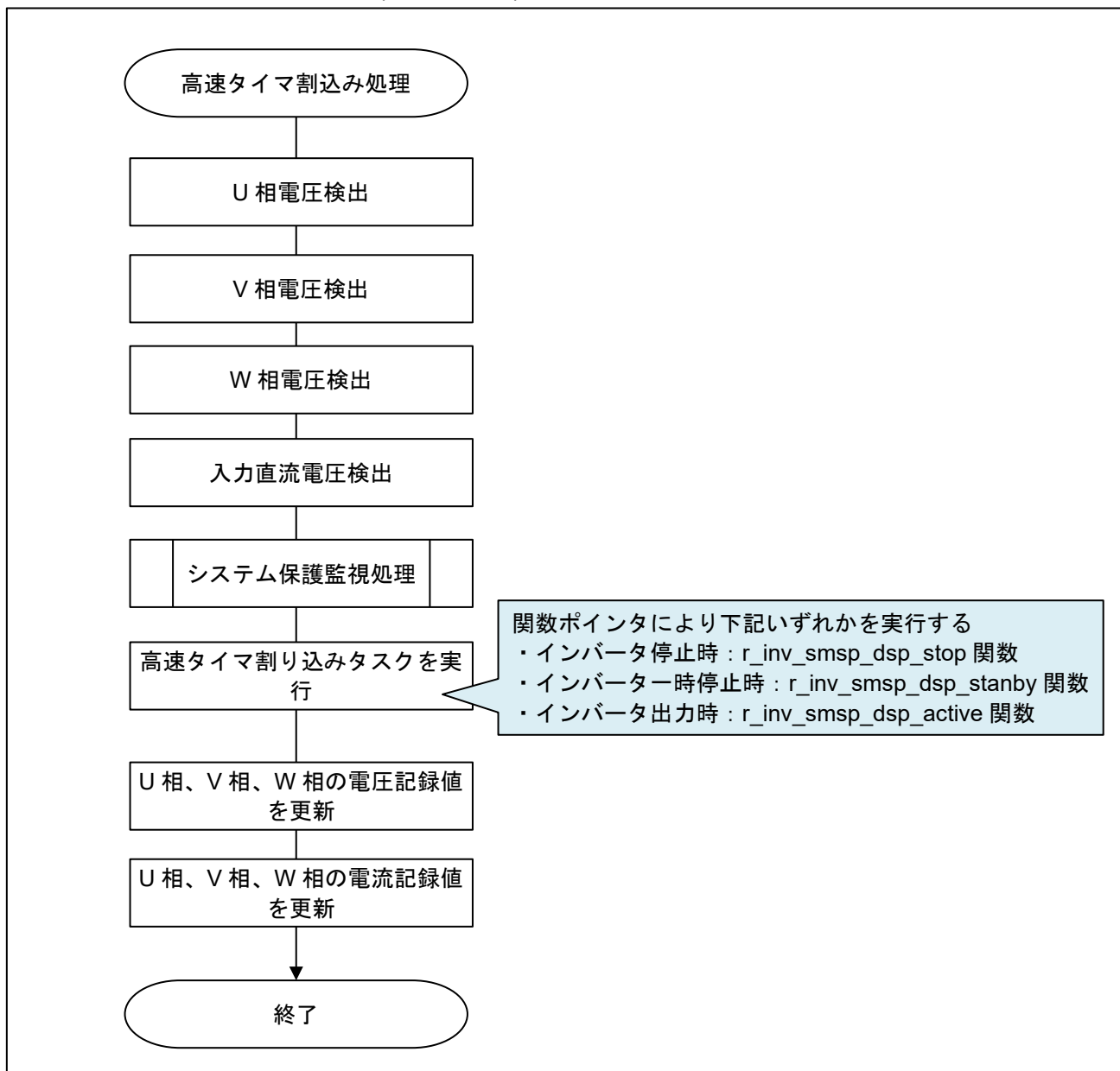
図 3-12 高速タイマ割り込み処理フローチャート
