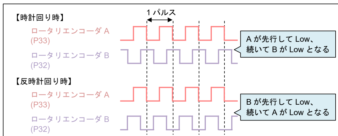
図 3-1 運転中キャリア周波数エンコーダの出力信号
