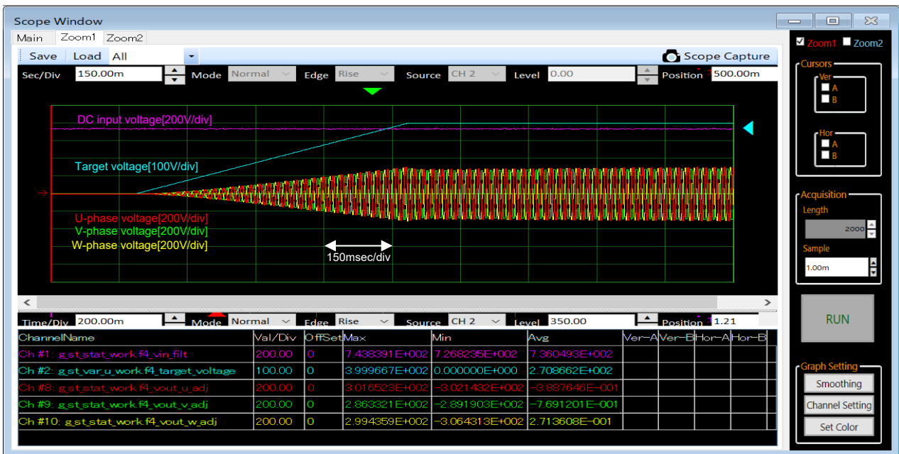
図 5-3 3 レベル動作モード/20kHz 時の起動波形
