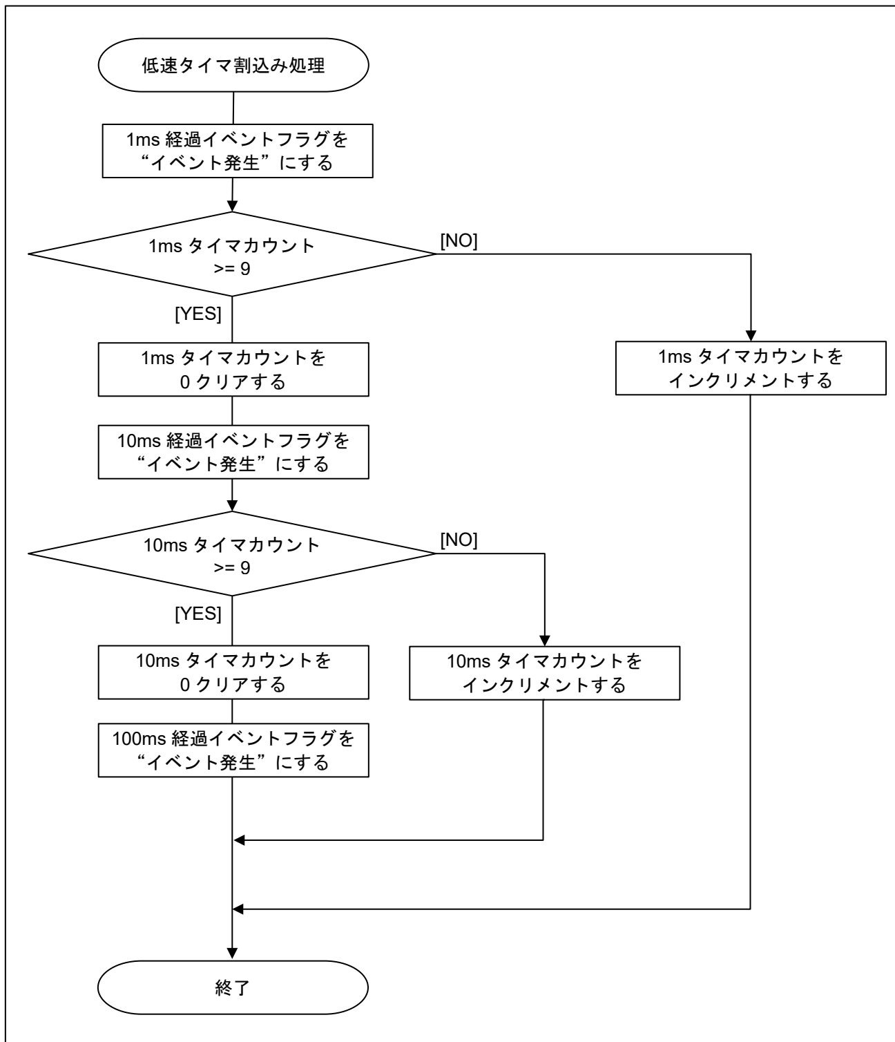
図 3-11 低速タイマ割り込み処理フローチャート
