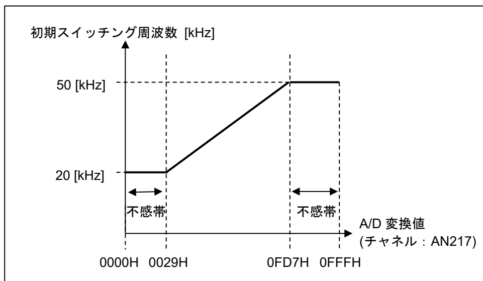
図 3-2 初期スイッチング周波数と A/D 変換値の関係
