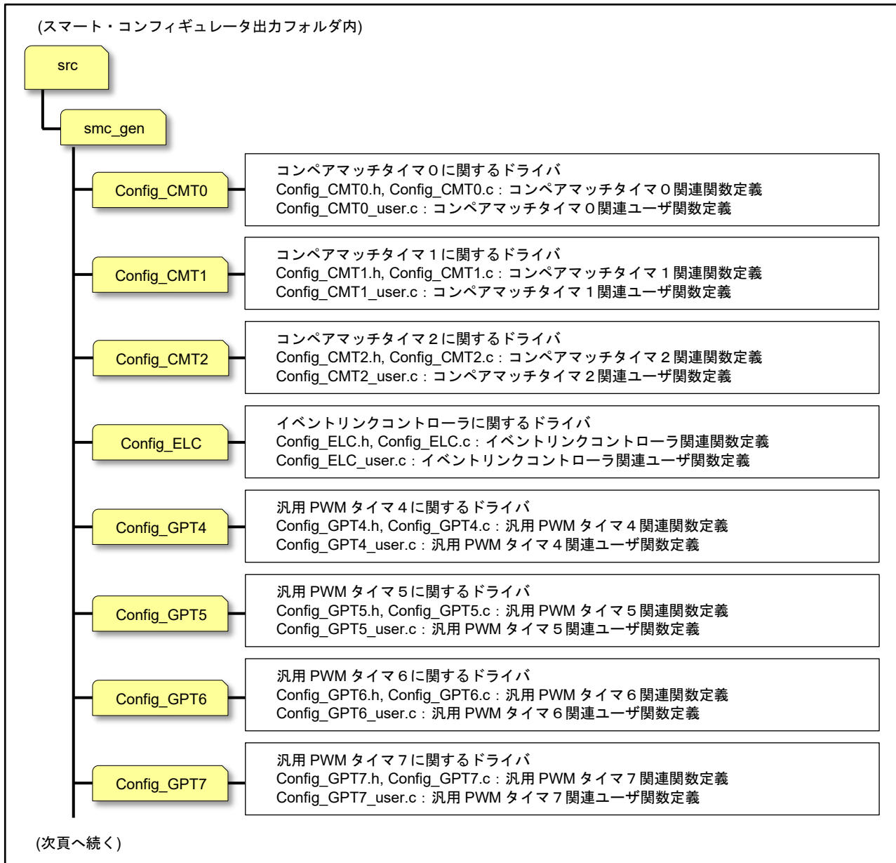
図 2-4 スマート・コンフィグレータのフォルダ・ファイル構成 (1/2)
