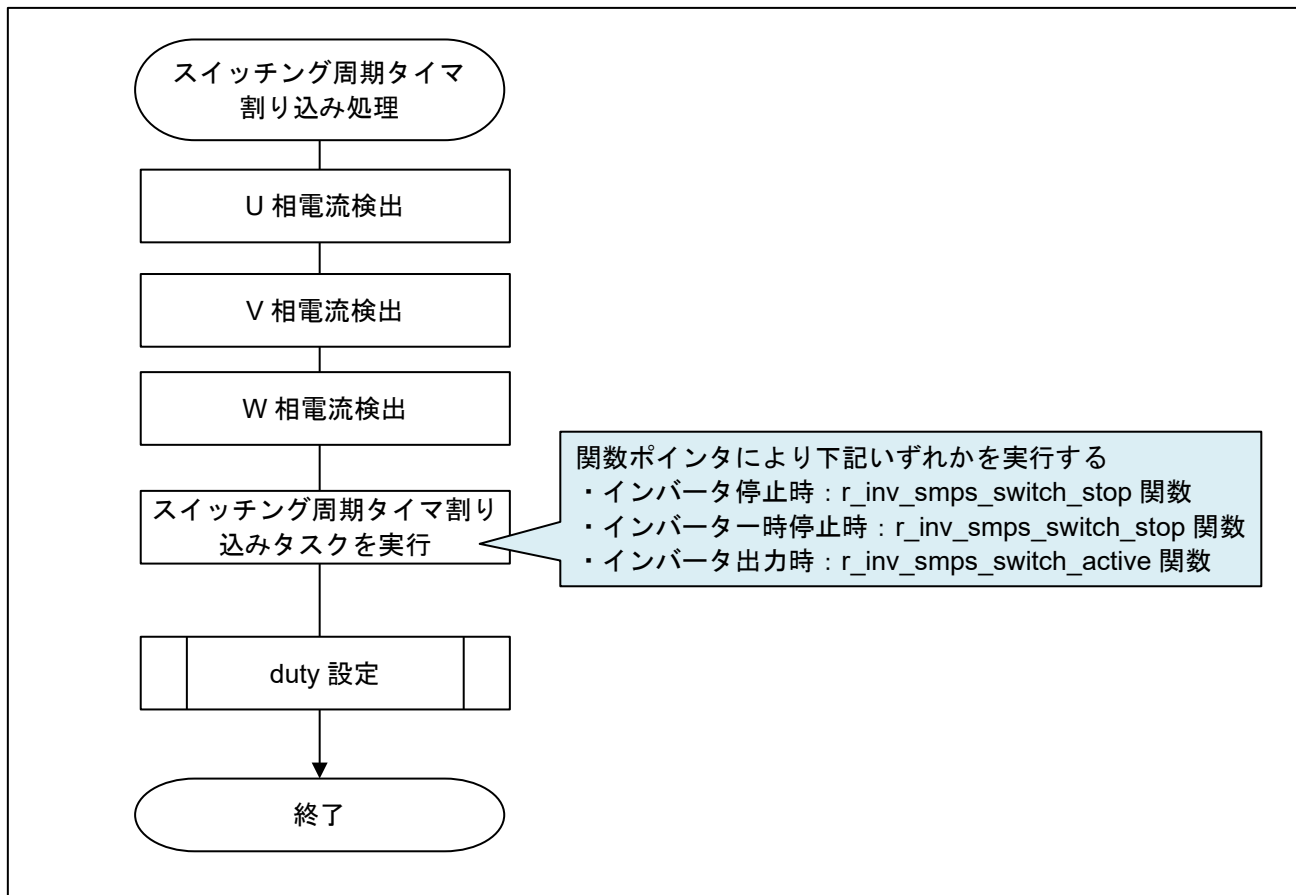
図 3-13 スイッチング周期タイマ割り込み処理フローチャート
