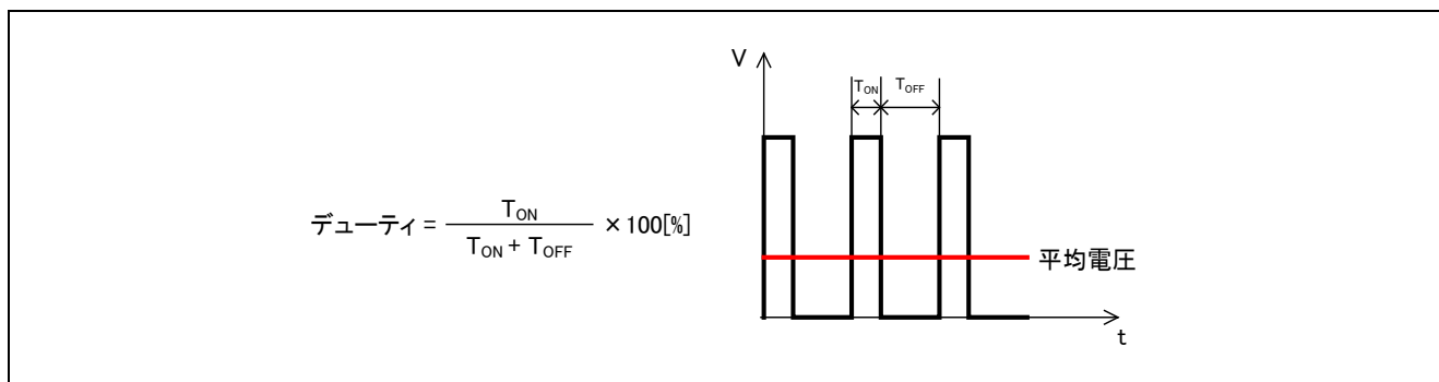
図 3-3 デューティの定義
