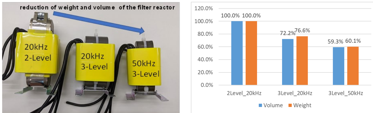
図 5-8 リアクトルサイズと重量の比較
