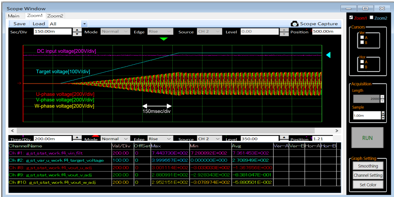
図 5-5 3 レベル動作モード/50kHz 時の起動波形
