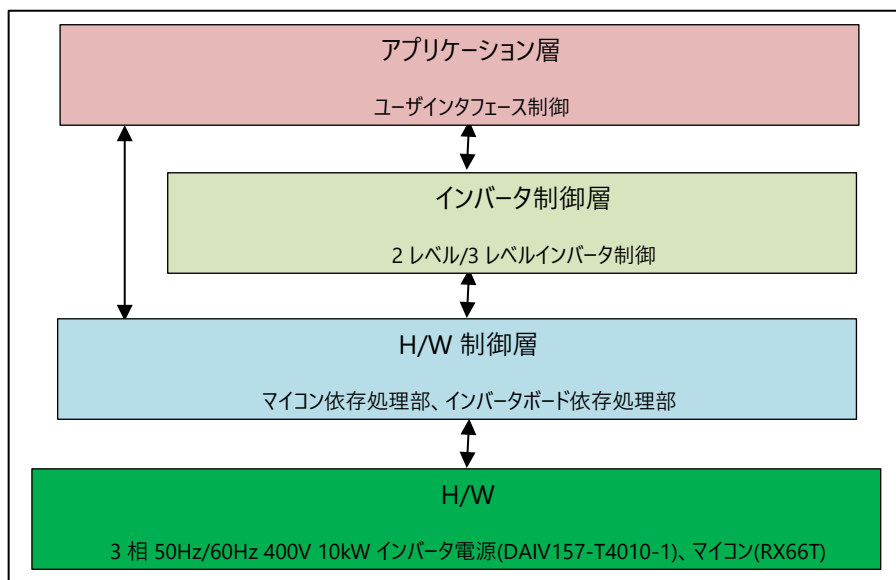
図 2-5 モジュール構成
