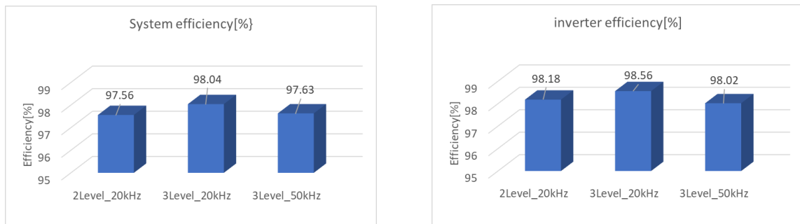
図 5-7 2 レベル及び 3 レベル動作モードにおける効率比較
