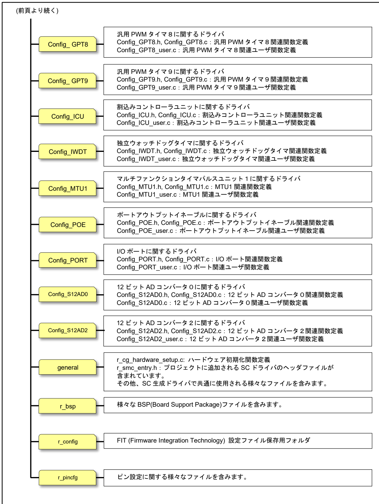
図 2-4 スマート・コンフィグレータのフォルダ・ファイル構成 (2/2)
