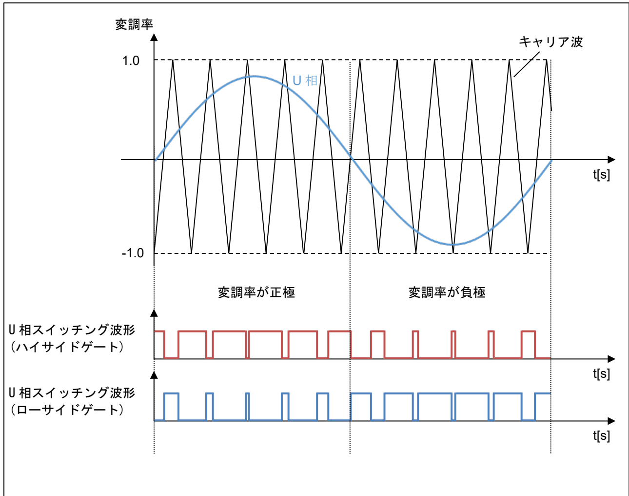
図 3-4 PWM 波形生成の概念図 (2 レベル動作)
