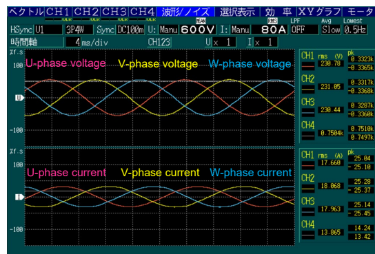
(b) 出力相電圧/相電流波形
