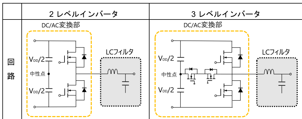
図 2-1 2 レベルインバータと 3 レベルインバータの回路比較
