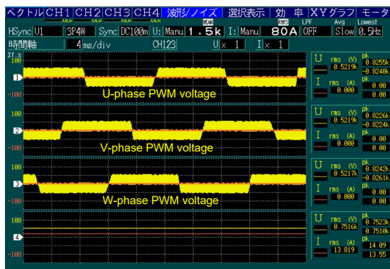
(a)PWM 出力波形
