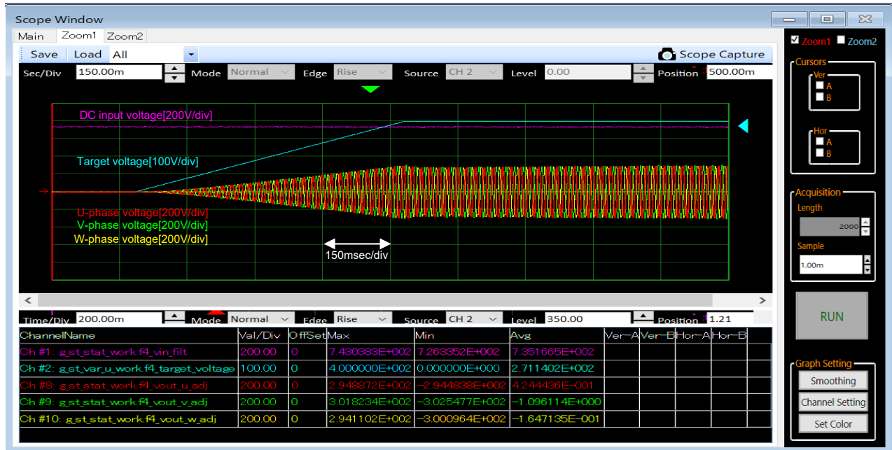
図 5-1 2 レベル動作モード/20kHz 時の起動波形
