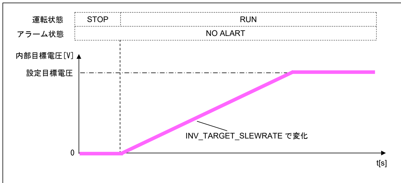
図 3-8 インバータ出力のソフトスタート内容
