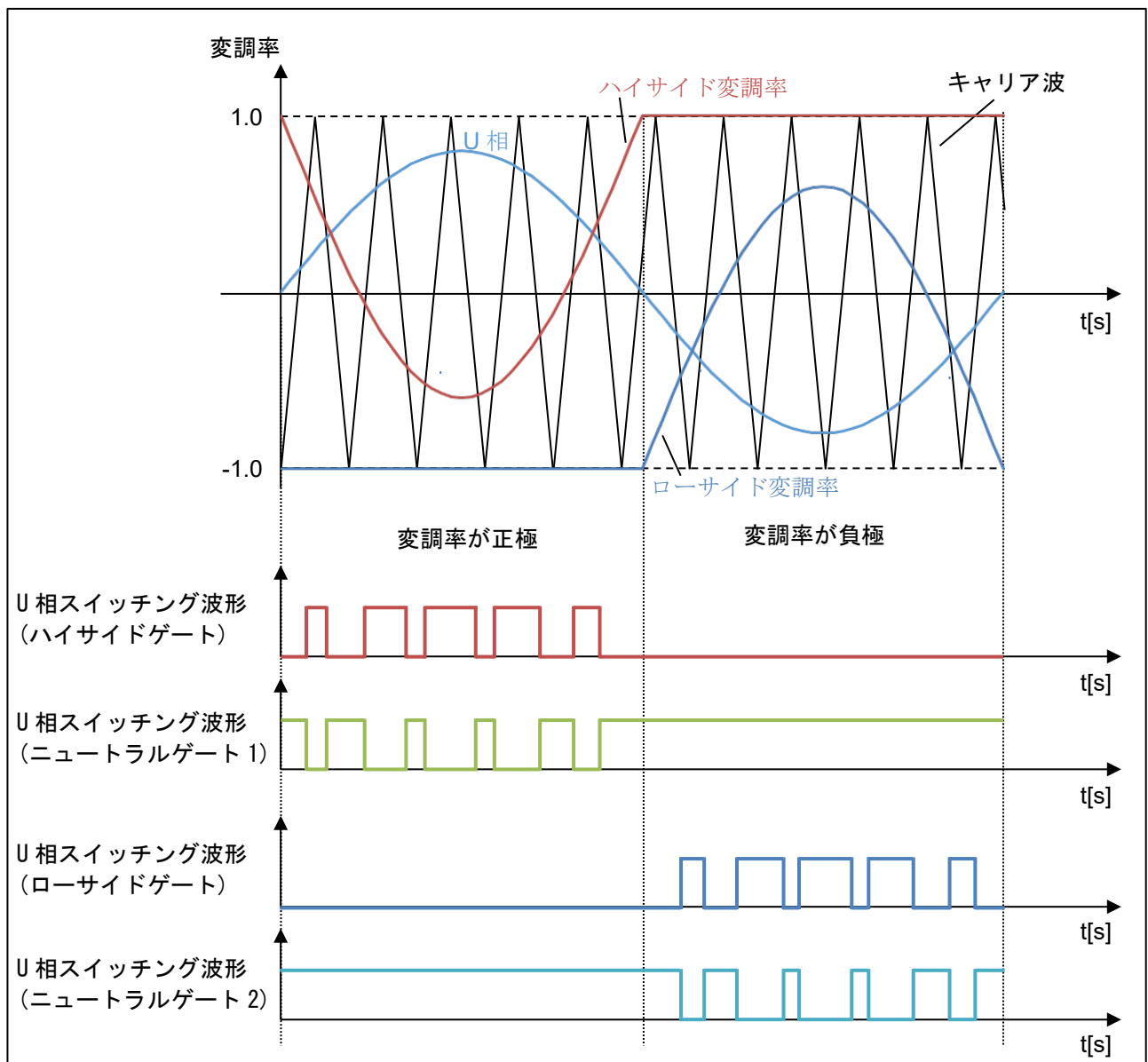
図 3-5 PWM 波形生成の概念図 (3 レベル動作)
