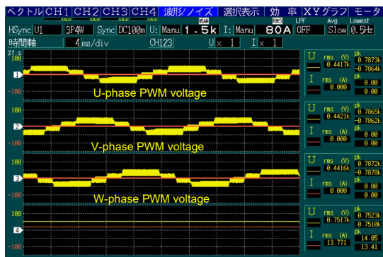
(a)PWM 出力波形
