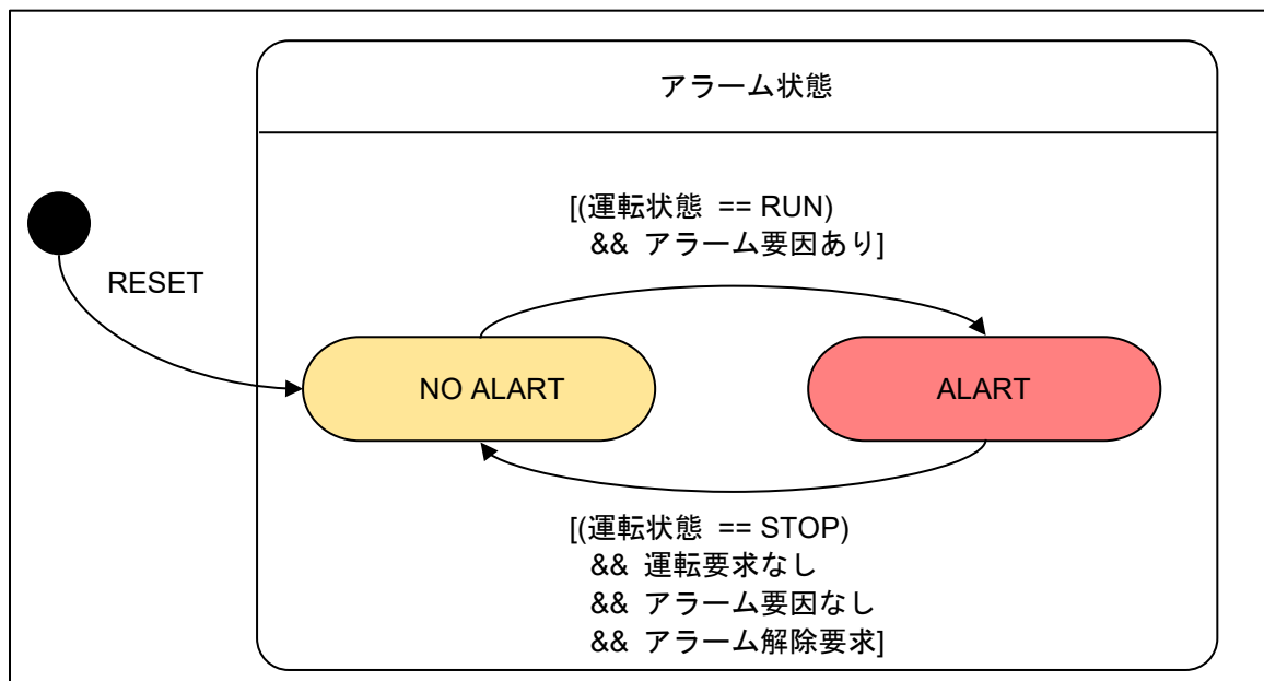
図 3-7 アラーム状態の状態遷移図
