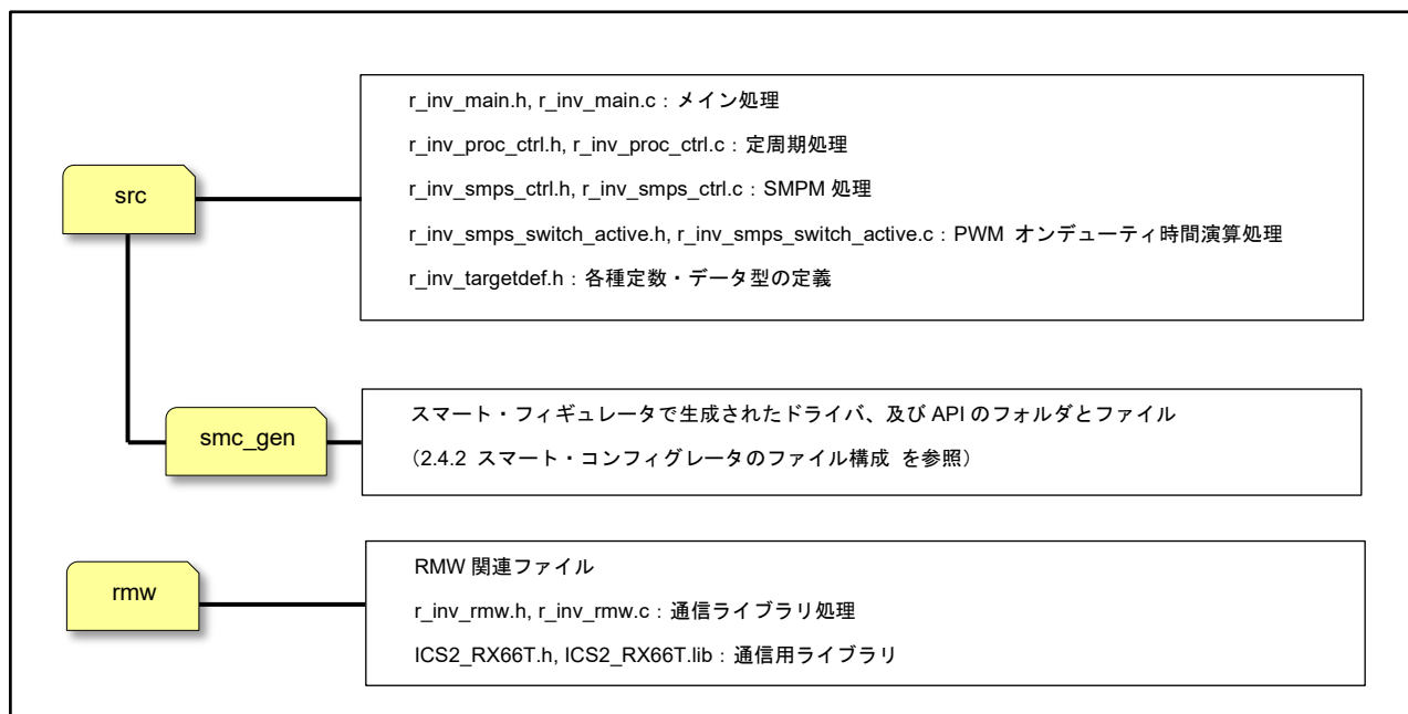
図 2-3 フォルダ・ファイル構成
