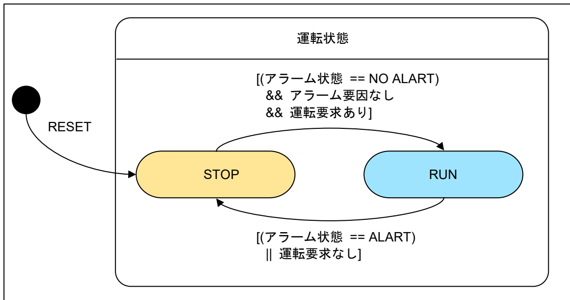
図 3-6 運転状態の状態遷移図
