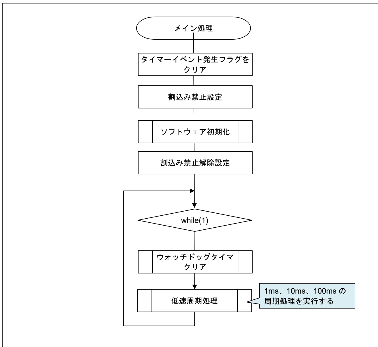
図 3-10 メイン処理フローチャート
