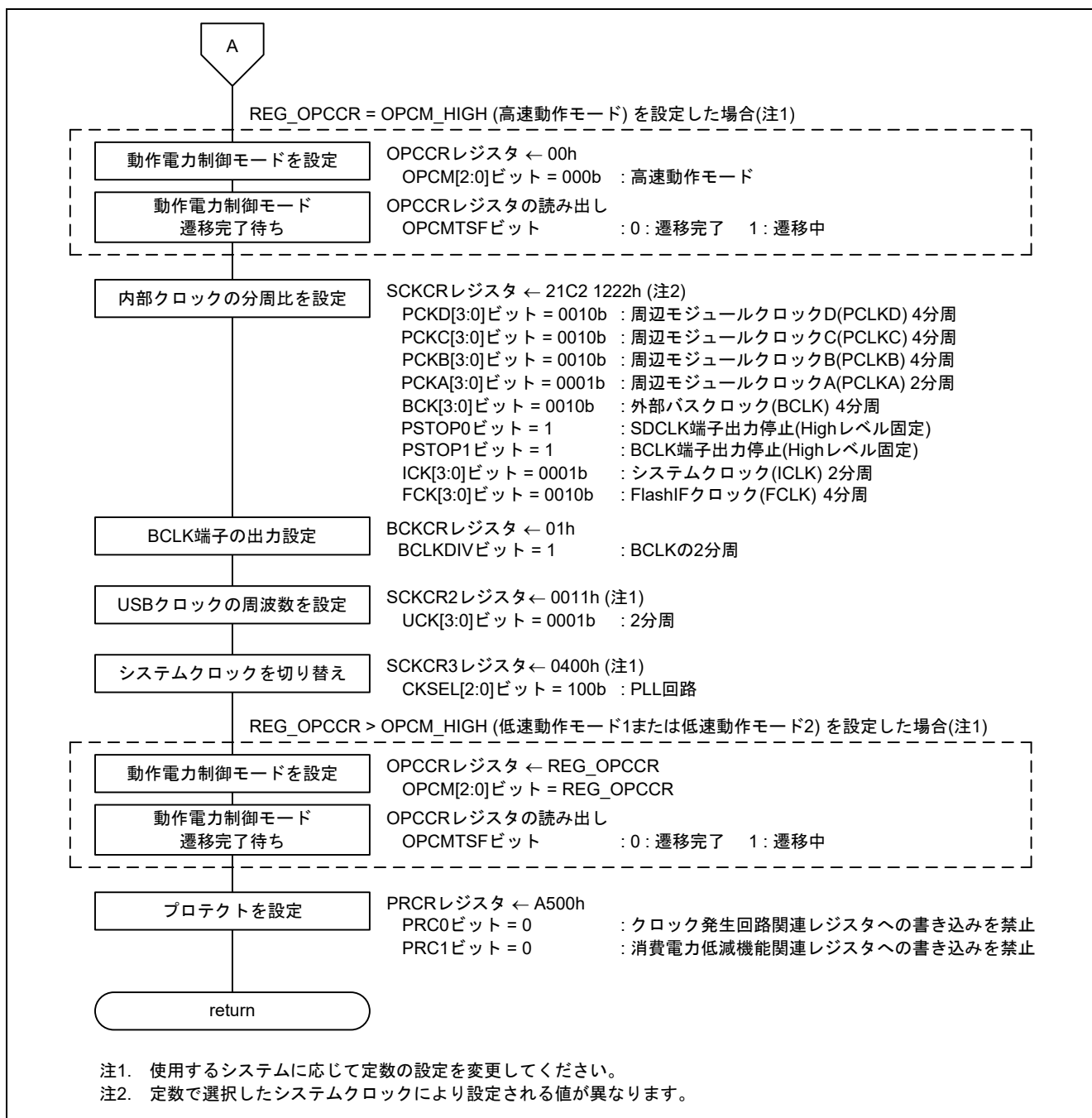
図 3.5 クロック初期設定(2/2)
