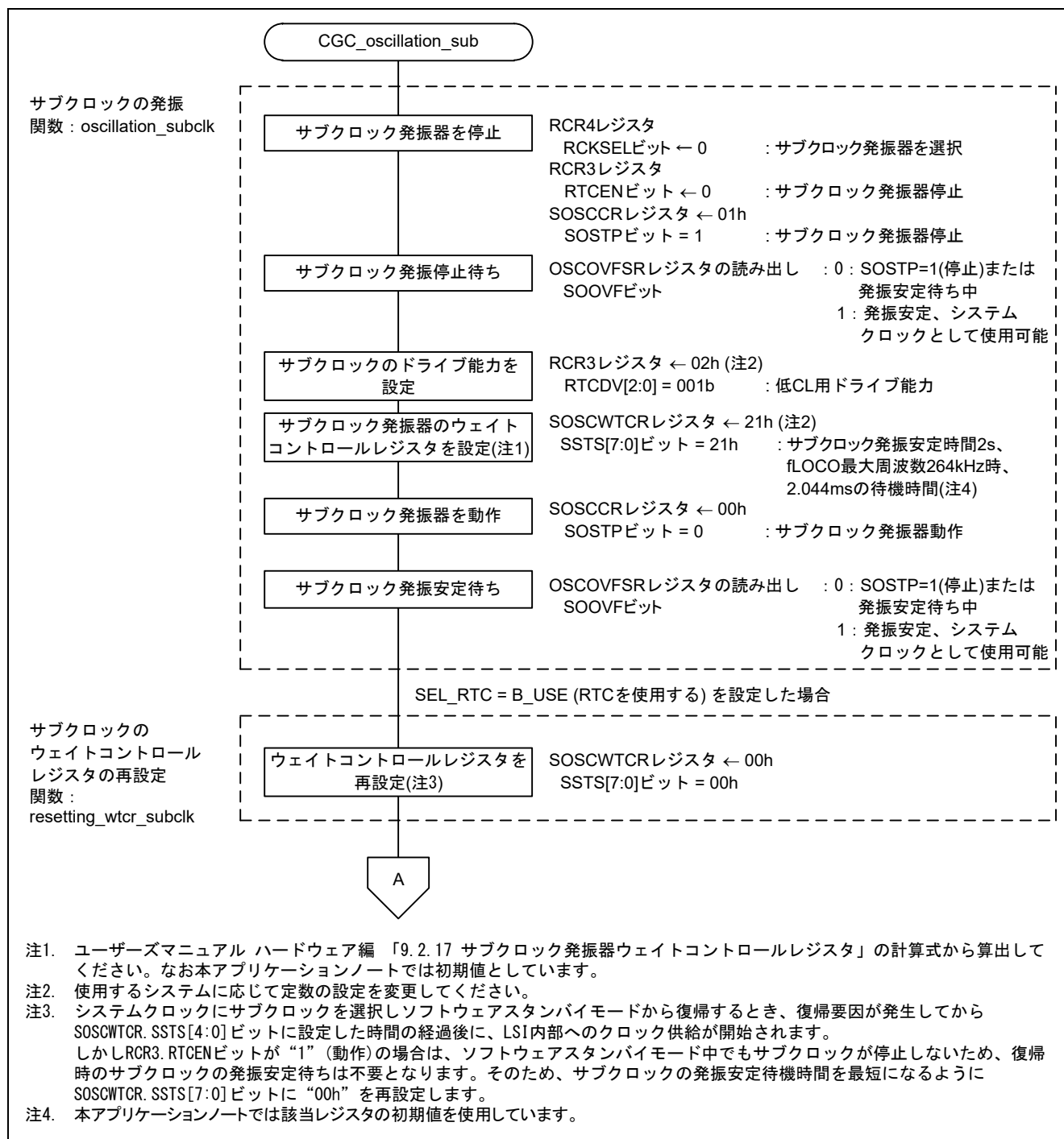
図 3.9 サブクロックの発振設定(1/2)
