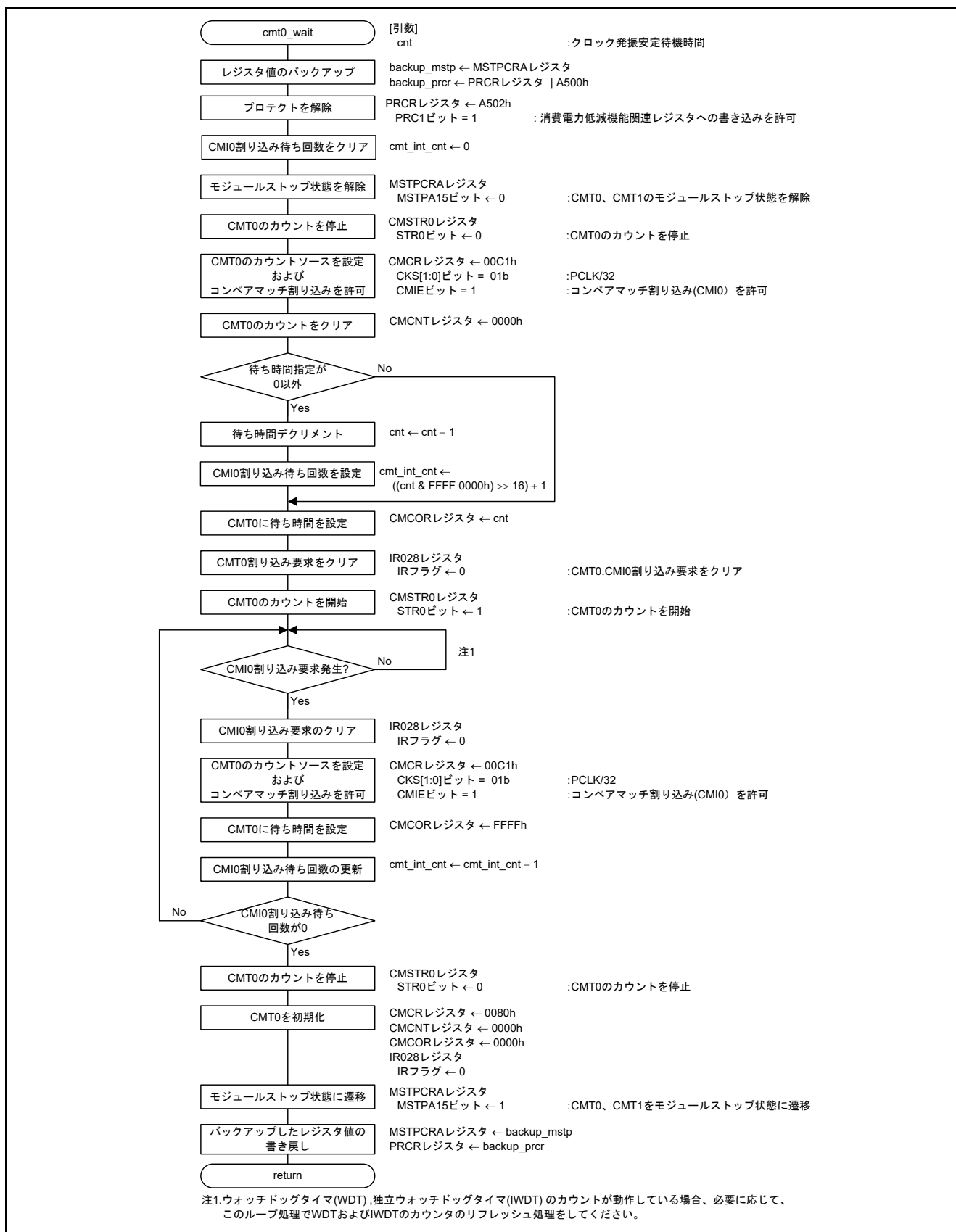
図 3.12 CMT0 によるソフトウェアウェイト
