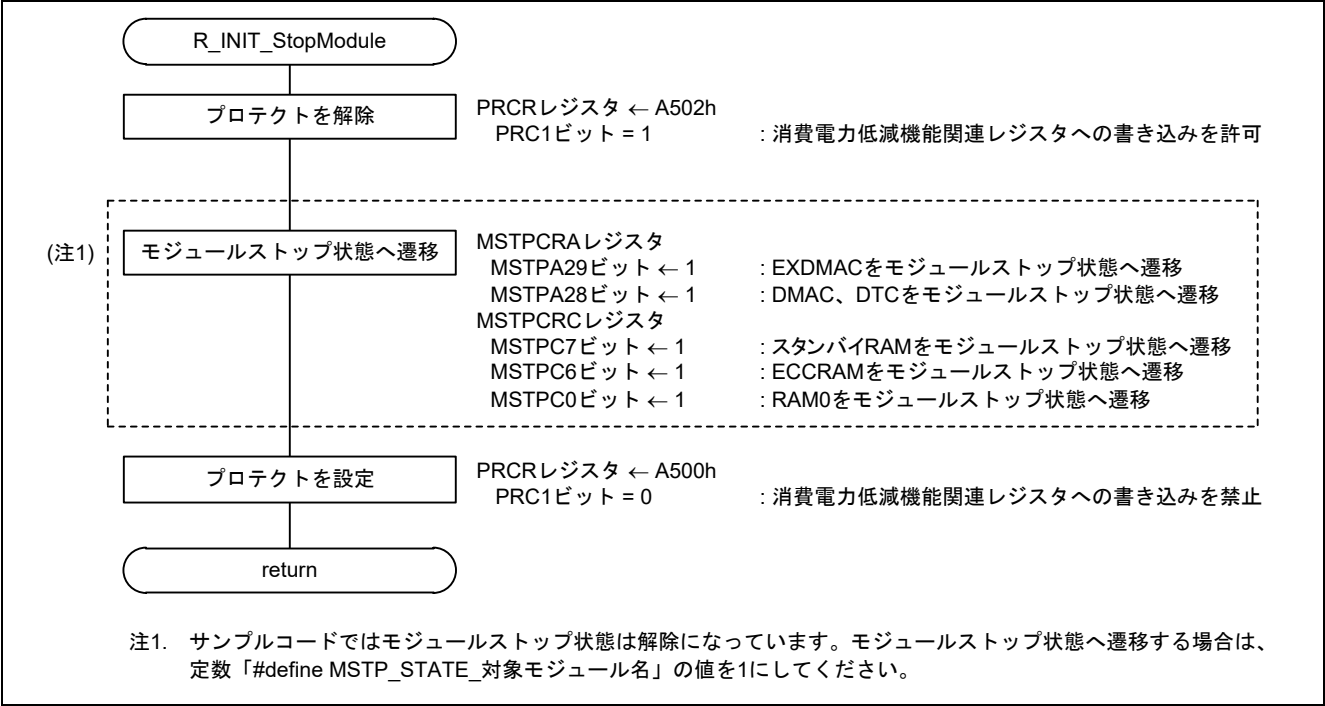
図 3.2 リセット後に動作している周辺機能の停止
