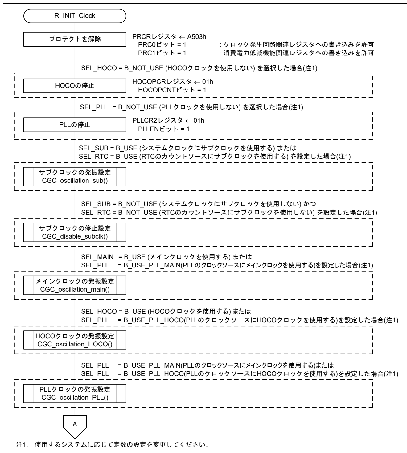
図 3.4 クロック初期設定(1/2)
