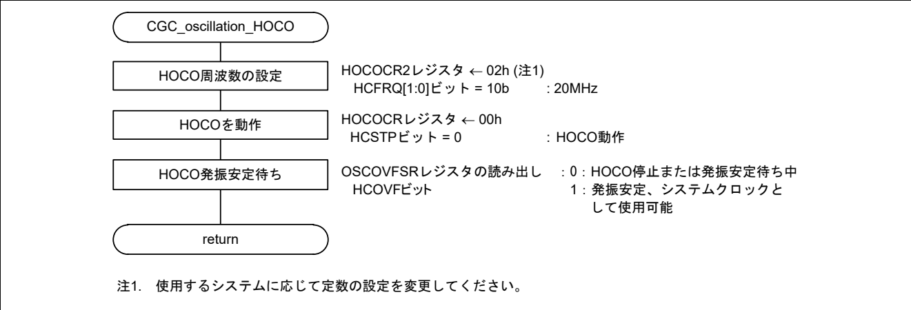
図 3.8 HOCO クロックの発振設定
