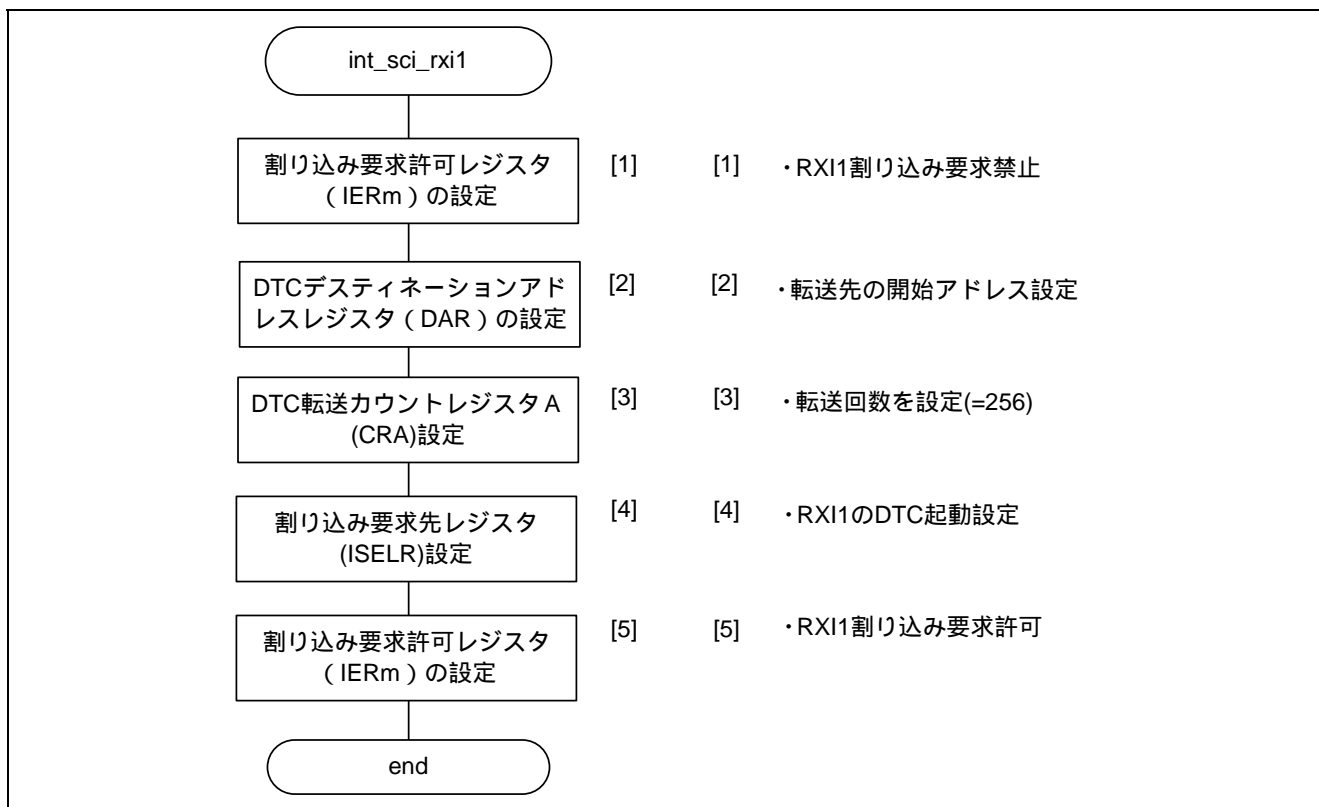
図 13 受信割り込み処理
