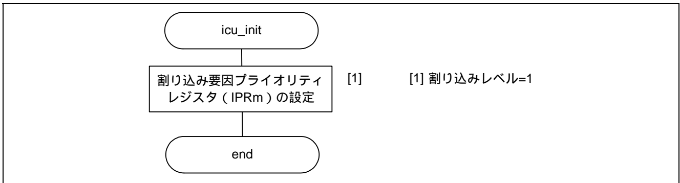
図 10 ICU 初期設定
