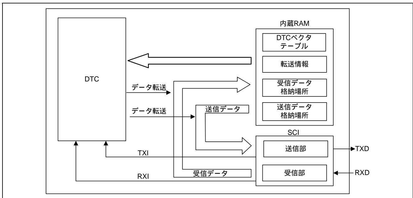
図 1 DTC を用いた調歩同期式シリアルデータ送受信の概要
