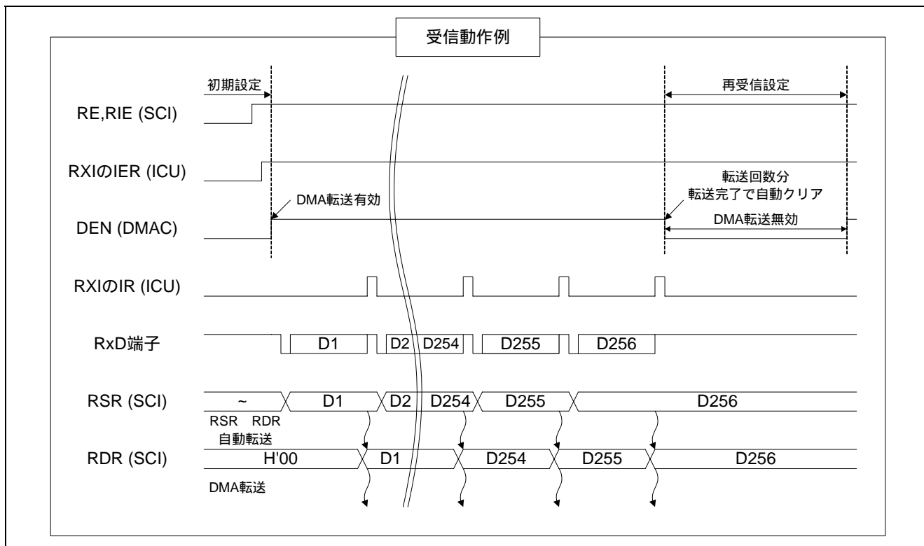
図 5 動作タイミング
