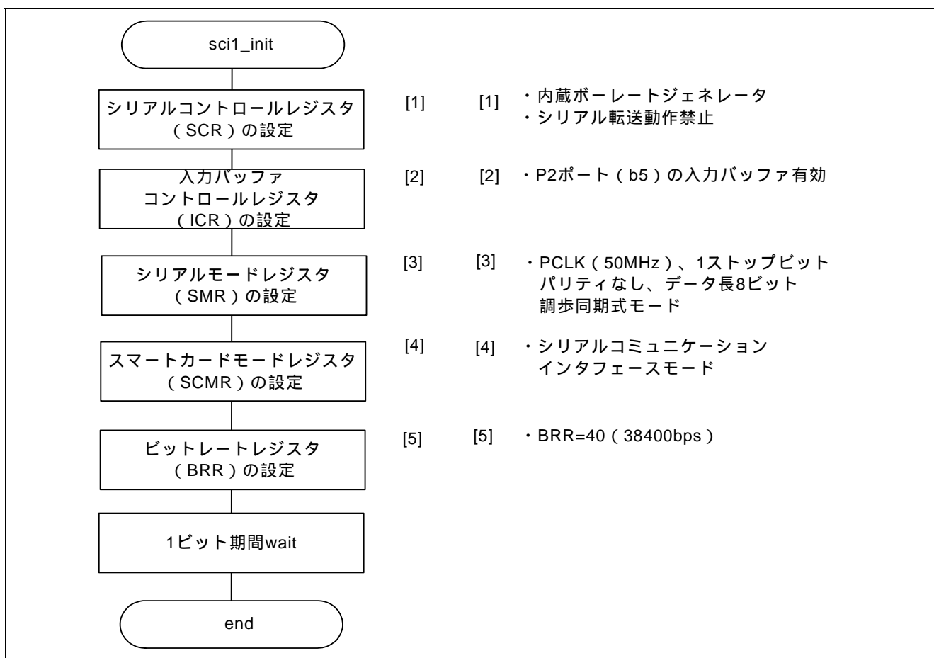
図 10 SCI 初期設定
