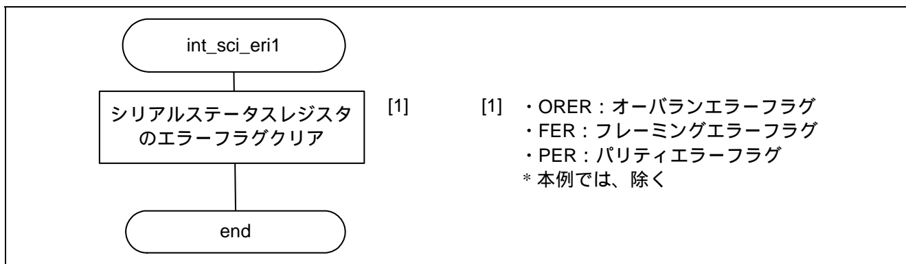
図 9 受信エラー割り込み
