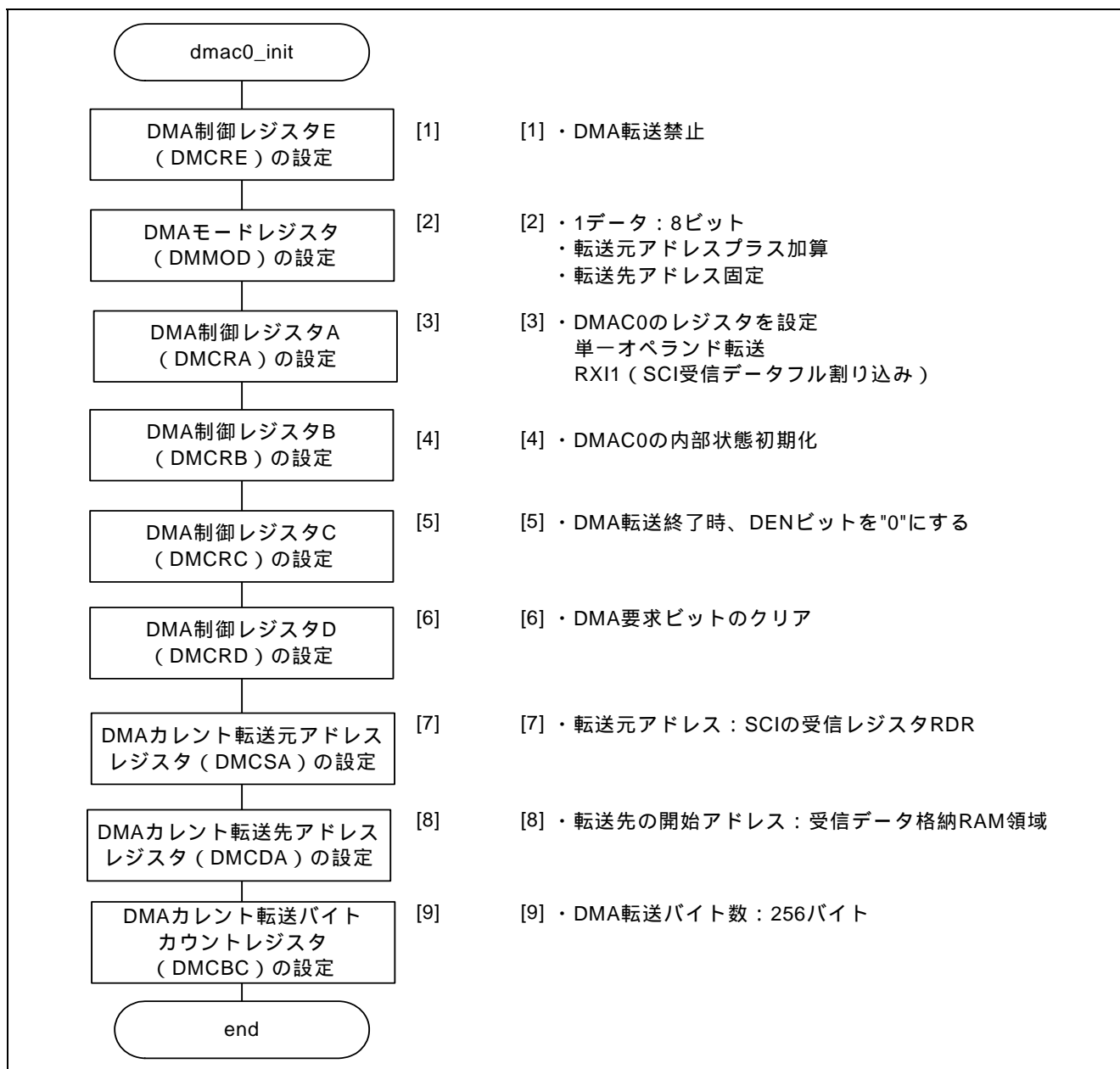
図 8 DMAC0 初期設定
