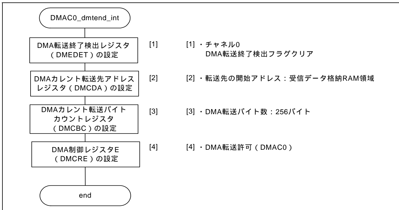
図 11 DMAC0 転送終了割り込み処理
