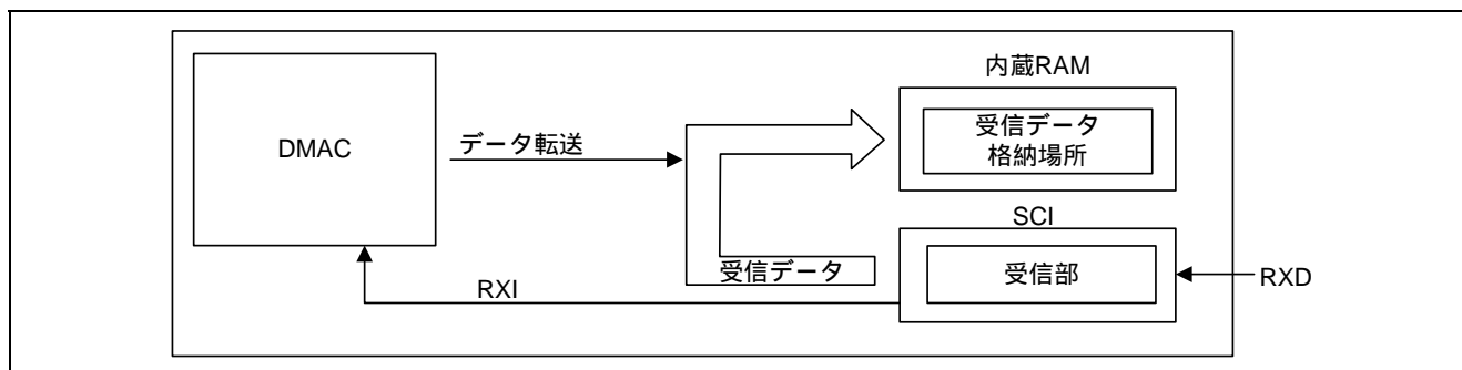
図 1 DMAC を用いた調歩同期式シリアルデータ受信の概要
