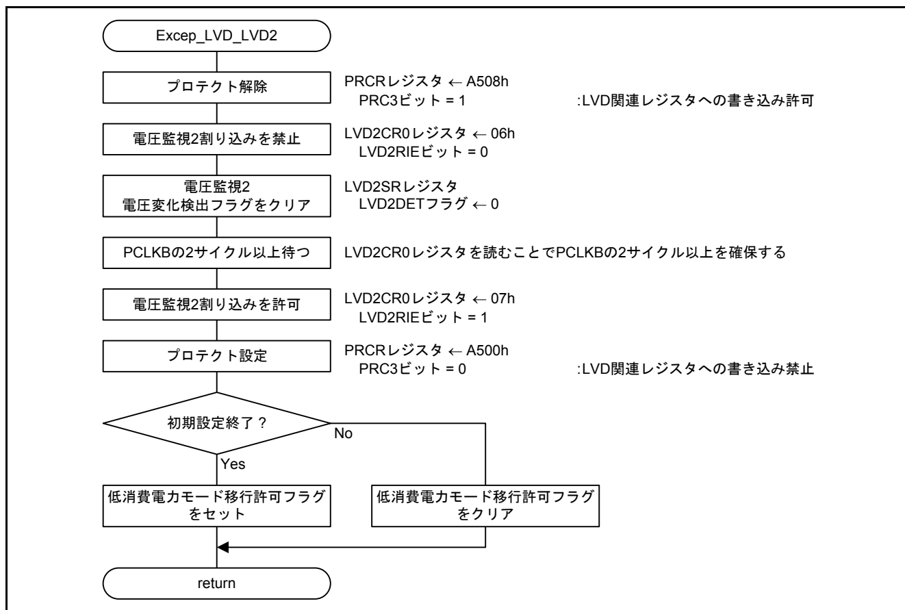
図5.17 LVD2 割り込み処理
