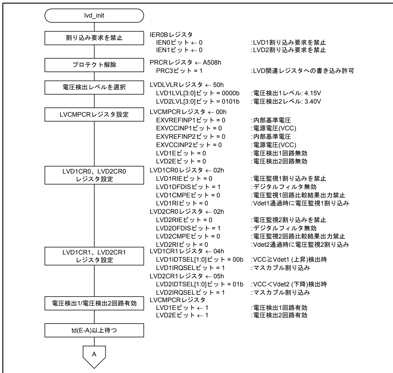
図5.12 LVD 初期設定(1/2)
