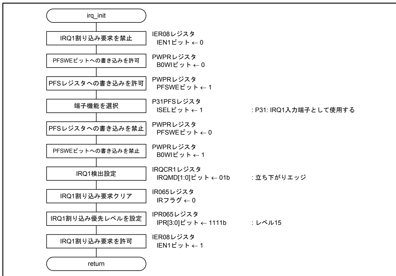
図5.11 IRQ 初期設定
