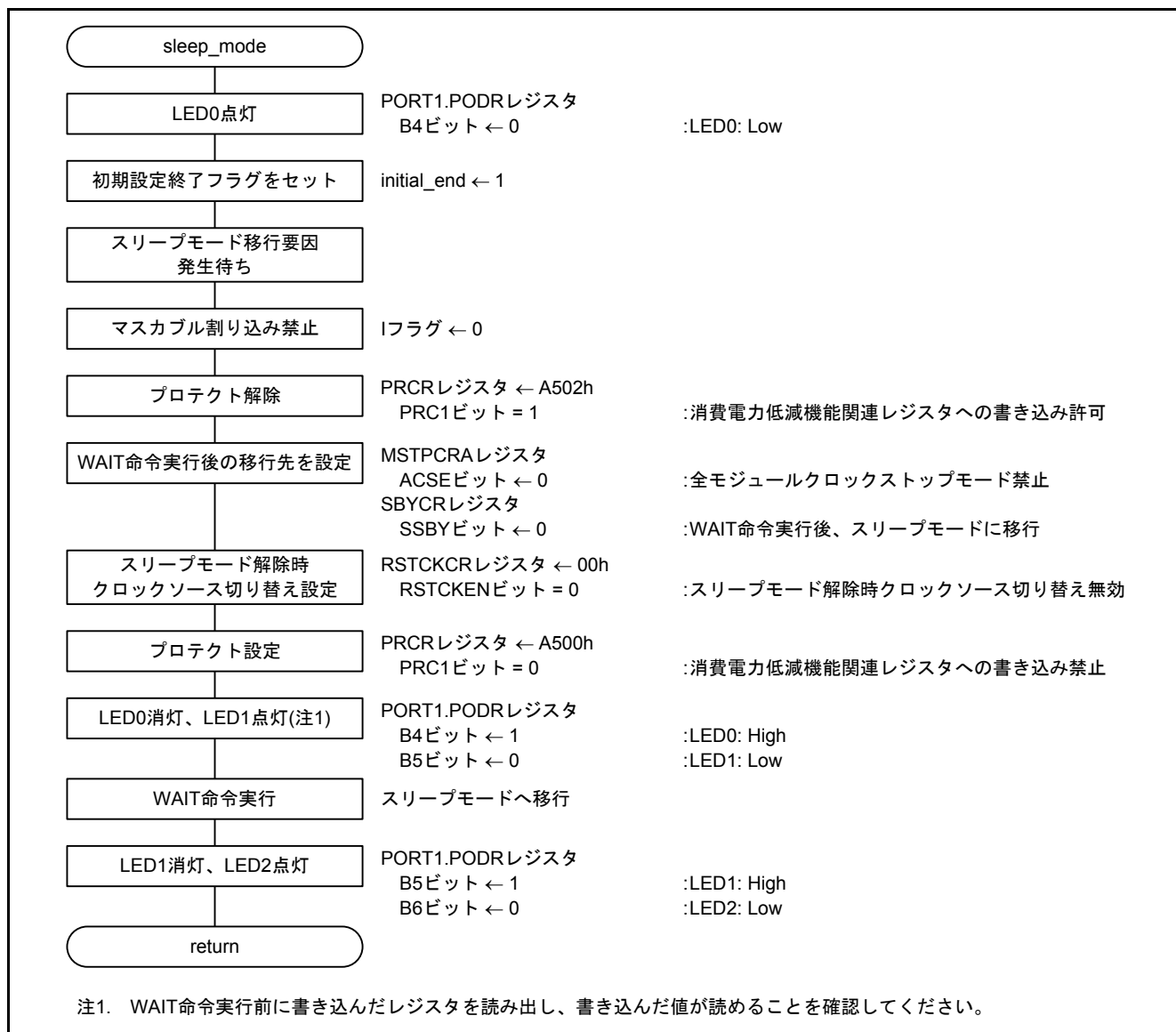
図5.9 スリープモード移行
