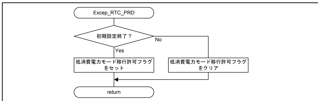
図5.18 RTC.PRD 割り込み処理
