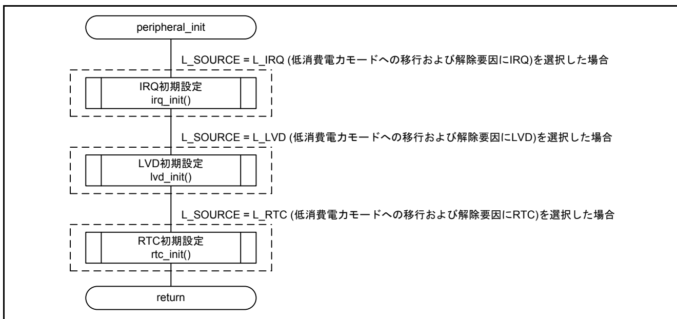
図5.8 周辺機能初期設定
