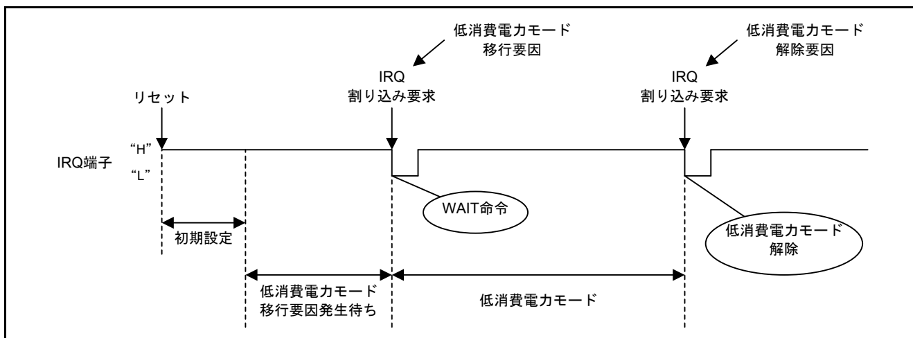
図5.3 IRQによる低消費電力モードへの移行と解除タイミング
