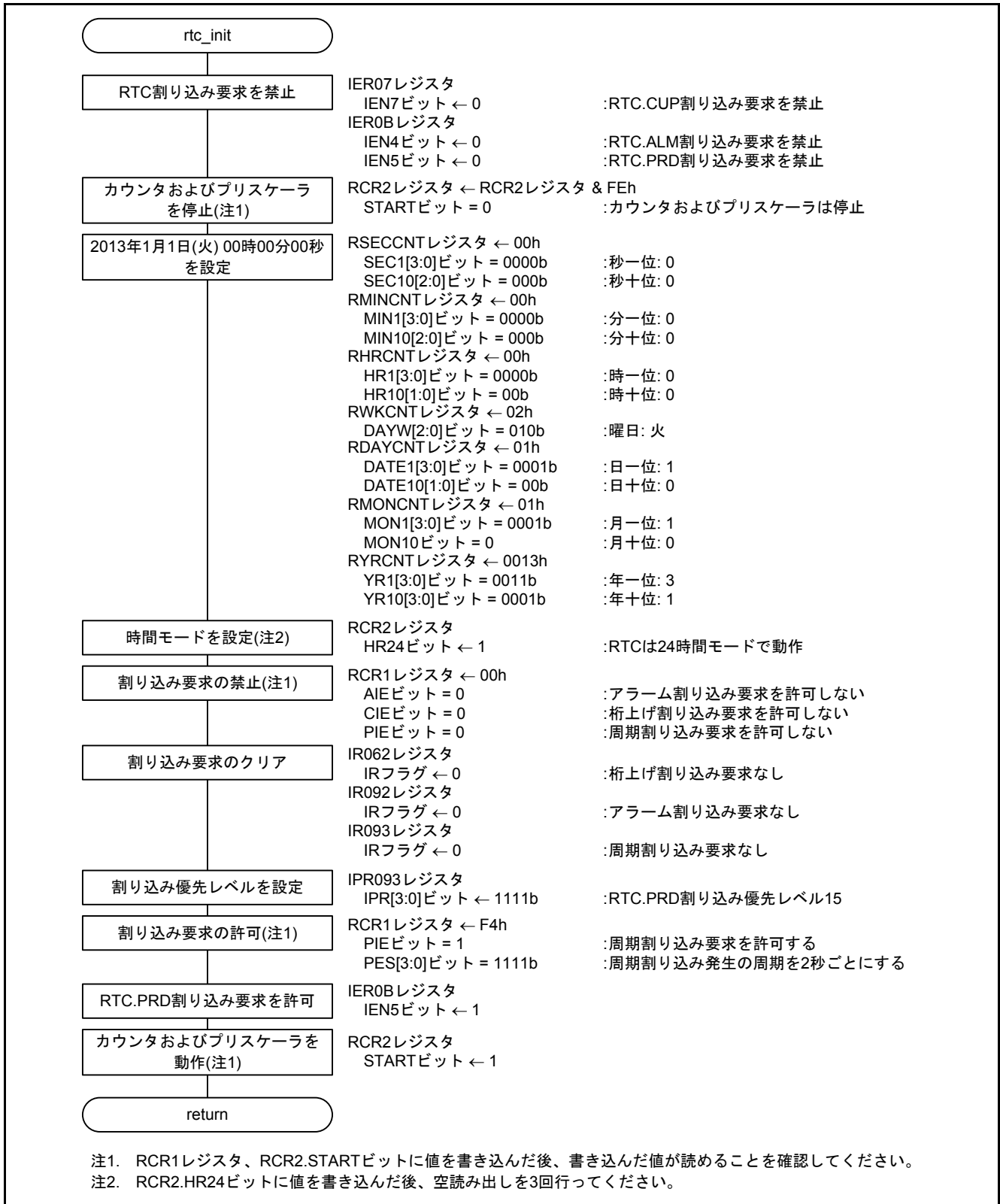
図5.14 RTC 初期設定
