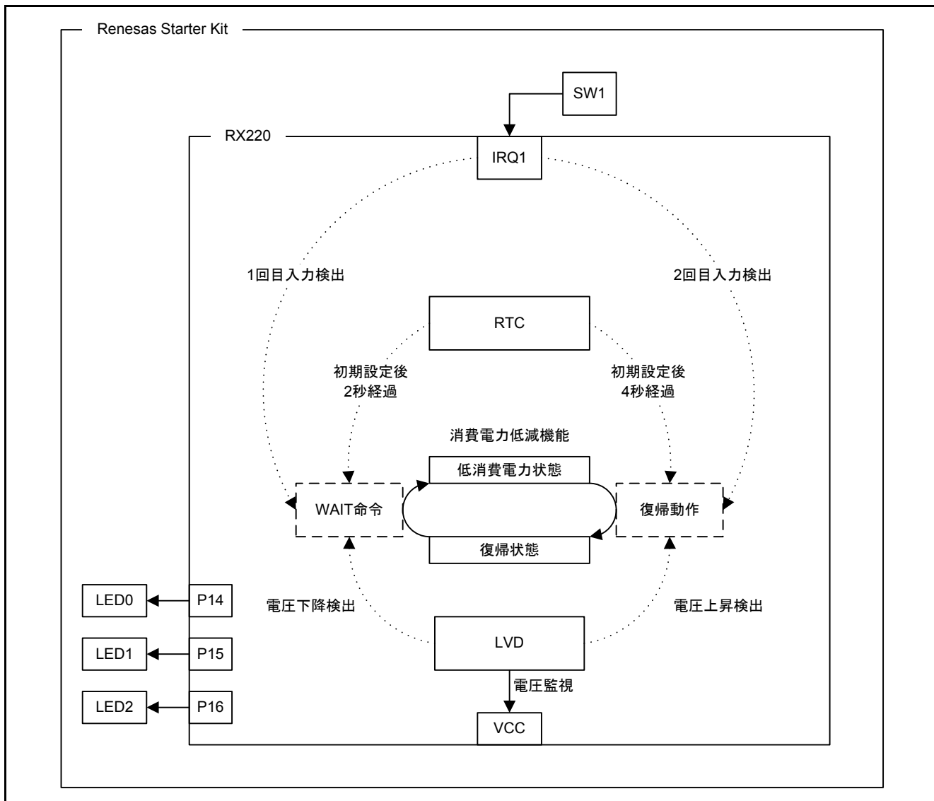
図1.1 ブロック図
