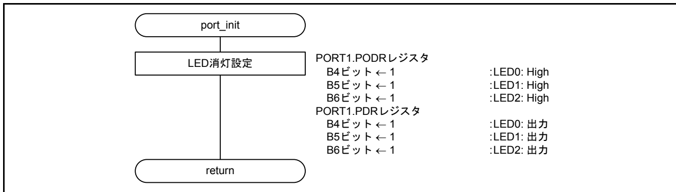
図5.7 ポート初期設定
