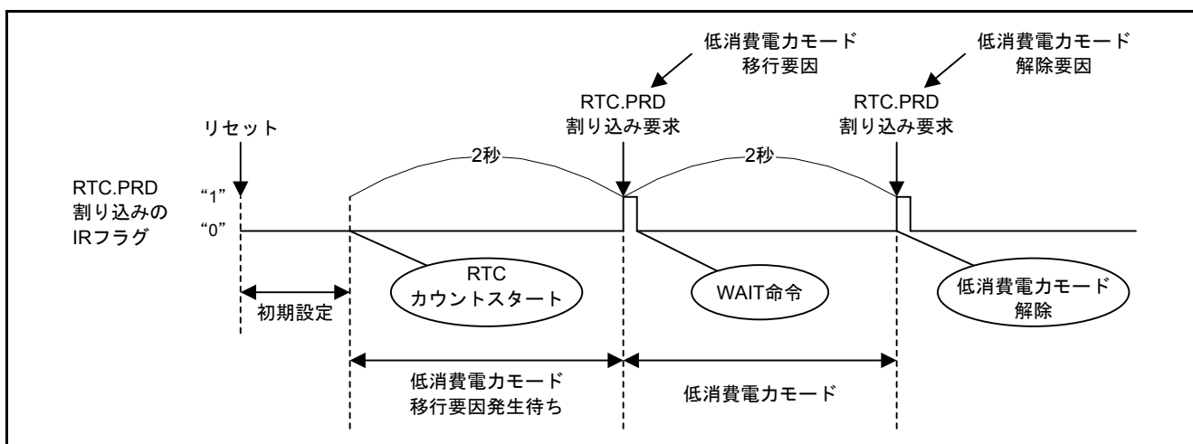
図5.4 RTCによる低消費電力モードへの移行と解除タイミング
