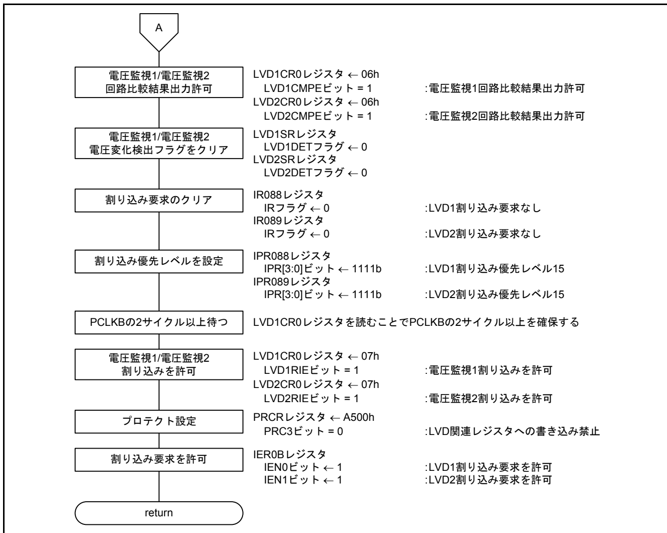
図5.13 LVD 初期設定(2/2)
