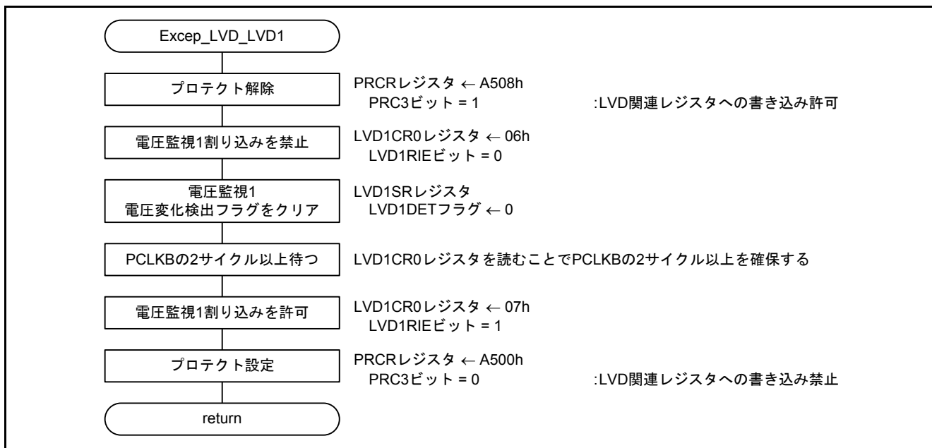
図5.16 LVD1 割り込み処理
