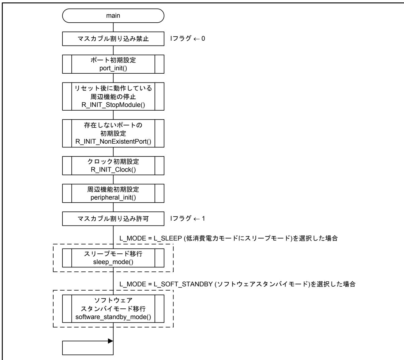
図5.6 メイン処理
