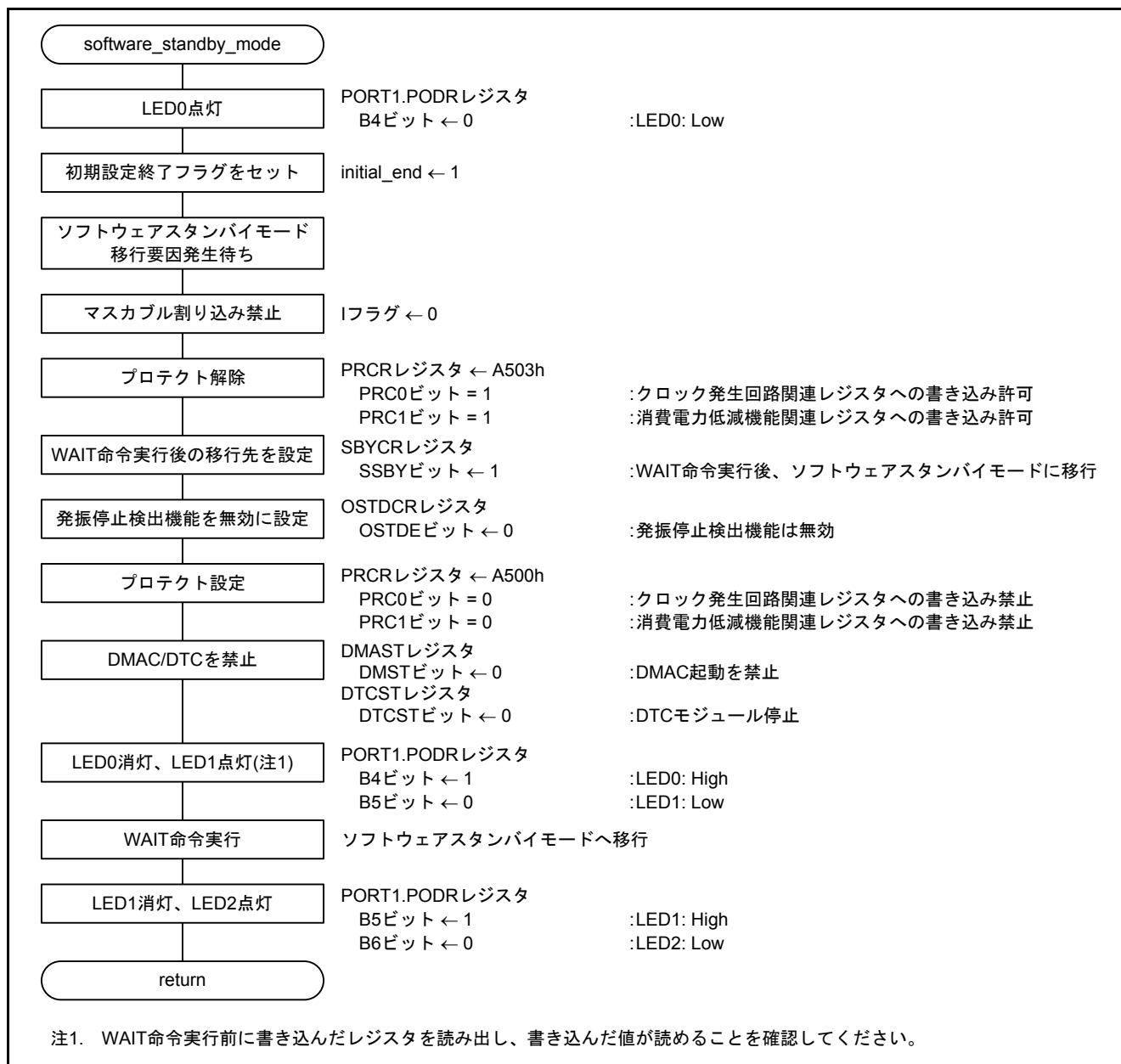
図5.10 ソフトウェアスタンバイモード移行
