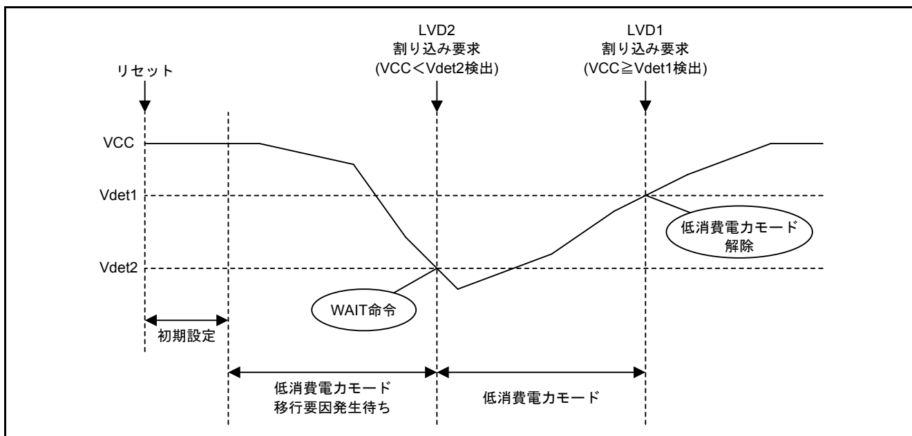
図5.5 LVDによる低消費電力モードへの移行と解除タイミング
