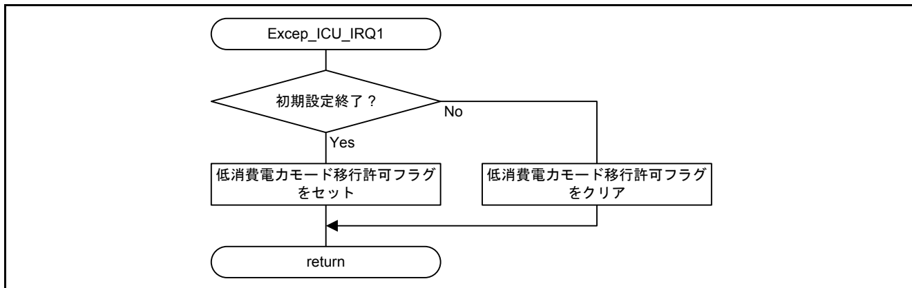
図5.15 IRQ1 割り込み処理
