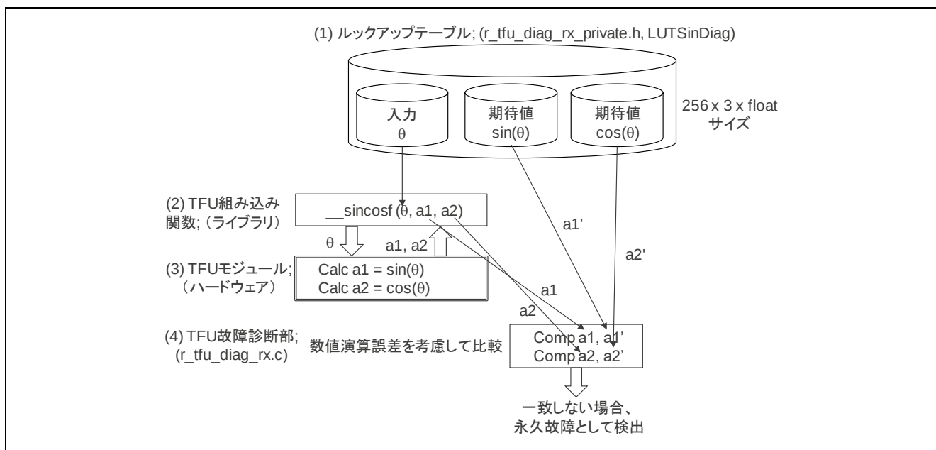
図 3.4 永久故障（正弦と余弦）
