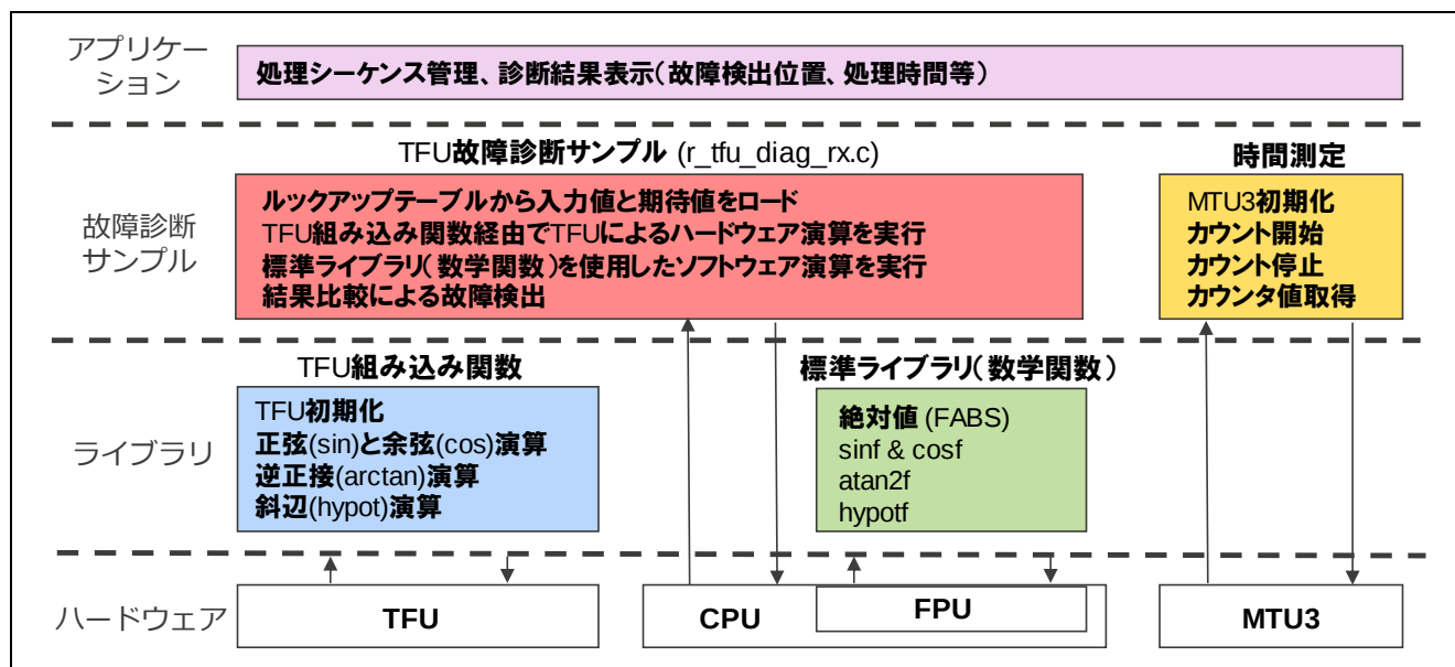
図 1.1 ソフトウェア構成
