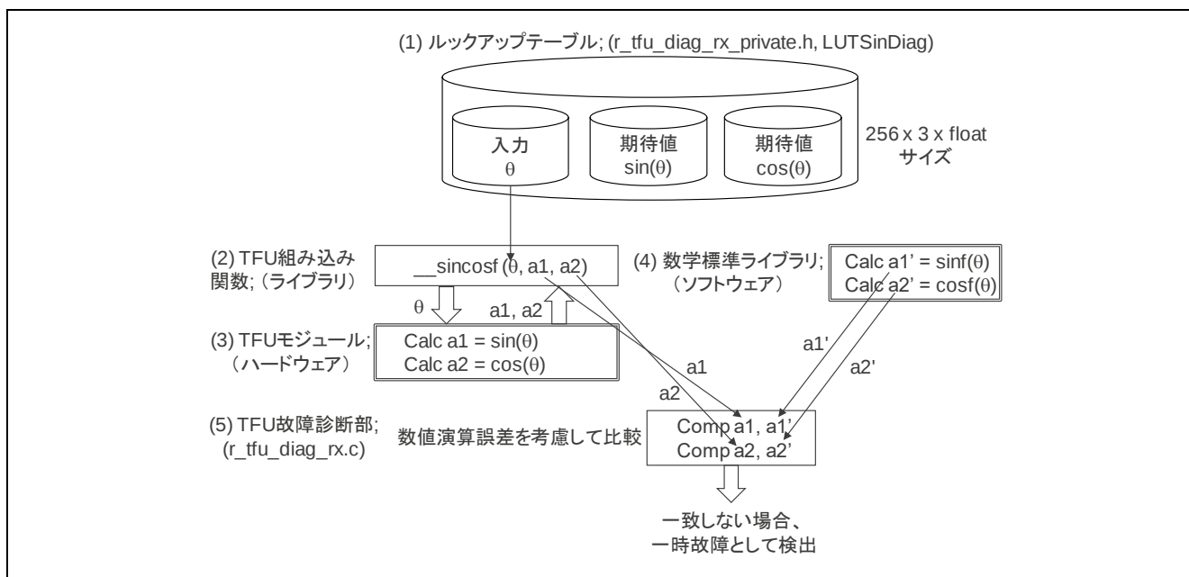
図 3.6 一時故障（正弦と余弦）
