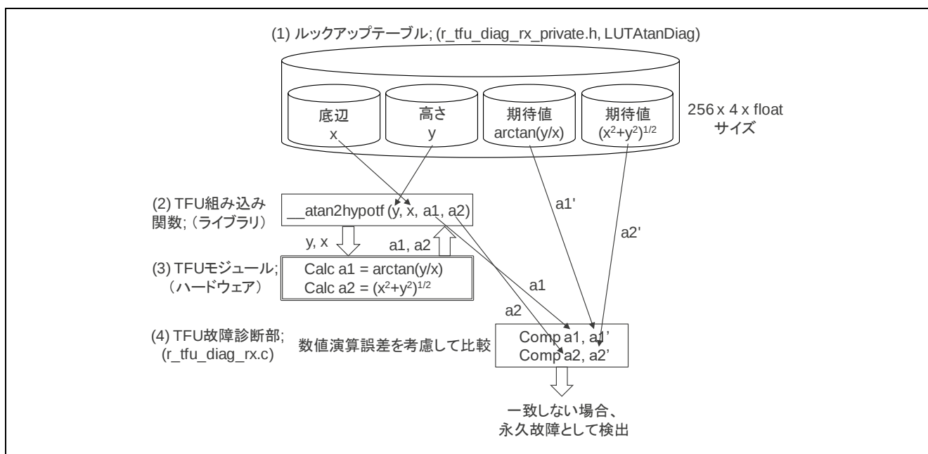
図 3.5 永久故障（逆正接と斜辺）
