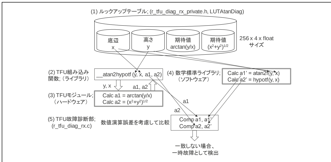
図 3.7 一時故障（逆正接と斜辺）
