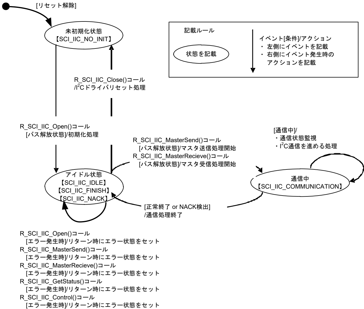
図 1.10 状態遷移図
