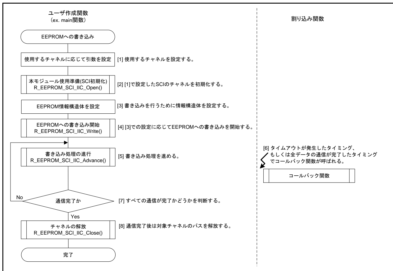
図 1.3 EEPROM への書き込み手順例
