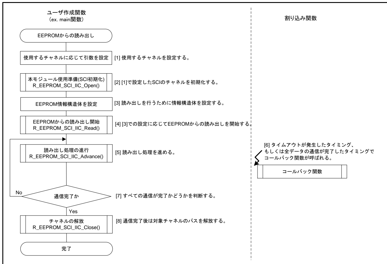
図 1.4 EEPROM からの読み出し手順例
