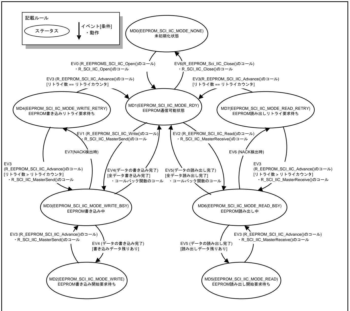
図 1.5 EEPROM アクセス (簡易 I 2 C) FIT モジュールの状態遷移図
