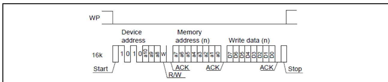
図 1.2 デバイスアドレスにメモリアドレスを含む一例
