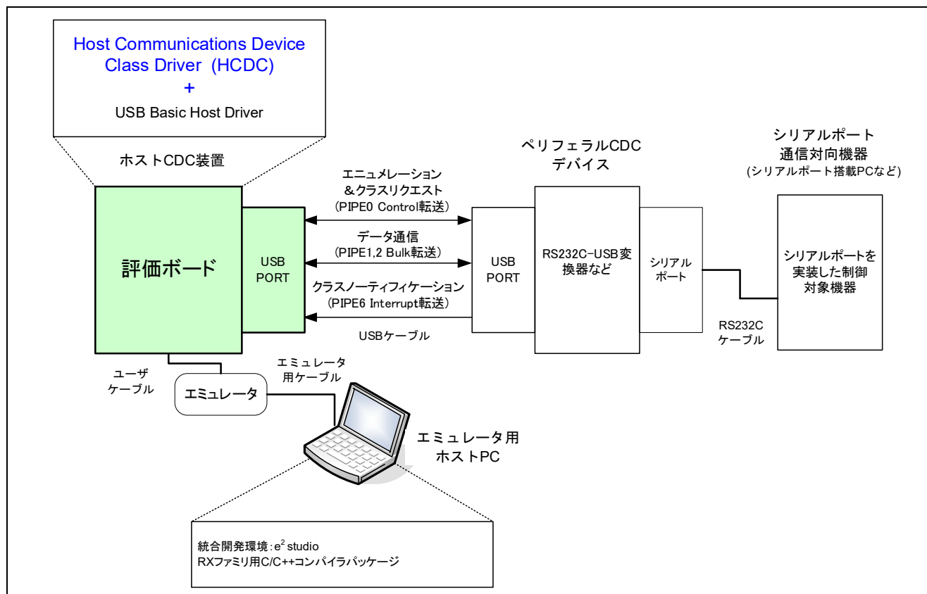
Figure 3-1 動作環境例
