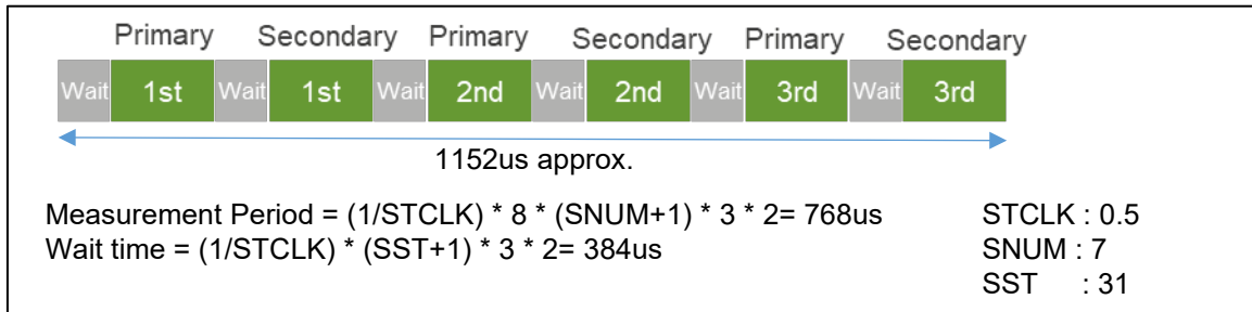
図 7 相互容量計測時間(CTSU2L)
