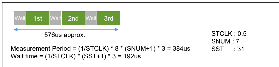
図 6 自己容量計測時間(CTS2L)
