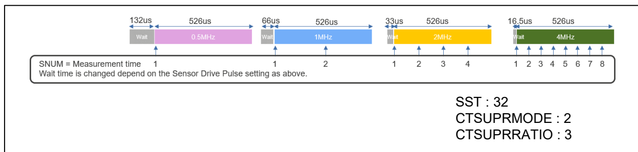
図 5 自己容量計測時間(CTS1)
