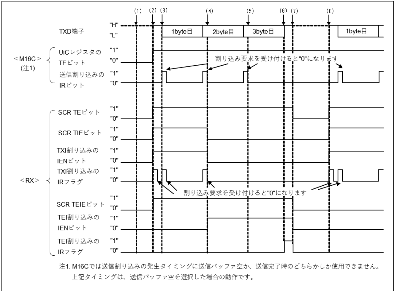
図 3.1 RX と M16C のタイミング相違点(3 バイトずつ送信する場合)
