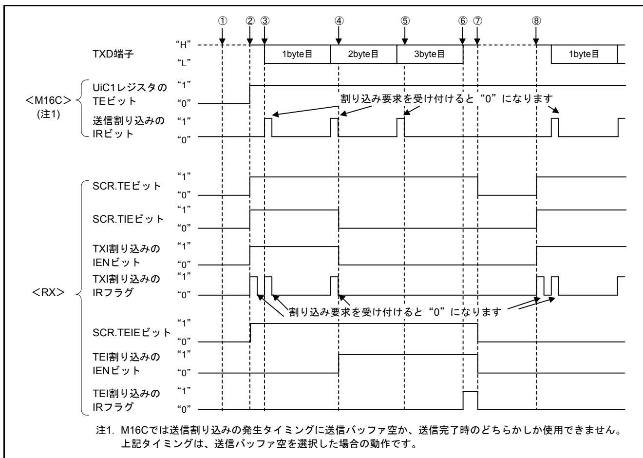
図3.1 RX と M16C のタイミング相違点(3 バイトずつ送信する場合)
