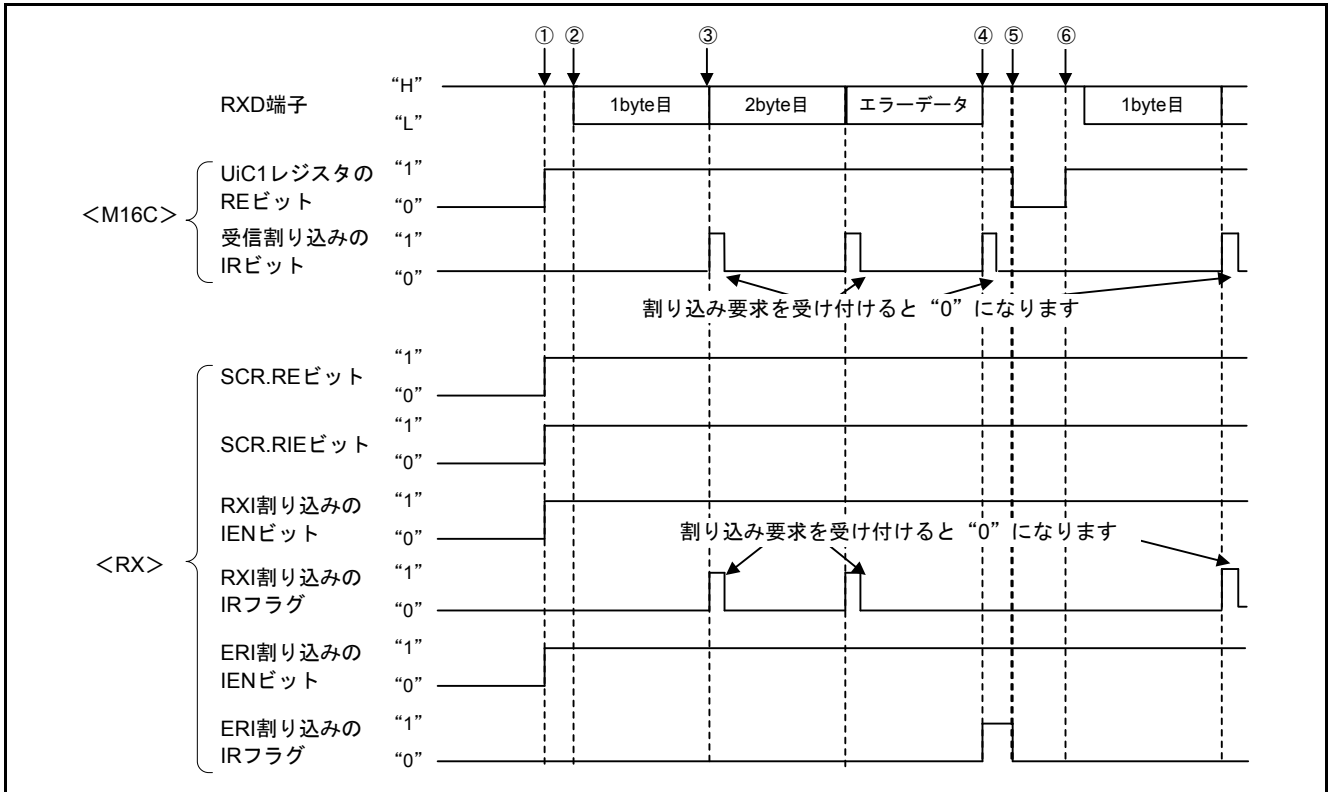
図3.2 RX と M16C のタイミング相違点(受信時)
