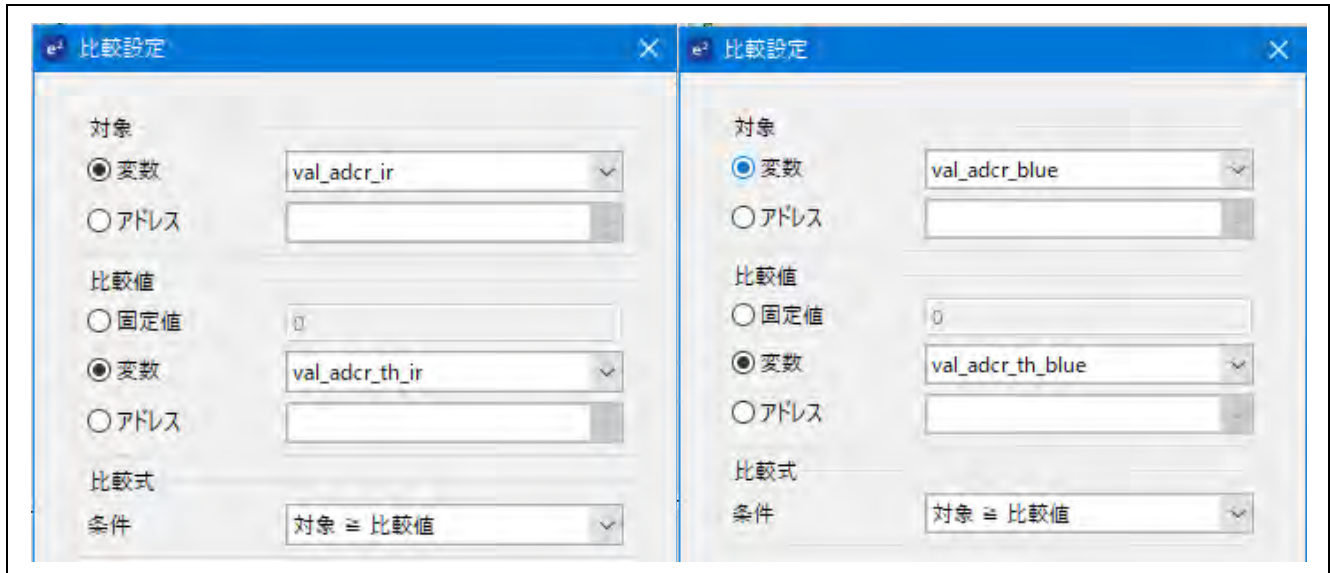
図 6-13 比較設定
