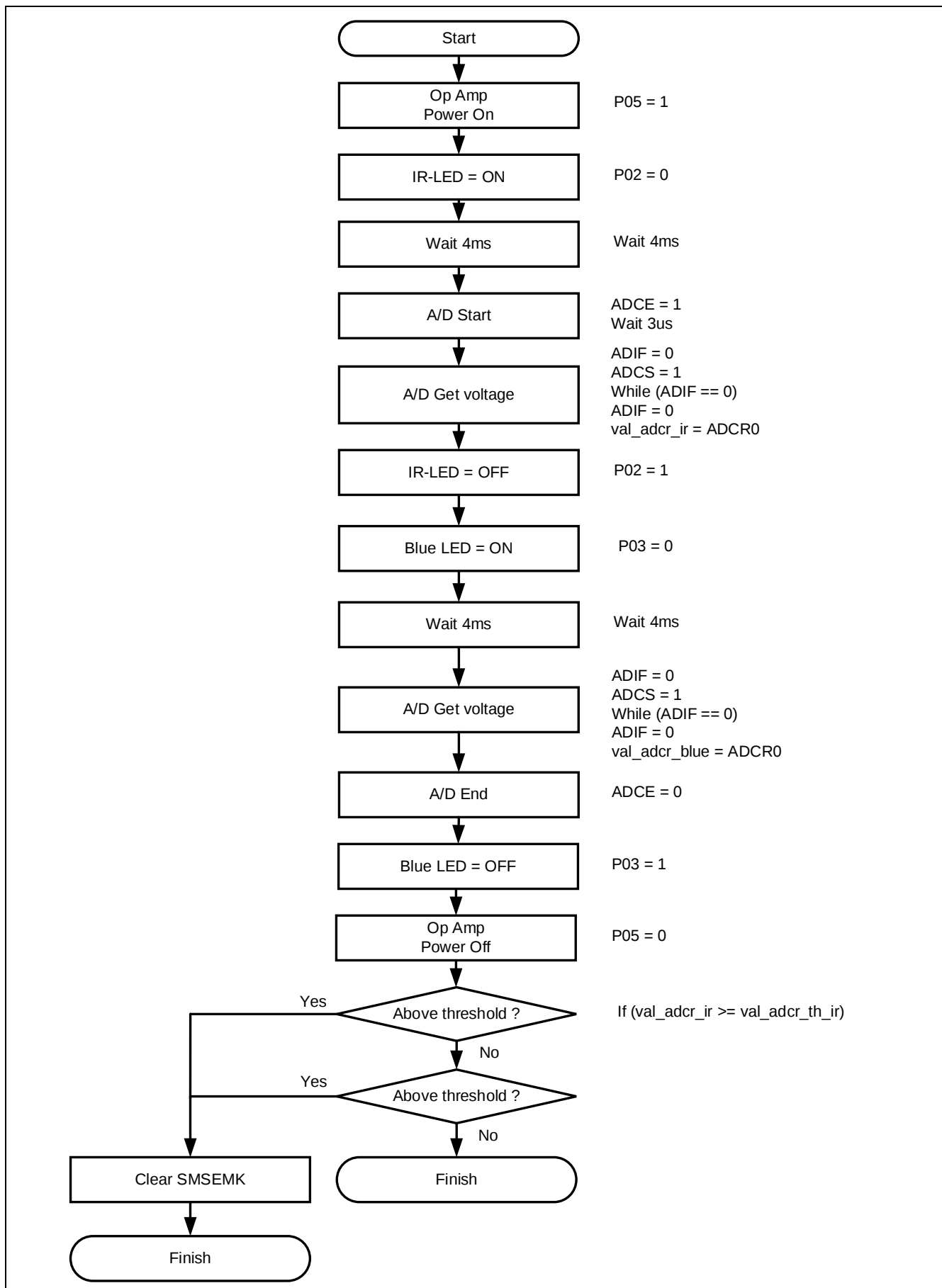
図 5-2 SMS 処理
