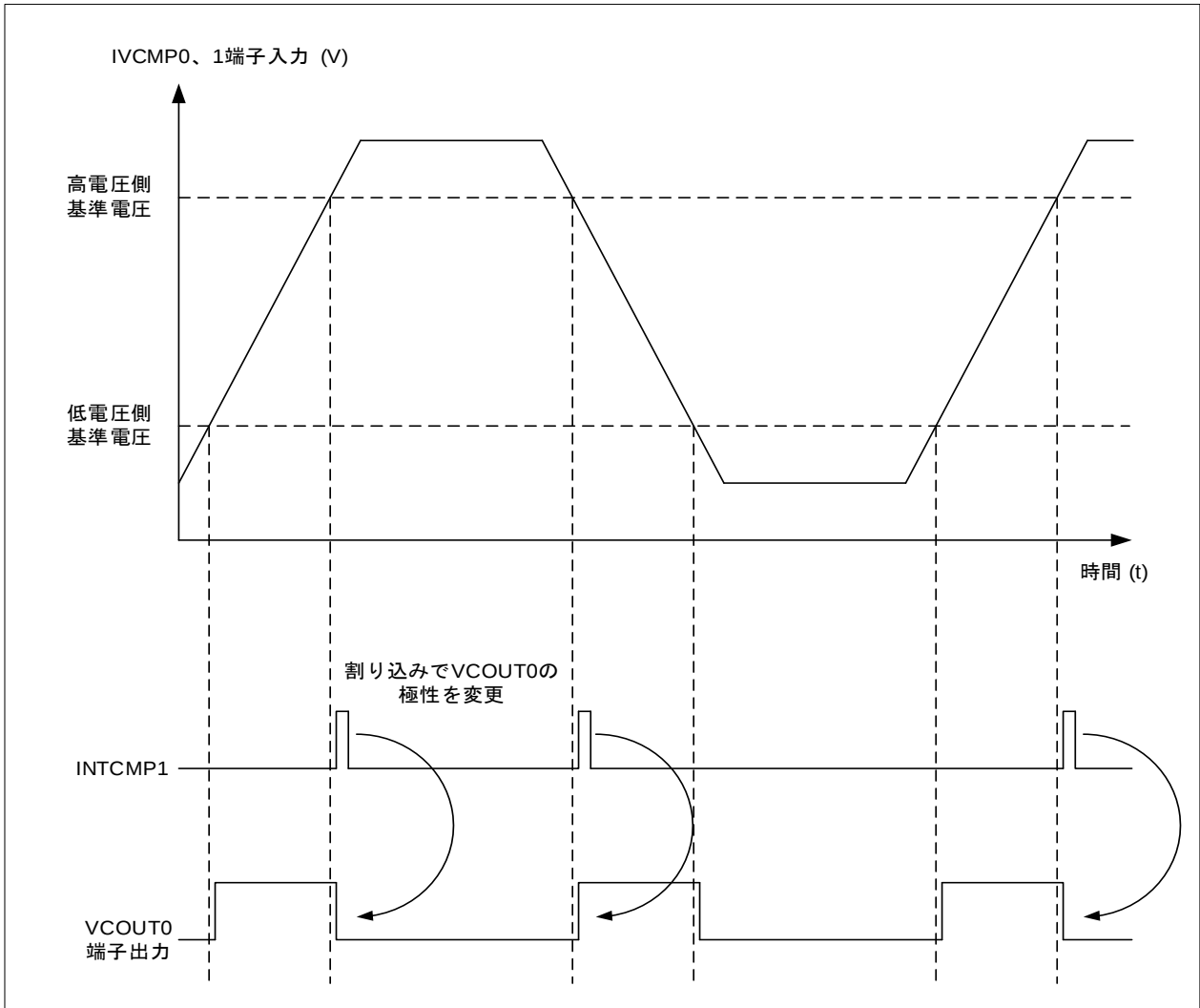
図 1-1 ウィンドウ・コンパレータの動作概要
