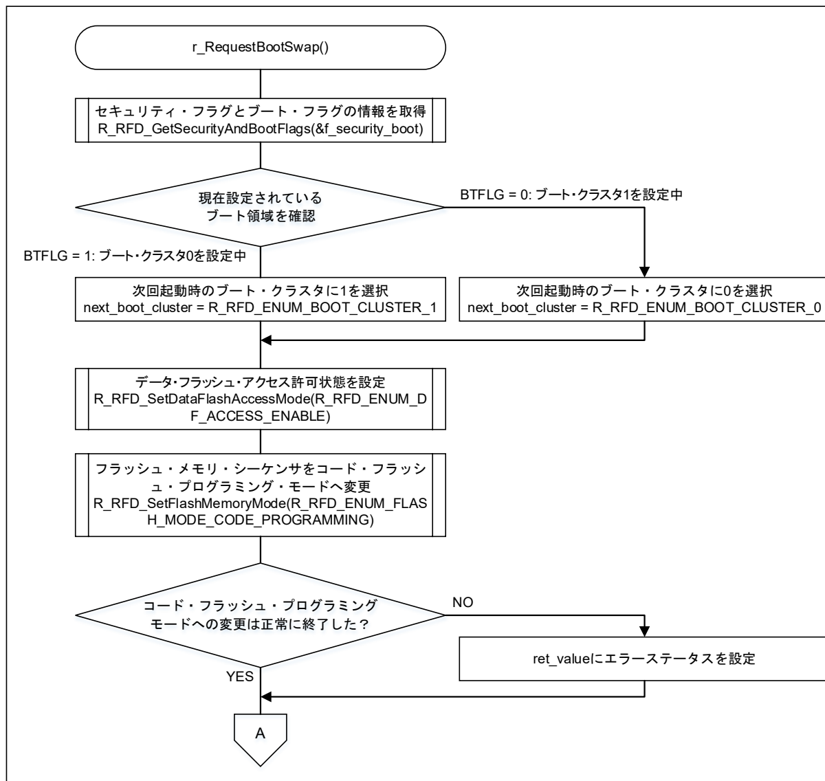
図 4-16 ブート・スワップ処理 (1/2)
