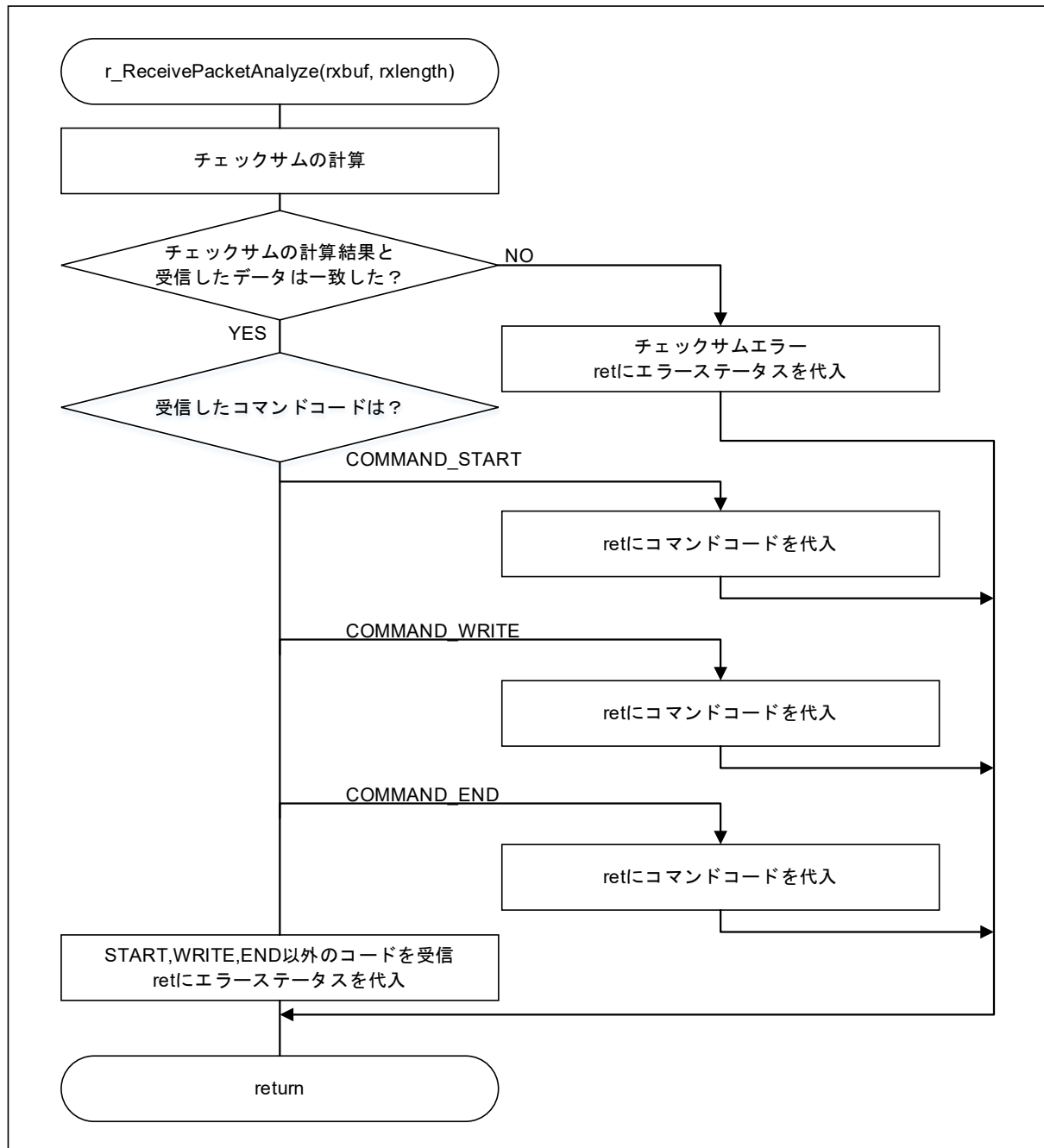
図 4-21 UART0 コマンド解析
