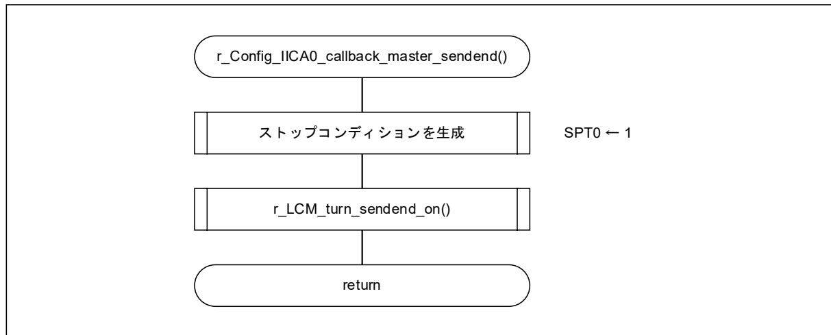
図 4-25 IICA0 送信完了割込み時の処理
