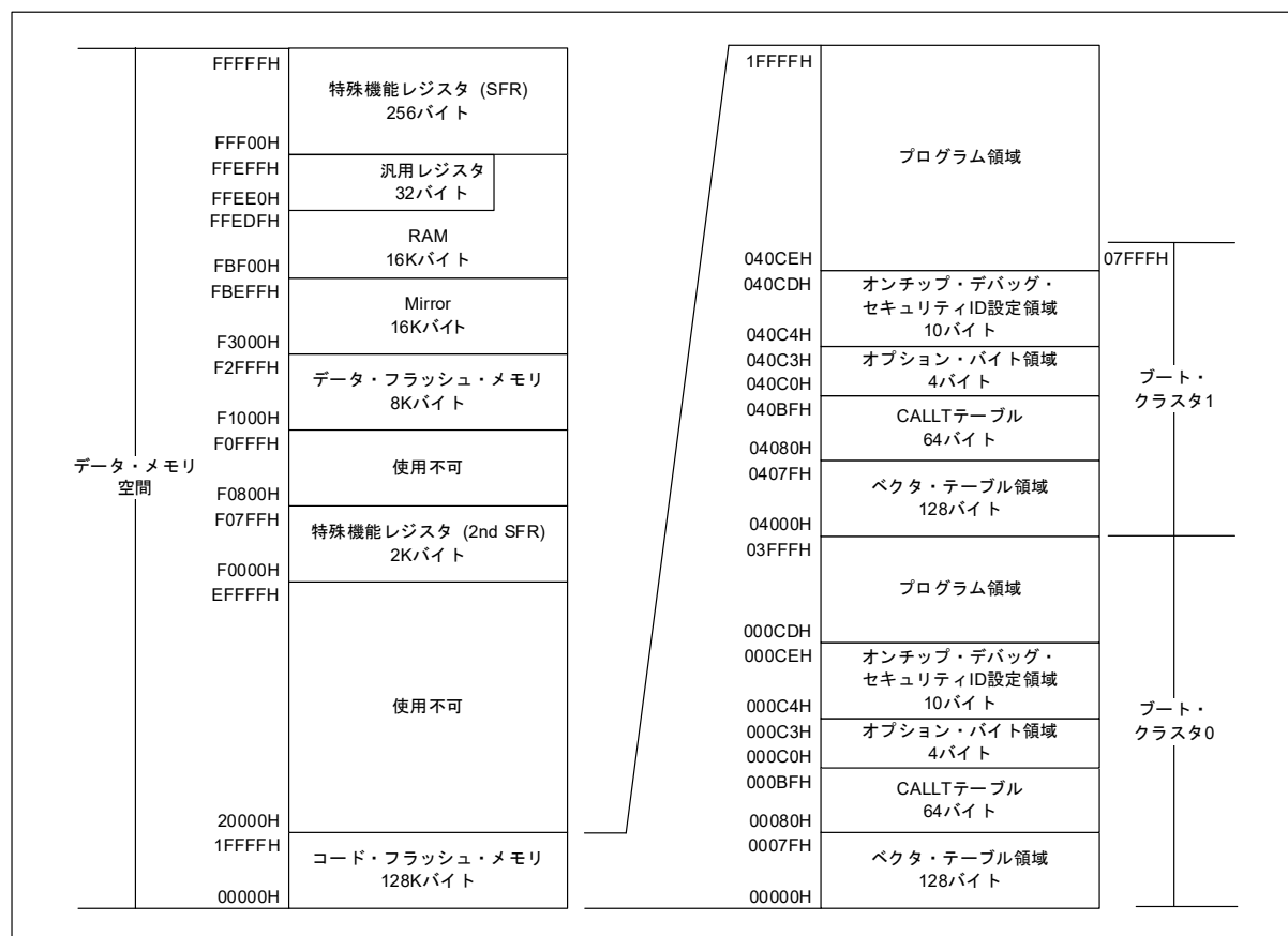
図 1-1 メモリ構成
