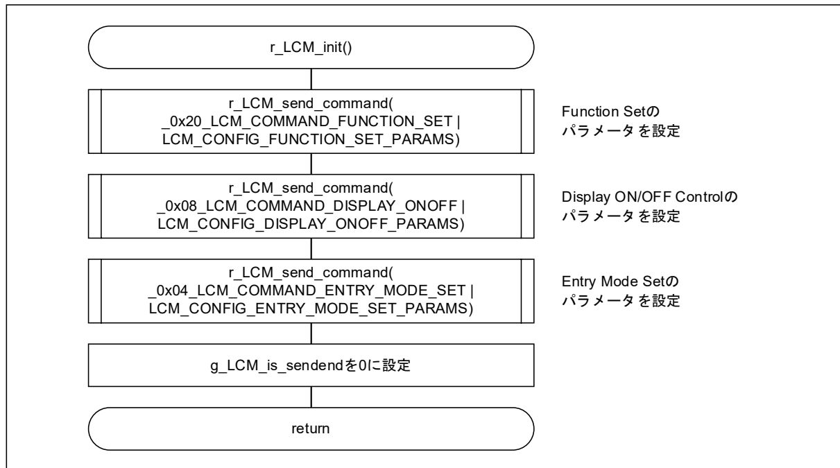
図 4-27 LCD モジュール初期化
