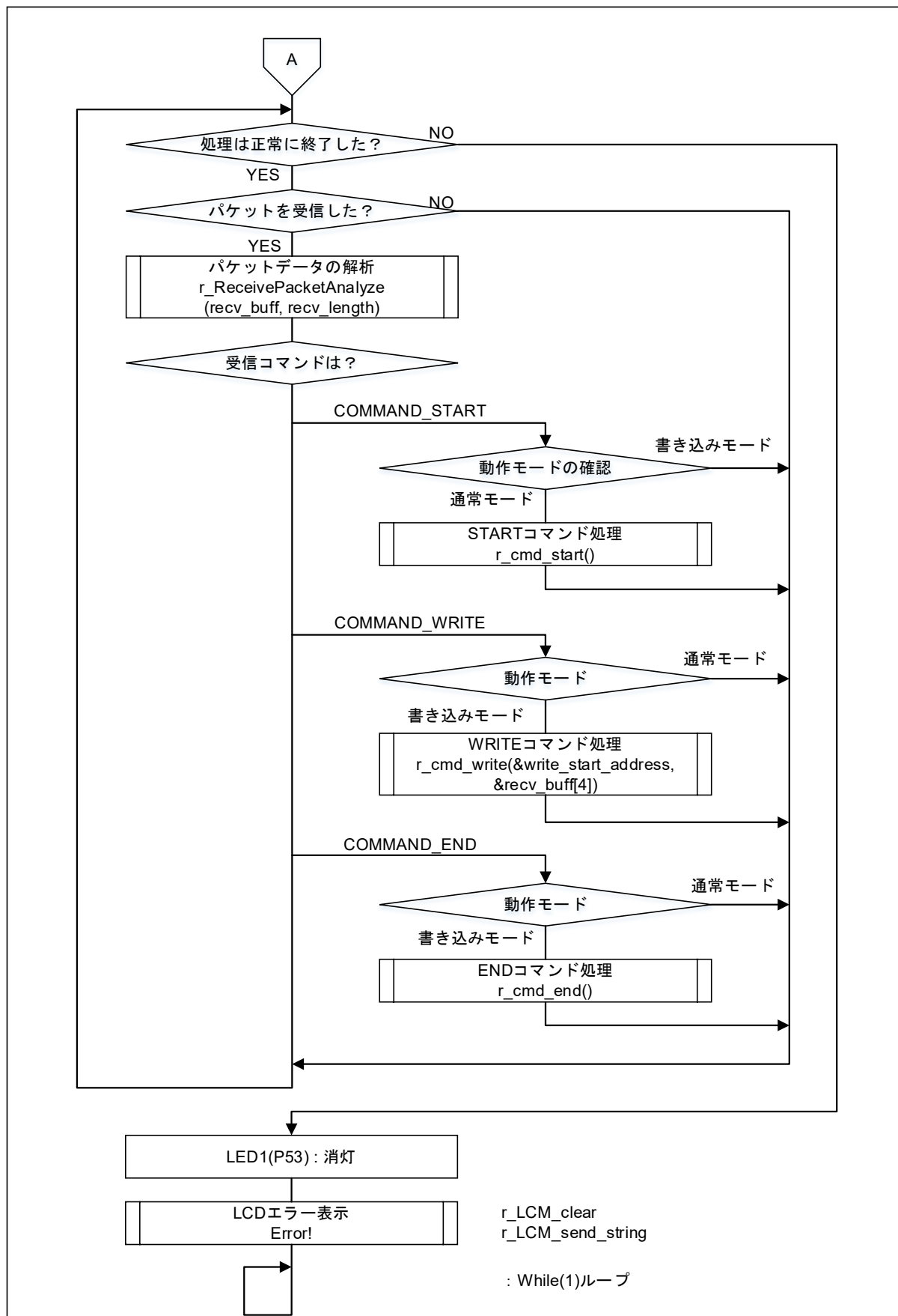
図 4-2 メイン処理 (2/2)
