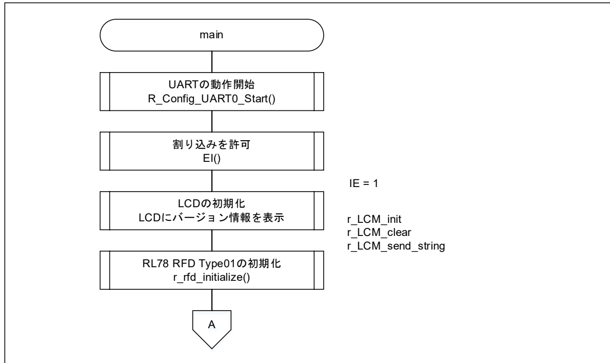
図 4-1 メイン処理 (1/2)
