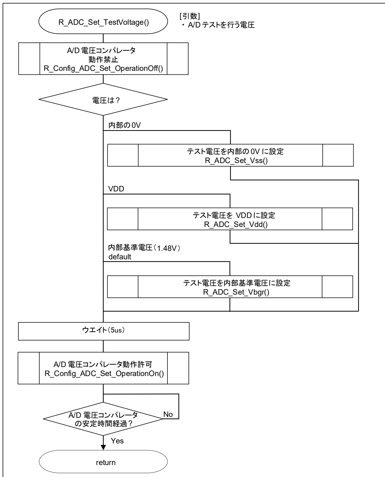
図 4 - 3 テスト電圧設定
