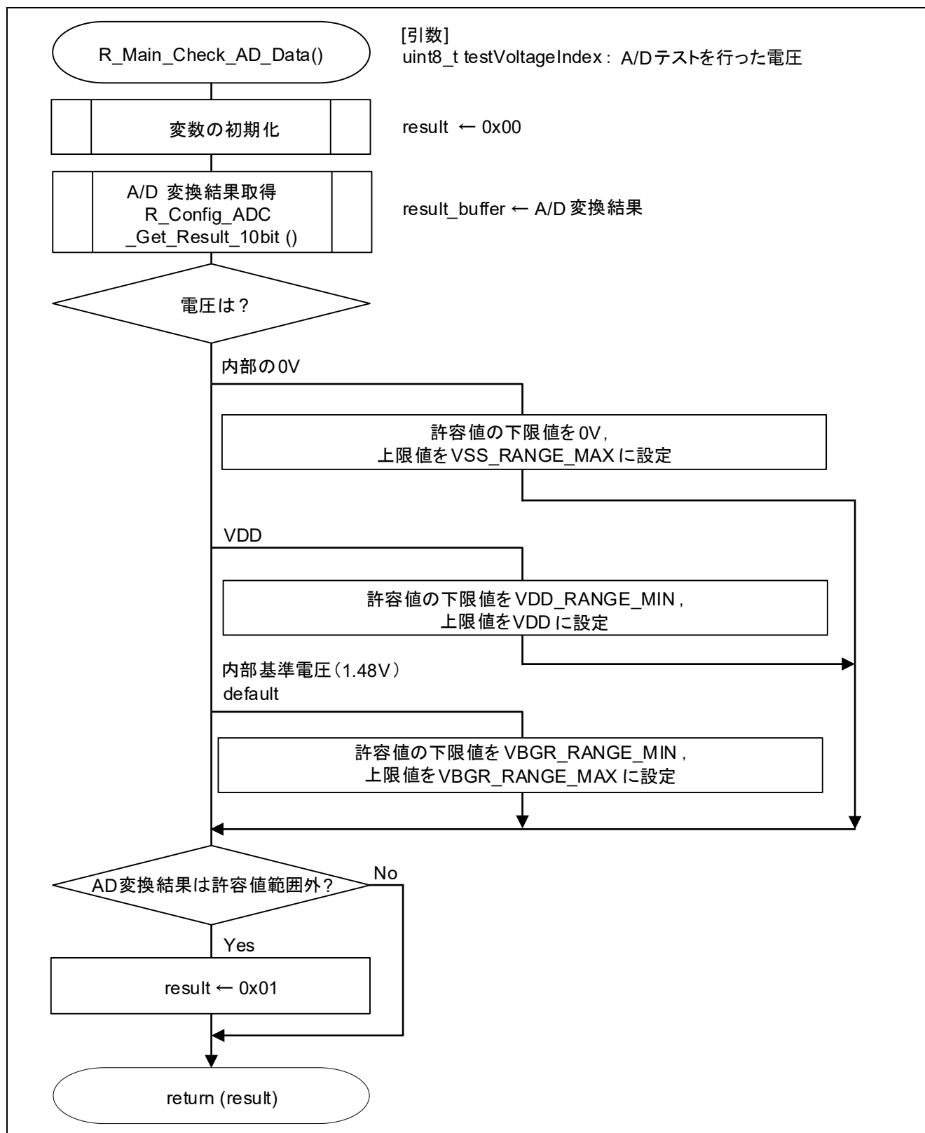
図 4 - 7 A/D 変換結果確認
