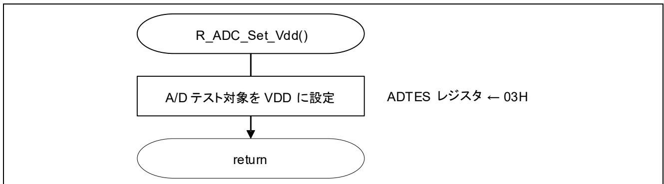
図 4 - 5 テスト電圧を VDD に設定
