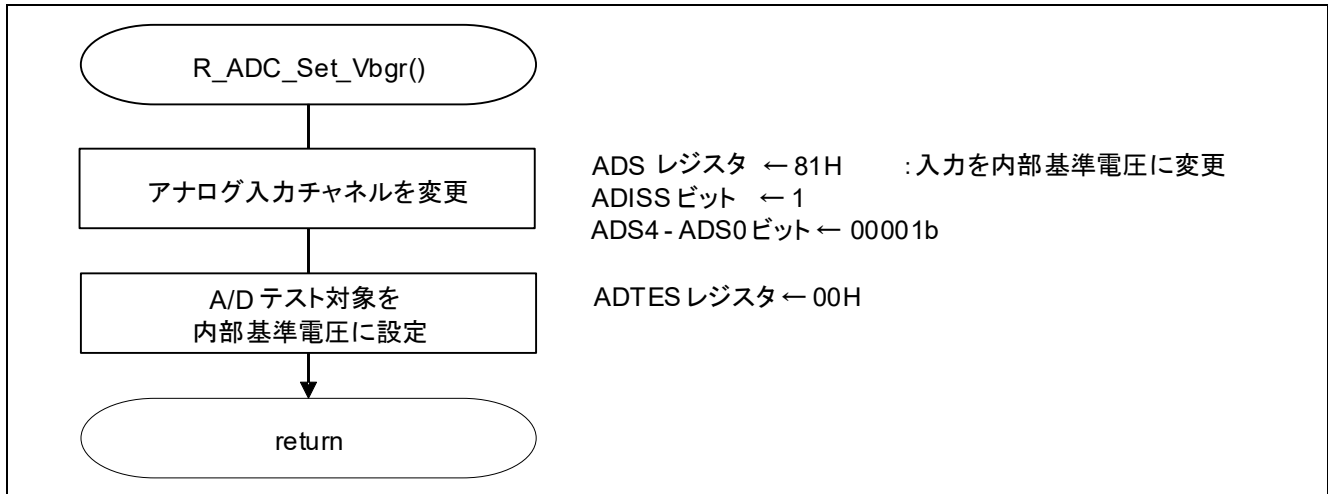
図 4 - 6 テスト電圧を内部基準電圧に設定
