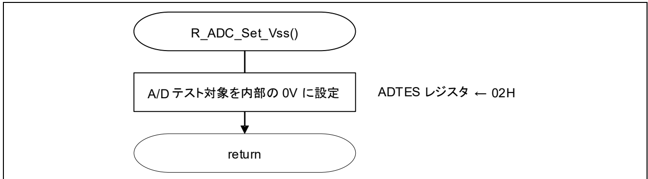
図 4 - 4 テスト電圧を内部の 0V に設定
